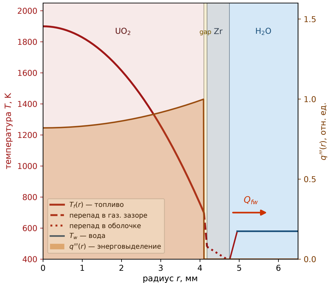
(б) Радиальные профили температуры и энерговыделения
