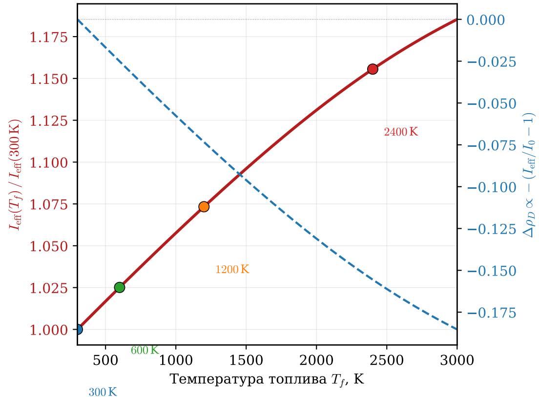
(б) Резонансный интеграл и доплеровский вклад
