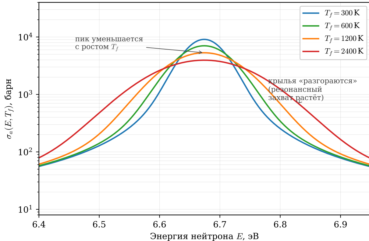
(а) Доплеровское уширение резонанса ^{238}\text{U} ( E_0 = 6,674 \text{ эВ} )
