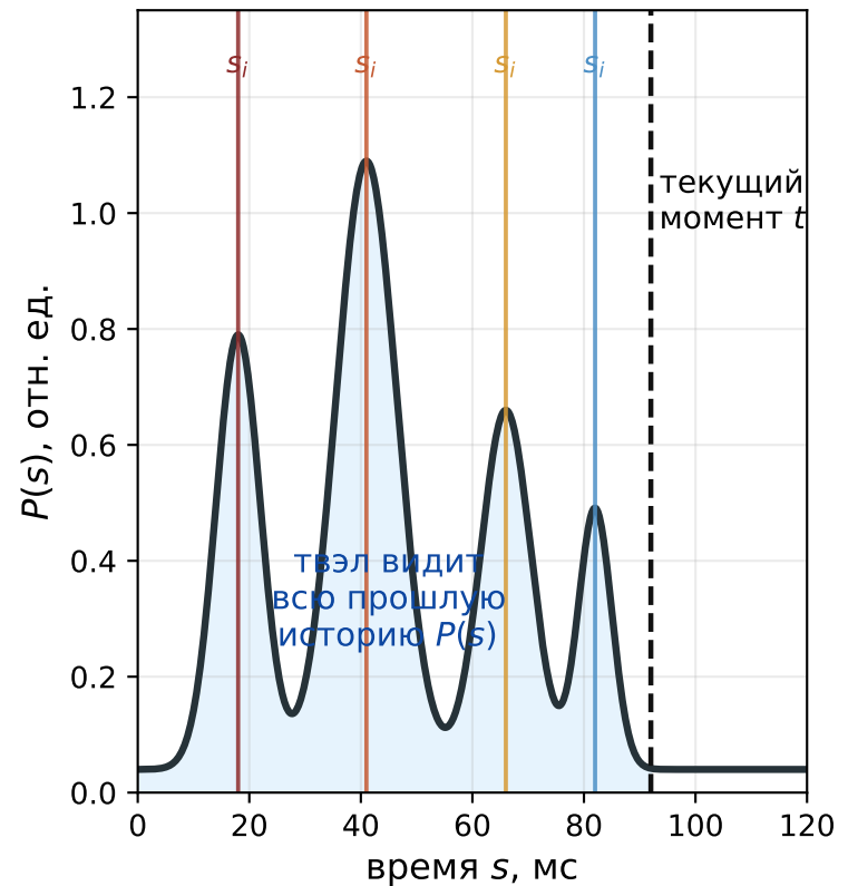
(а) История мощности
