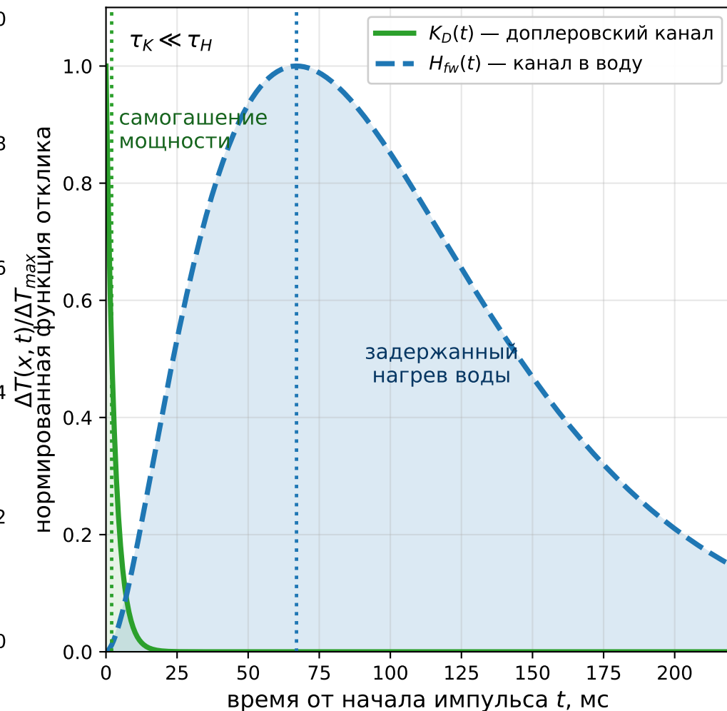
(б) Два выхода одного температурного следа
