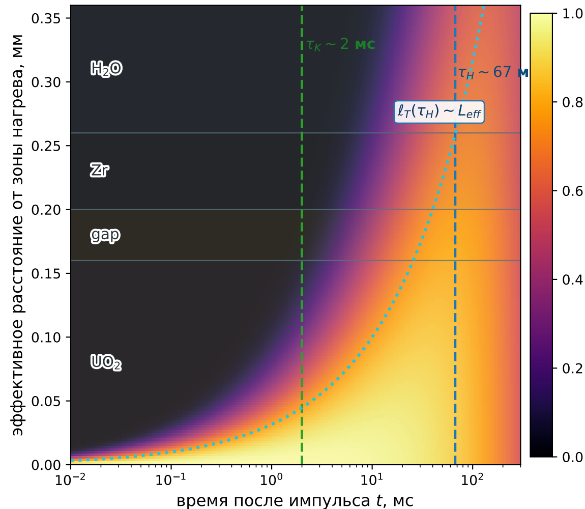
(а) Тепловой след: l_T(t) = \sqrt{\alpha_f t}
