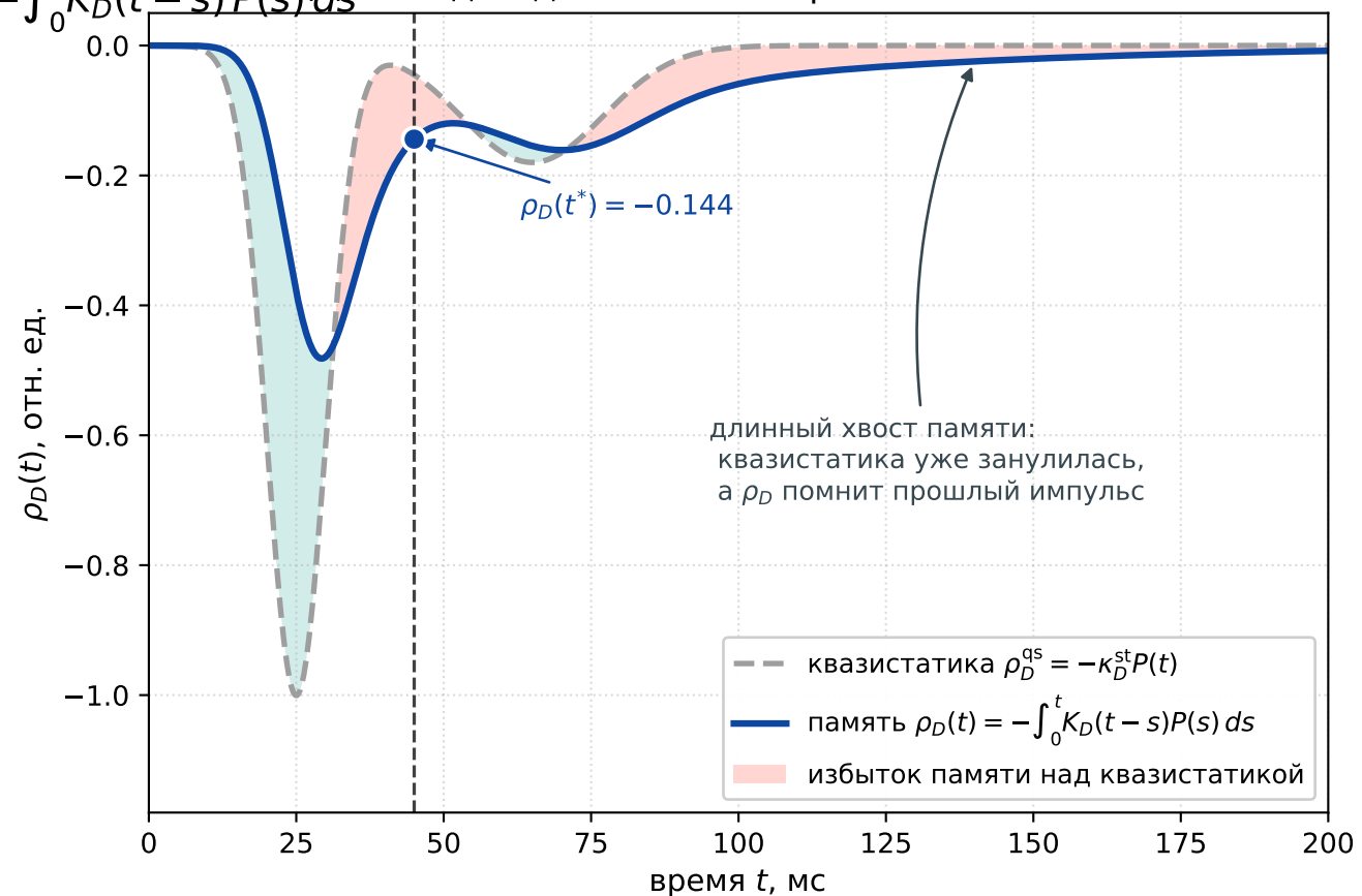
(г) Выход модели: память против квазистатики
