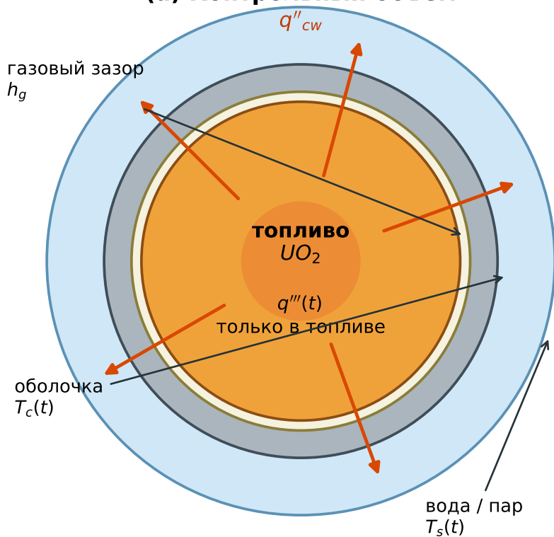
(а) Контрольный объем
