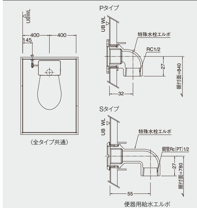
給水管立ち上げ位置
