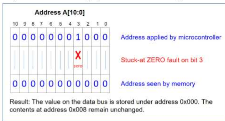
Abbildung 8: Beispiel eines Stuck-at ZERO Fehlers auf dem Address Bus
