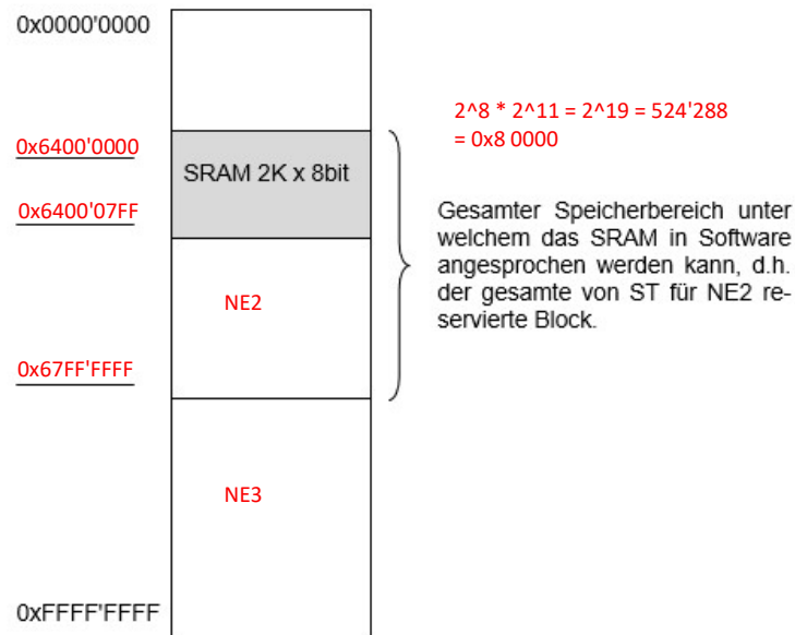
Abbildung 5: Memory Map mit Speicherbereichen
