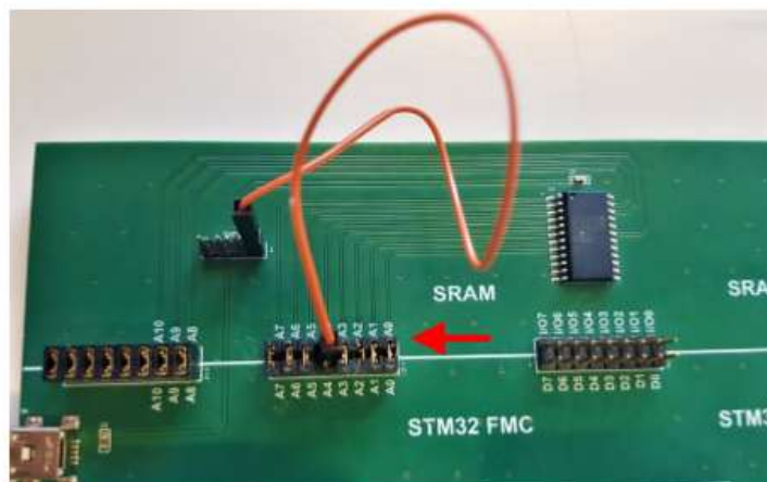
Abbildung 10: SRAM Zusatzboard mit Jumperkabel und Stuck-at-Address Fehler
