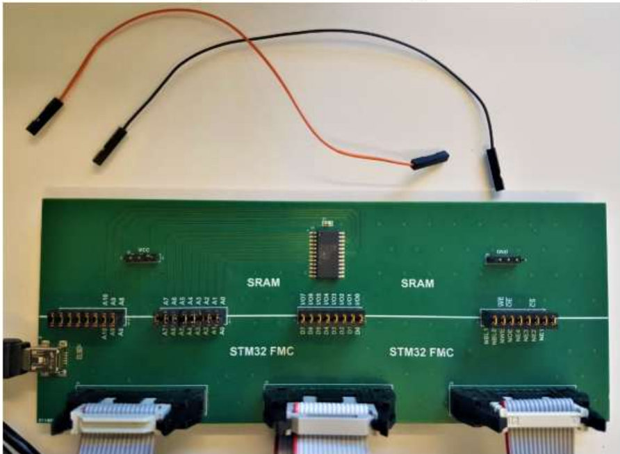
Abbildung 3: SRAM Zusatzboard mit Jumperkabel
