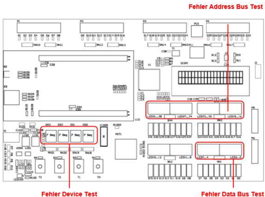
Abbildung 12: Anzeige von fehlgeschlagenen Tests auf CT-Board
