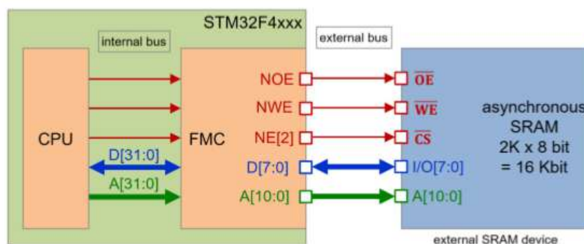
Abbildung 1: Anschluss SRAM an STM32 Microcontroller
