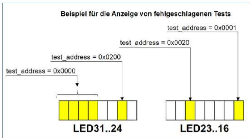
Abbildung 9: Anzeige von fehlgeschlagenen Address Bus Tests
