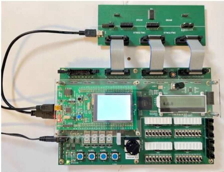
Abbildung 2: CT-Board mit angeschlossenem SRAM Zusatzboard
