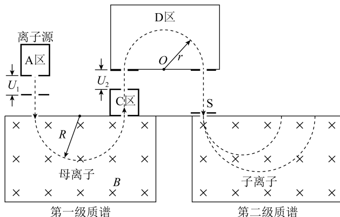
第一级质谱
