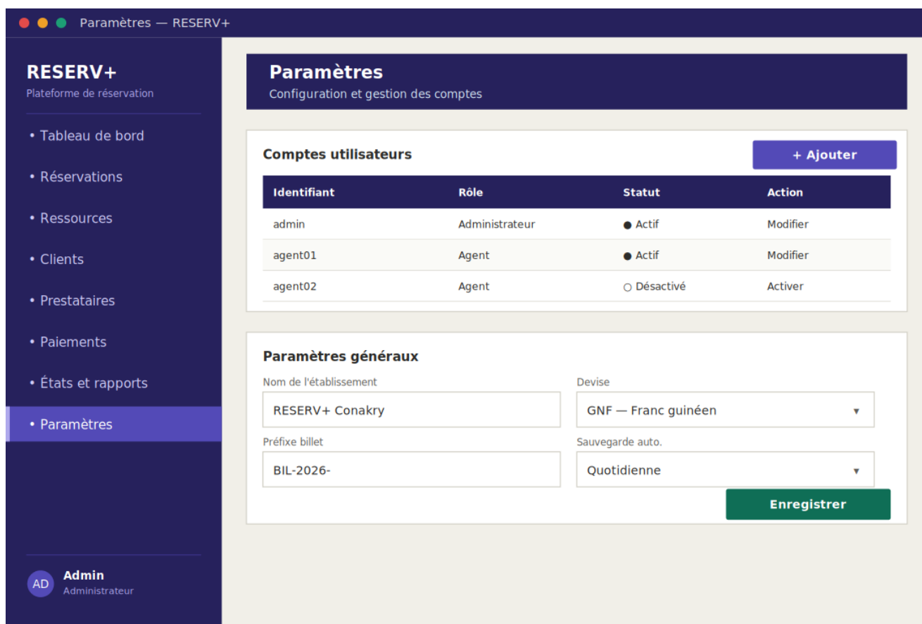
Figure 10 — Configuration et gestion des comptes
