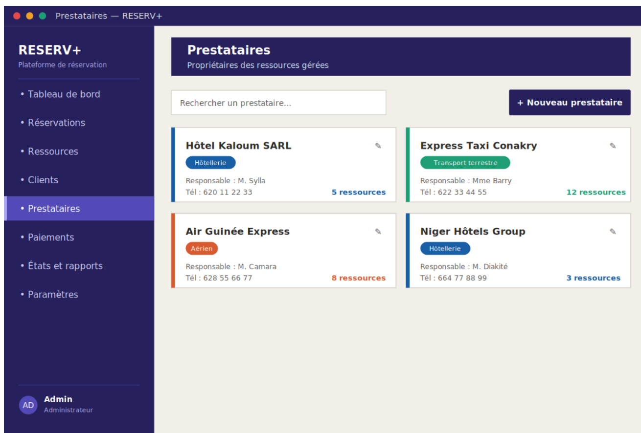
Figure 7 — Fiches des prestataires propriétaires des ressources
