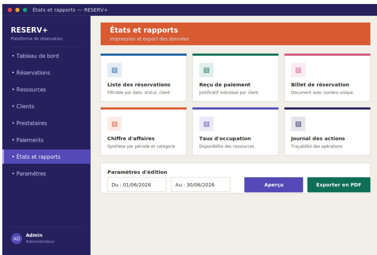
Figure 9 — Centre d'édition des états imprimables
