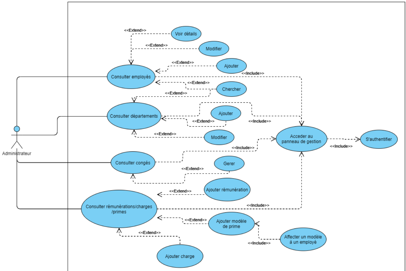
FIGURE 3.2 – Diagramme de cas d'utilisation pour l'Administrateur
