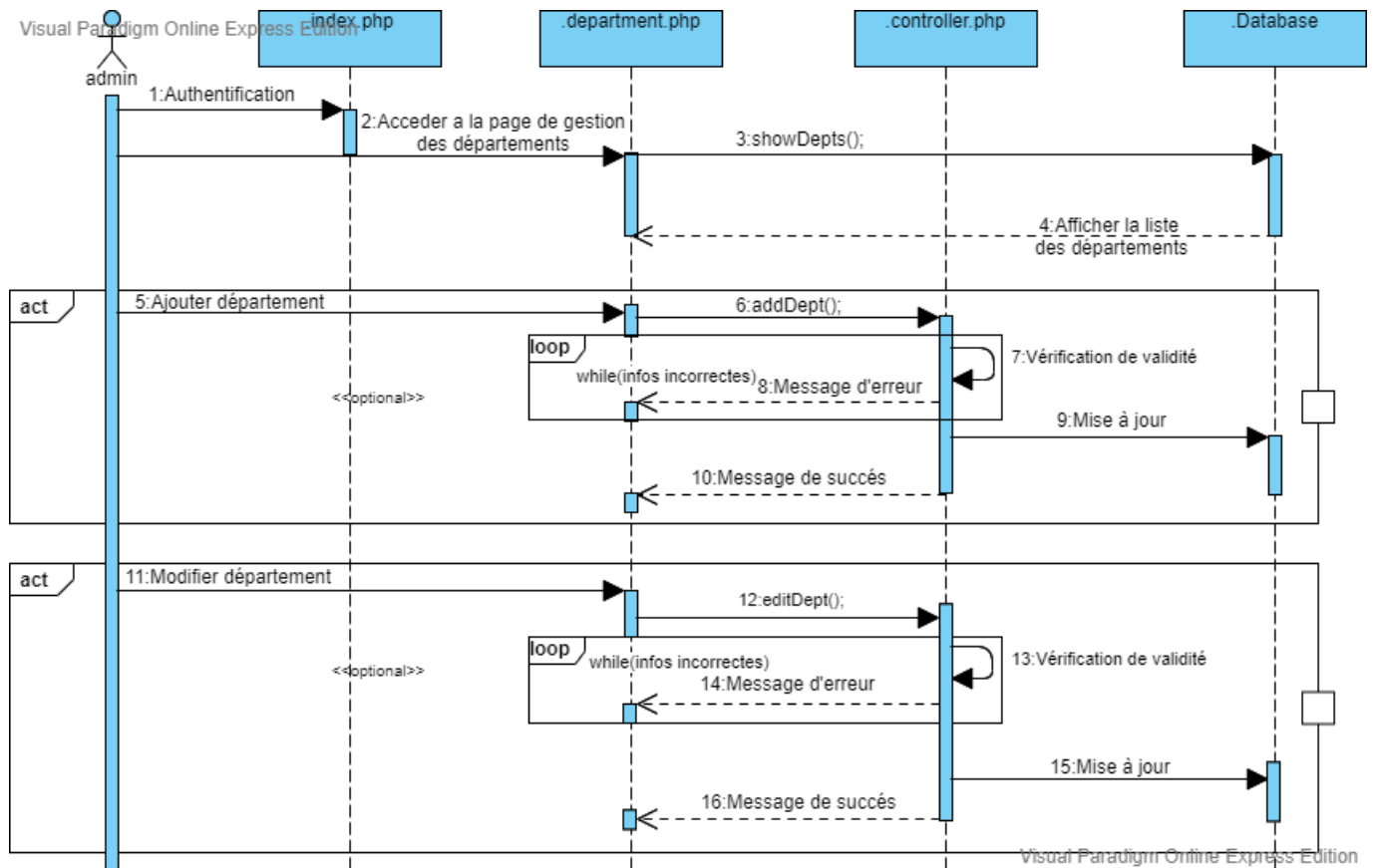
FIGURE 3.6 – Diagramme de séquence du scénario "Gérer les départements"
