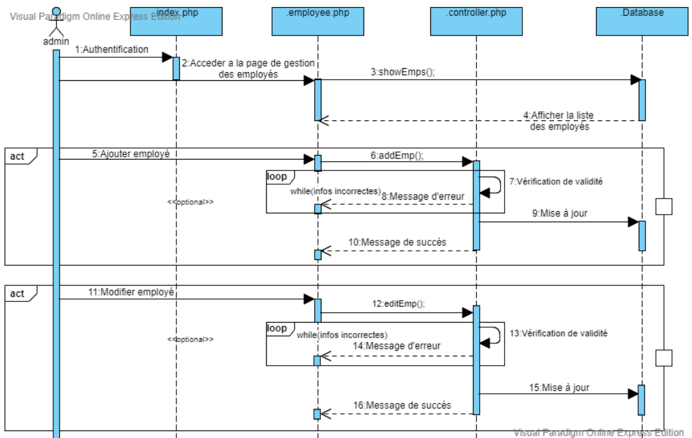
FIGURE 3.5 – Diagramme de séquence du scénario "Gérer les employés"
