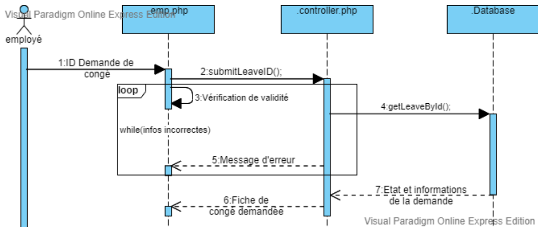
FIGURE 3.10 – Diagramme de séquence du scénario "Consulter l'état d'une demande de congé"
