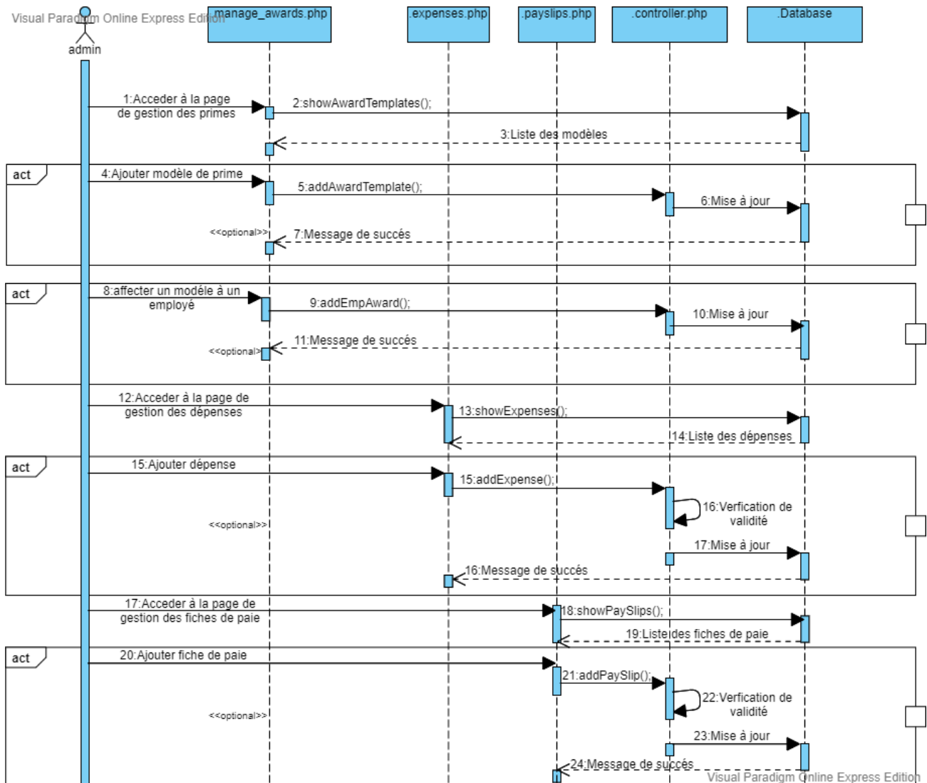
FIGURE 3.8 – Diagramme de séquence du scénario "Gestion du module finance"
