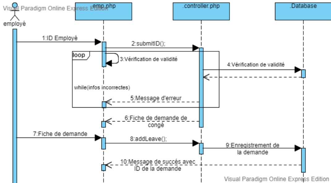
FIGURE 3.9 – Diagramme de séquence du scénario "Déposer une demande de congé"
