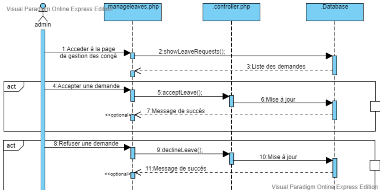
FIGURE 3.7 – Diagramme de séquence du scénario "Gérer les congés"
