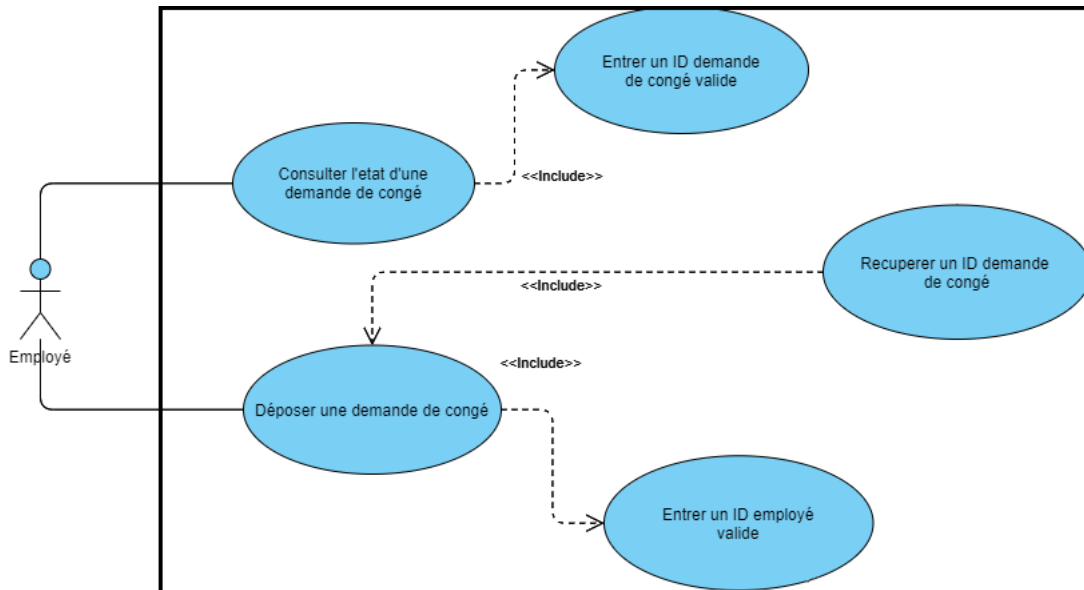
FIGURE 3.3 – Diagramme de cas d'utilisation pour l'Employé
