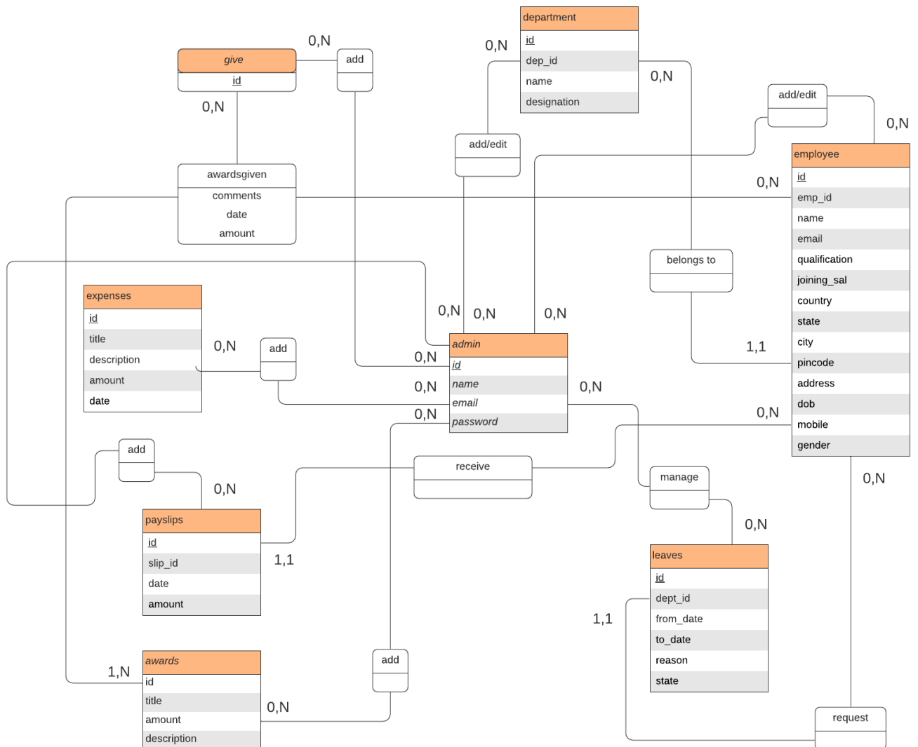
FIGURE 3.1 – Modèle conceptuel de données
