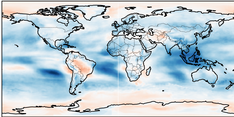
\Delta\text{CLT} : Hadley – GFDL
