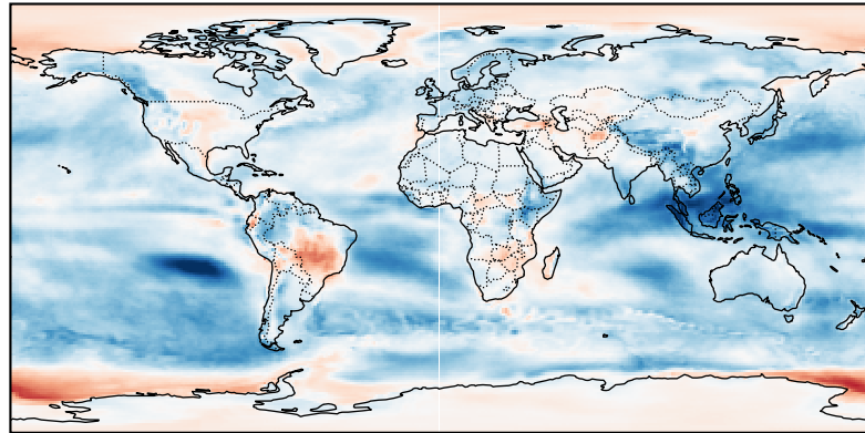
\Delta\text{SW} : Hadley – GFDL
