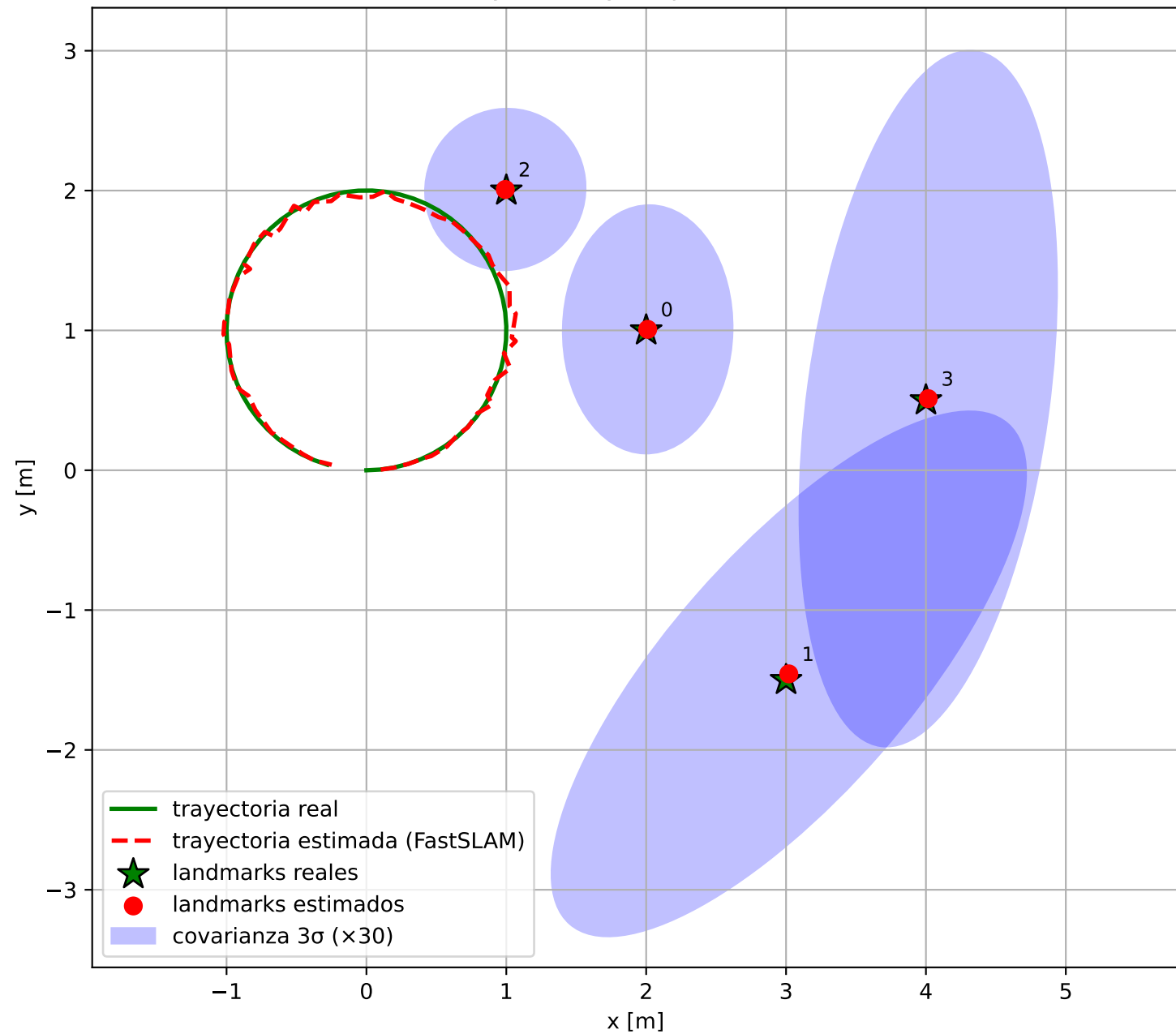
TP5 - FastSLAM: trayectoria y mapa de landmarks estimados
