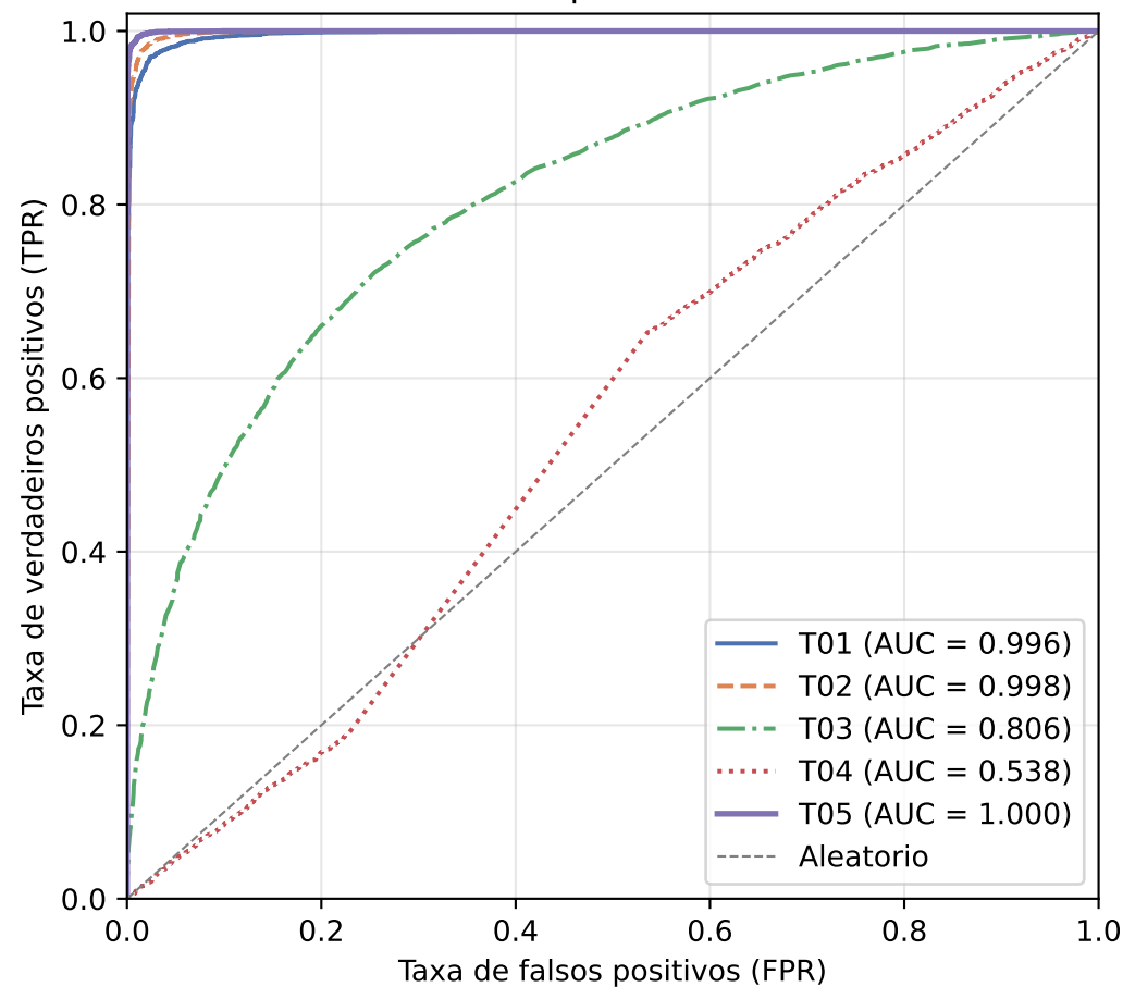
Curvas ROC - protocolo standard
