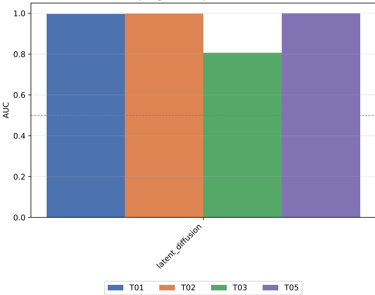
AUC por gerador - protocolo standard
