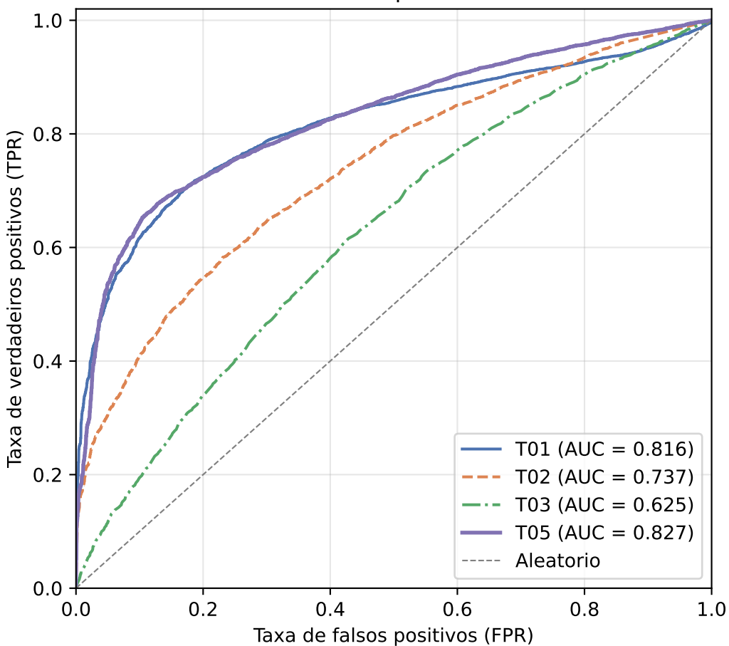
Curvas ROC - protocolo ood
