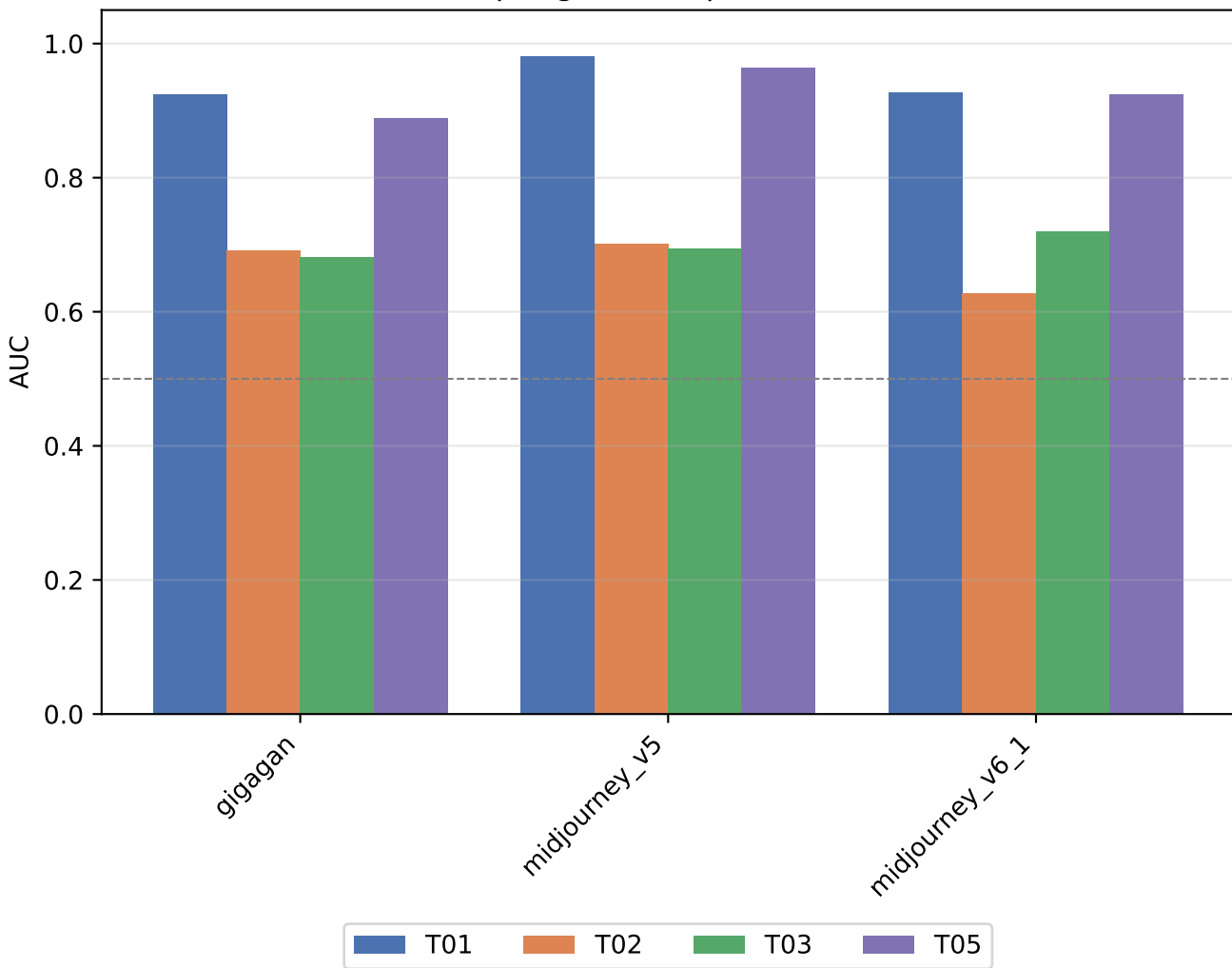
AUC por gerador - protocolo ood
