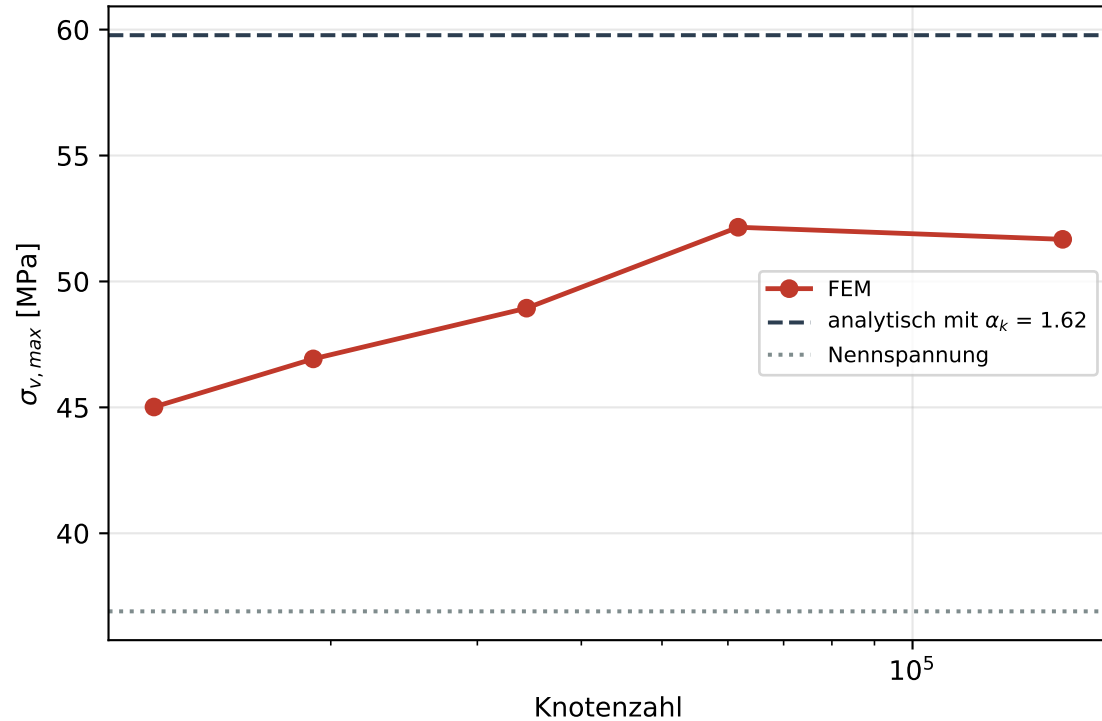
Netzkonvergenz Vergleichsspannung
