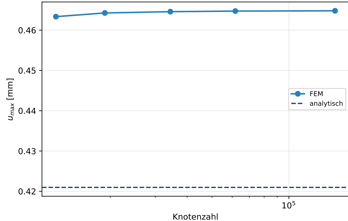
Netzkonvergenz Verformung
