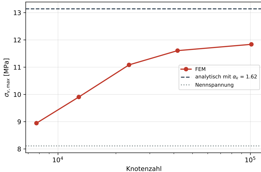
Netzkonvergenz Vergleichsspannung
