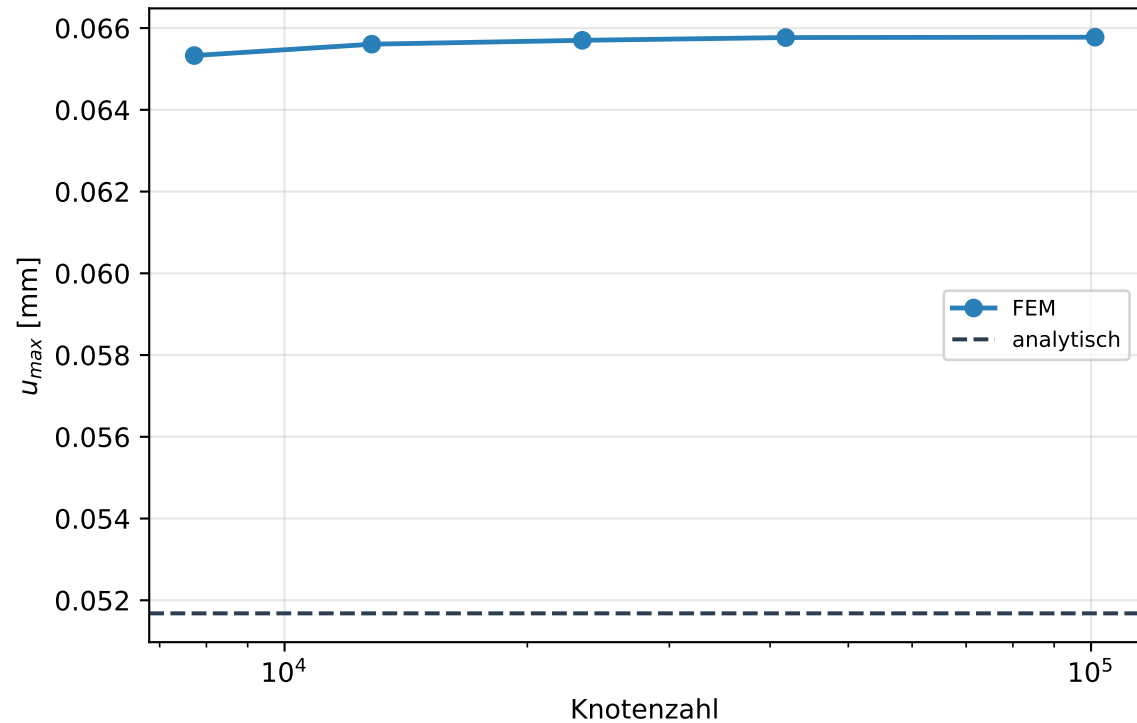
Netzkonvergenz Verformung
