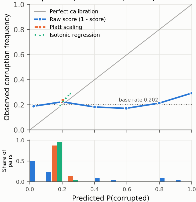
helpfulness, eta = 20% (diverse)
