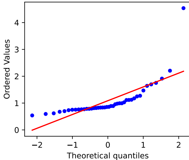
Q-Q plot: FIMO hits per motif 1e6 Shapiro-Wilk p = 1.57e-09 , n = 42
