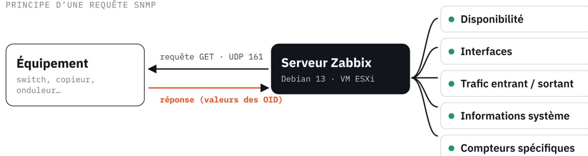
PRINCIPE D'UNE REQUÊTE SNMP
