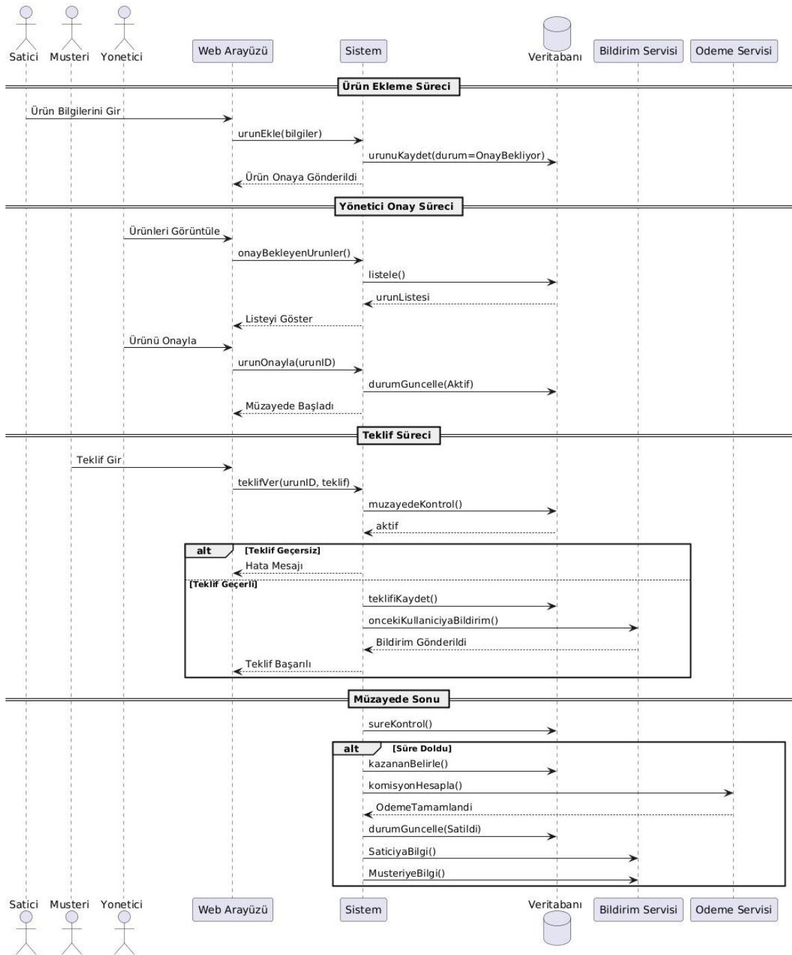
Şekil 6: Aktörler ve Sistem Bileşenleri Arasındaki Sequence (Sıra) Diyagramı
