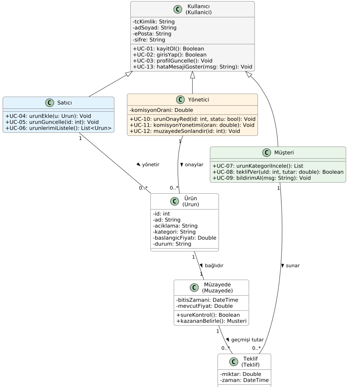
Şekil 2: Online Müzayede Sistemi'nin nesne yönelimli (OOP) mimarisini, veri modellerini ve sınıflar arasındaki hiyerarşik ilişkileri tanımlayan Sınıf Diyagramı
