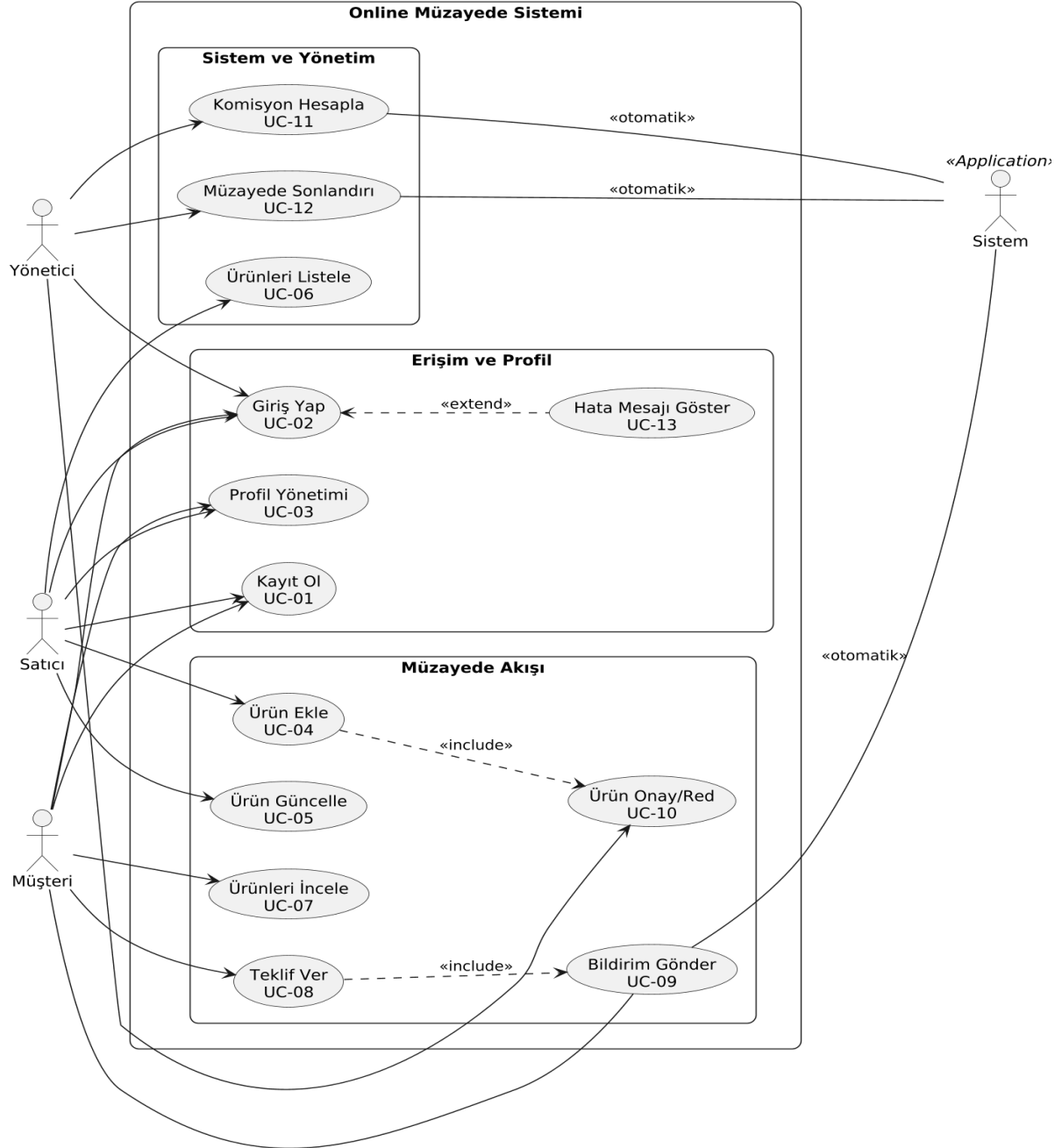
Şekil 1: Online Müzayede Sistemi'nin işlevsel kapsamını ve kullanıcı rollerini (Satıcı, Müşteri, Yönetici) gösteren Use Case Diyagramı
