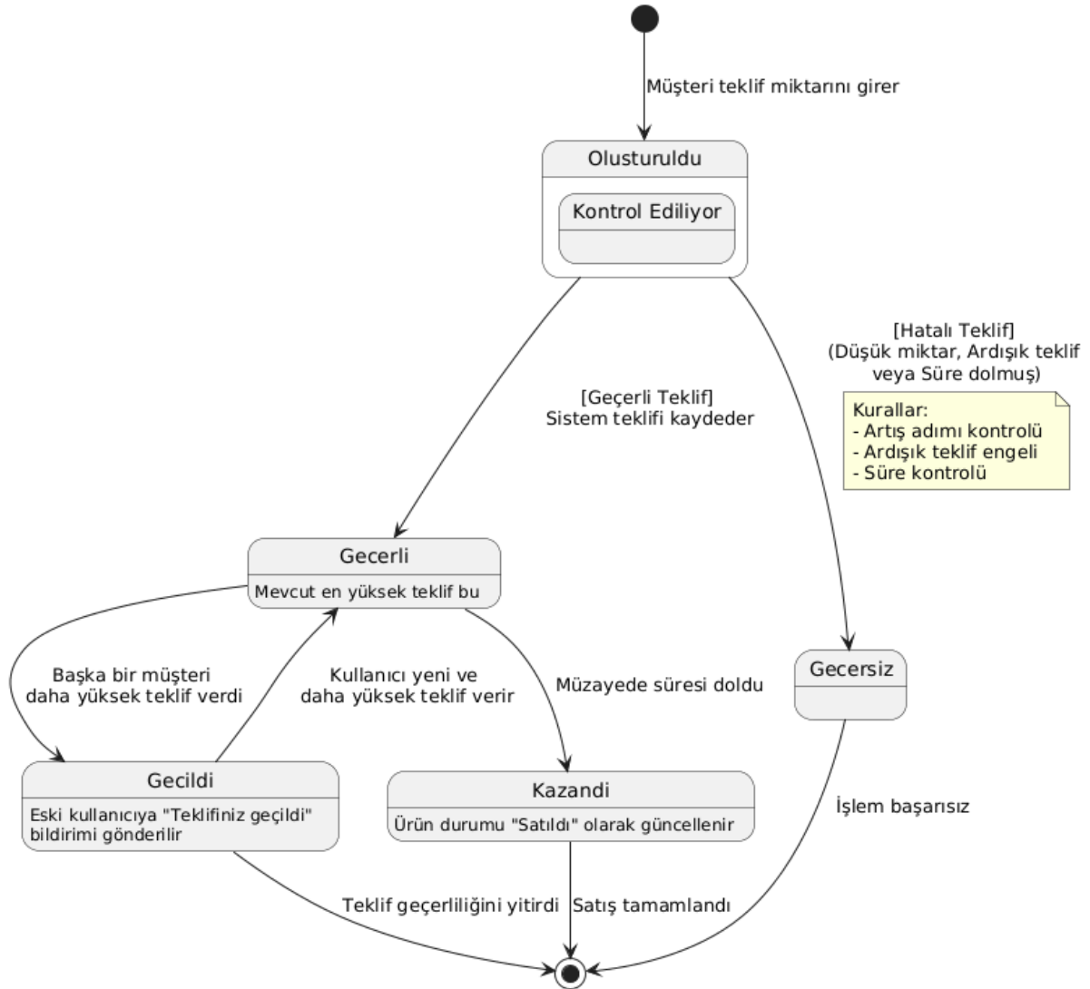
Şekil 4: Teklif Durum Diyagramı
