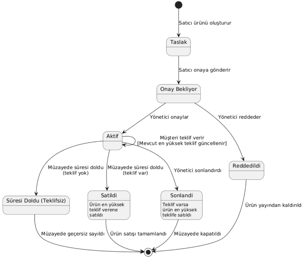
Şekil 3: Ürün Durum Diyagramı
