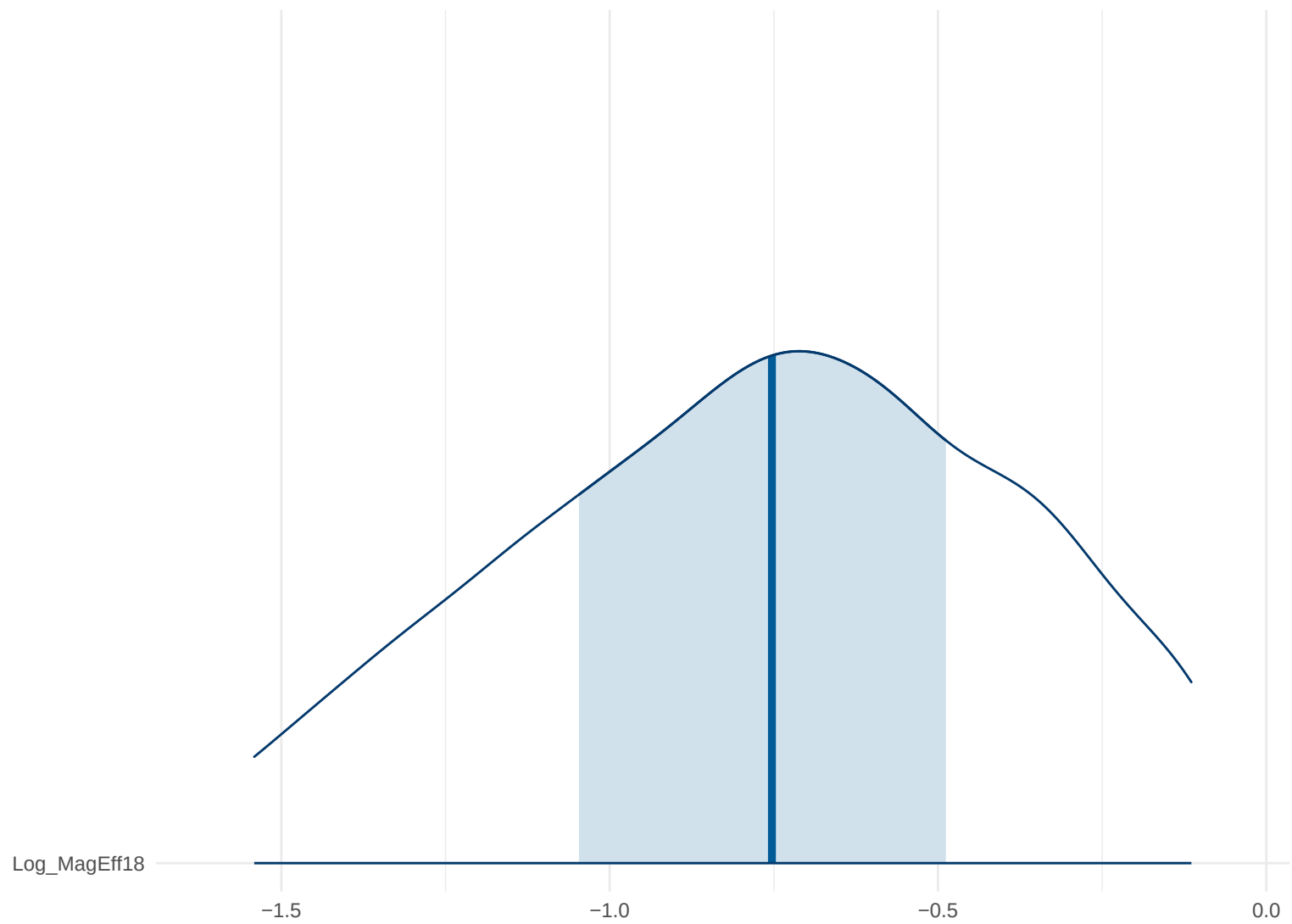
Posterior Density: Log_MagEff18
