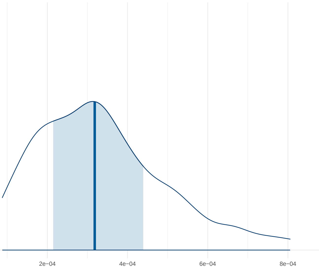
Posterior Density: Mig323
