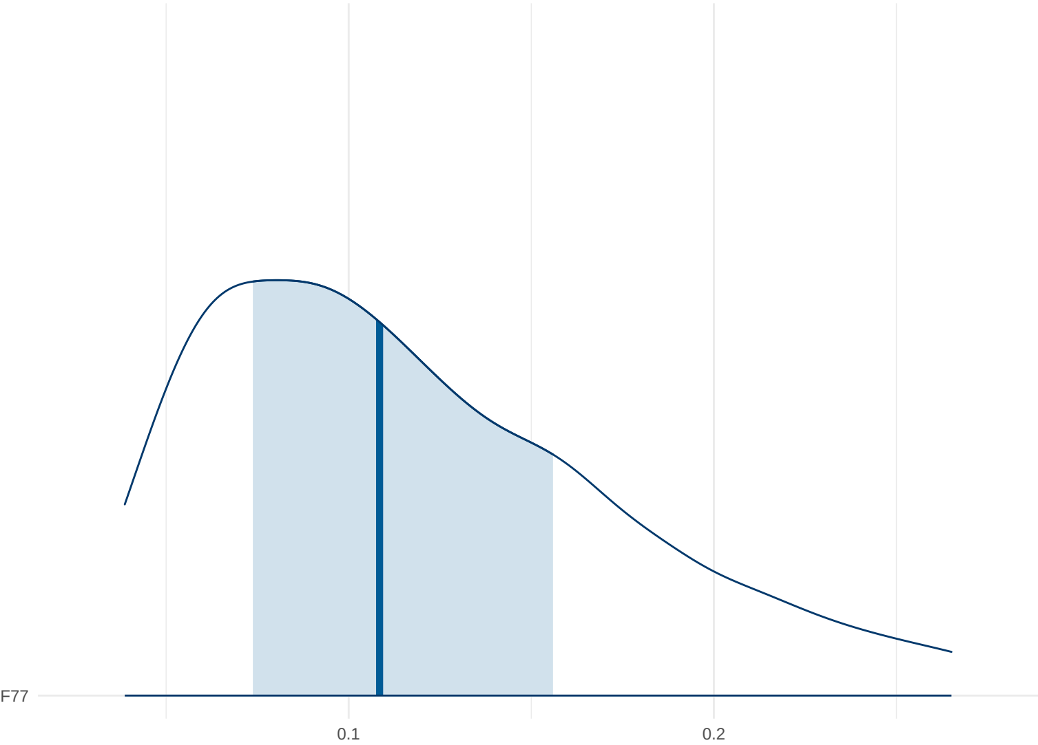
Posterior Density: F77
