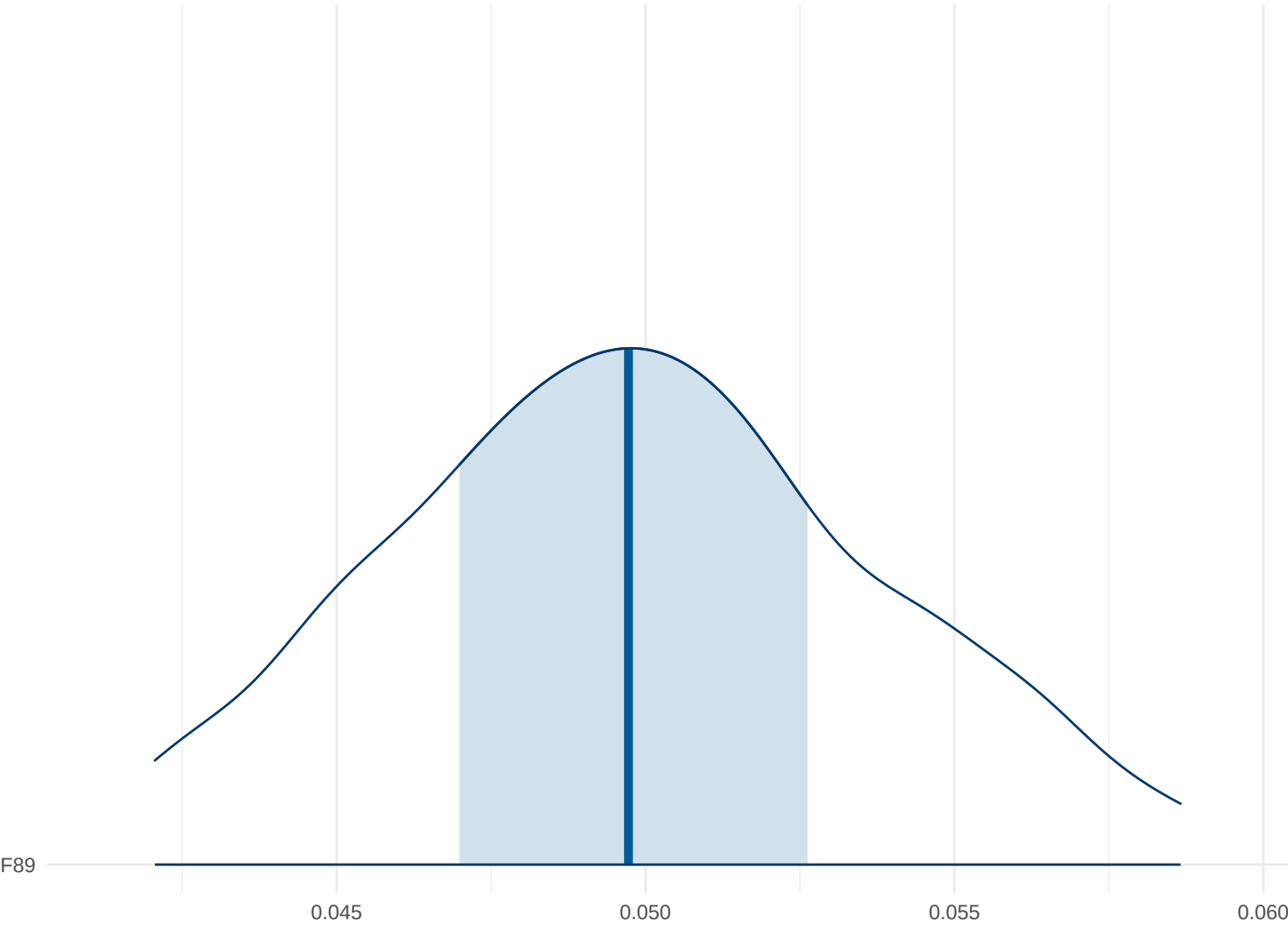
Posterior Density: F89
