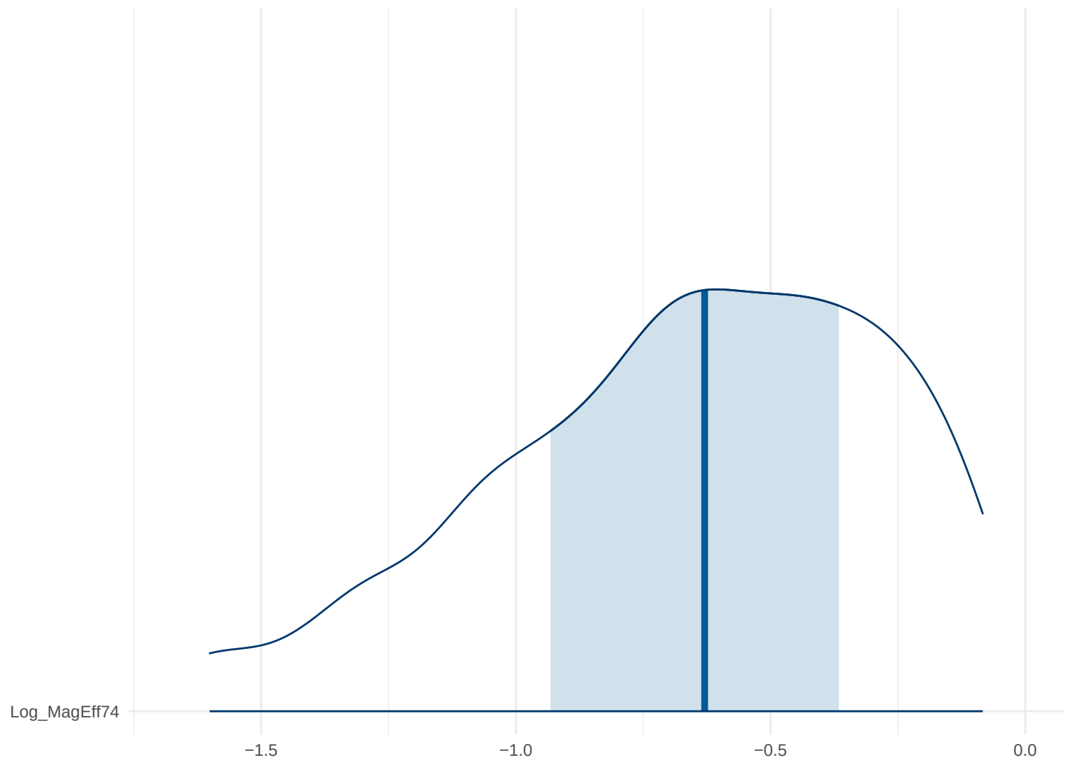
Posterior Density: Log_MagEff74
