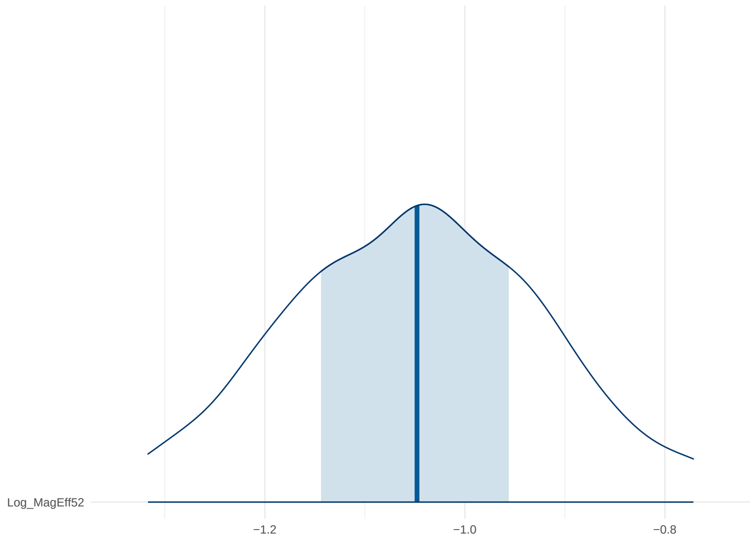
Posterior Density: Log_MagEff52
