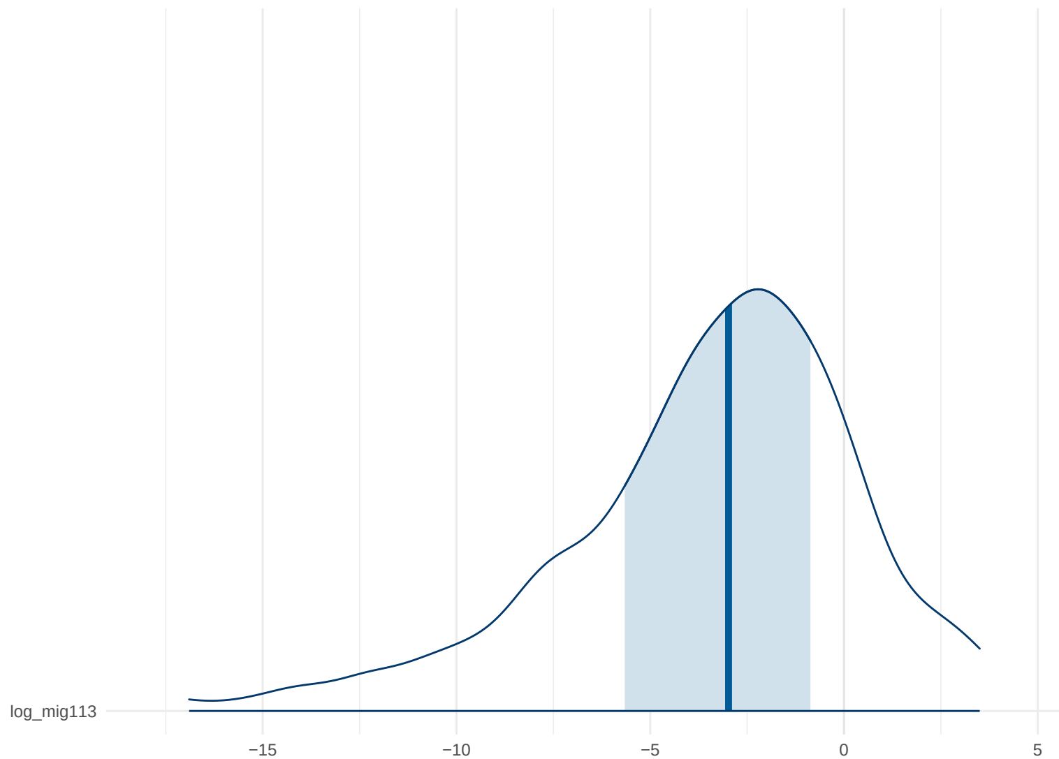
Posterior Density: log_mig113
