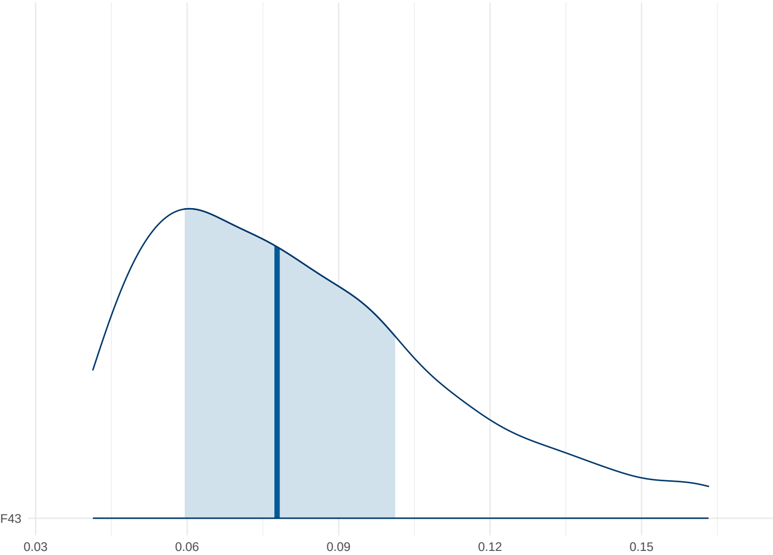
Posterior Density: F43
