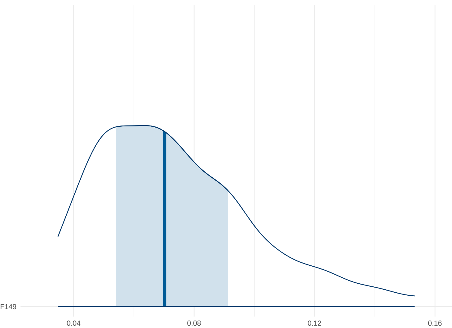
Posterior Density: F149
