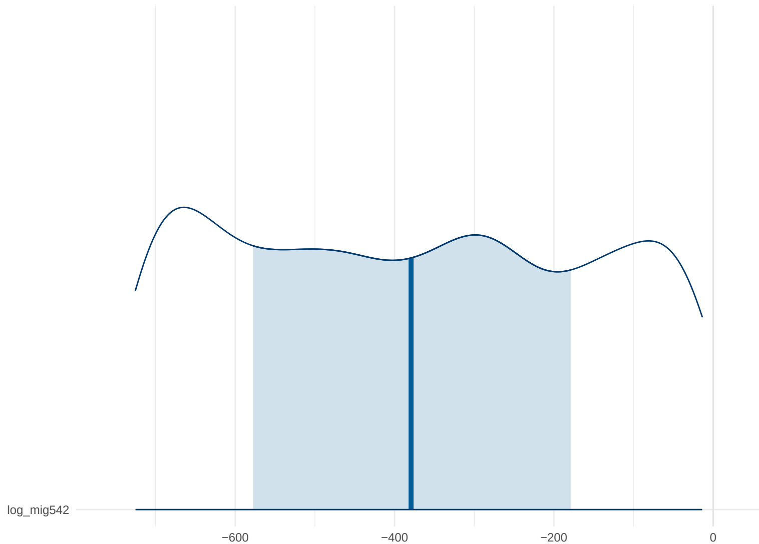
Posterior Density: log_mig542
