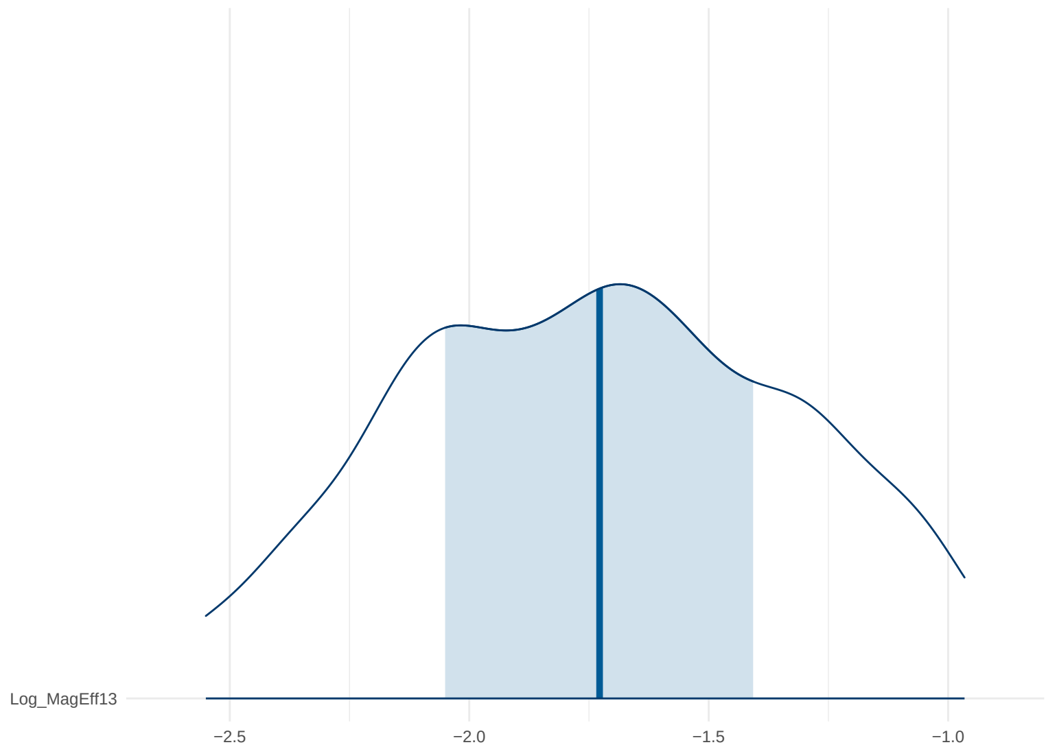
Posterior Density: Log_MagEff13
