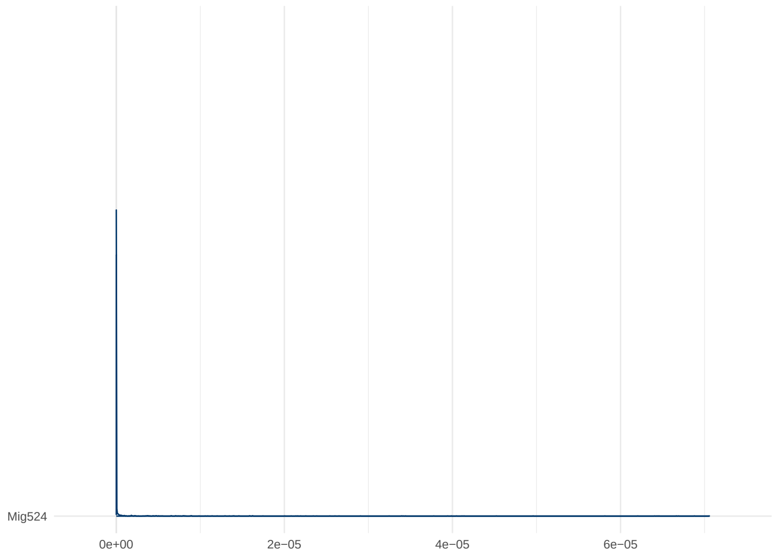
Posterior Density: Mig524
