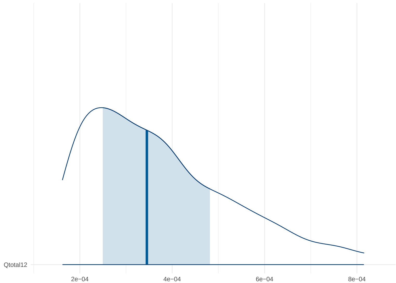
Posterior Density: Qtotal12
