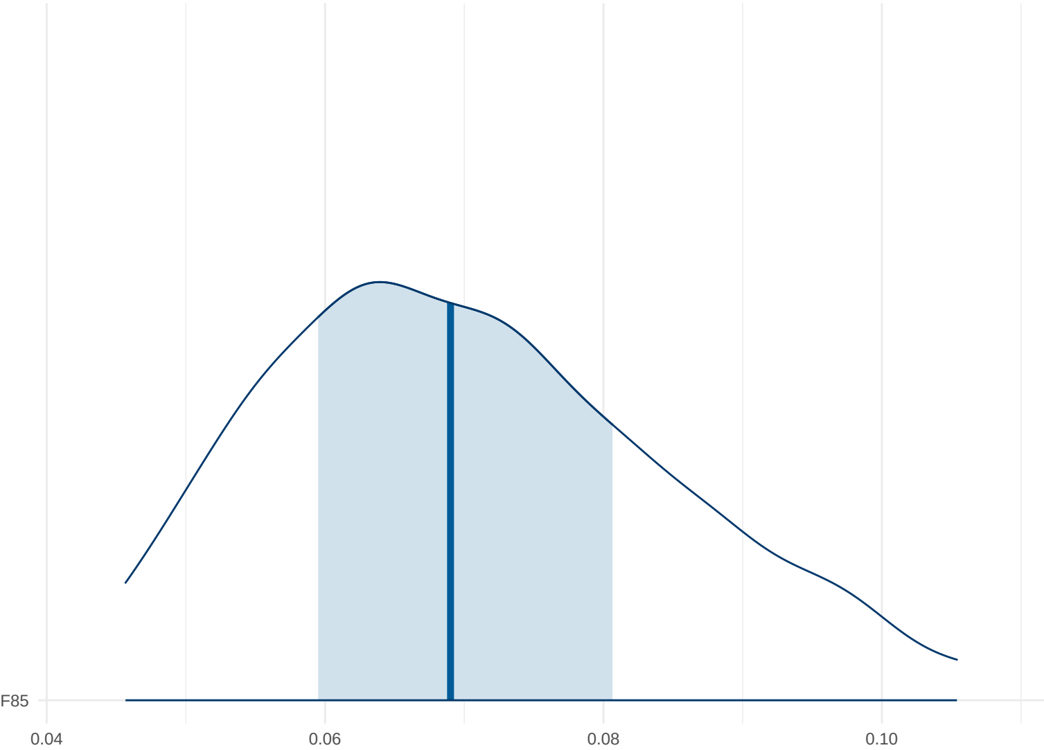
Posterior Density: F85
