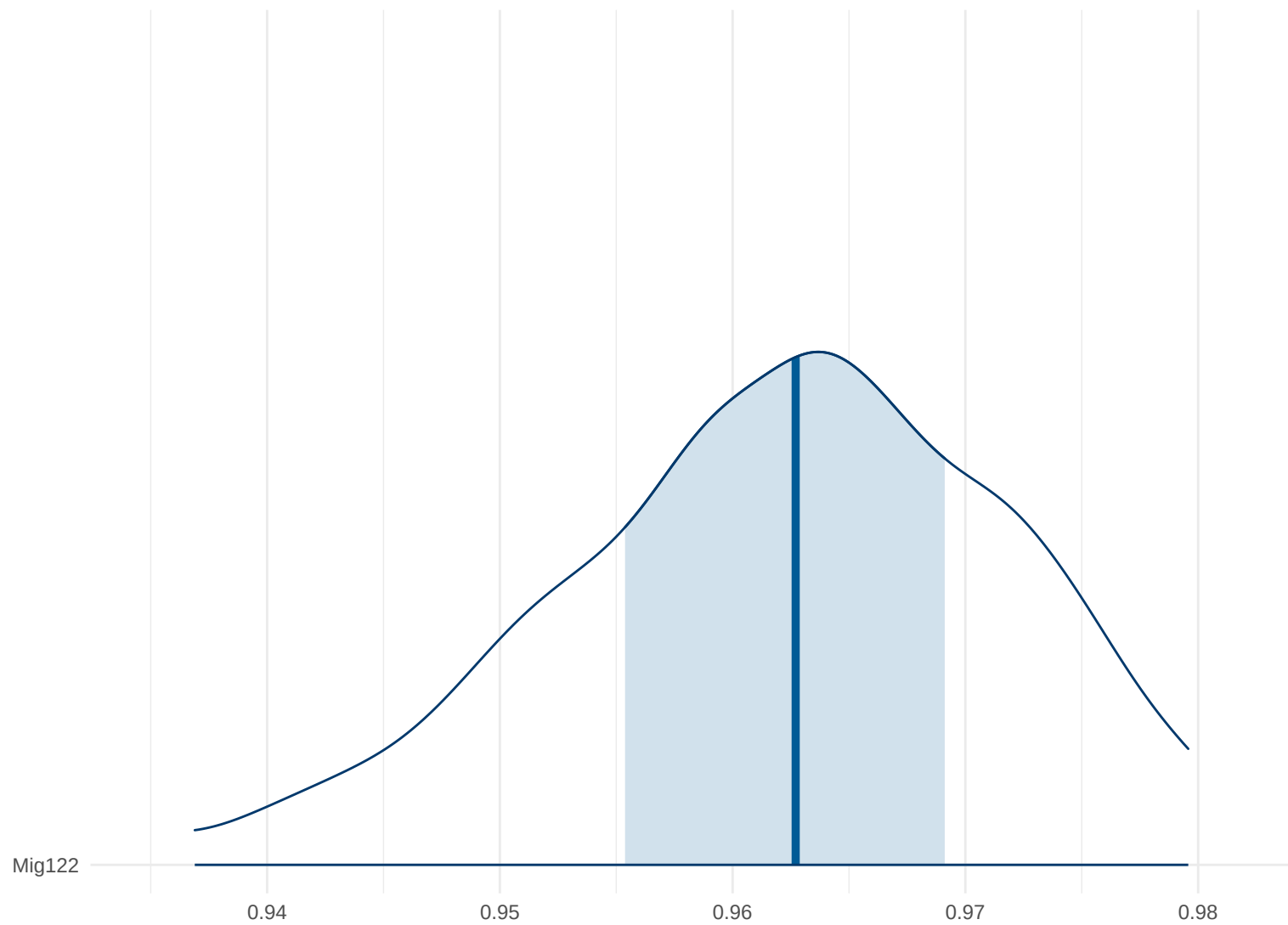
Posterior Density: Mig122
