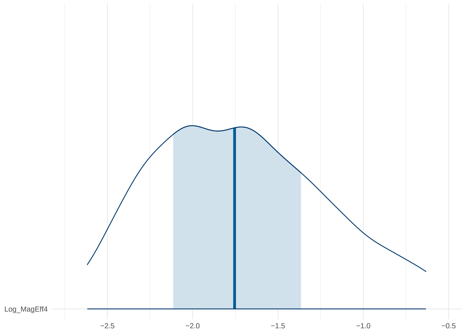
Posterior Density: Log_MagEff4
