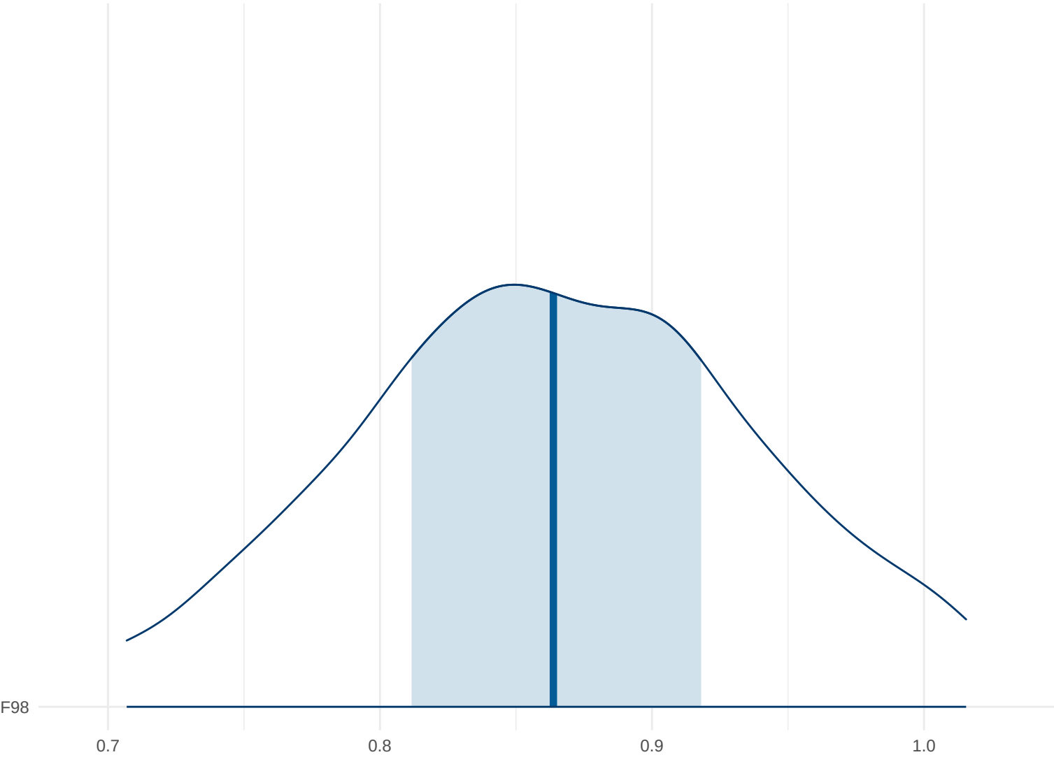
Posterior Density: F98
