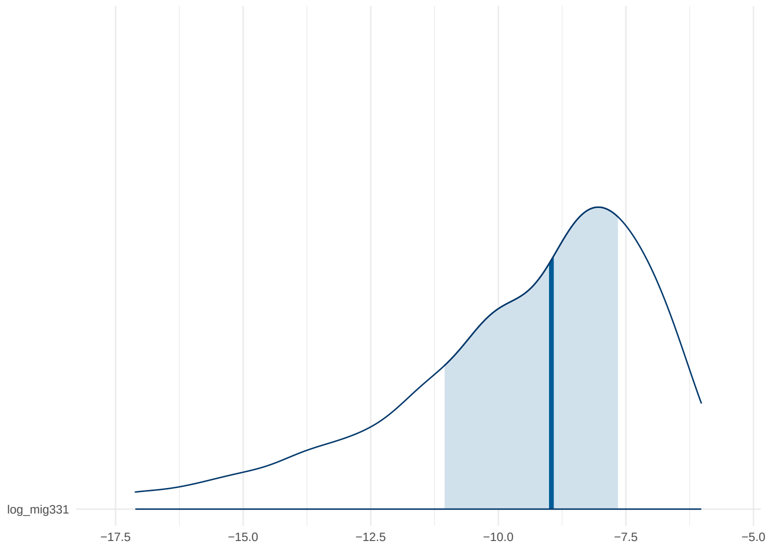
Posterior Density: log_mig331
