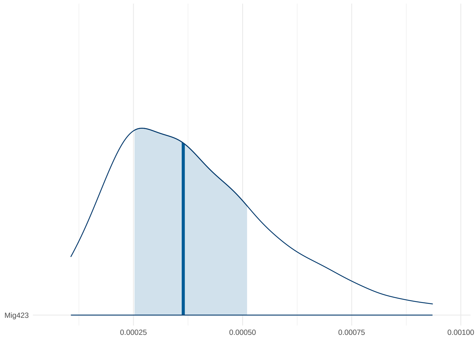
Posterior Density: Mig423
