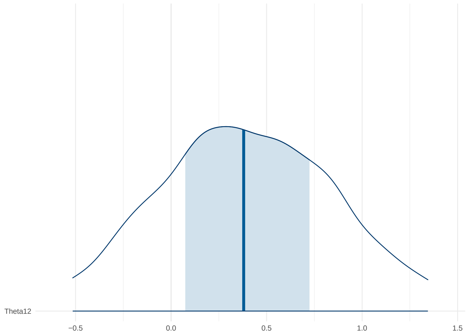
Posterior Density: Theta12
