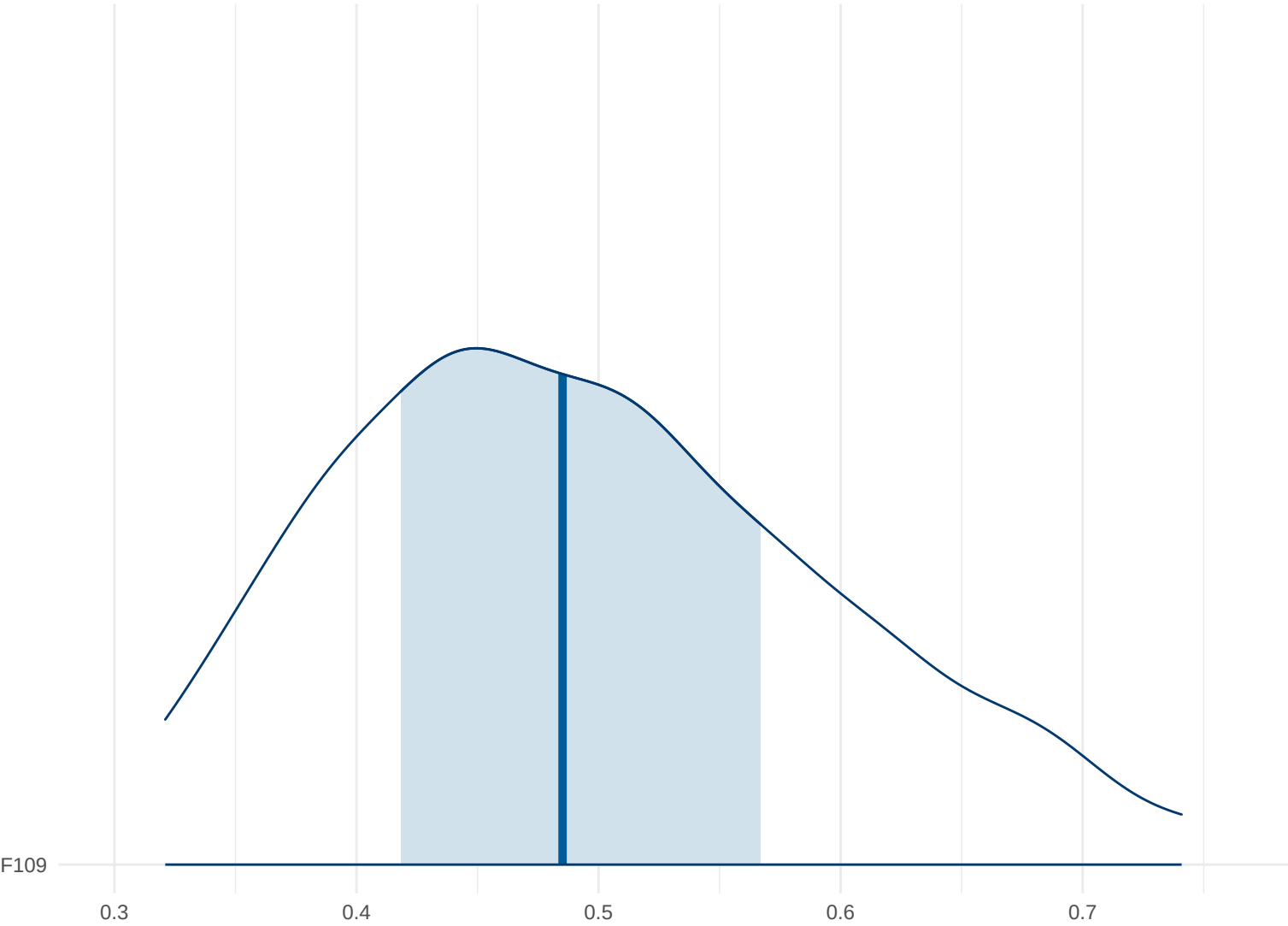
Posterior Density: F109
