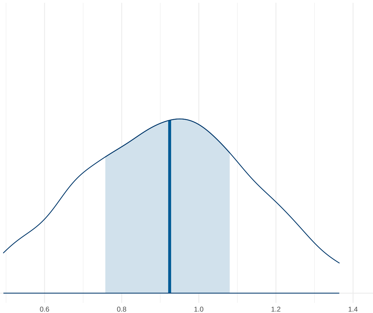
Posterior Density: Theta19
