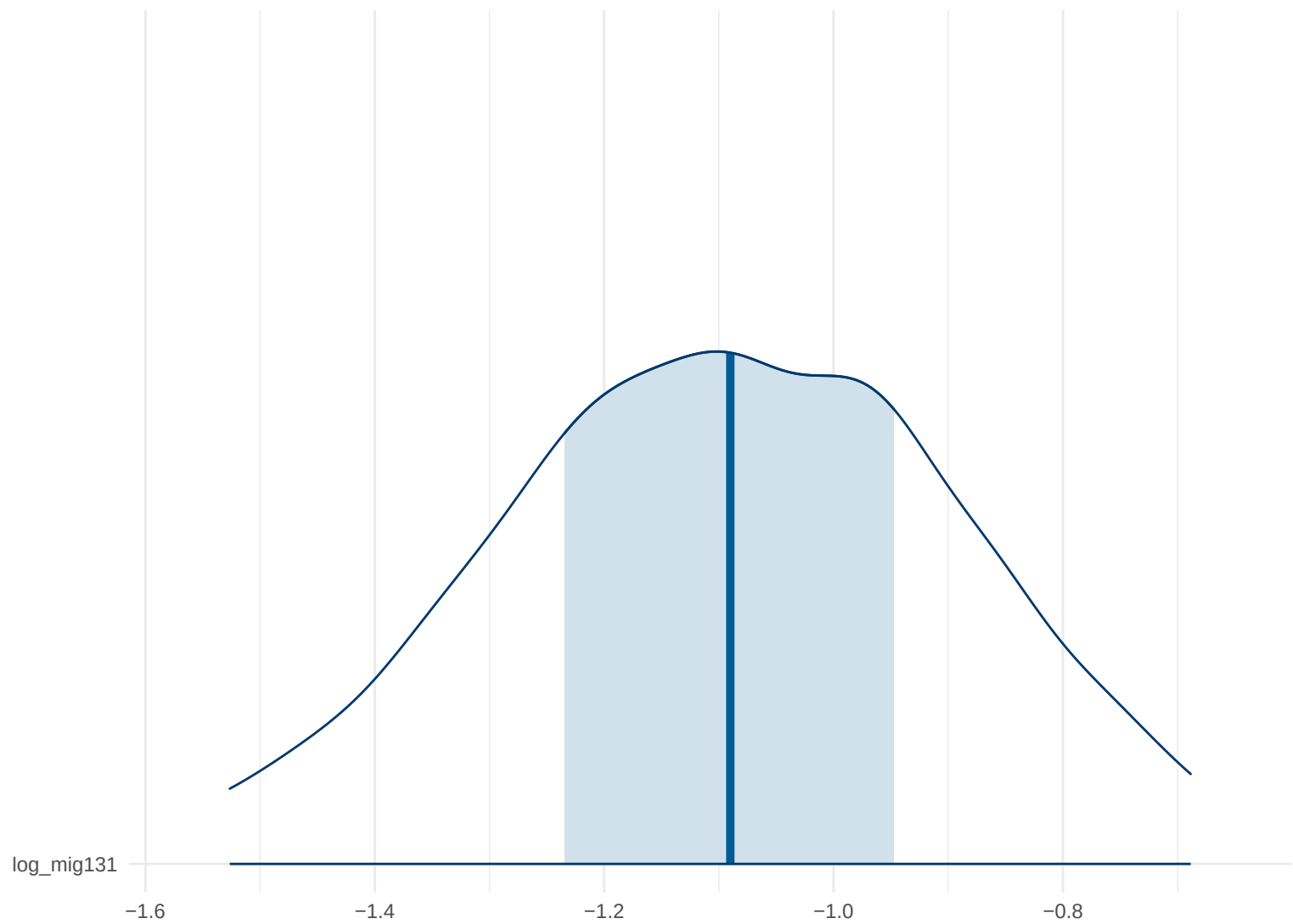
Posterior Density: log_mig131
