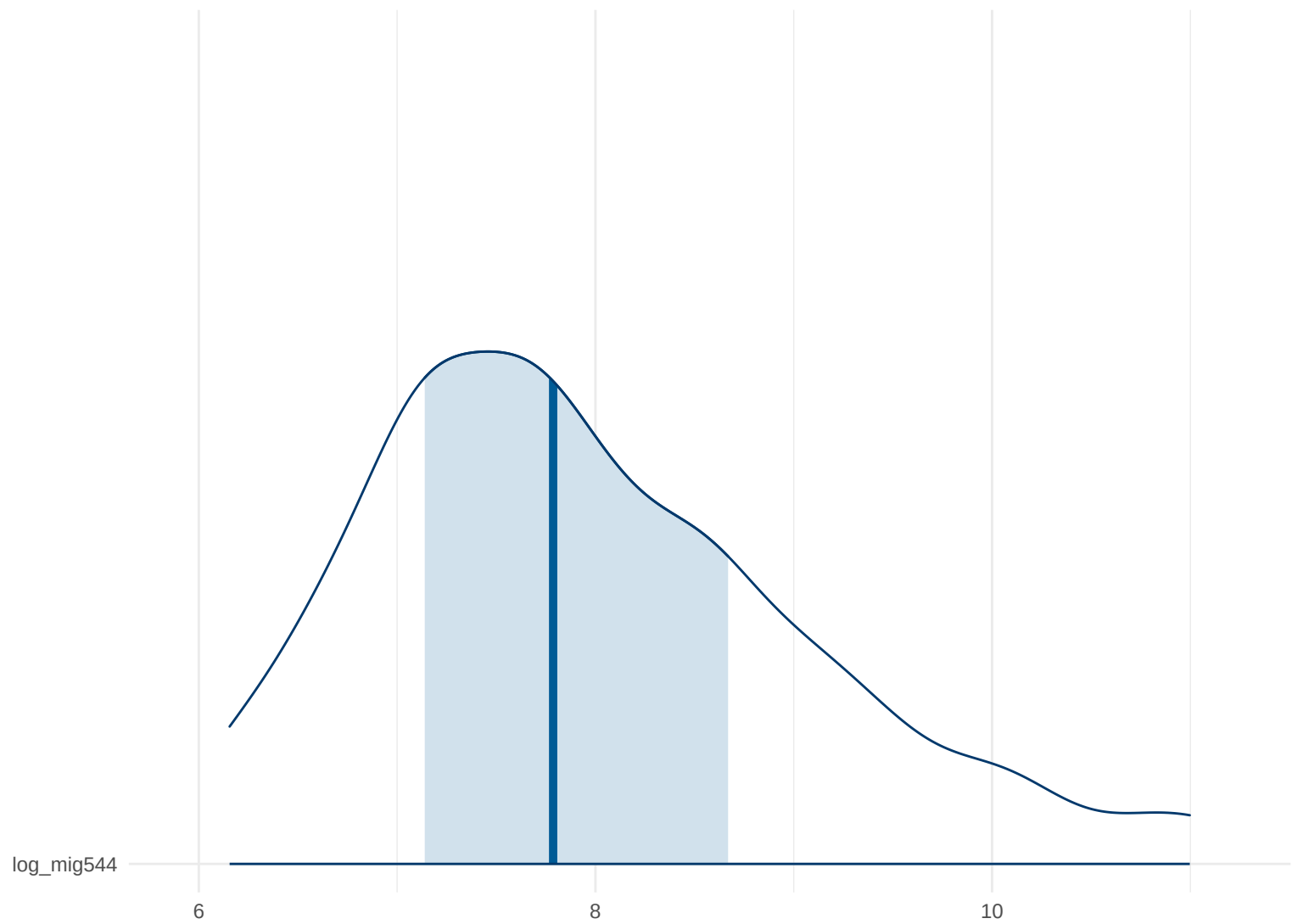
Posterior Density: log_mig544
