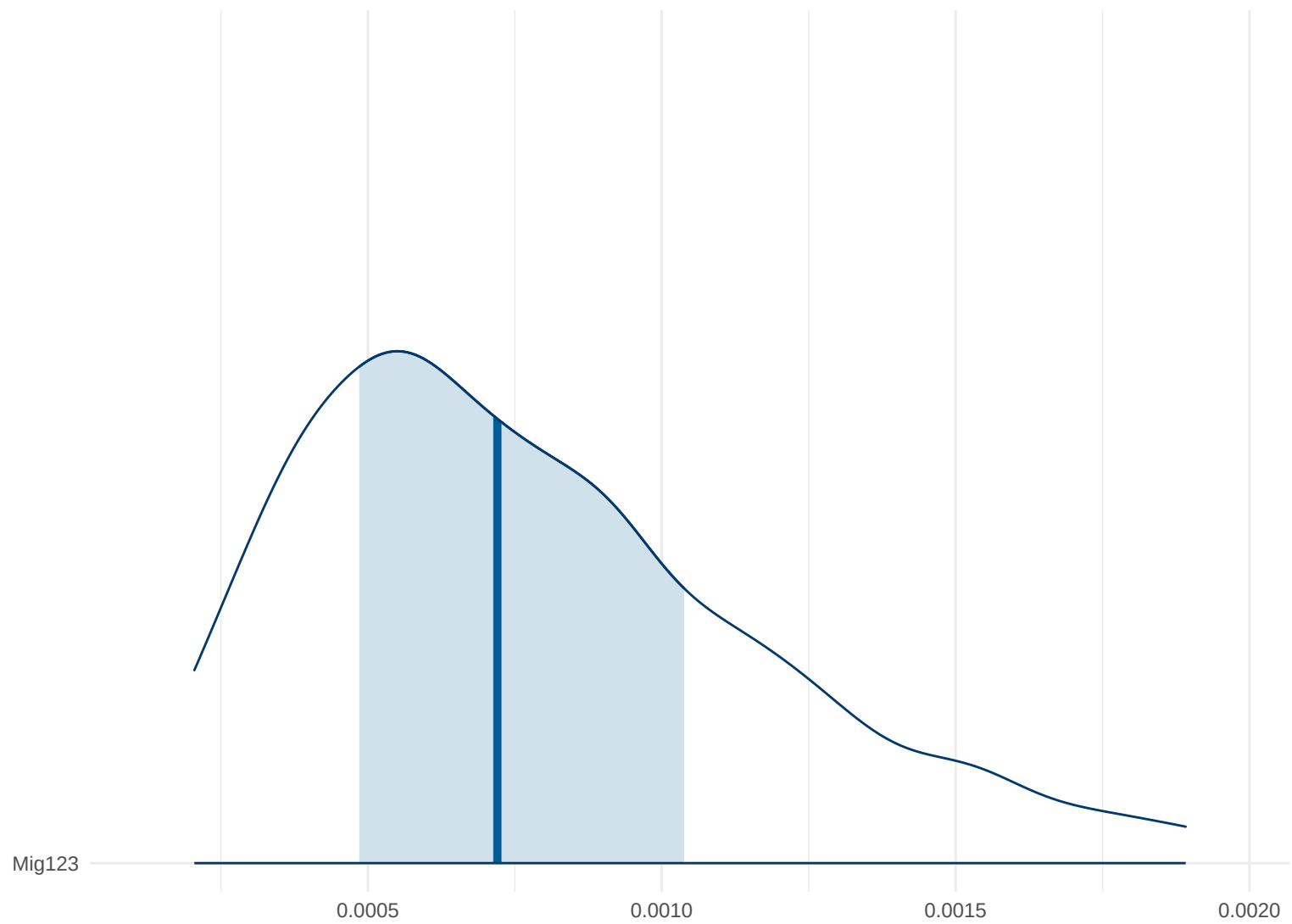
Posterior Density: Mig123
