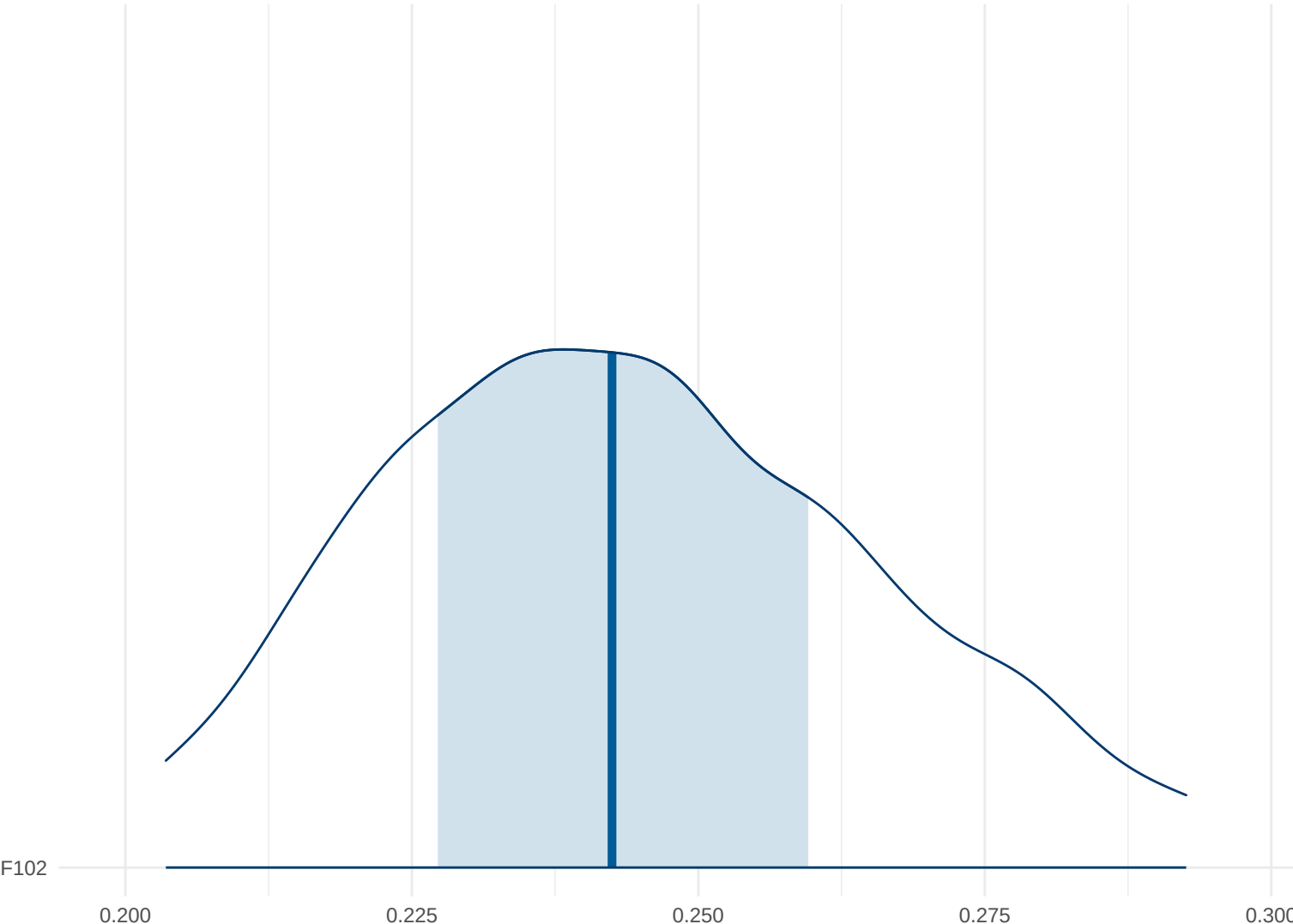
Posterior Density: F102
