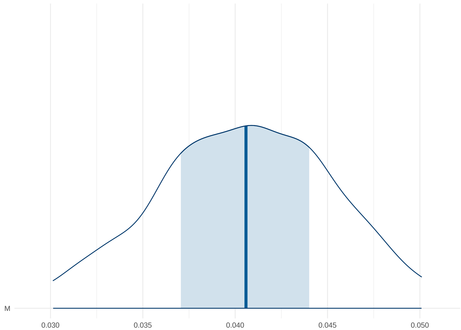
Posterior Density: M
