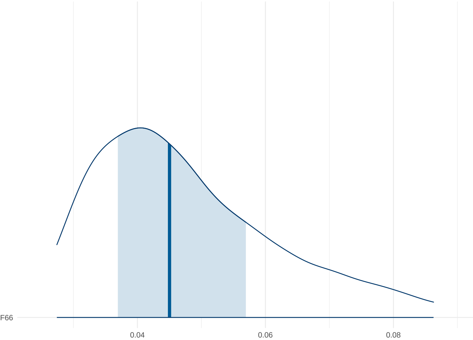
Posterior Density: F66
