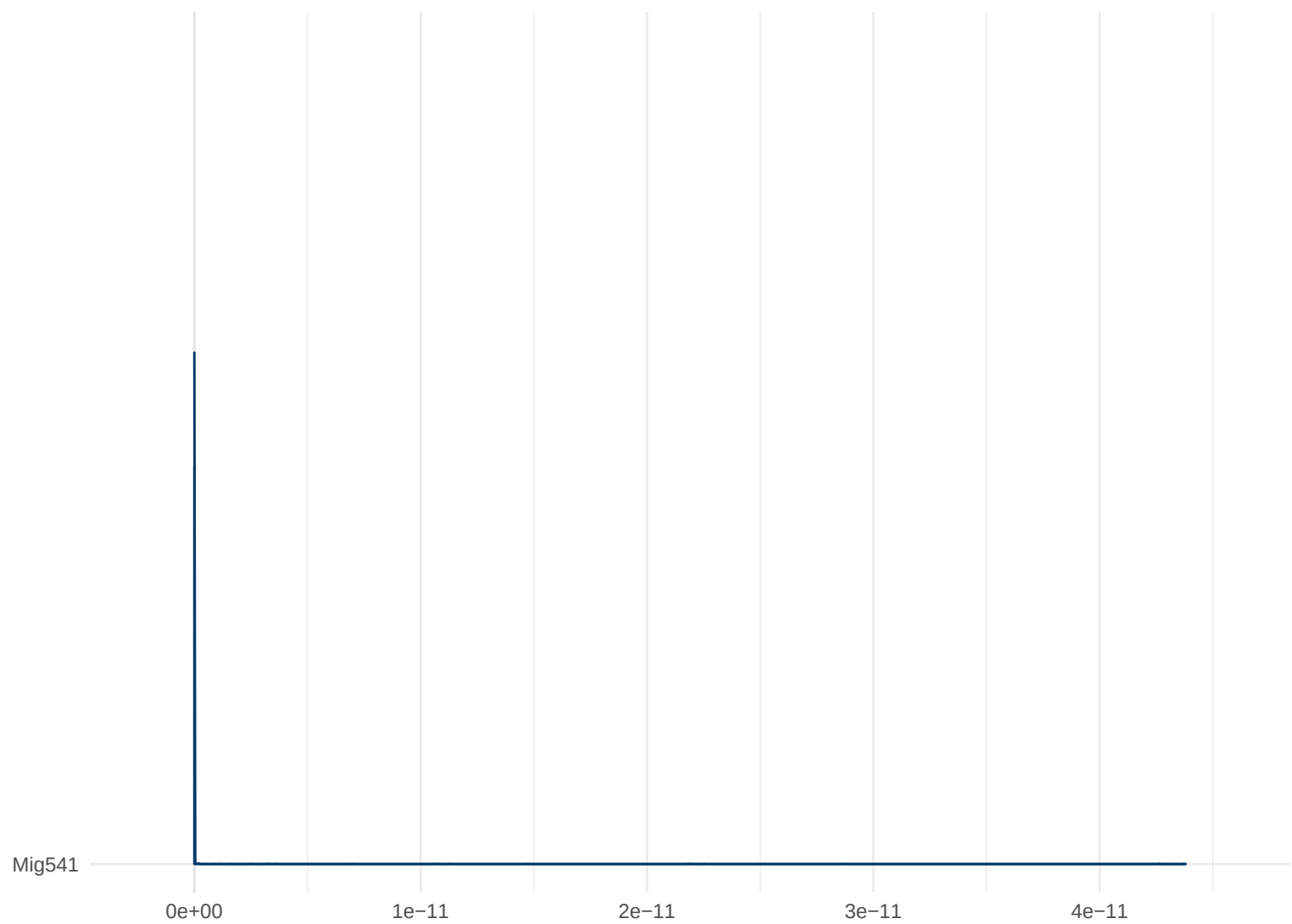
Posterior Density: Mig541
