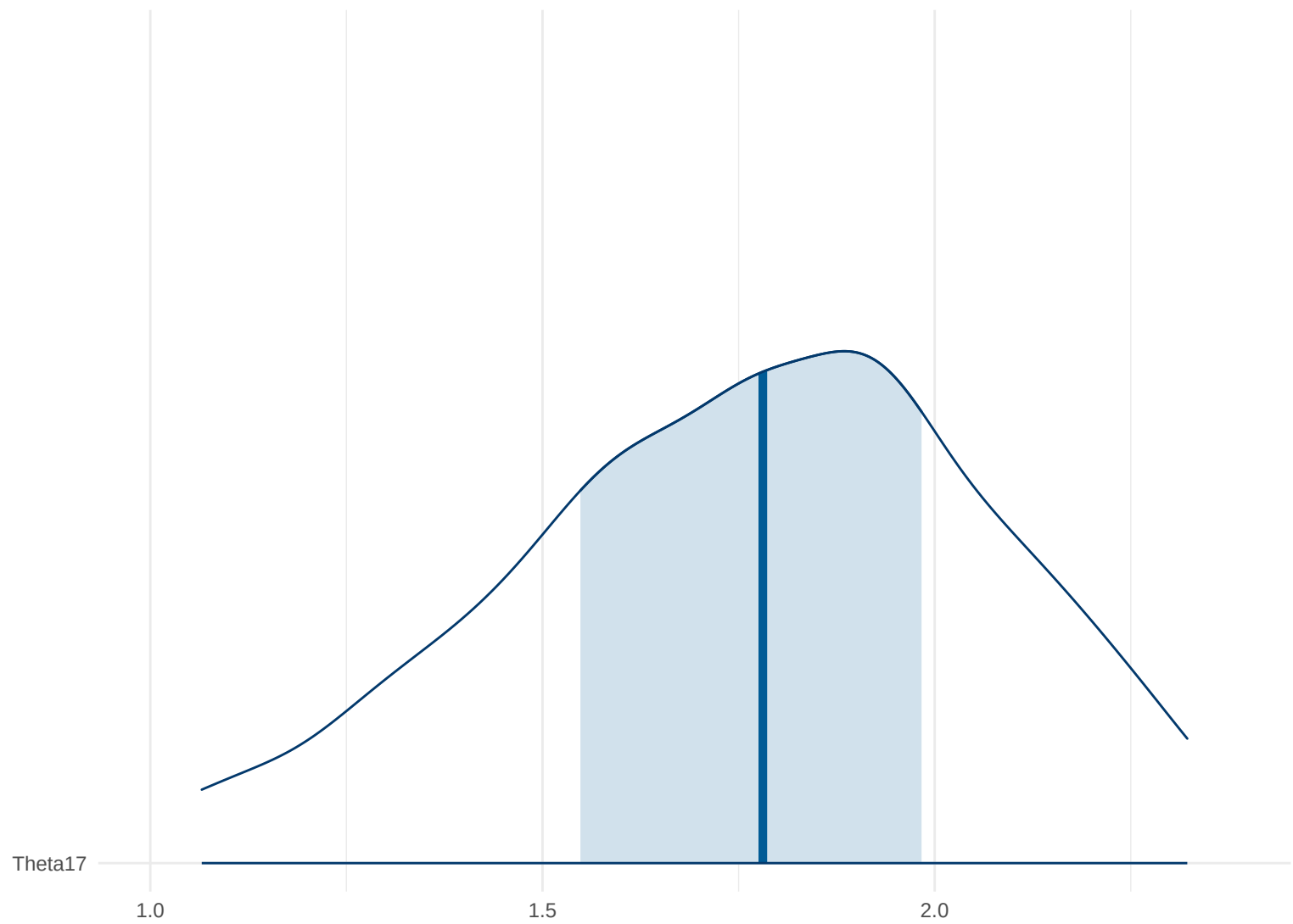
Posterior Density: Theta17
