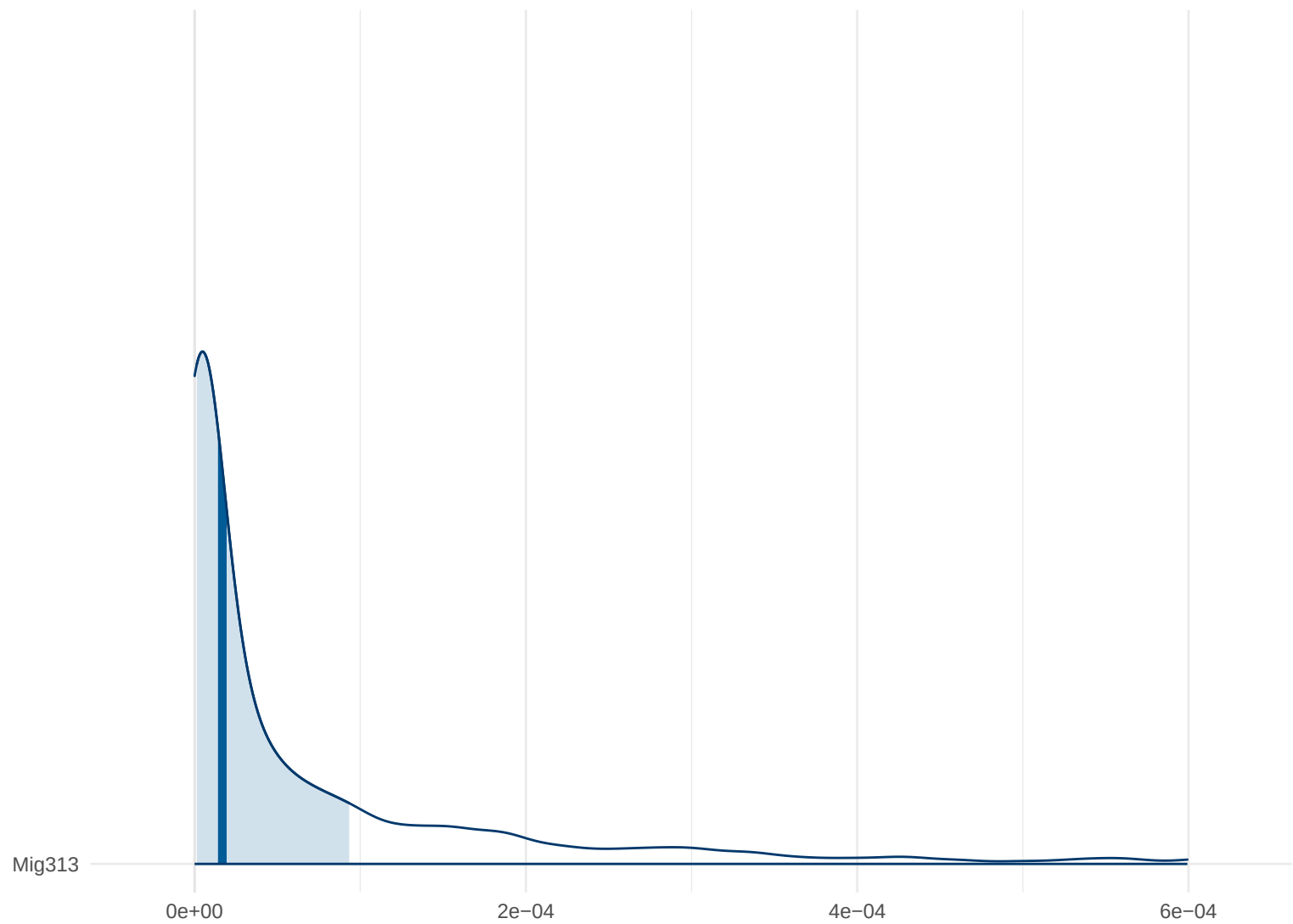
Posterior Density: Mig313
