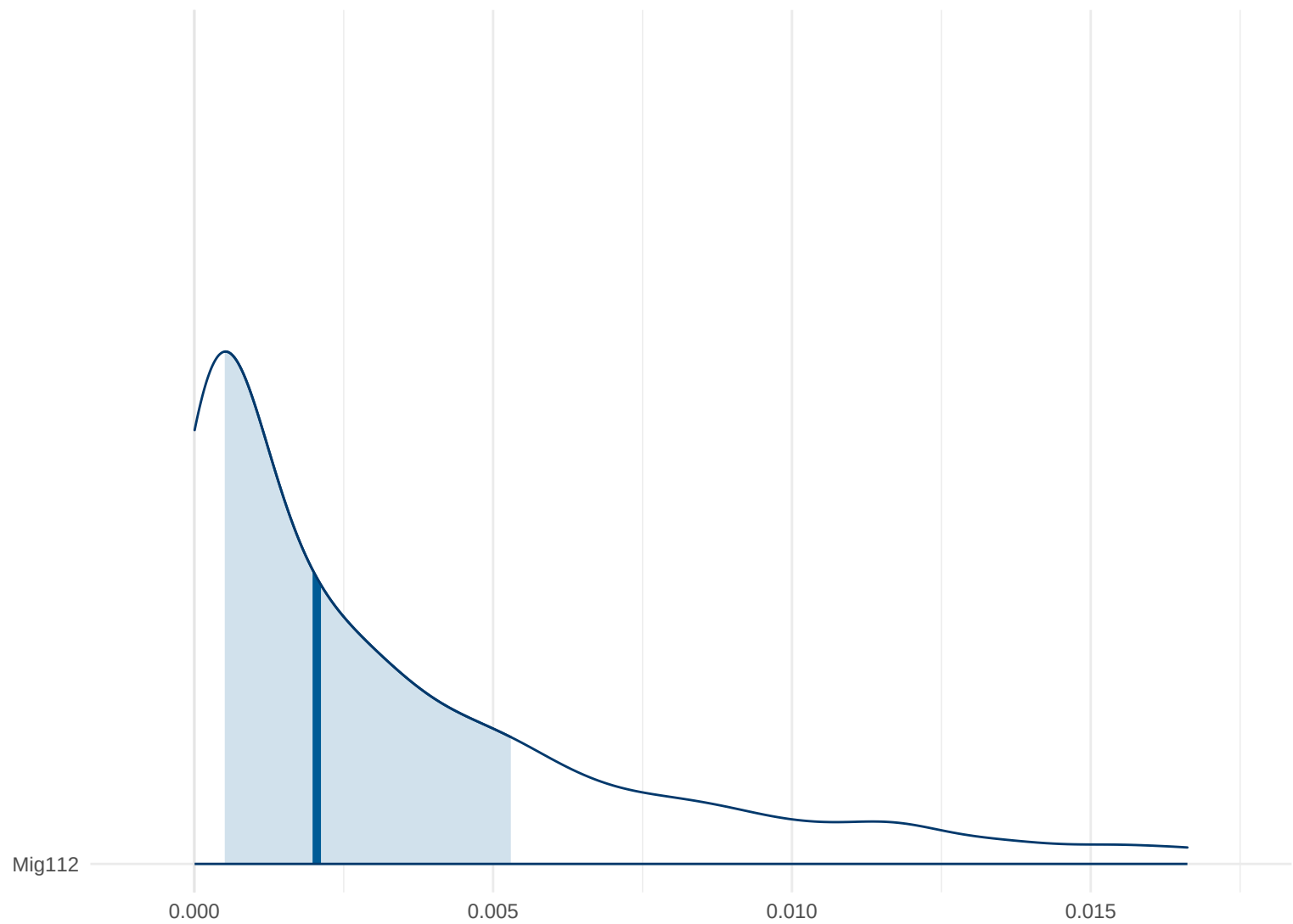
Posterior Density: Mig112
