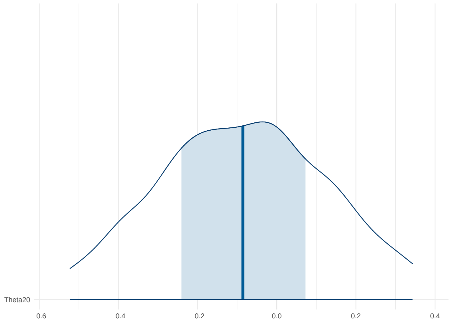
Posterior Density: Theta20
