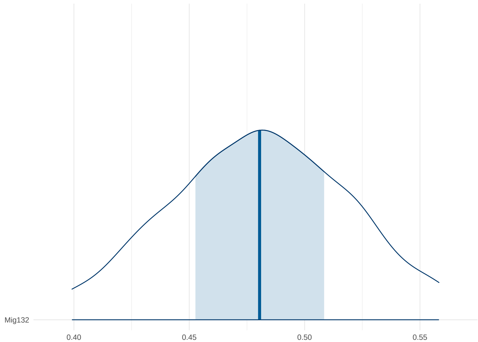
Posterior Density: Mig132
