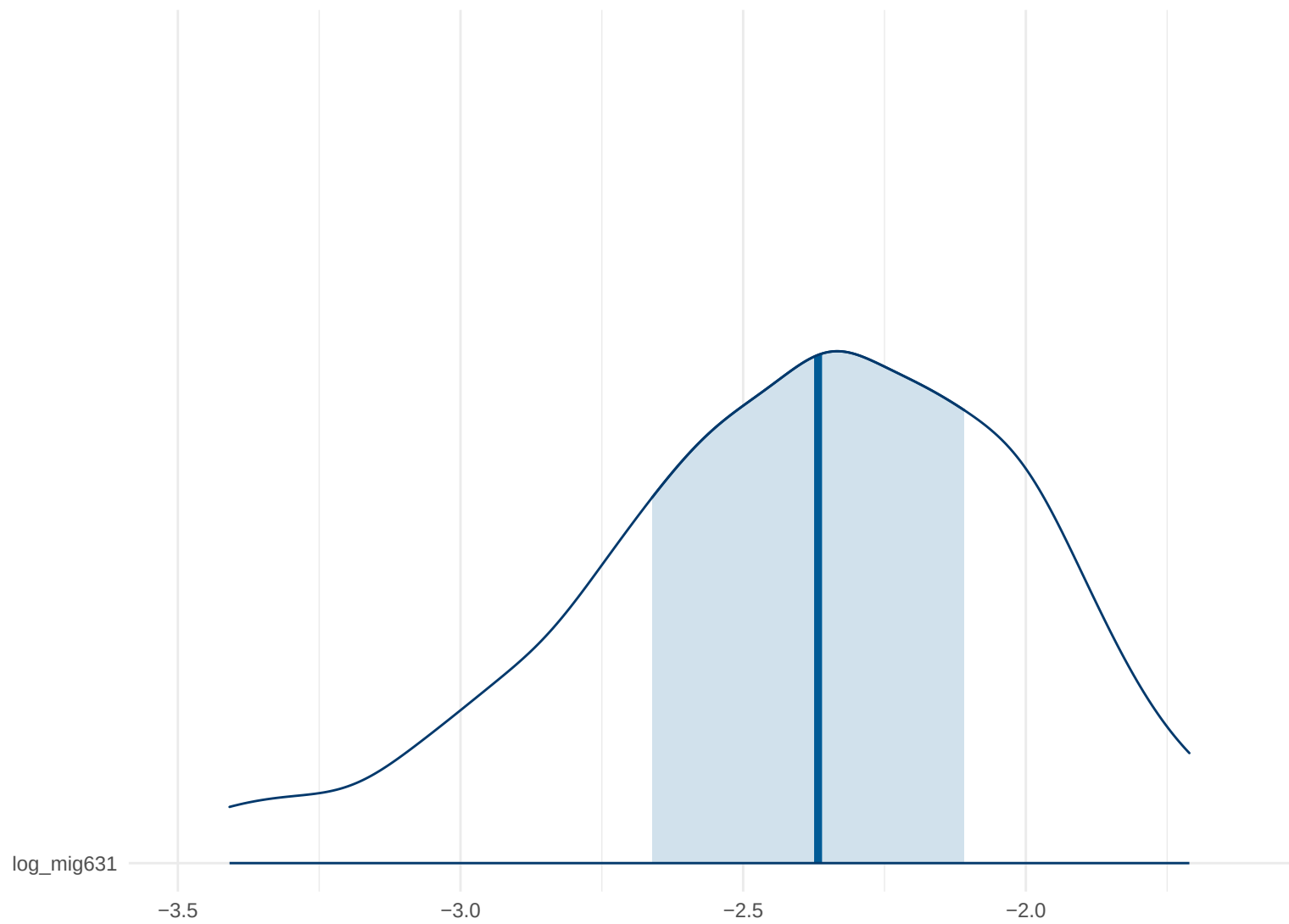
Posterior Density: log_mig631
