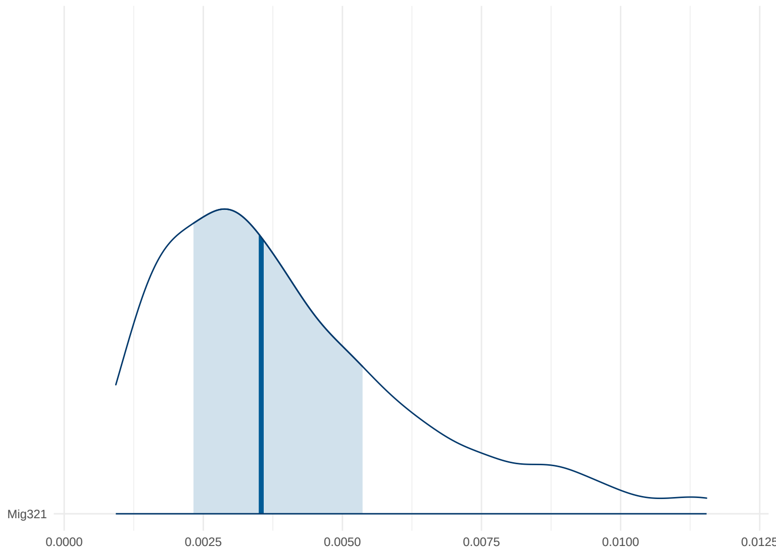
Posterior Density: Mig321
