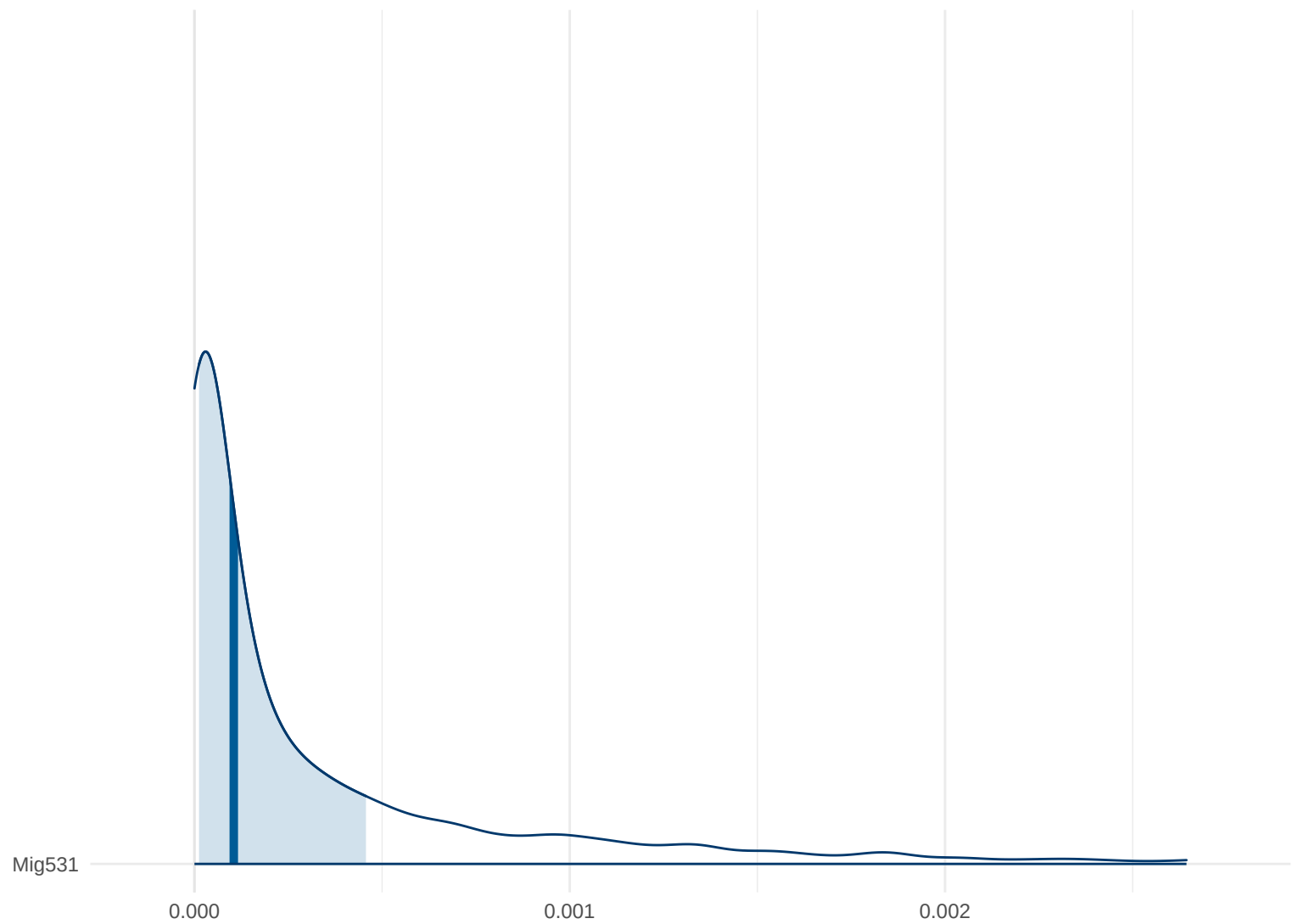
Posterior Density: Mig531
