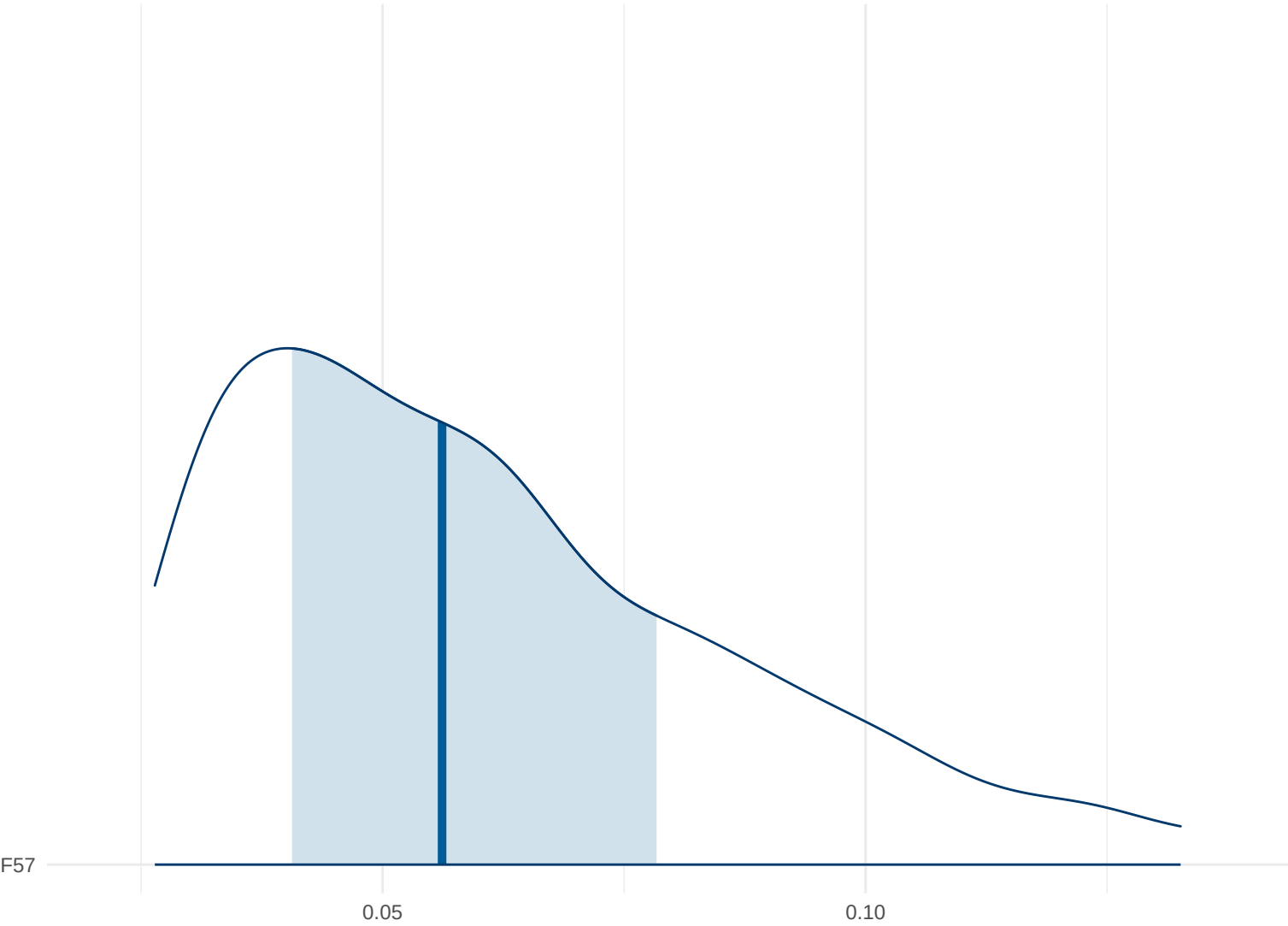
Posterior Density: F57
