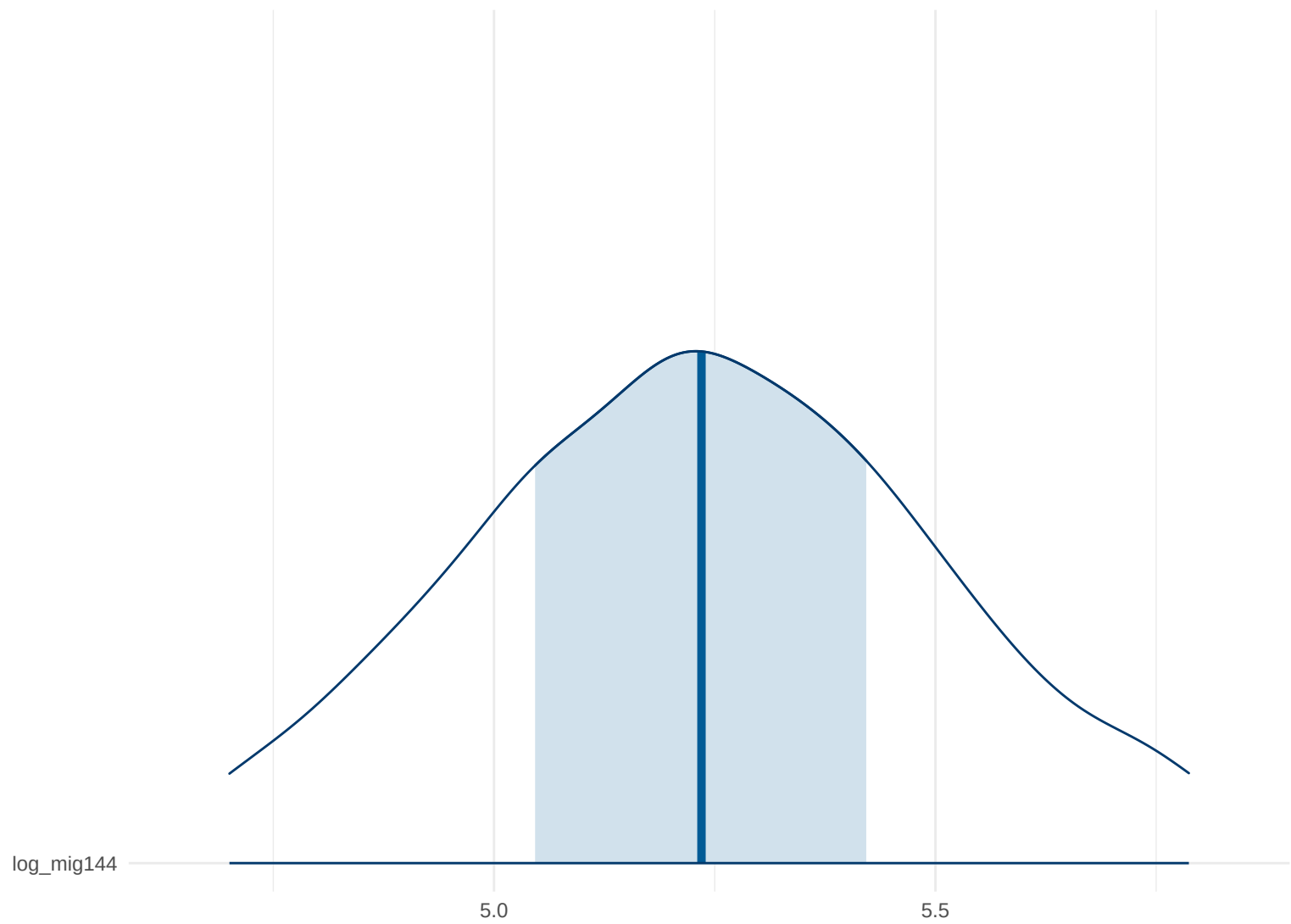
Posterior Density: log_mig144
