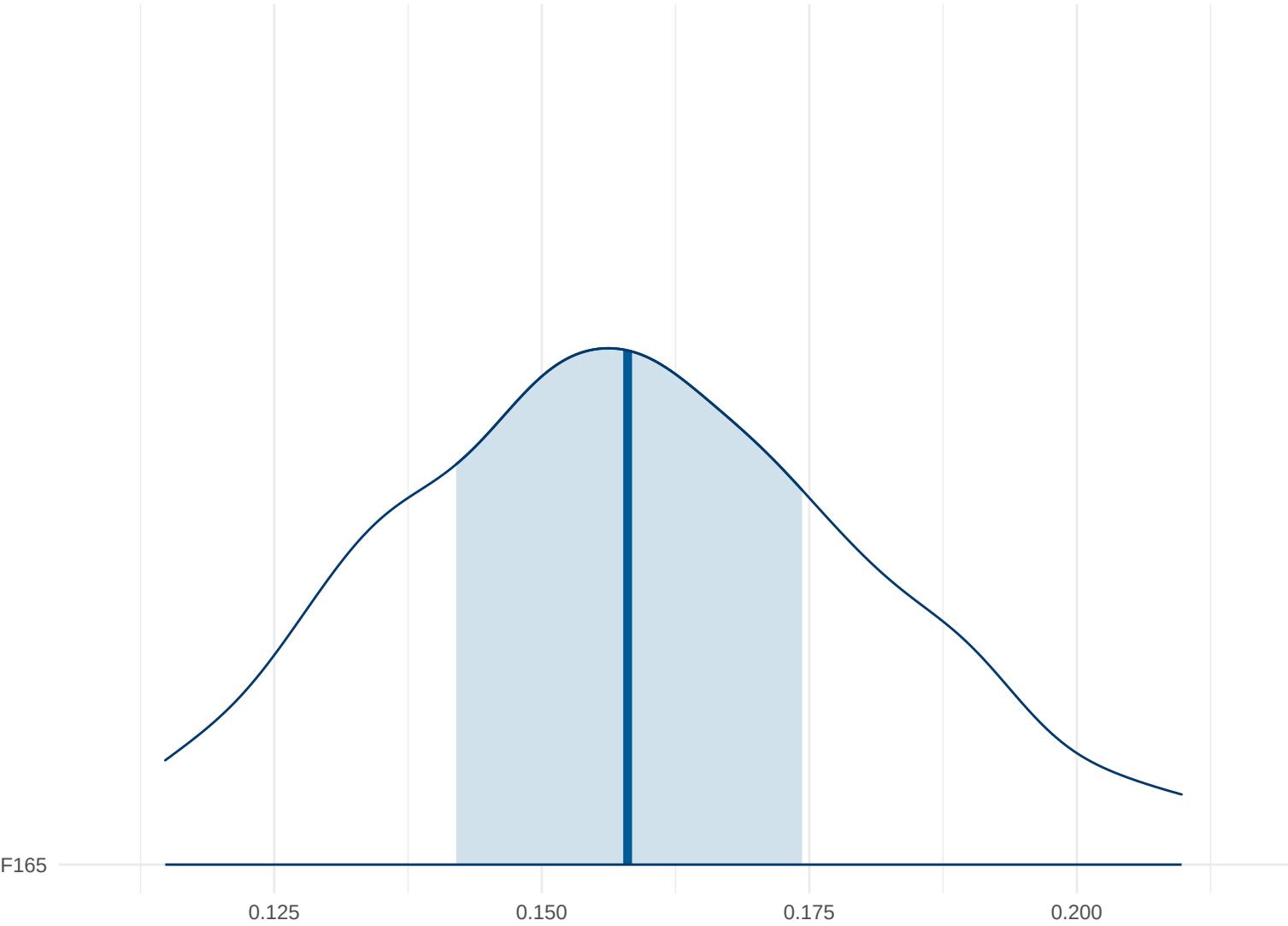
Posterior Density: F165
