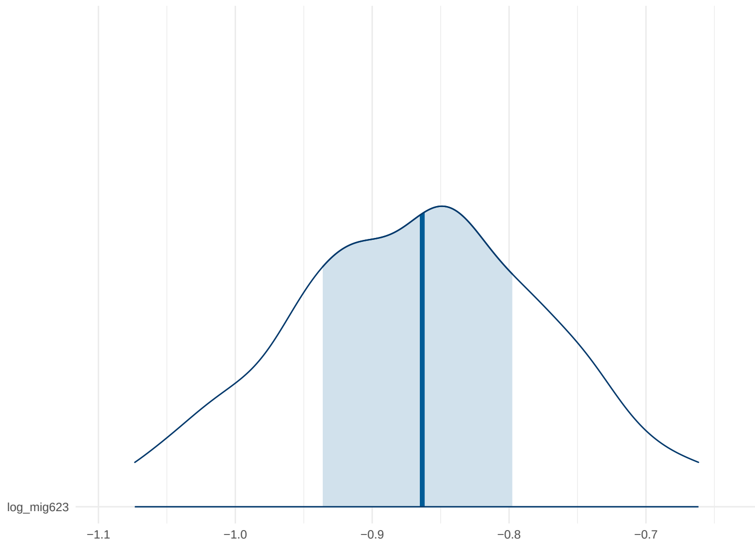
Posterior Density: log_mig623
