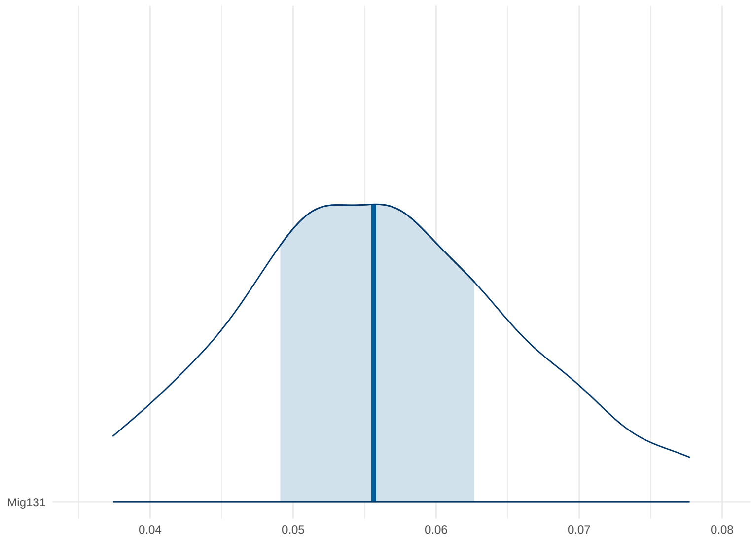
Posterior Density: Mig131
