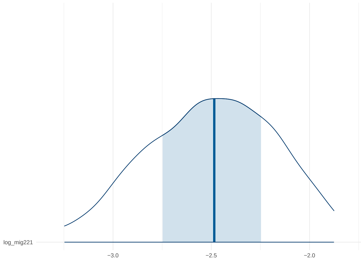
Posterior Density: log_mig221
