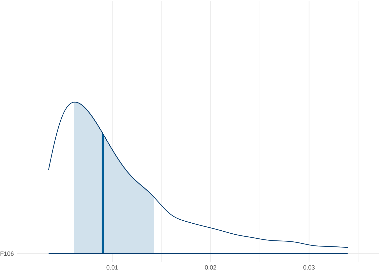
Posterior Density: F106
