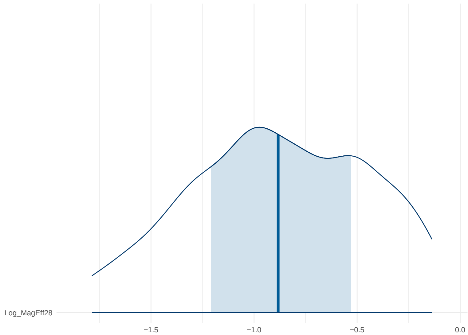
Posterior Density: Log_MagEff28
