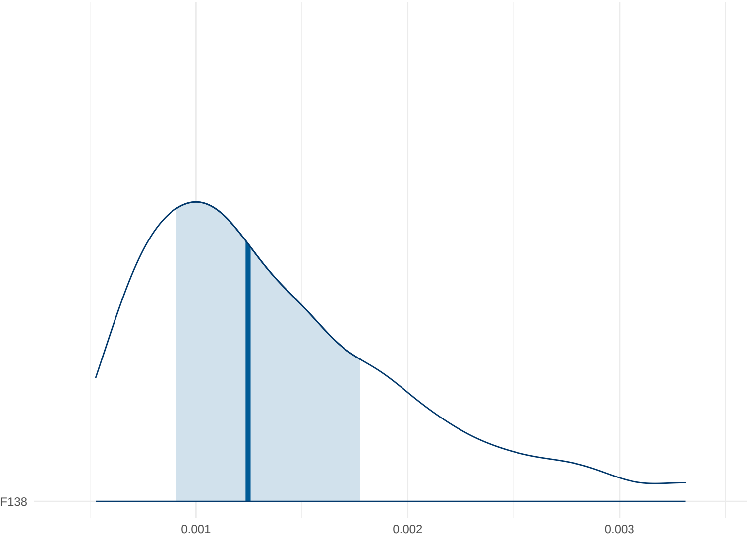
Posterior Density: F138
