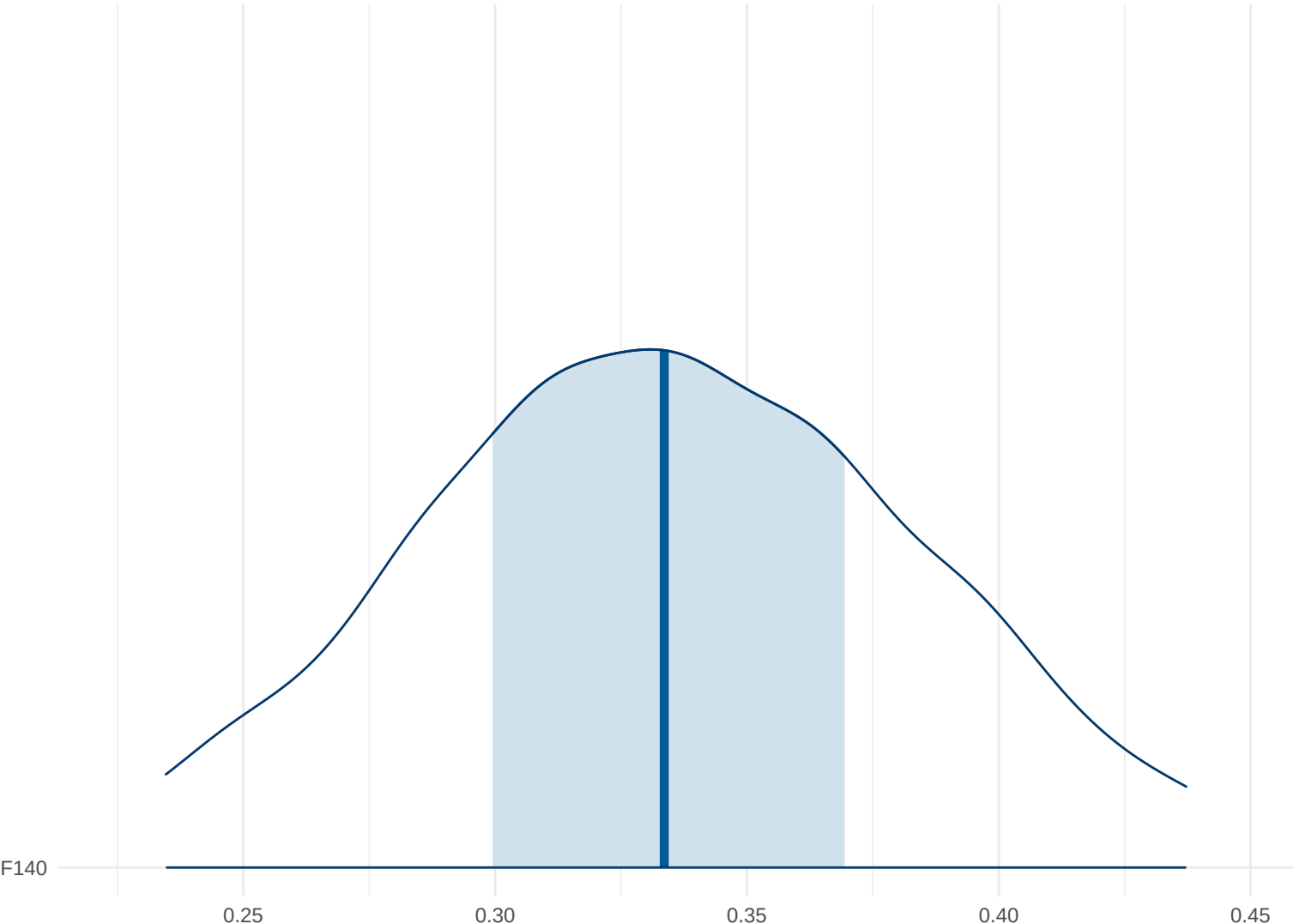
Posterior Density: F140
