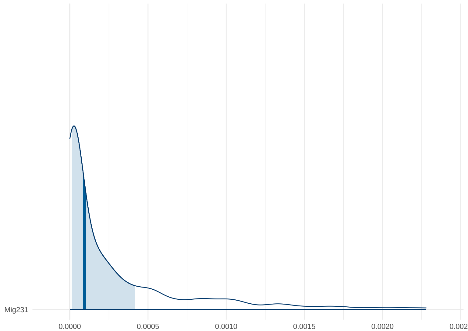
Posterior Density: Mig231
