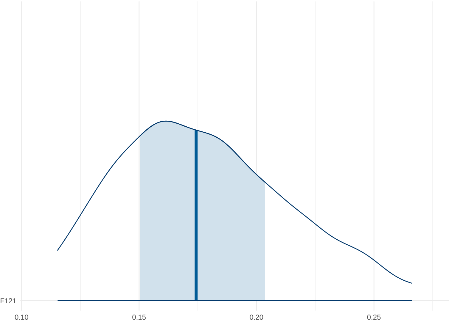
Posterior Density: F121
