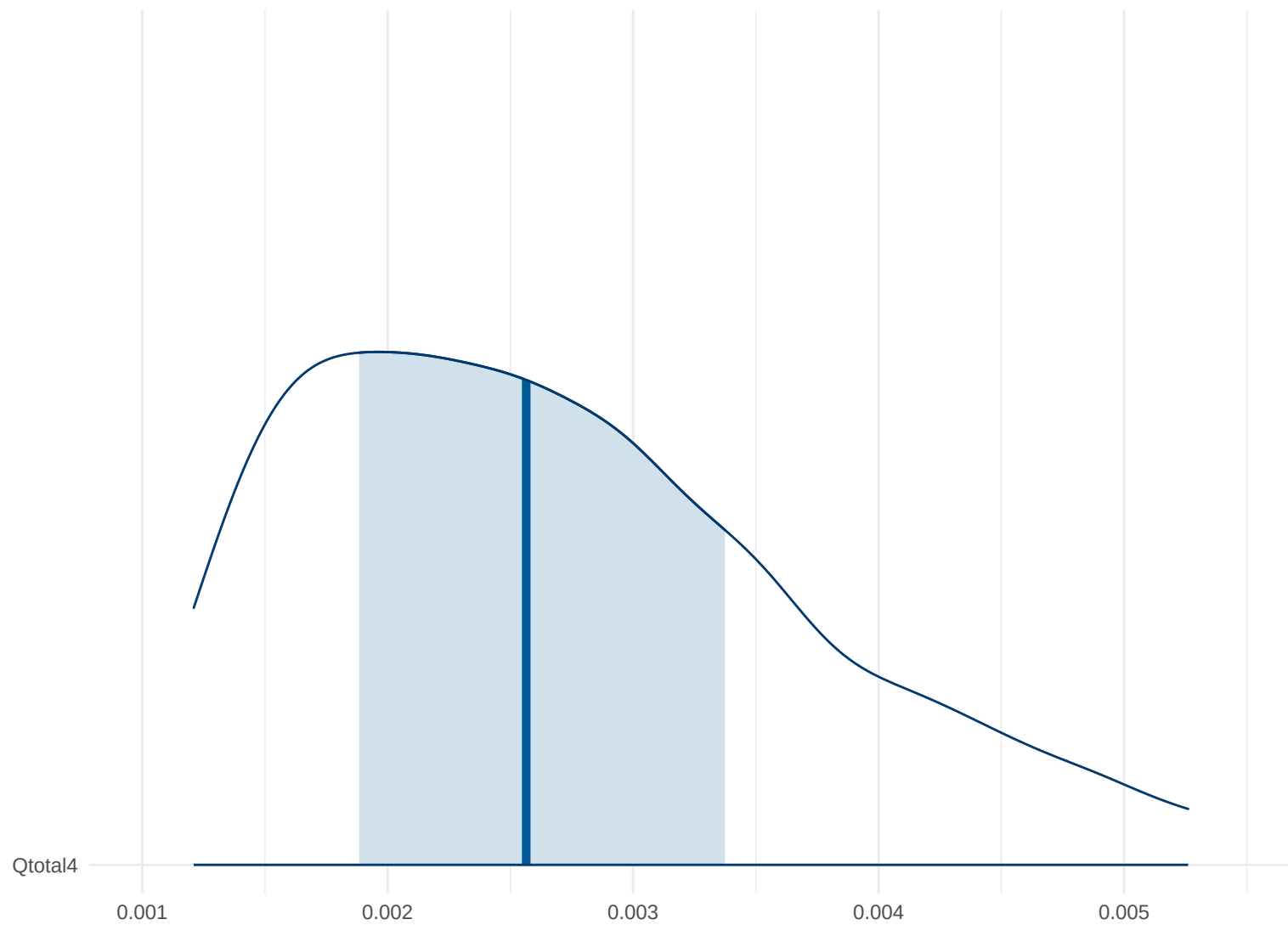
Posterior Density: Qtotal4
