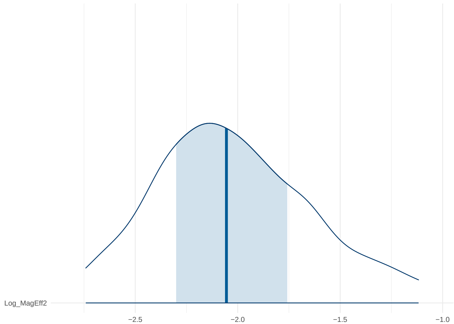
Posterior Density: Log_MagEff2
