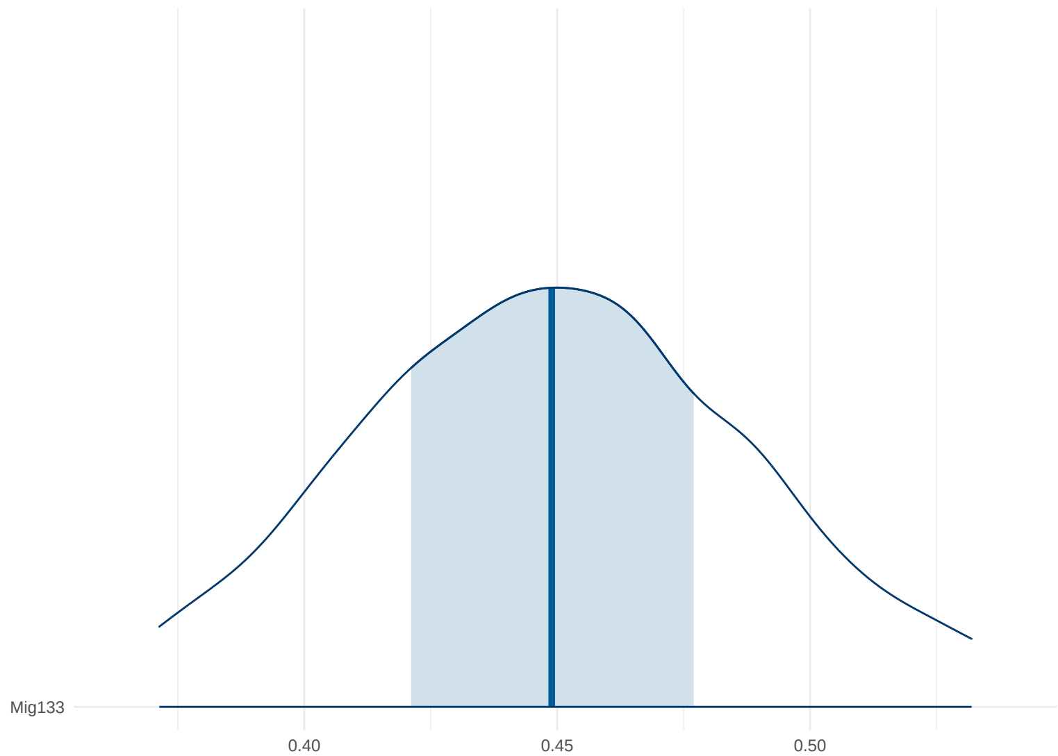
Posterior Density: Mig133
