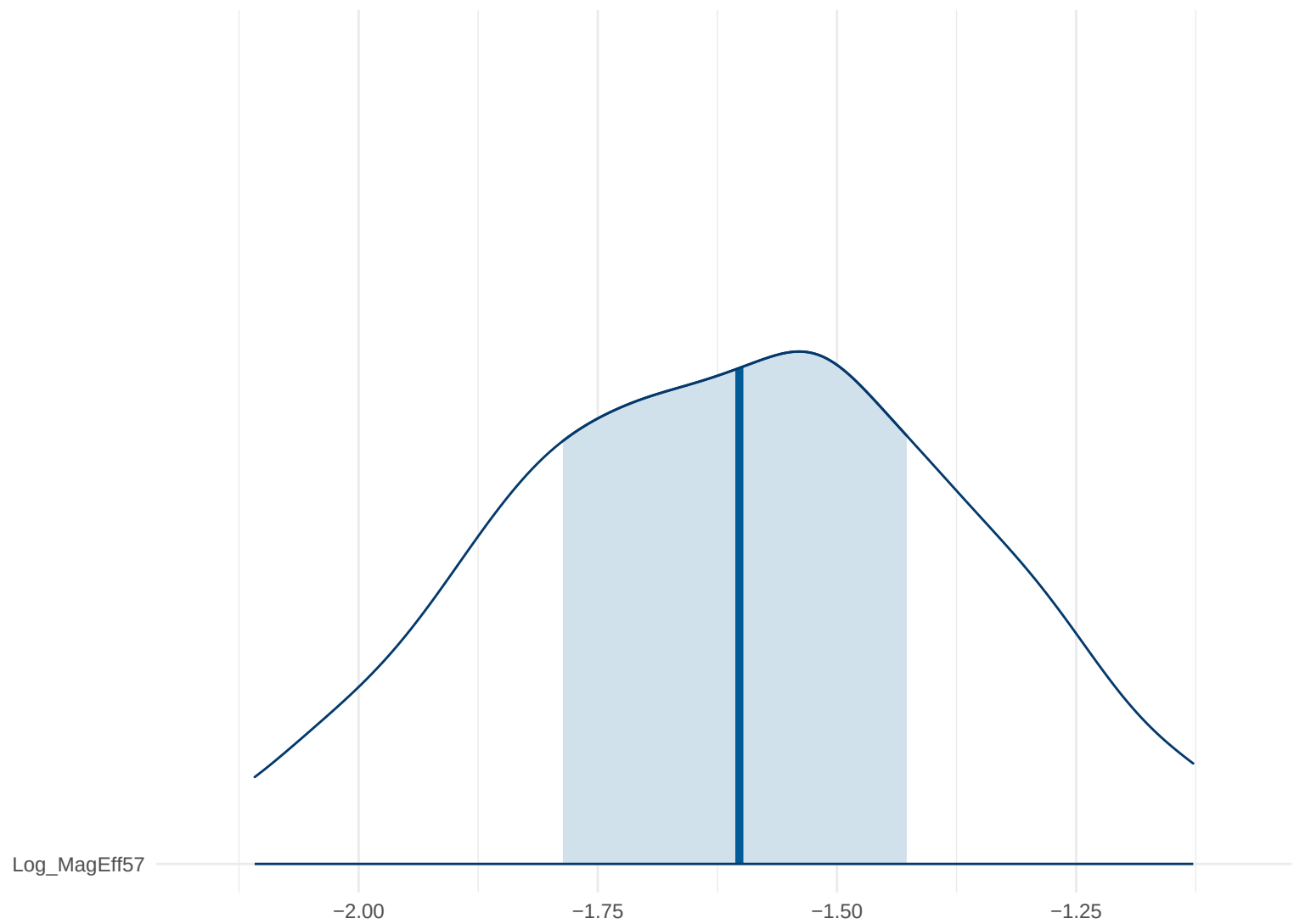
Posterior Density: Log_MagEff57
