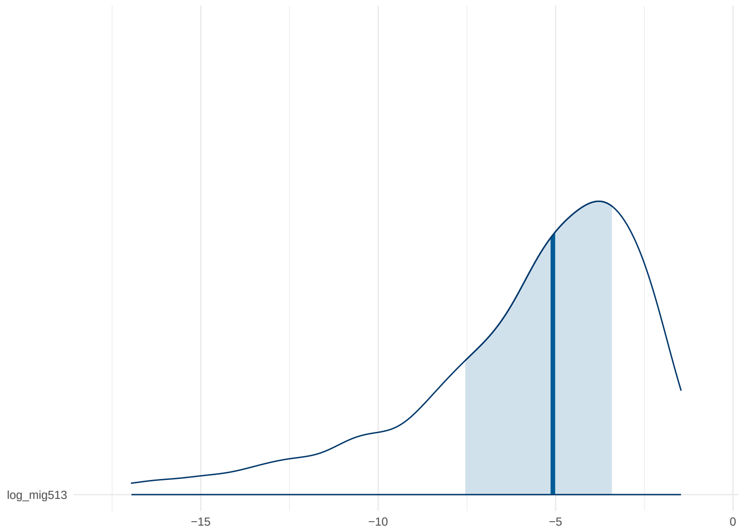
Posterior Density: log_mig513
