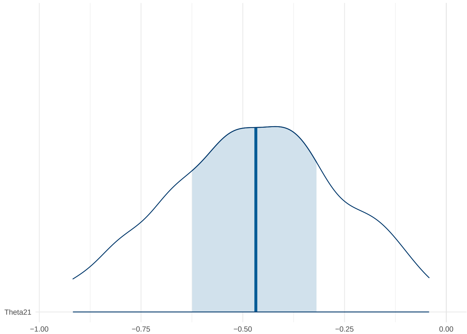
Posterior Density: Theta21
