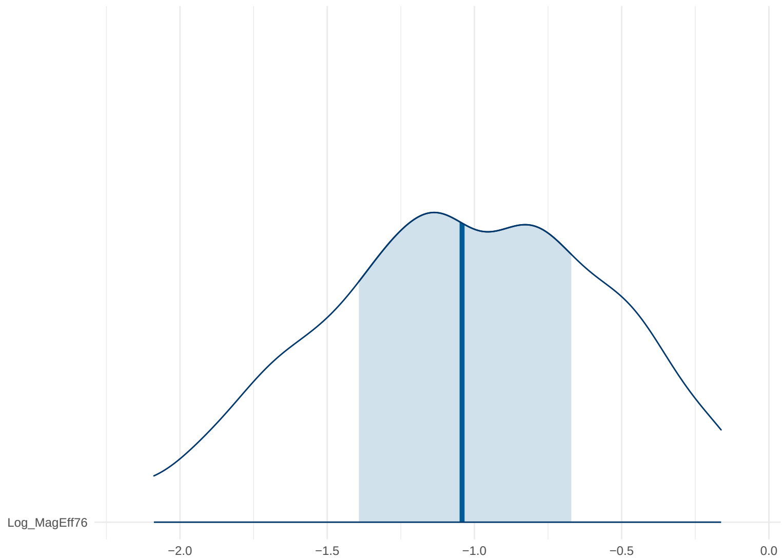
Posterior Density: Log_MagEff76
