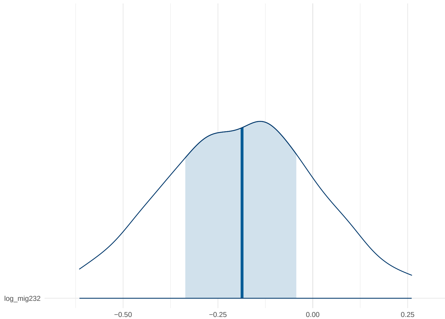
Posterior Density: log_mig232
