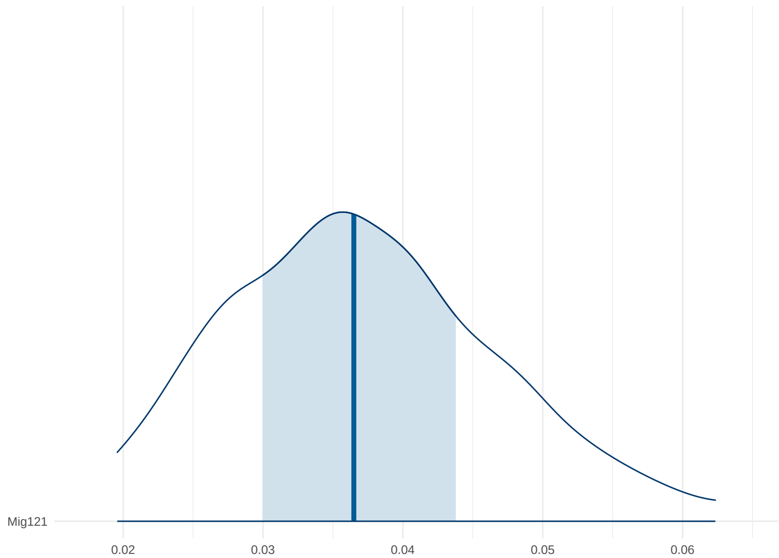
Posterior Density: Mig121
