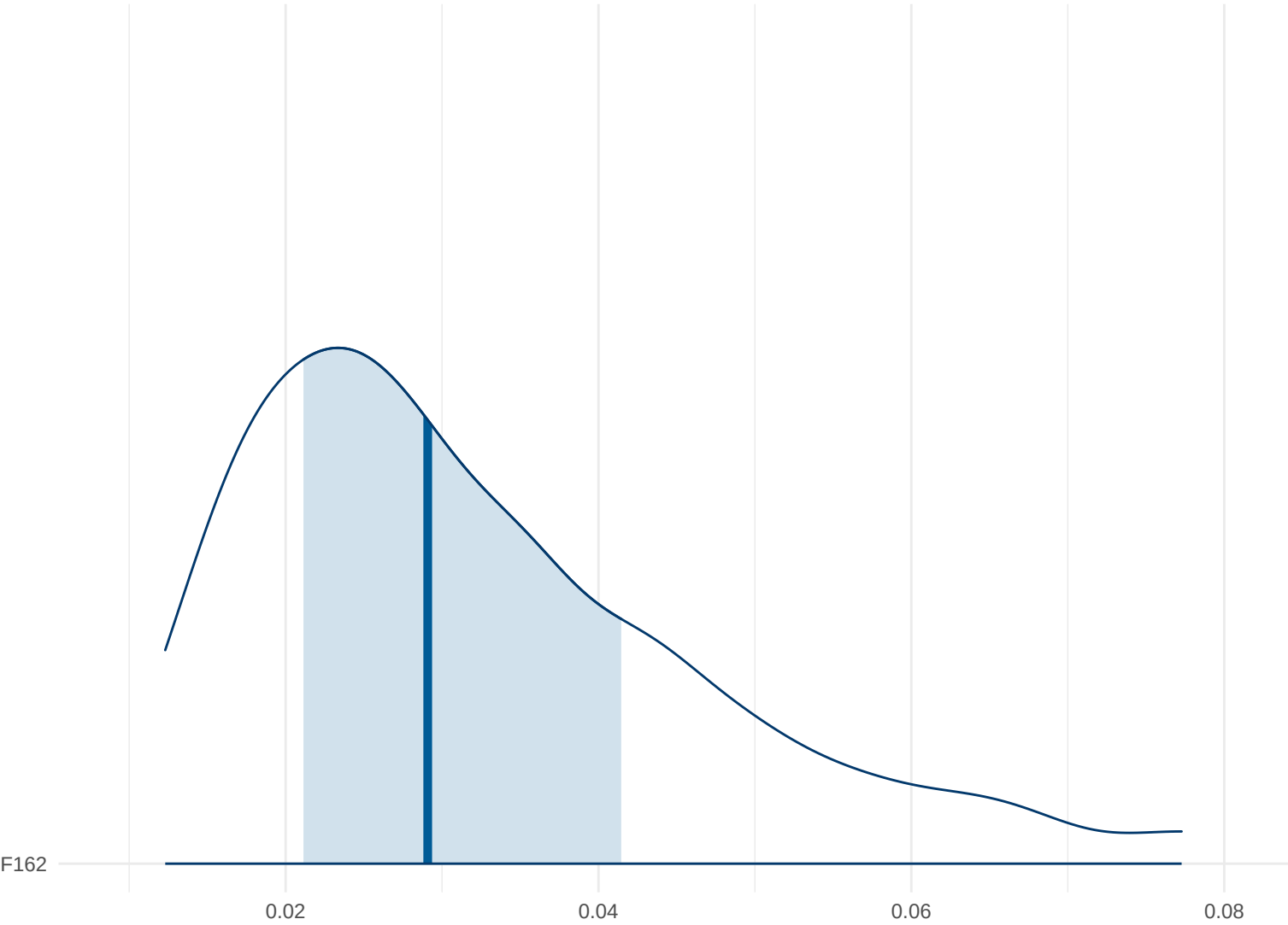
Posterior Density: F162
