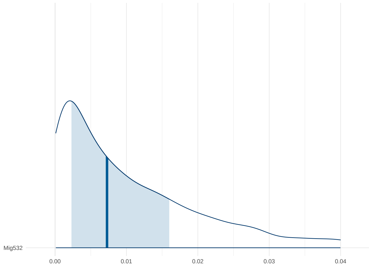
Posterior Density: Mig532
