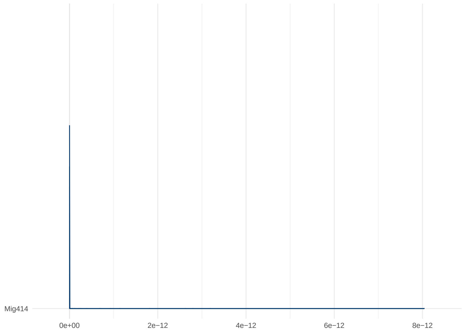
Posterior Density: Mig414
