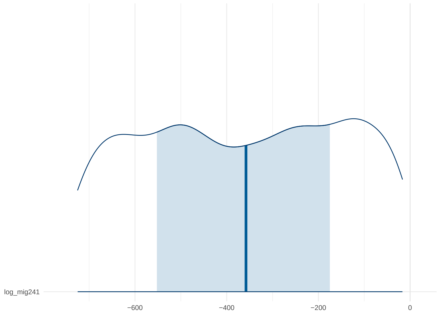
Posterior Density: log_mig241
