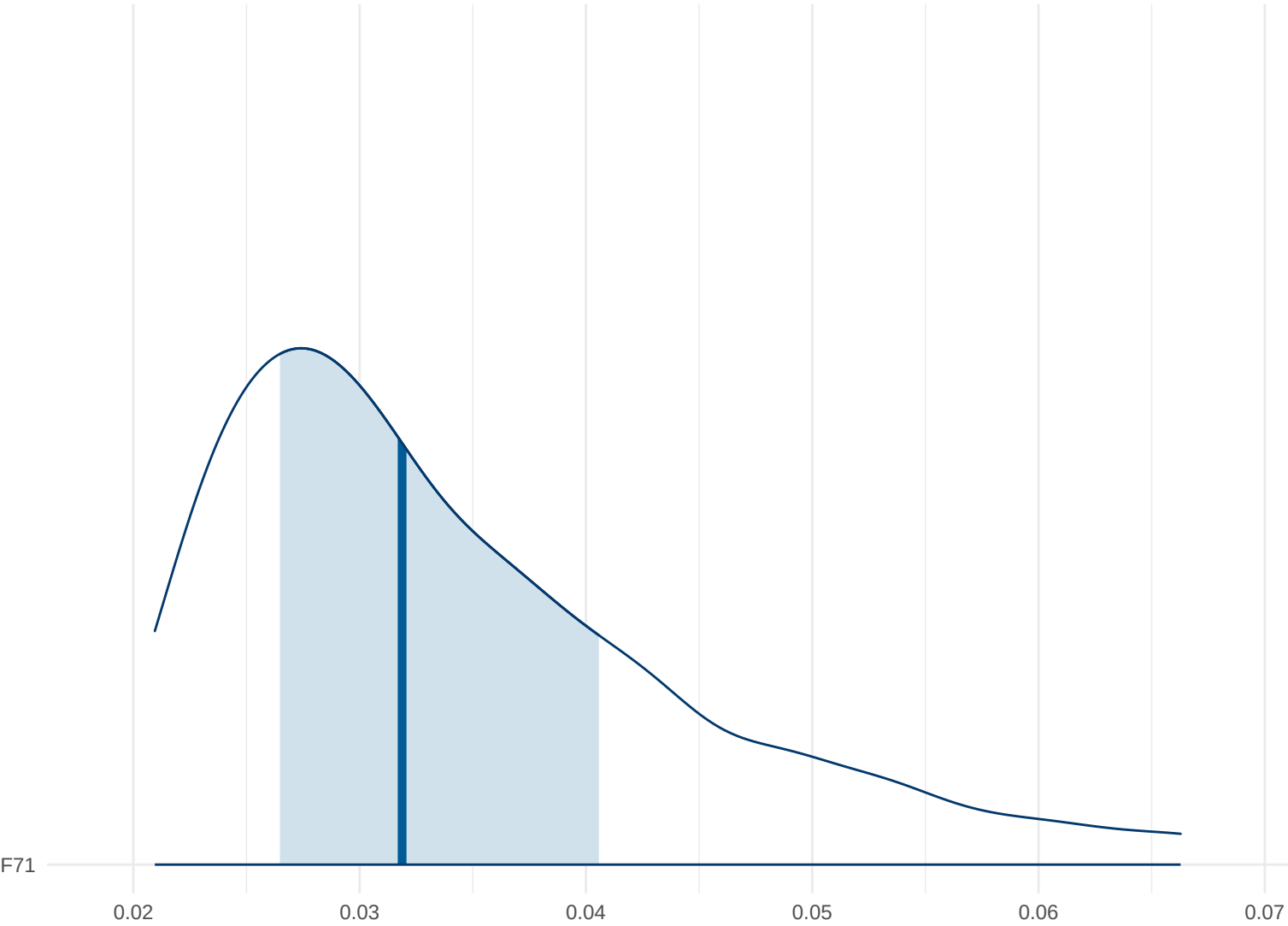
Posterior Density: F71
