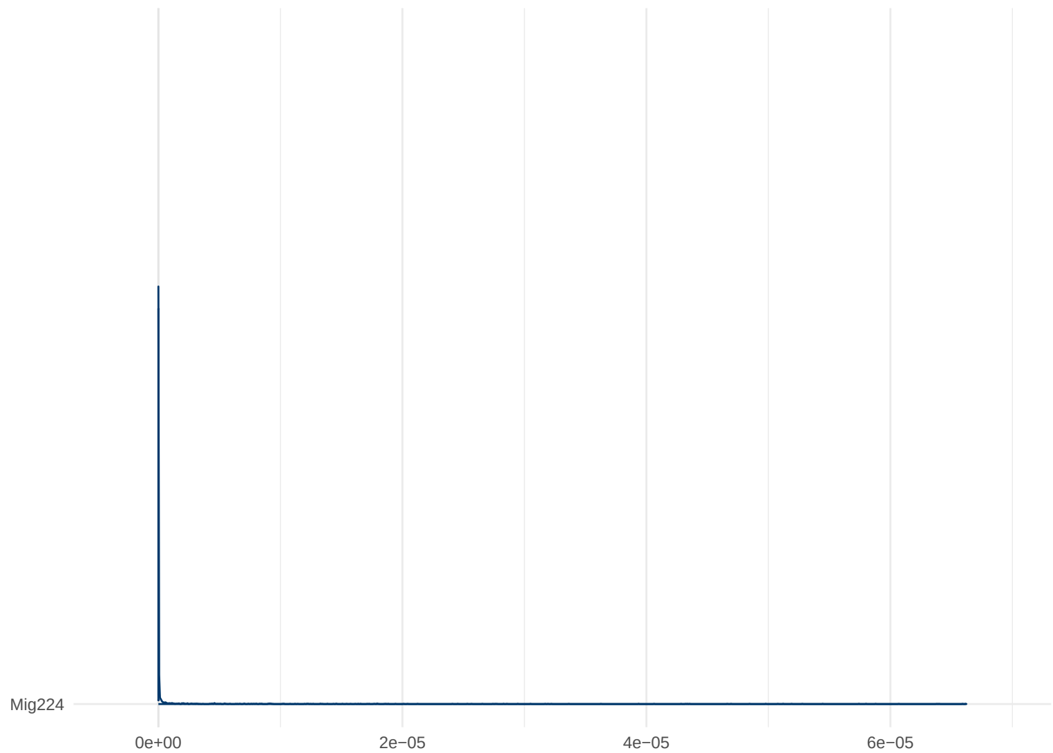
Posterior Density: Mig224
