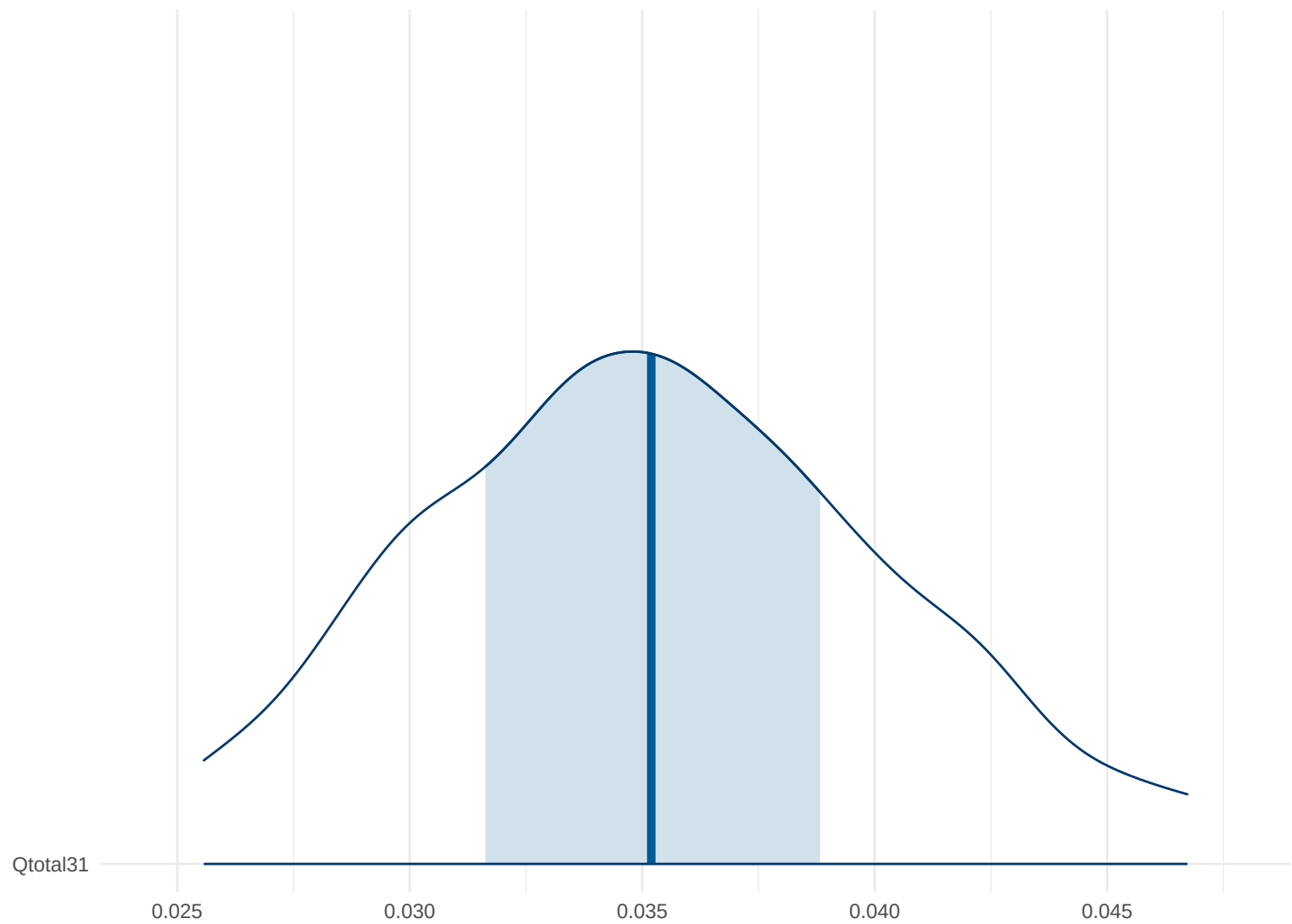
Posterior Density: Qtotal31
