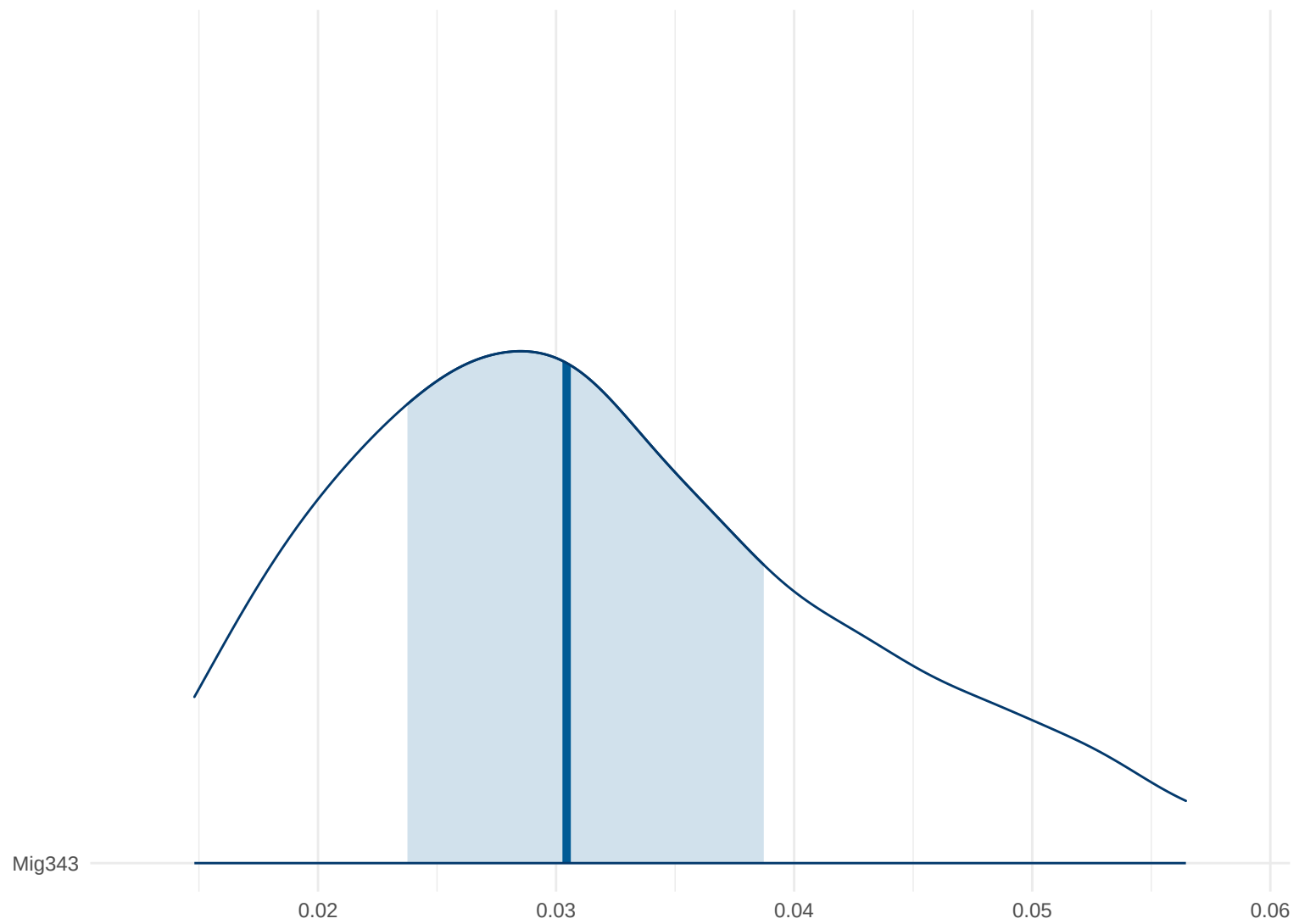
Posterior Density: Mig343
