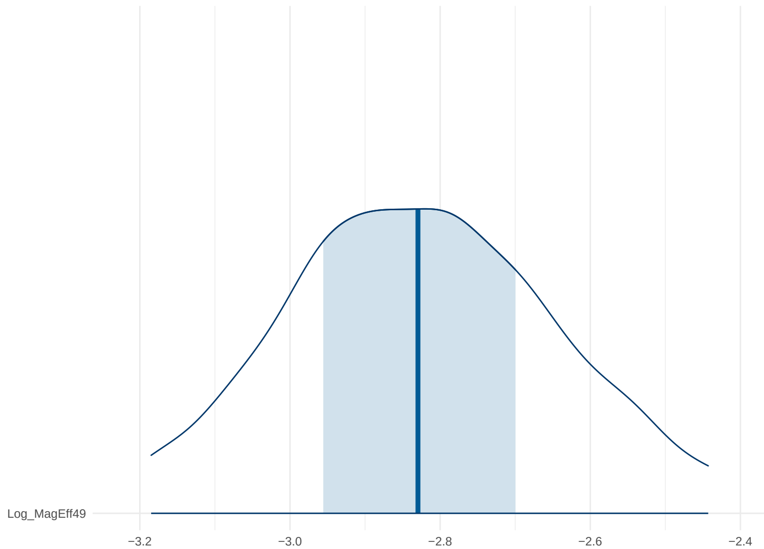
Posterior Density: Log_MagEff49
