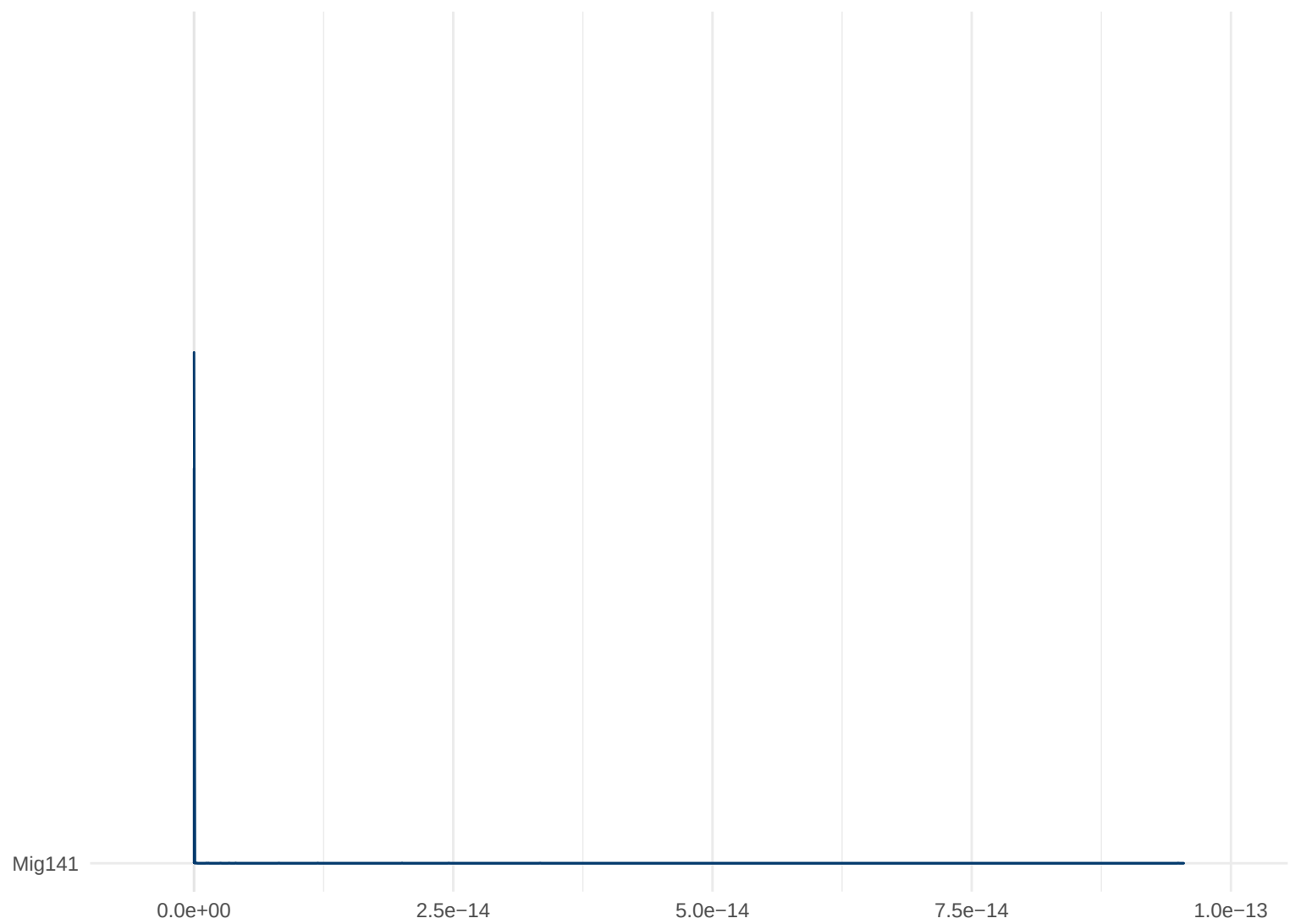
Posterior Density: Mig141
