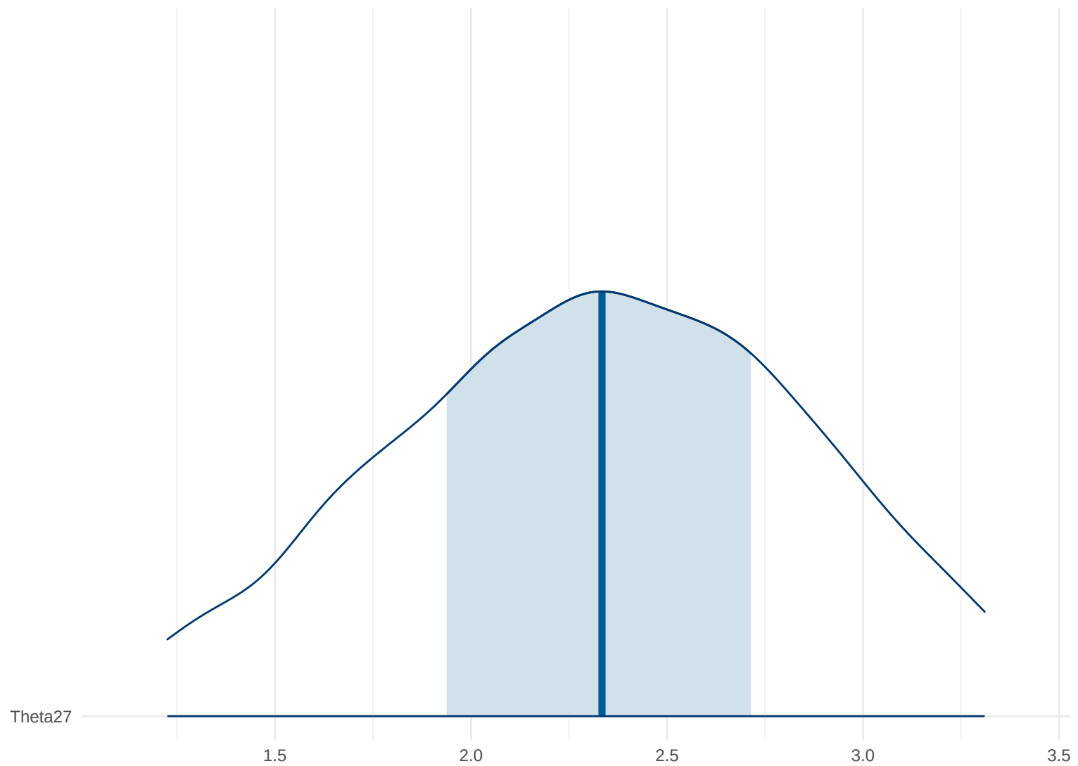
Posterior Density: Theta27
