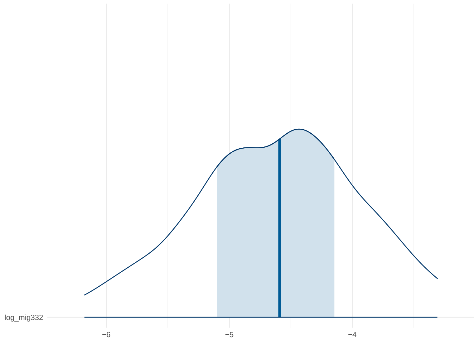
Posterior Density: log_mig332
