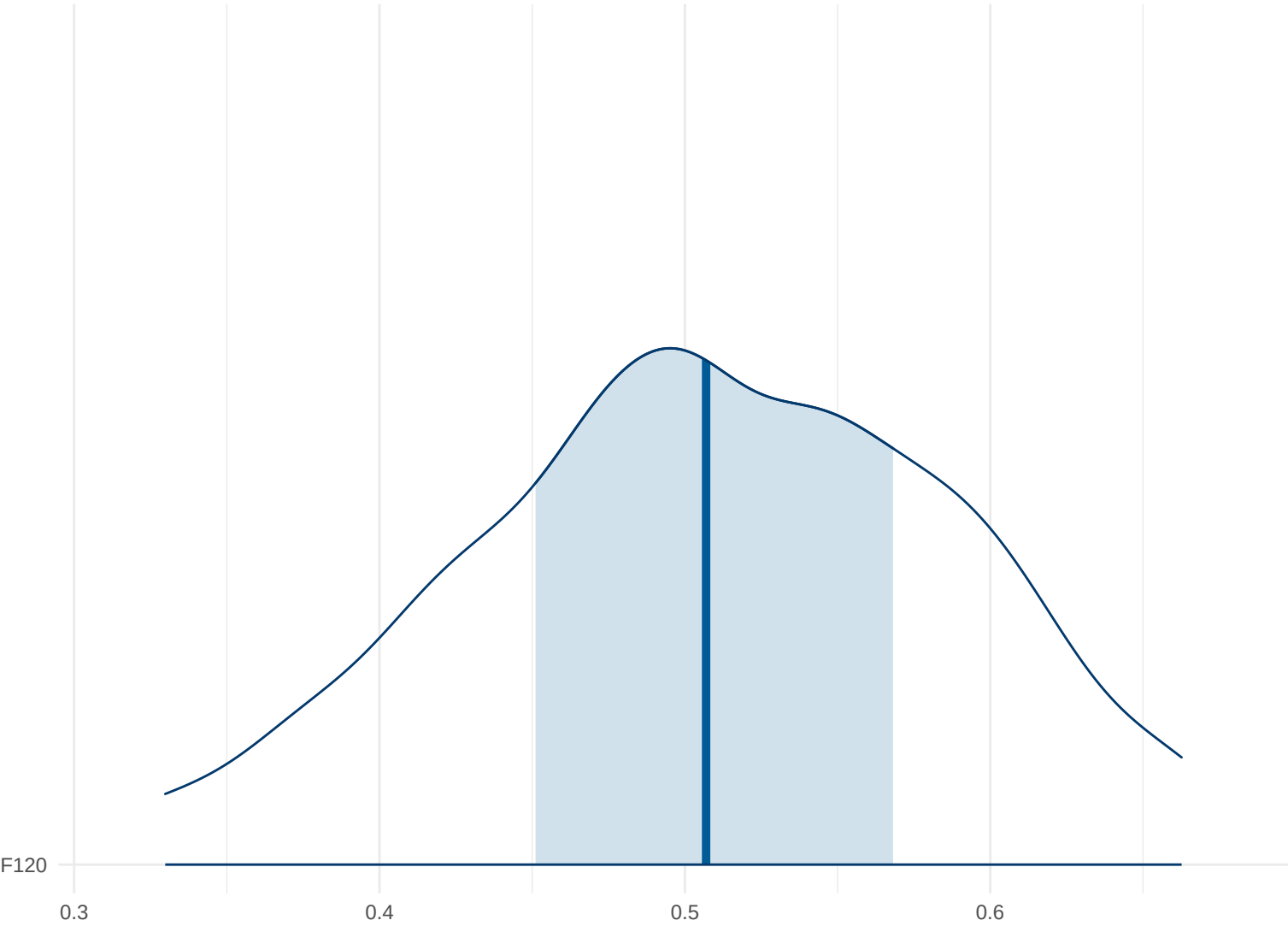
Posterior Density: F120
