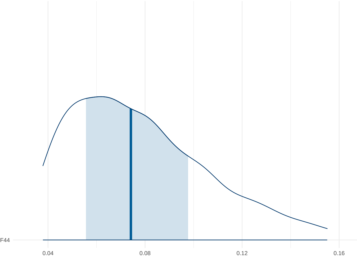
Posterior Density: F44
