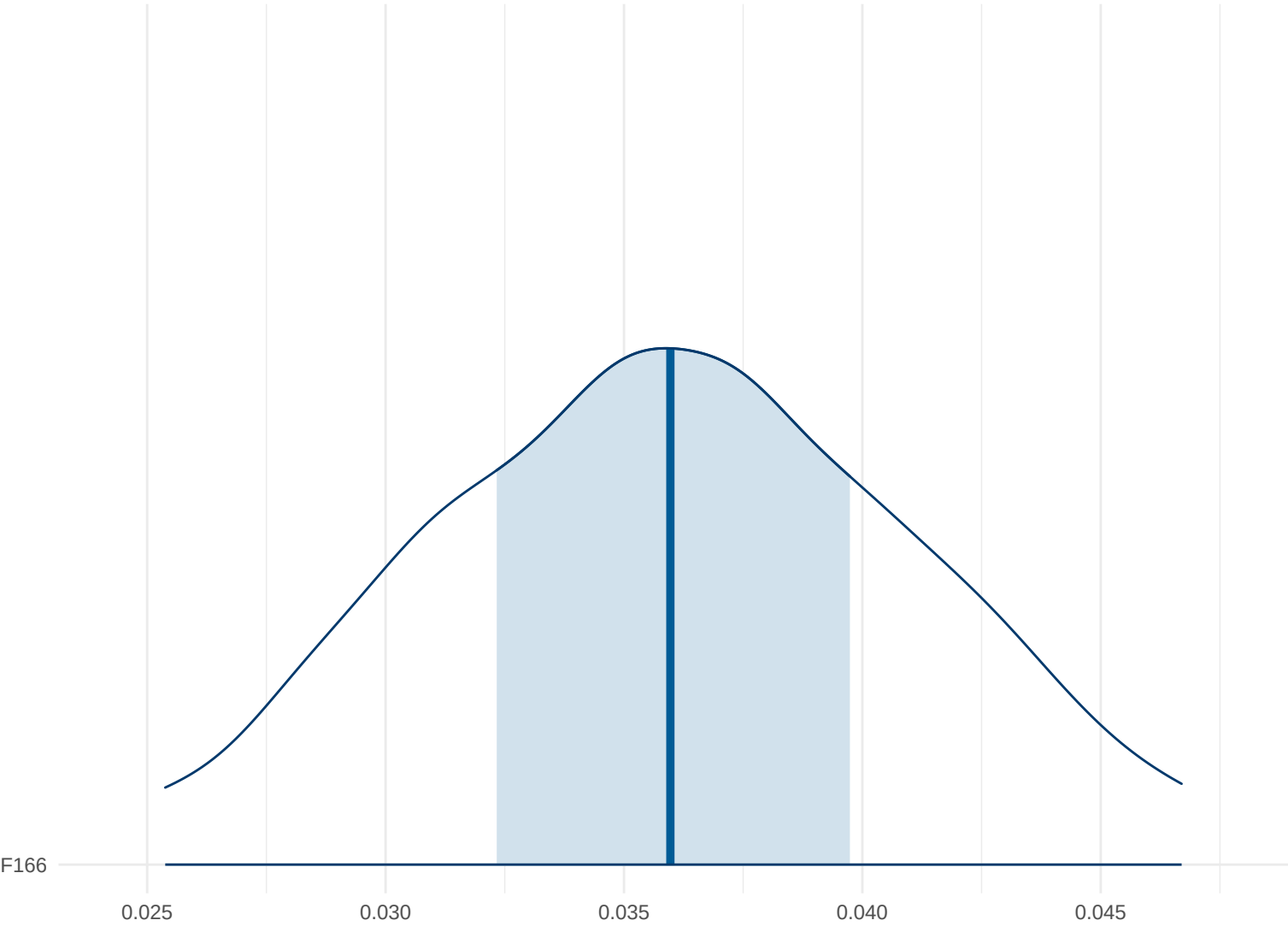
Posterior Density: F166
