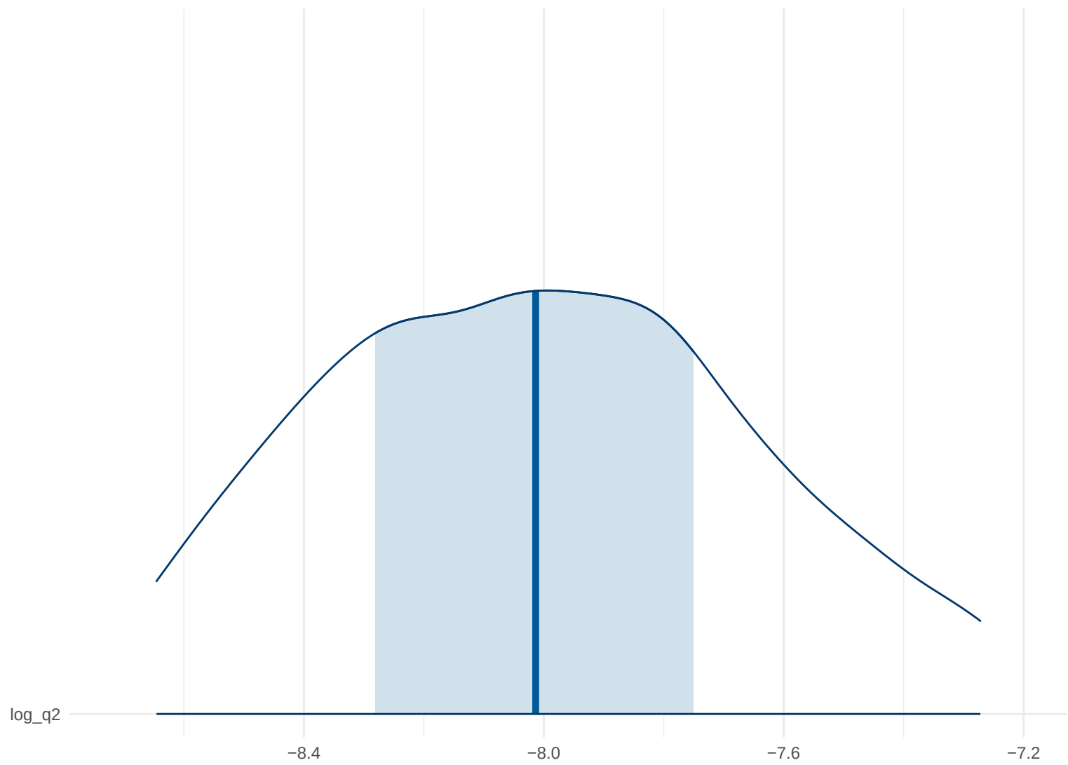
Posterior Density: \log\_q2
