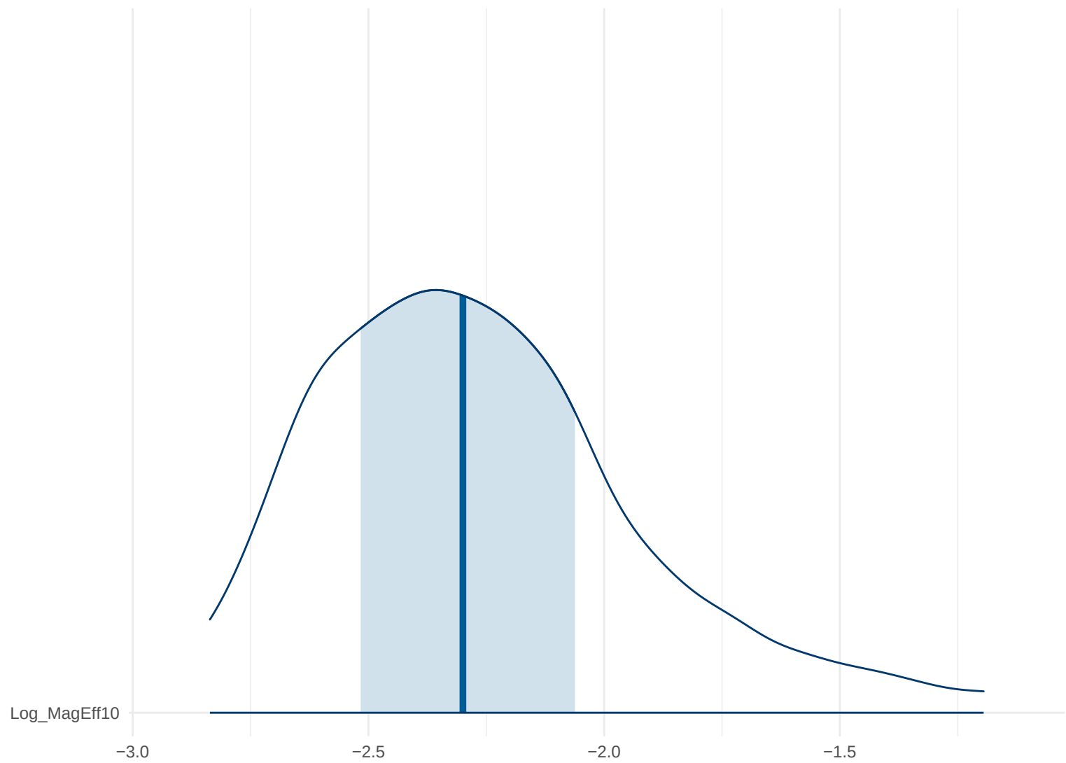
Posterior Density: Log_MagEff10
