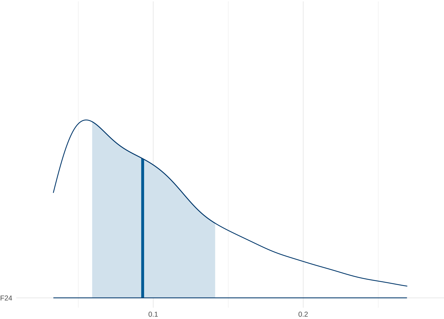
Posterior Density: F24
