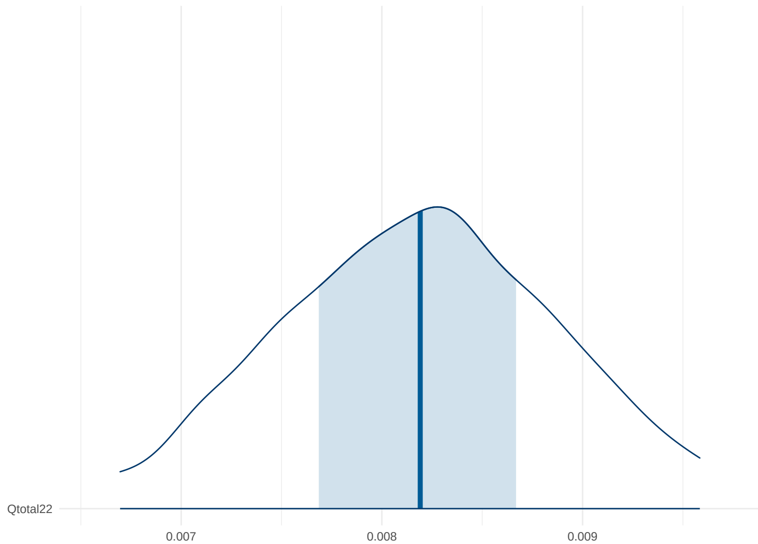
Posterior Density: Qtotal22
