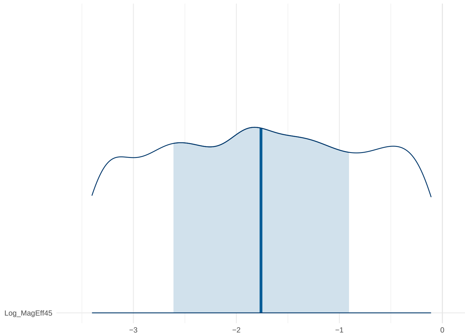
Posterior Density: Log_MagEff45
