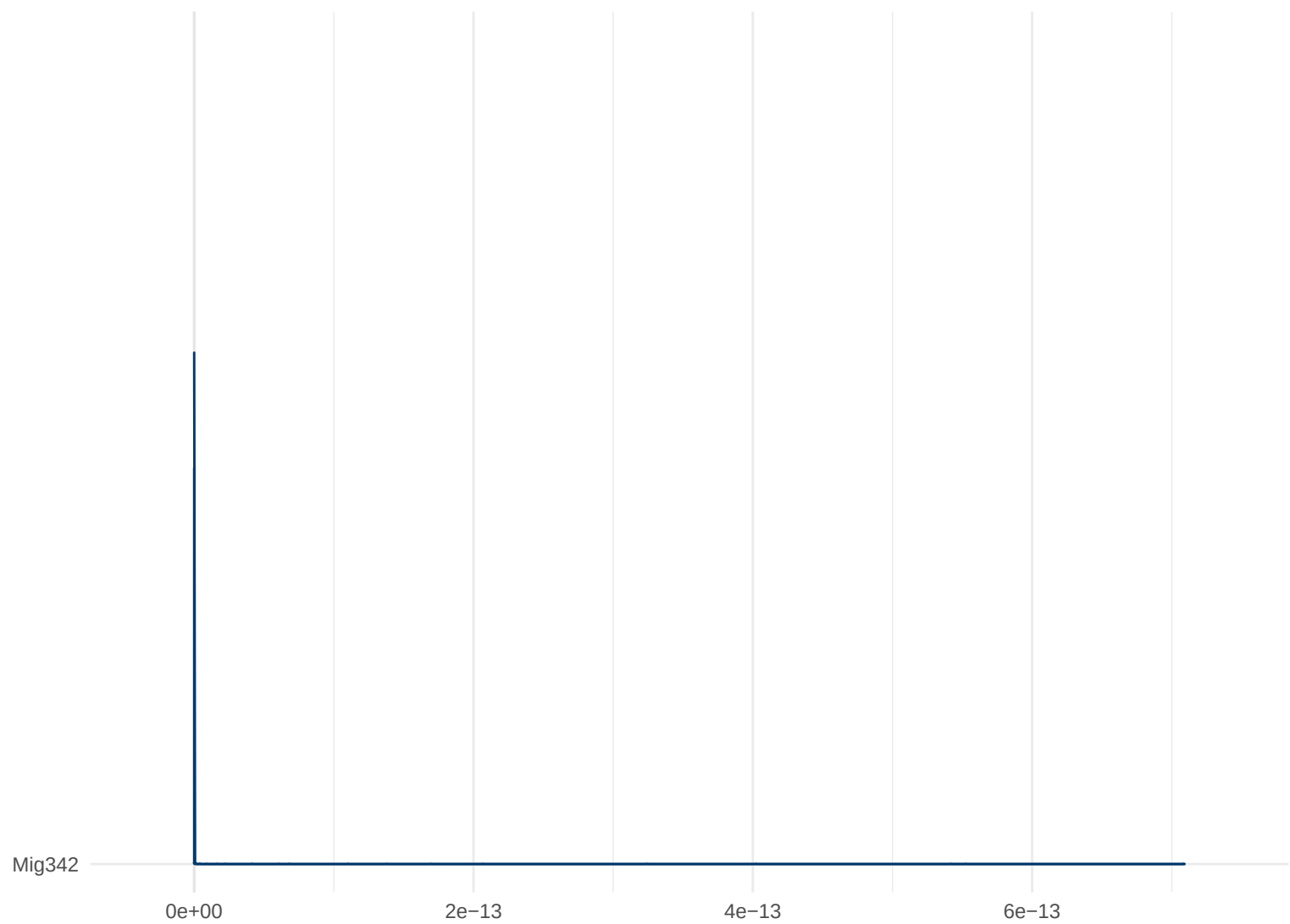
Posterior Density: Mig342
