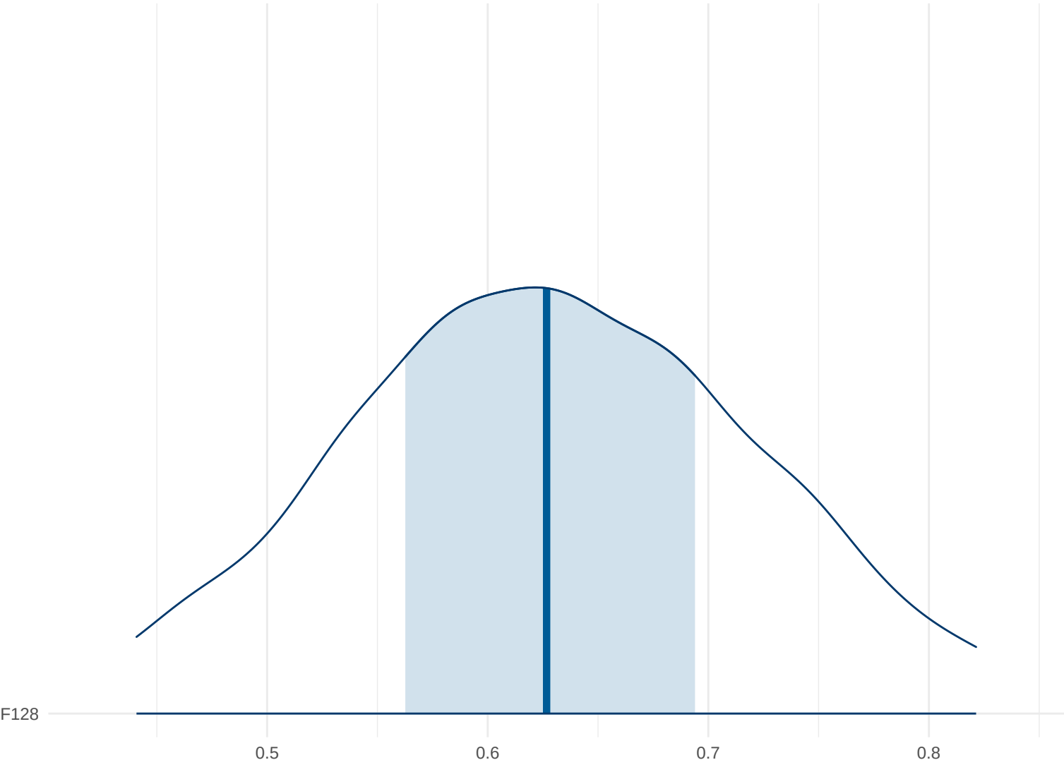
Posterior Density: F128
