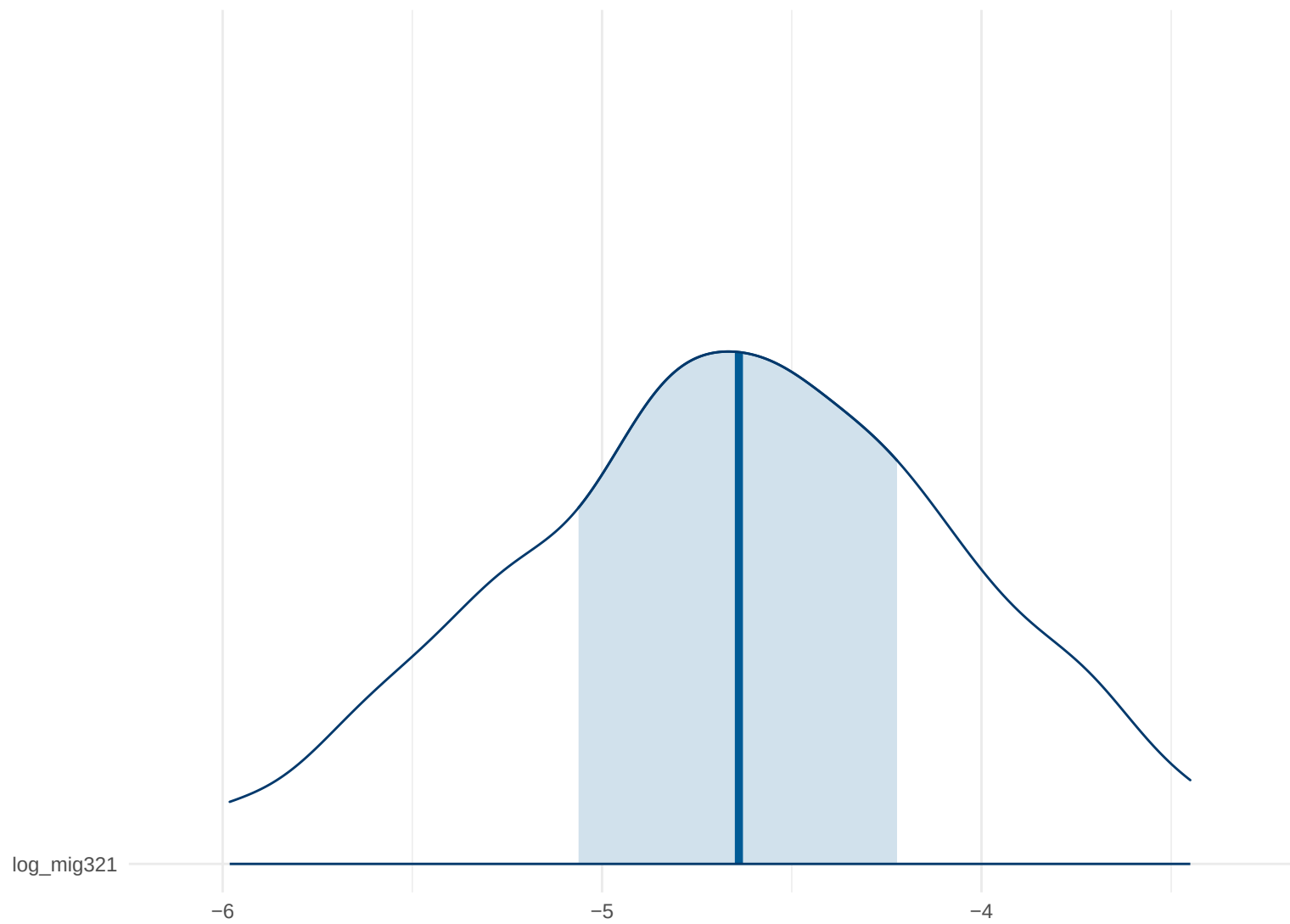
Posterior Density: log_mig321
