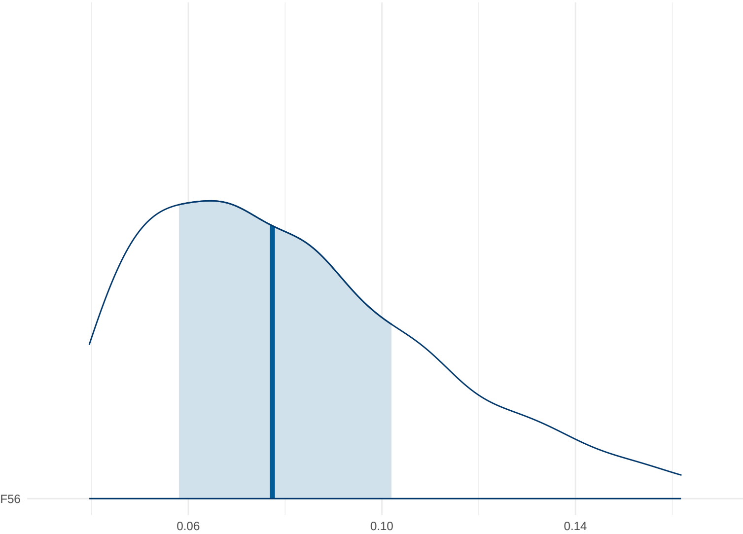
Posterior Density: F56
