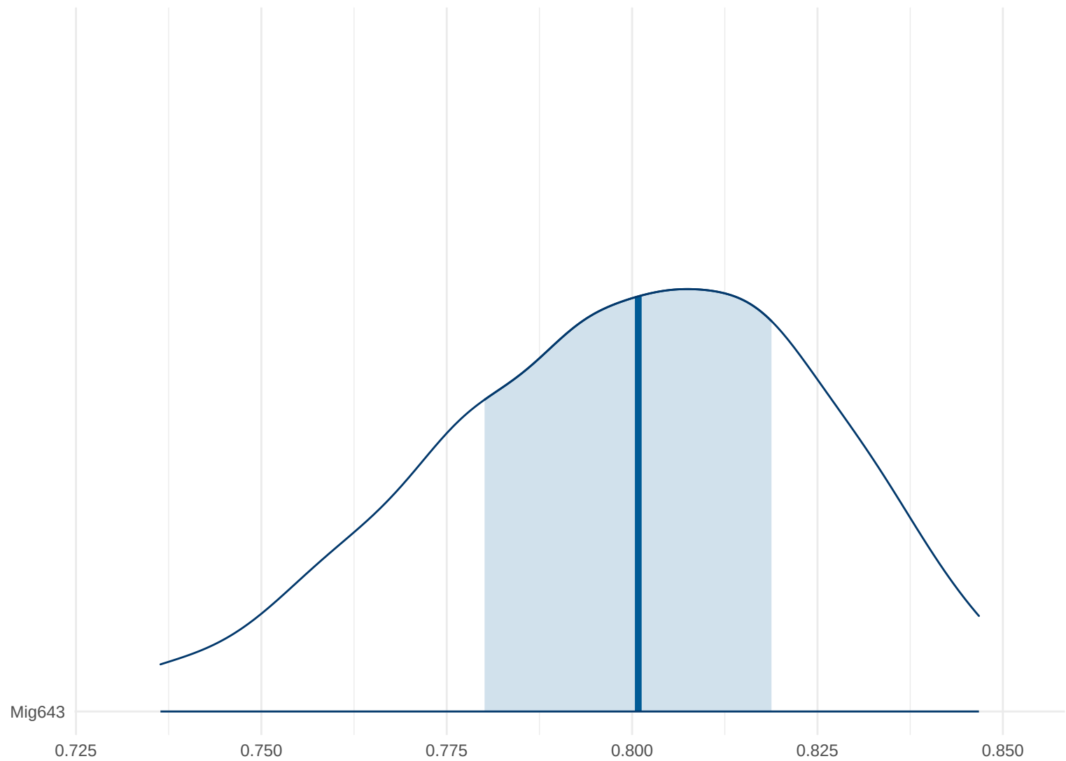
Posterior Density: Mig643
