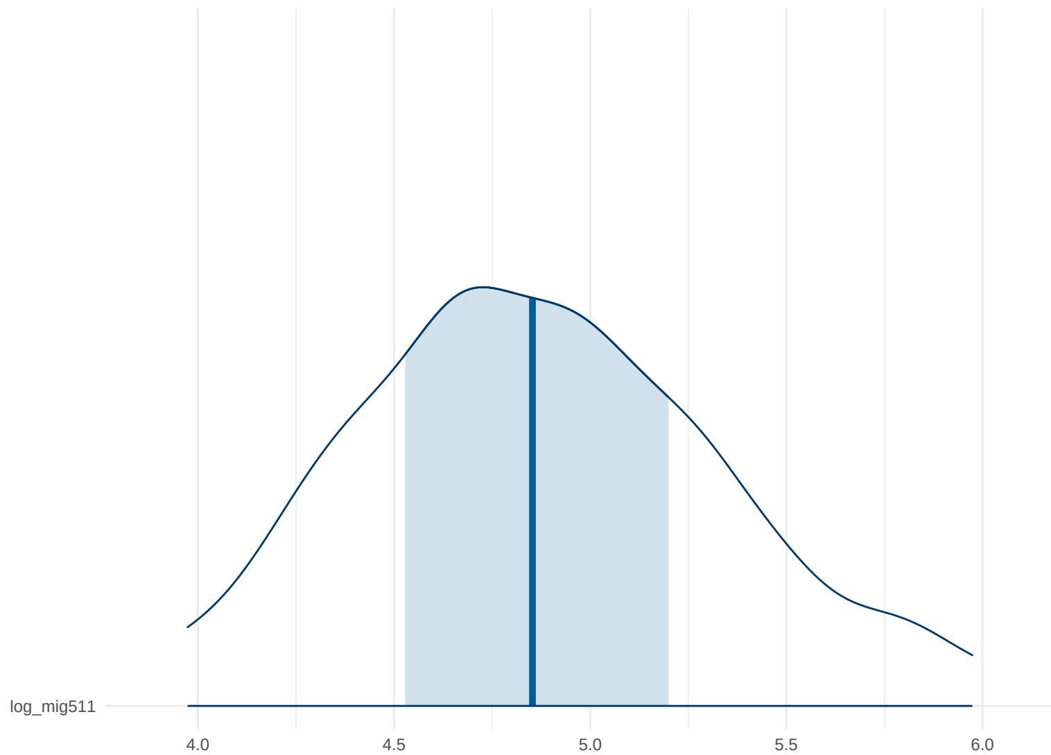
Posterior Density: log_mig511
