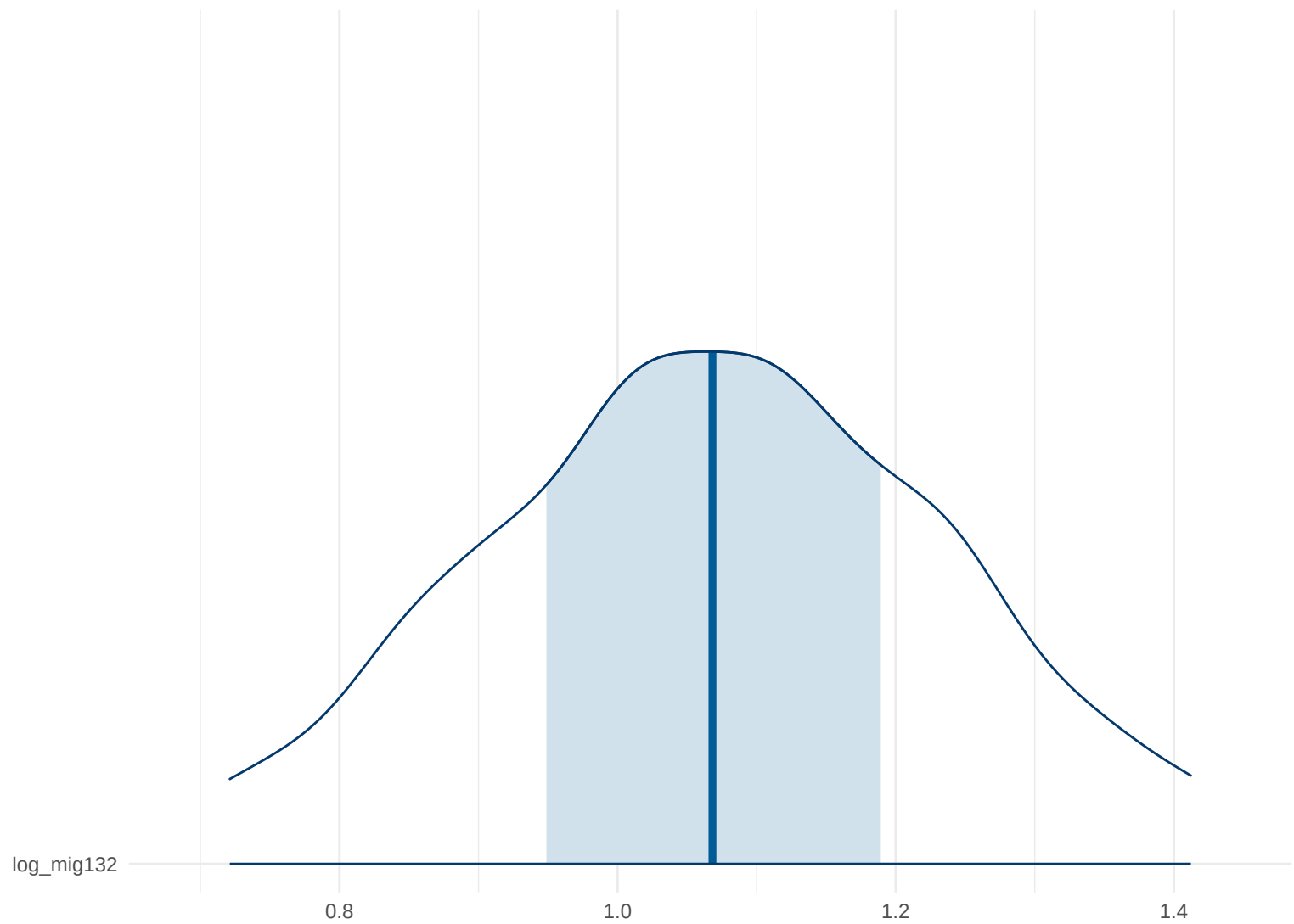
Posterior Density: log_mig132
