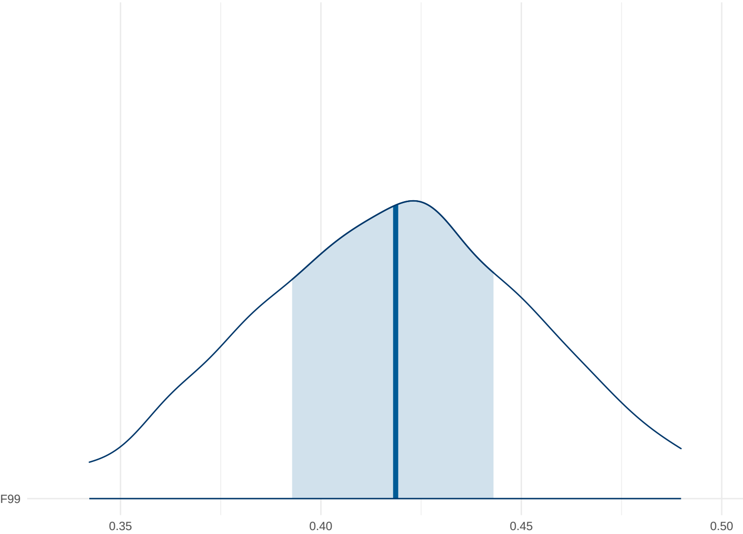
Posterior Density: F99
