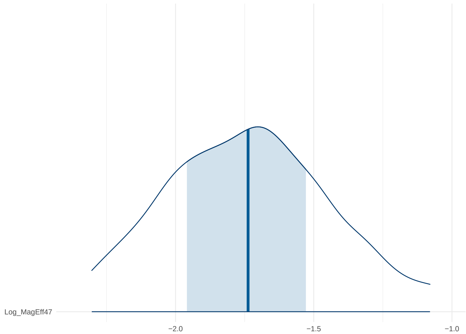
Posterior Density: Log_MagEff47
