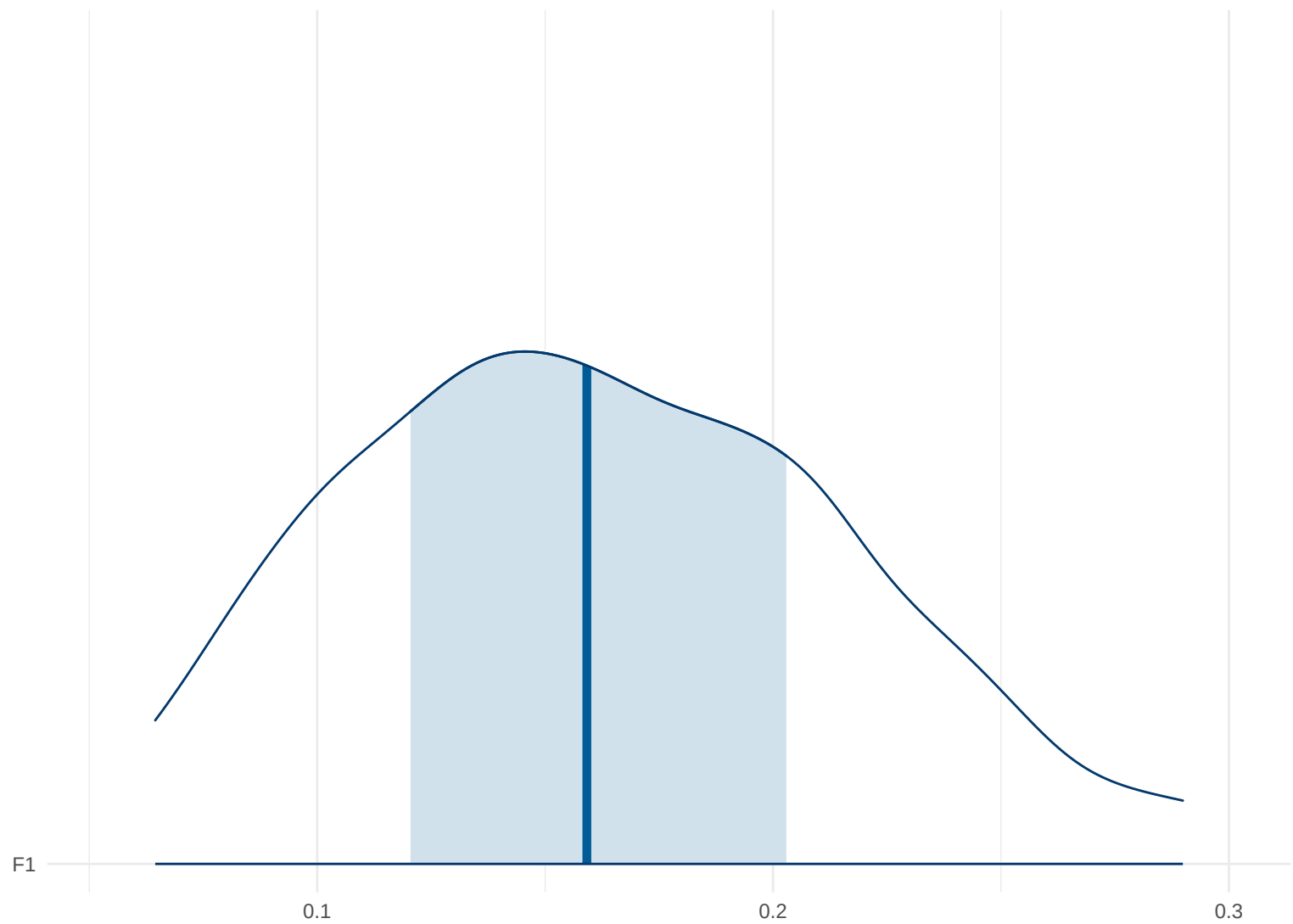
Posterior Density: F1
