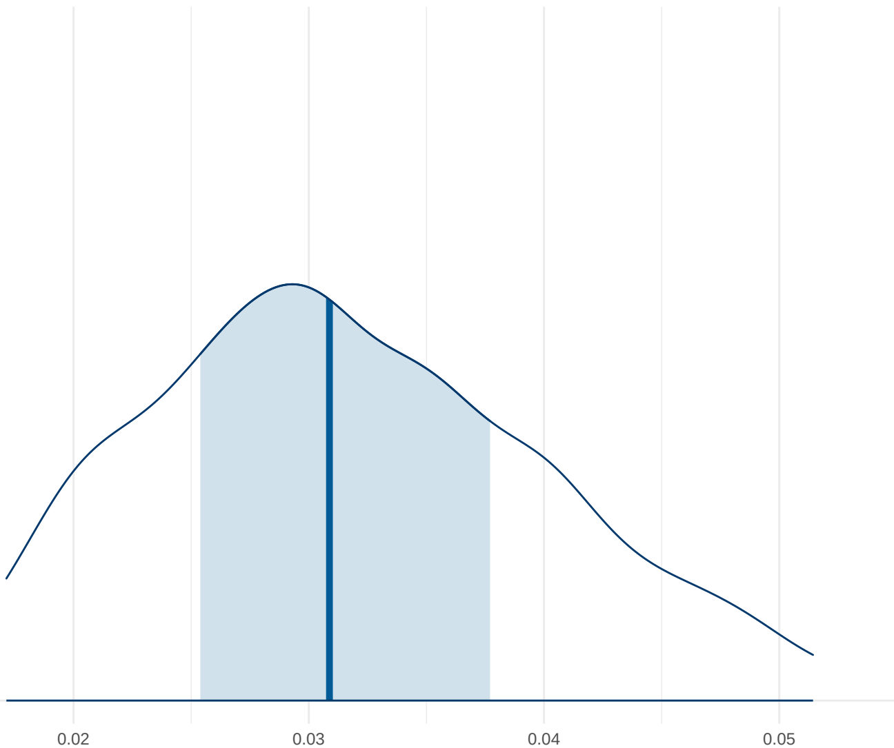
Posterior Density: Mig642
