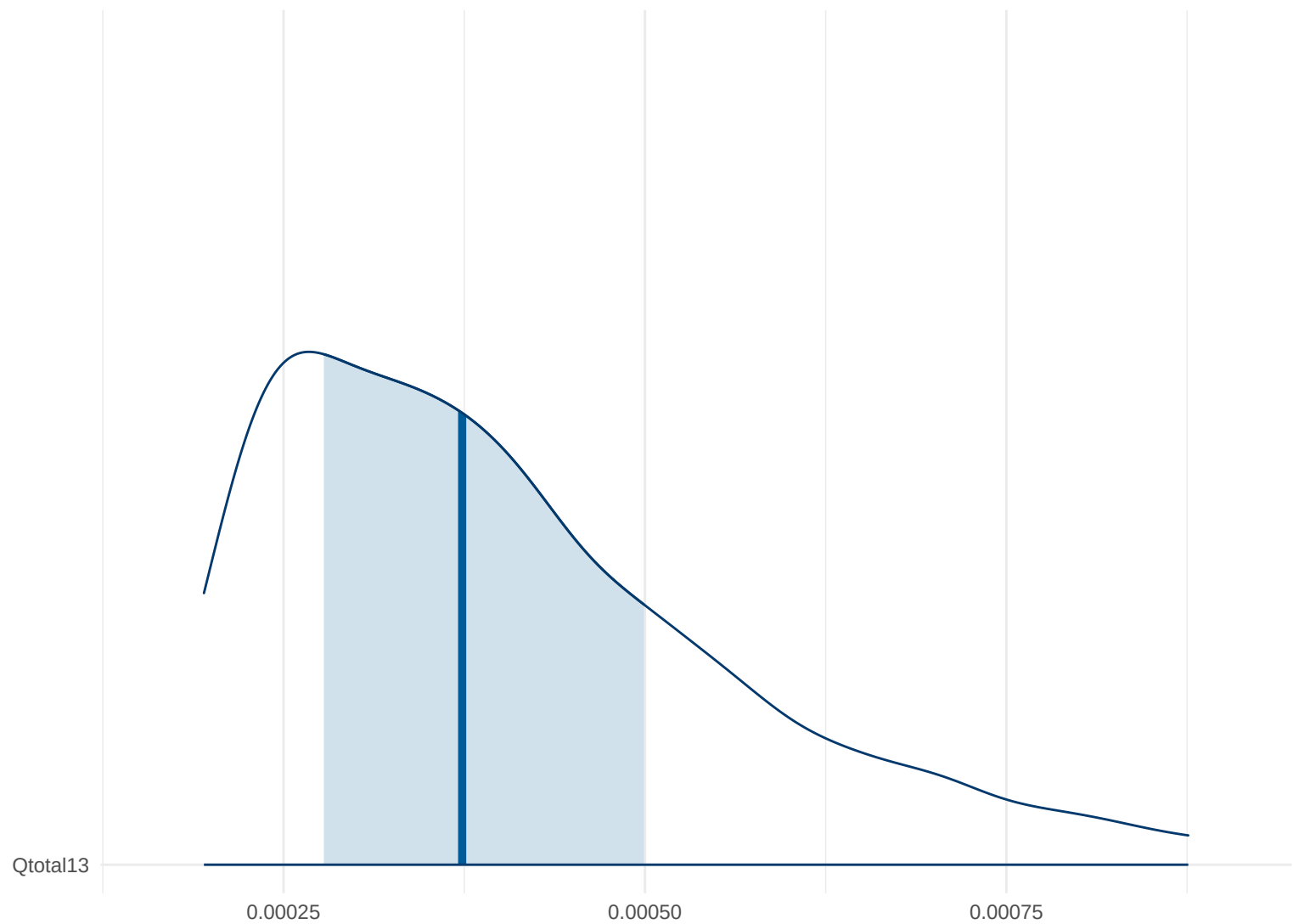
Posterior Density: Qtotal13
