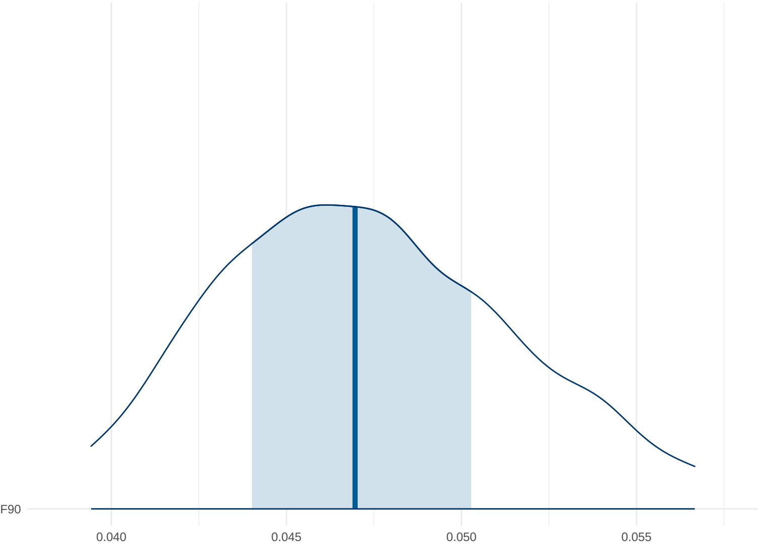
Posterior Density: F90
