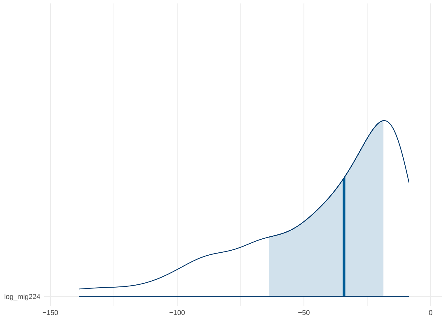
Posterior Density: log_mig224
