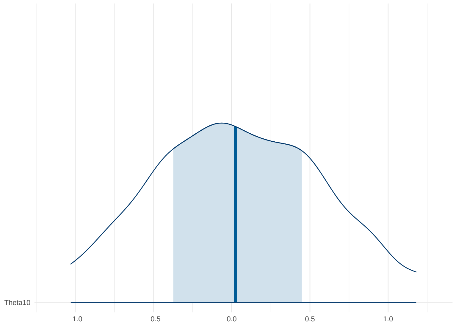
Posterior Density: Theta10
