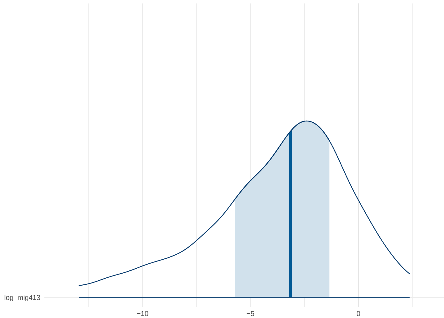
Posterior Density: log_mig413
