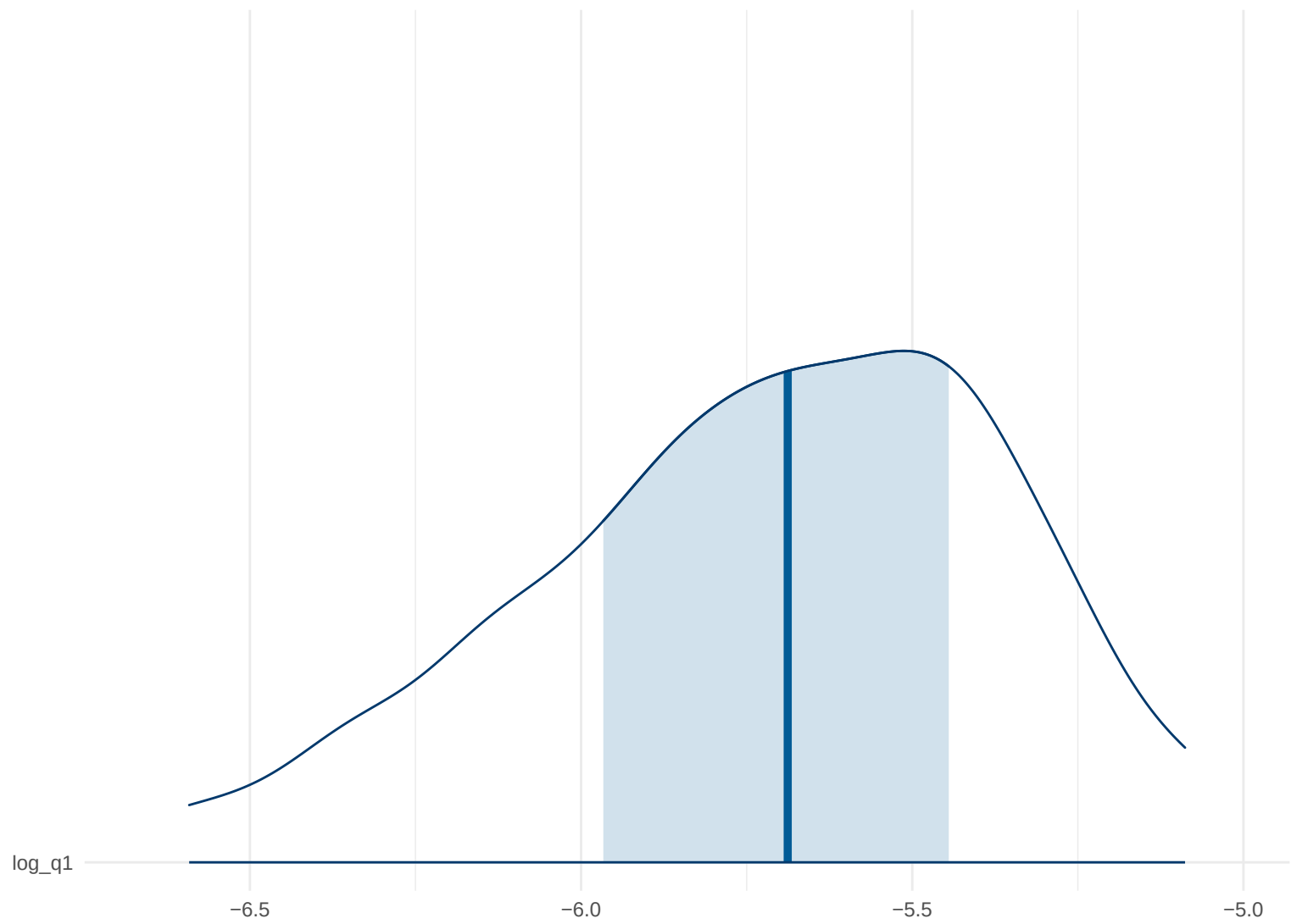
Posterior Density: log_q1
