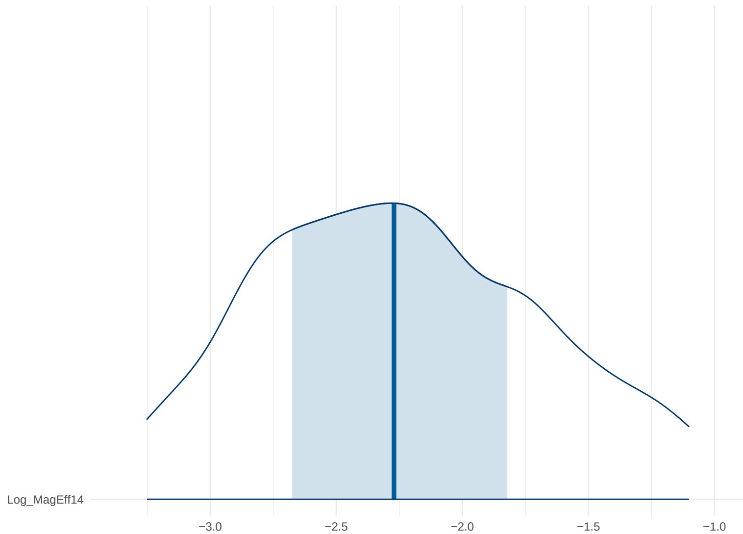
Posterior Density: Log_MagEff14
