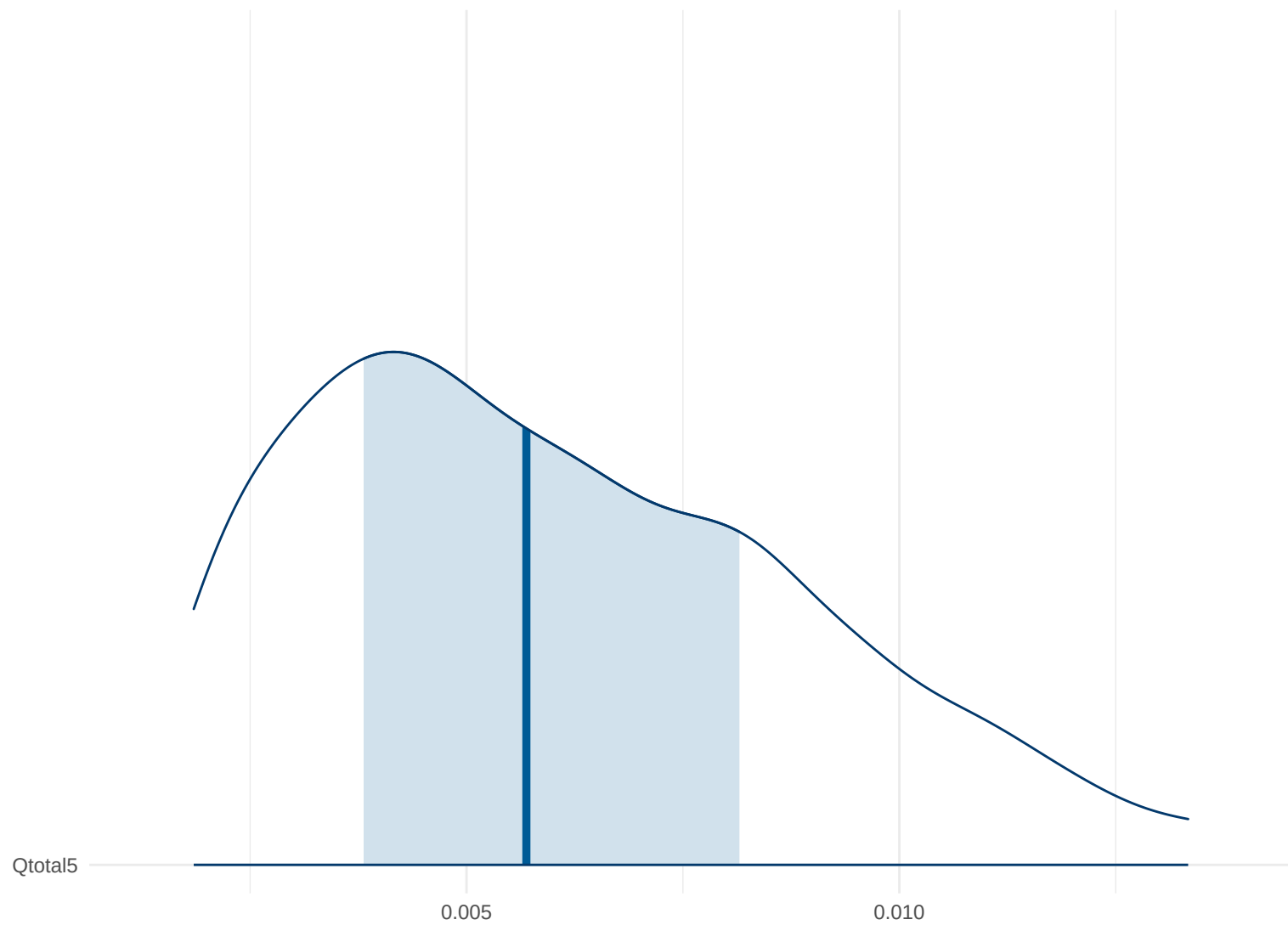
Posterior Density: Qtotal5
