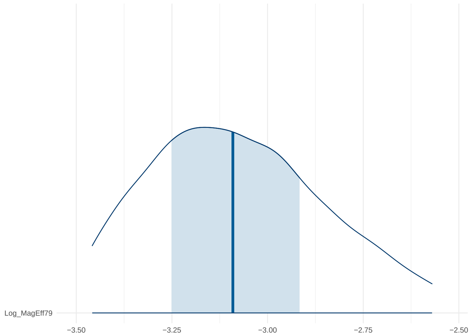
Posterior Density: Log_MagEff79
