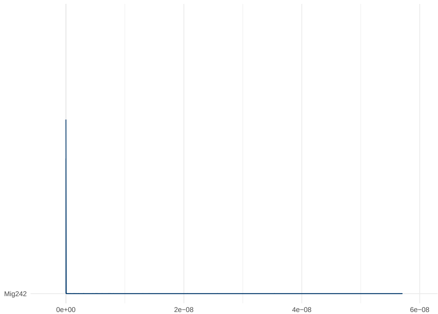
Posterior Density: Mig242
