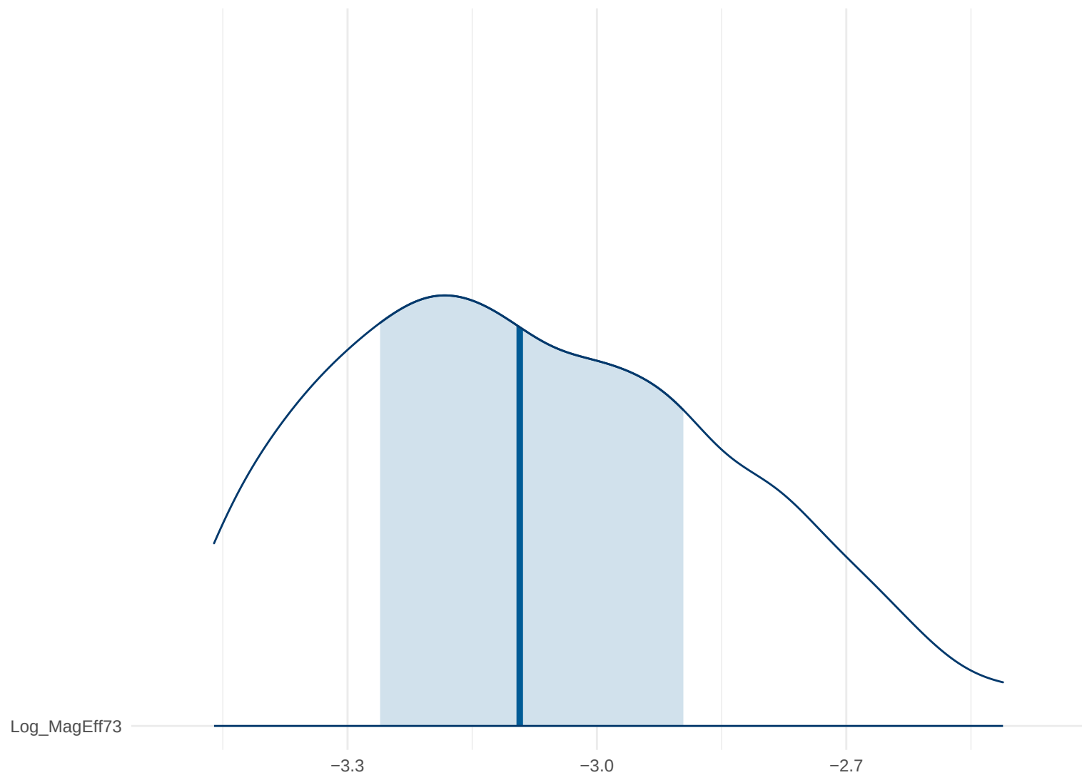
Posterior Density: Log_MagEff73
