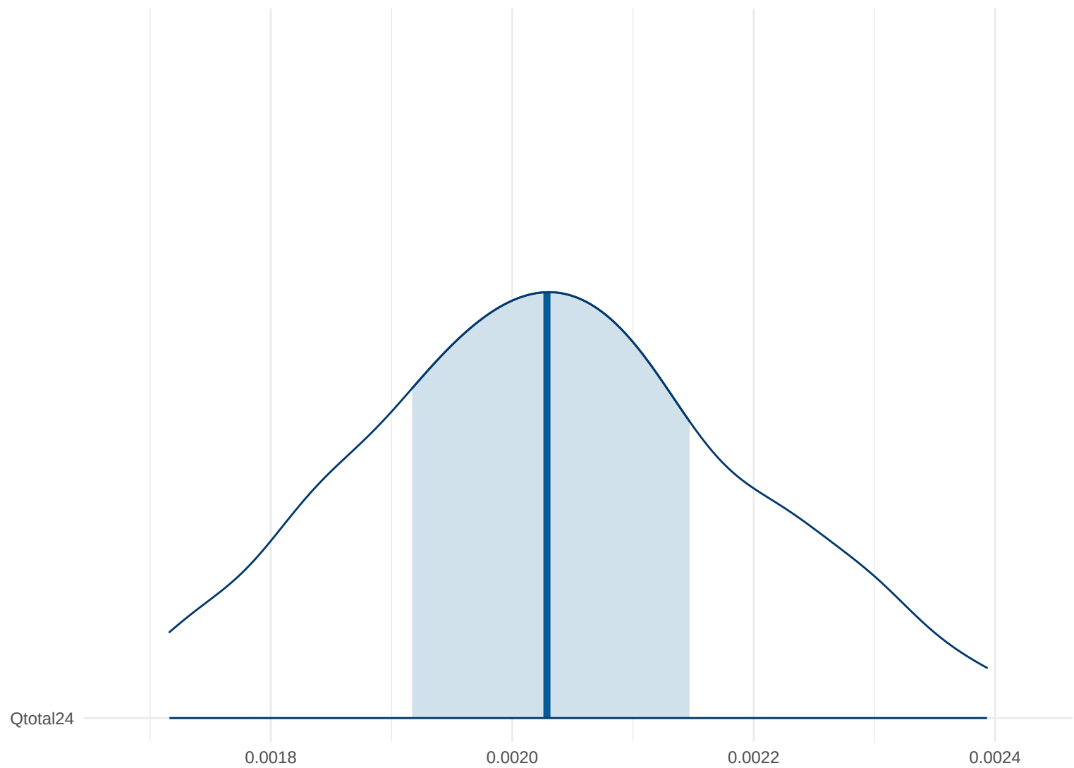
Posterior Density: Qtotal24
