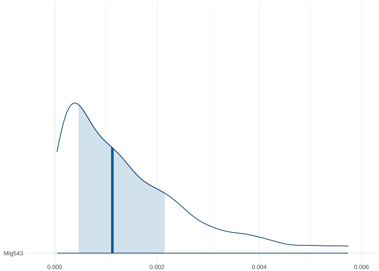
Posterior Density: Mig543
