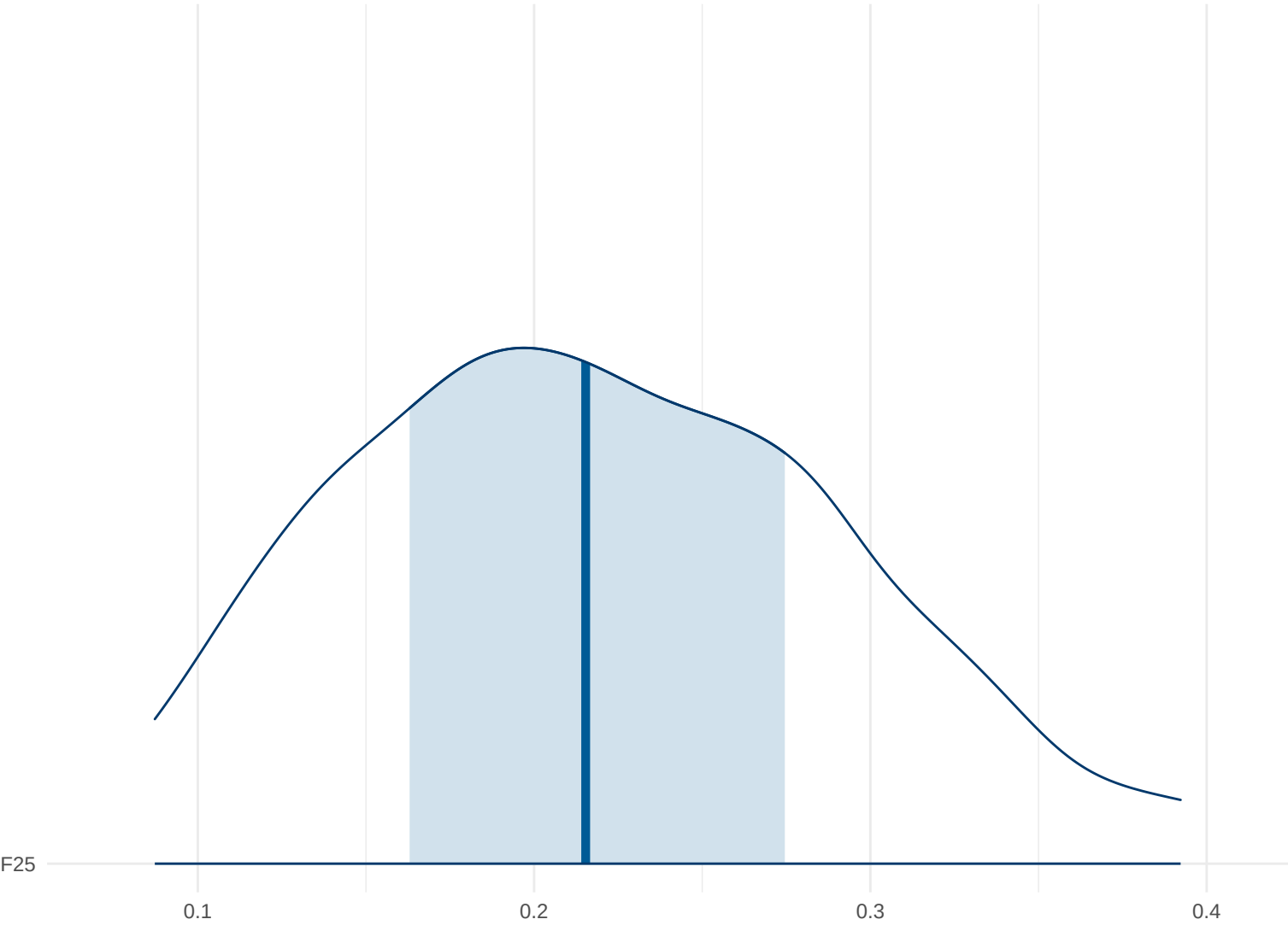
Posterior Density: F25
