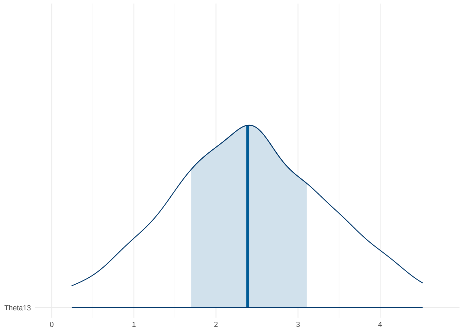
Posterior Density: Theta13
