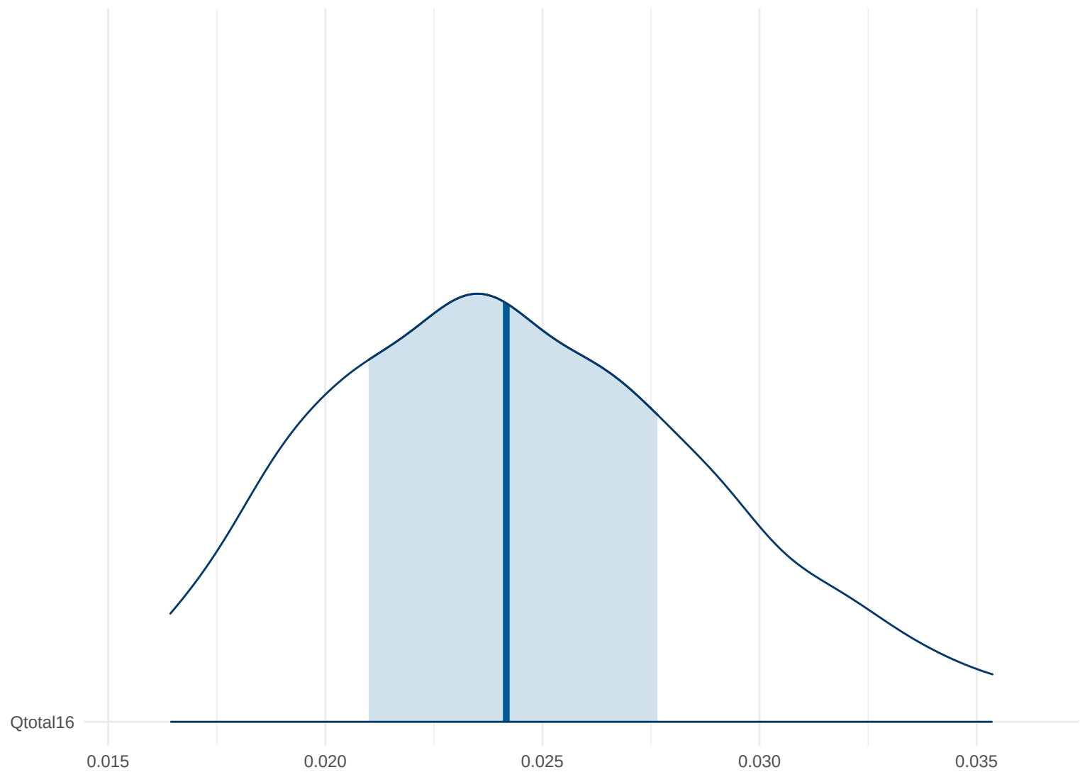
Posterior Density: Qtotal16
