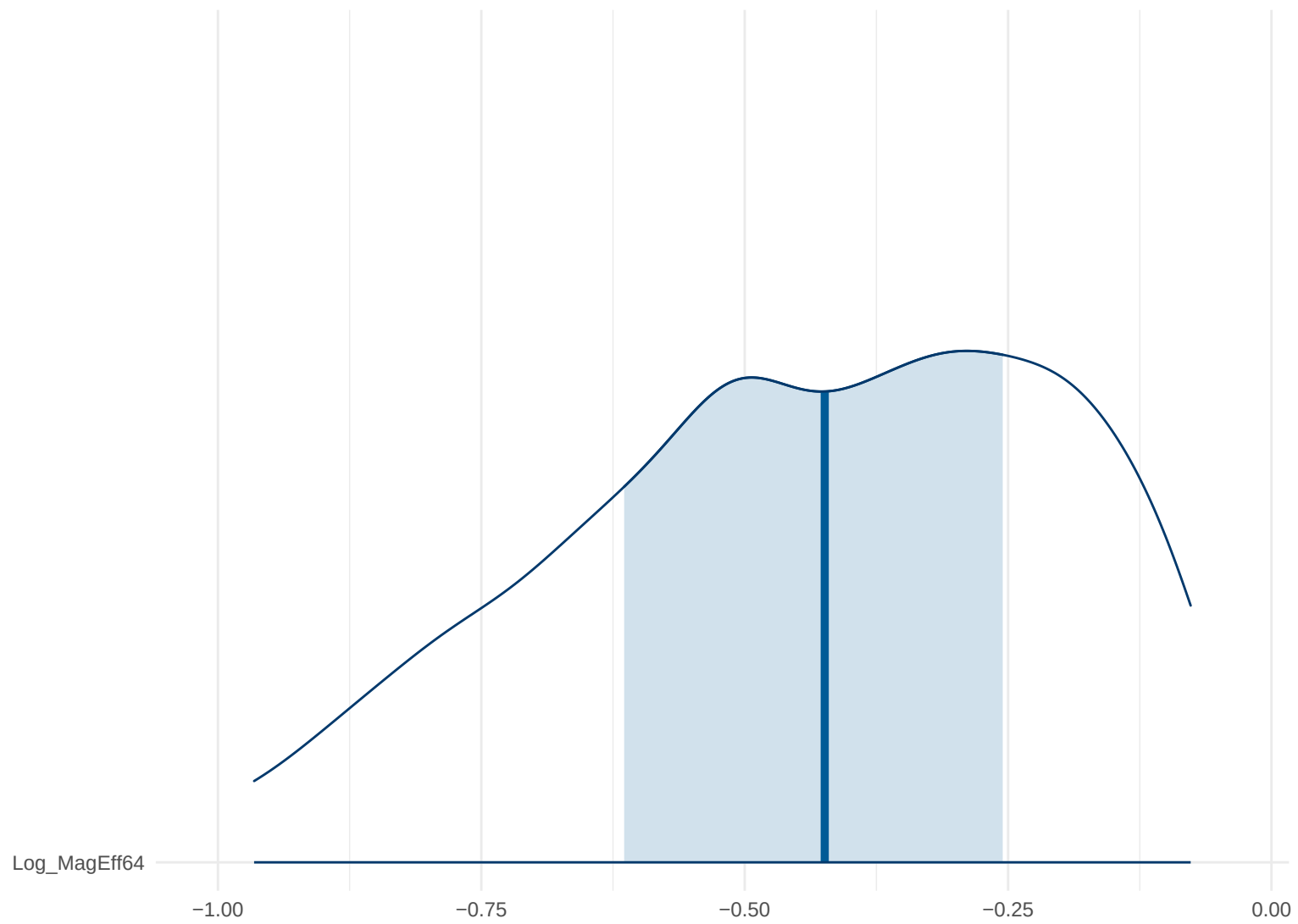
Posterior Density: Log_MagEff64
