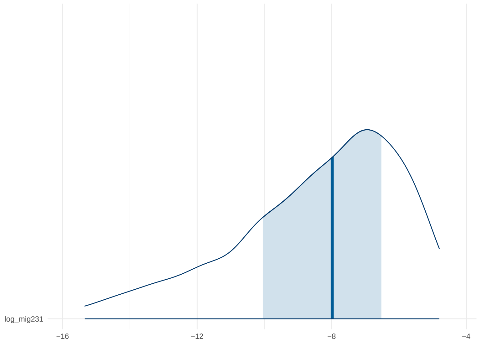
Posterior Density: log_mig231
