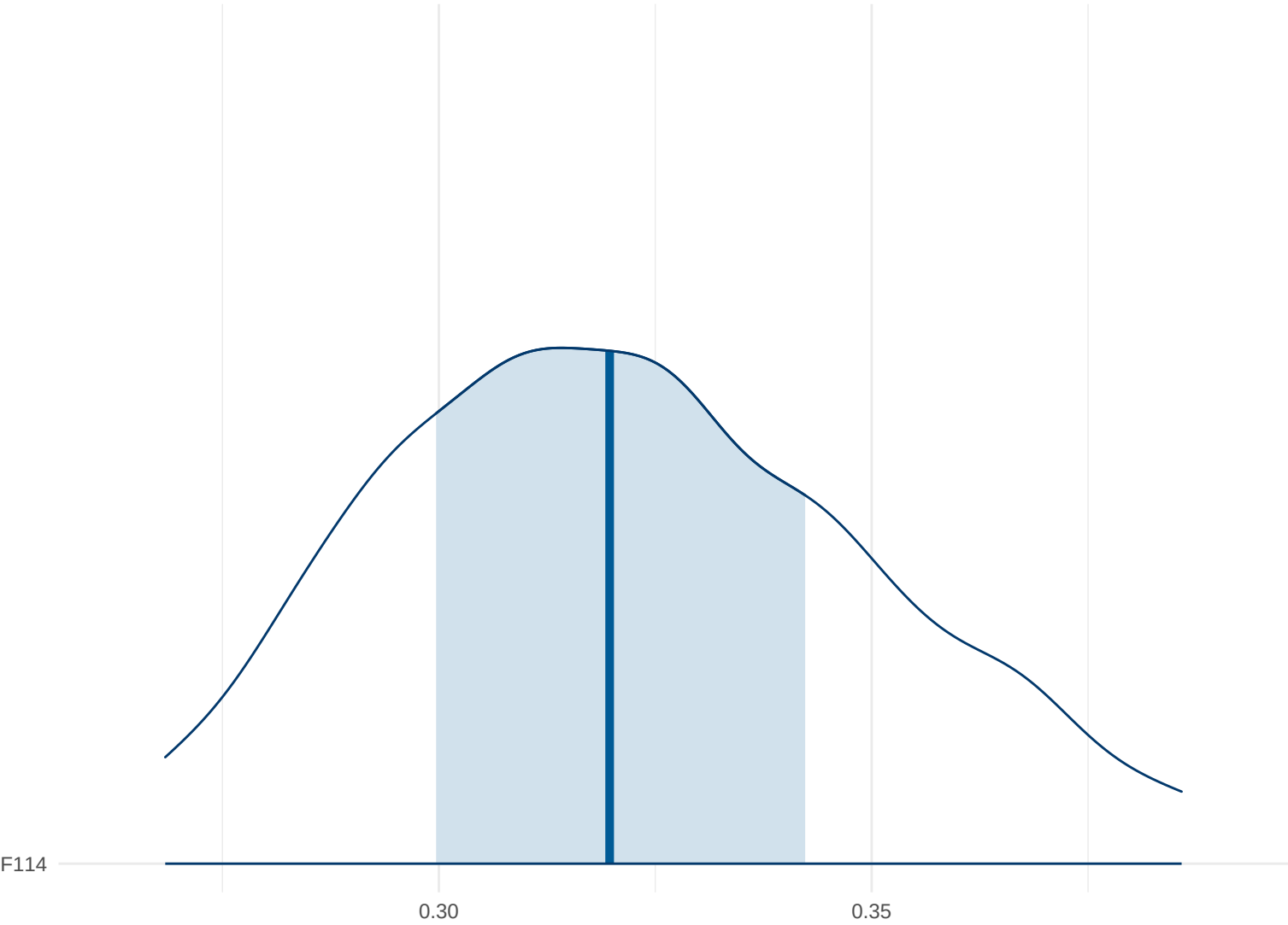
Posterior Density: F114
