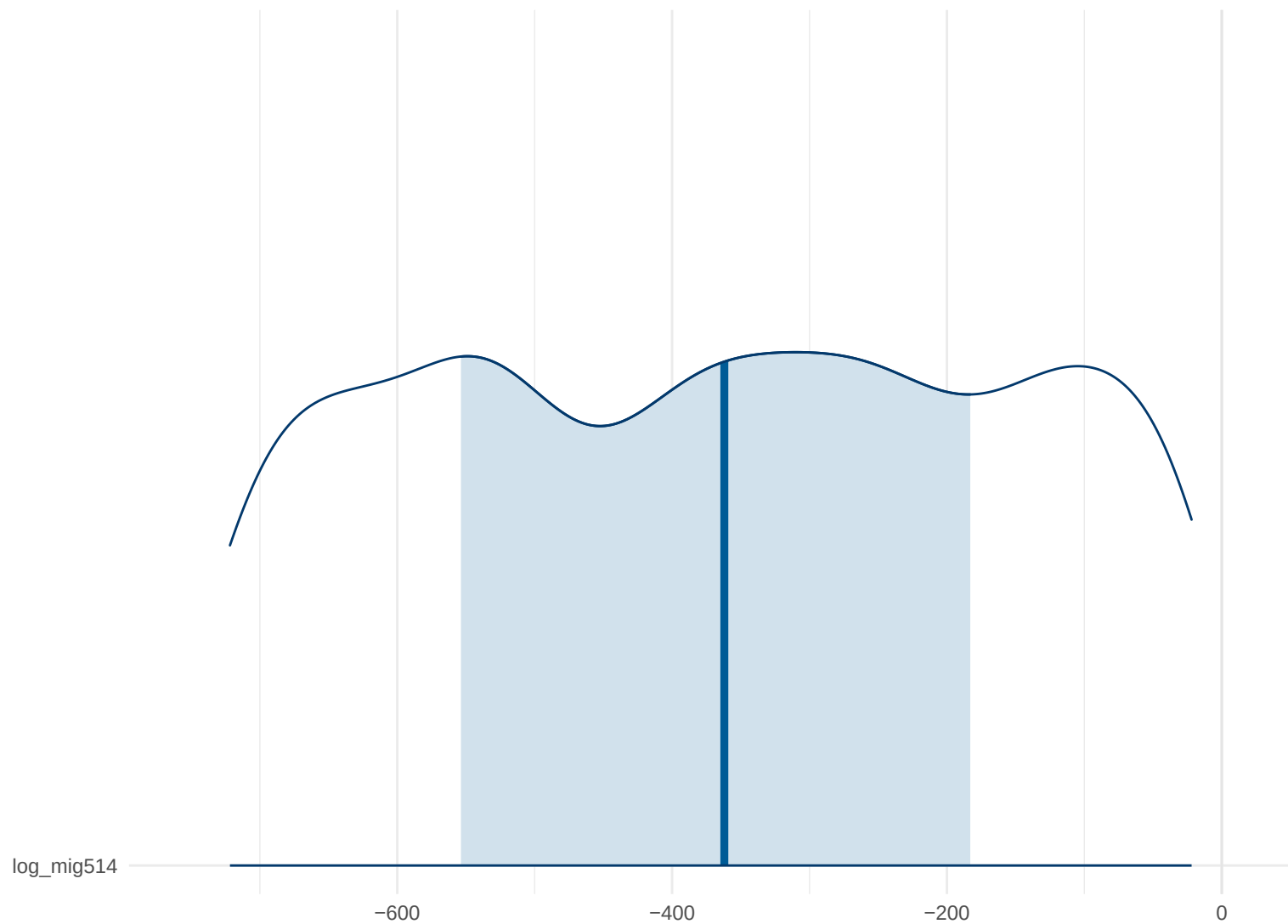
Posterior Density: log_mig514
