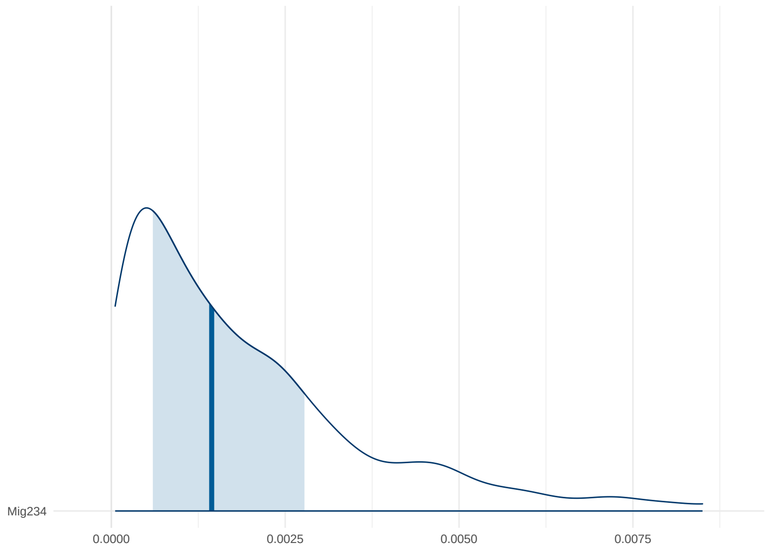
Posterior Density: Mig234
