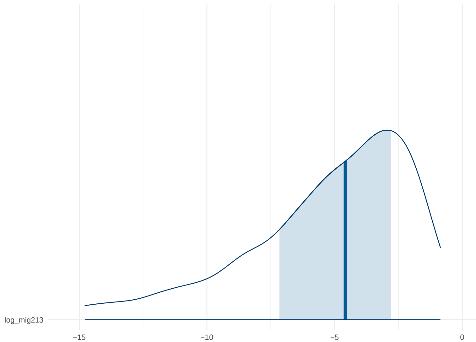
Posterior Density: log_mig213
