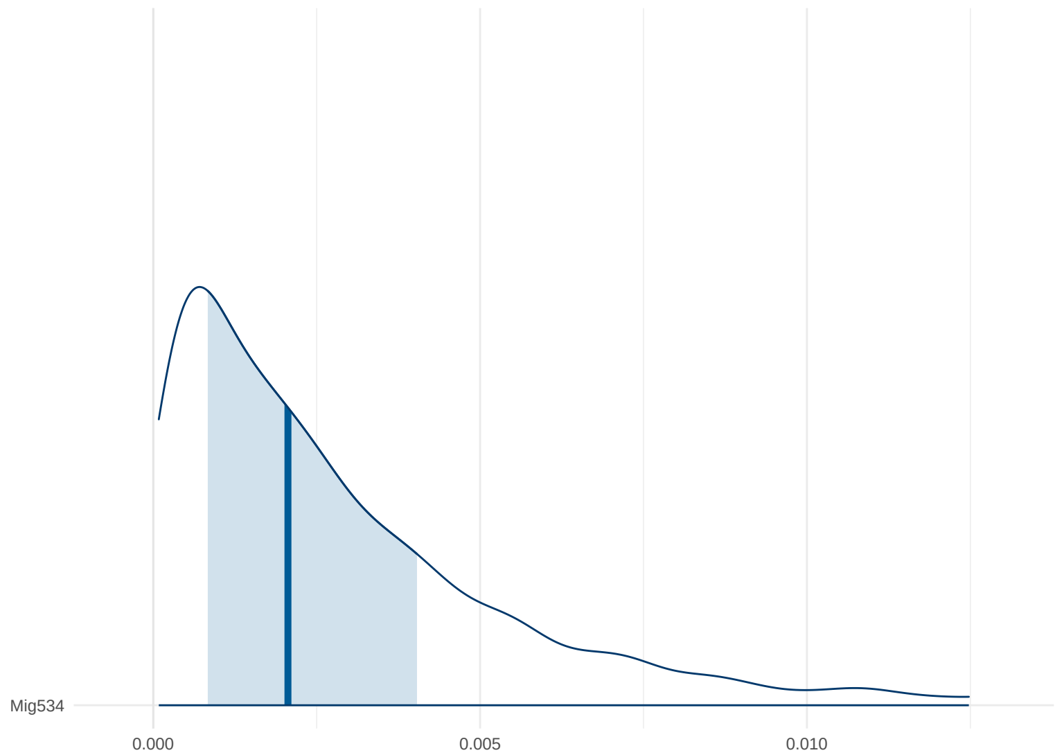
Posterior Density: Mig534
