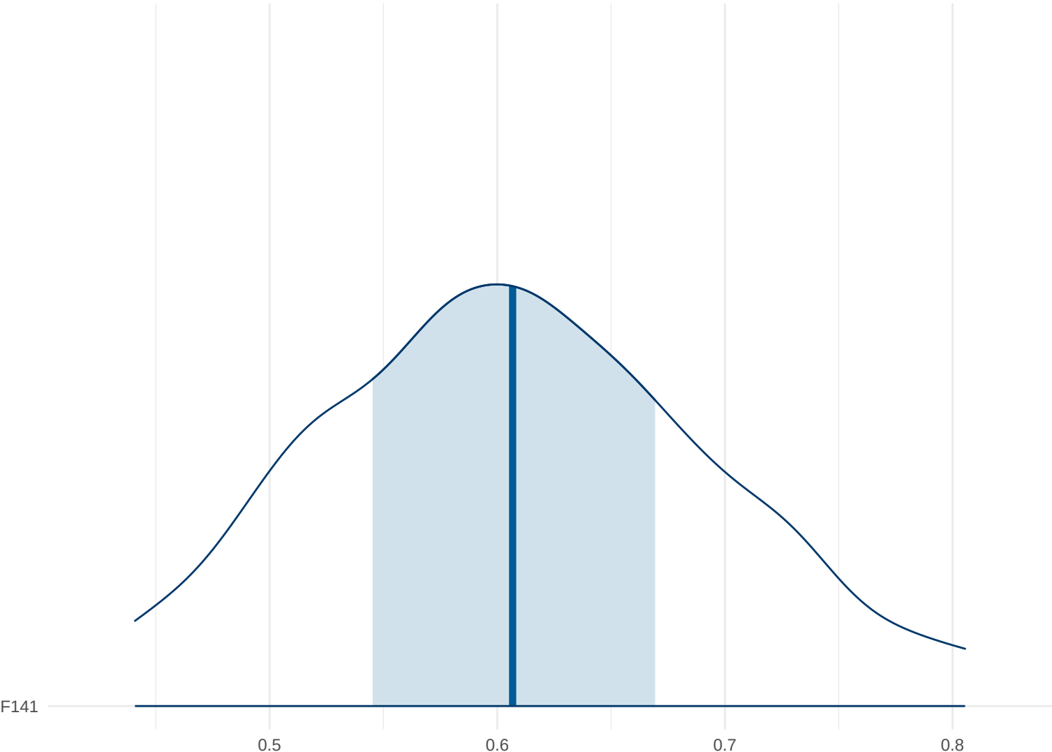
Posterior Density: F141
