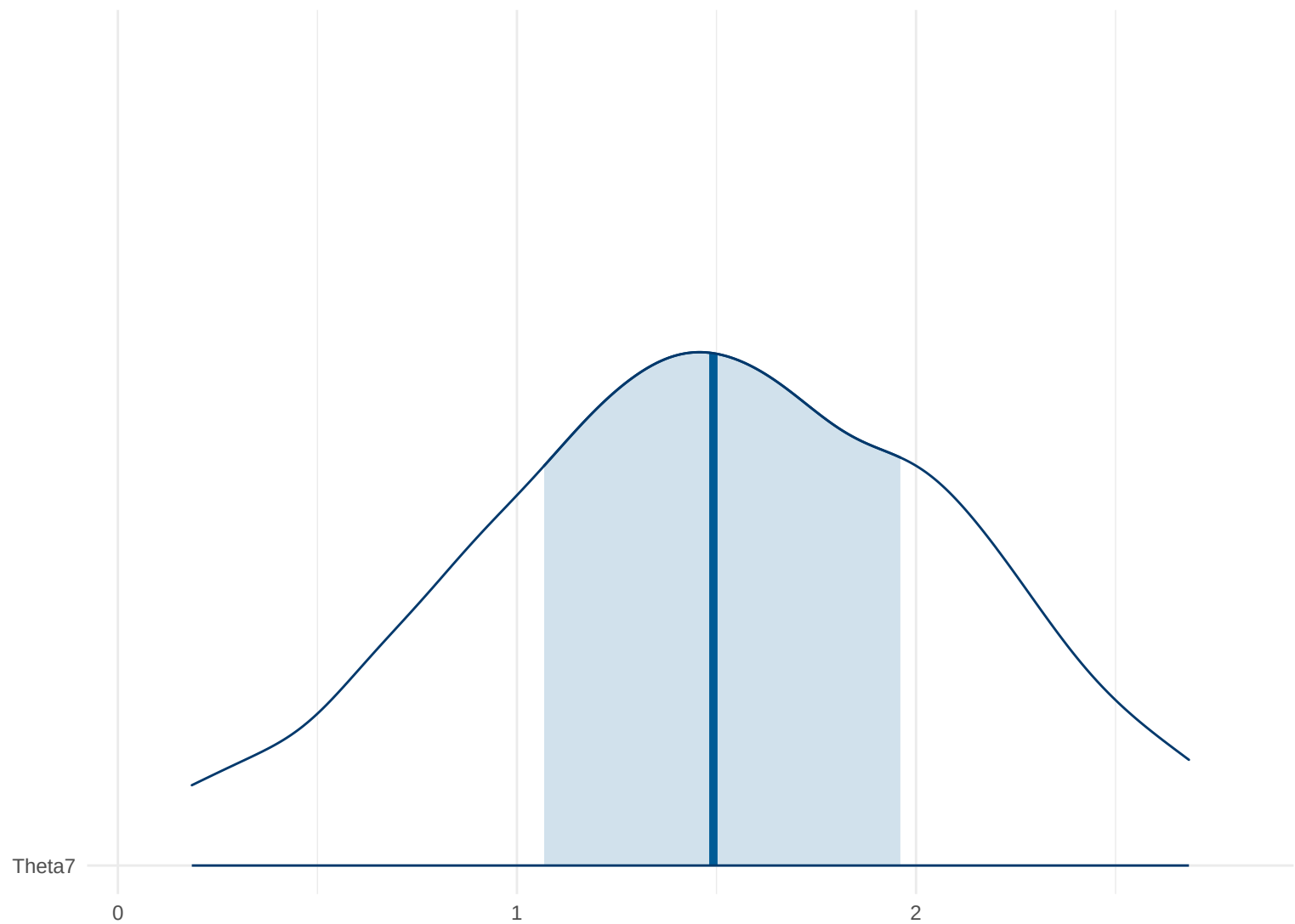
Posterior Density: Theta7
