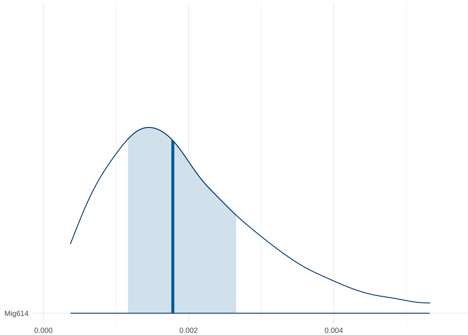
Posterior Density: Mig614
