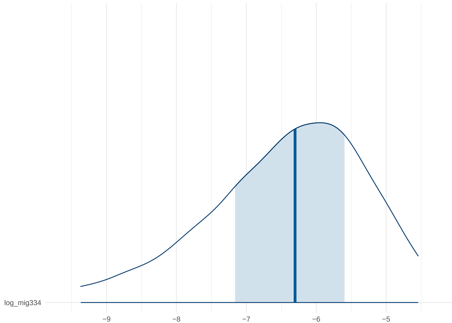
Posterior Density: log_mig334
