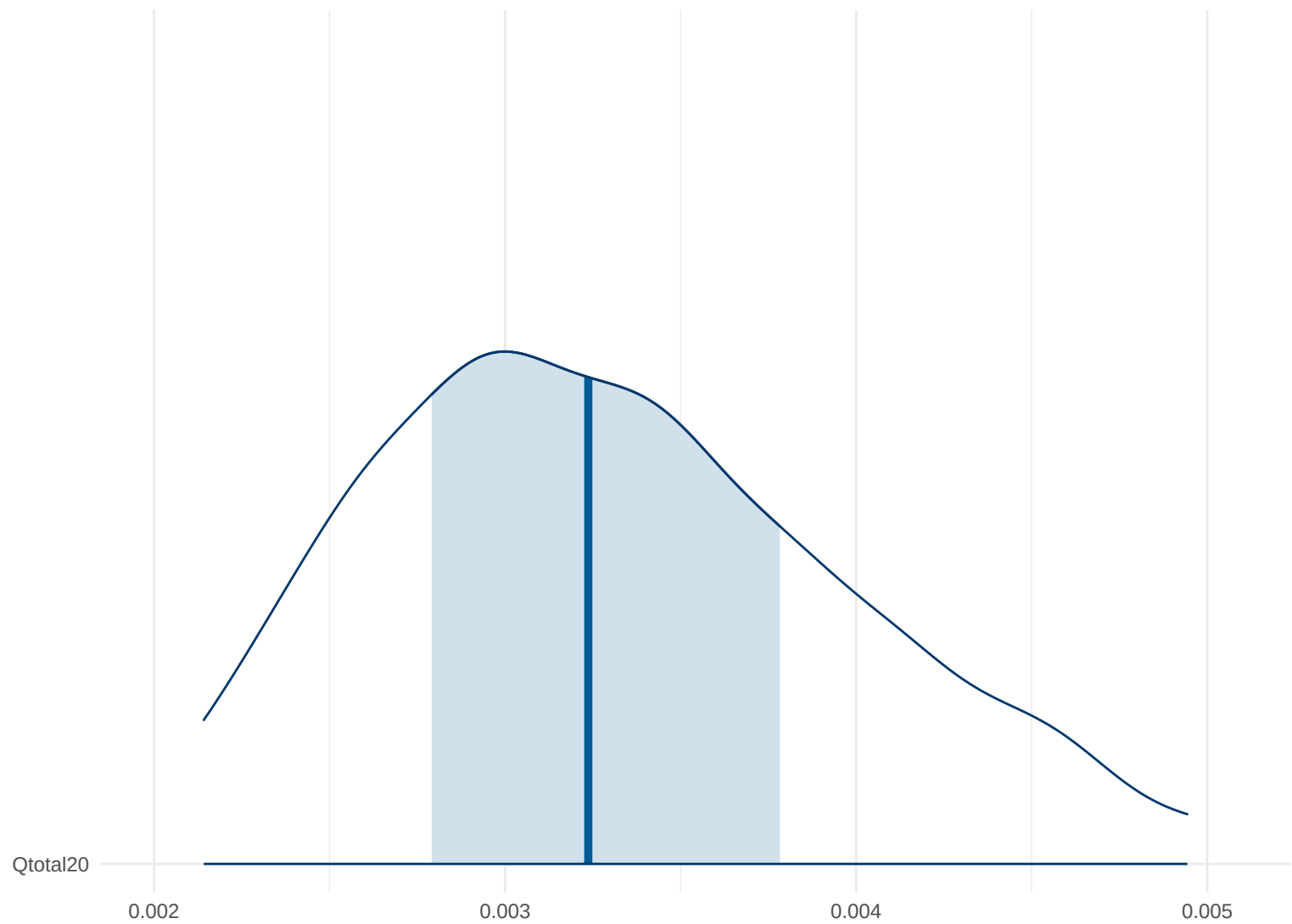
Posterior Density: Qtotal20
