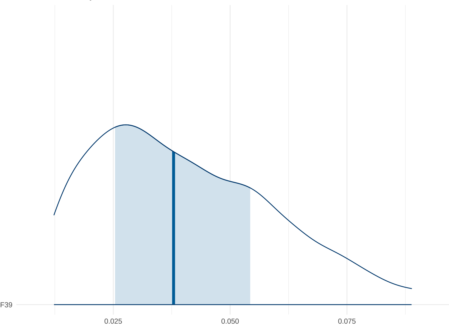
Posterior Density: F39
