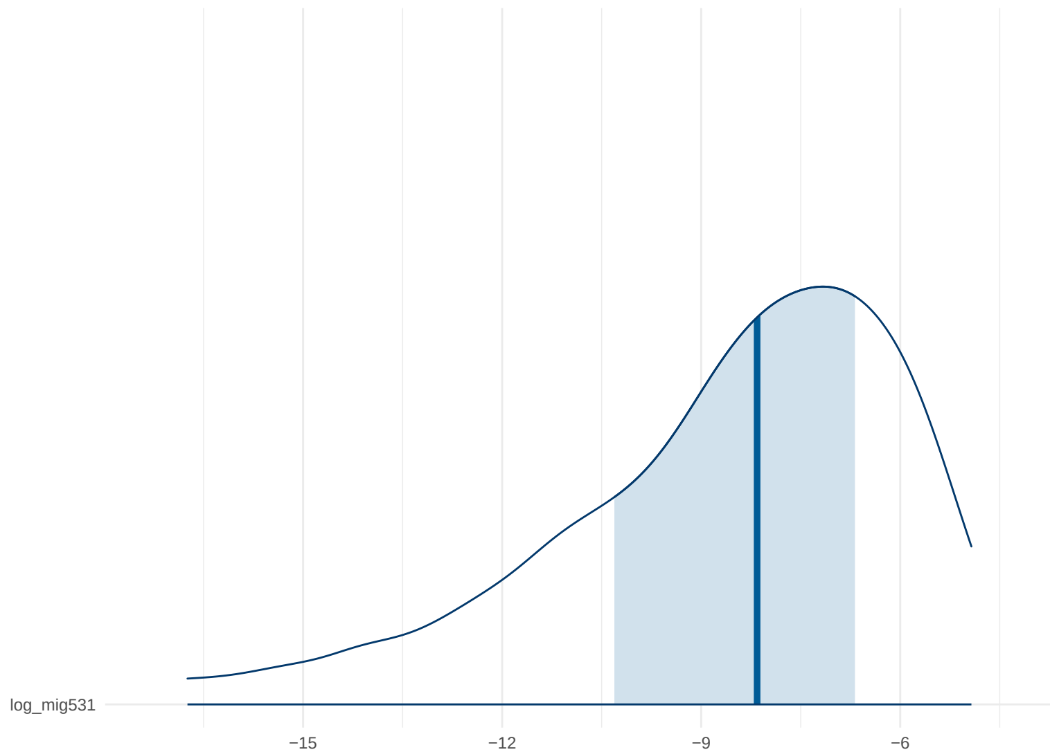
Posterior Density: log_mig531
