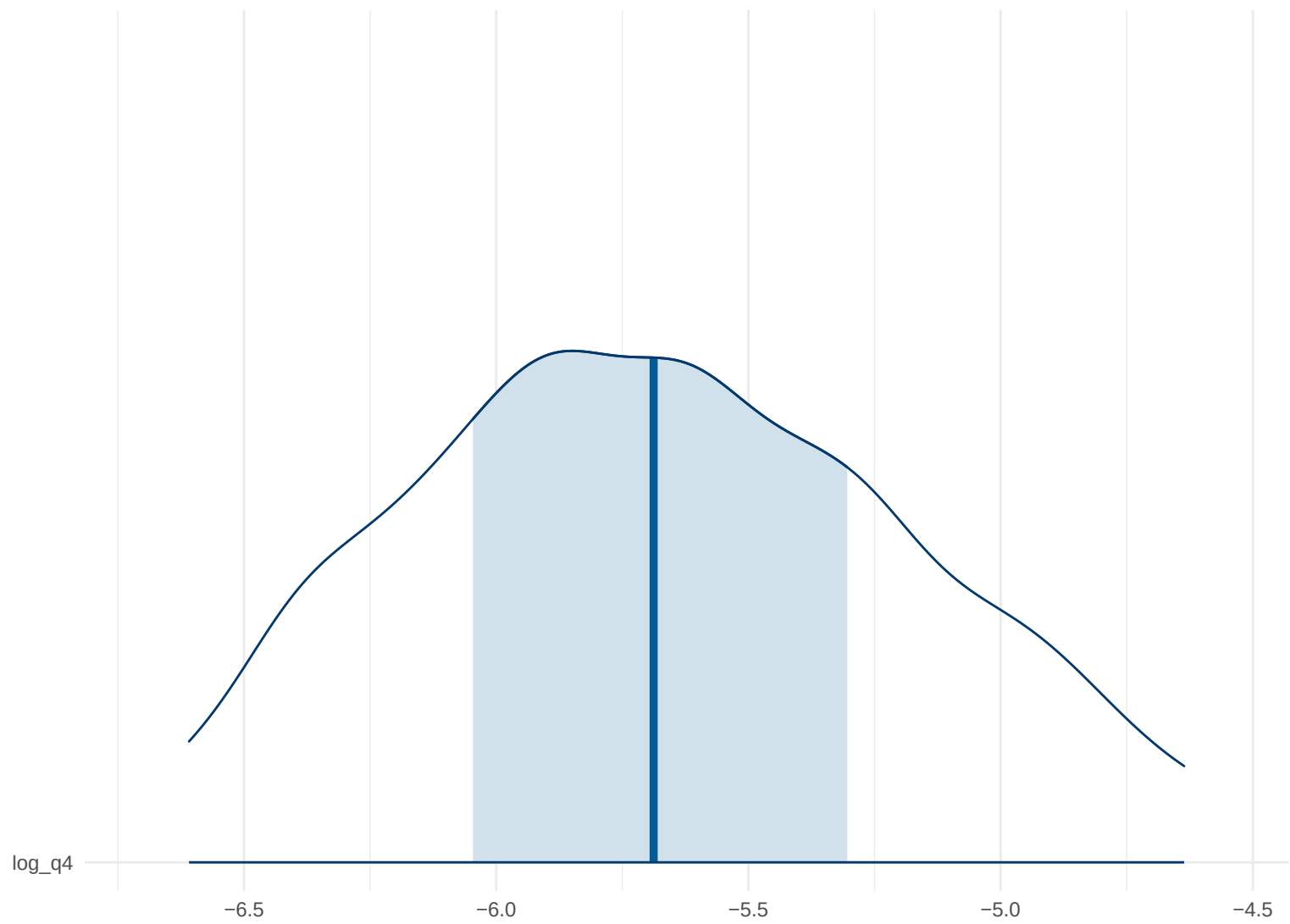
Posterior Density: log_q4
