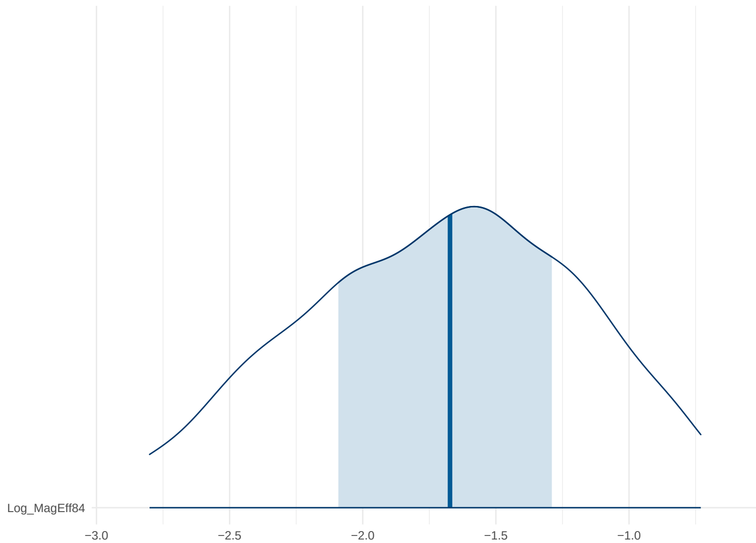
Posterior Density: Log_MagEff84
