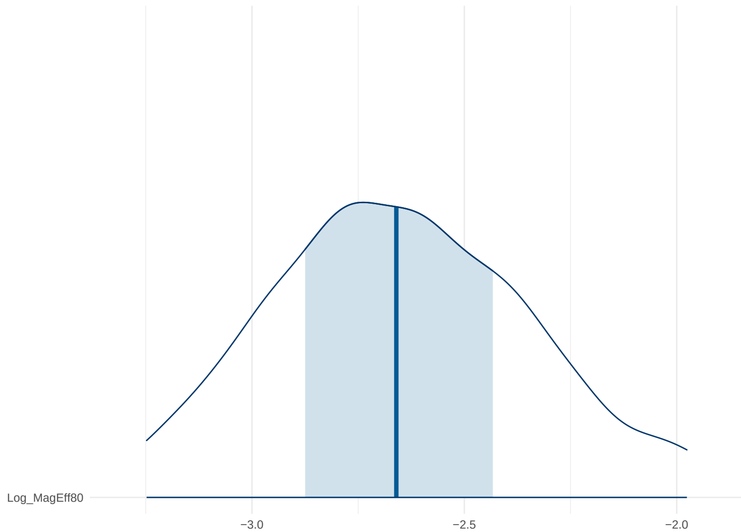
Posterior Density: Log_MagEff80
