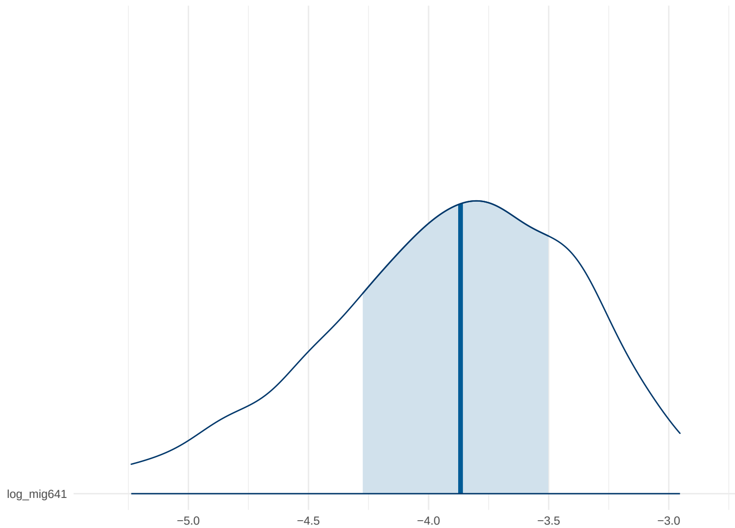
Posterior Density: log_mig641
