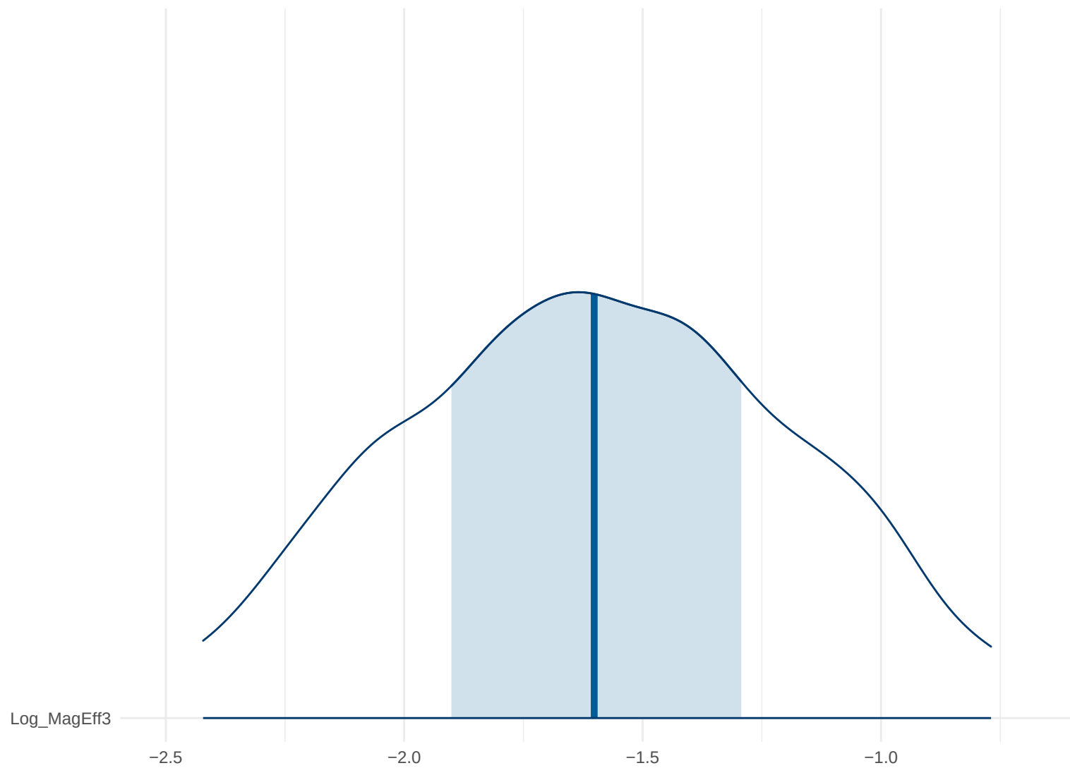
Posterior Density: Log_MagEff3
