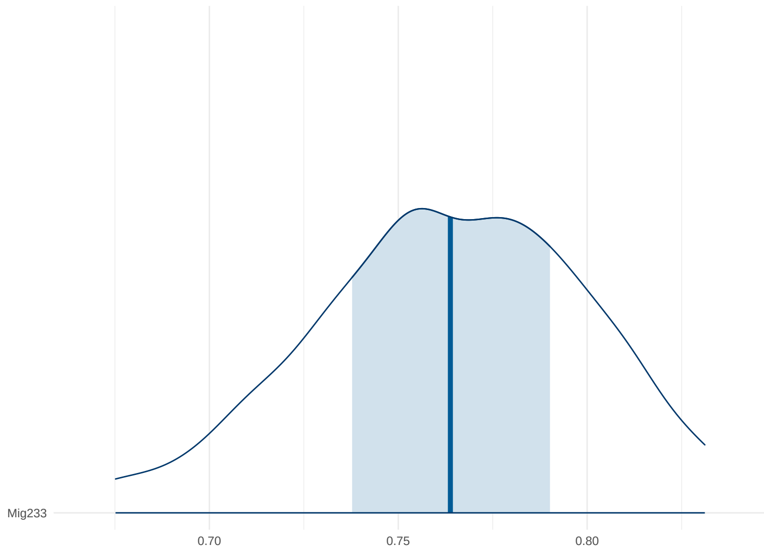
Posterior Density: Mig233
