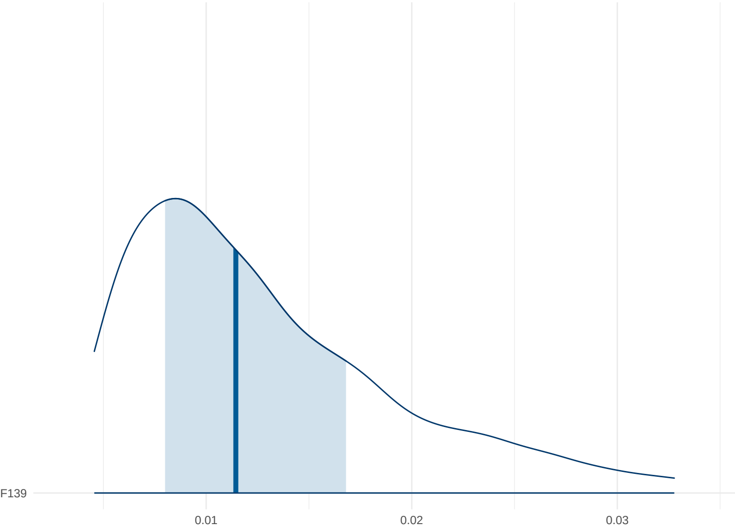
Posterior Density: F139
