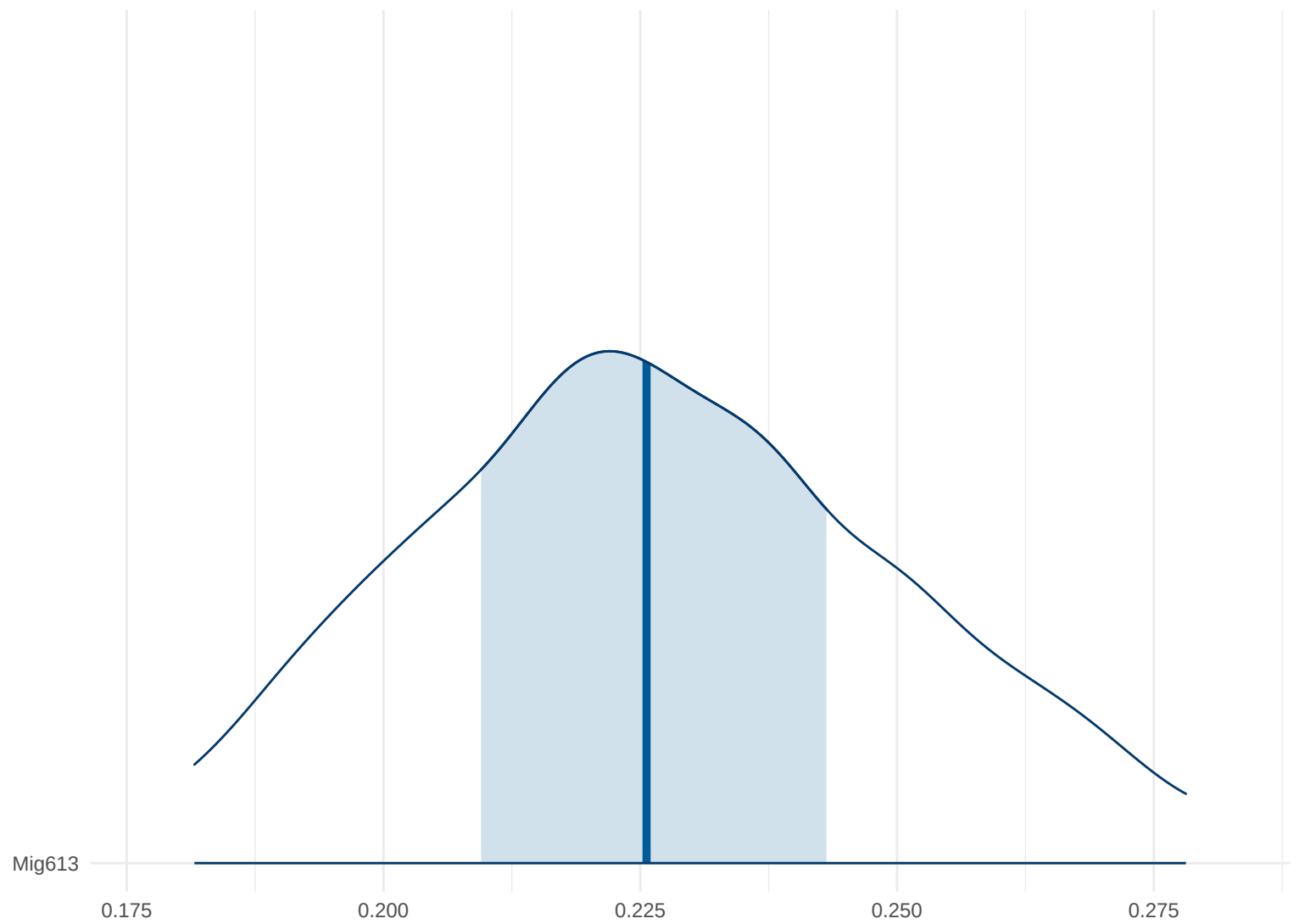
Posterior Density: Mig613
