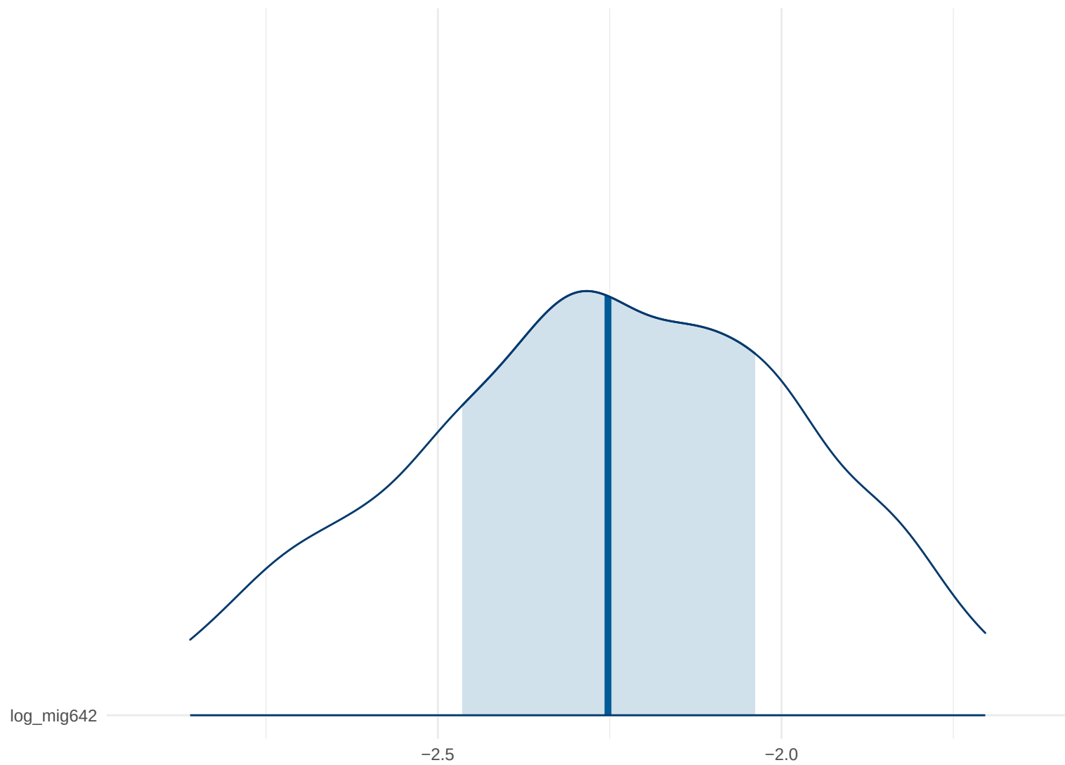
Posterior Density: log_mig642
