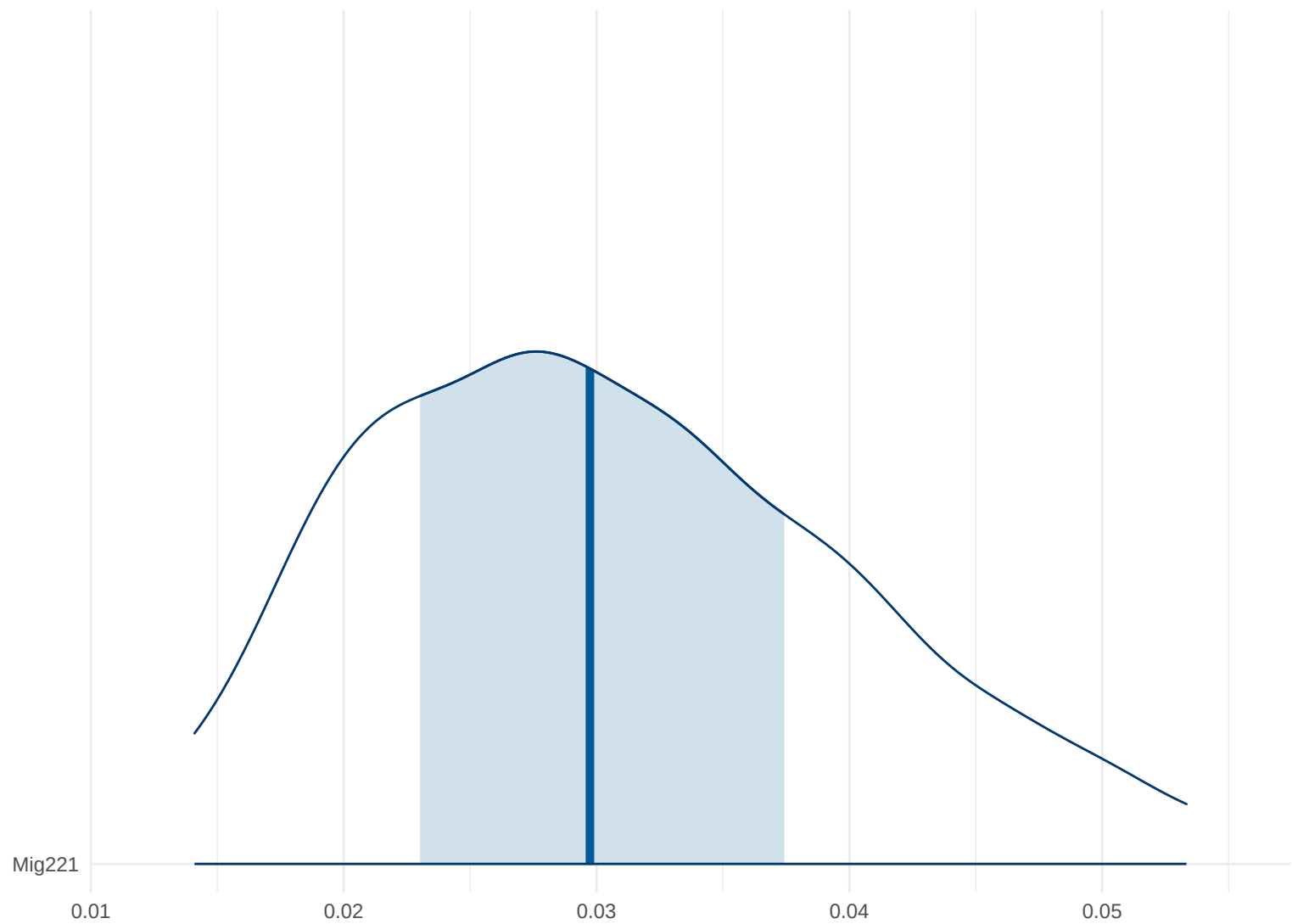
Posterior Density: Mig221
