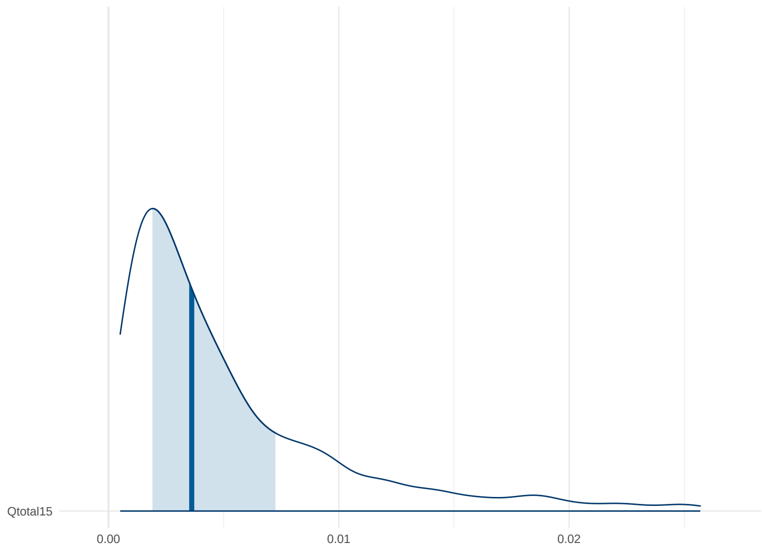
Posterior Density: Qtotal15
