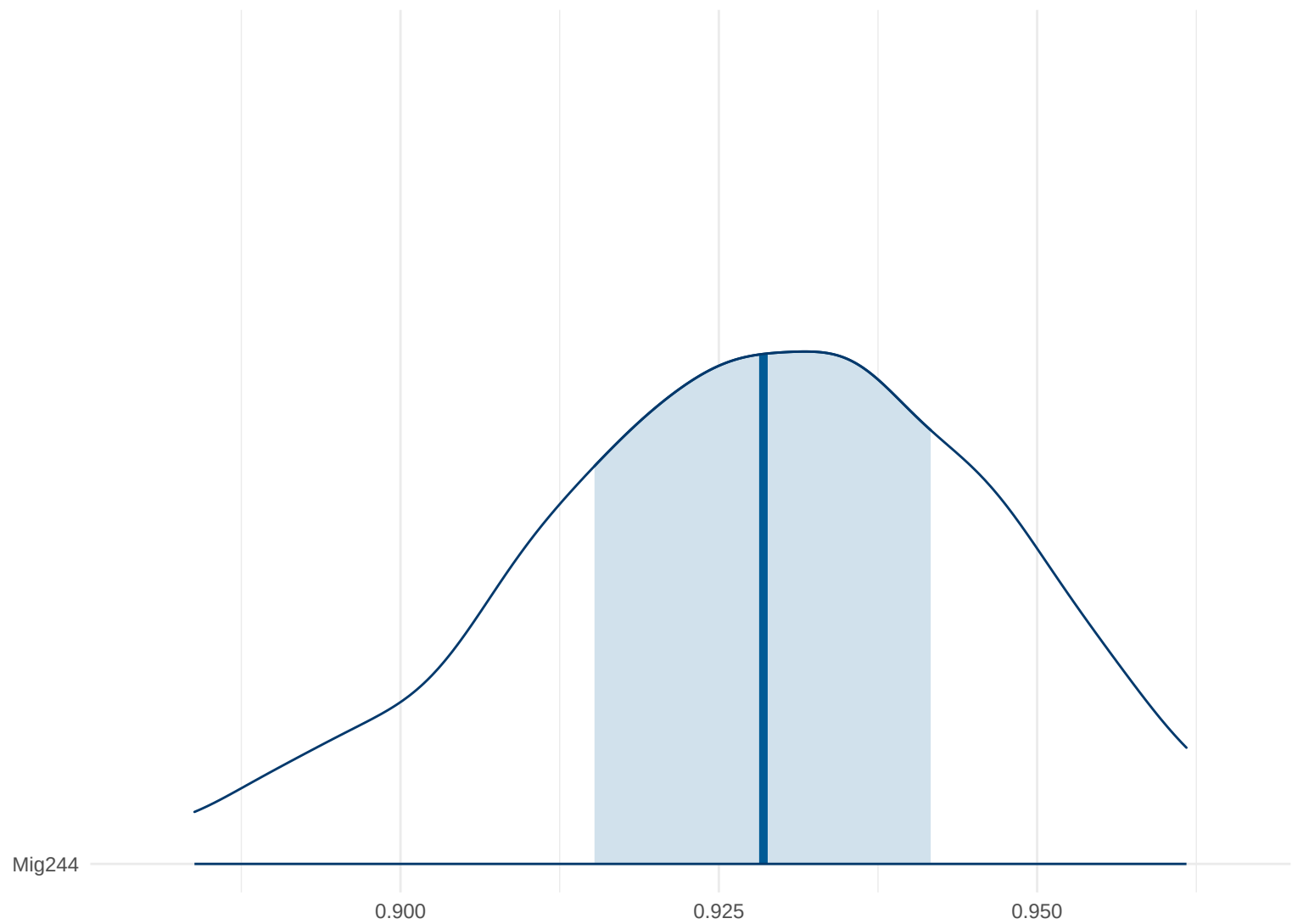
Posterior Density: Mig244
