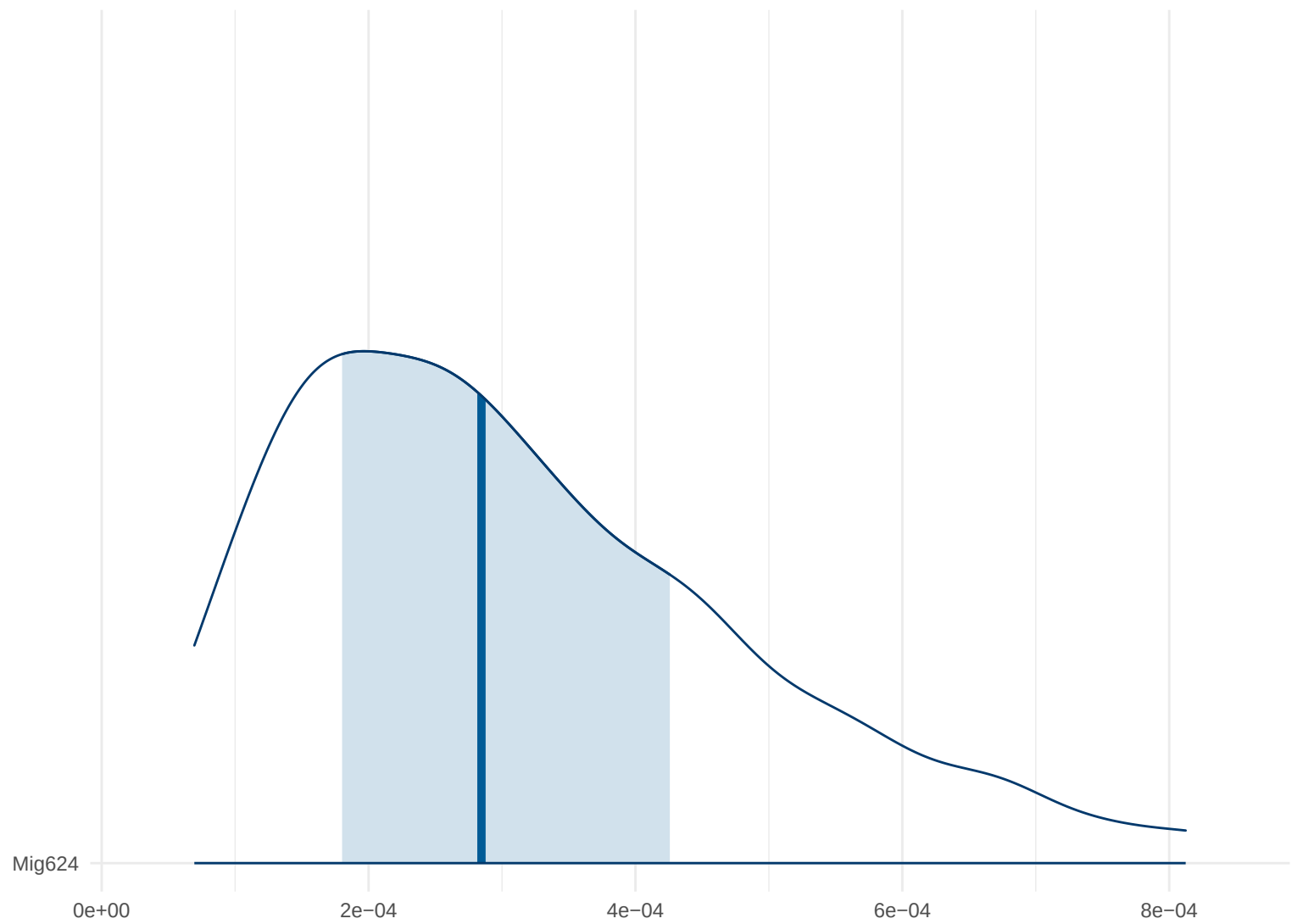
Posterior Density: Mig624
