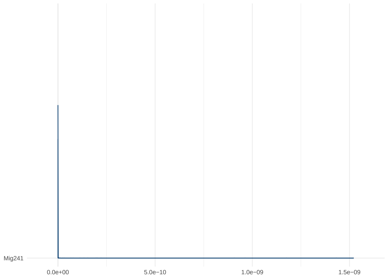
Posterior Density: Mig241
