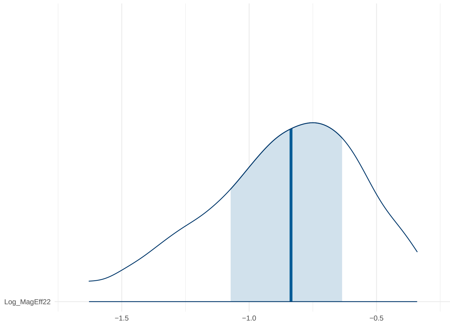
Posterior Density: Log_MagEff22
