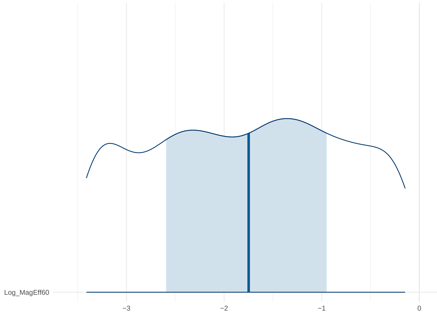
Posterior Density: Log_MagEff60
