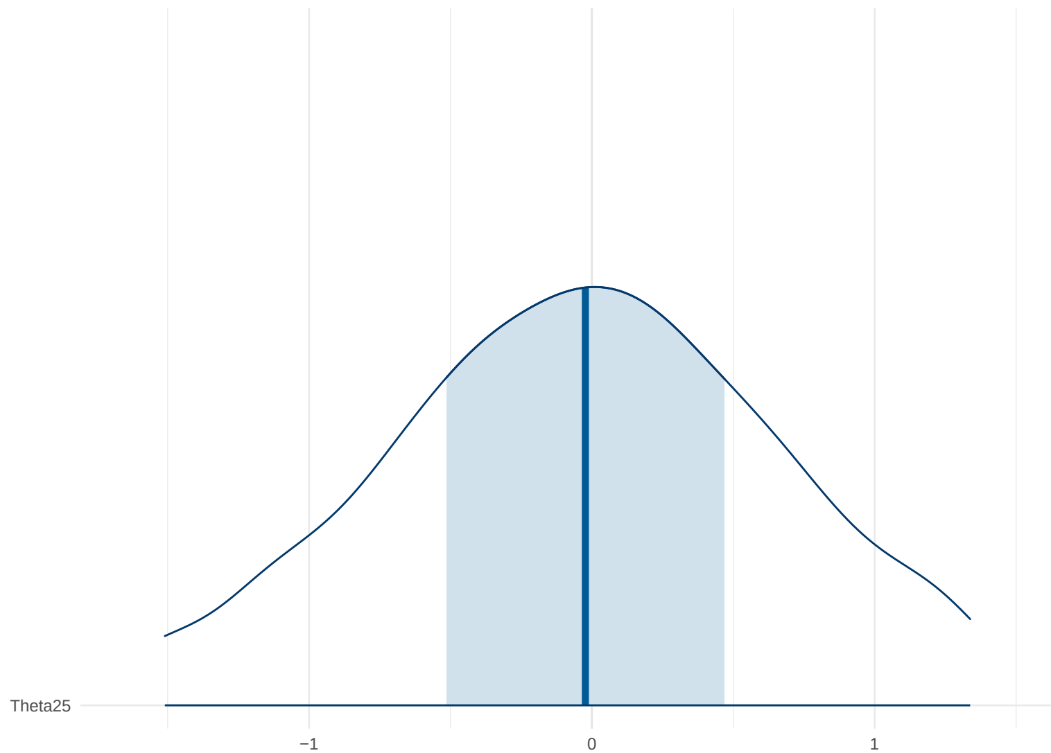
Posterior Density: Theta25
