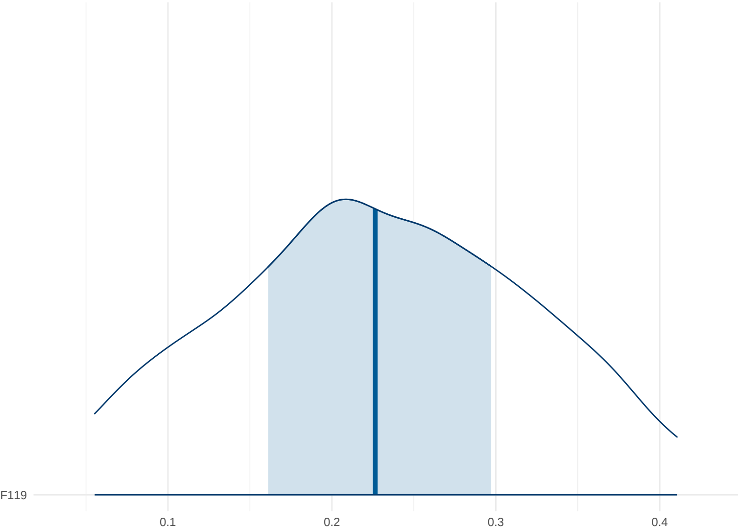
Posterior Density: F119
