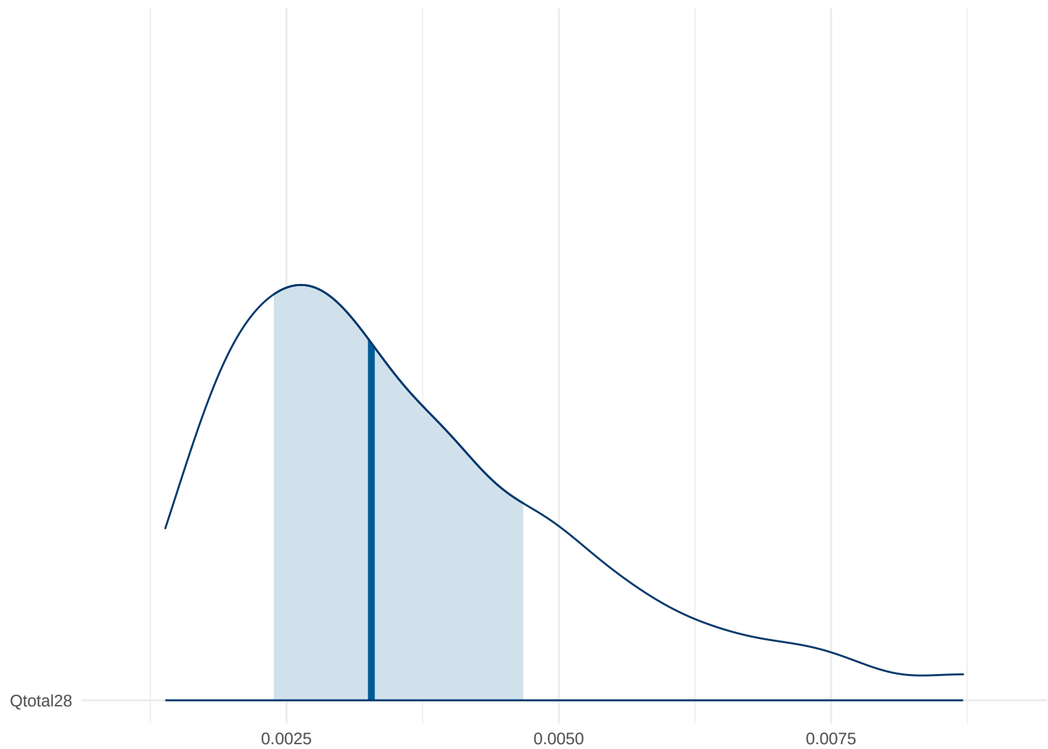
Posterior Density: Qtotal28
