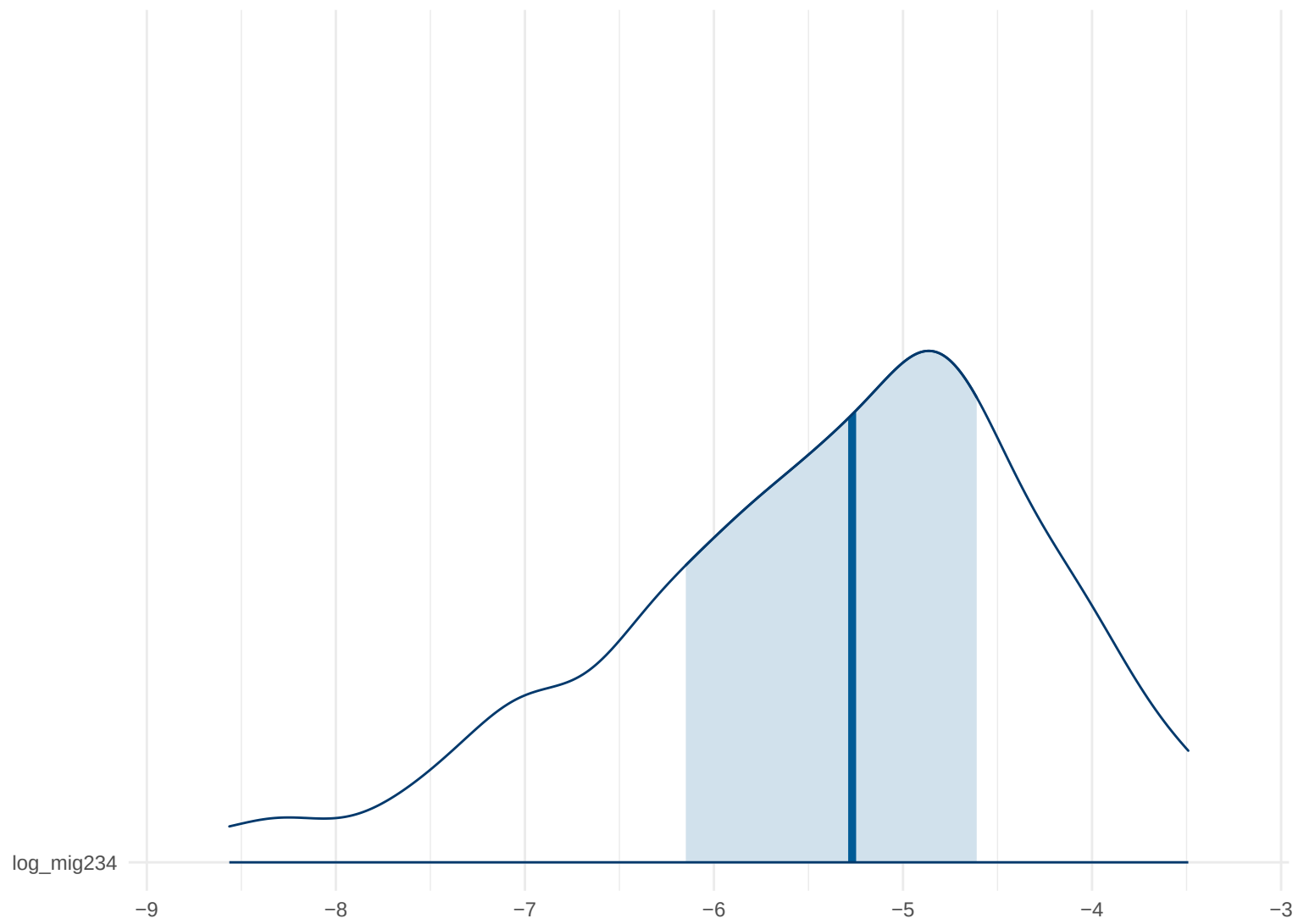
Posterior Density: log_mig234
