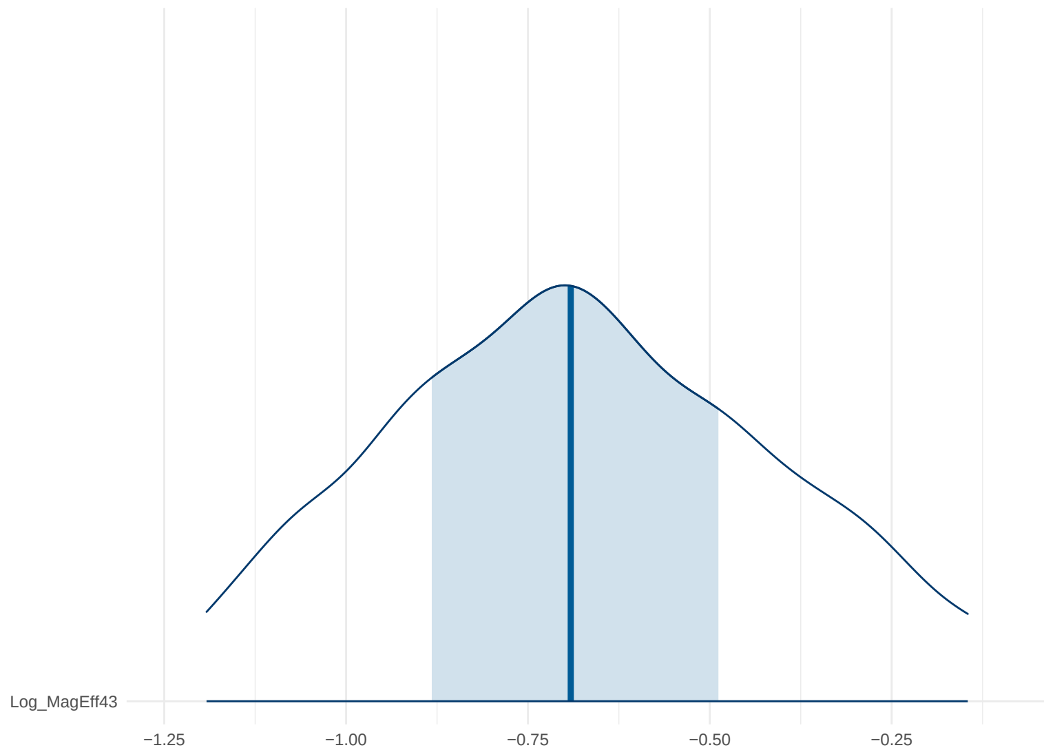
Posterior Density: Log_MagEff43
