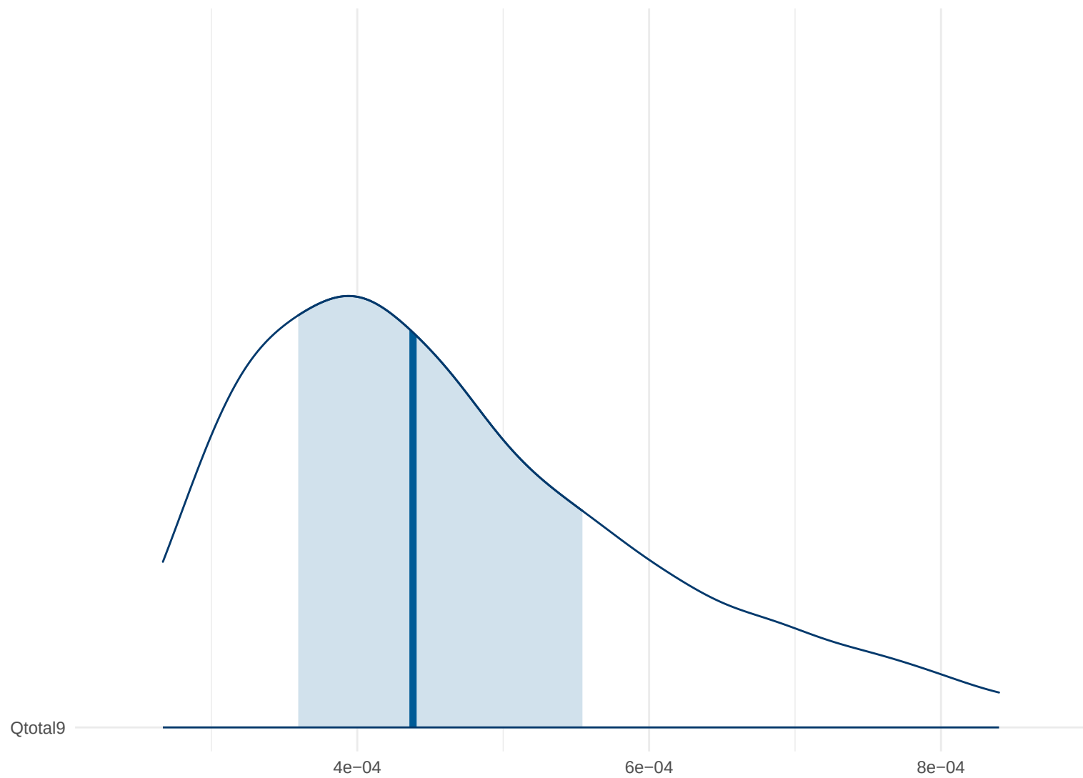
Posterior Density: Qtotal9
