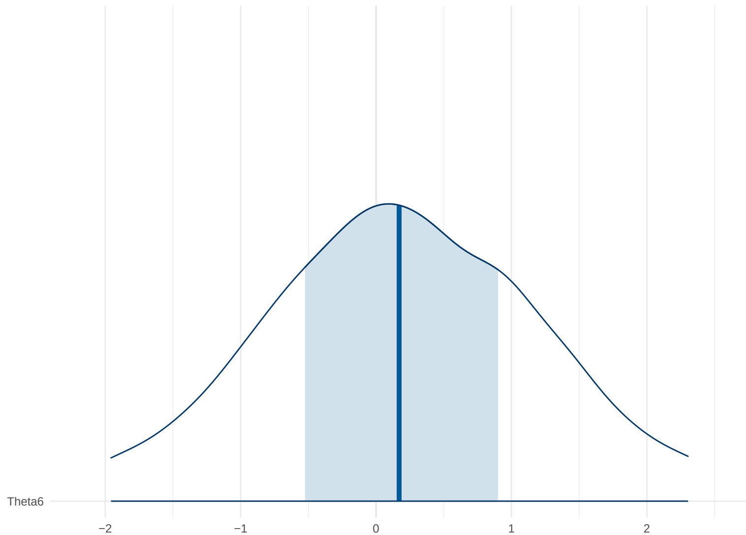
Posterior Density: Theta6
