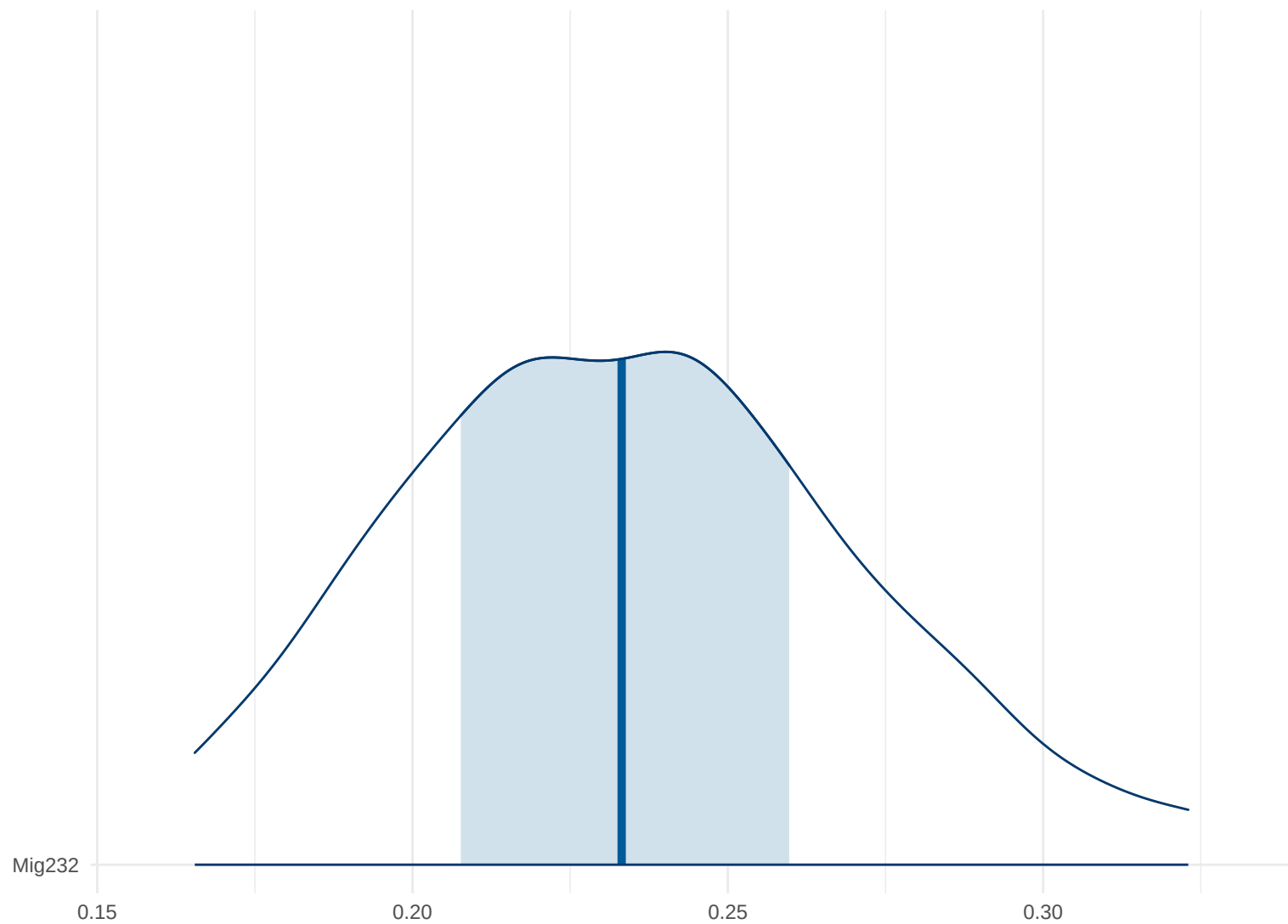
Posterior Density: Mig232
