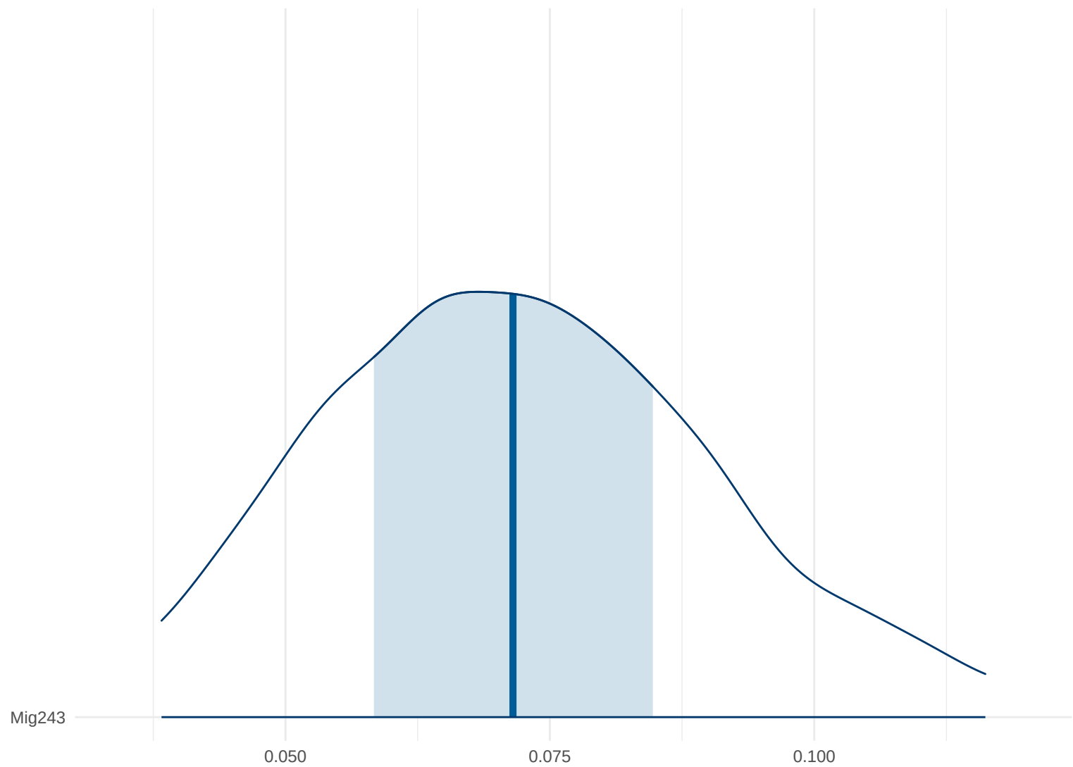
Posterior Density: Mig243
