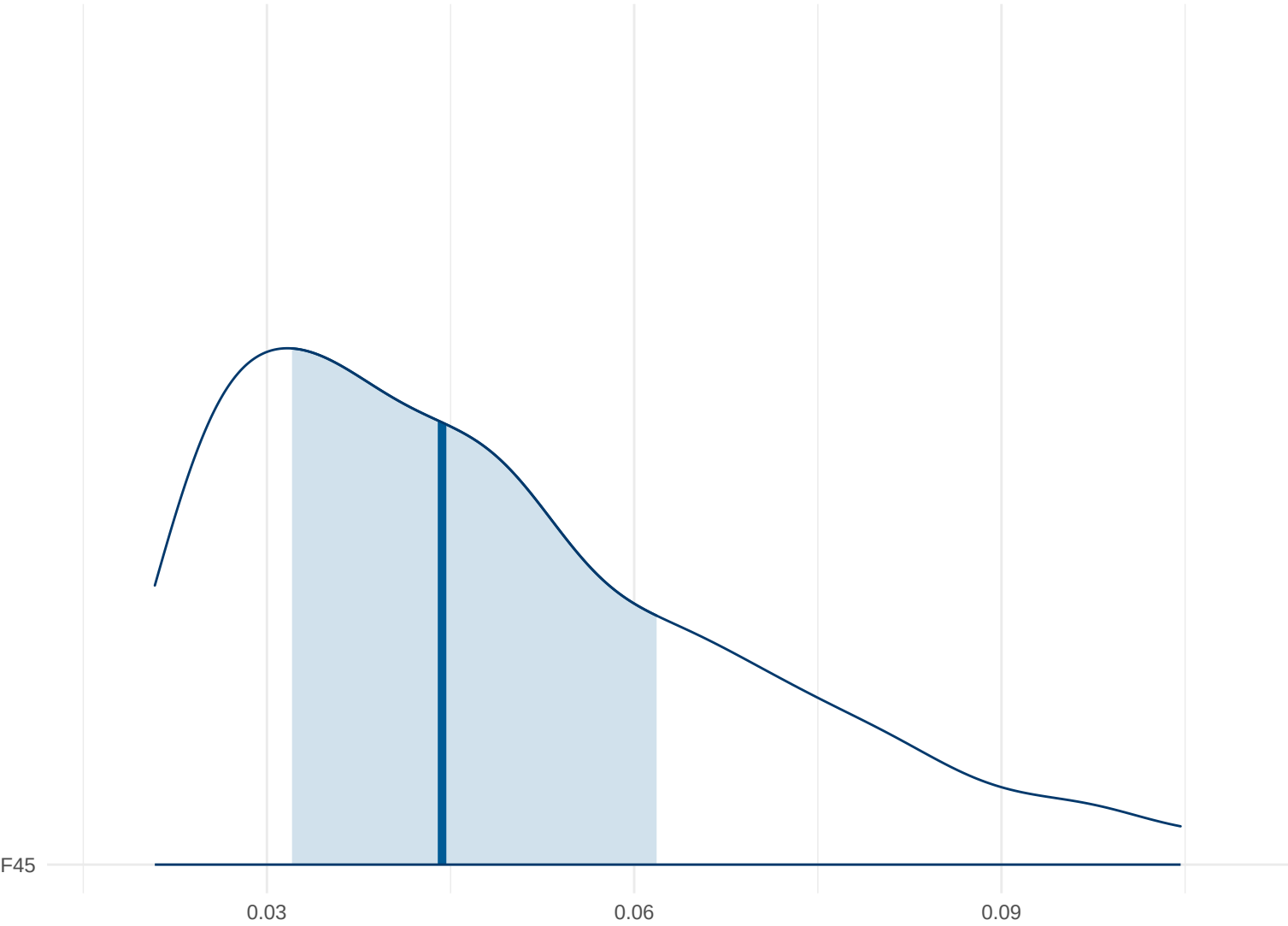
Posterior Density: F45
