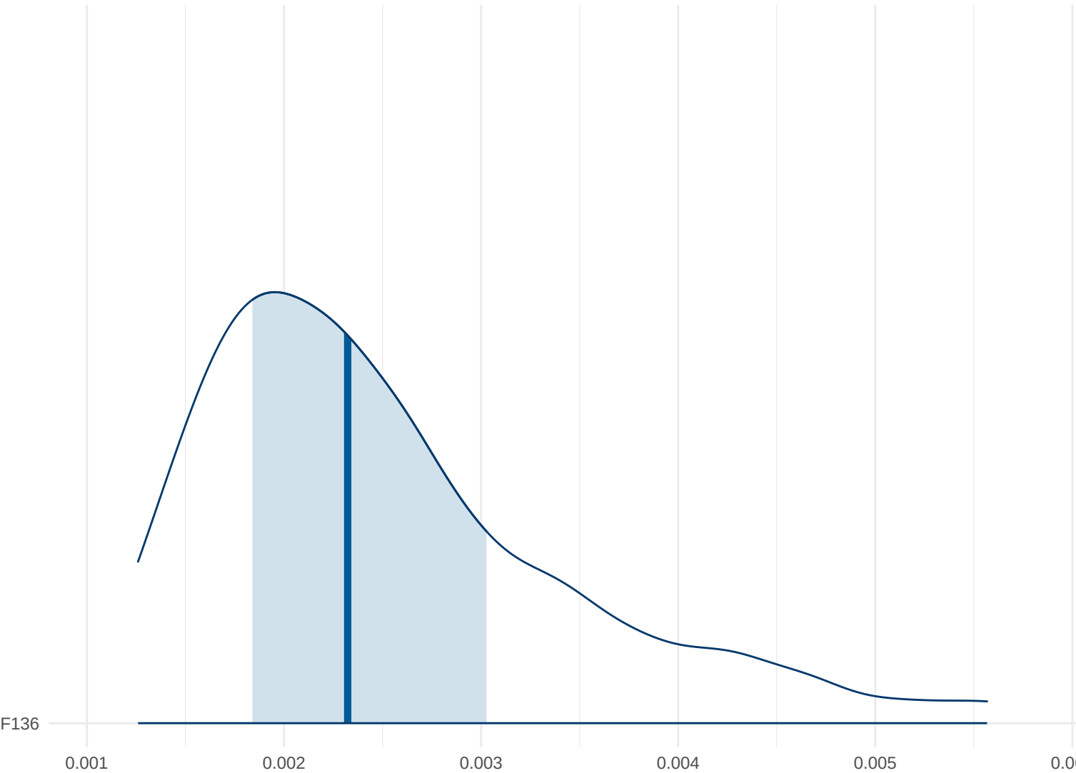
Posterior Density: F136
