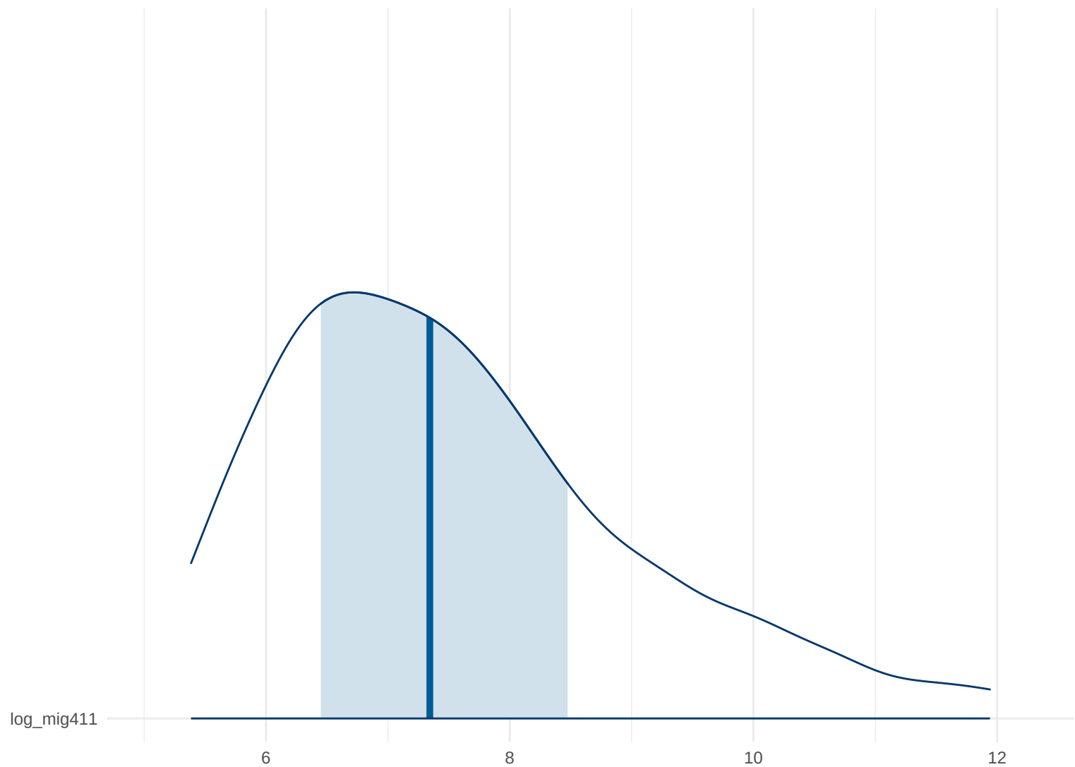
Posterior Density: log_mig411
