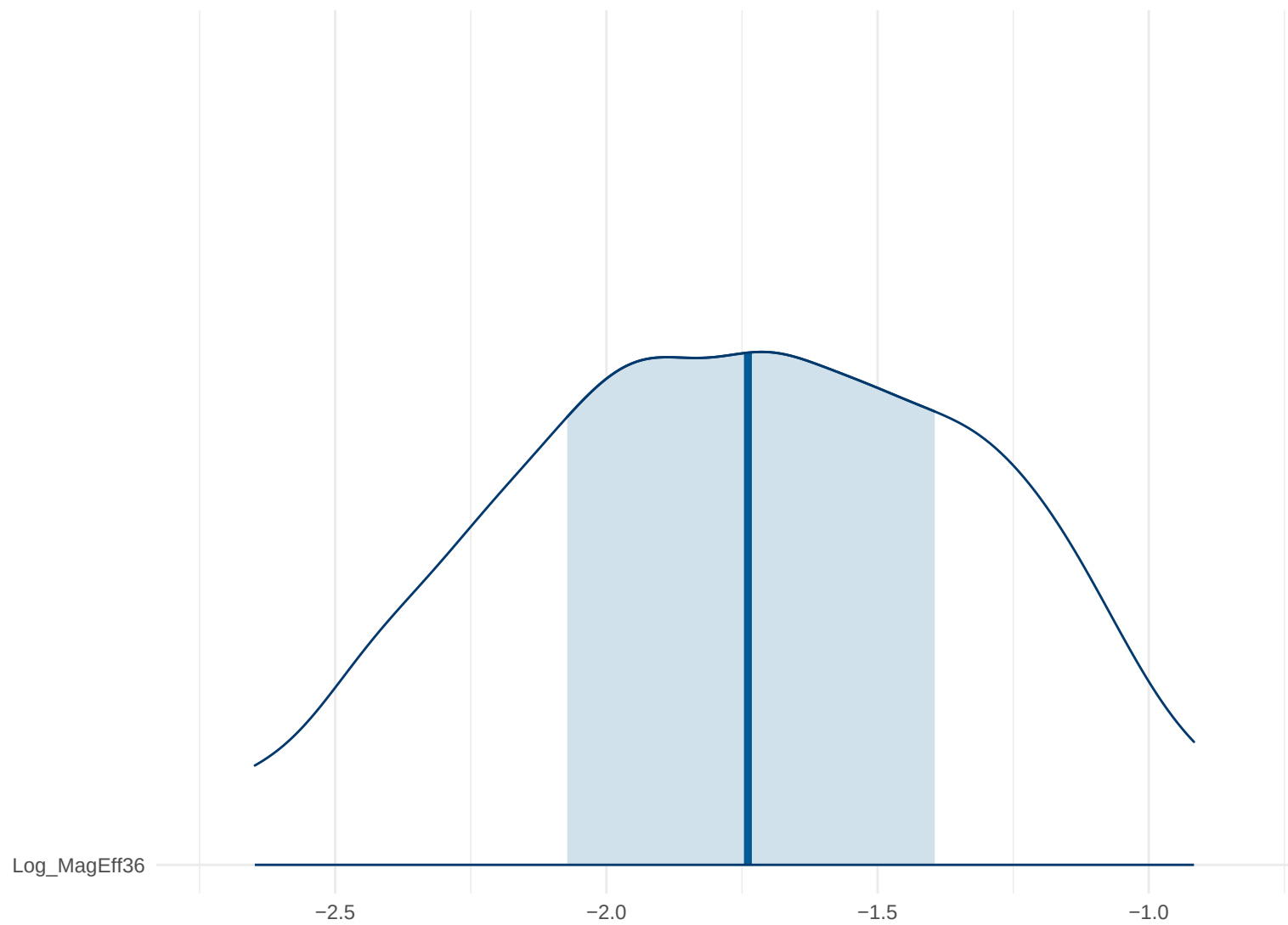
Posterior Density: Log_MagEff36
