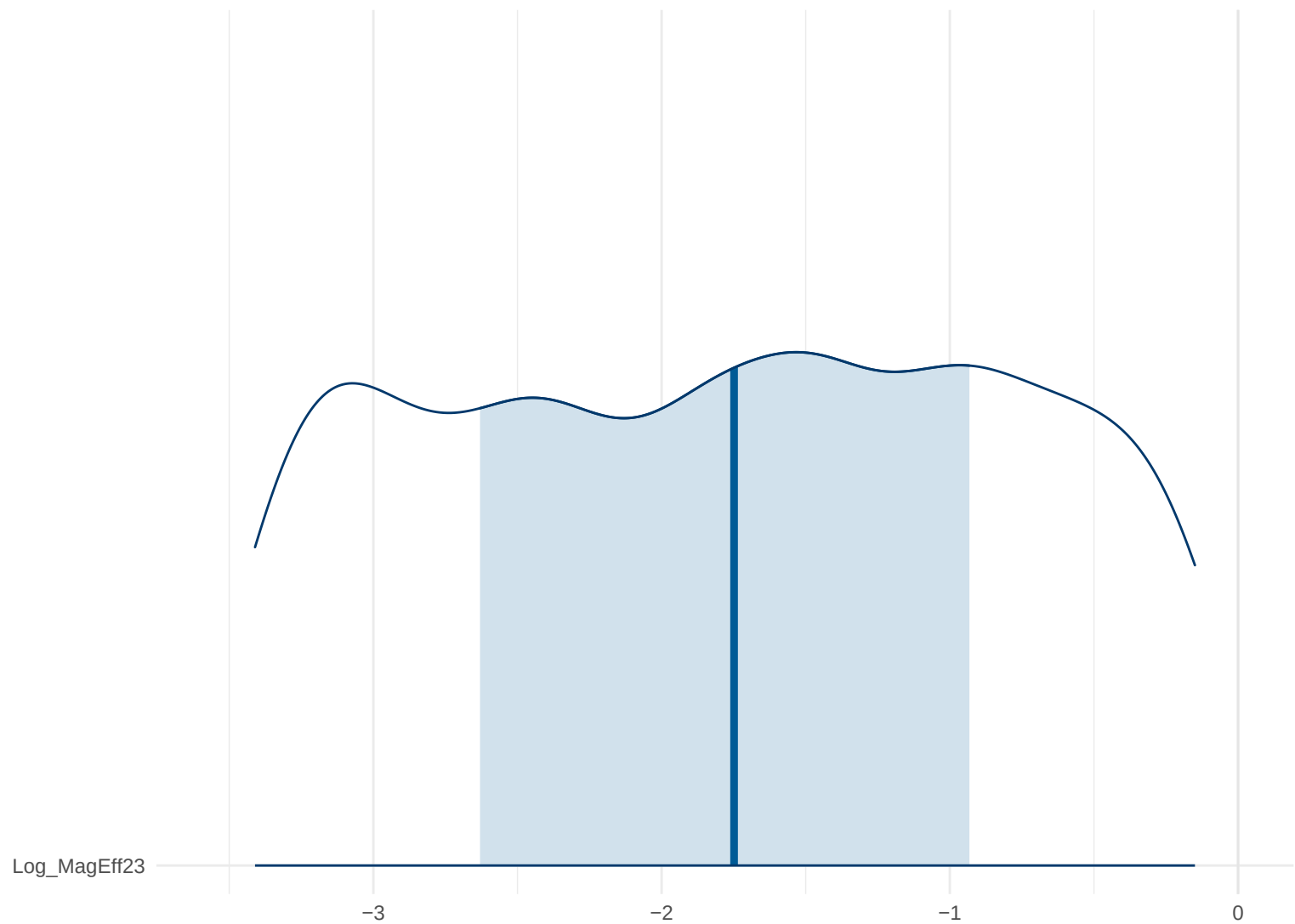
Posterior Density: Log_MagEff23
