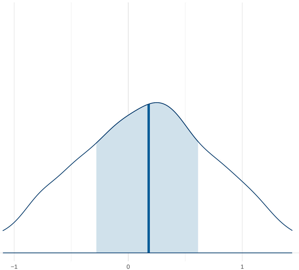
Posterior Density: Theta24
