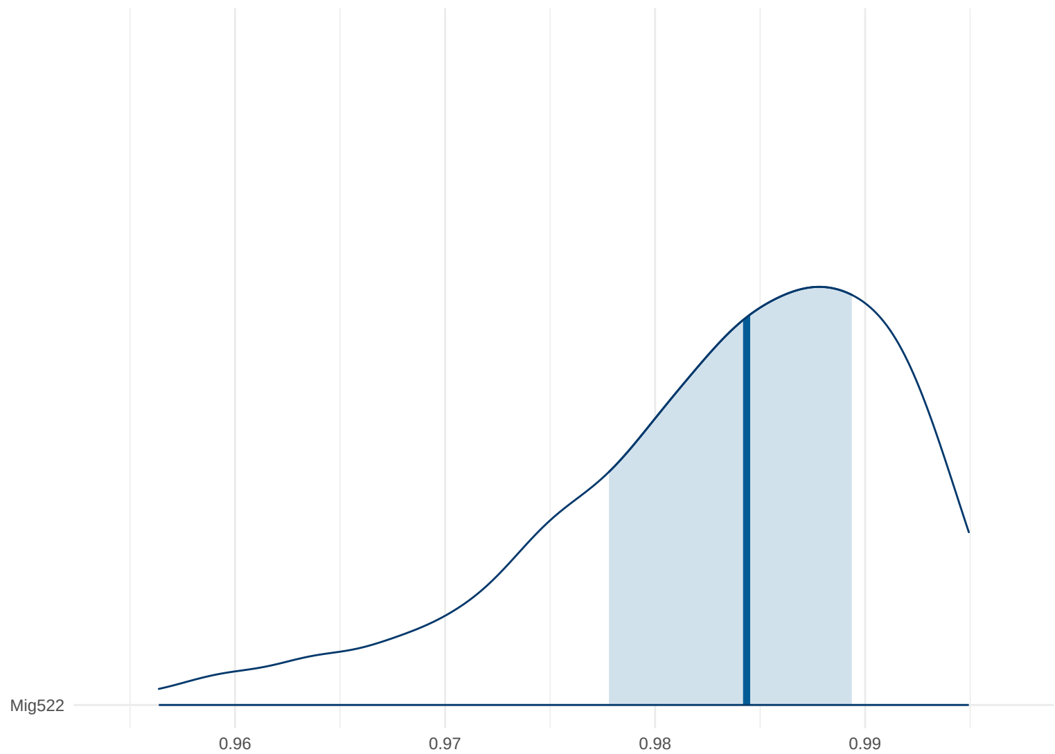
Posterior Density: Mig522
