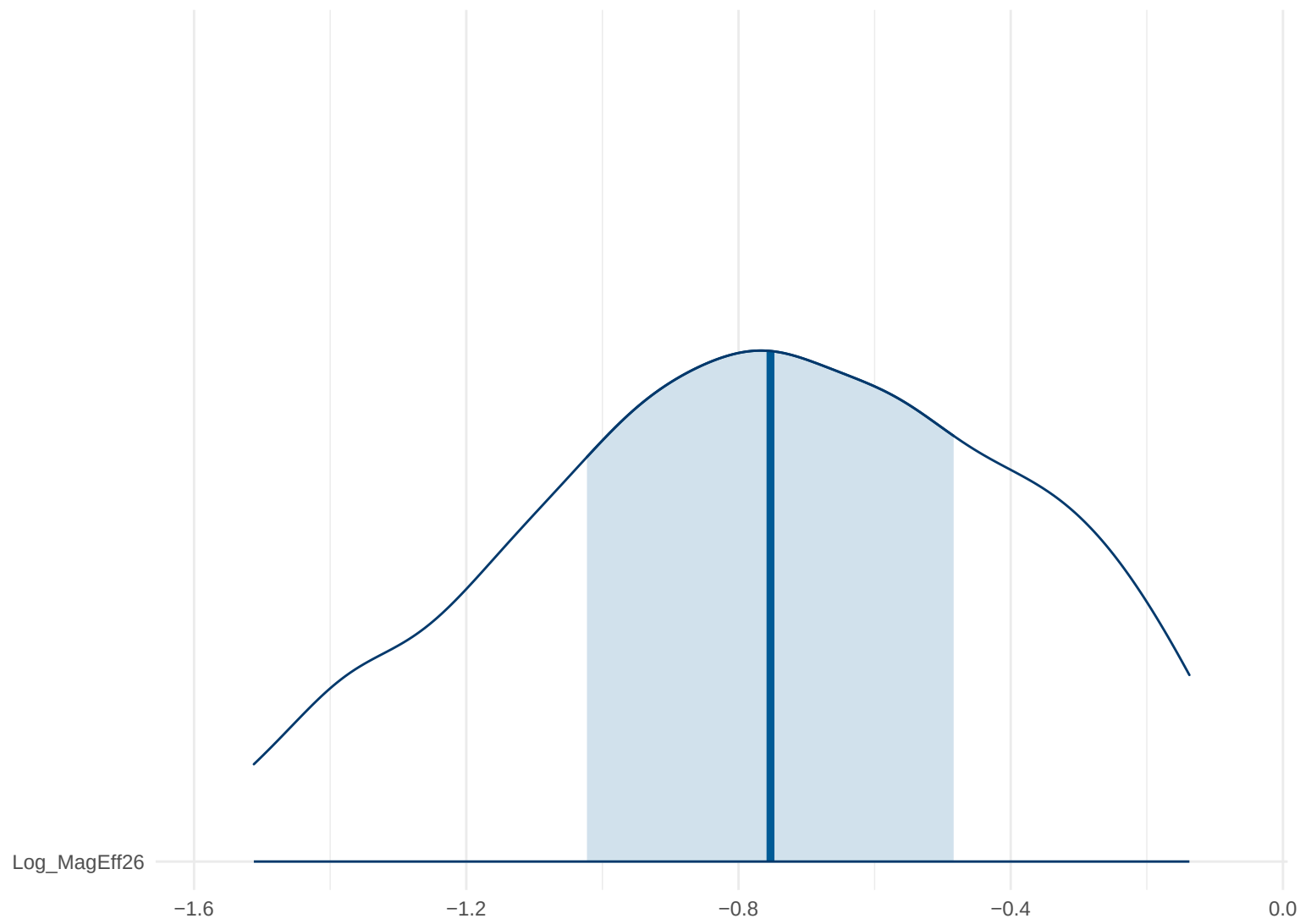
Posterior Density: Log_MagEff26
