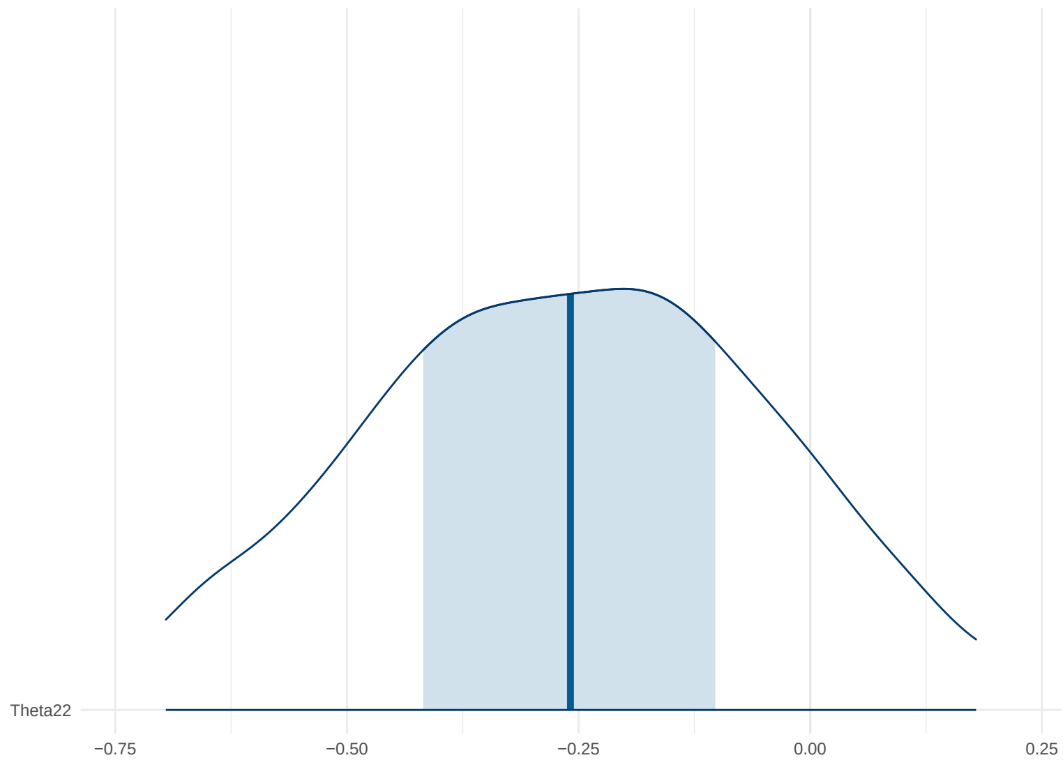
Posterior Density: Theta22
