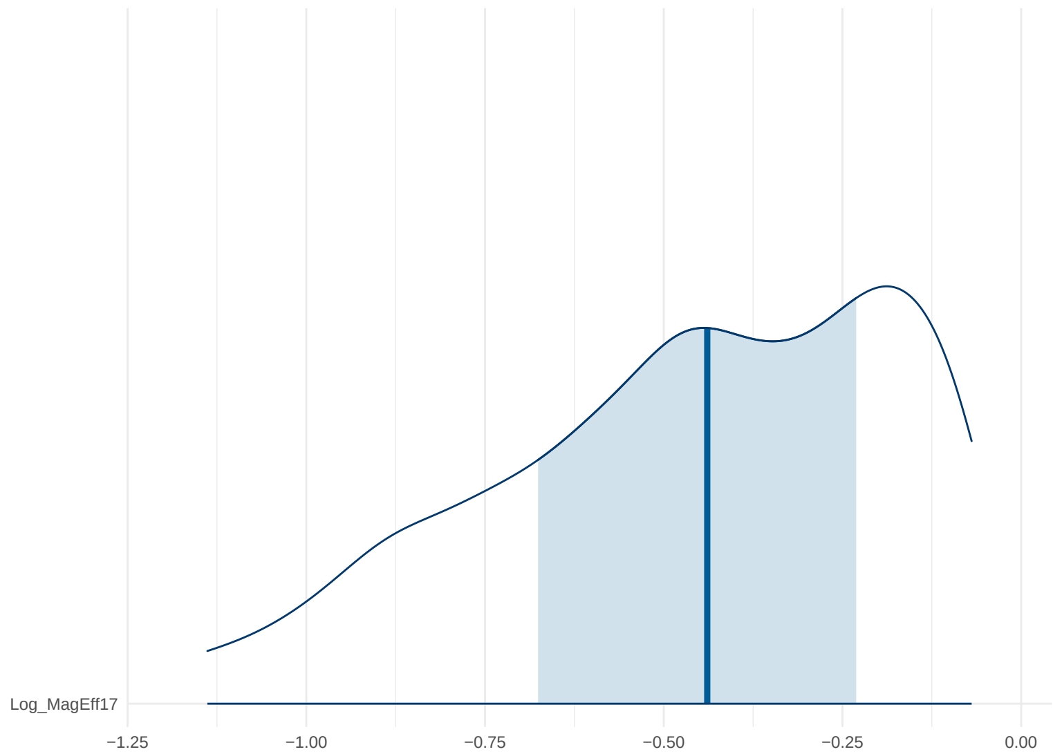
Posterior Density: Log_MagEff17
