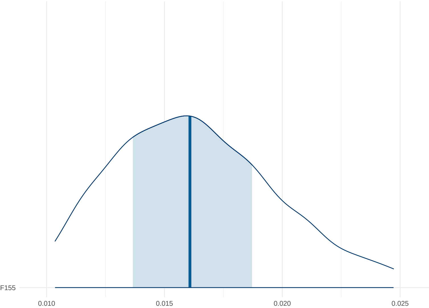
Posterior Density: F155
