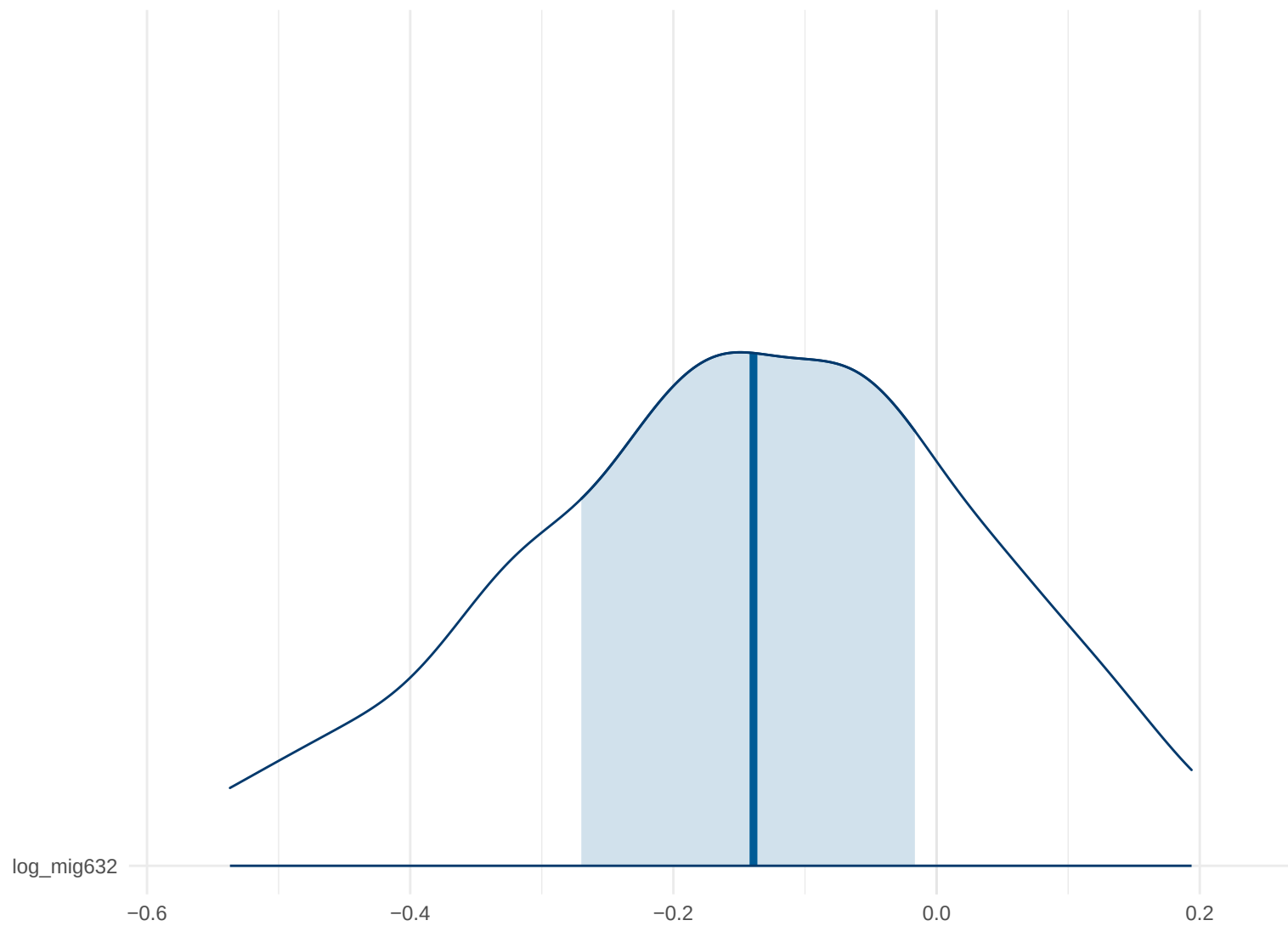
Posterior Density: log_mig632
