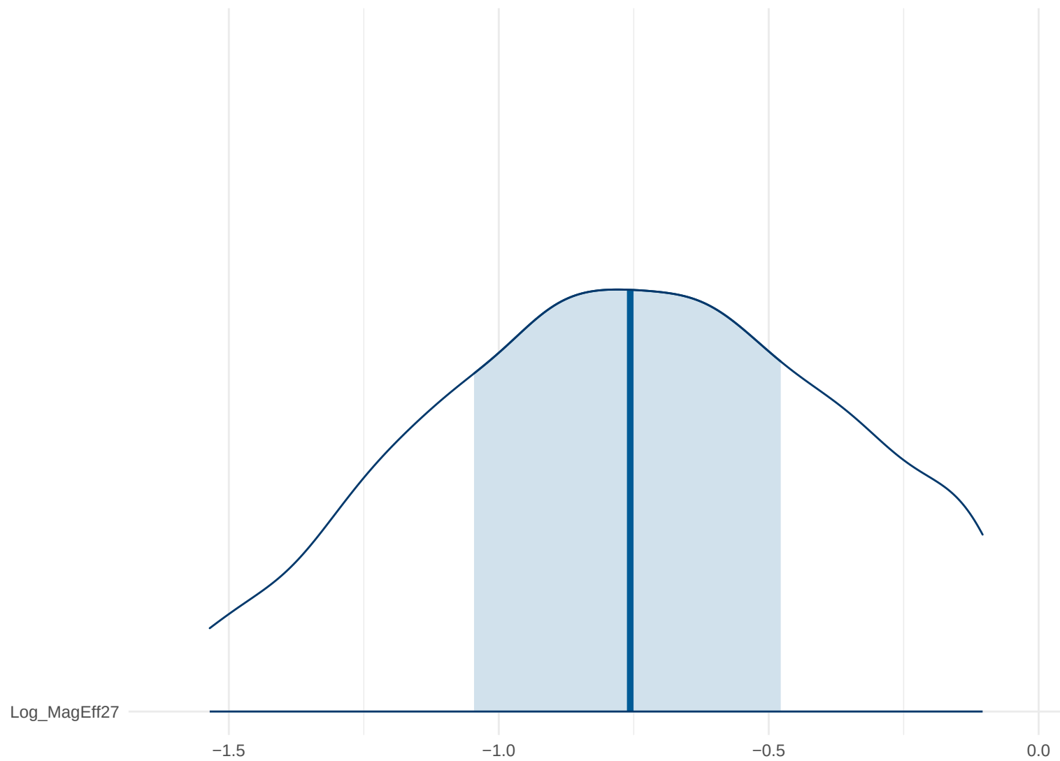
Posterior Density: Log_MagEff27
