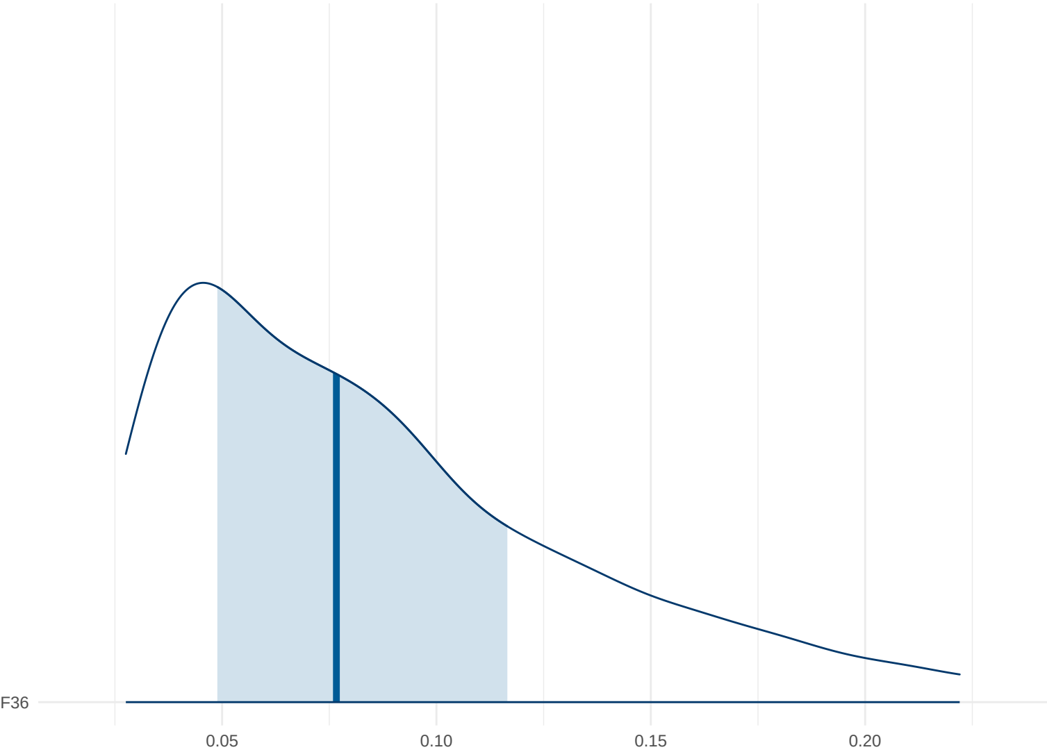
Posterior Density: F36
