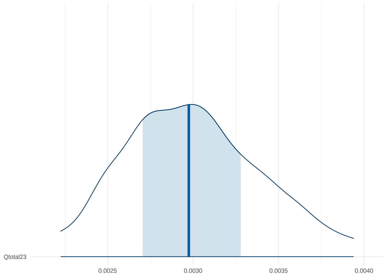
Posterior Density: Qtotal23
