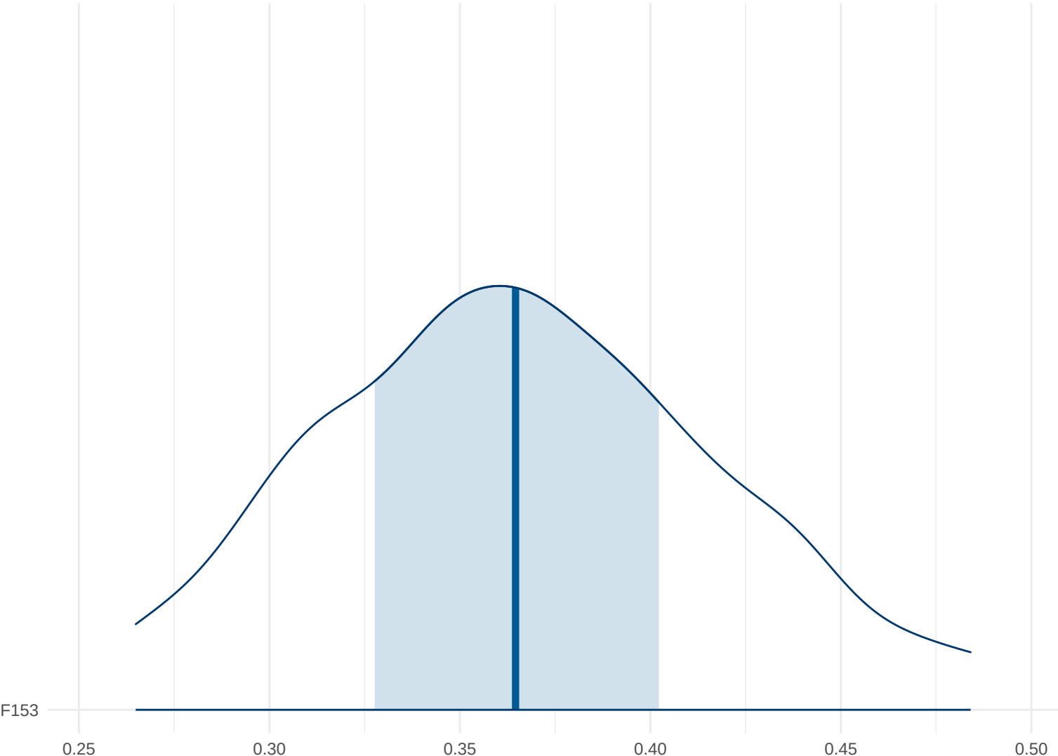
Posterior Density: F153
