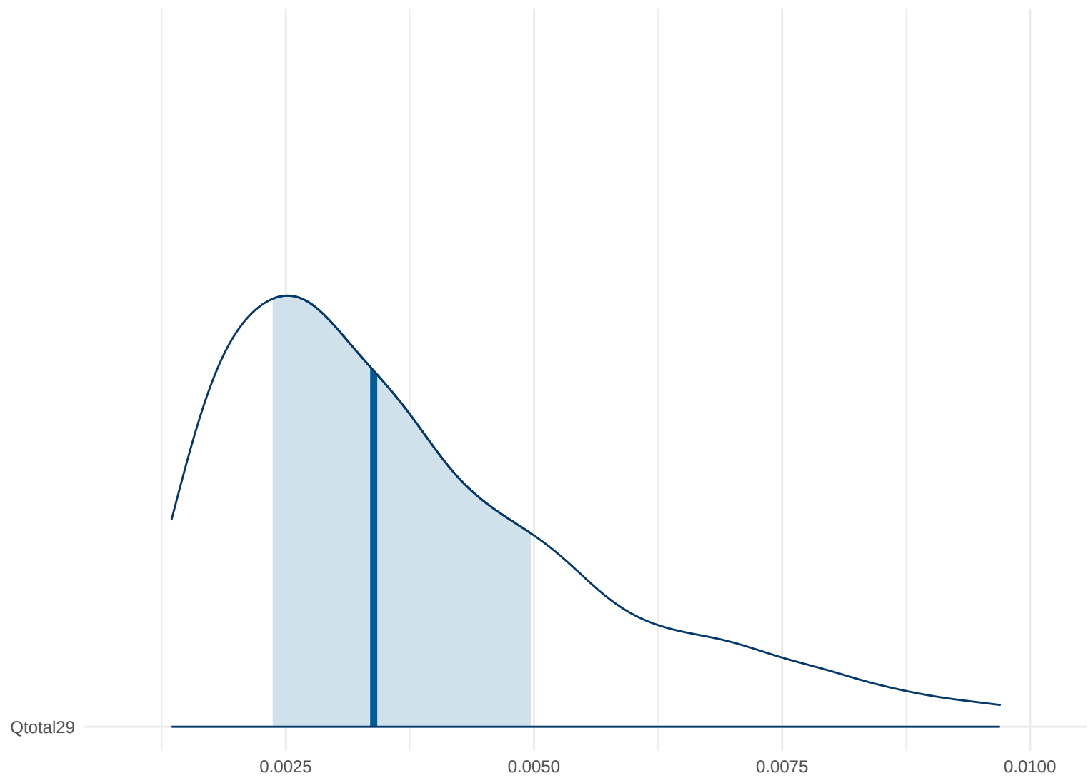
Posterior Density: Qtotal29
