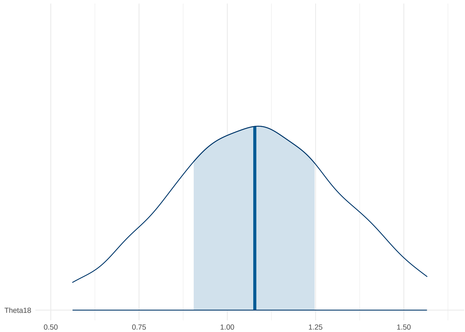
Posterior Density: Theta18
