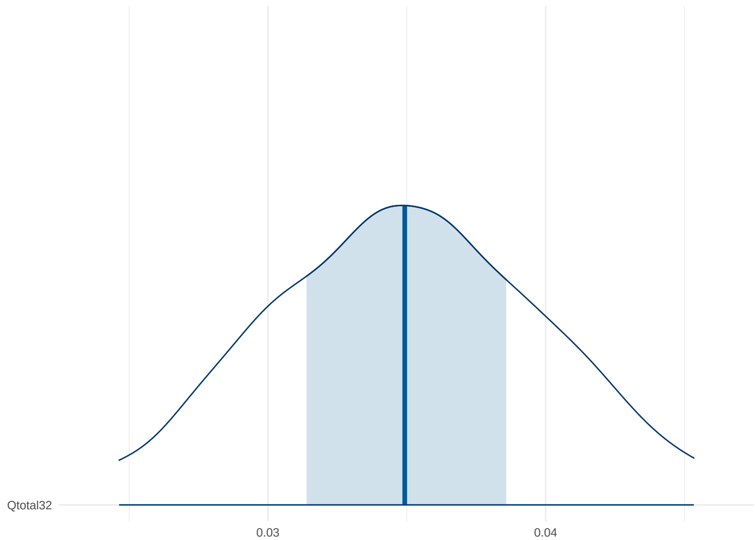
Posterior Density: Qtotal32
