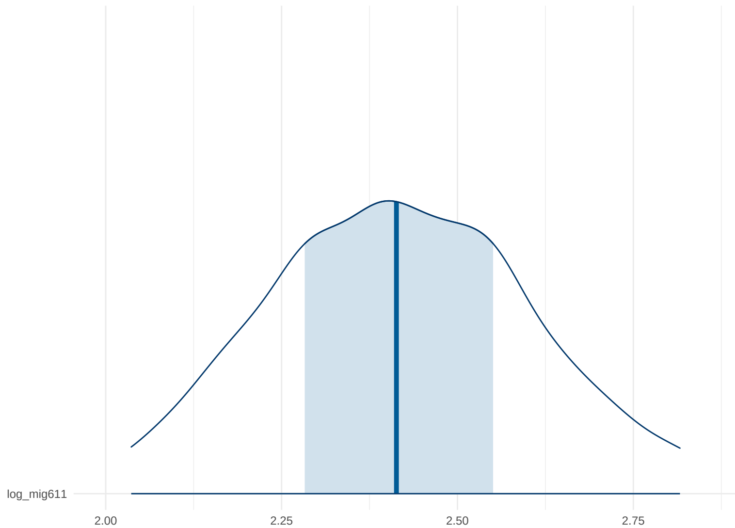
Posterior Density: log_mig611
