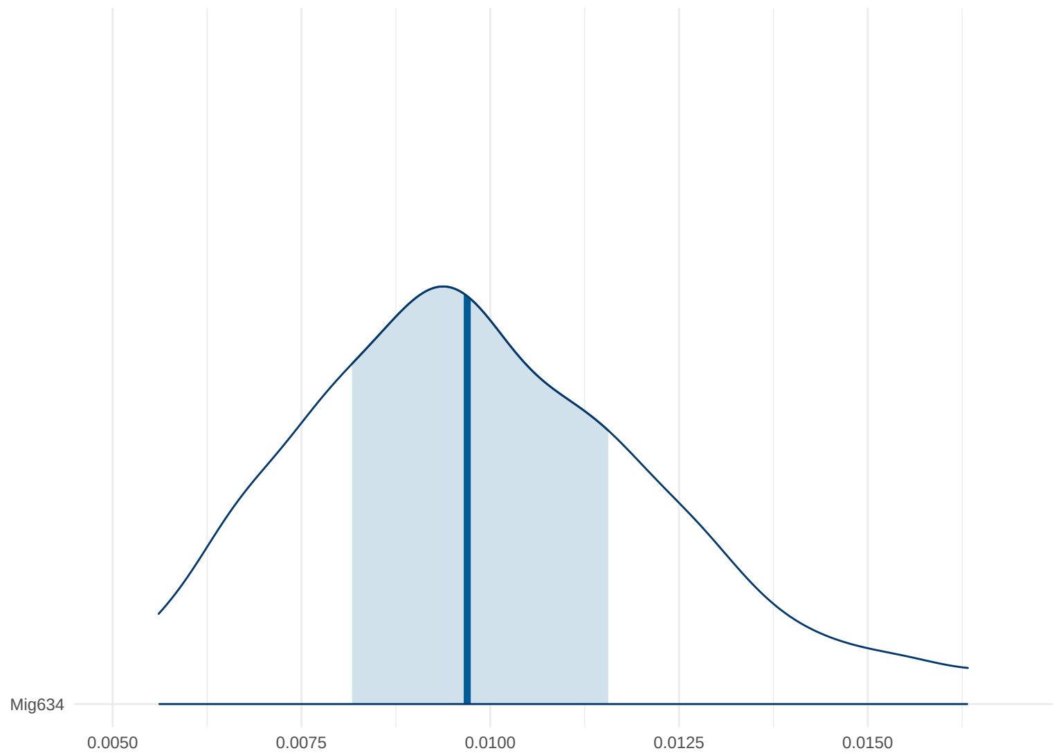
Posterior Density: Mig634
