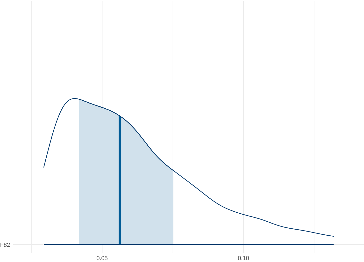
Posterior Density: F82
