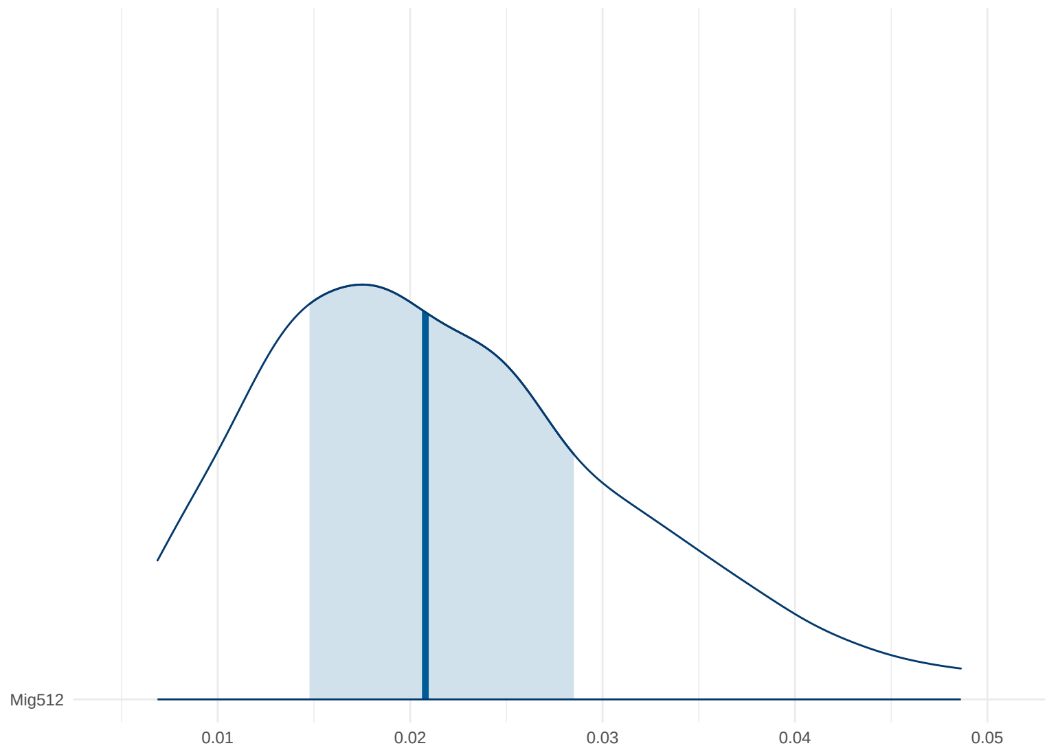
Posterior Density: Mig512
