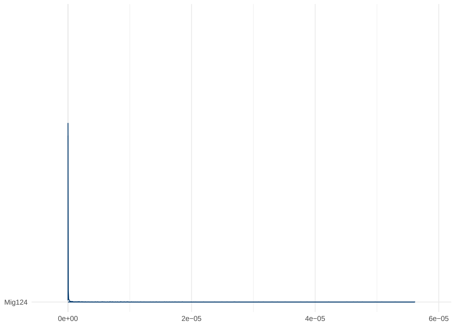
Posterior Density: Mig124
