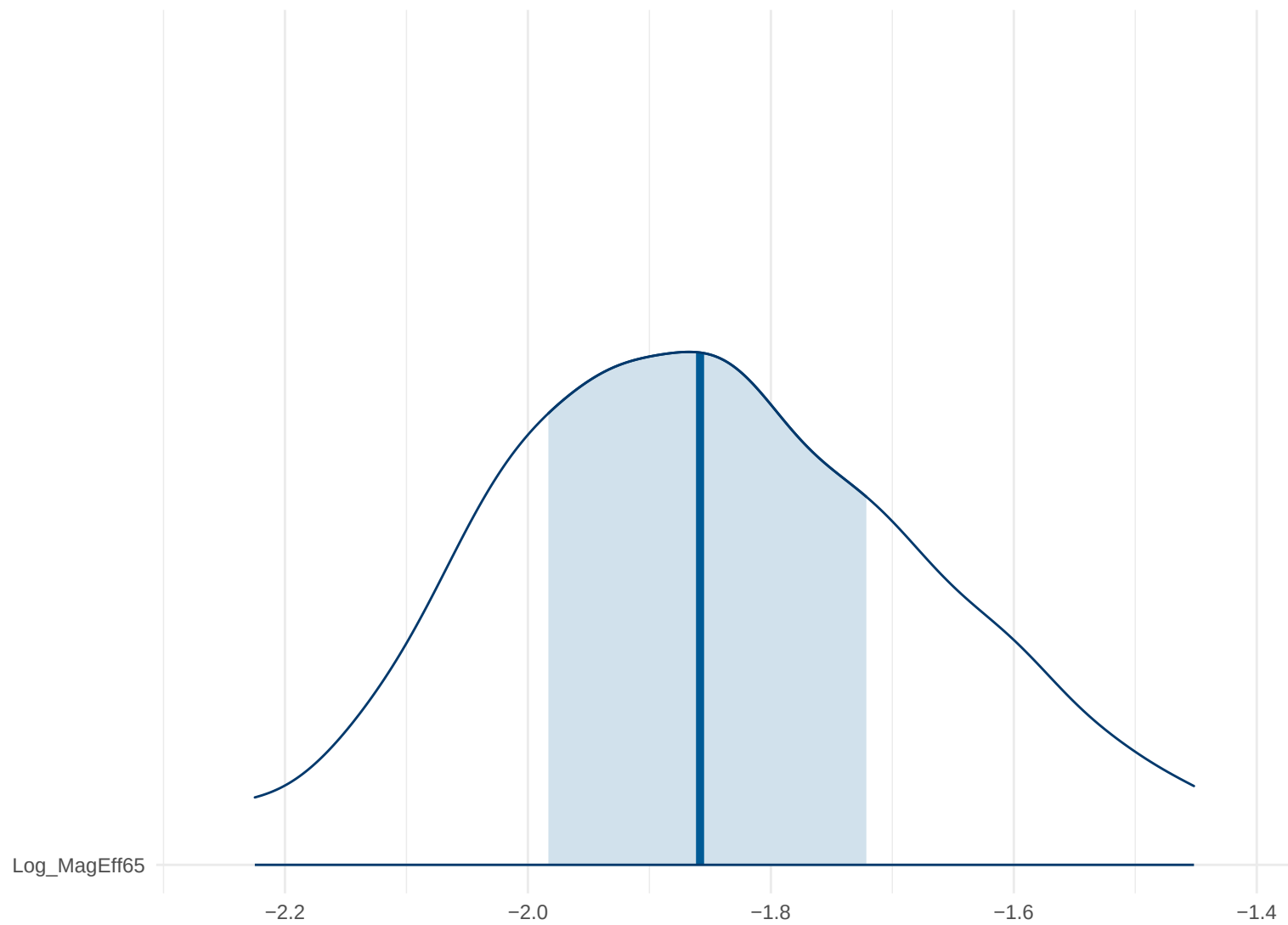
Posterior Density: Log_MagEff65
