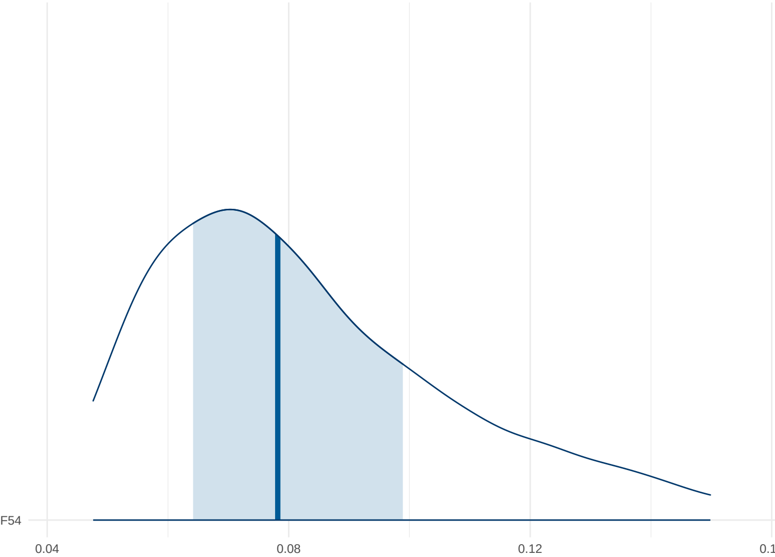
Posterior Density: F54
