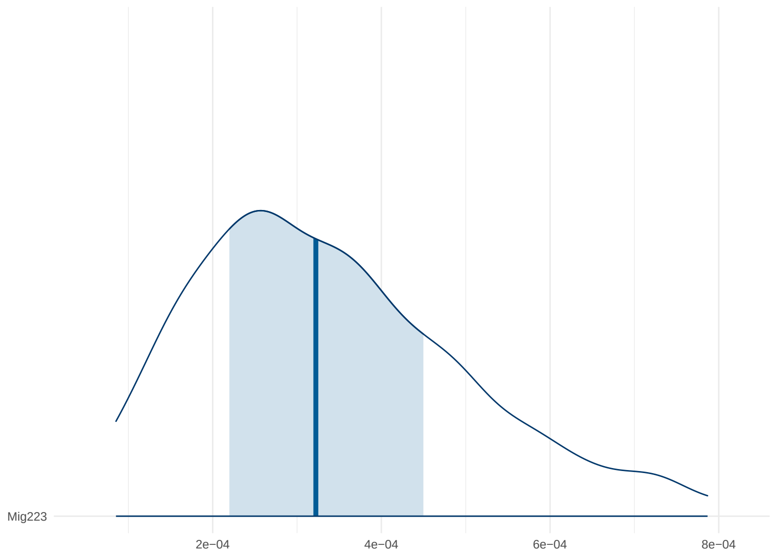
Posterior Density: Mig223
