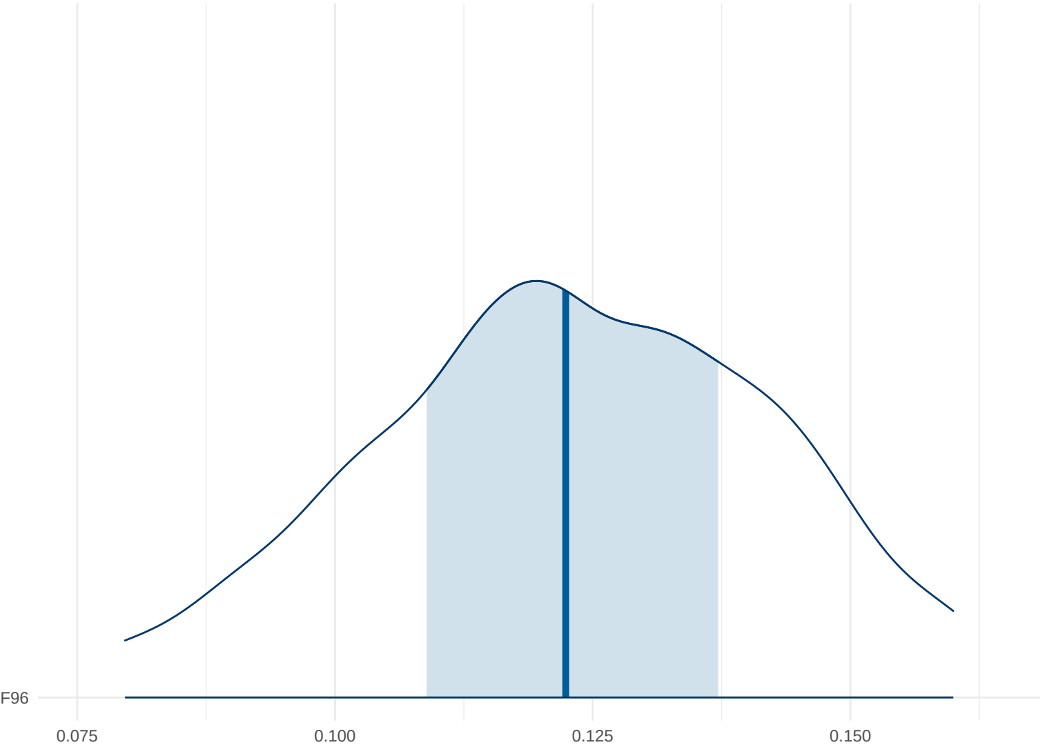
Posterior Density: F96
