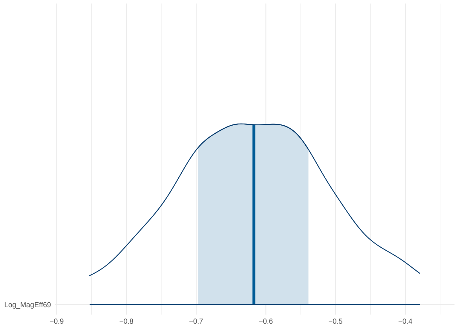
Posterior Density: Log_MagEff69
