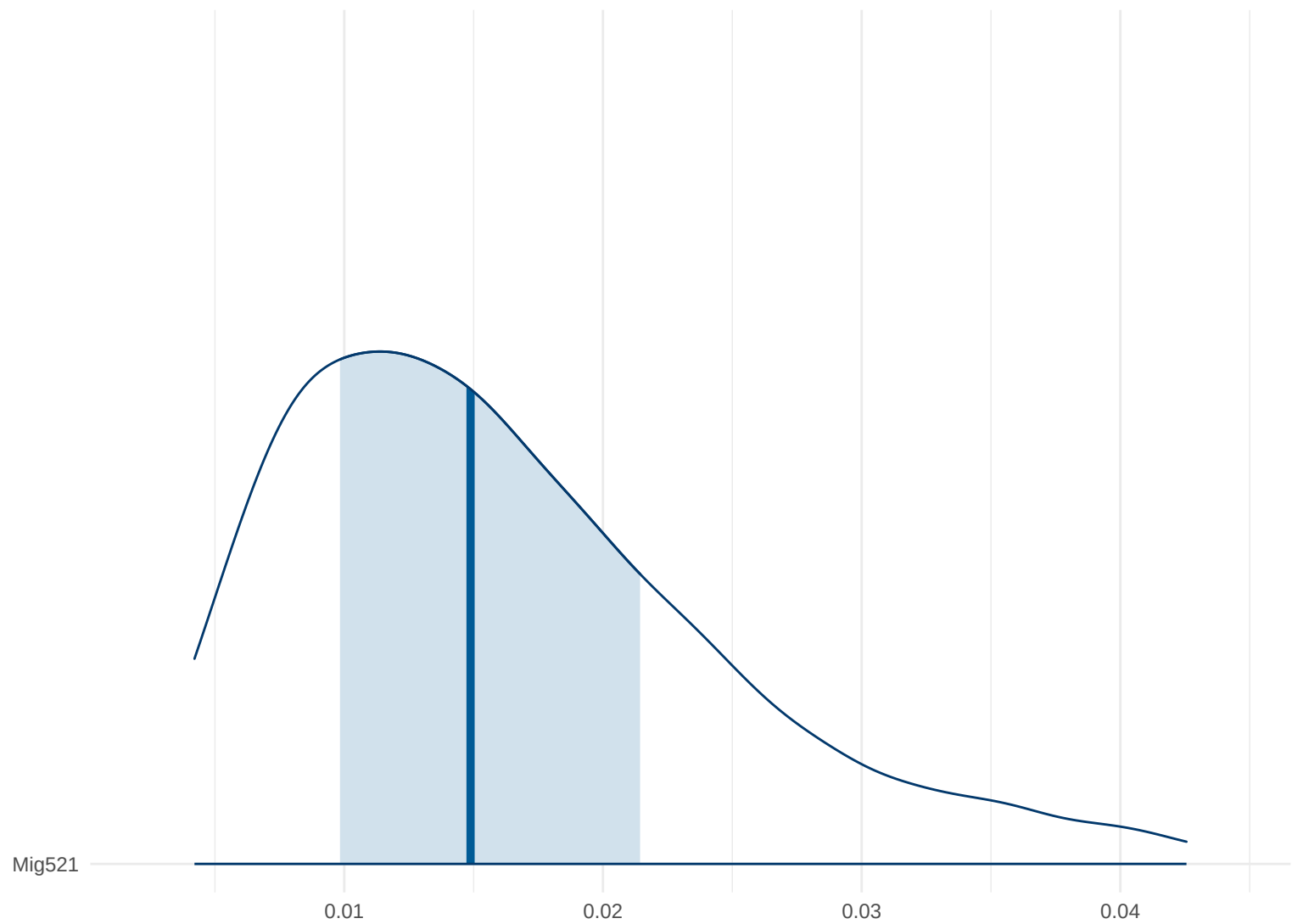
Posterior Density: Mig521
