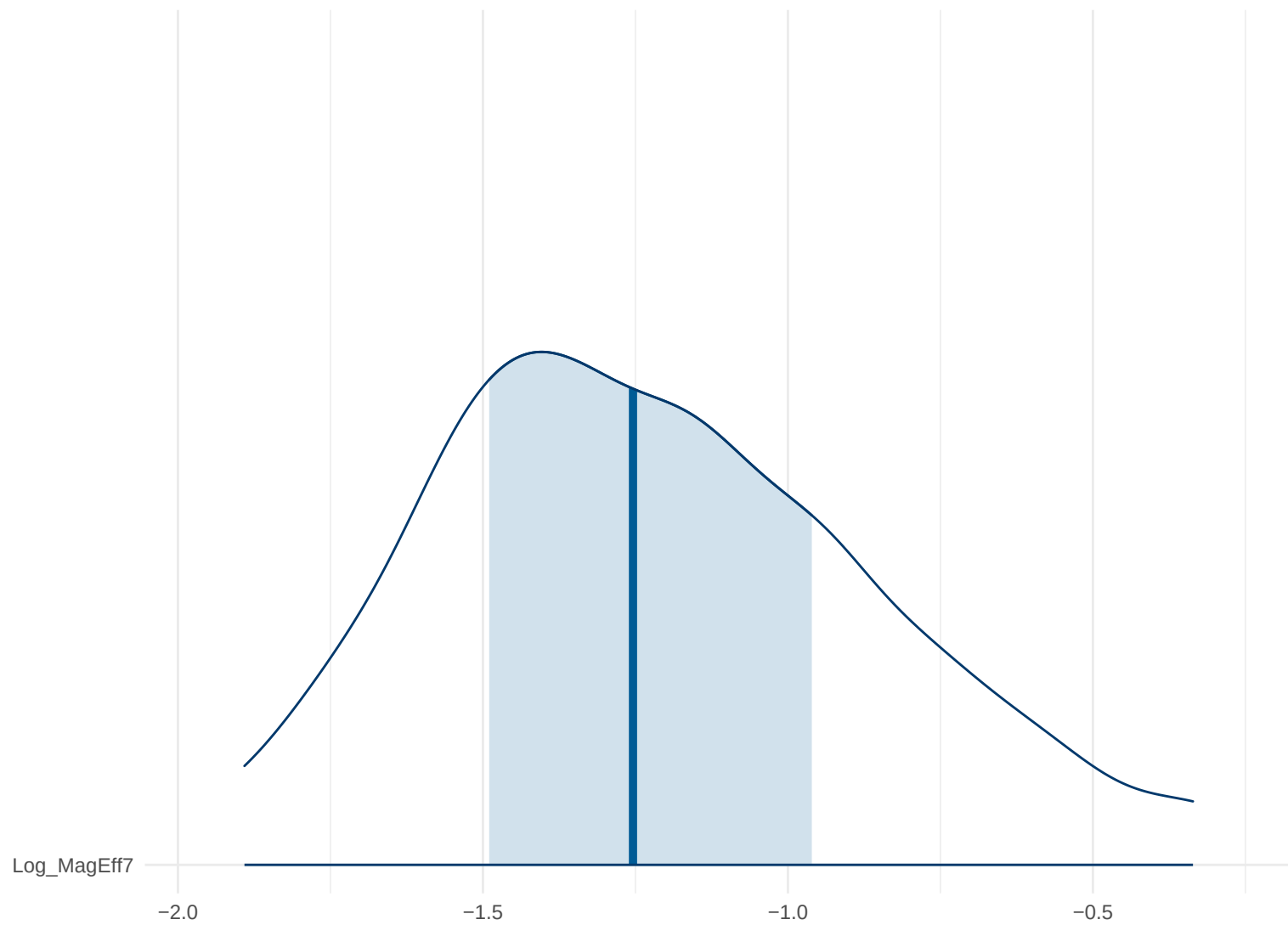
Posterior Density: Log_MagEff7
