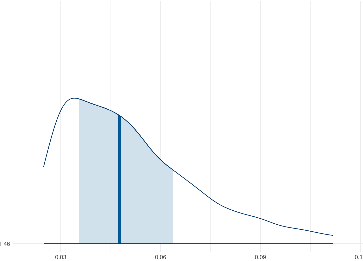
Posterior Density: F46
