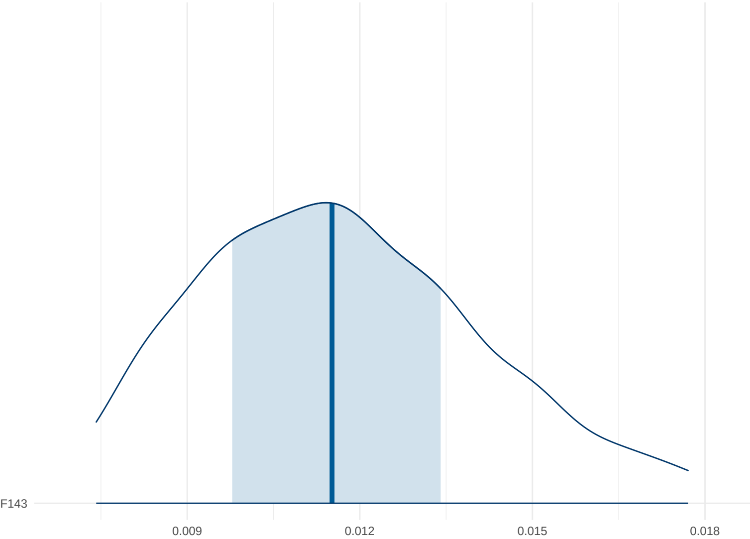
Posterior Density: F143
