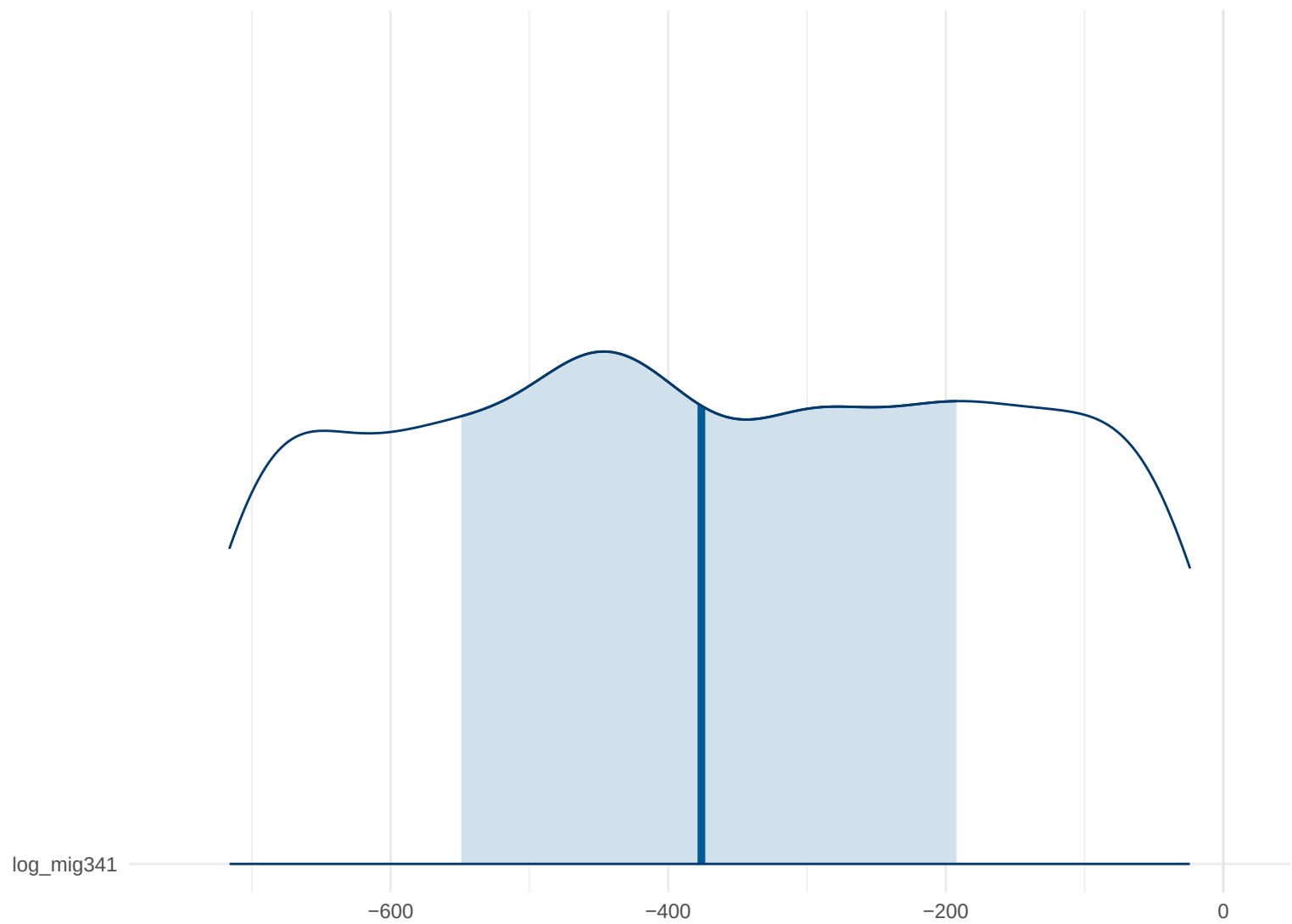
Posterior Density: log_mig341
