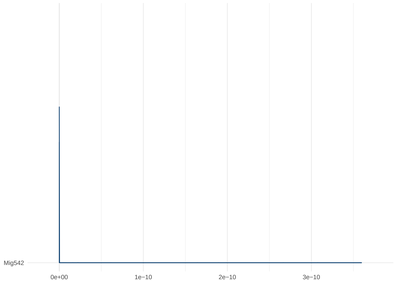
Posterior Density: Mig542
