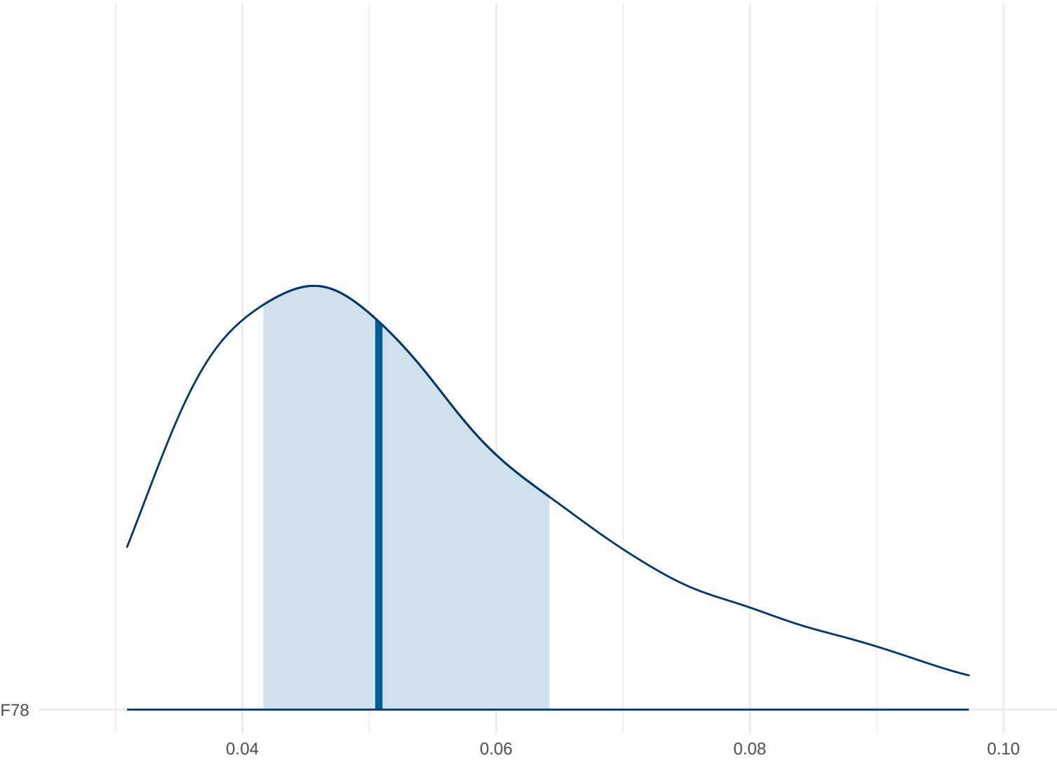
Posterior Density: F78
