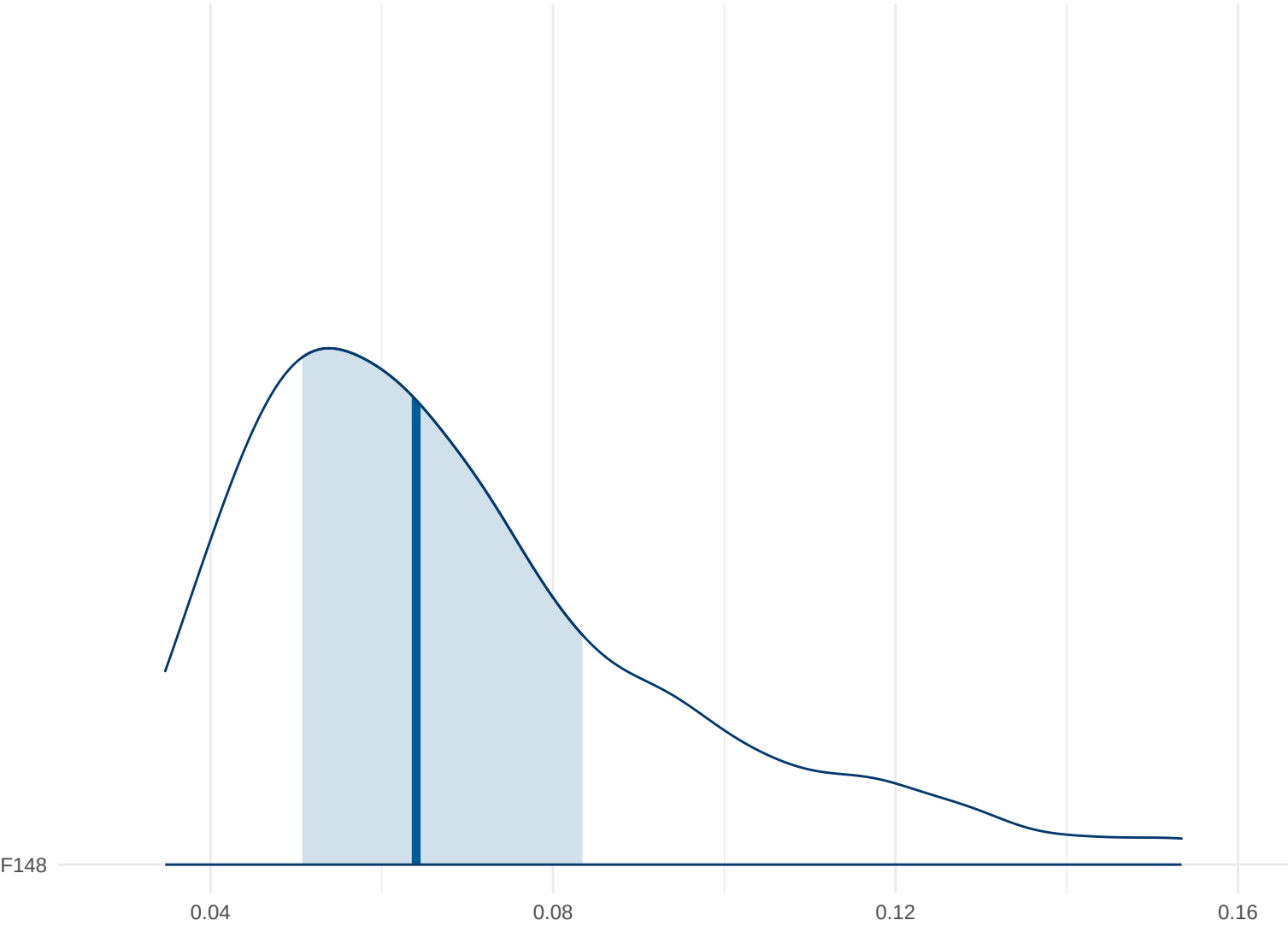
Posterior Density: F148
