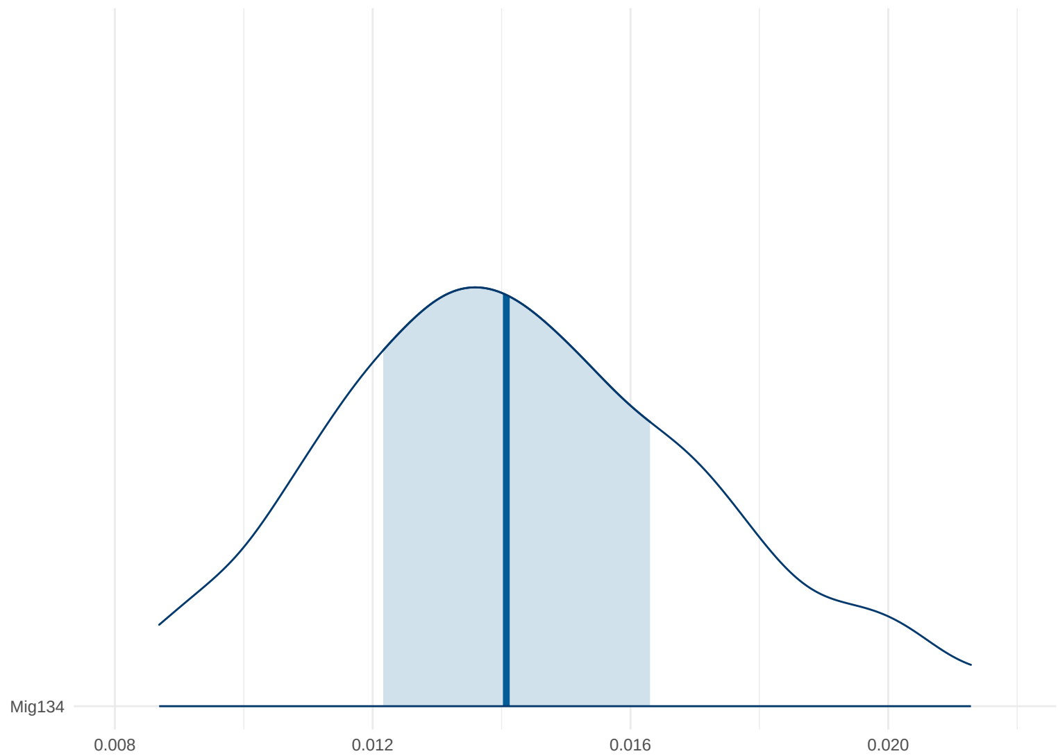
Posterior Density: Mig134
