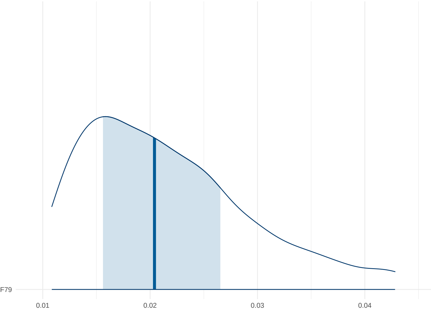
Posterior Density: F79
