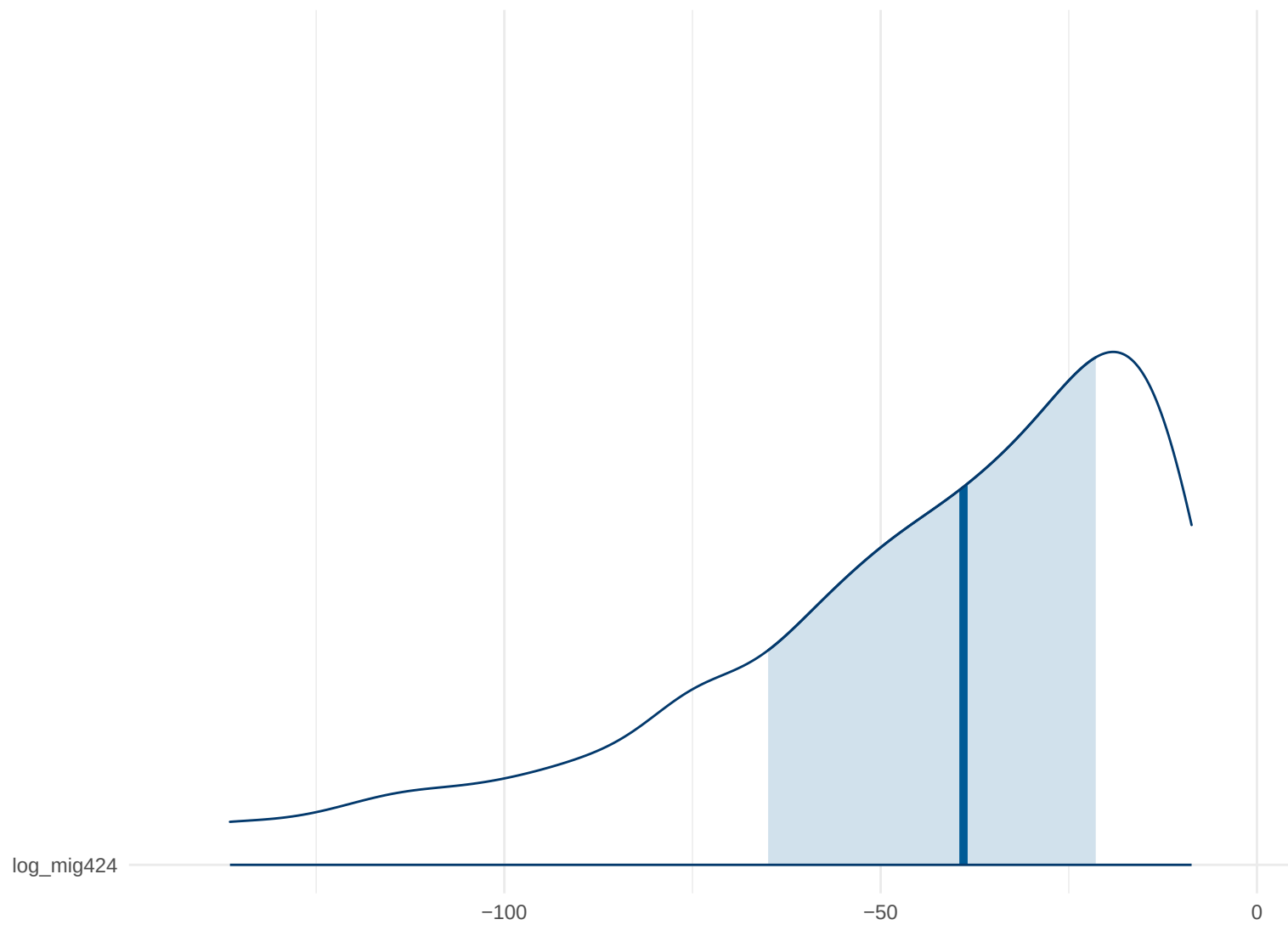
Posterior Density: log_mig424
