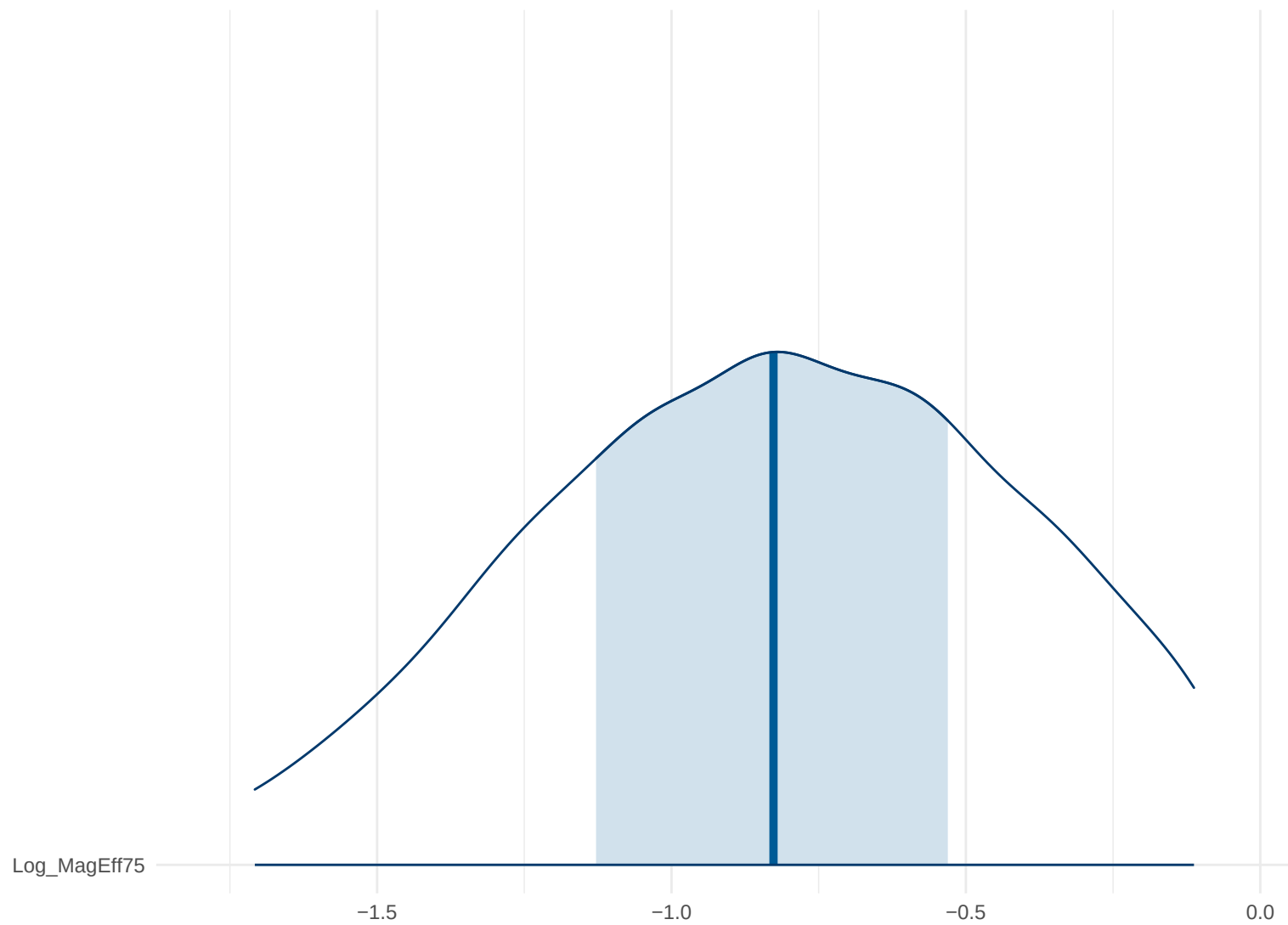
Posterior Density: Log_MagEff75
