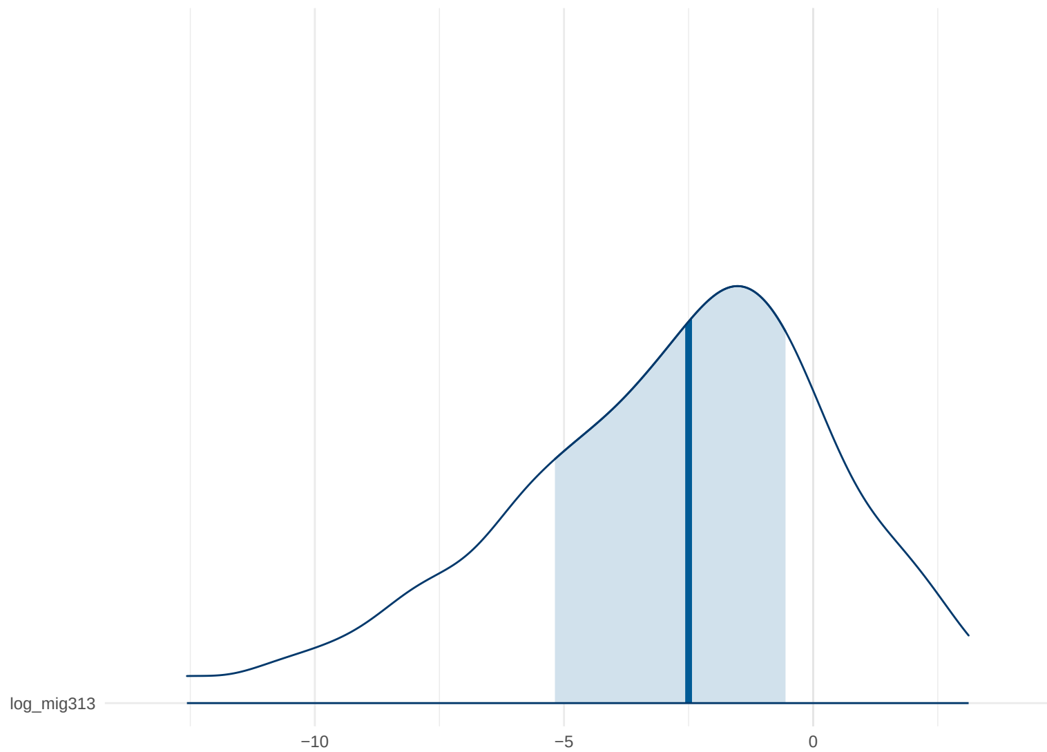
Posterior Density: log_mig313
