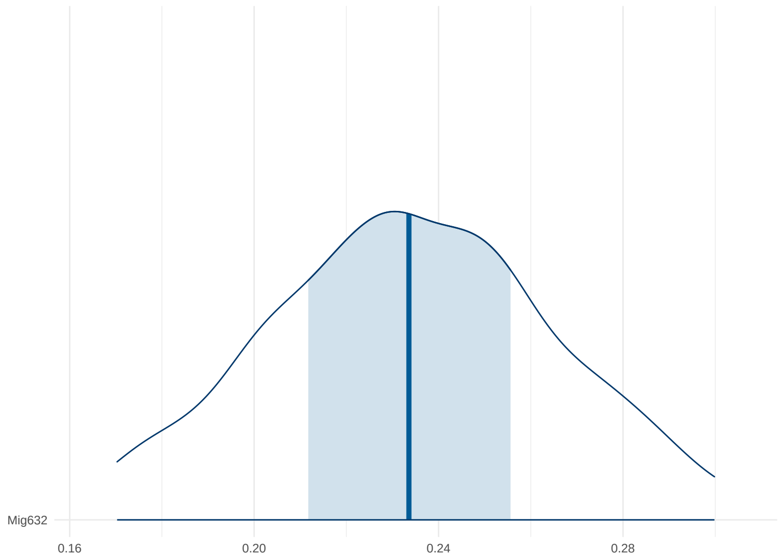
Posterior Density: Mig632
