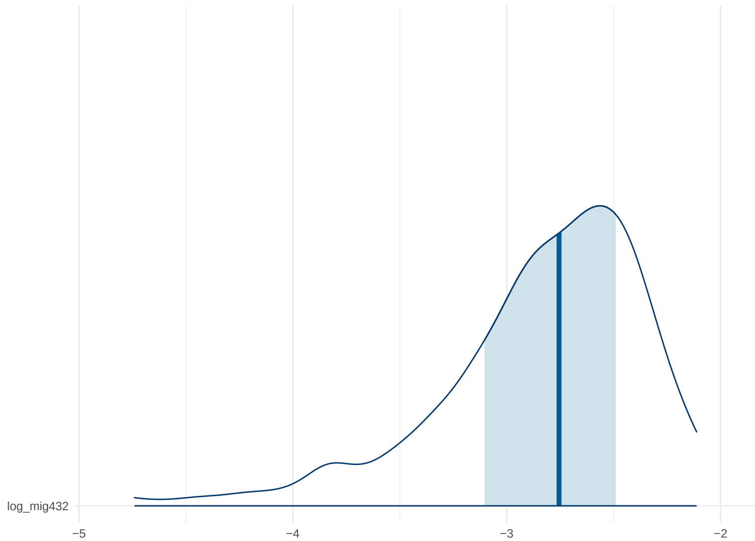
Posterior Density: log_mig432
