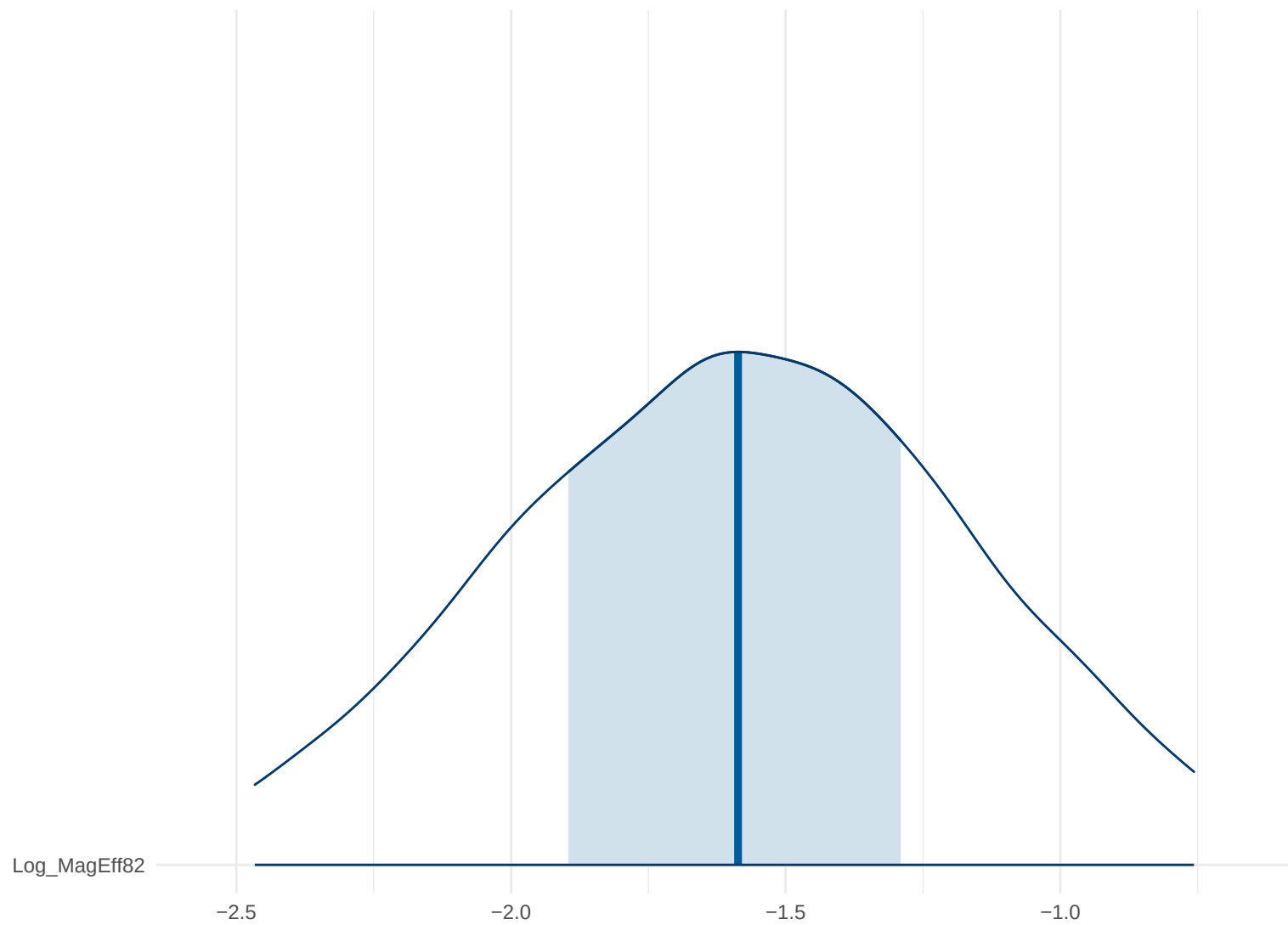
Posterior Density: Log_MagEff82
