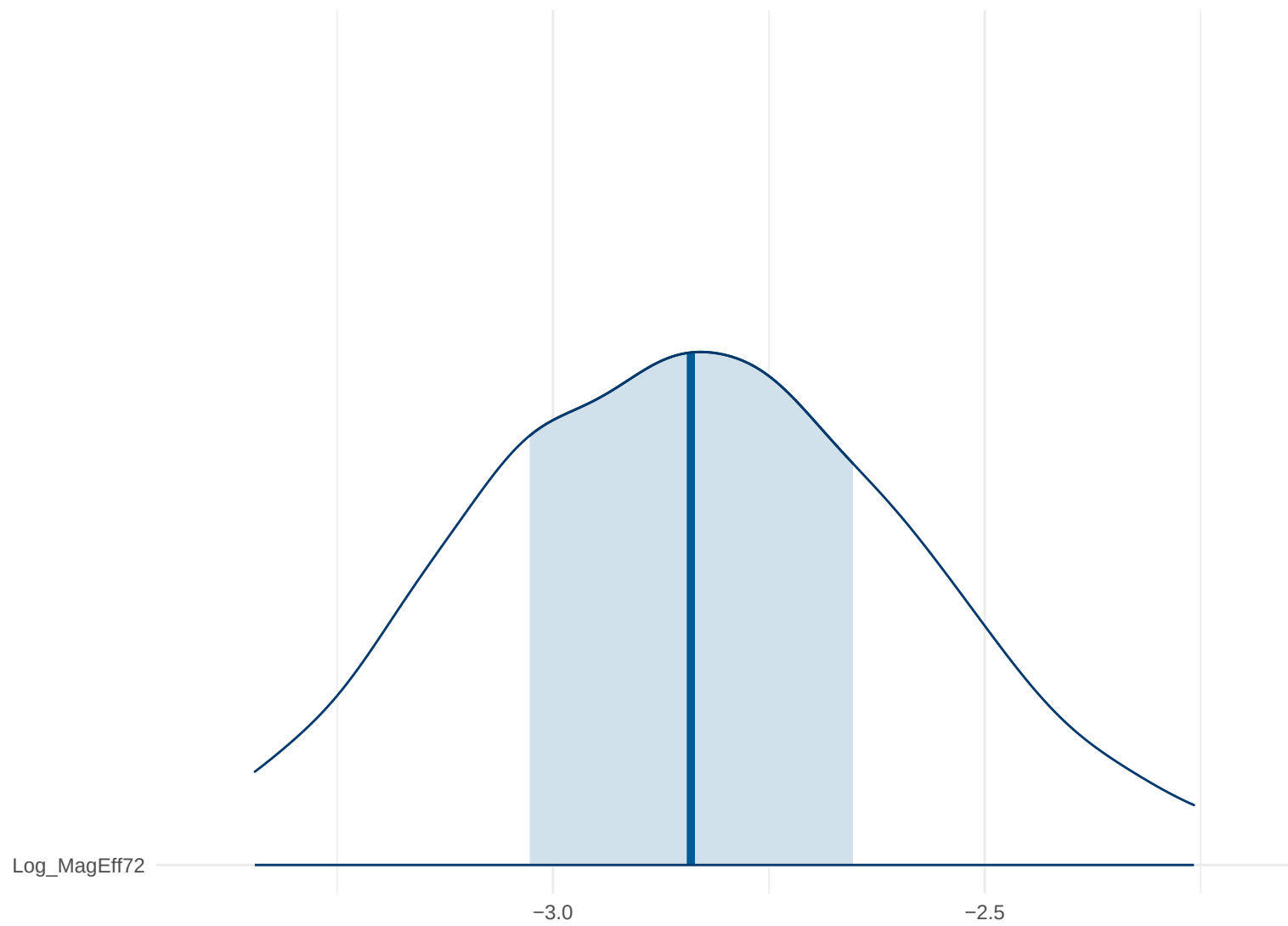
Posterior Density: Log_MagEff72
