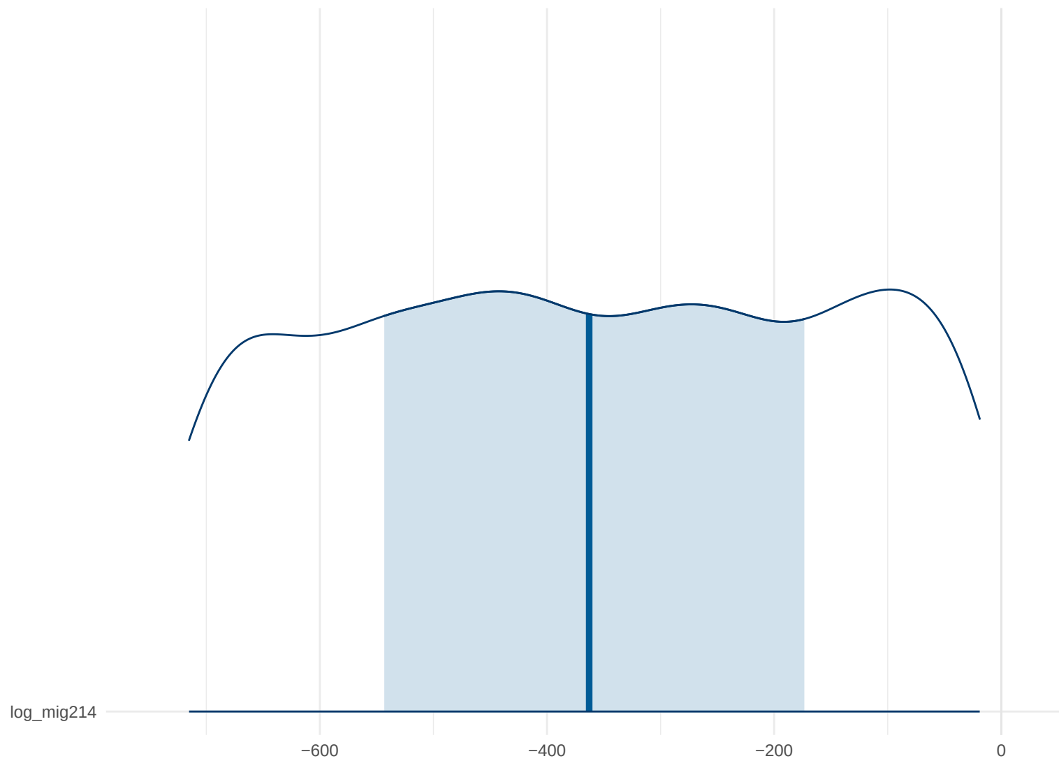
Posterior Density: log_mig214
