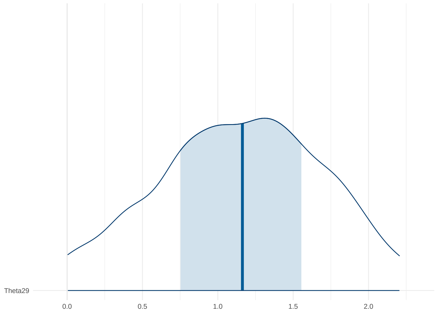
Posterior Density: Theta29
