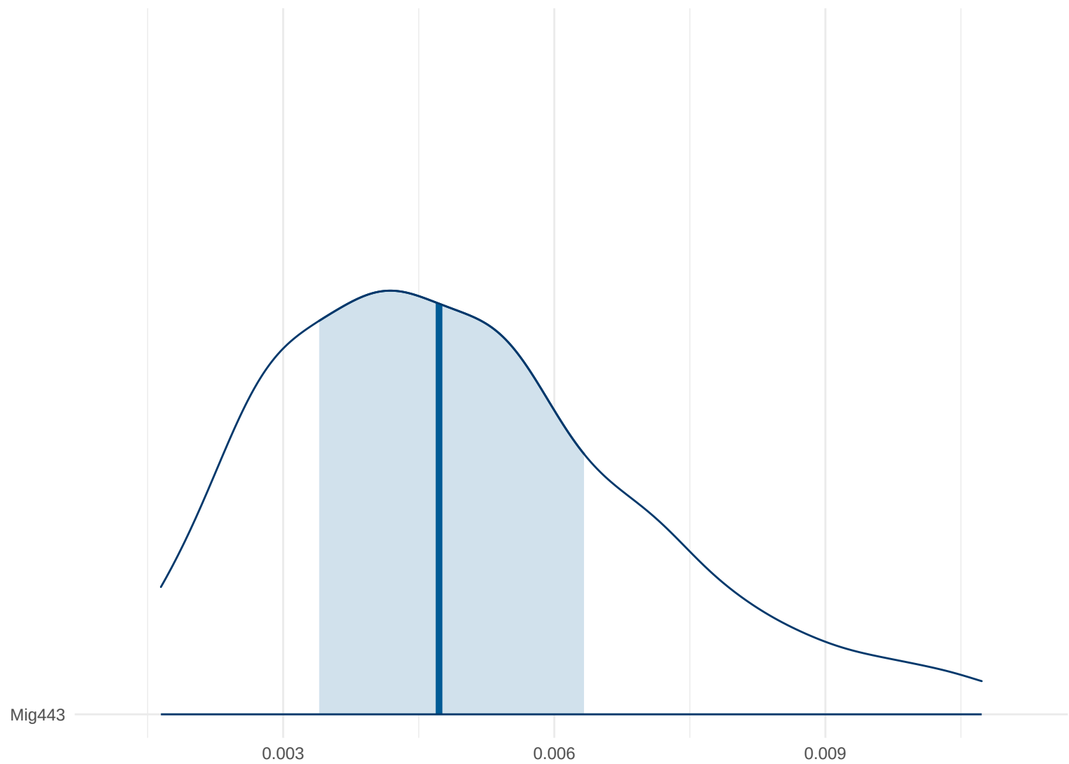
Posterior Density: Mig443
