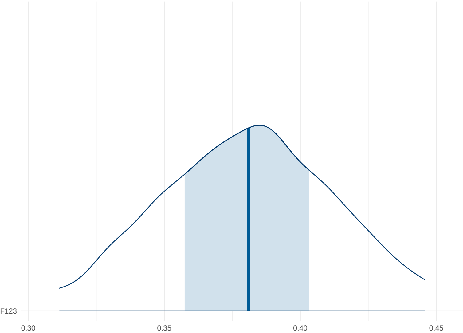
Posterior Density: F123
