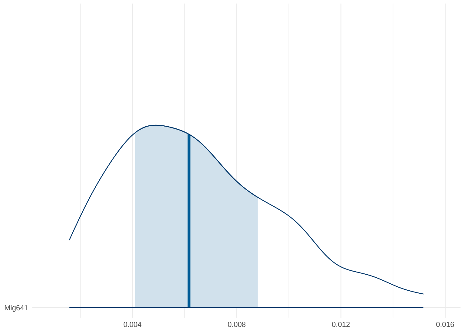
Posterior Density: Mig641
