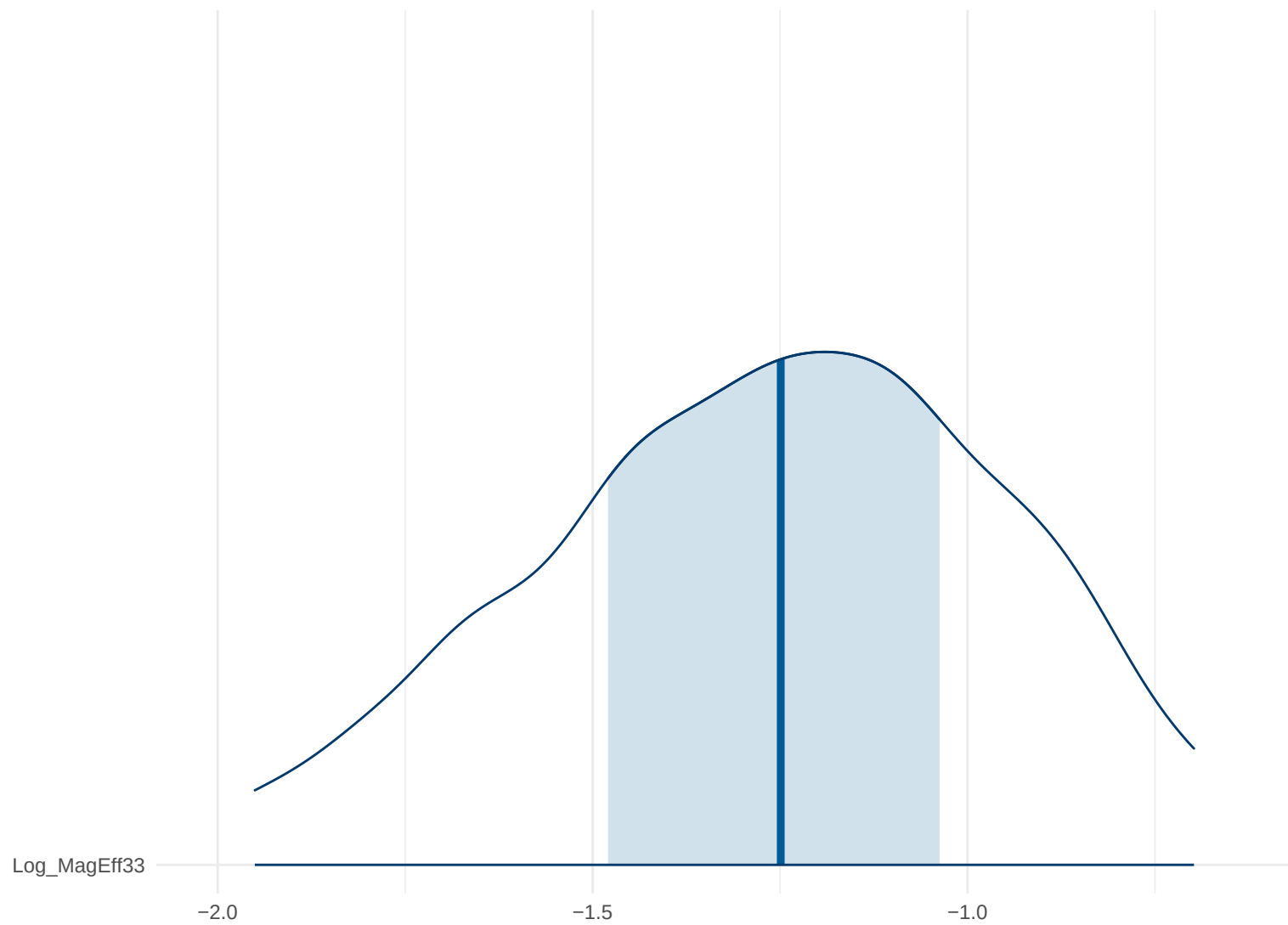
Posterior Density: Log_MagEff33
