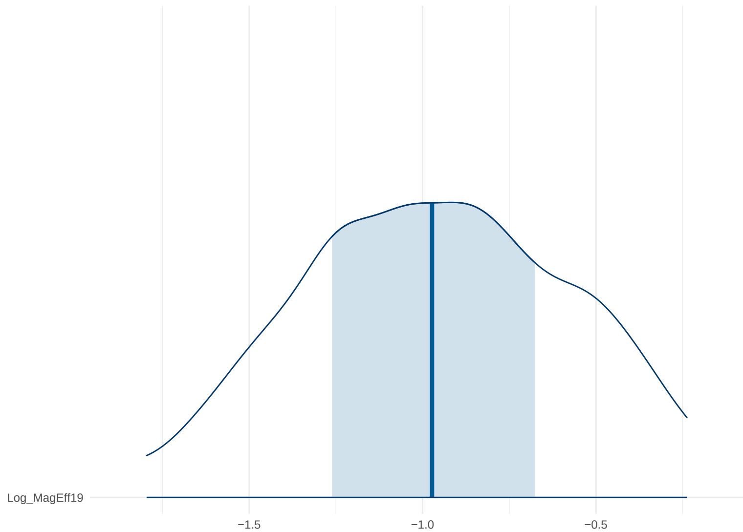
Posterior Density: Log_MagEff19
