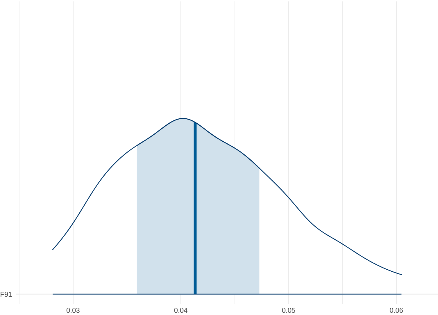
Posterior Density: F91
