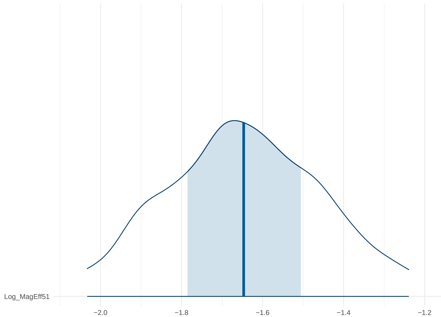
Posterior Density: Log_MagEff51
