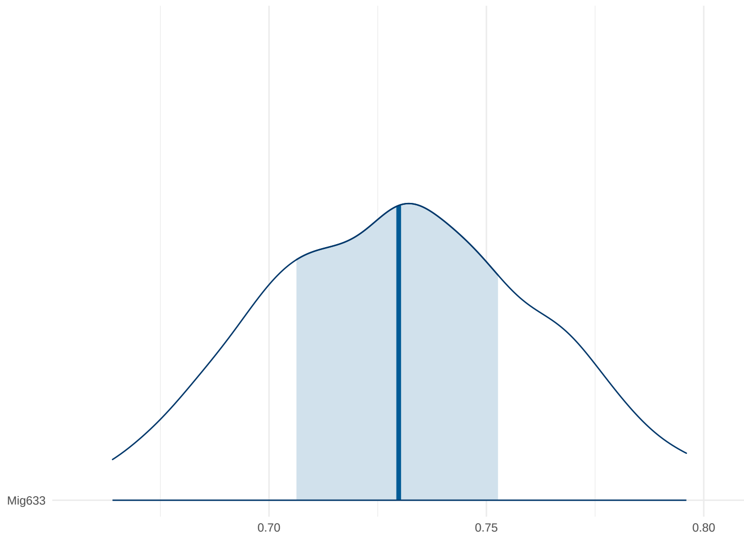
Posterior Density: Mig633
