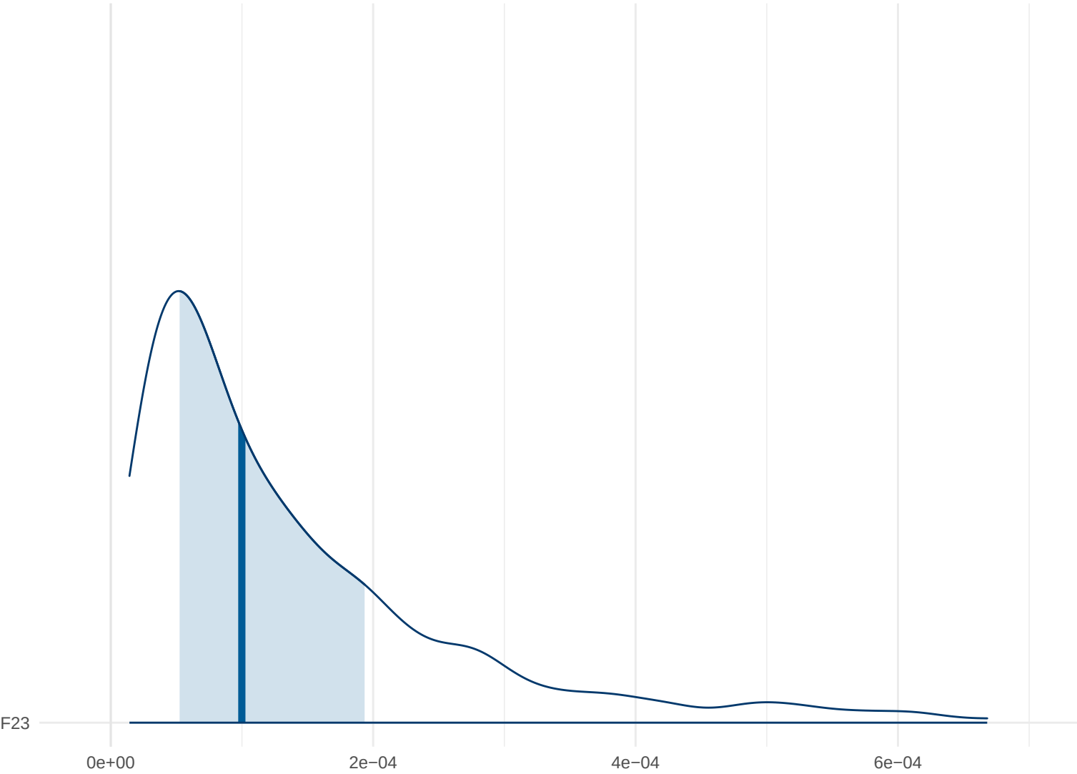
Posterior Density: F23
