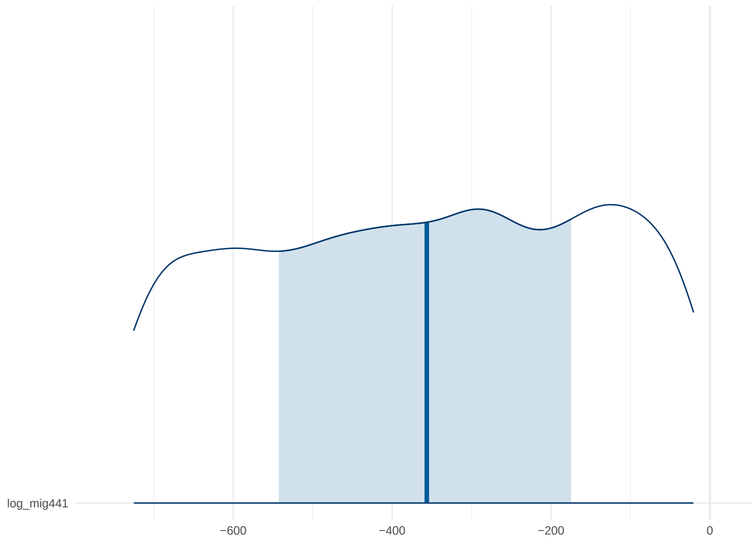
Posterior Density: log_mig441
