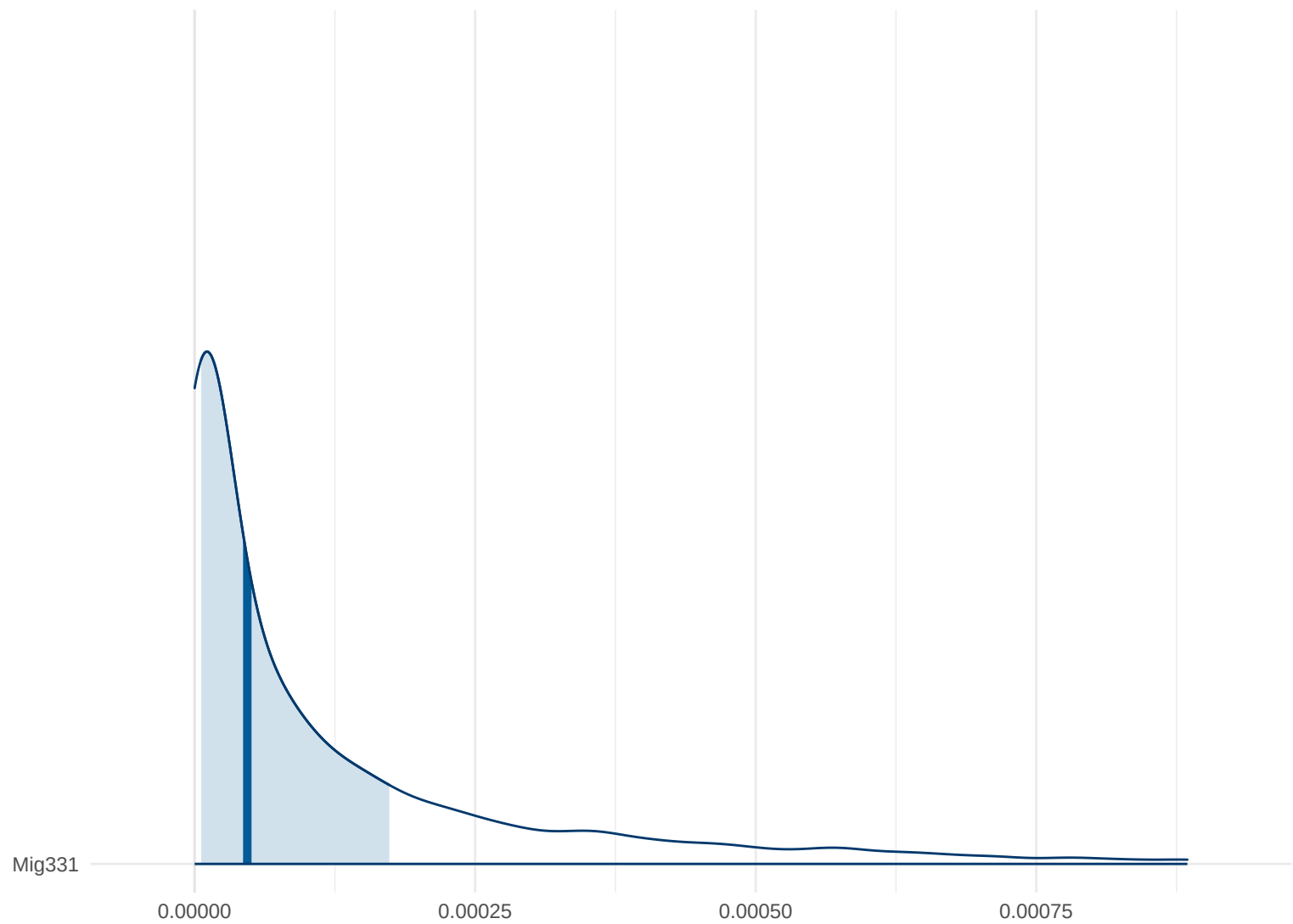
Posterior Density: Mig331
