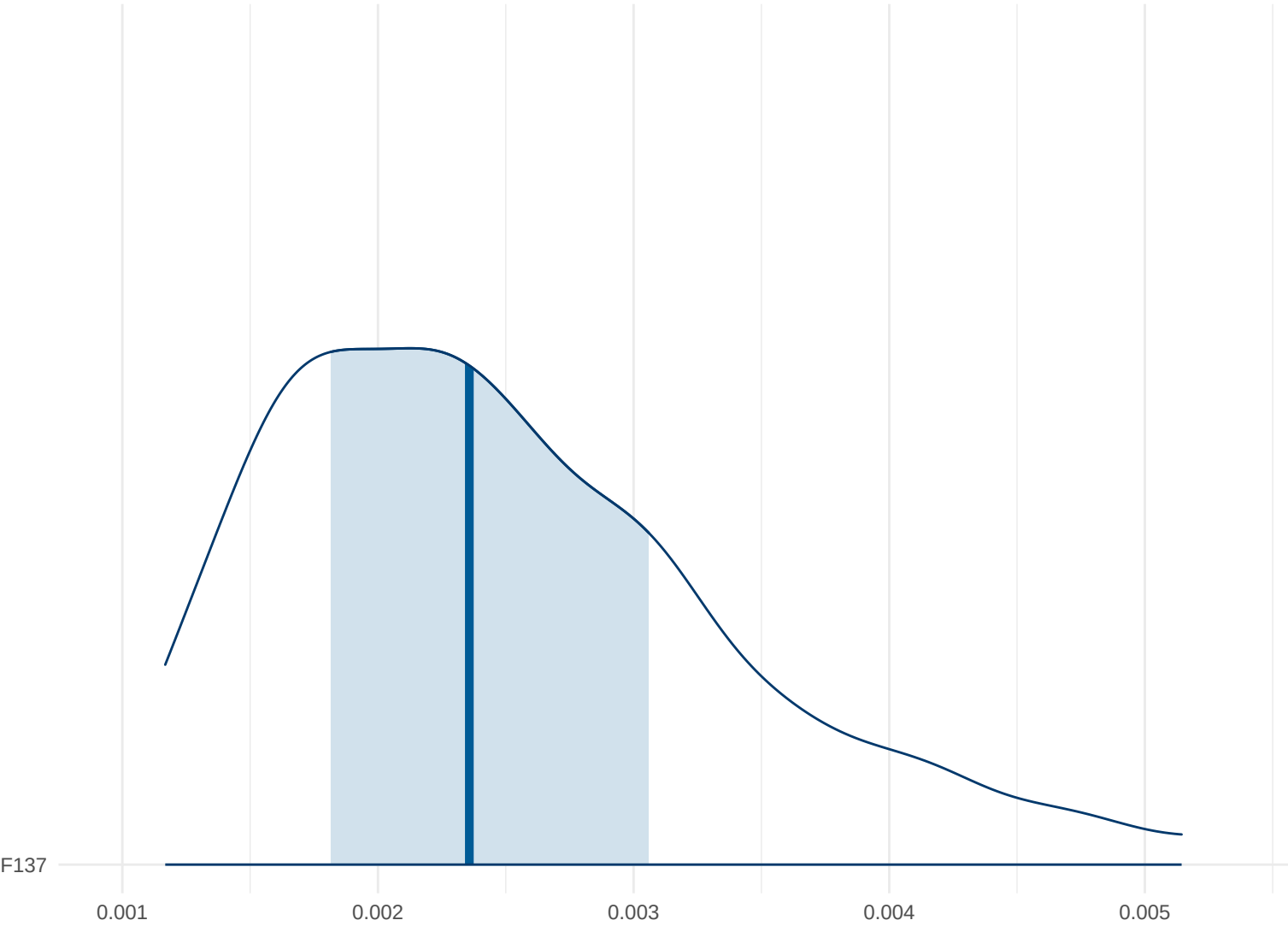
Posterior Density: F137
