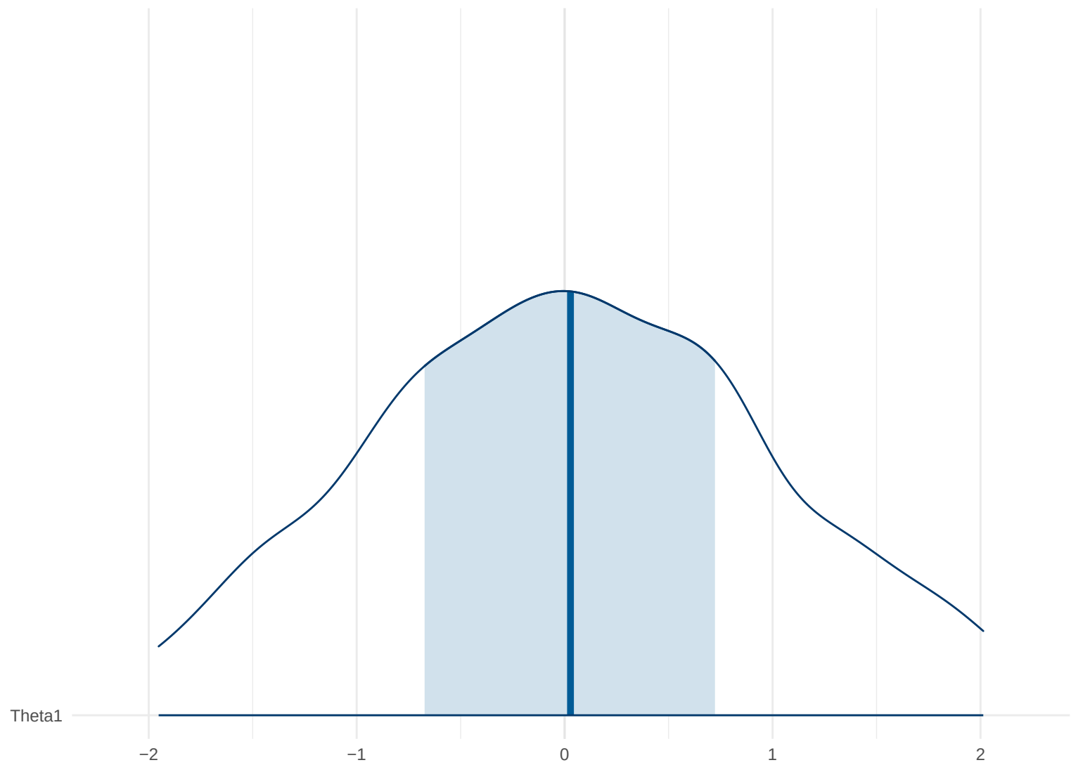
Posterior Density: Theta1
