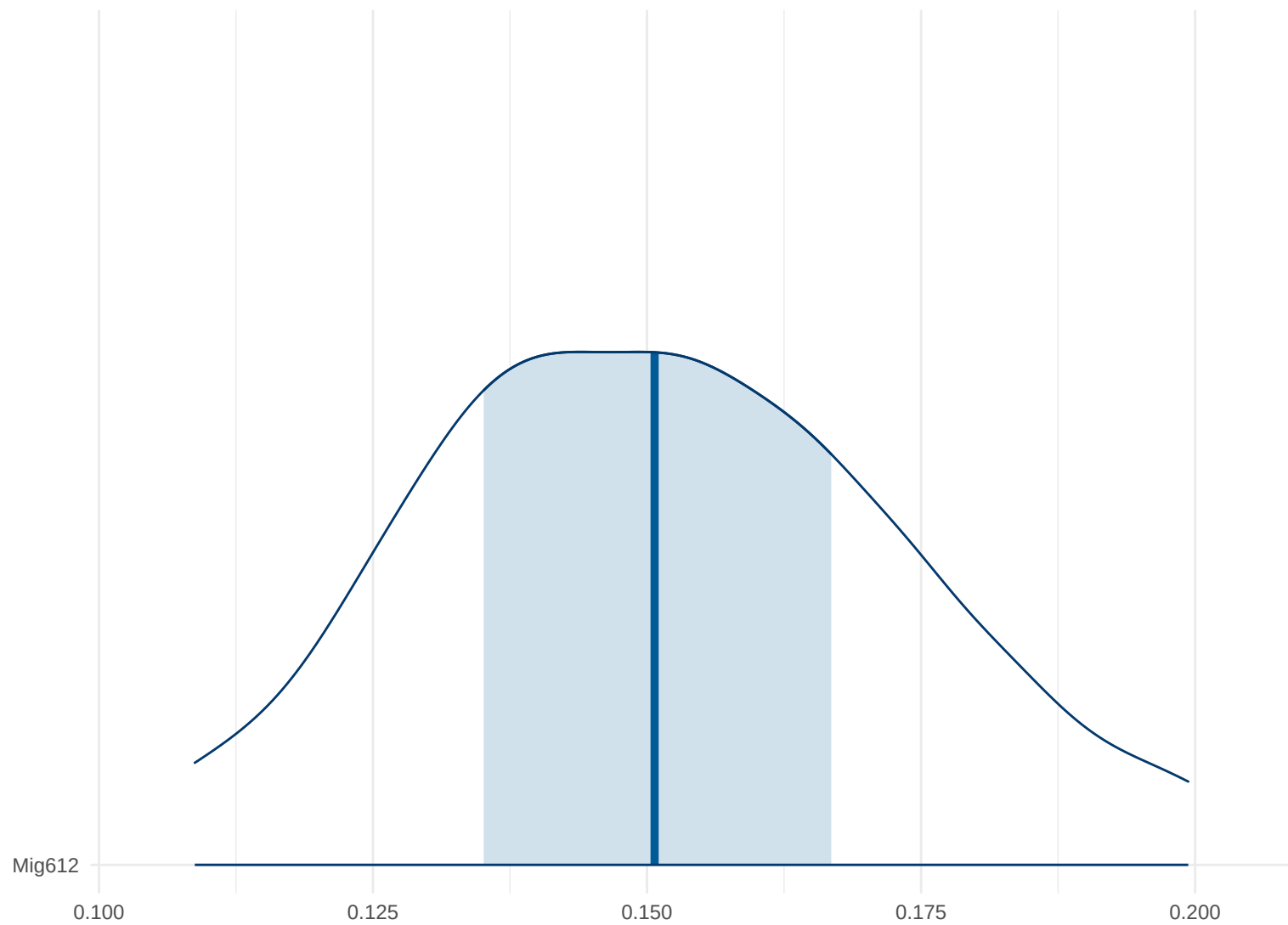
Posterior Density: Mig612
