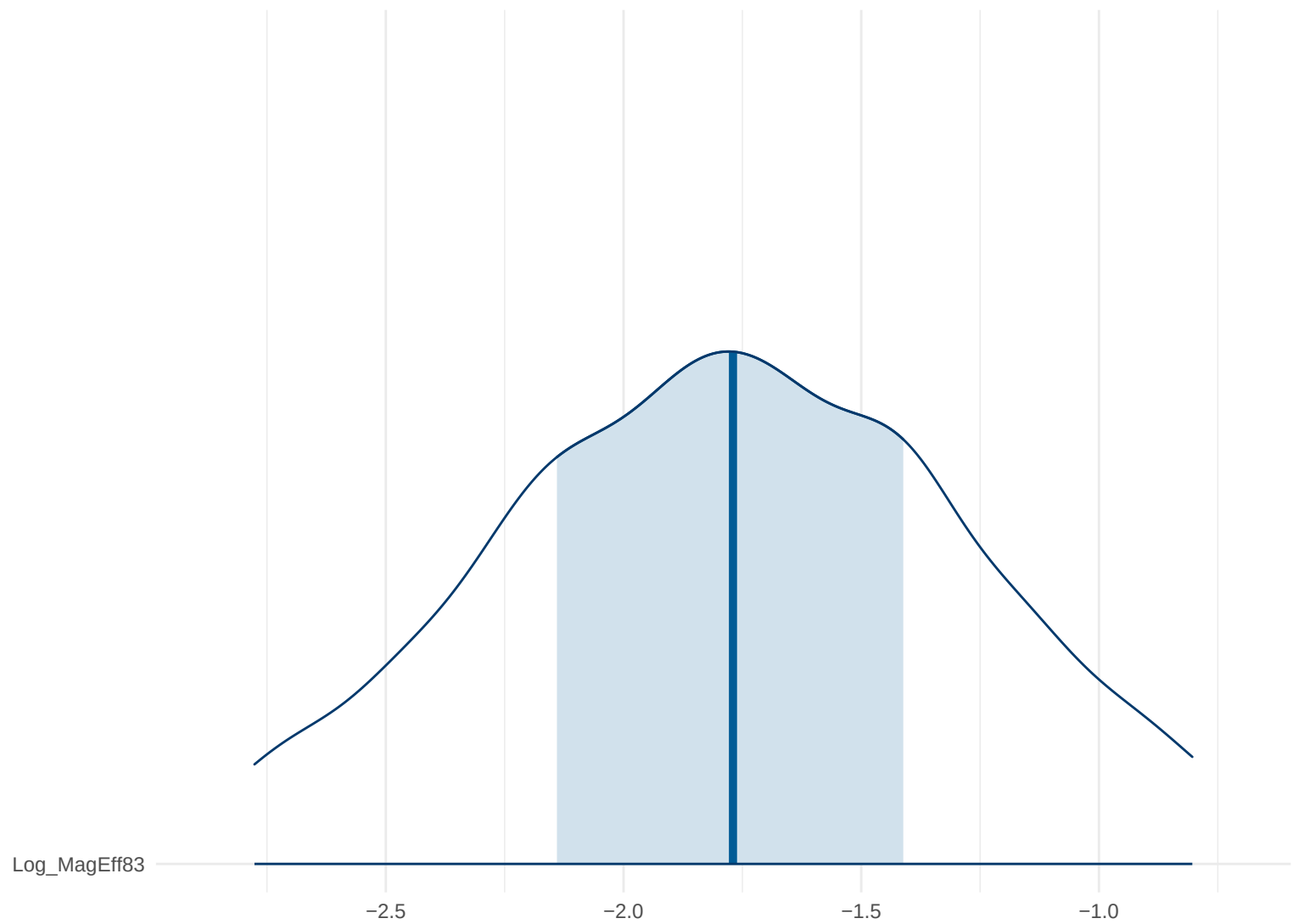
Posterior Density: Log_MagEff83
