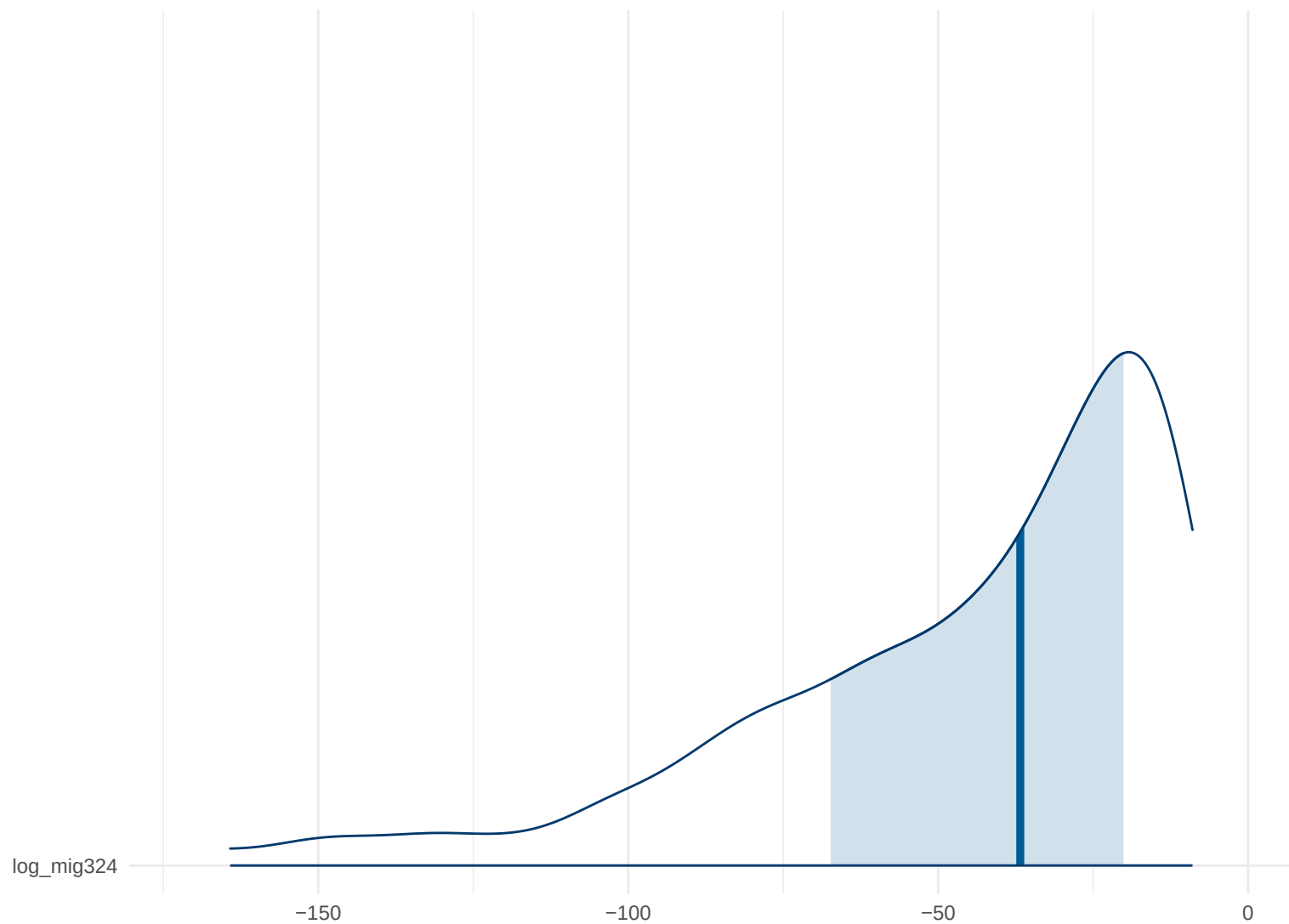
Posterior Density: log_mig324
