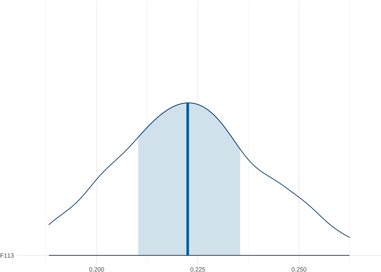
Posterior Density: F113
