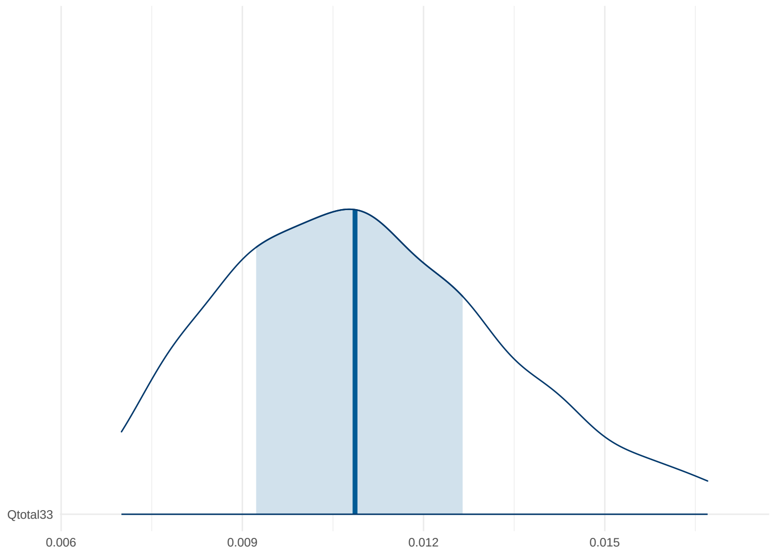
Posterior Density: Qtotal33
