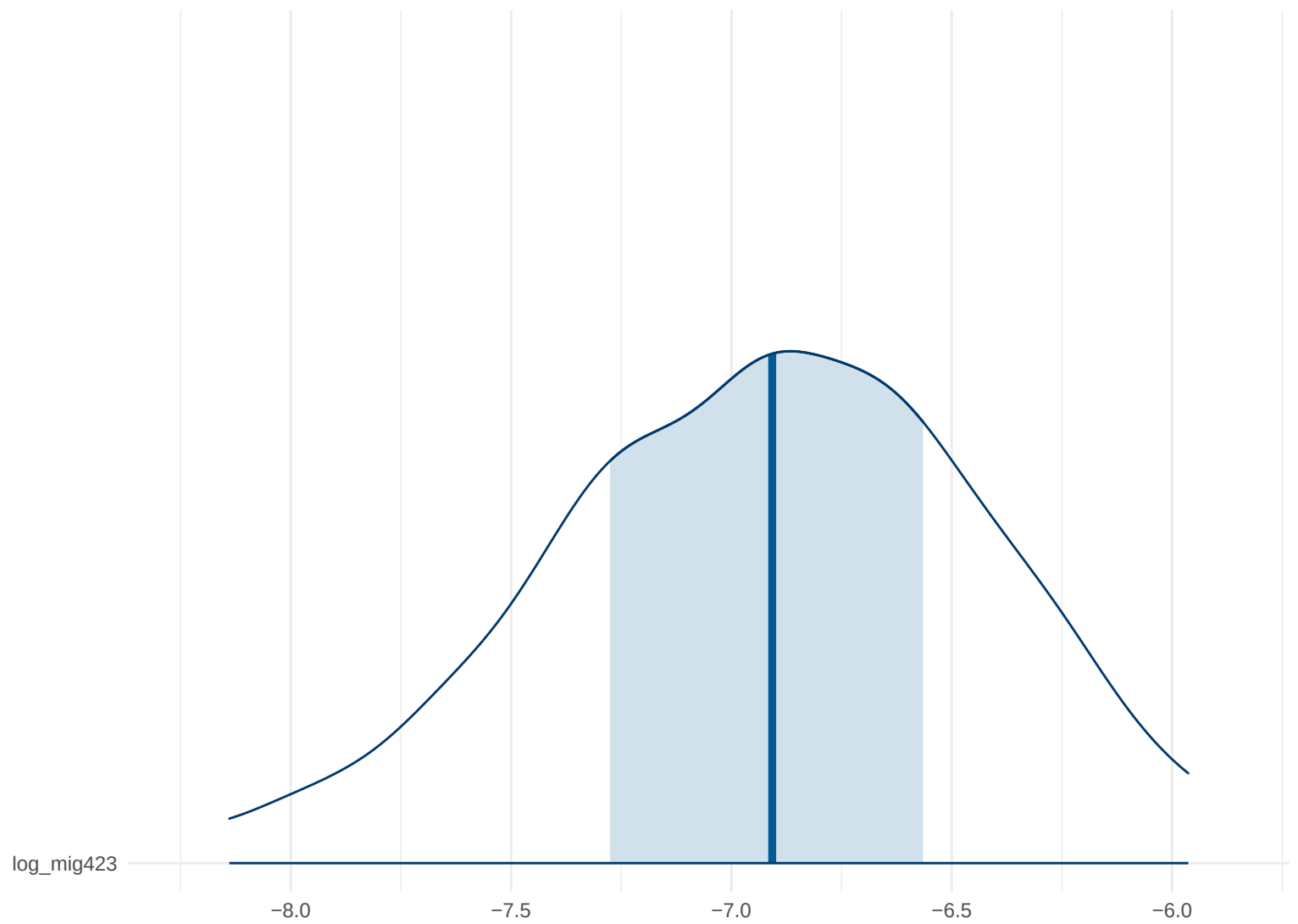
Posterior Density: log_mig423
