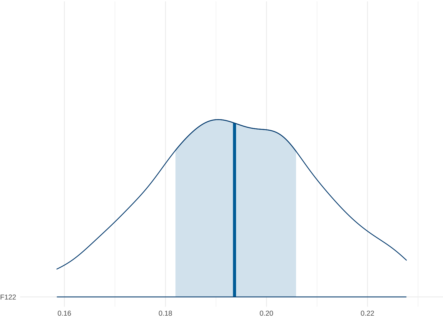
Posterior Density: F122
