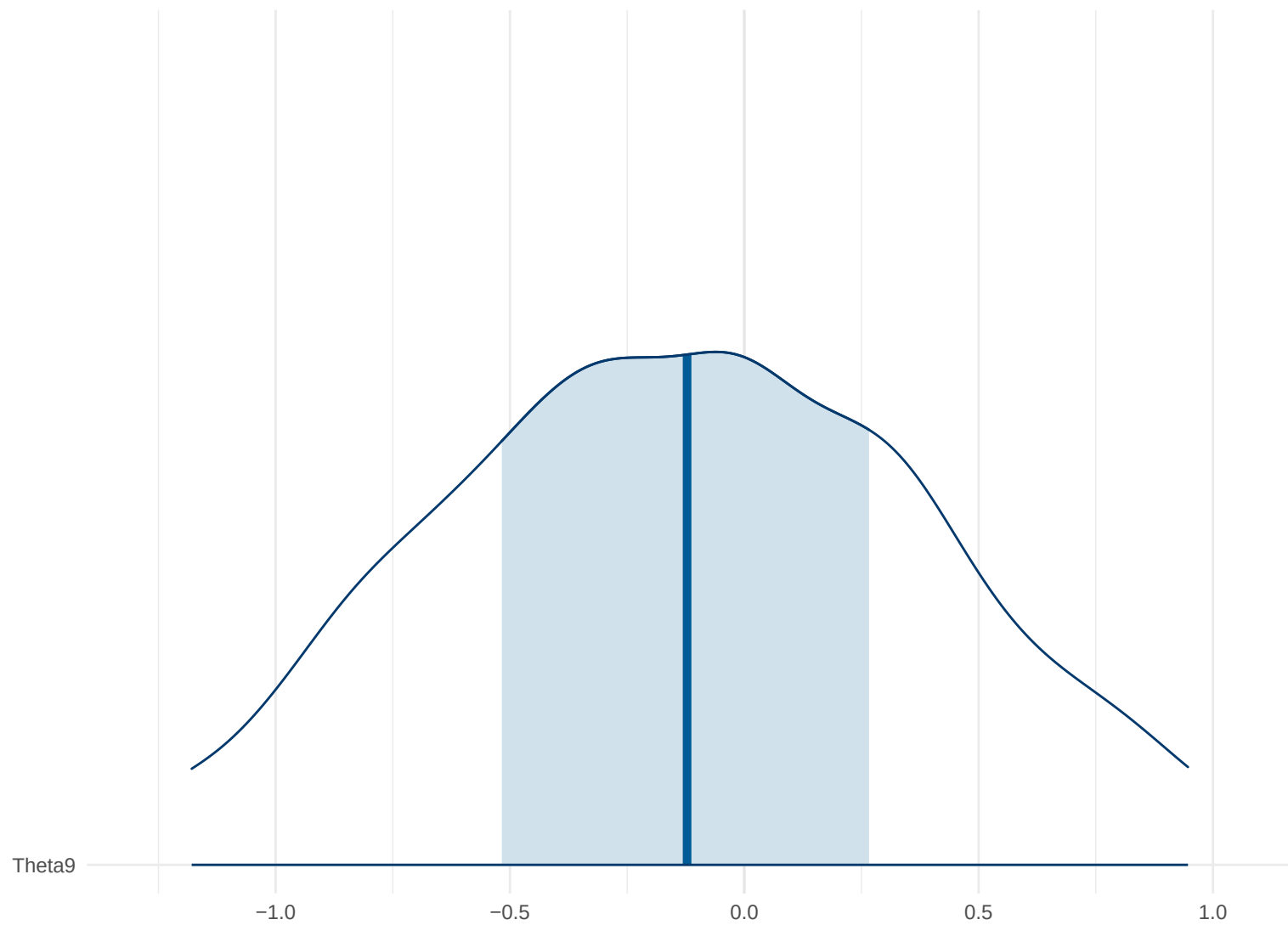
Posterior Density: Theta9
