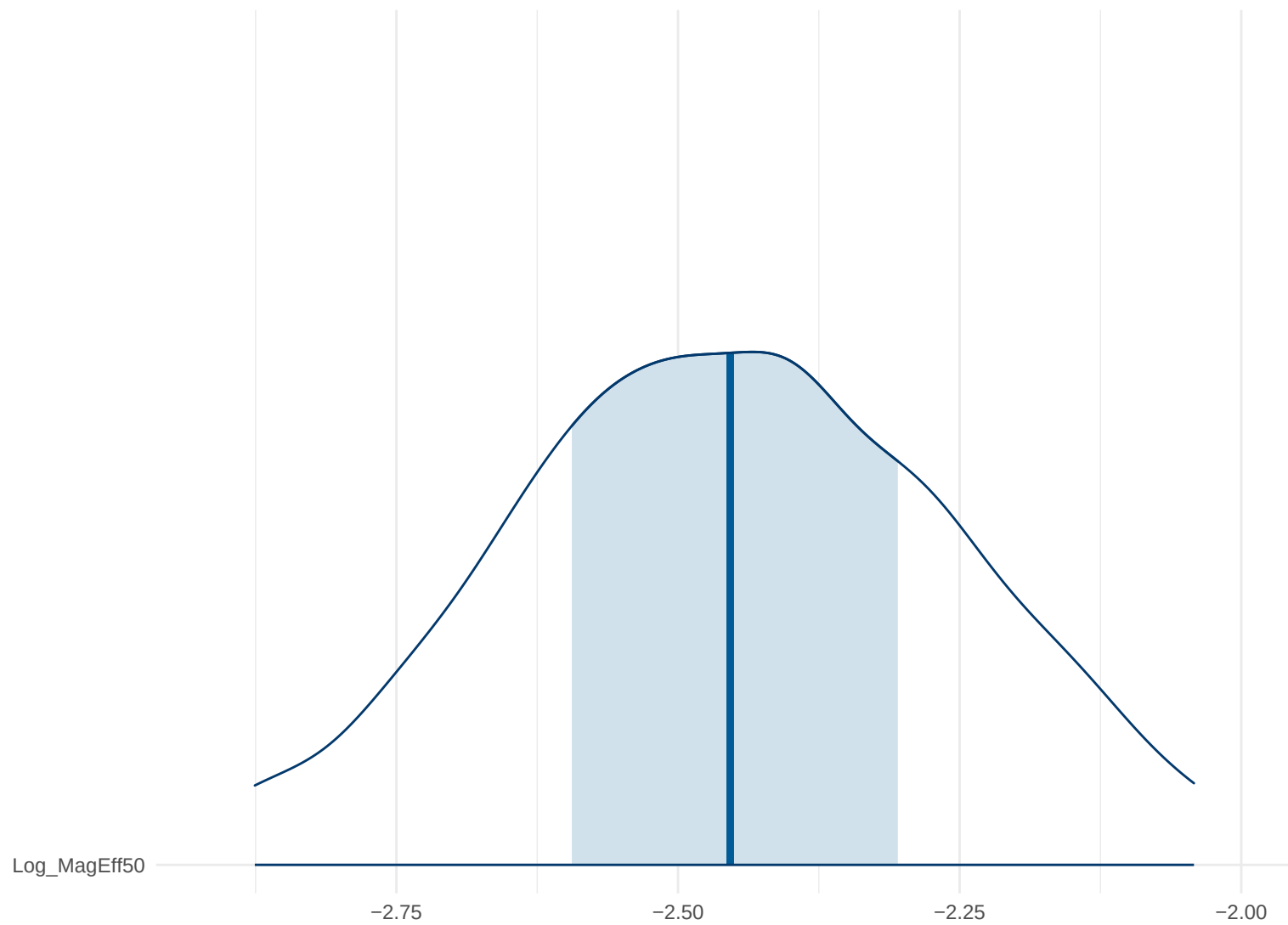
Posterior Density: Log_MagEff50
