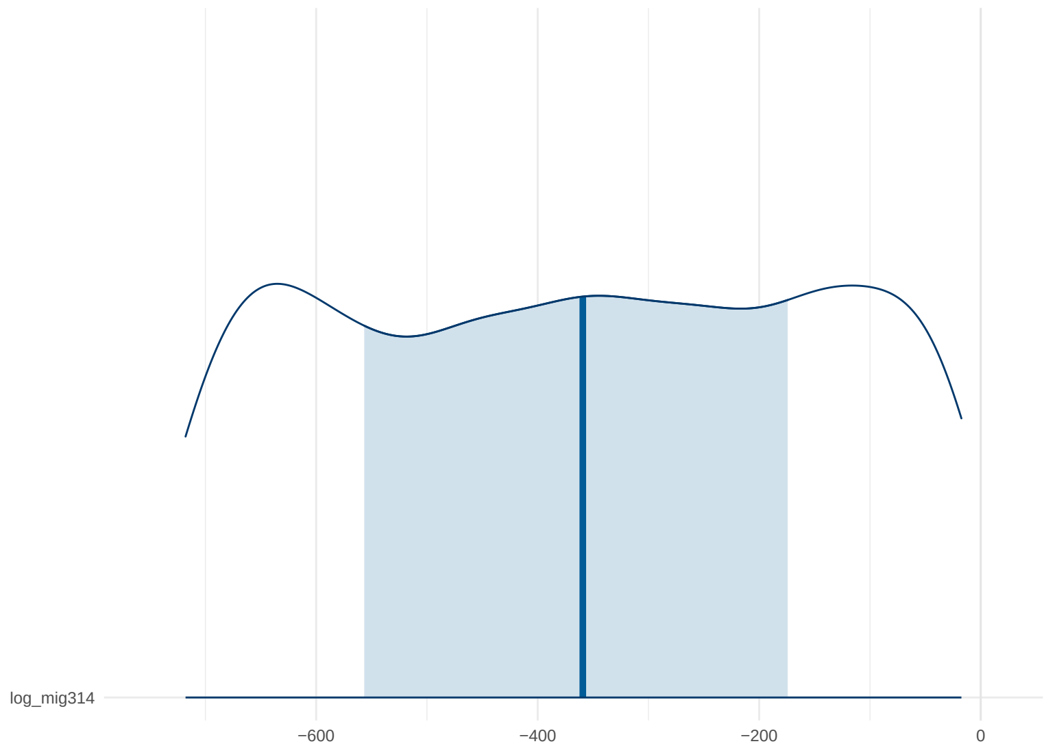
Posterior Density: log_mig314
