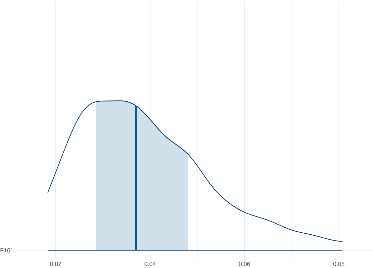
Posterior Density: F161
