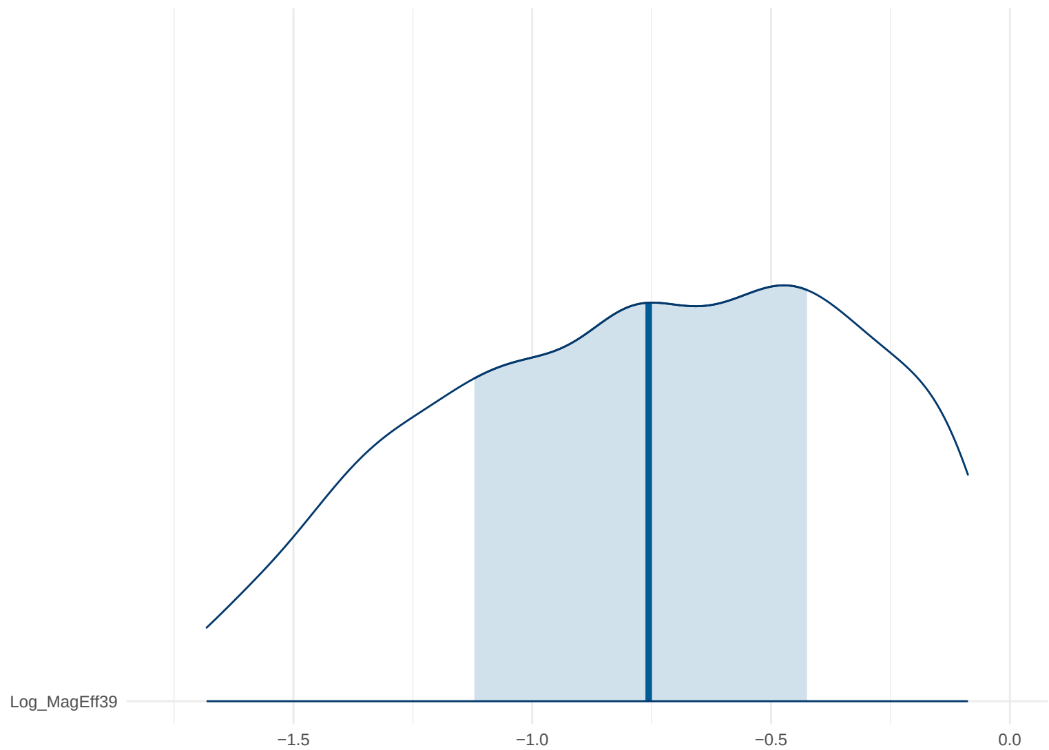
Posterior Density: Log_MagEff39
