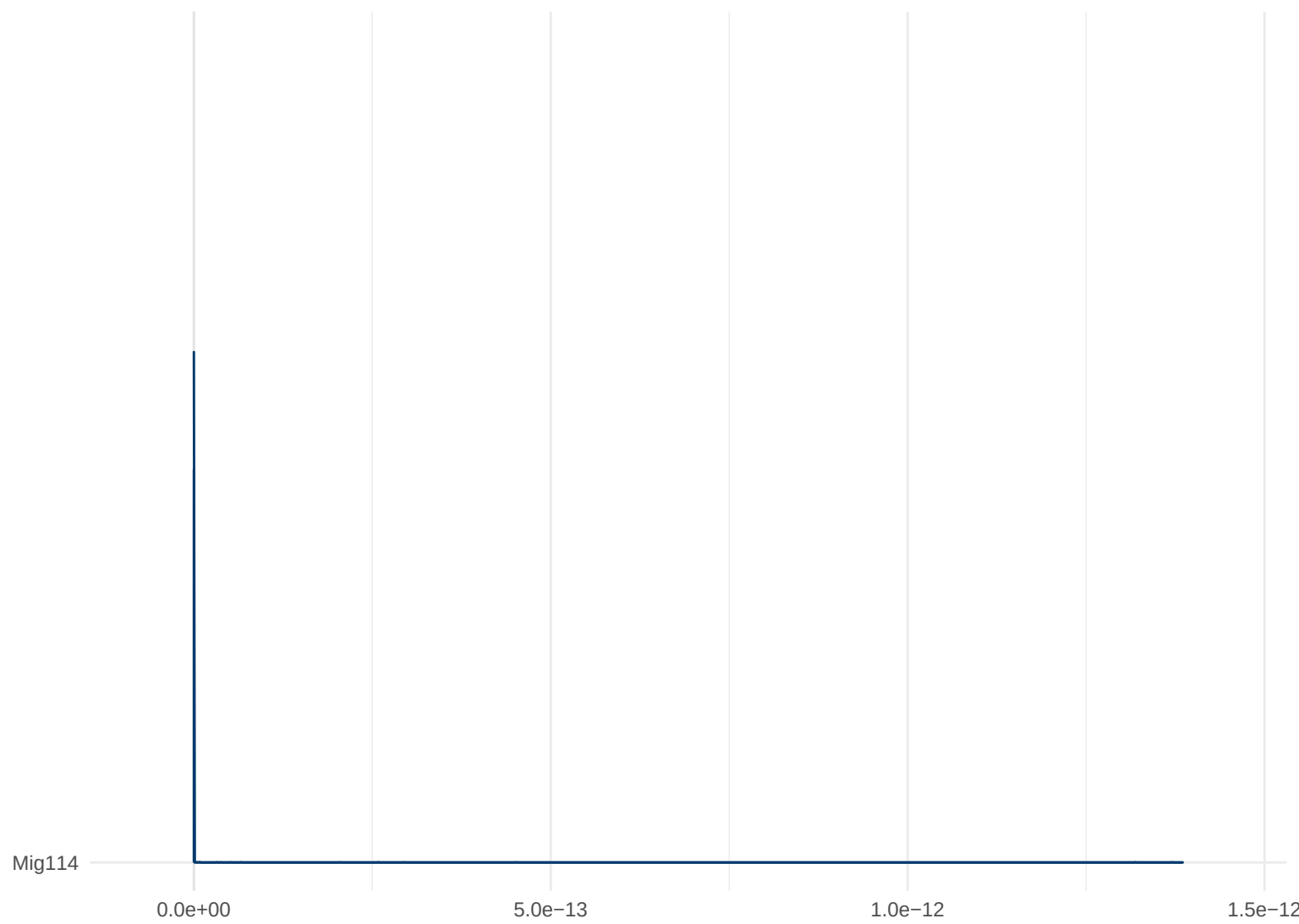
Posterior Density: Mig114
