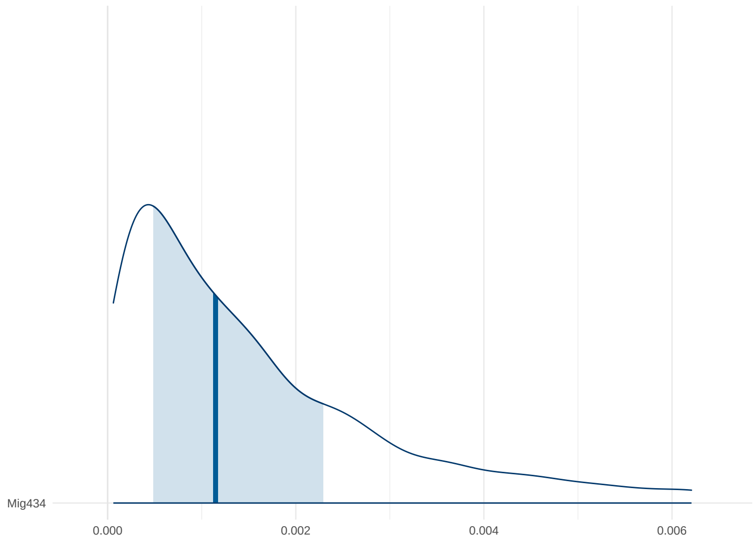
Posterior Density: Mig434
