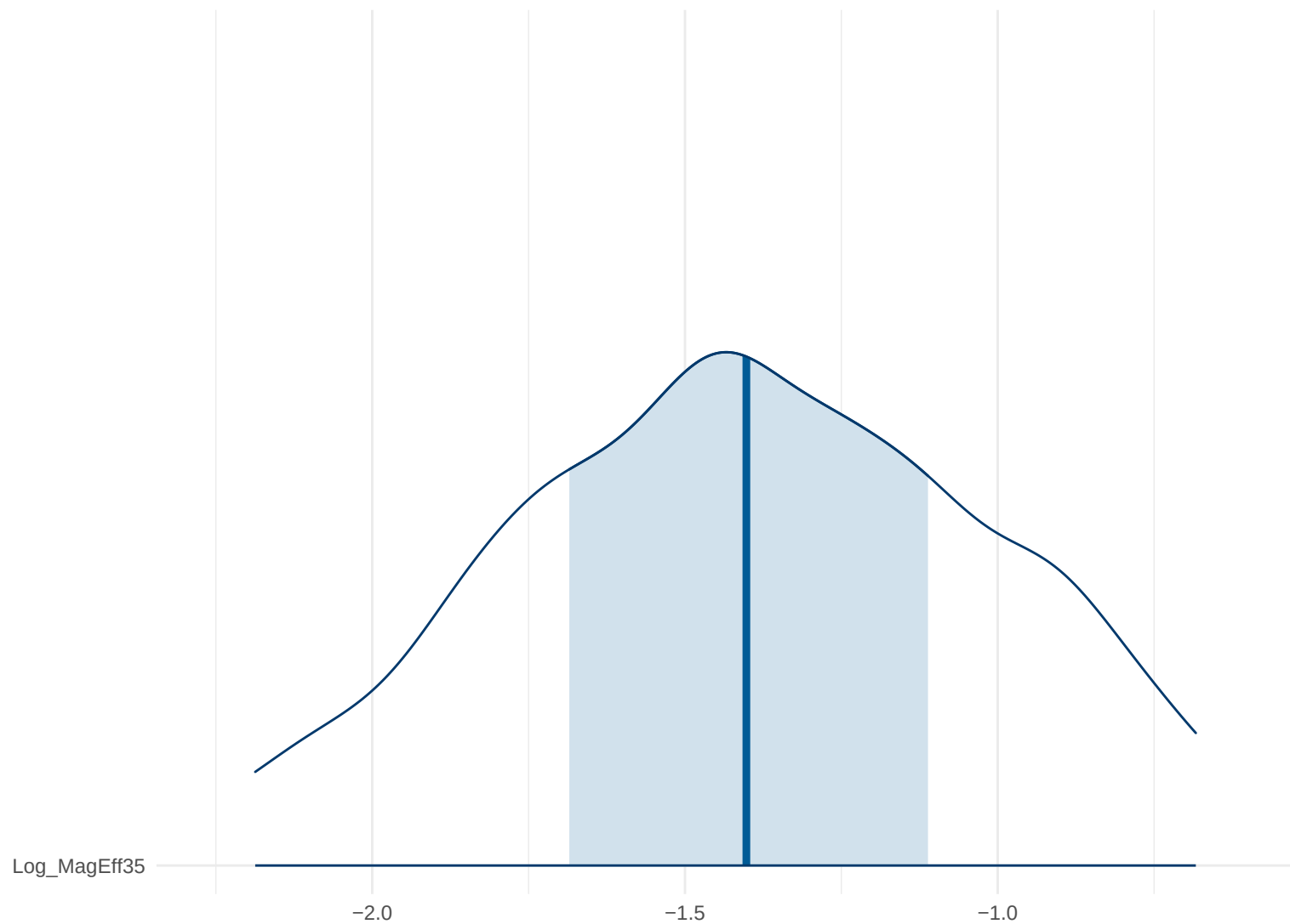
Posterior Density: Log_MagEff35
