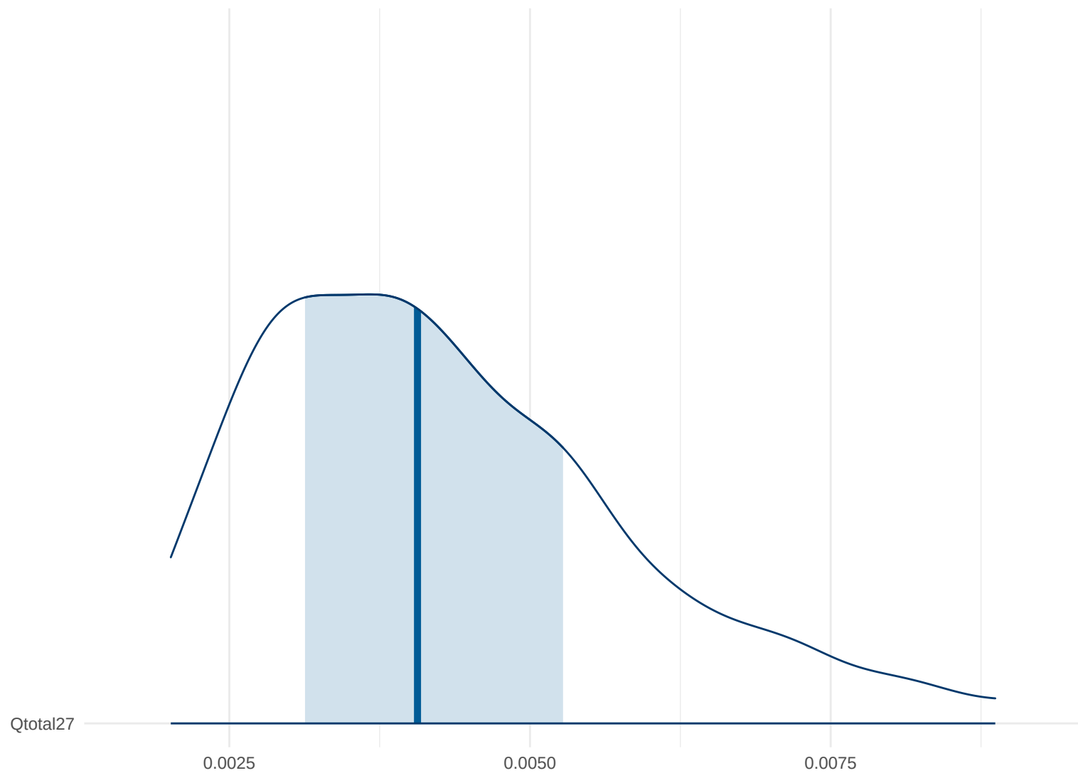
Posterior Density: Qtotal27
