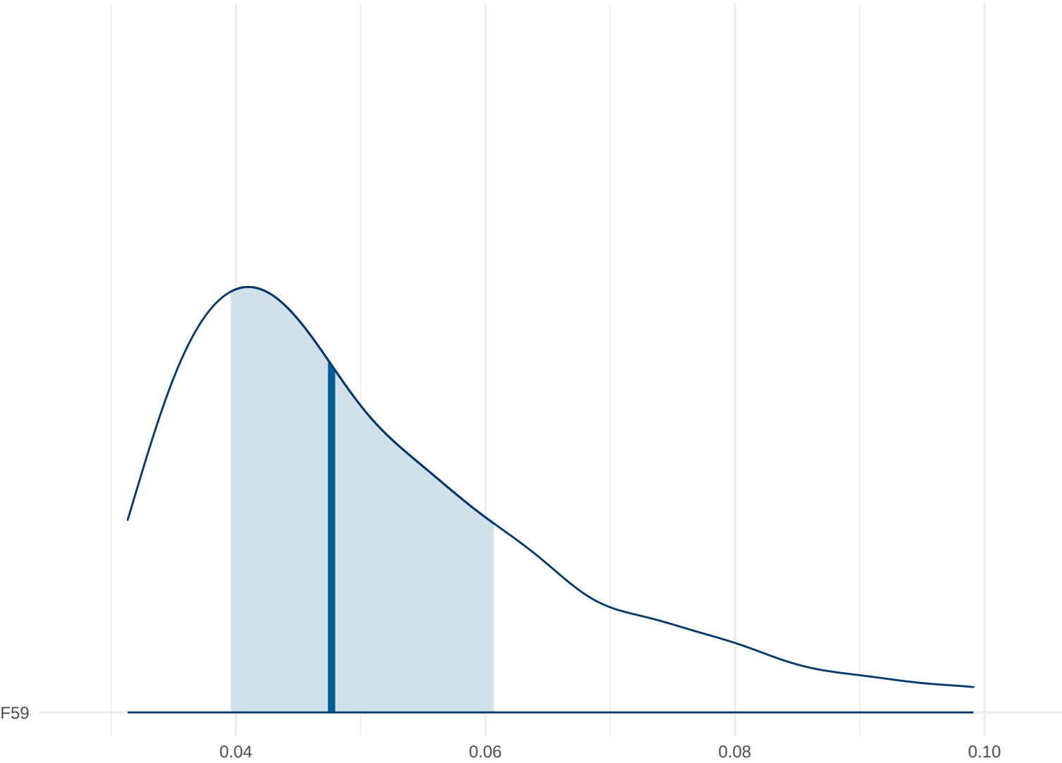
Posterior Density: F59
