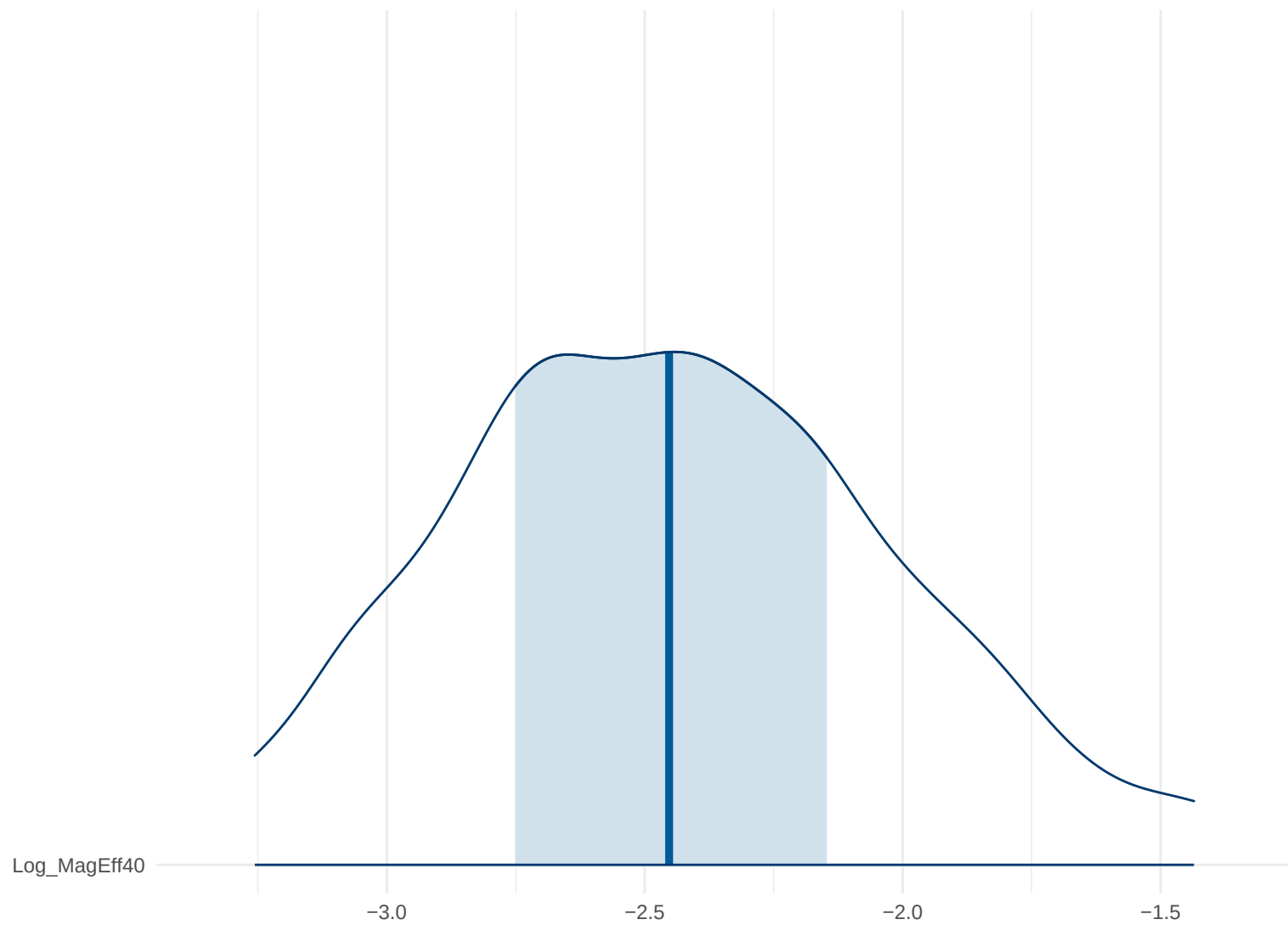
Posterior Density: Log_MagEff40
