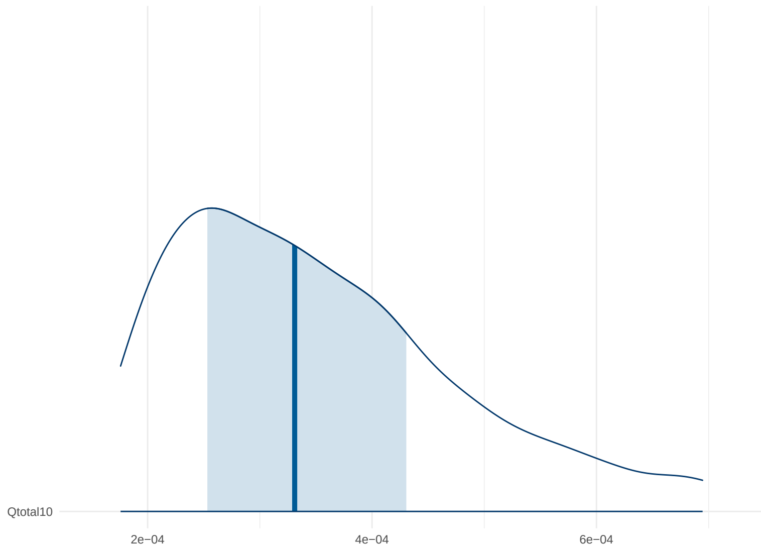
Posterior Density: Qtotal10
