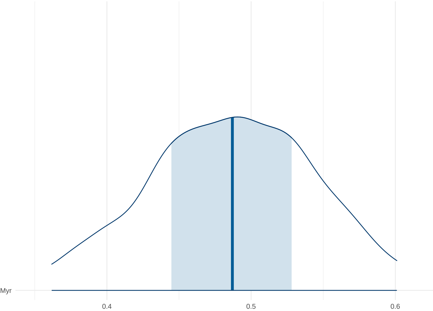
Posterior Density: Myr
