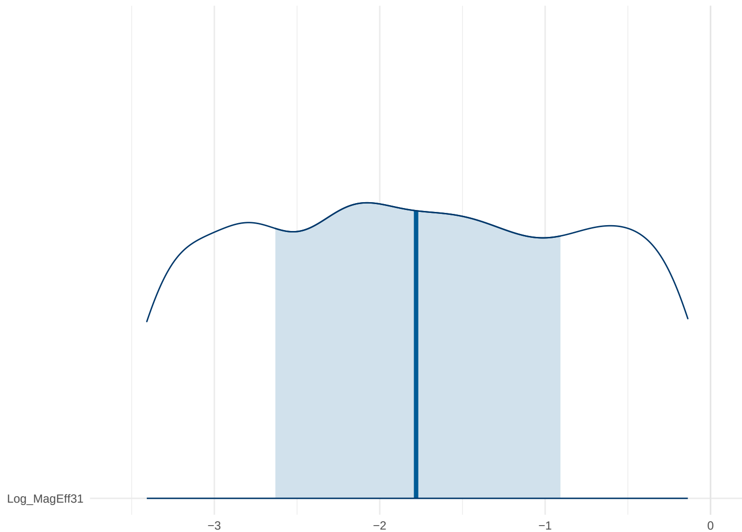
Posterior Density: Log_MagEff31
