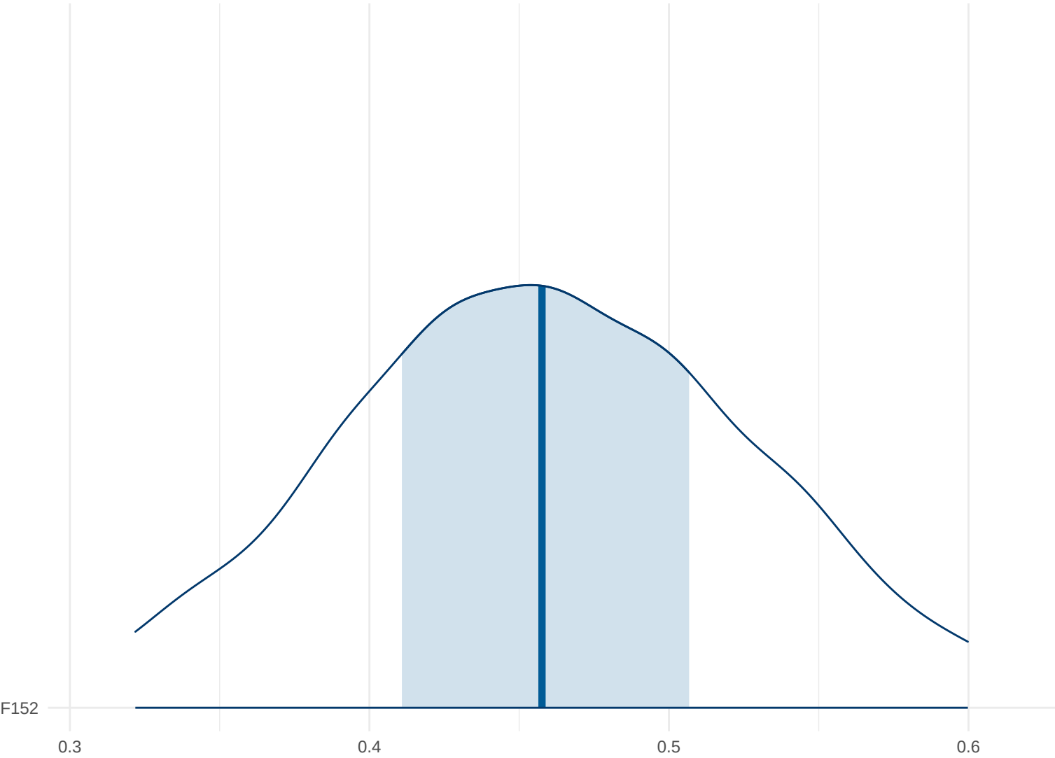
Posterior Density: F152
