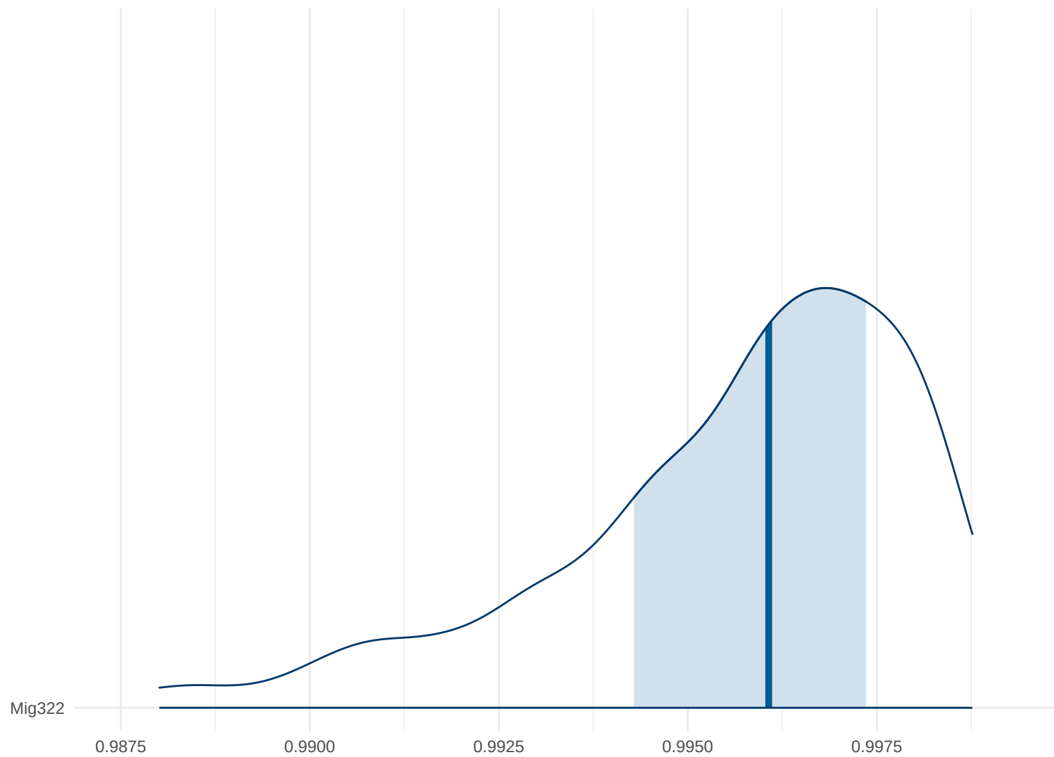
Posterior Density: Mig322
