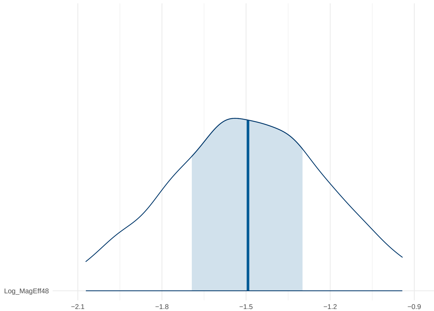
Posterior Density: Log_MagEff48
