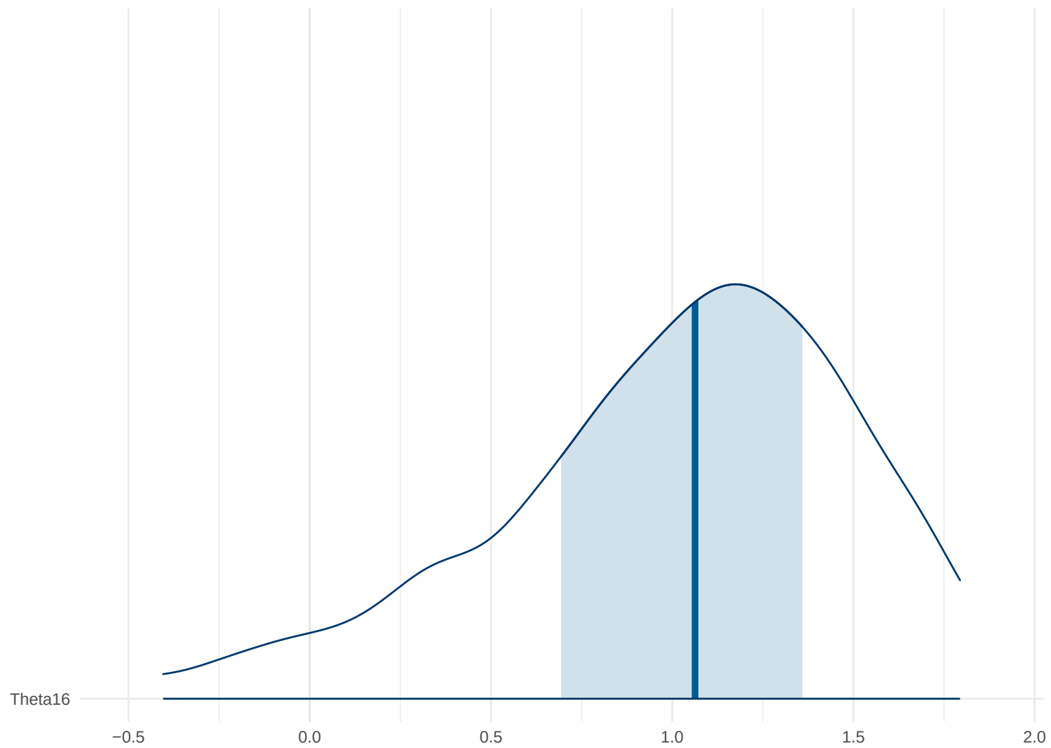
Posterior Density: Theta16
