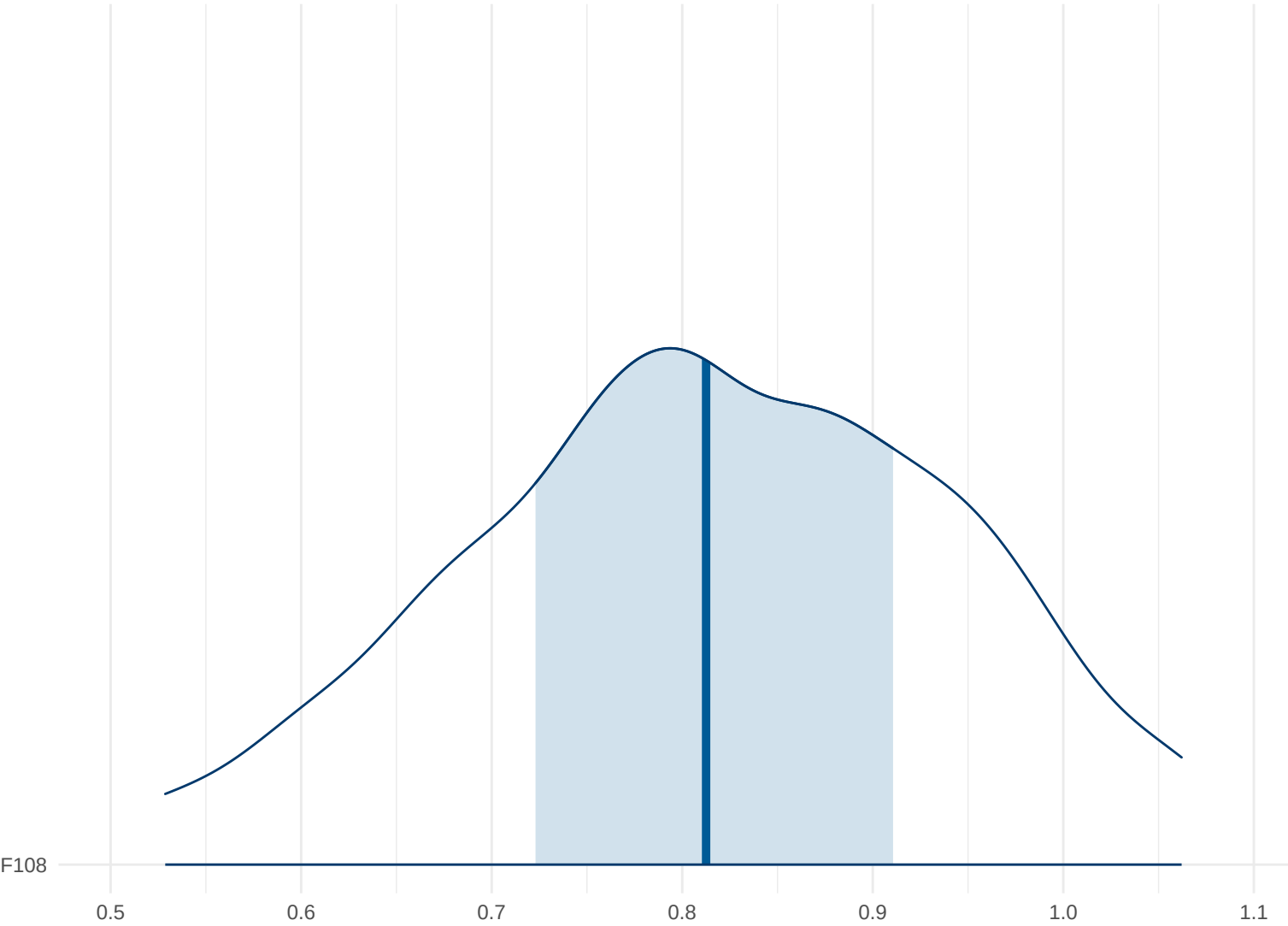
Posterior Density: F108
