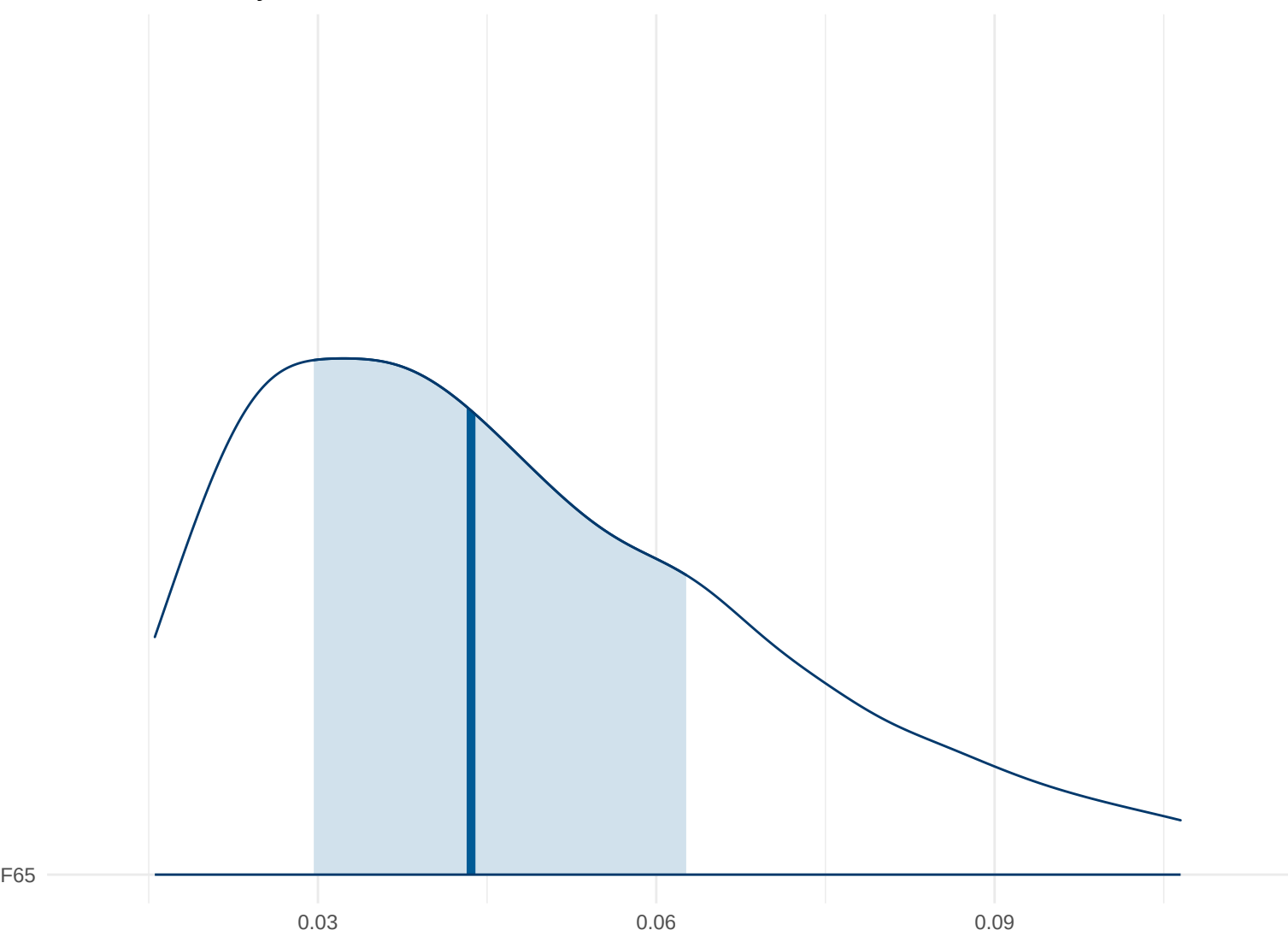
Posterior Density: F65
