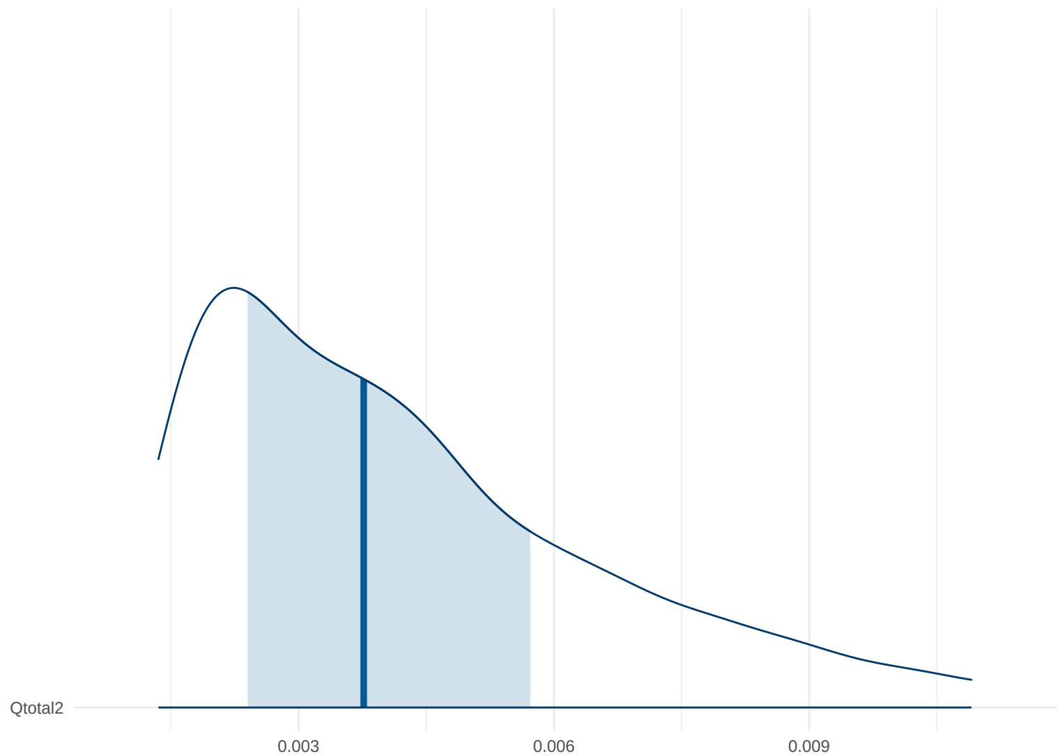
Posterior Density: Qtotal2
