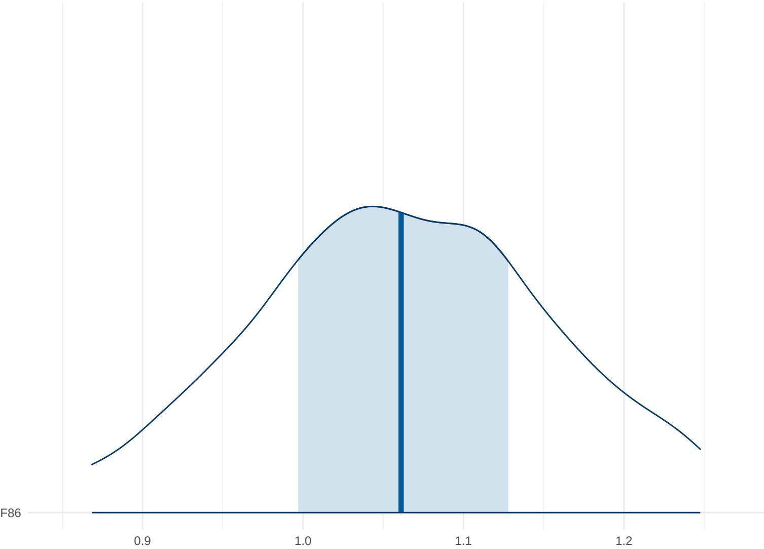
Posterior Density: F86
