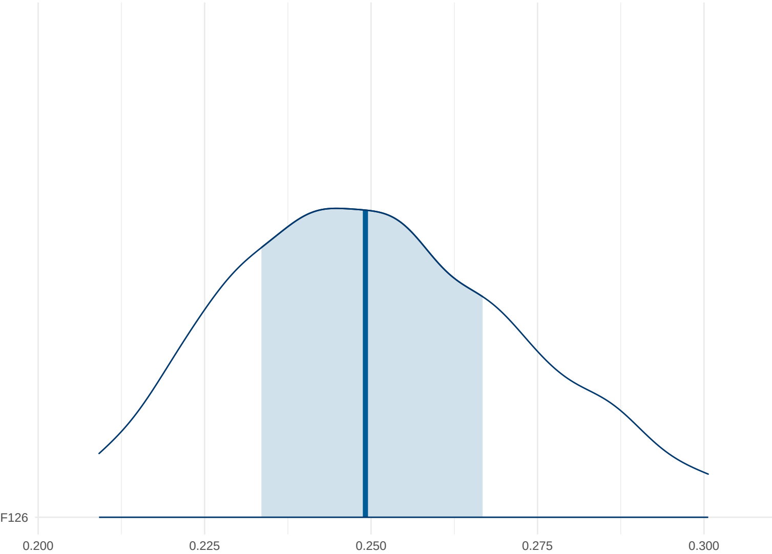
Posterior Density: F126
