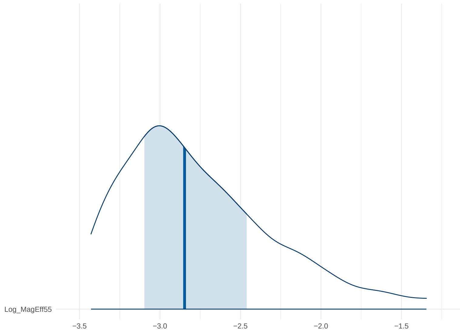
Posterior Density: Log_MagEff55
