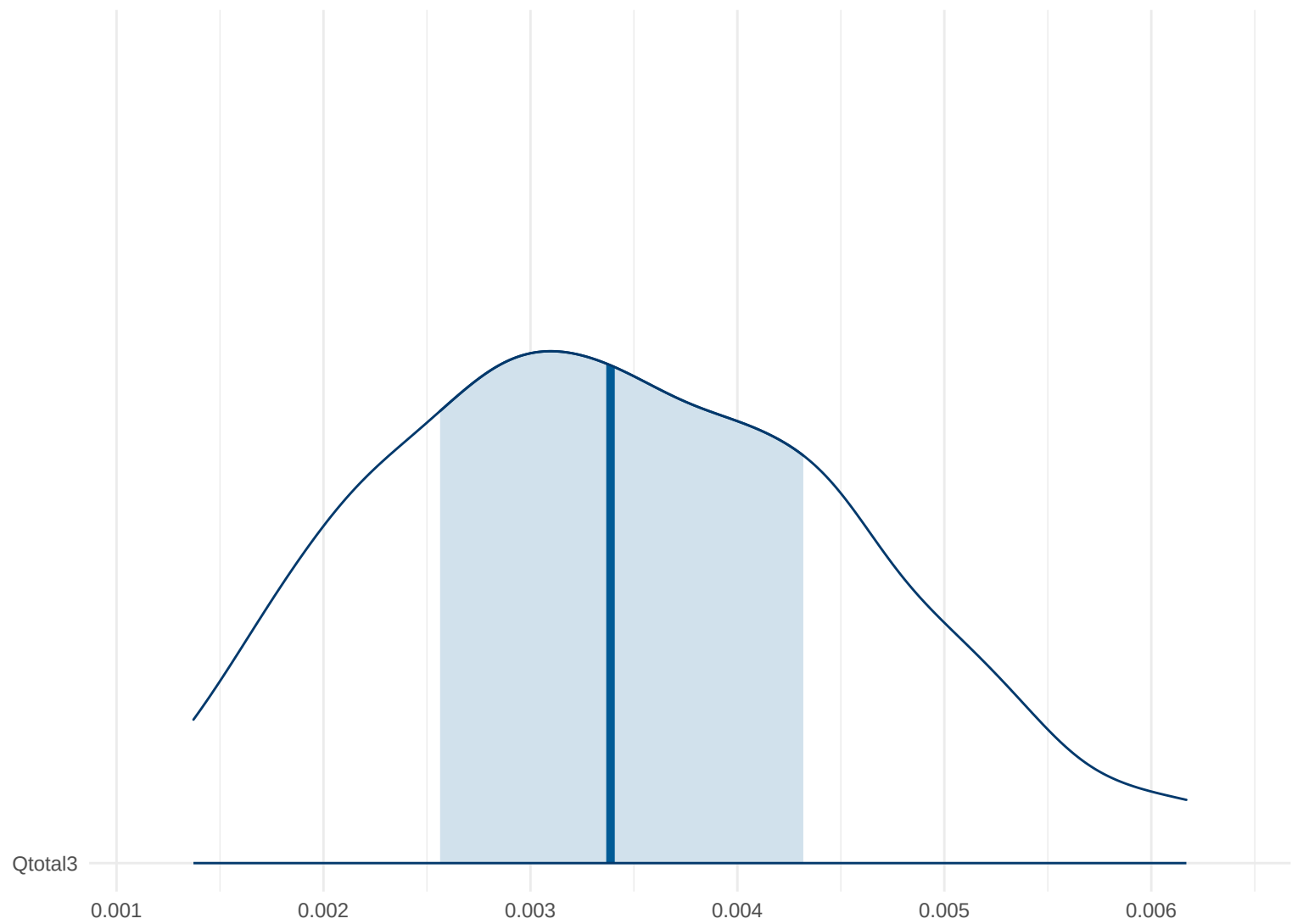
Posterior Density: Qtotal3
