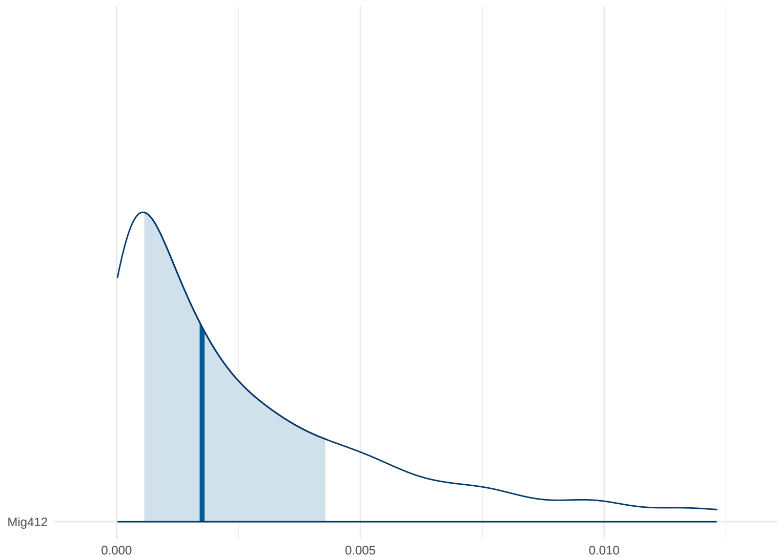
Posterior Density: Mig412
