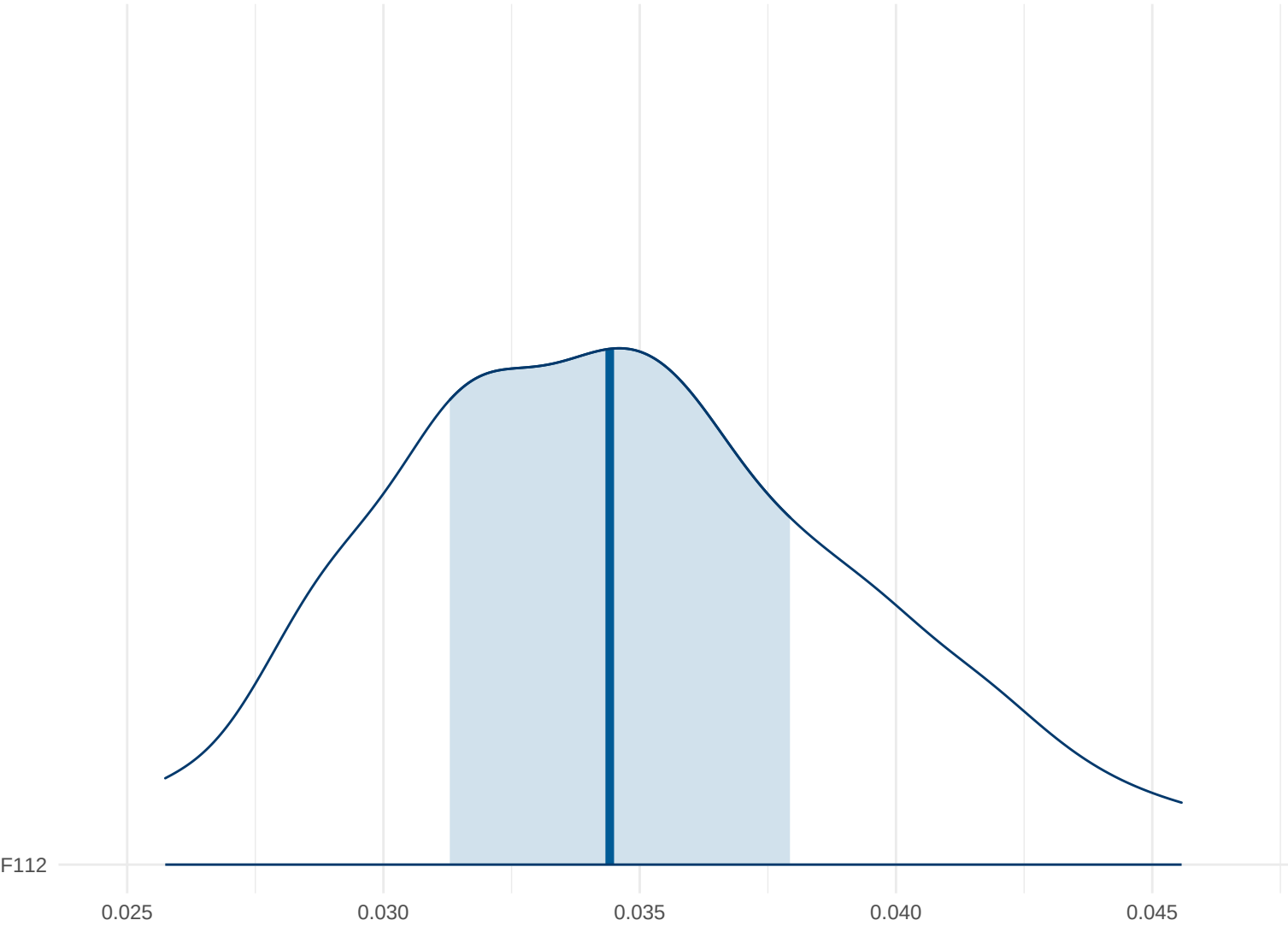
Posterior Density: F112
