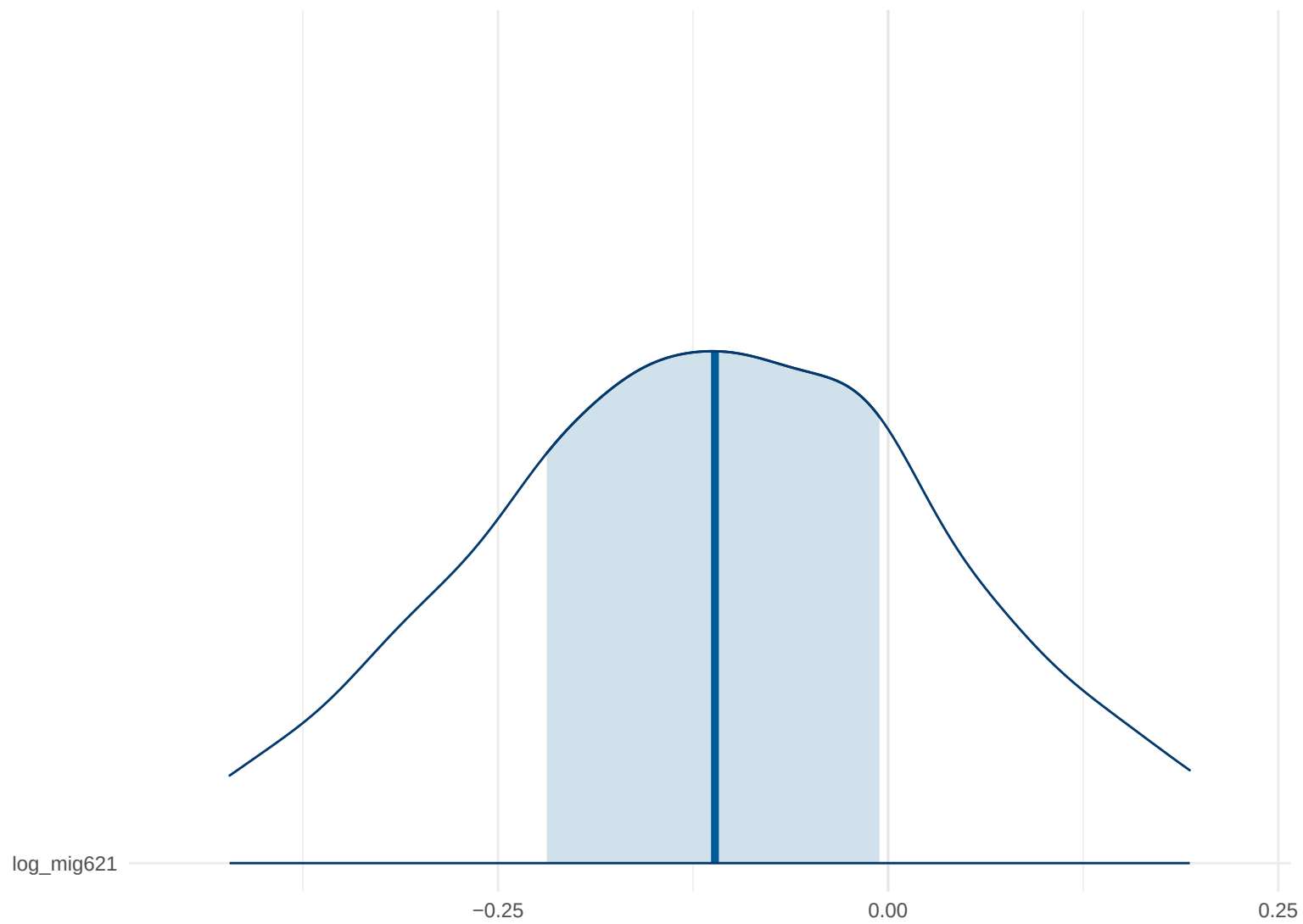
Posterior Density: log_mig621
