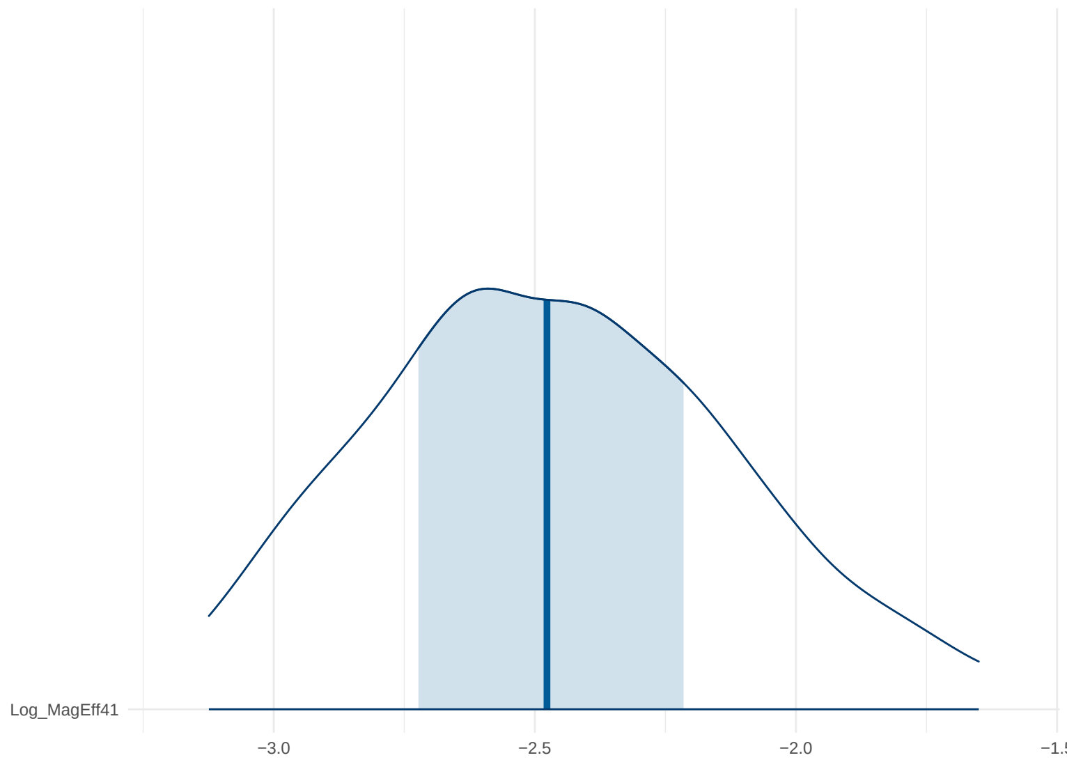
Posterior Density: Log_MagEff41
