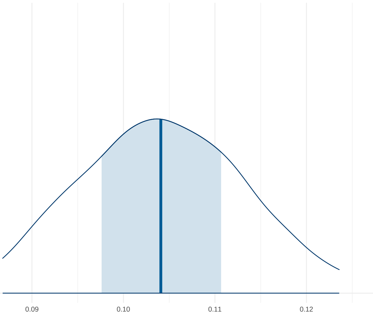
Posterior Density: Mig623
