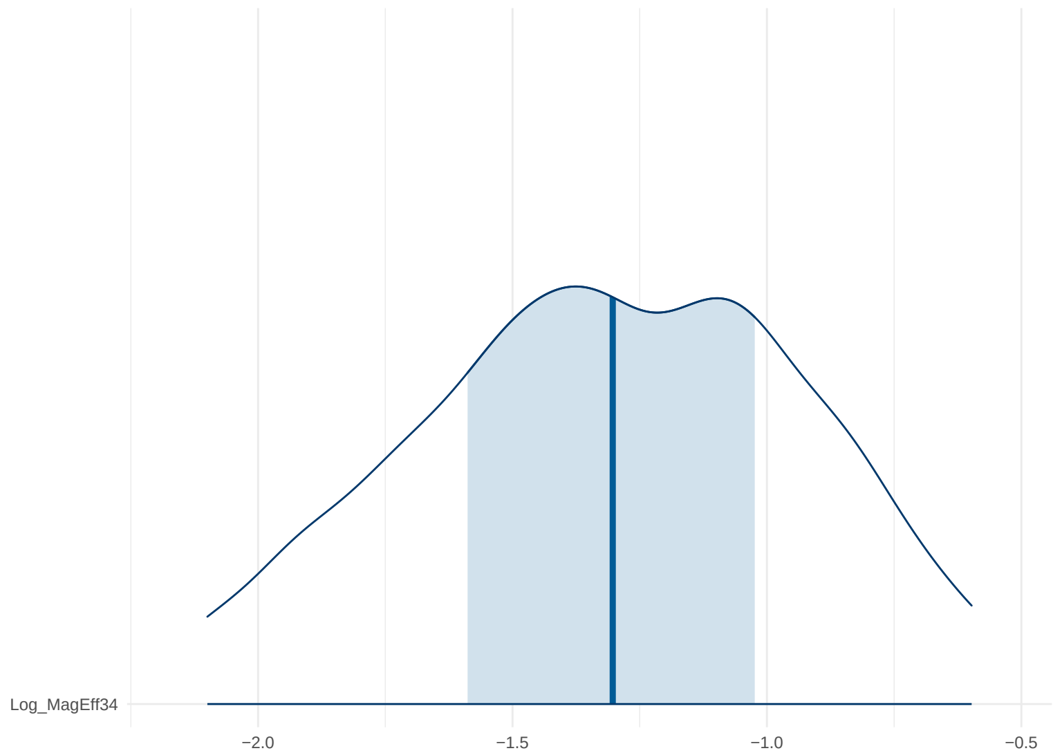
Posterior Density: Log_MagEff34
