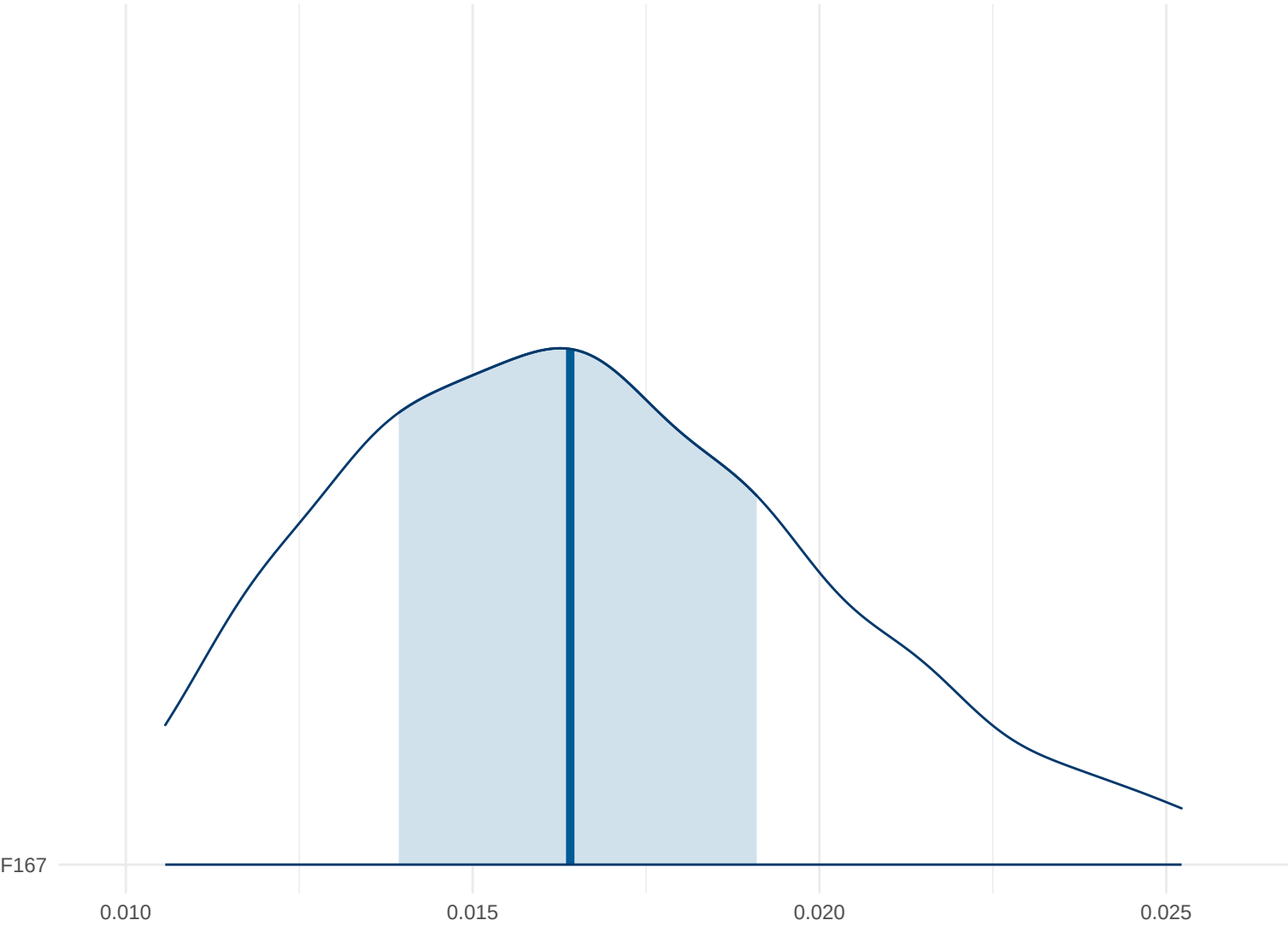
Posterior Density: F167
