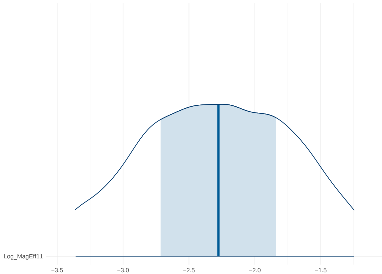
Posterior Density: Log_MagEff11
