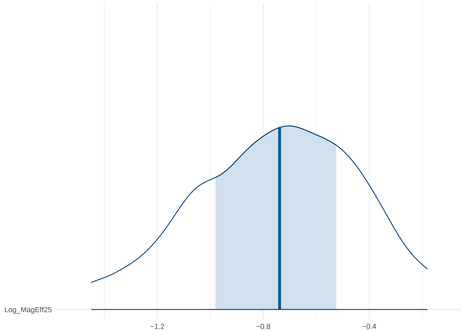
Posterior Density: Log_MagEff25
