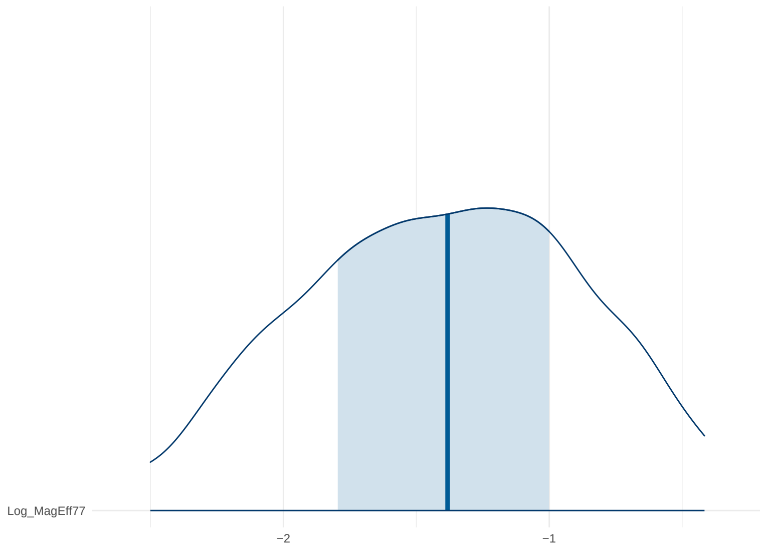
Posterior Density: Log_MagEff77
