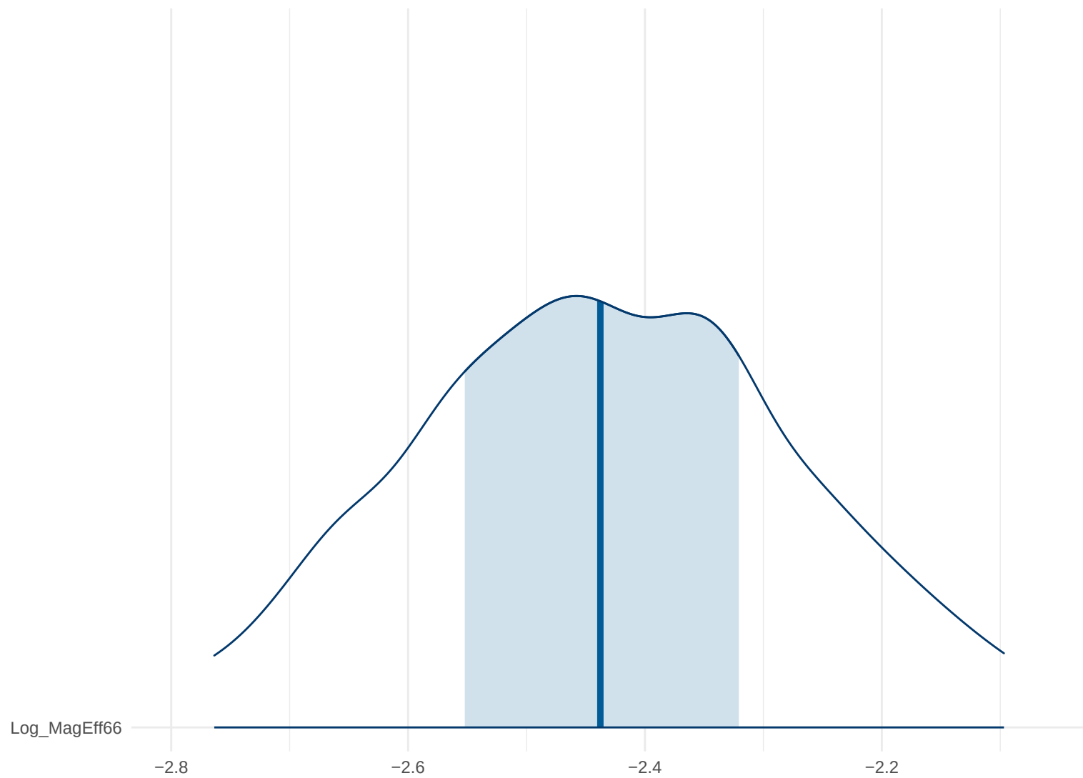
Posterior Density: Log_MagEff66
