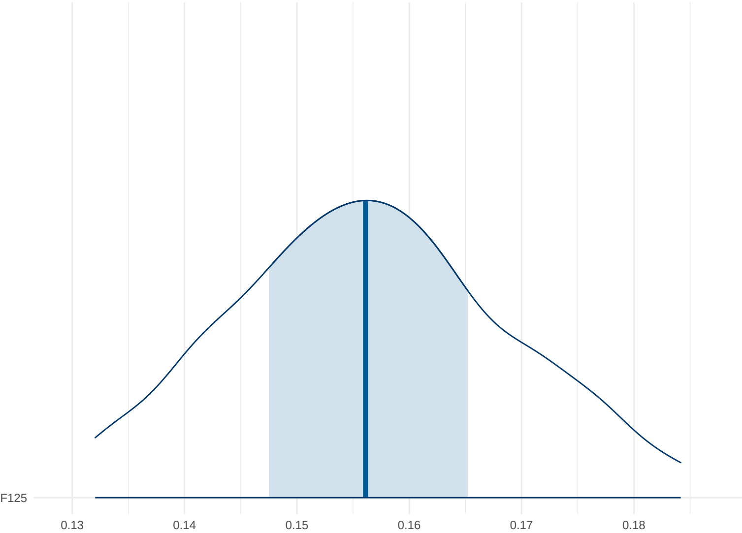
Posterior Density: F125
