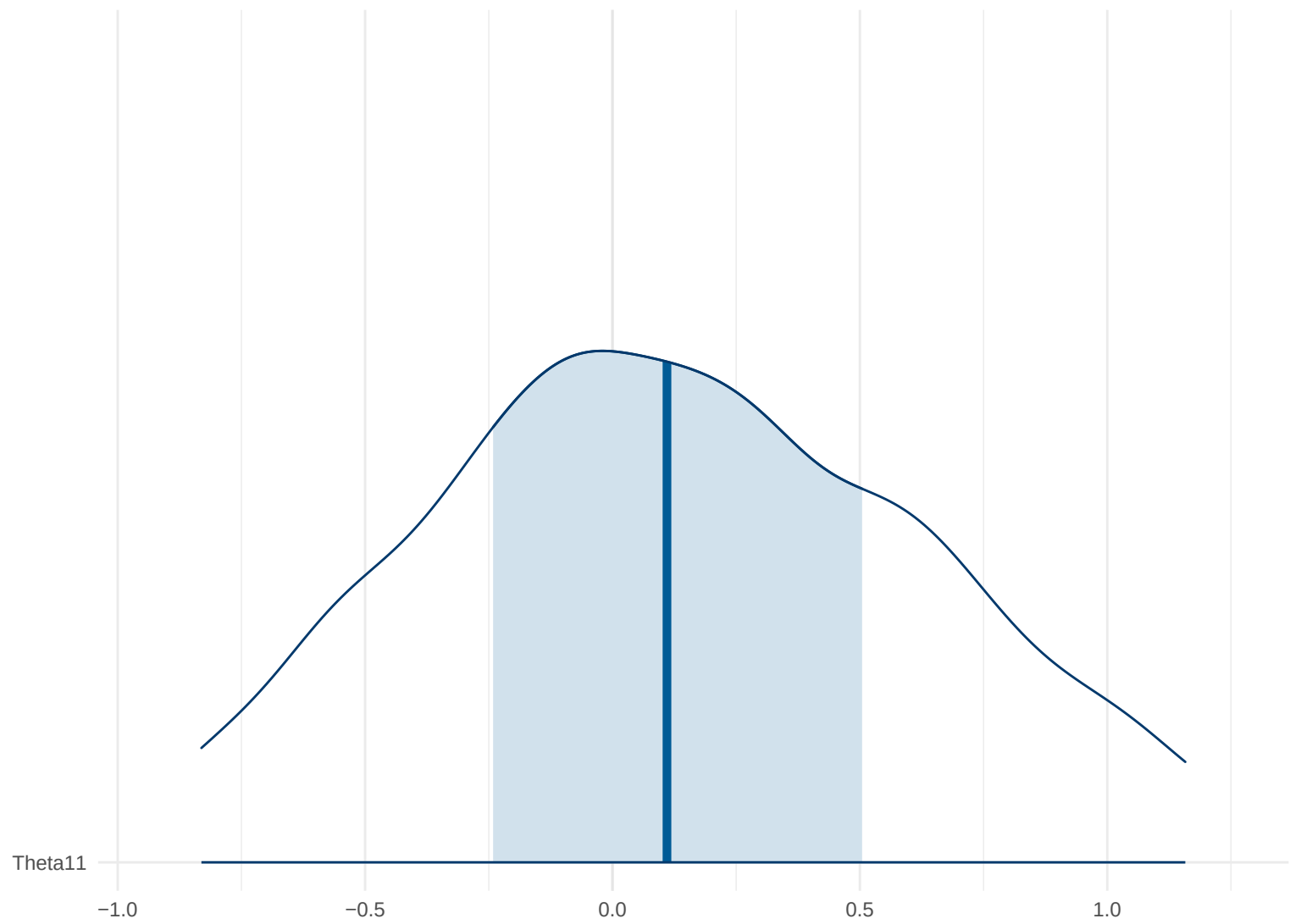
Posterior Density: Theta11
