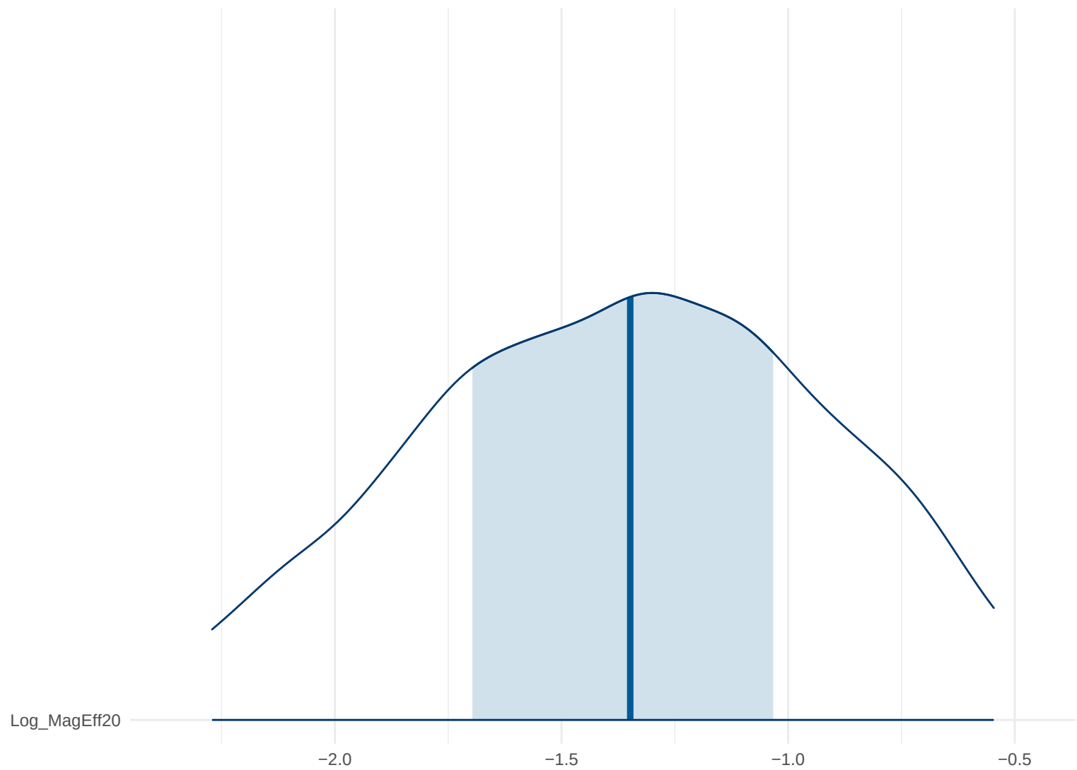
Posterior Density: Log_MagEff20
