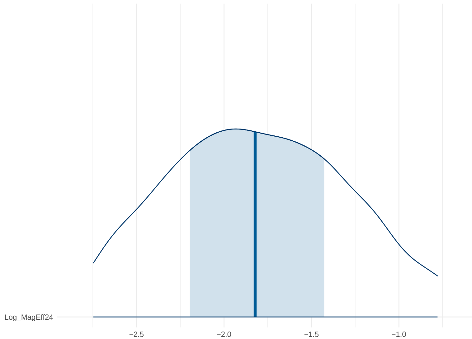
Posterior Density: Log_MagEff24
