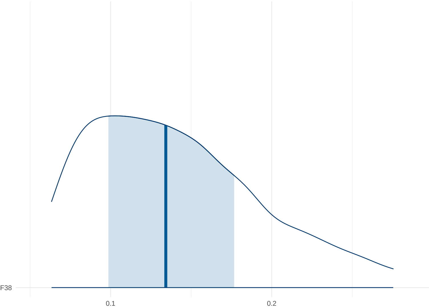
Posterior Density: F38
