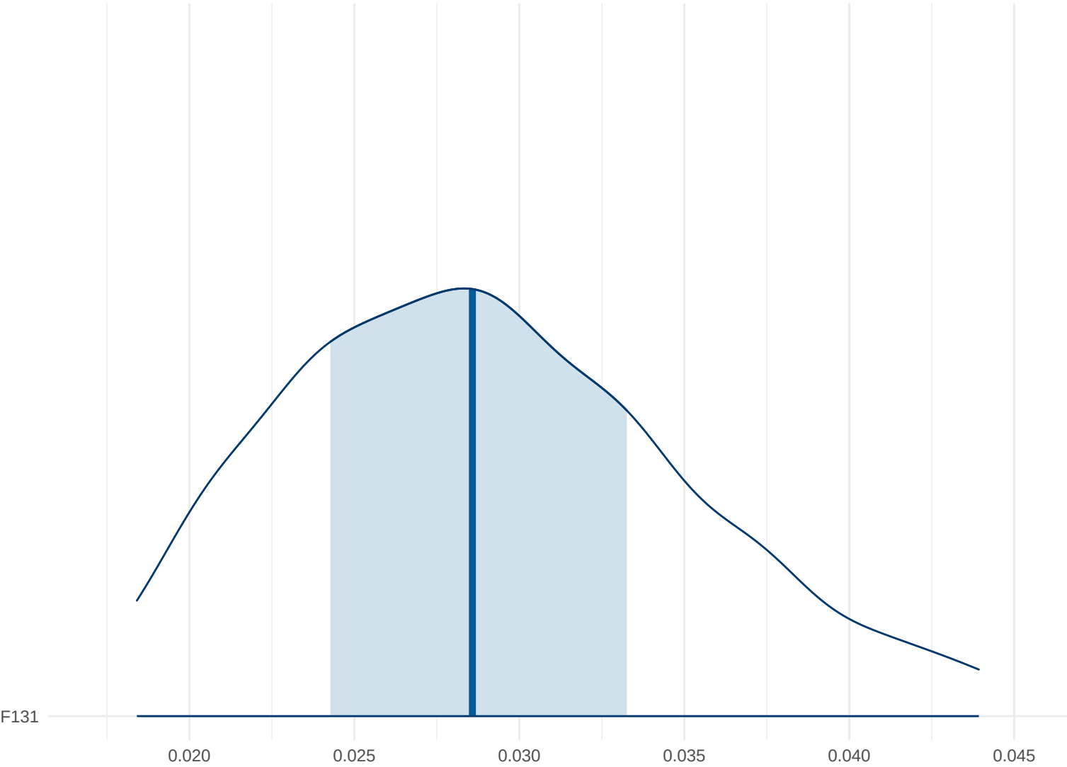
Posterior Density: F131
