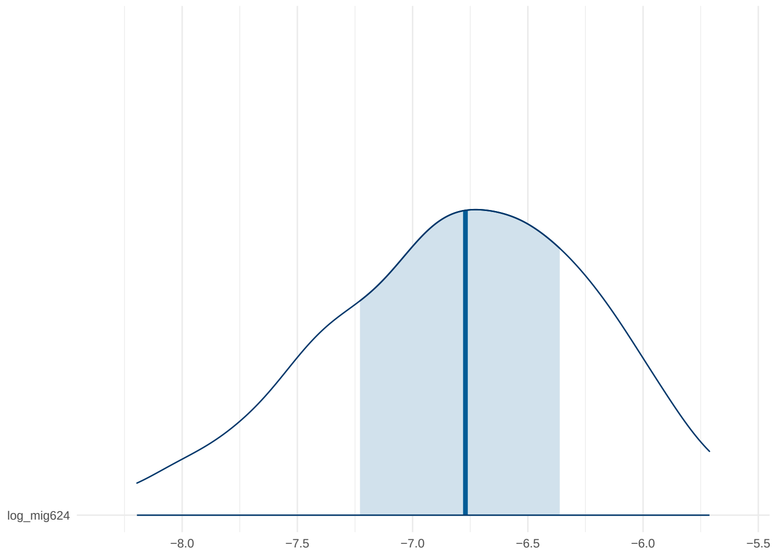
Posterior Density: log_mig624
