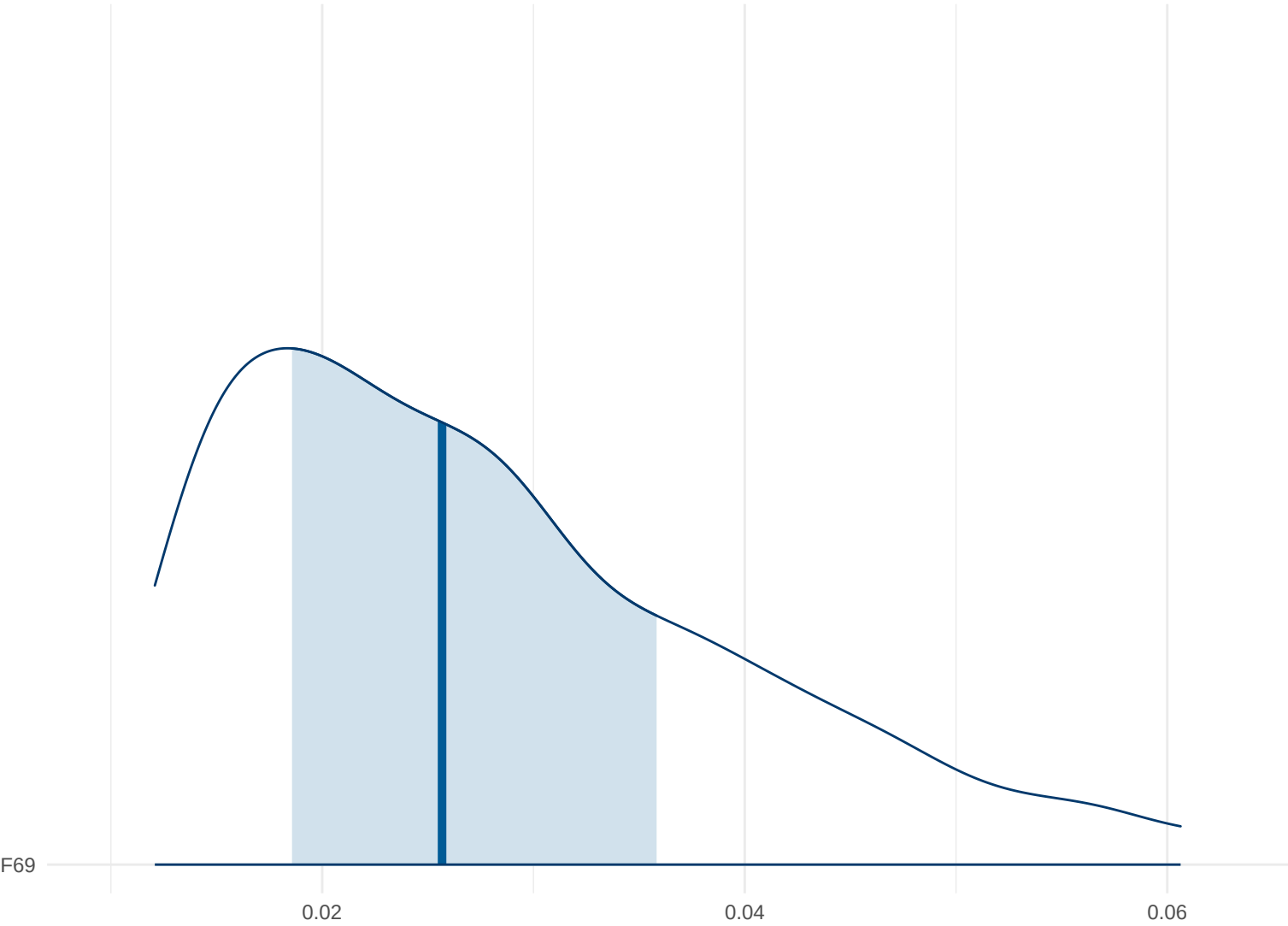
Posterior Density: F69
