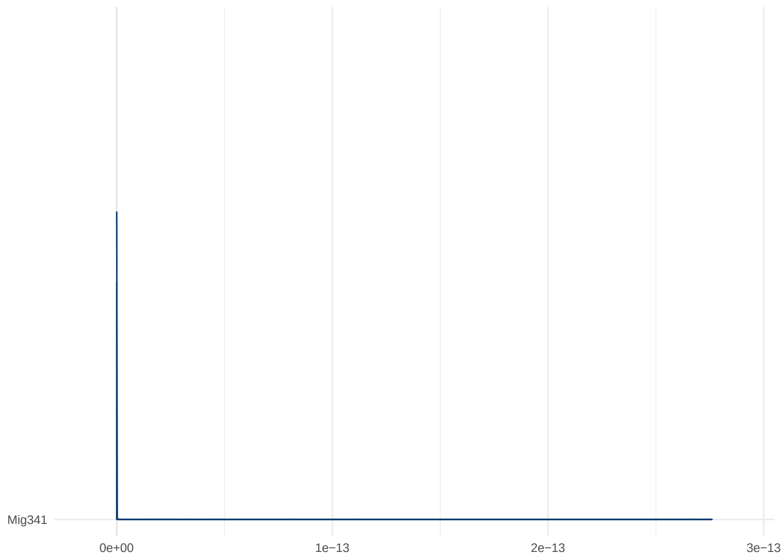
Posterior Density: Mig341
