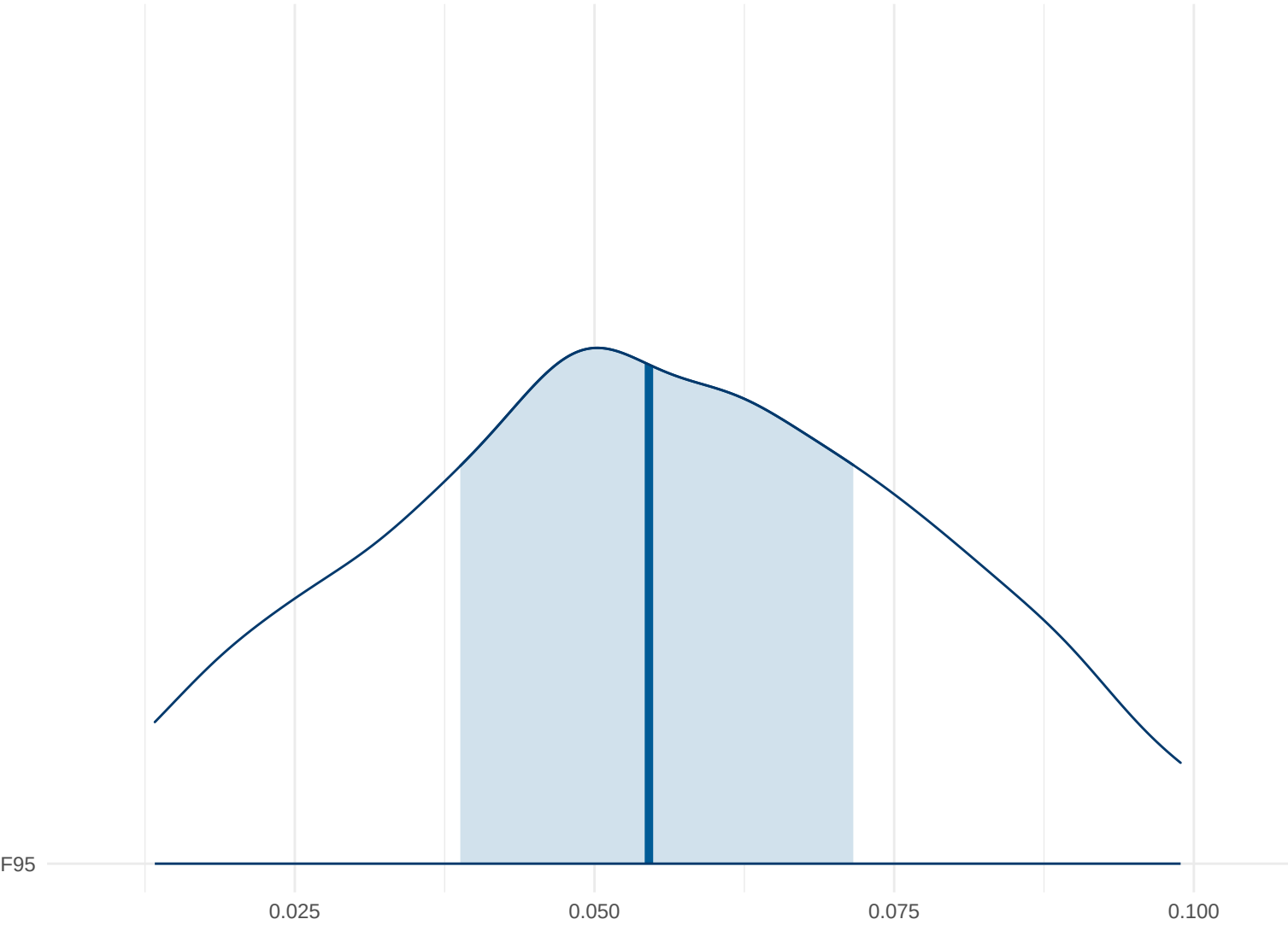
Posterior Density: F95
