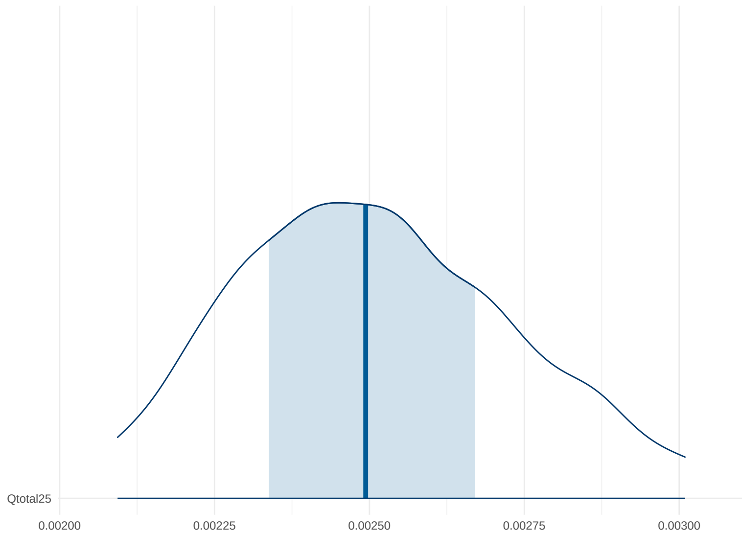
Posterior Density: Qtotal25
