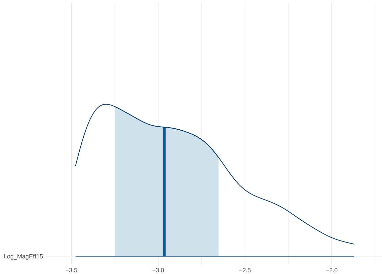
Posterior Density: Log_MagEff15
