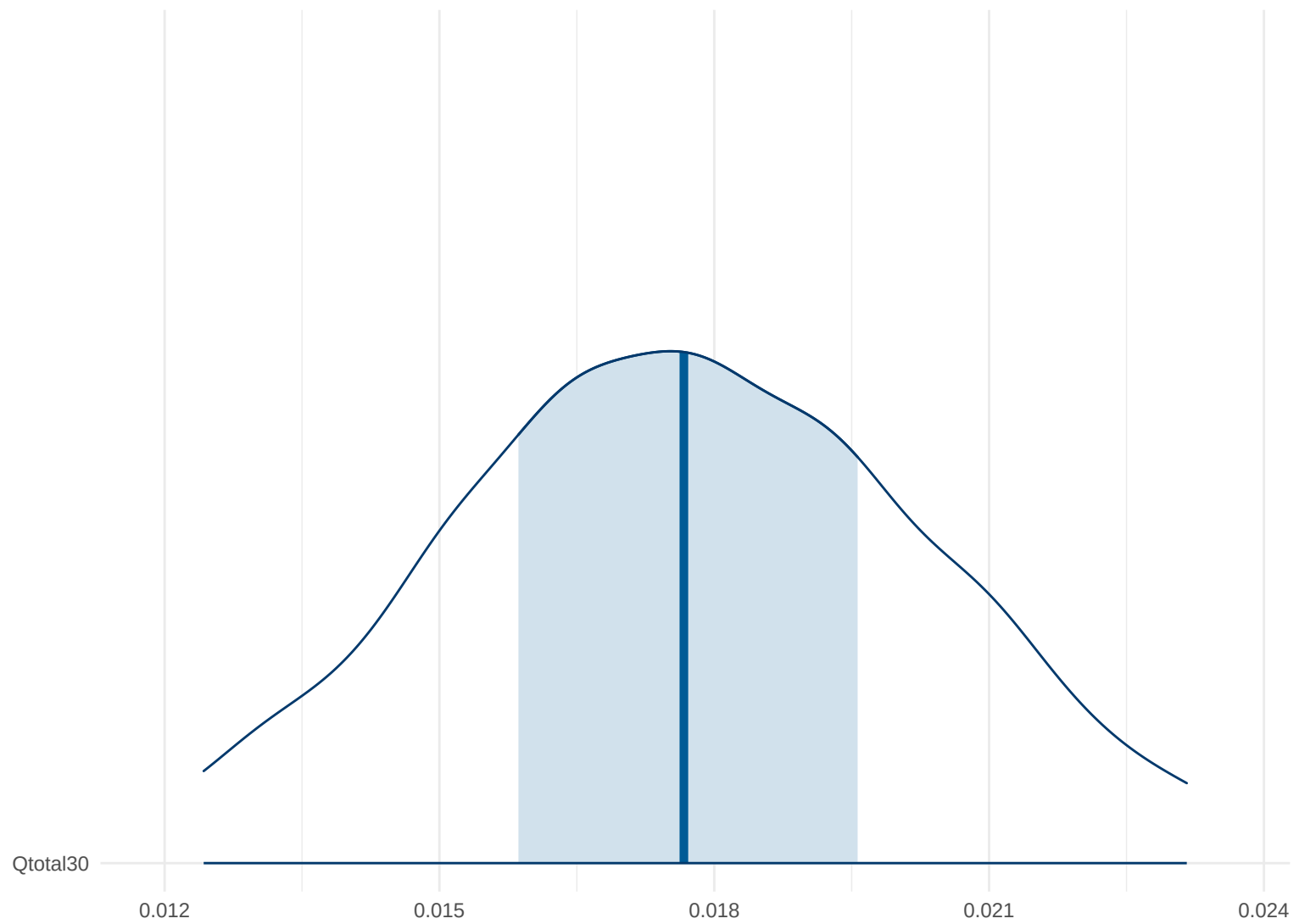
Posterior Density: Qtotal30
