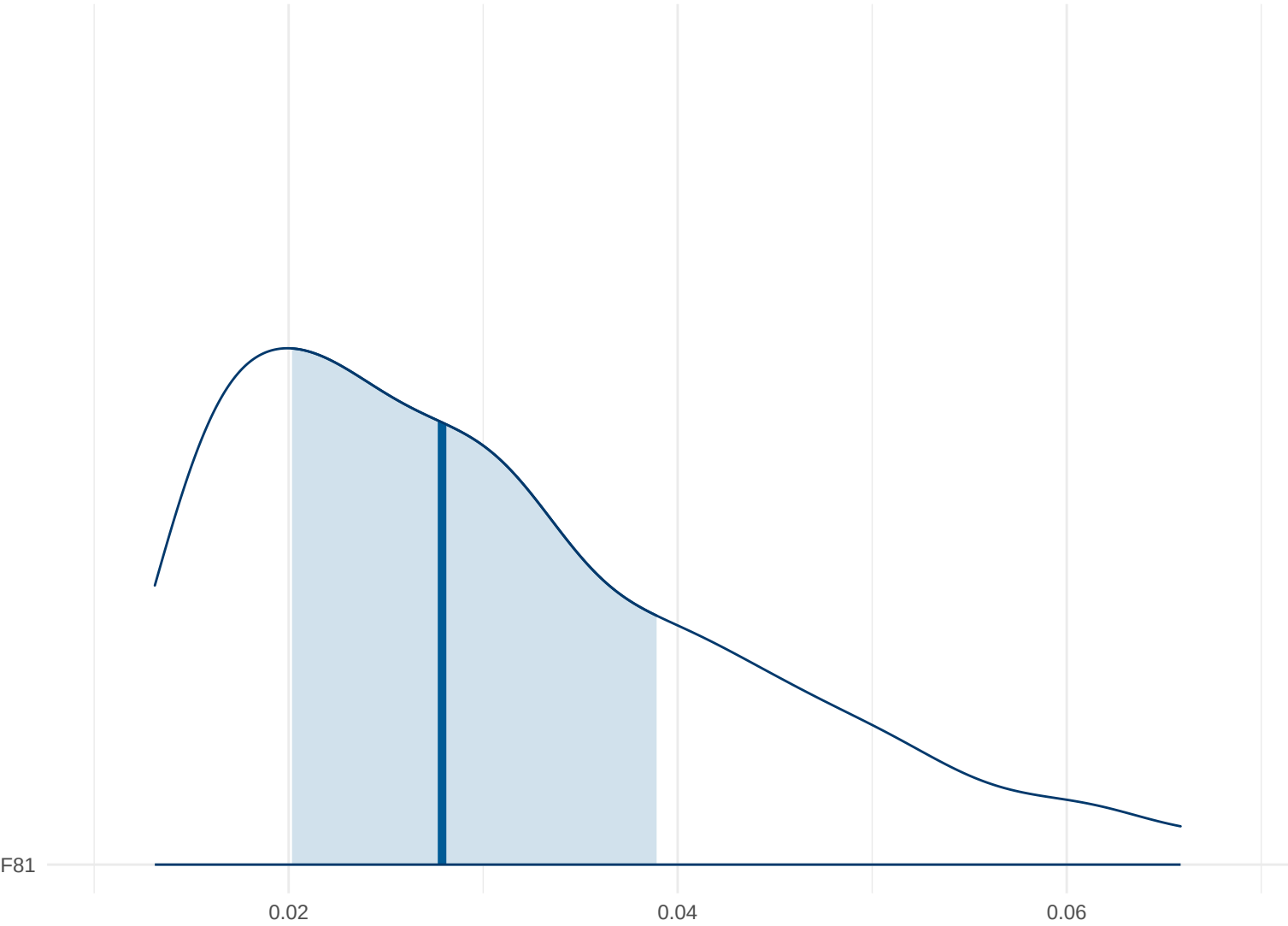
Posterior Density: F81
