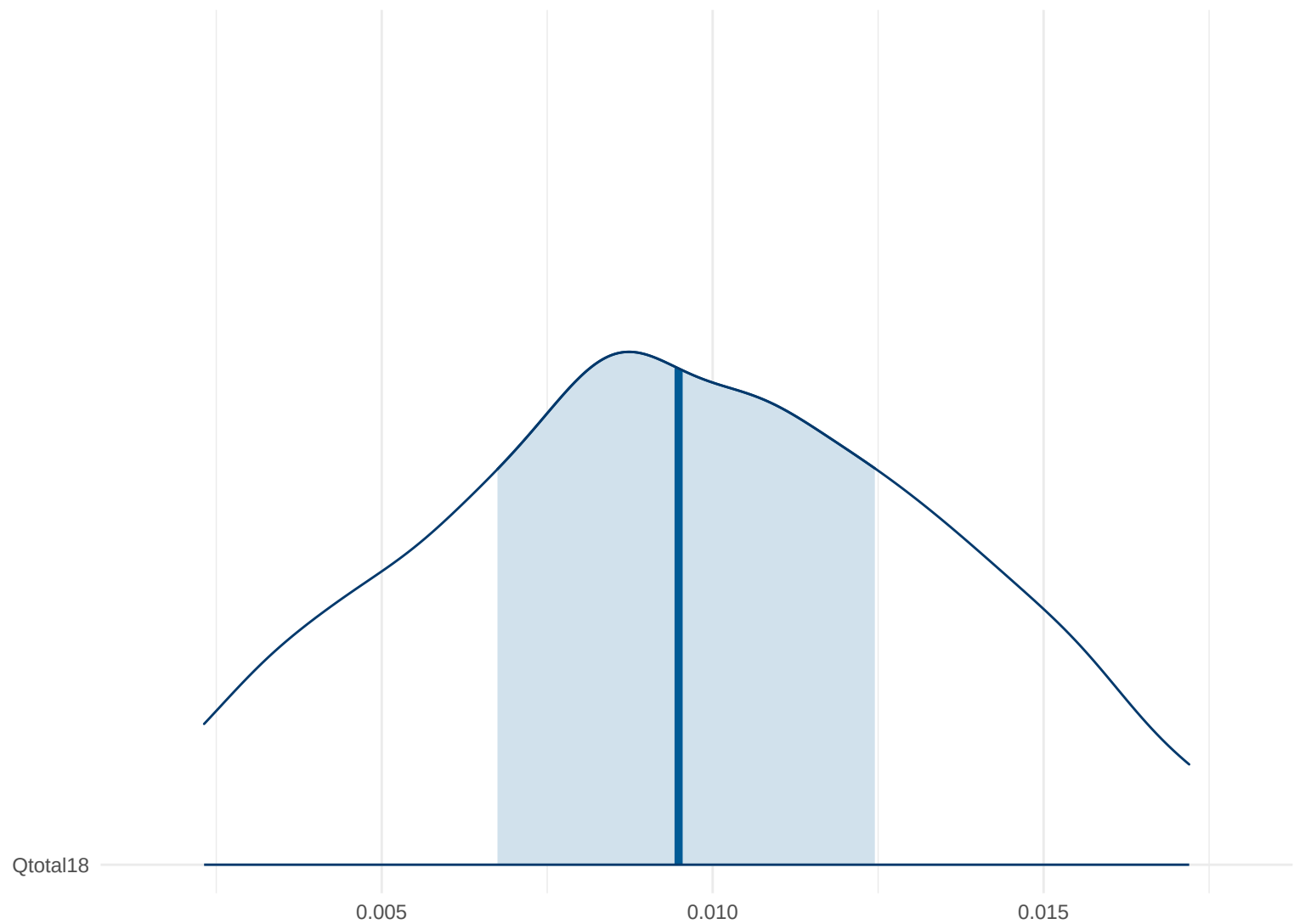
Posterior Density: Qtotal18
