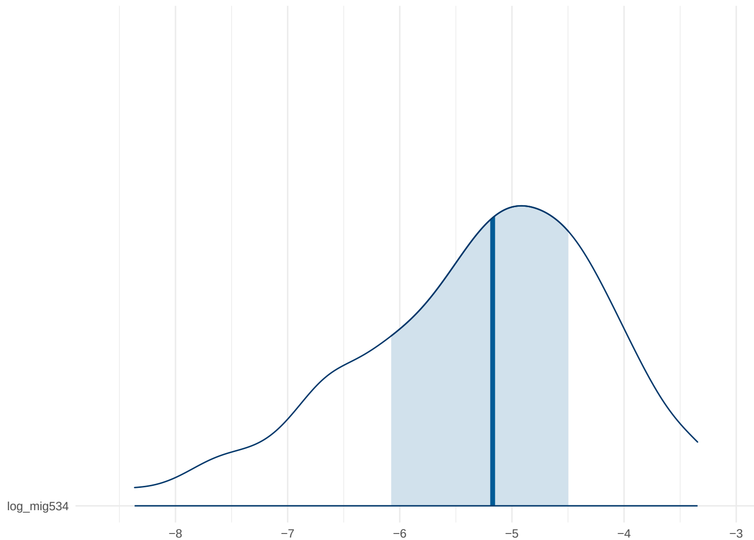
Posterior Density: log_mig534
