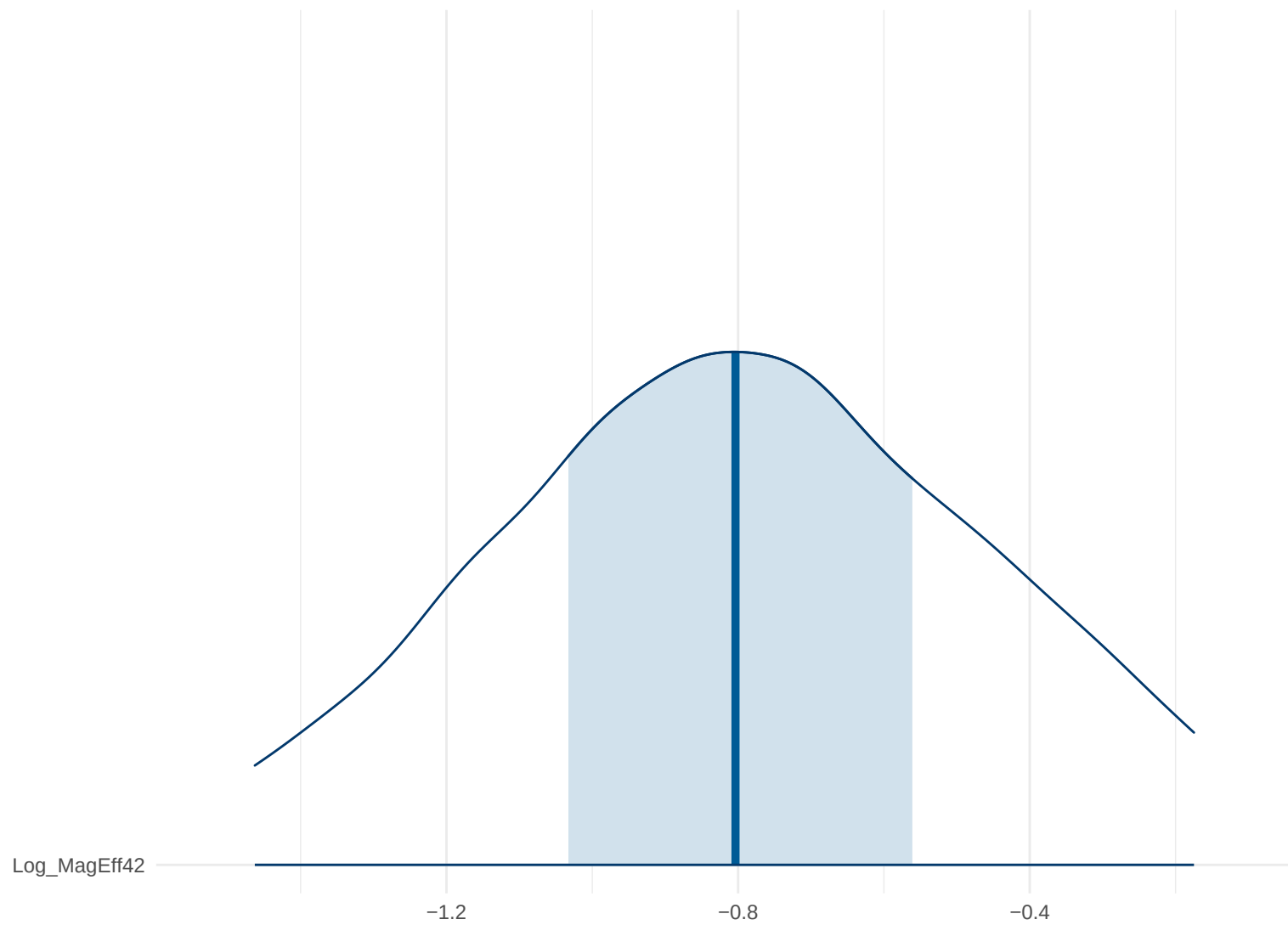
Posterior Density: Log_MagEff42
