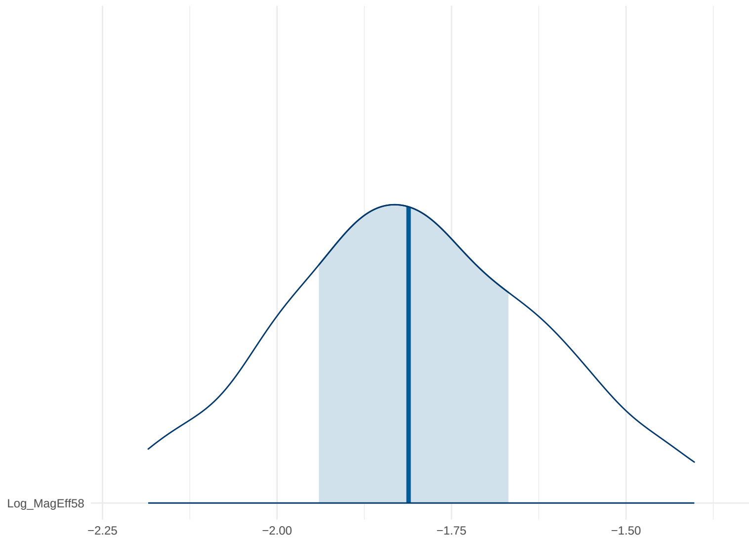
Posterior Density: Log_MagEff58
