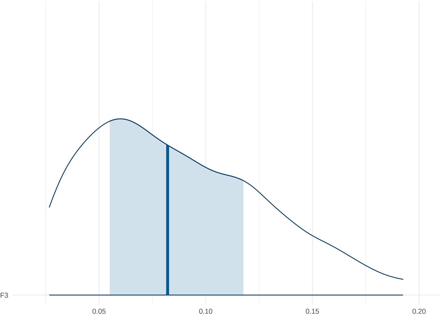
Posterior Density: F3
