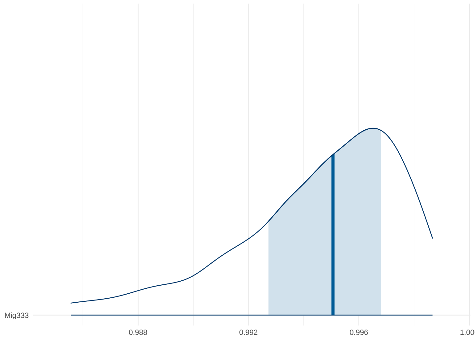
Posterior Density: Mig333
