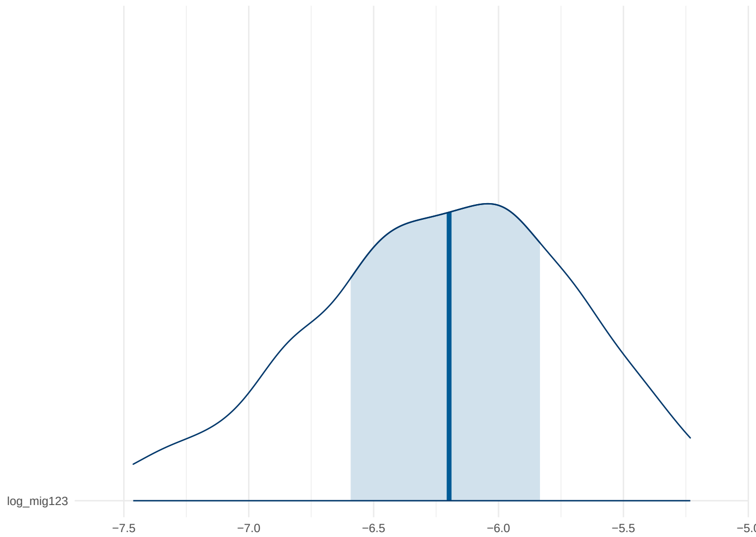
Posterior Density: log_mig123
