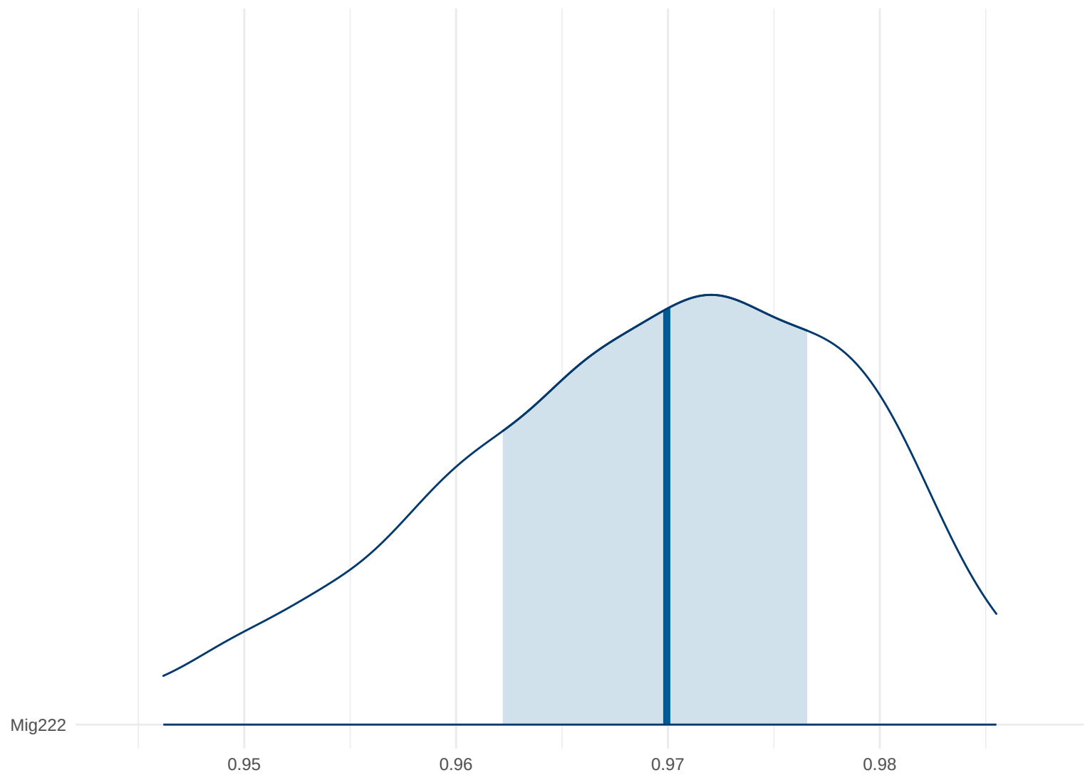
Posterior Density: Mig222
