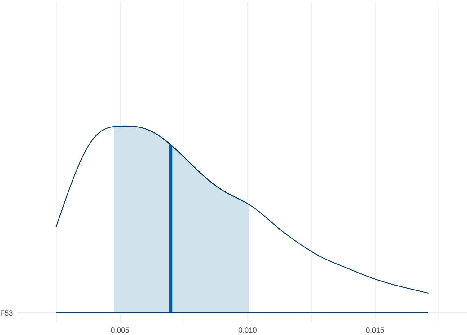
Posterior Density: F53
