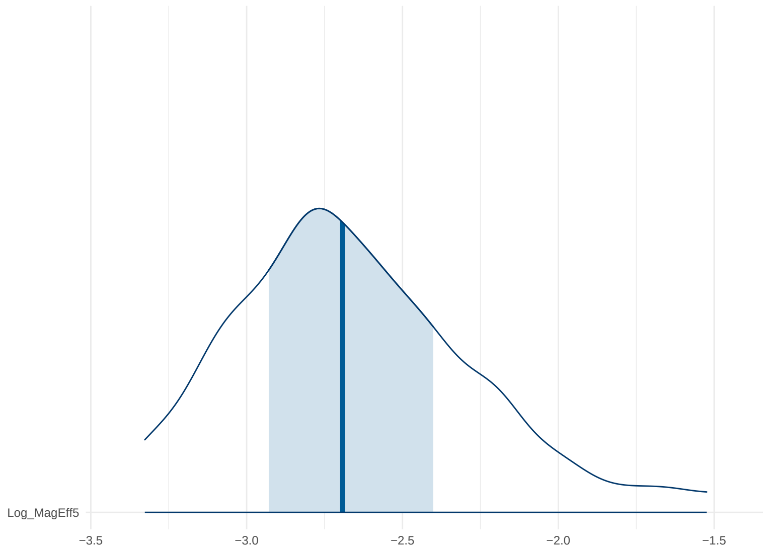
Posterior Density: Log_MagEff5
