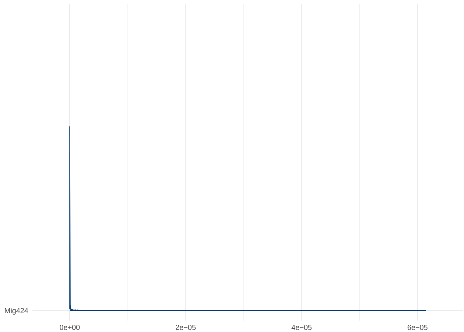
Posterior Density: Mig424
