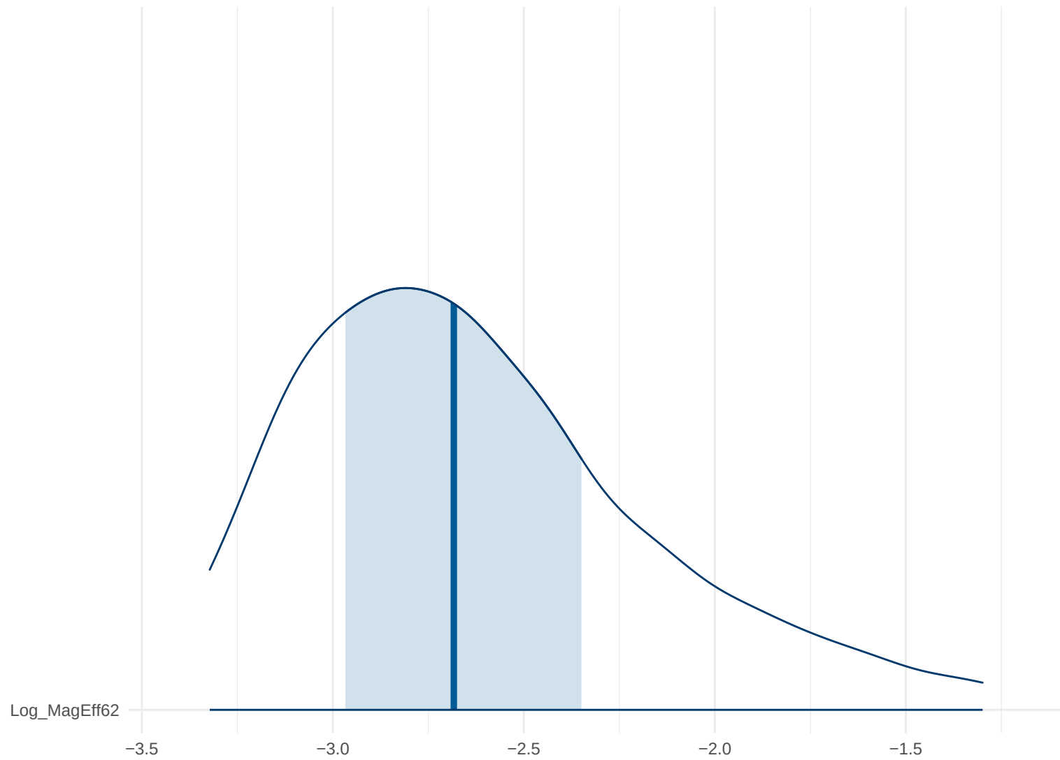
Posterior Density: Log_MagEff62
