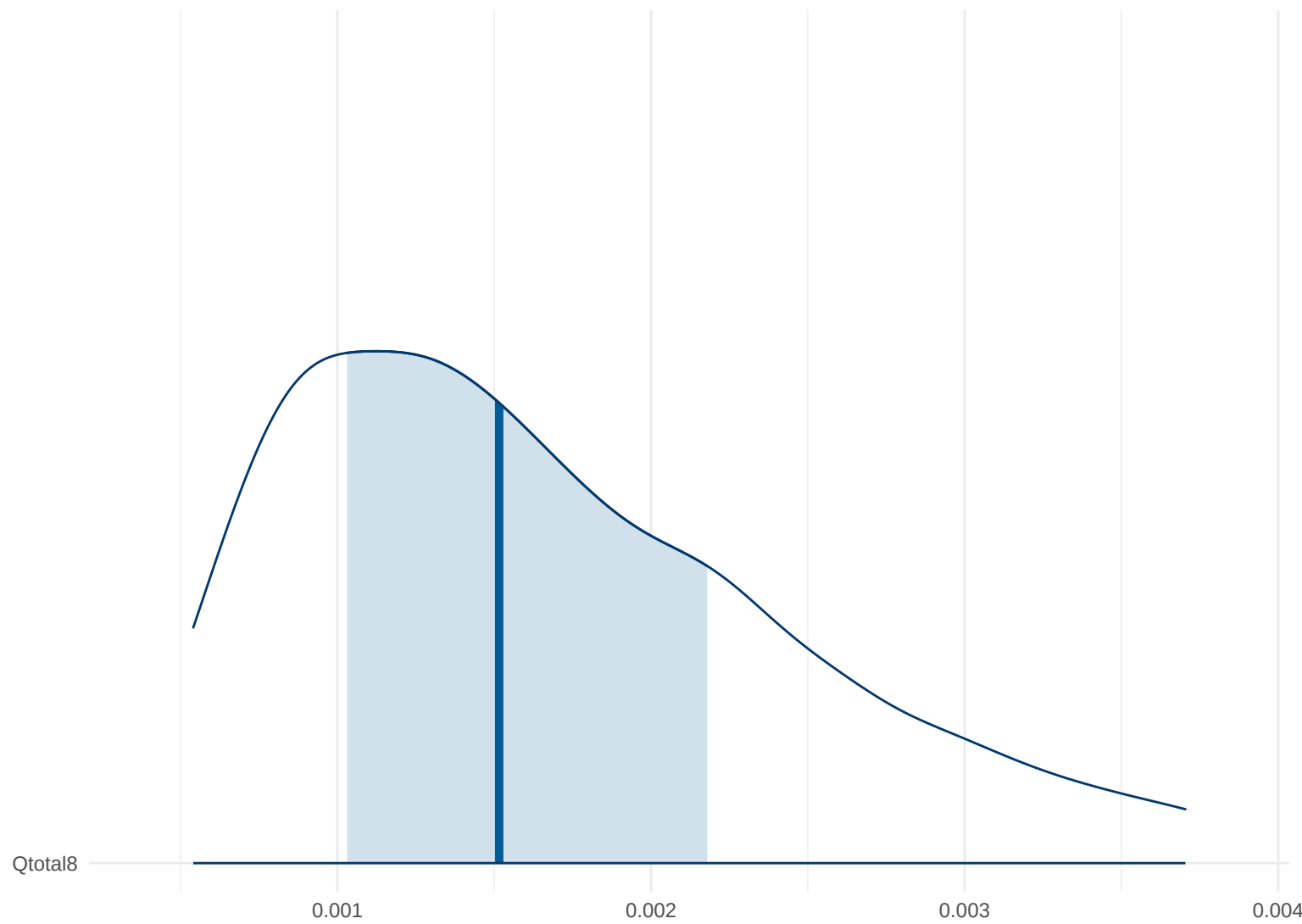
Posterior Density: Qtotal8
