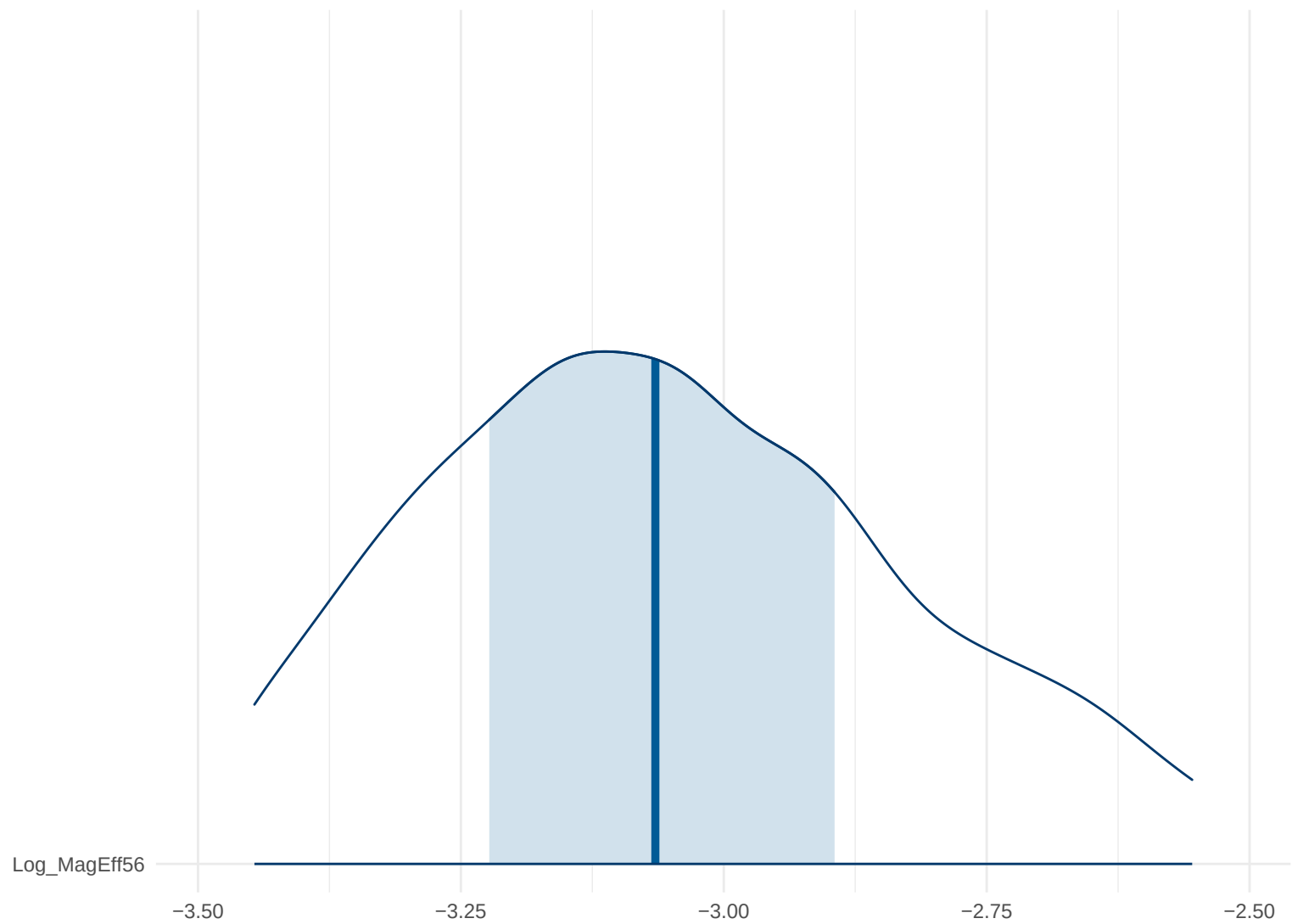
Posterior Density: Log_MagEff56
