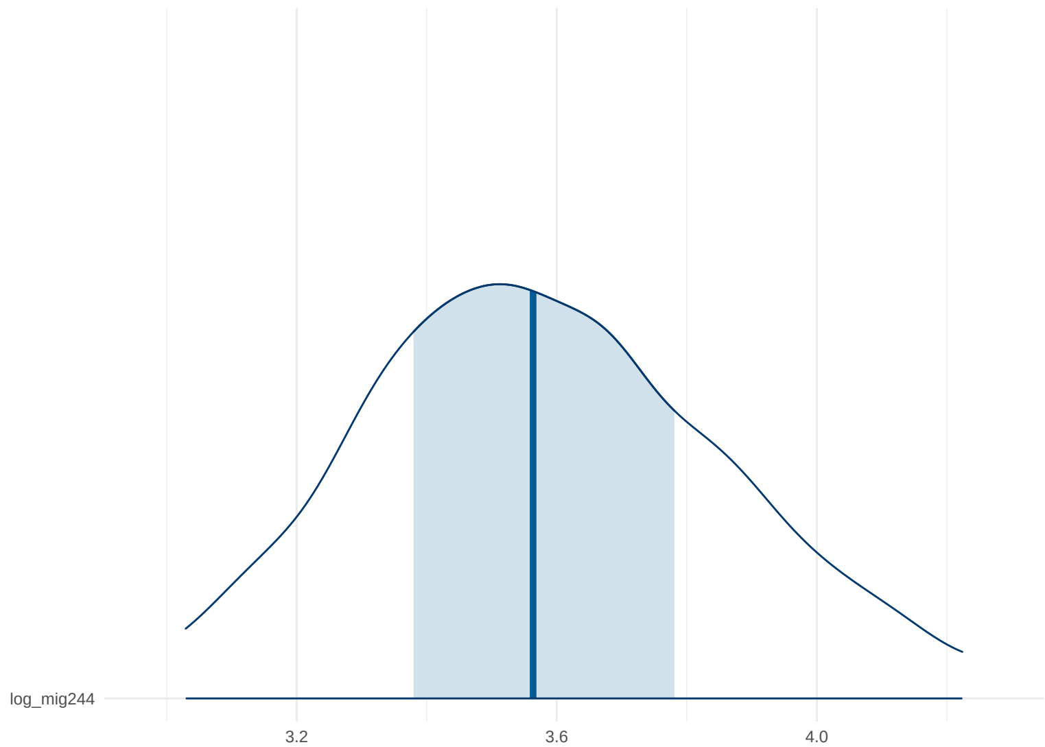
Posterior Density: log_mig244
