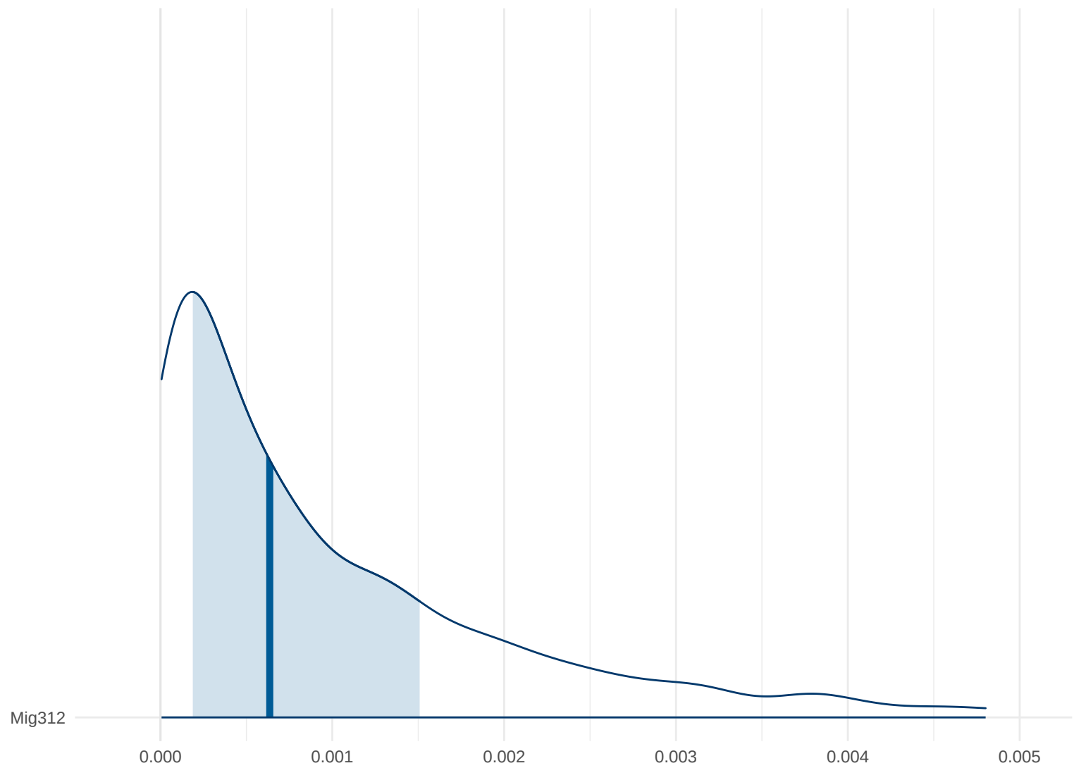
Posterior Density: Mig312
