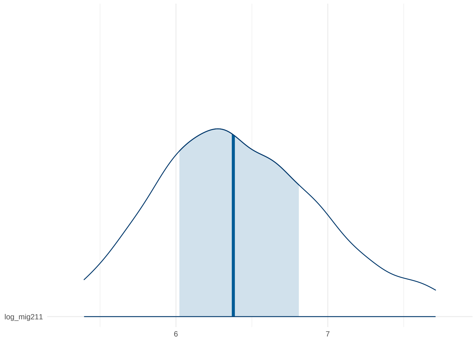
Posterior Density: log_mig211
