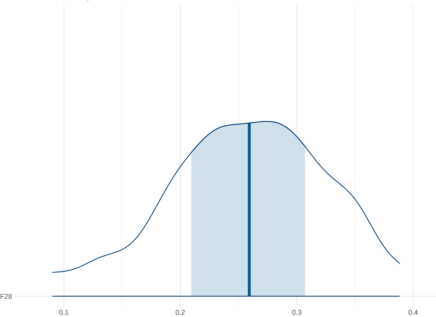
Posterior Density: F28
