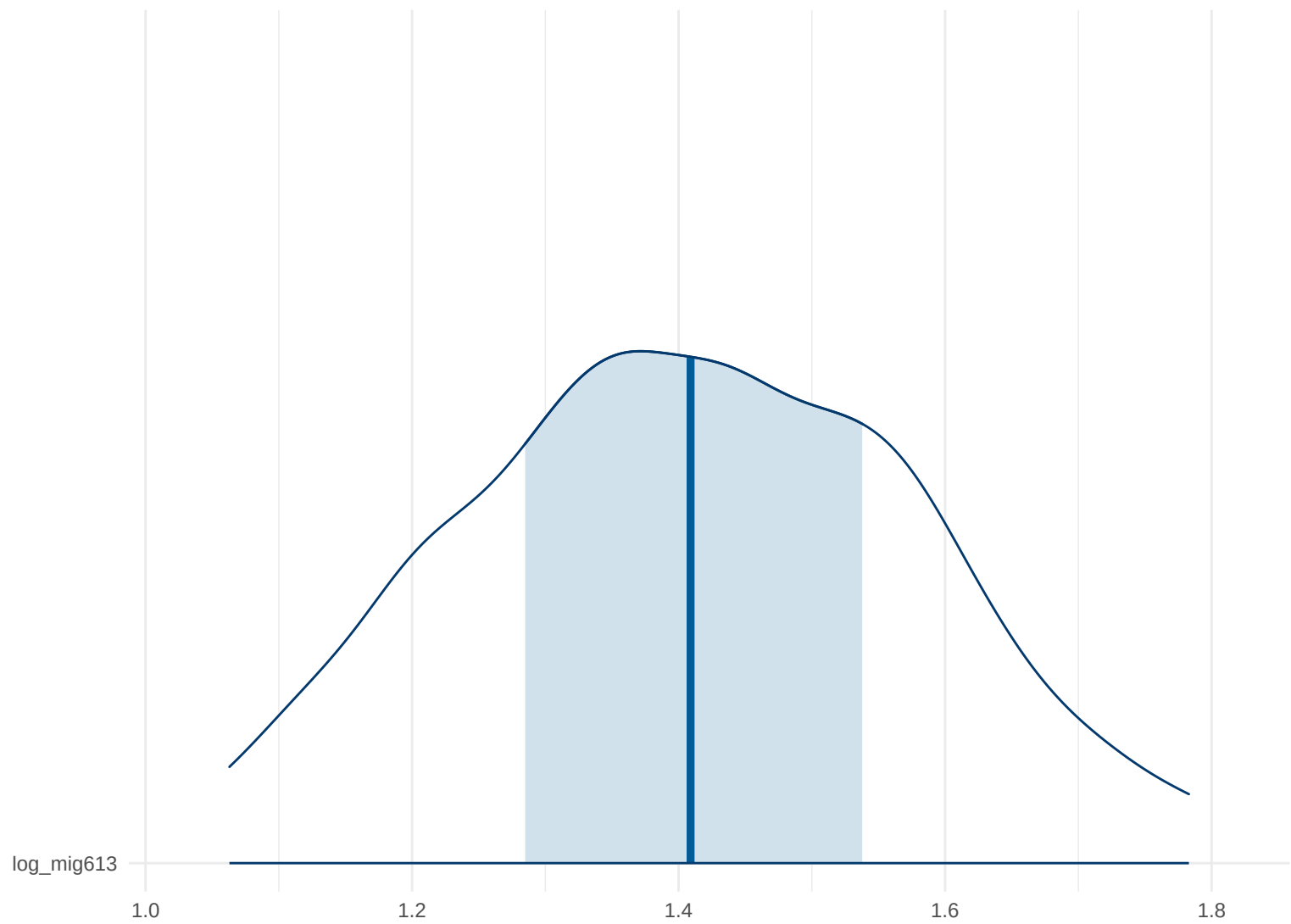
Posterior Density: log_mig613
