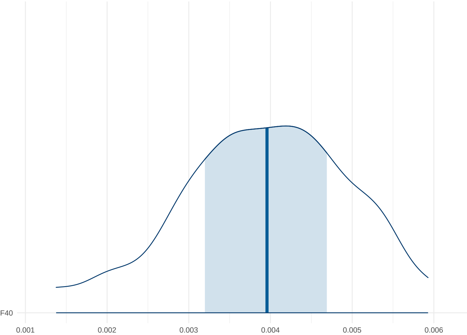
Posterior Density: F40
