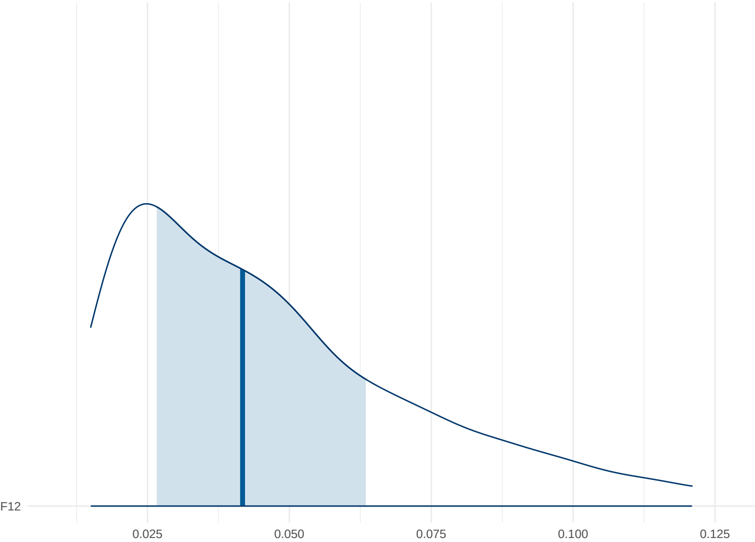
Posterior Density: F12
