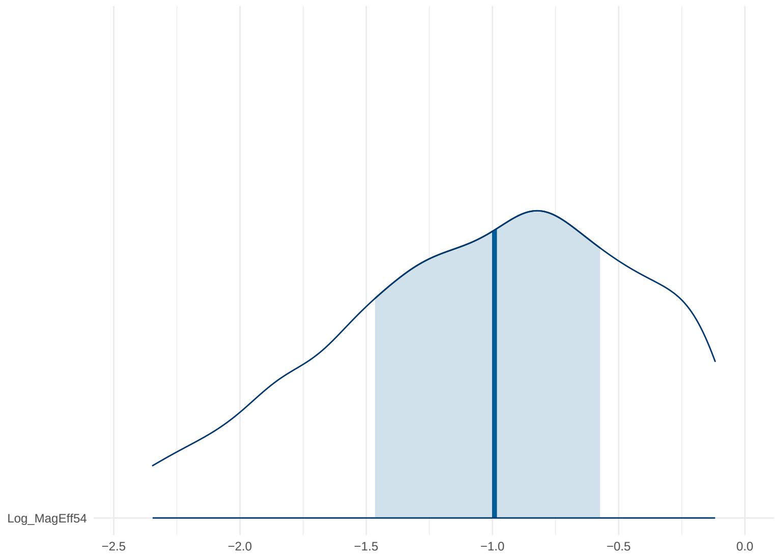
Posterior Density: Log_MagEff54
