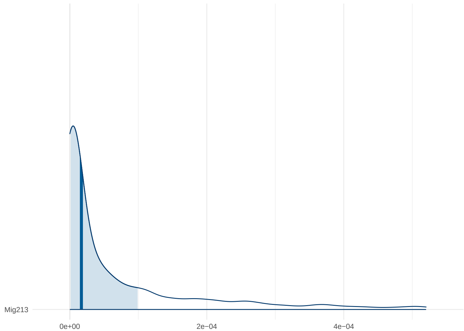
Posterior Density: Mig213
