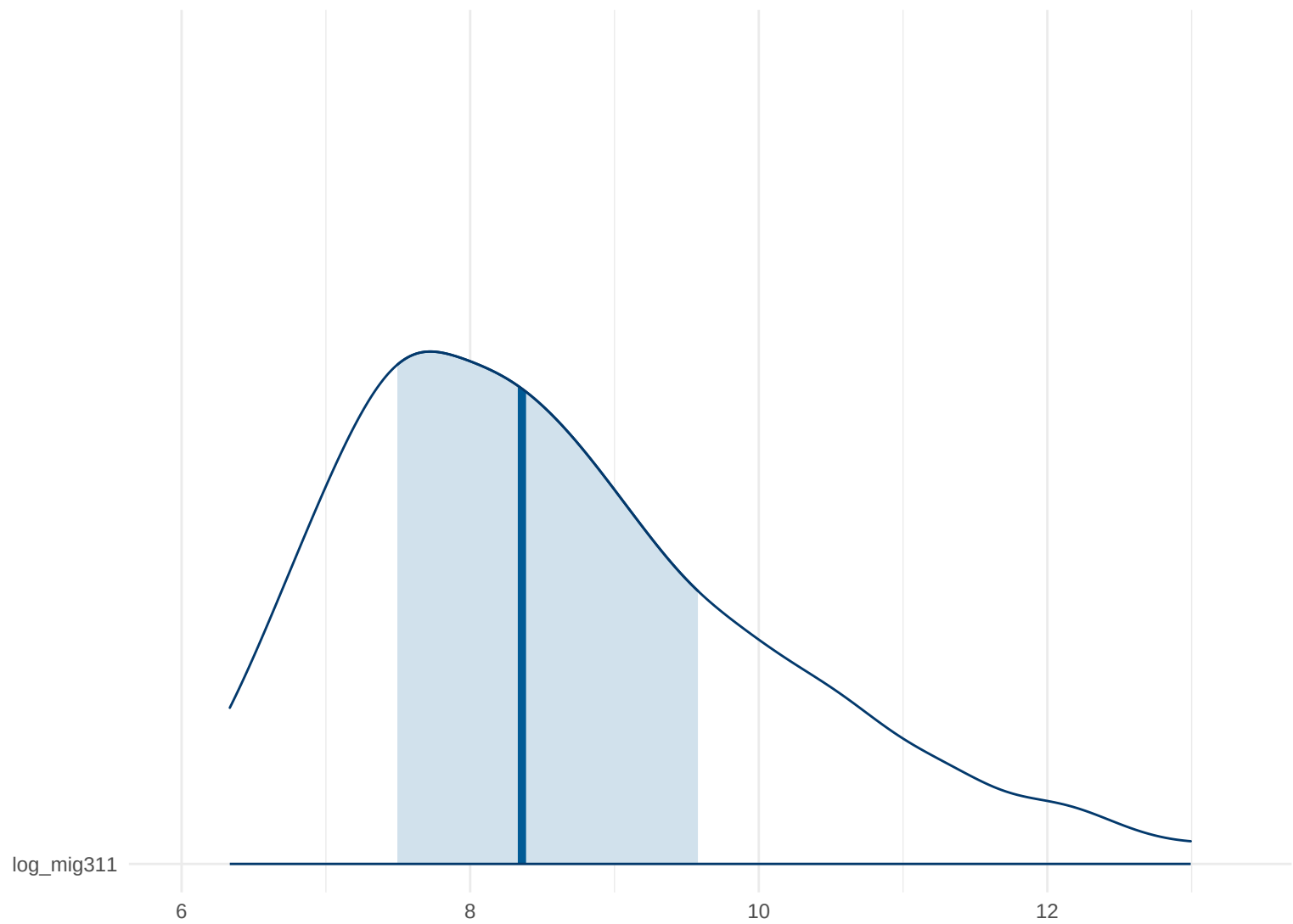
Posterior Density: log_mig311
