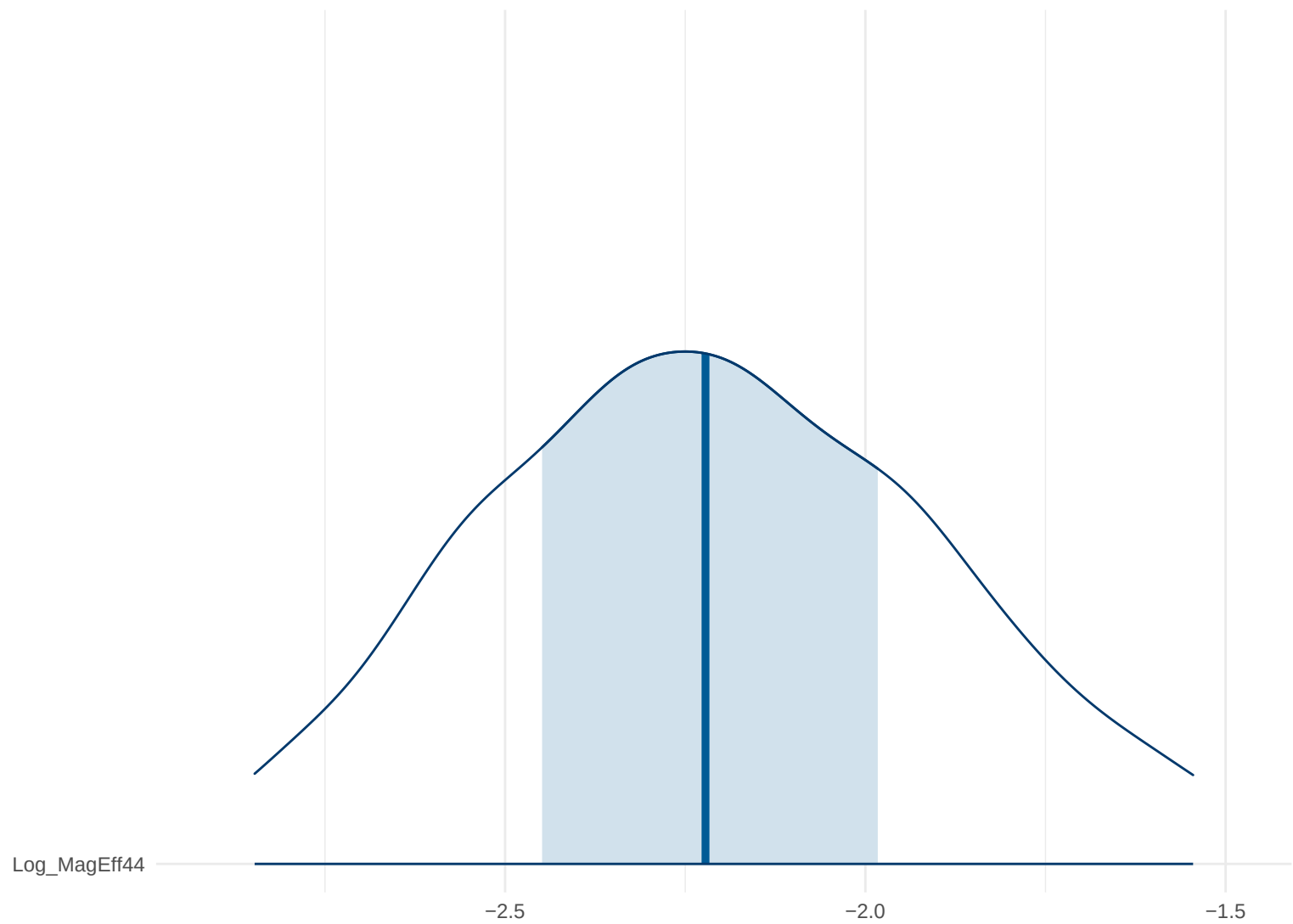
Posterior Density: Log_MagEff44
