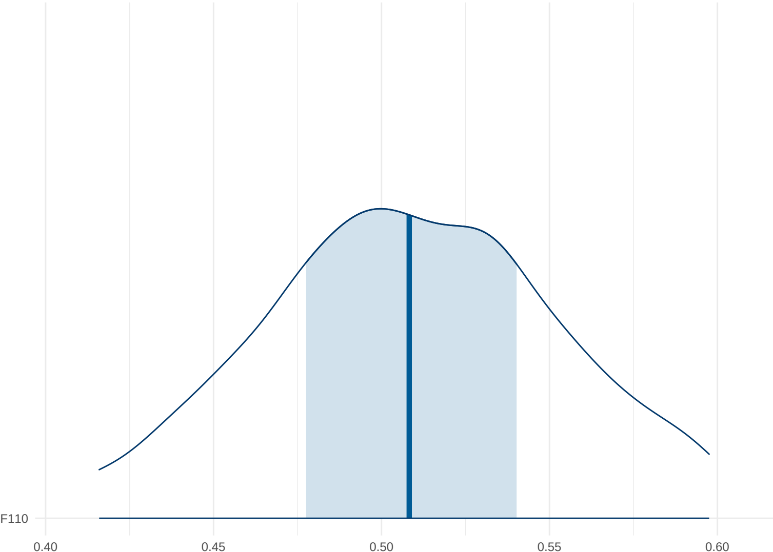
Posterior Density: F110
