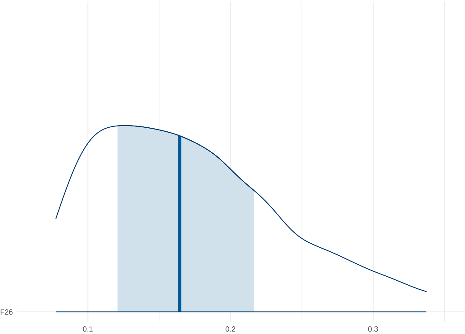
Posterior Density: F26
