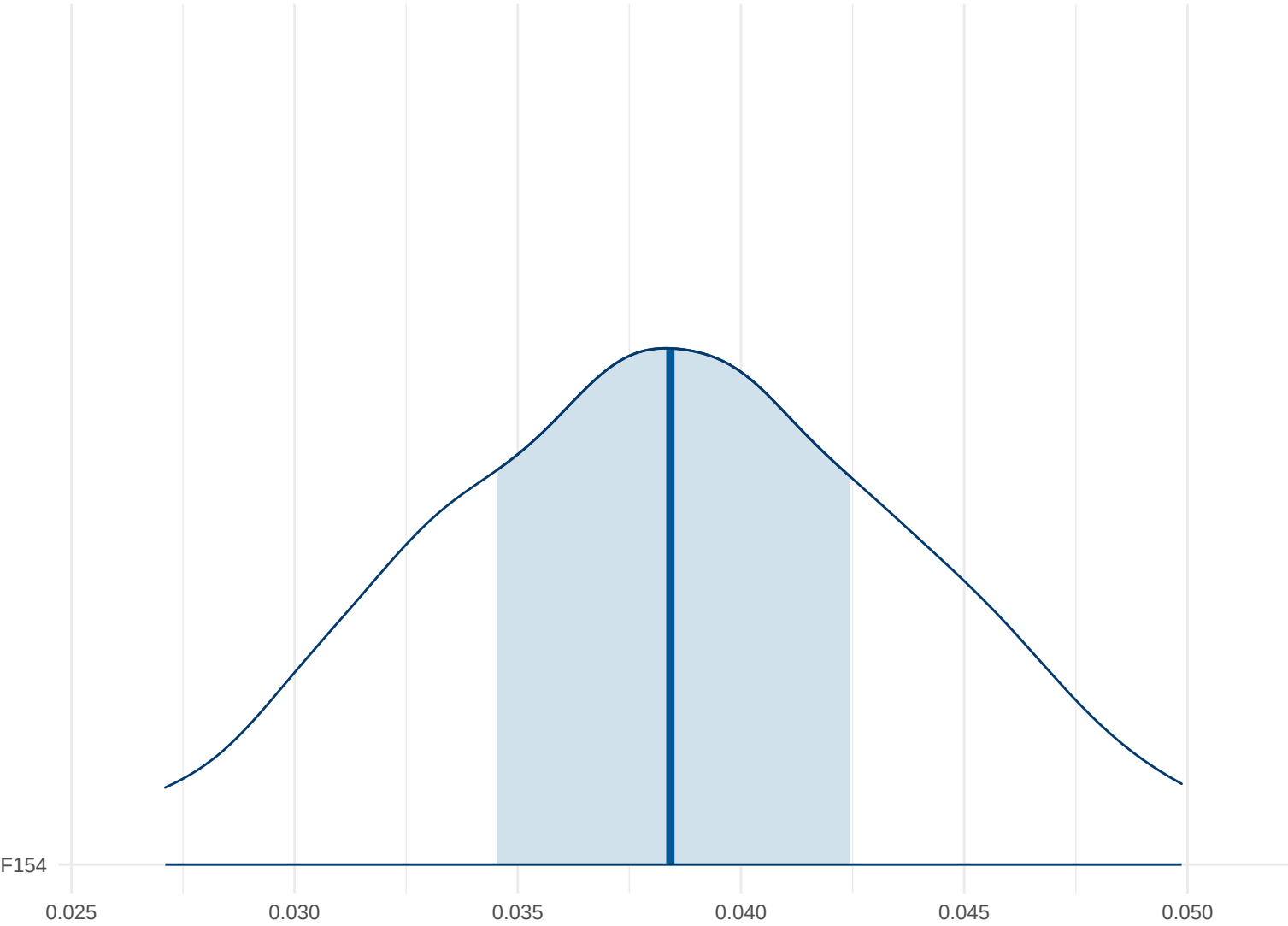
Posterior Density: F154
