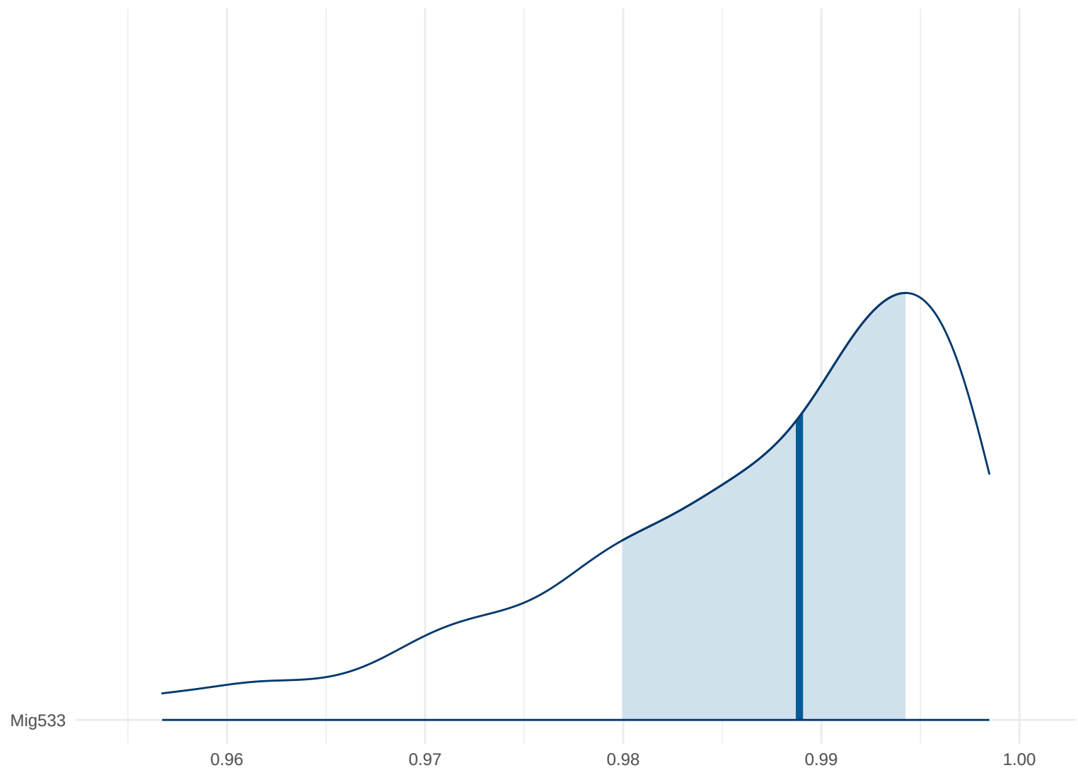
Posterior Density: Mig533
