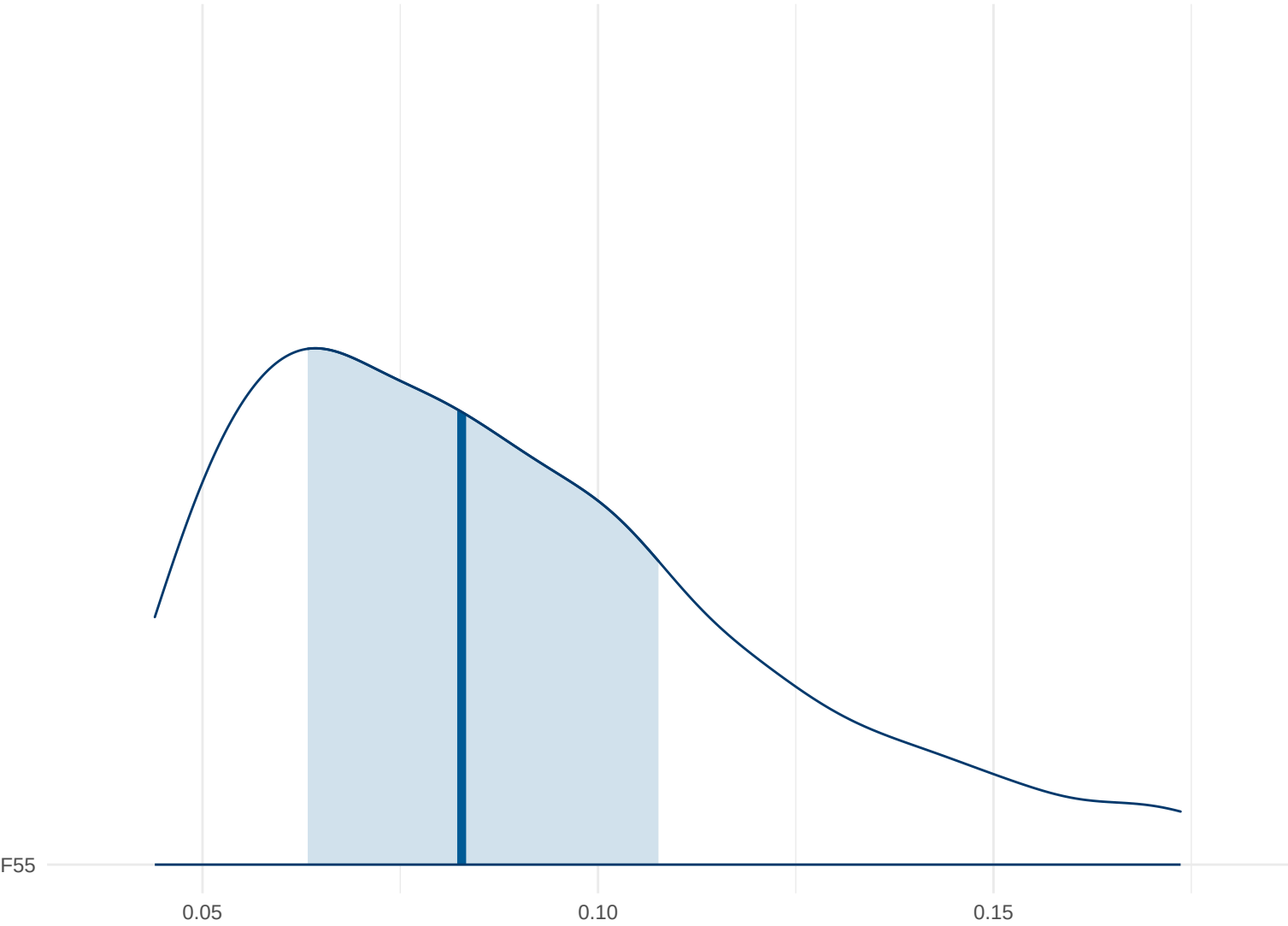
Posterior Density: F55
