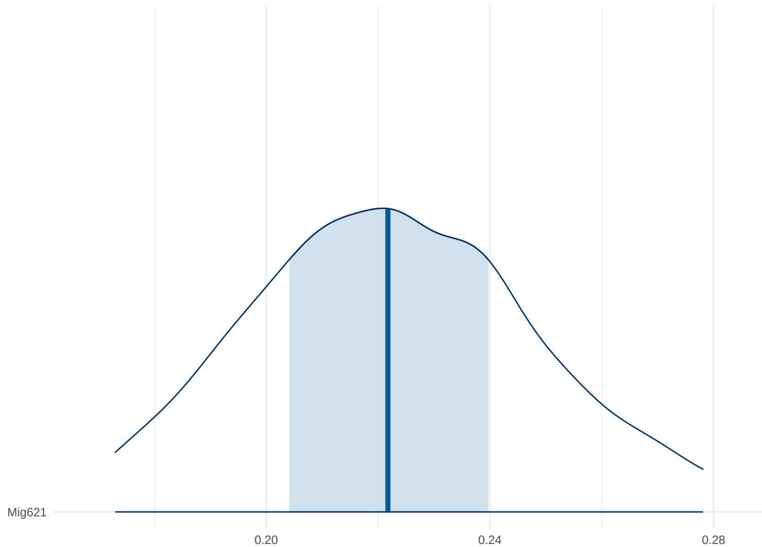
Posterior Density: Mig621
