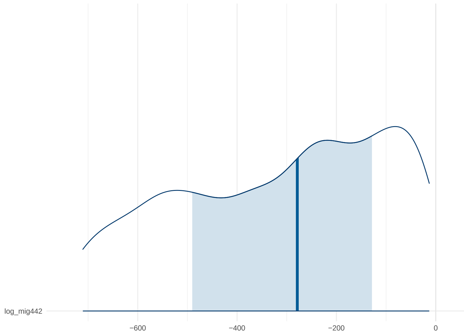
Posterior Density: log_mig442
