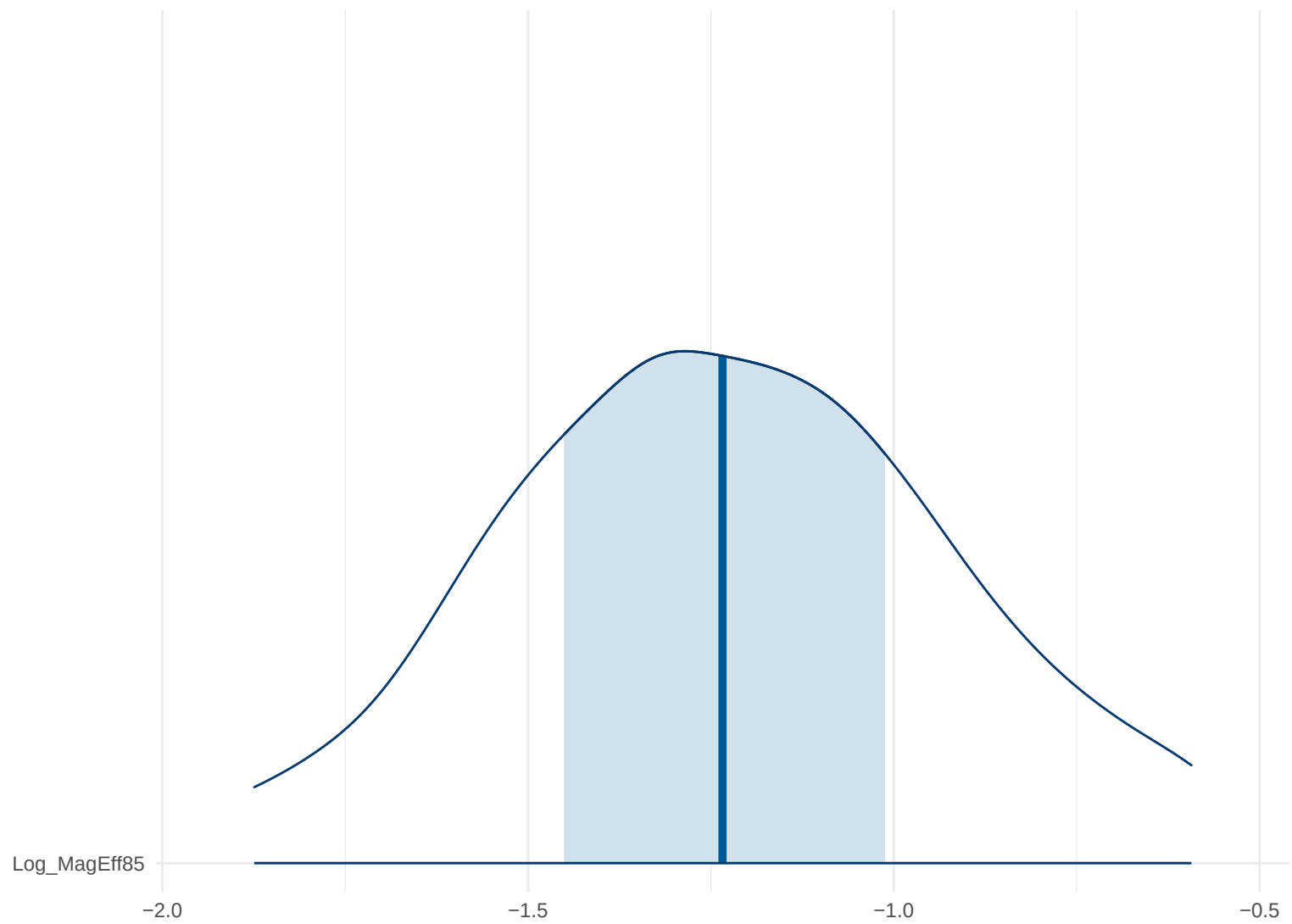
Posterior Density: Log_MagEff85
