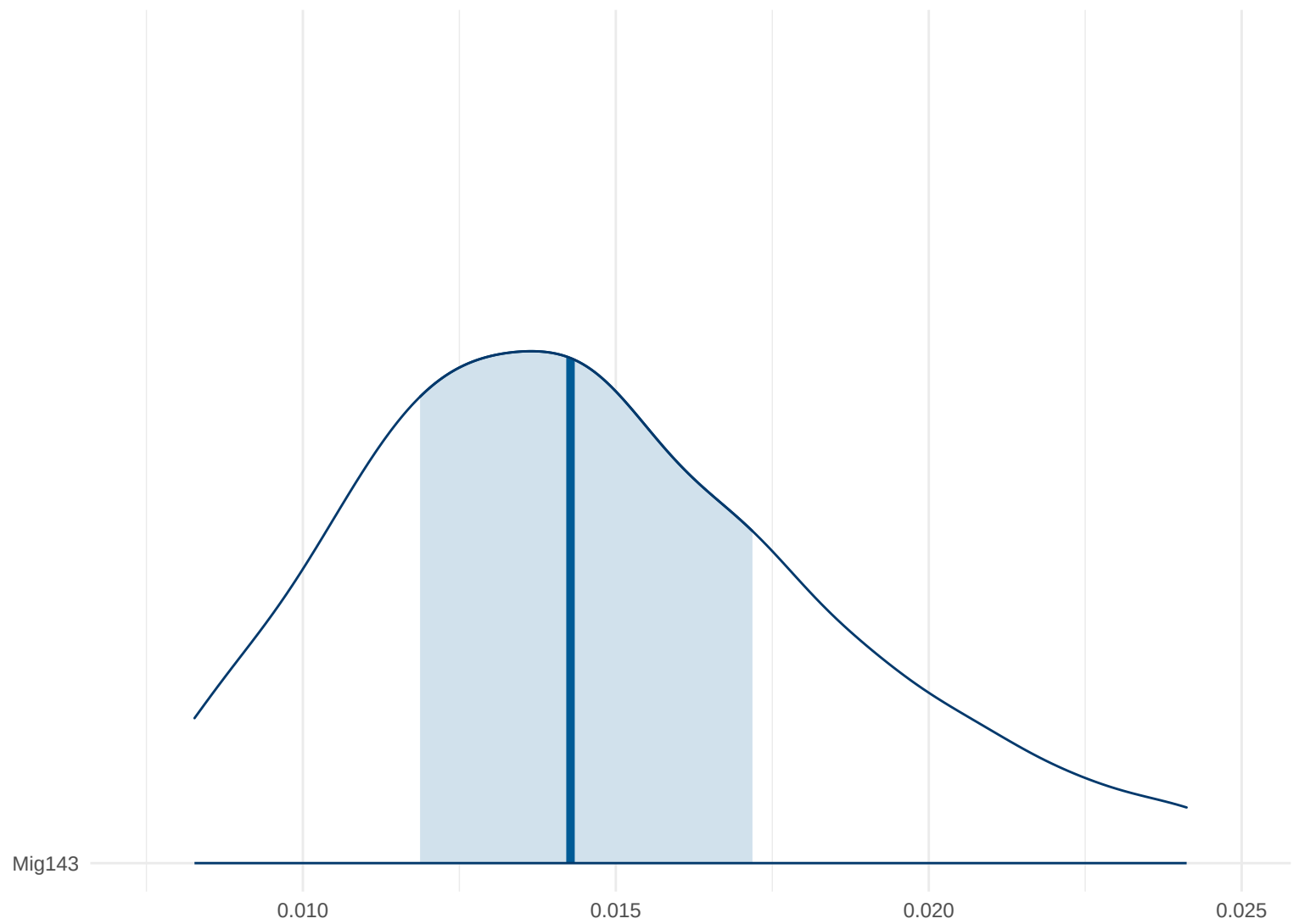
Posterior Density: Mig143
