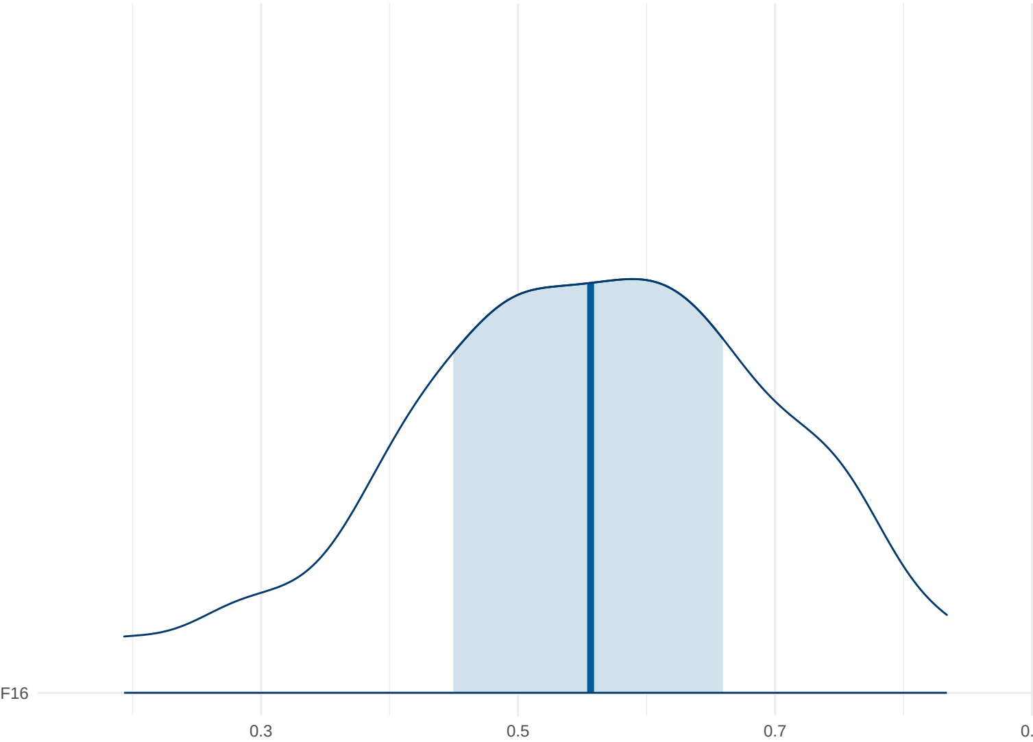
Posterior Density: F16
