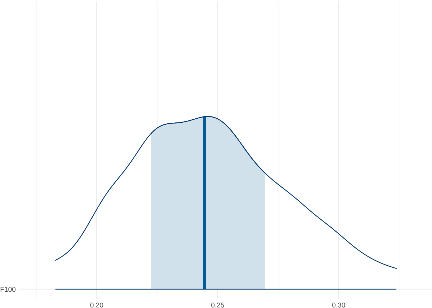
Posterior Density: F100
