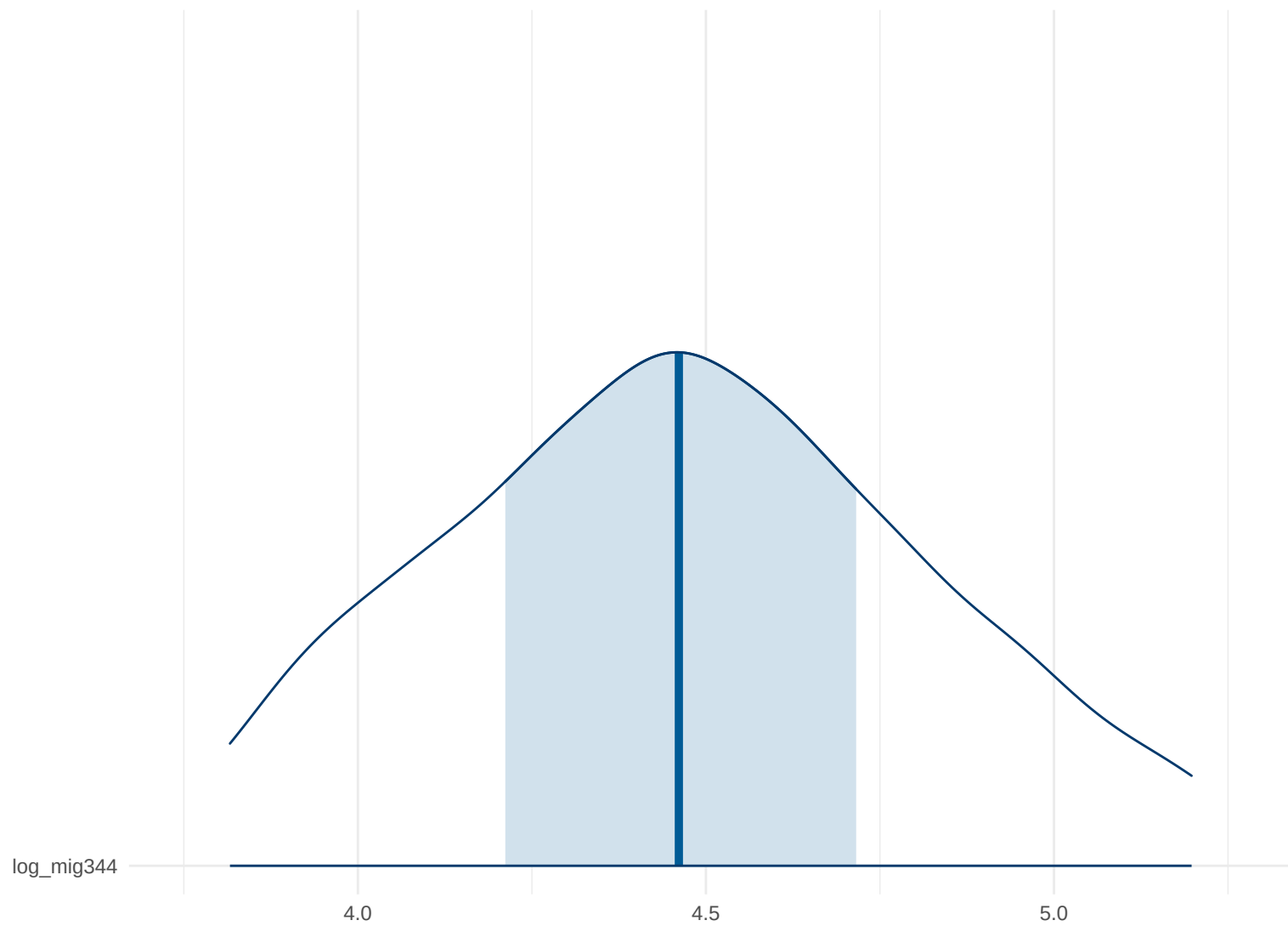
Posterior Density: log_mig344
