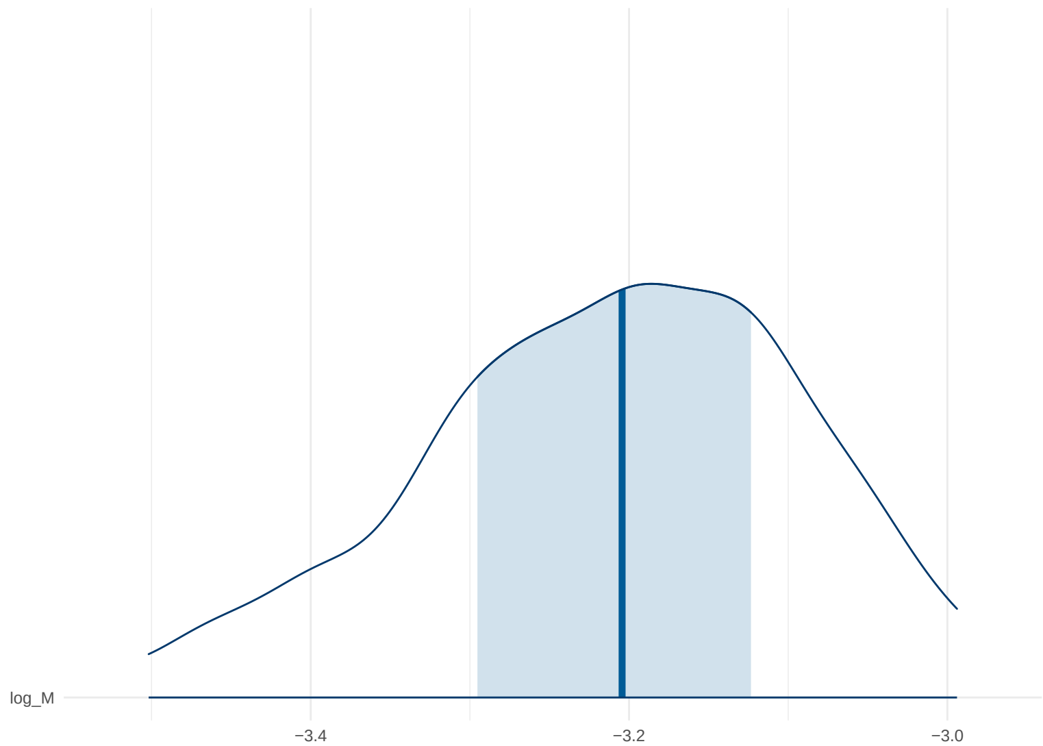
Posterior Density: log_M
