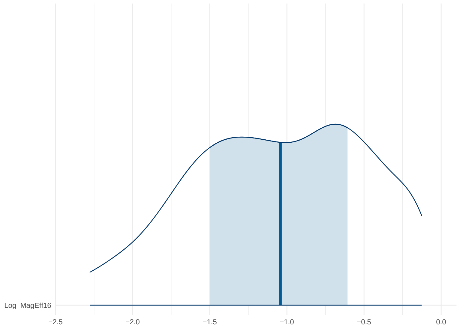
Posterior Density: Log_MagEff16
