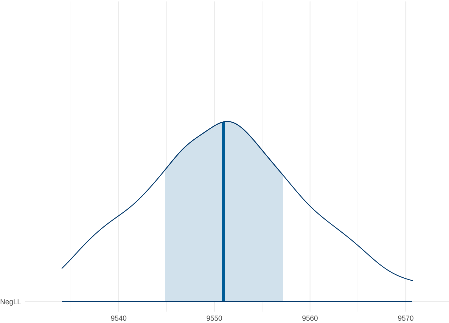
Posterior Density: NegLL
