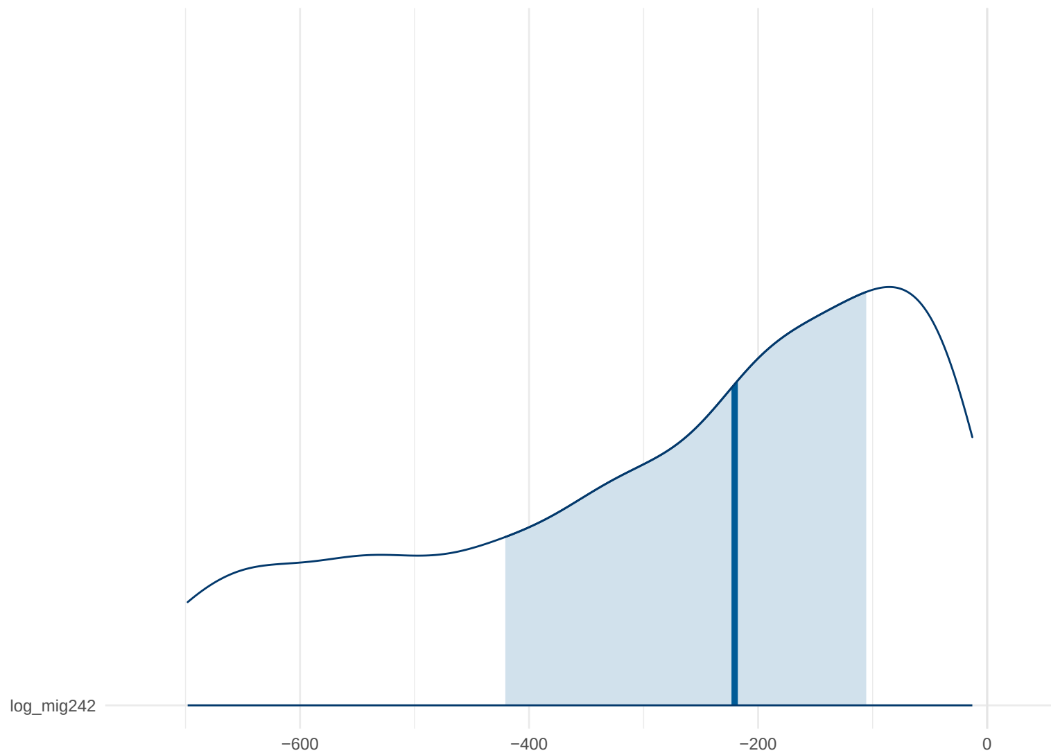
Posterior Density: log_mig242
