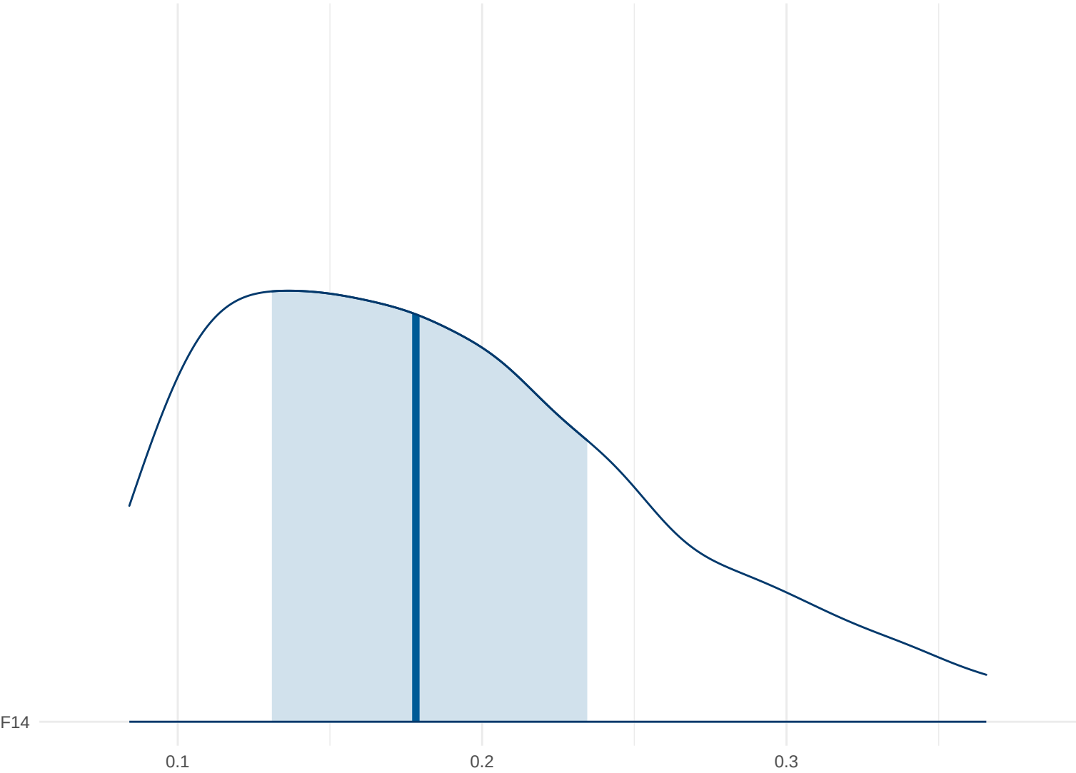
Posterior Density: F14
