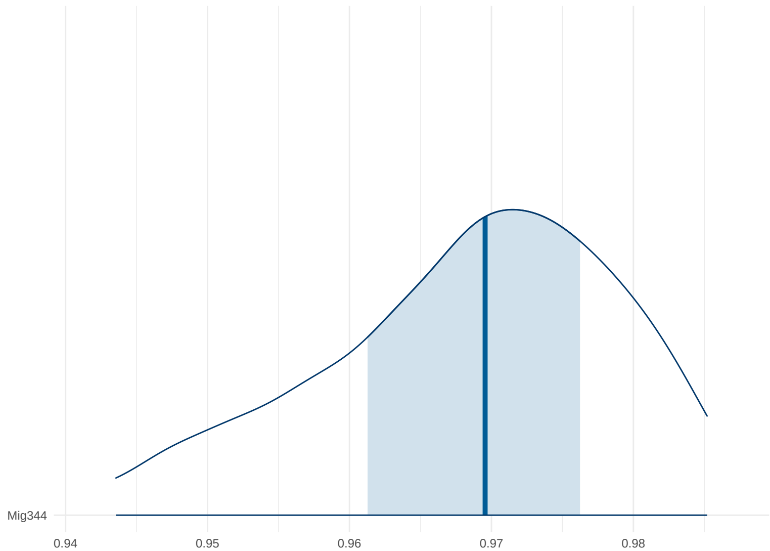
Posterior Density: Mig344
