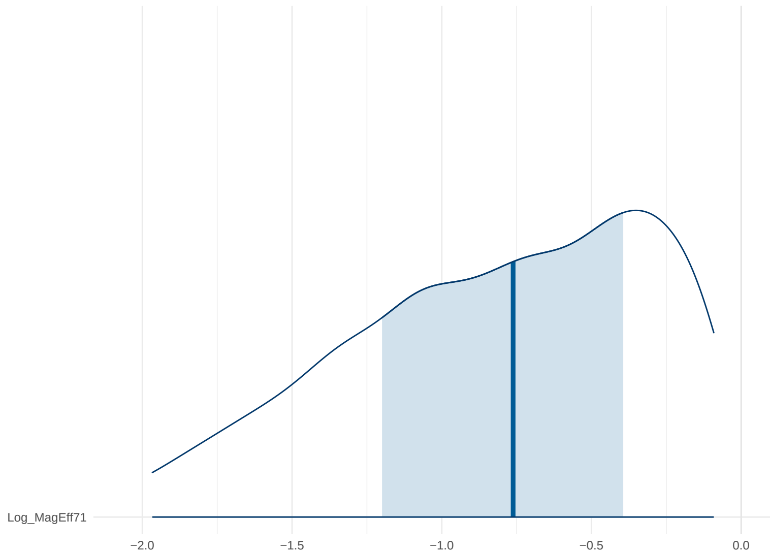
Posterior Density: Log_MagEff71
