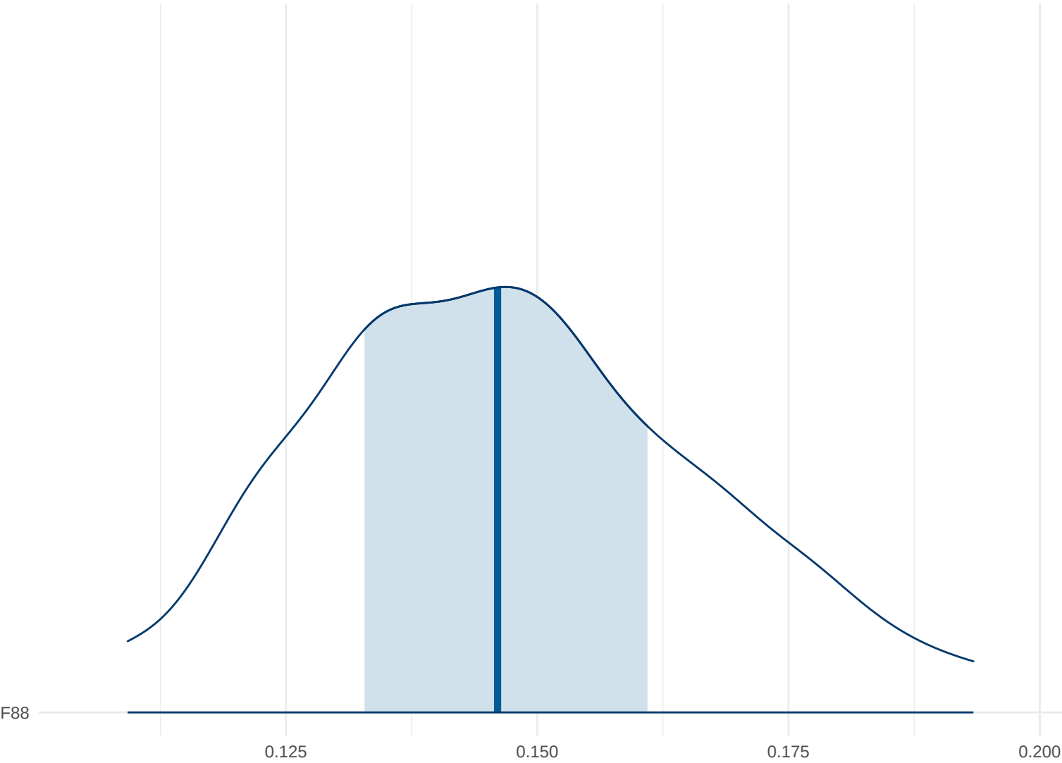
Posterior Density: F88
