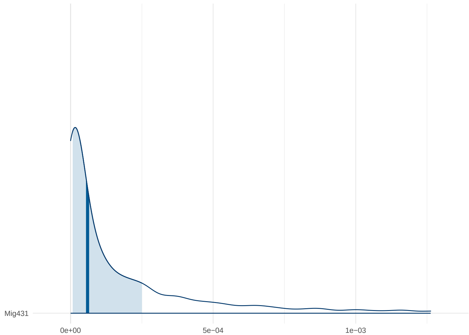
Posterior Density: Mig431
