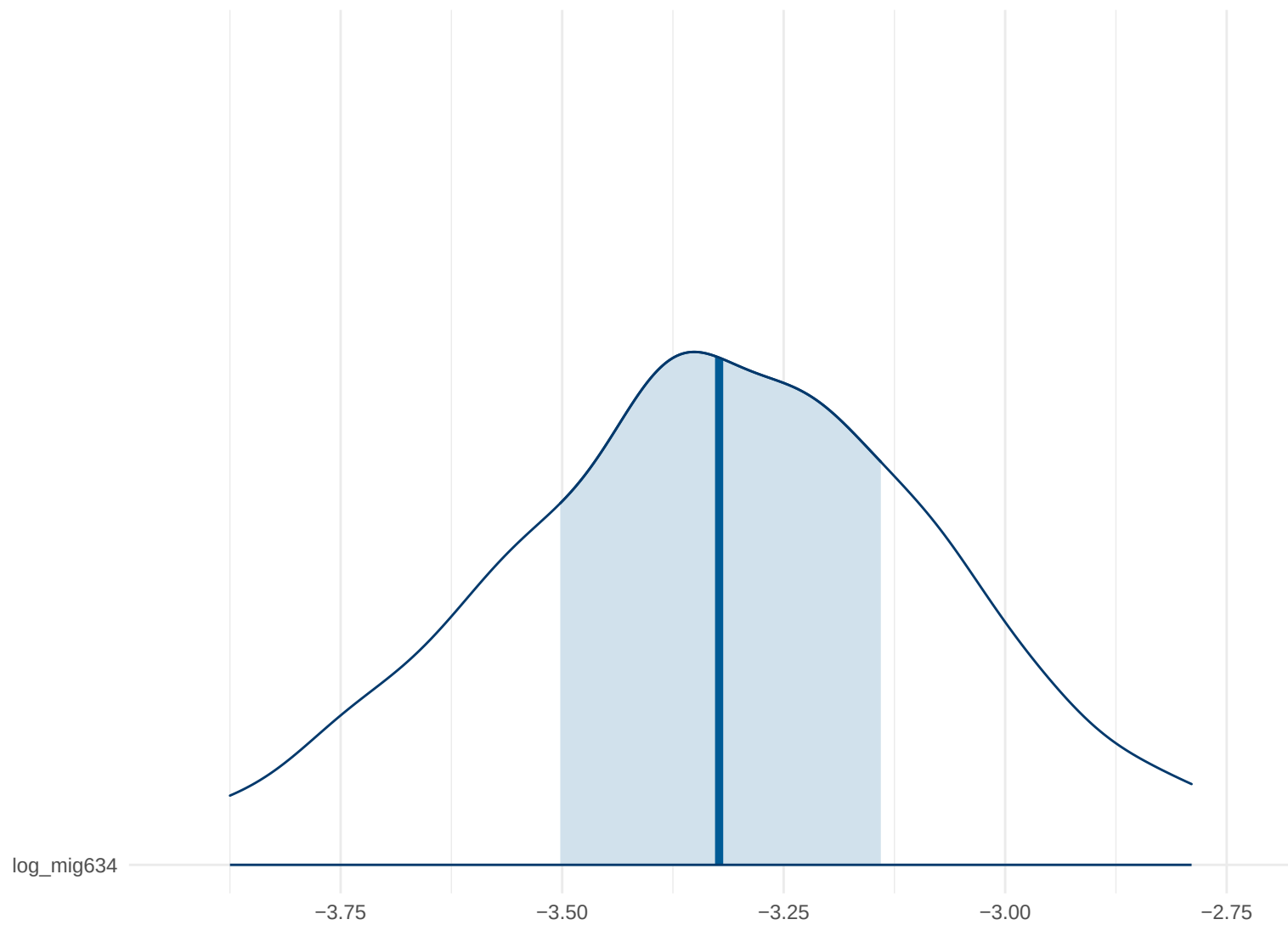
Posterior Density: log_mig634
