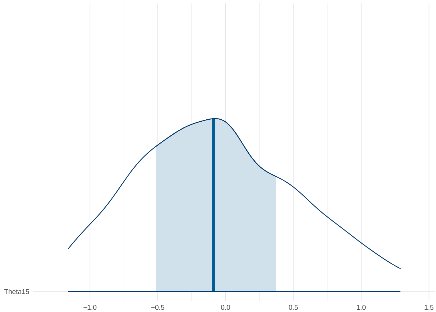
Posterior Density: Theta15
