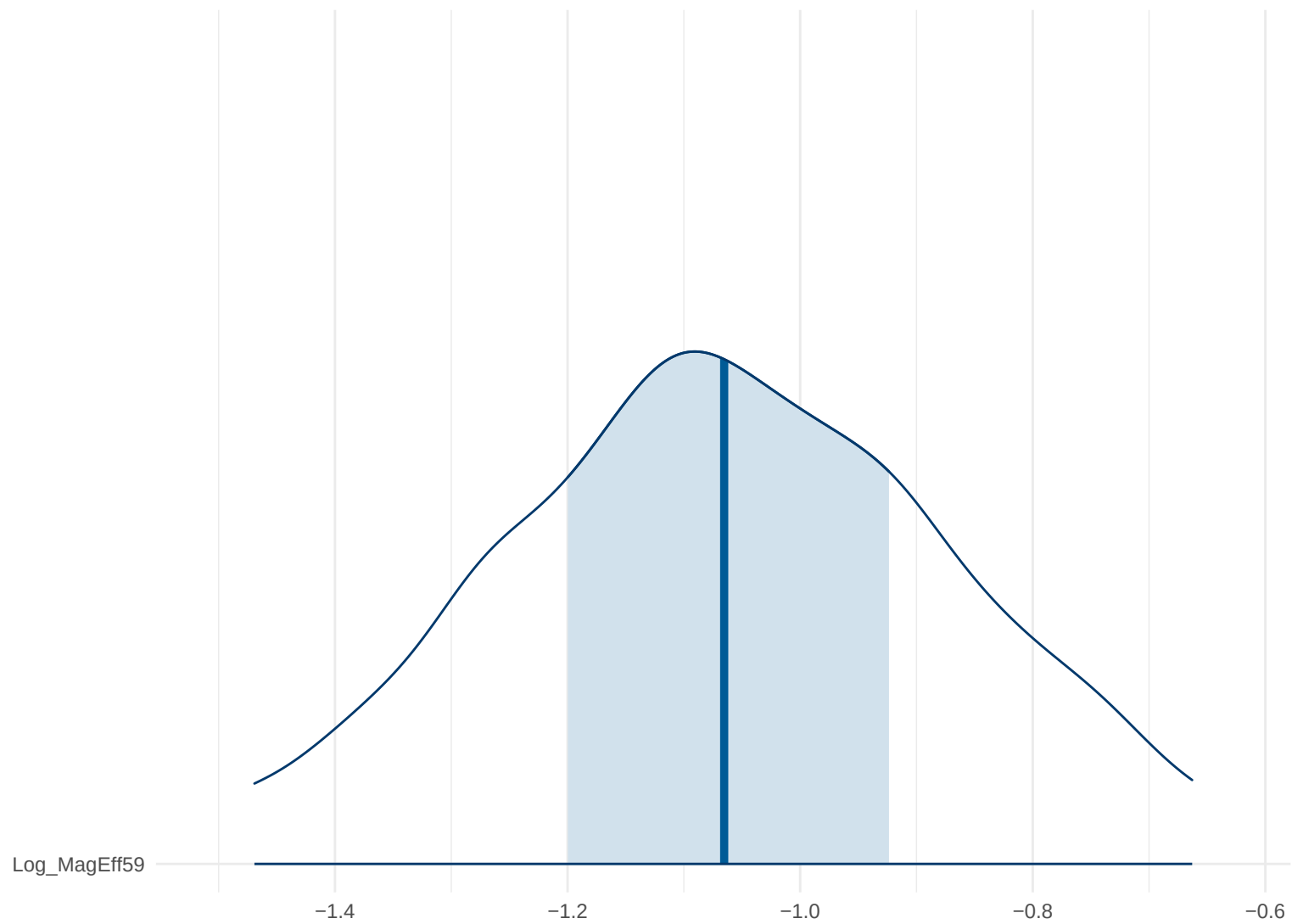
Posterior Density: Log_MagEff59
