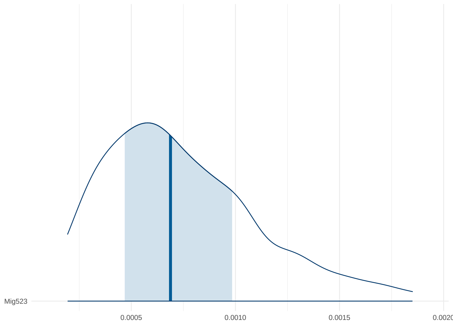
Posterior Density: Mig523
