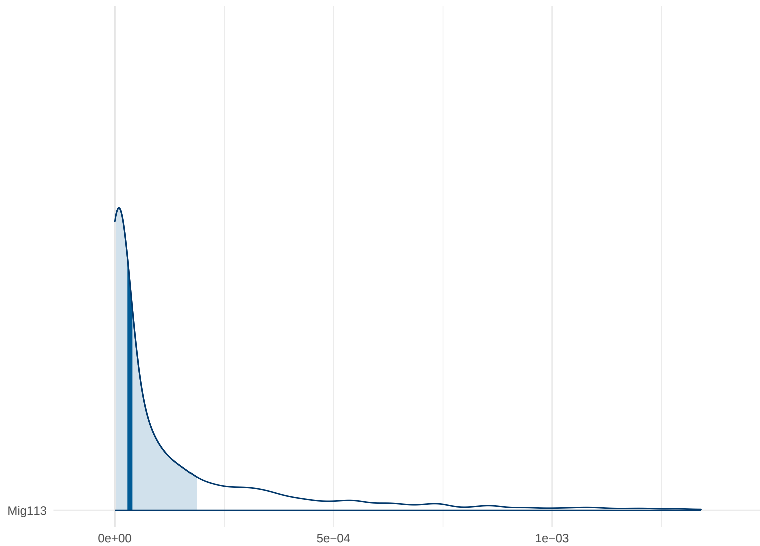
Posterior Density: Mig113
