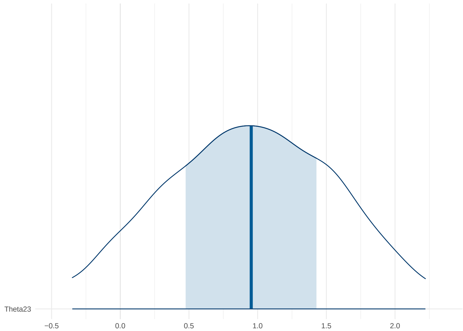
Posterior Density: Theta23
