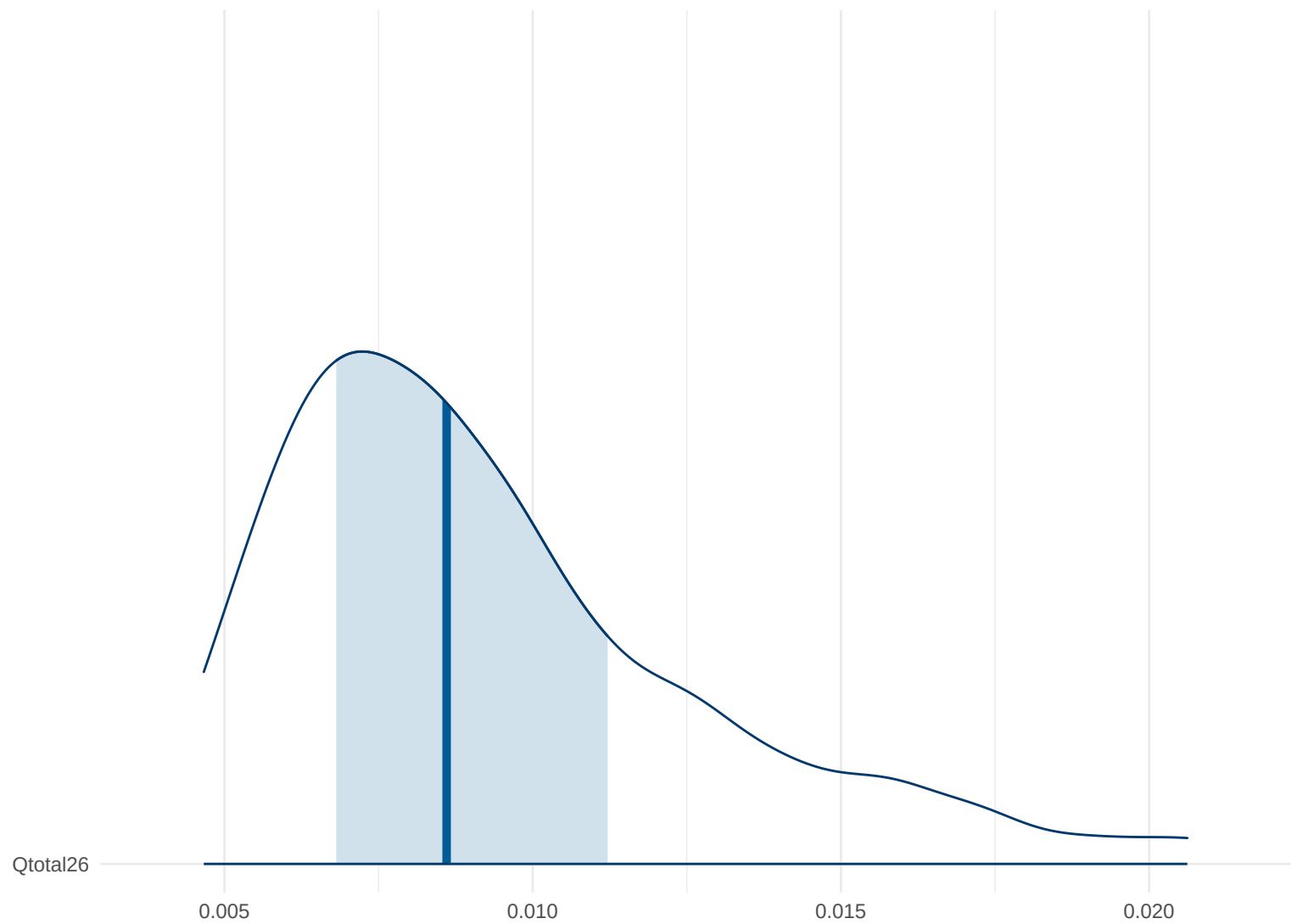
Posterior Density: Qtotal26
