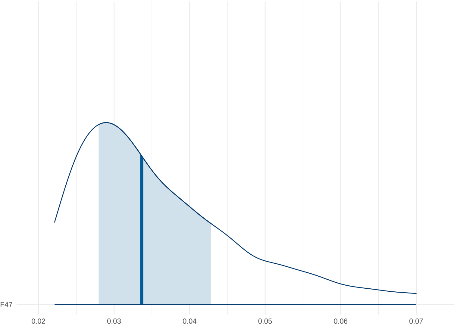
Posterior Density: F47
