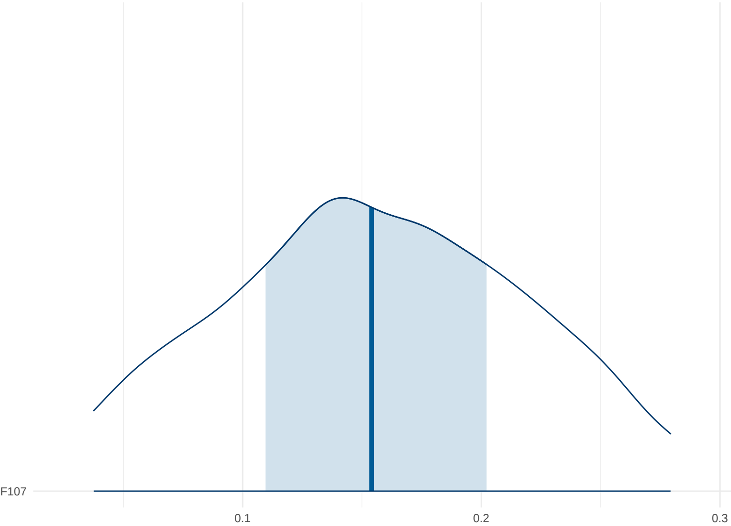
Posterior Density: F107
