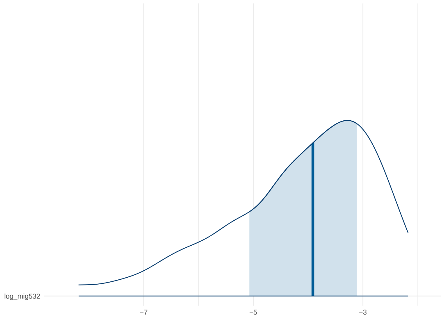
Posterior Density: log_mig532
