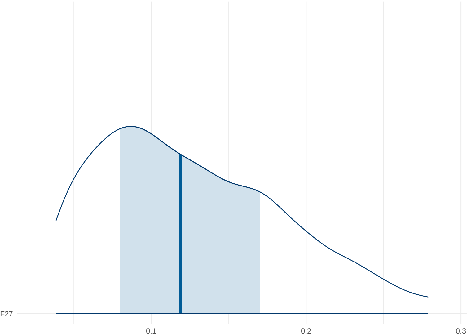
Posterior Density: F27
