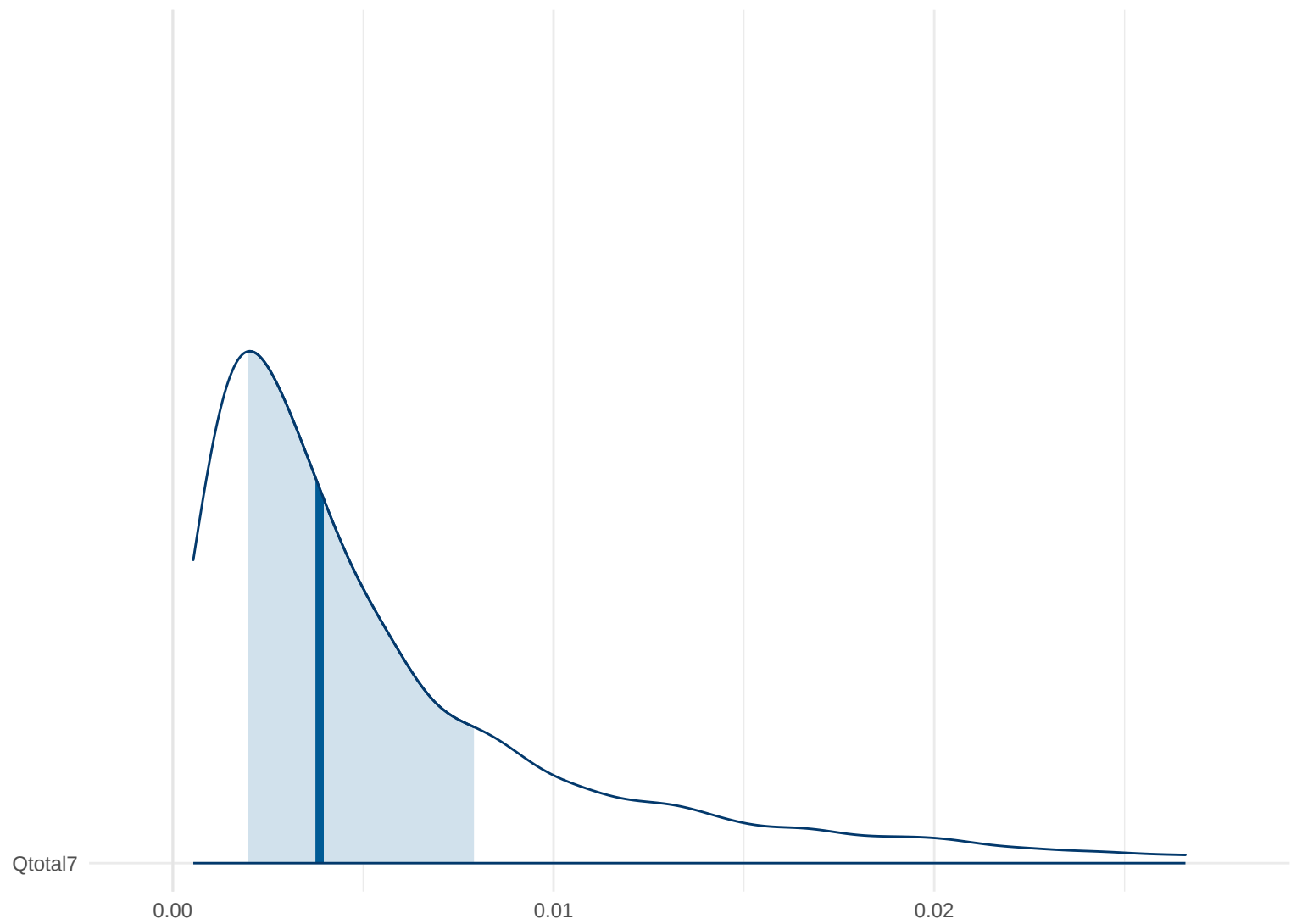
Posterior Density: Qtotal7
