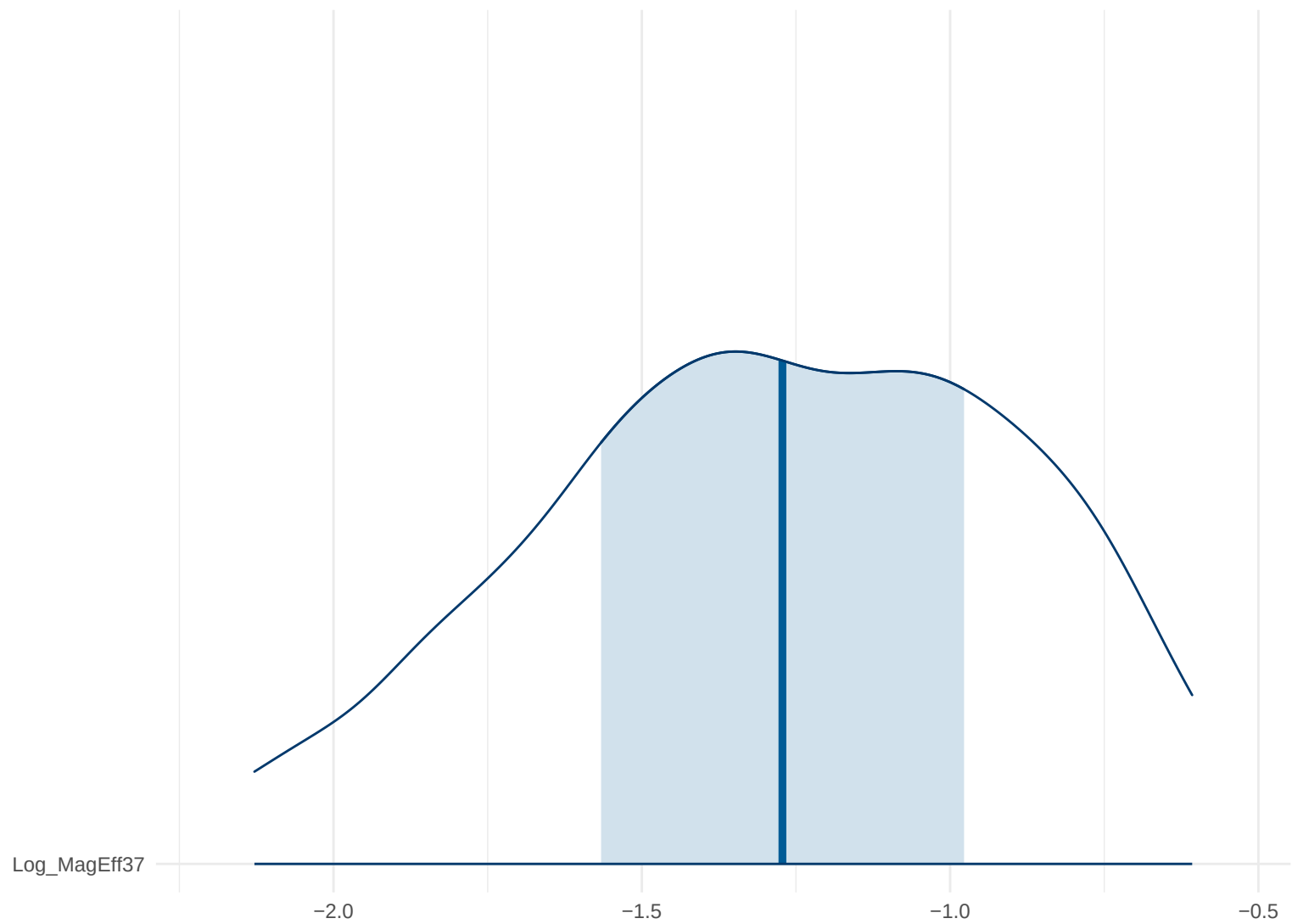
Posterior Density: Log_MagEff37
