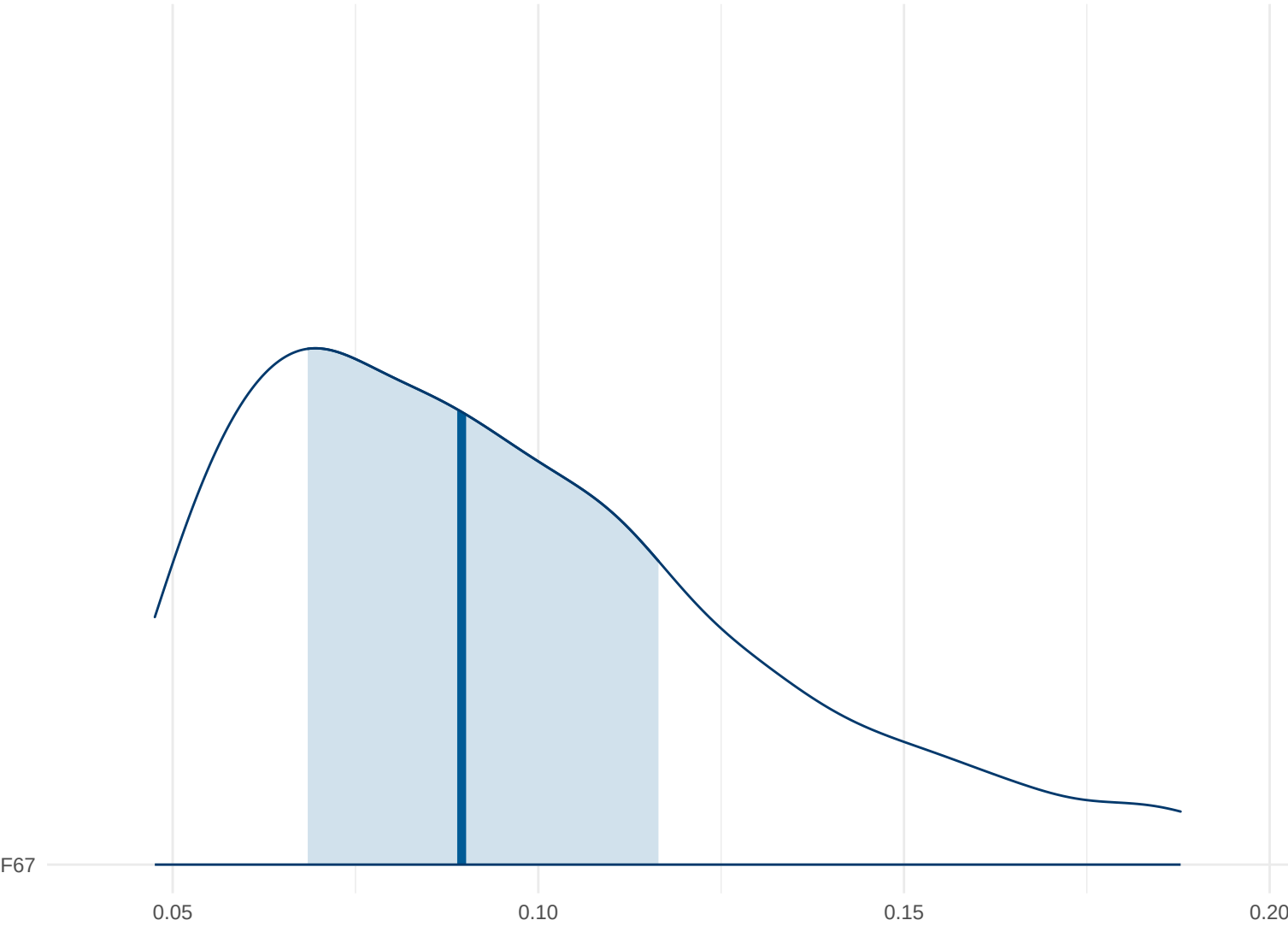
Posterior Density: F67
