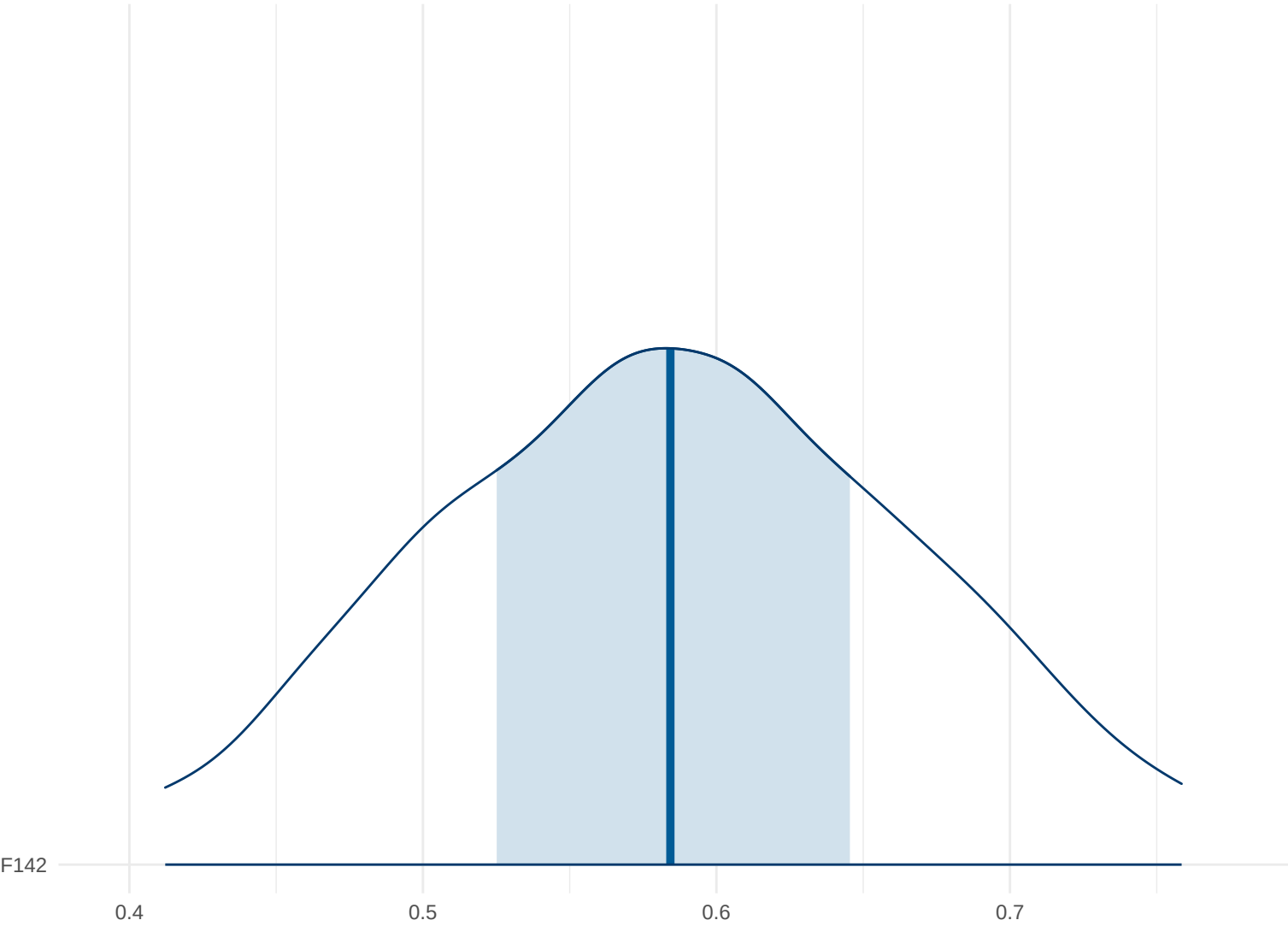
Posterior Density: F142
