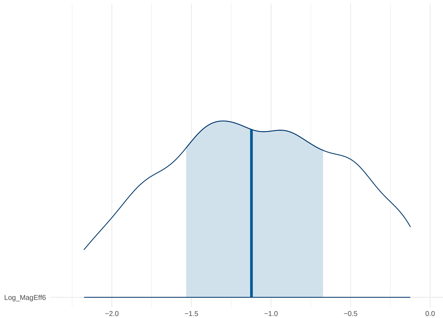
Posterior Density: Log_MagEff6
