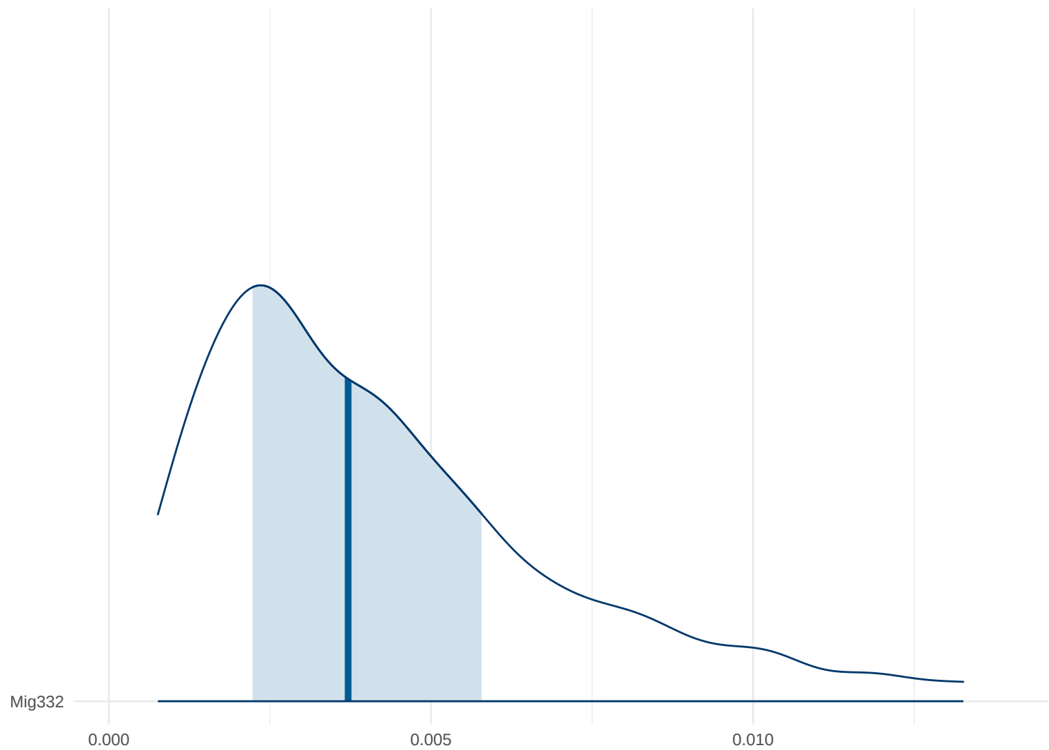
Posterior Density: Mig332
