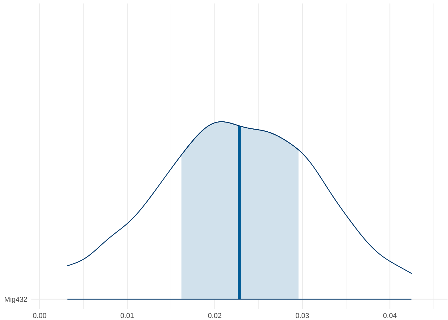
Posterior Density: Mig432
