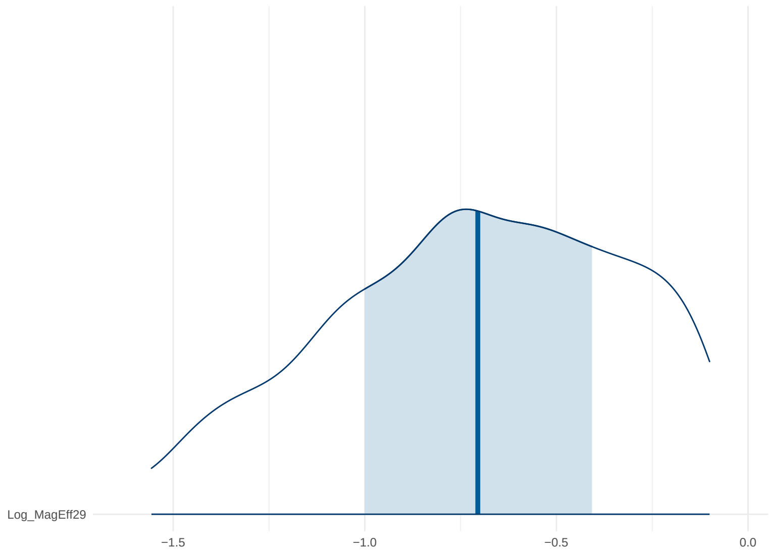
Posterior Density: Log_MagEff29
