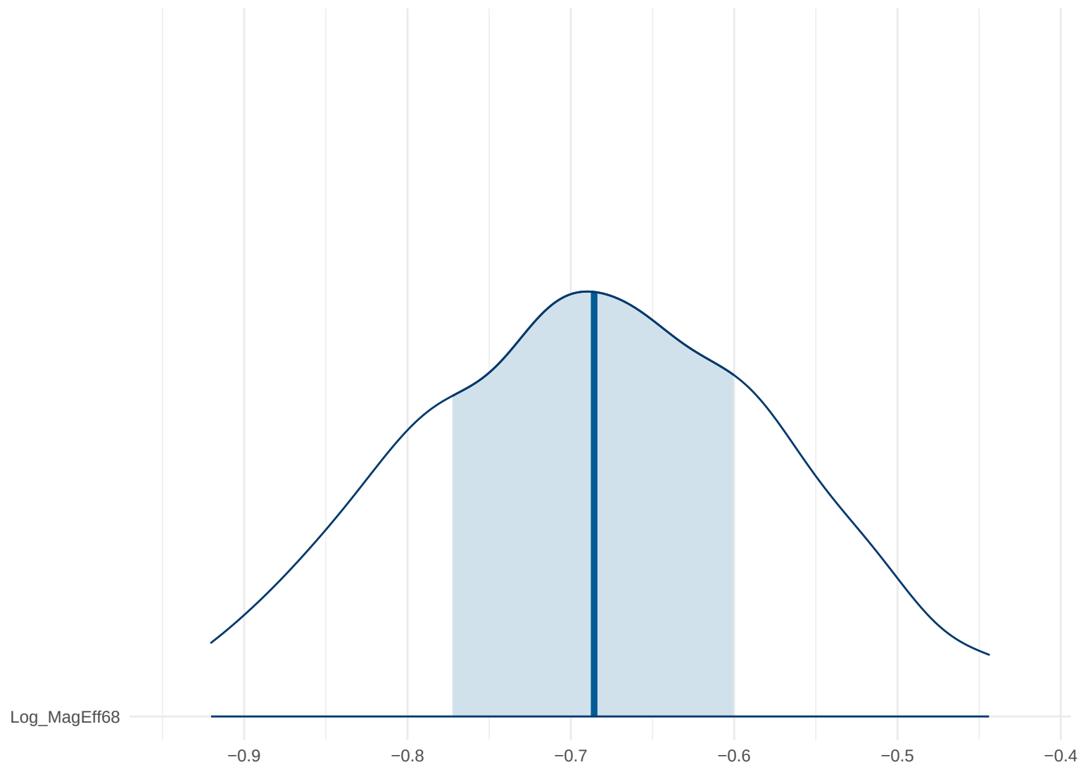
Posterior Density: Log_MagEff68
