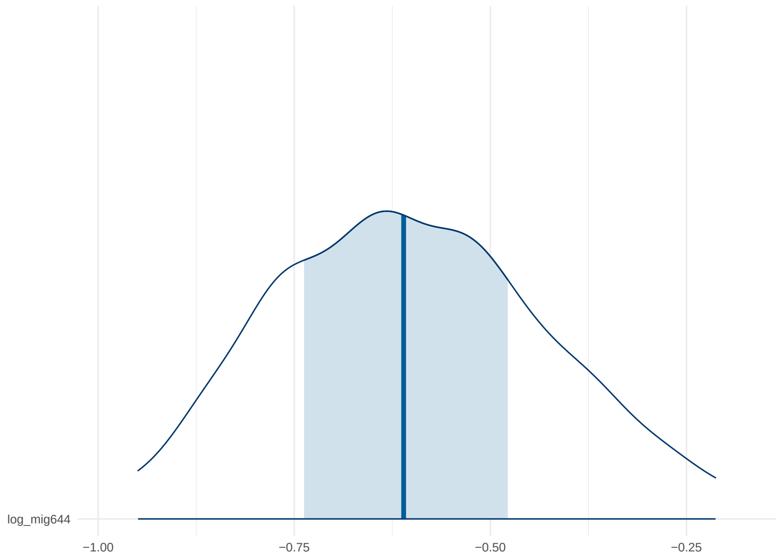
Posterior Density: log_mig644
