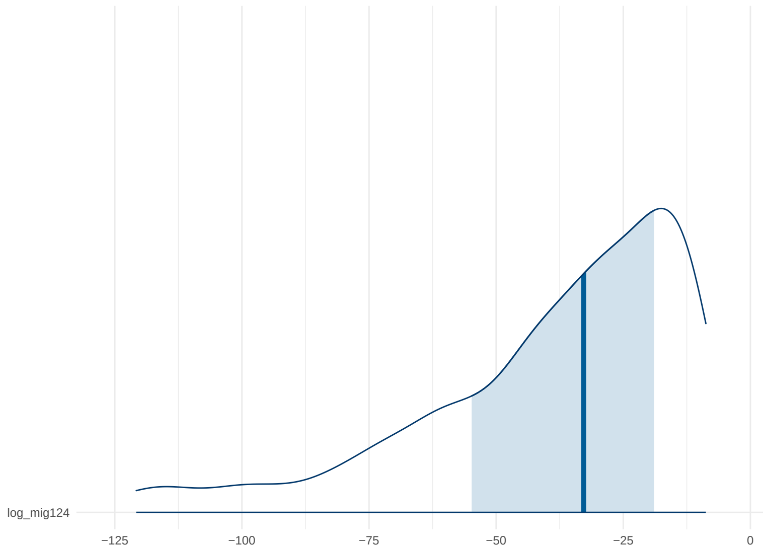
Posterior Density: log_mig124
