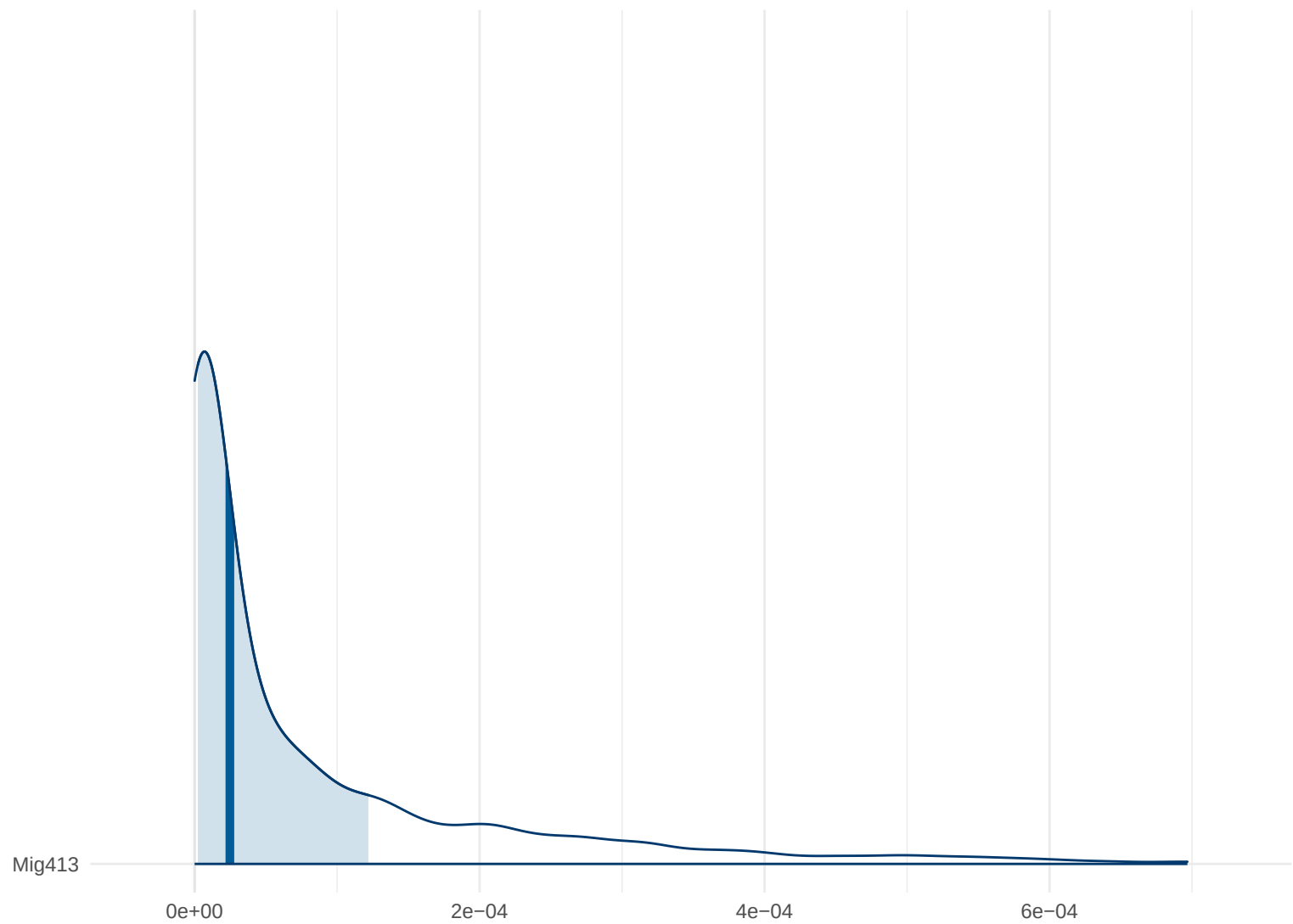
Posterior Density: Mig413
