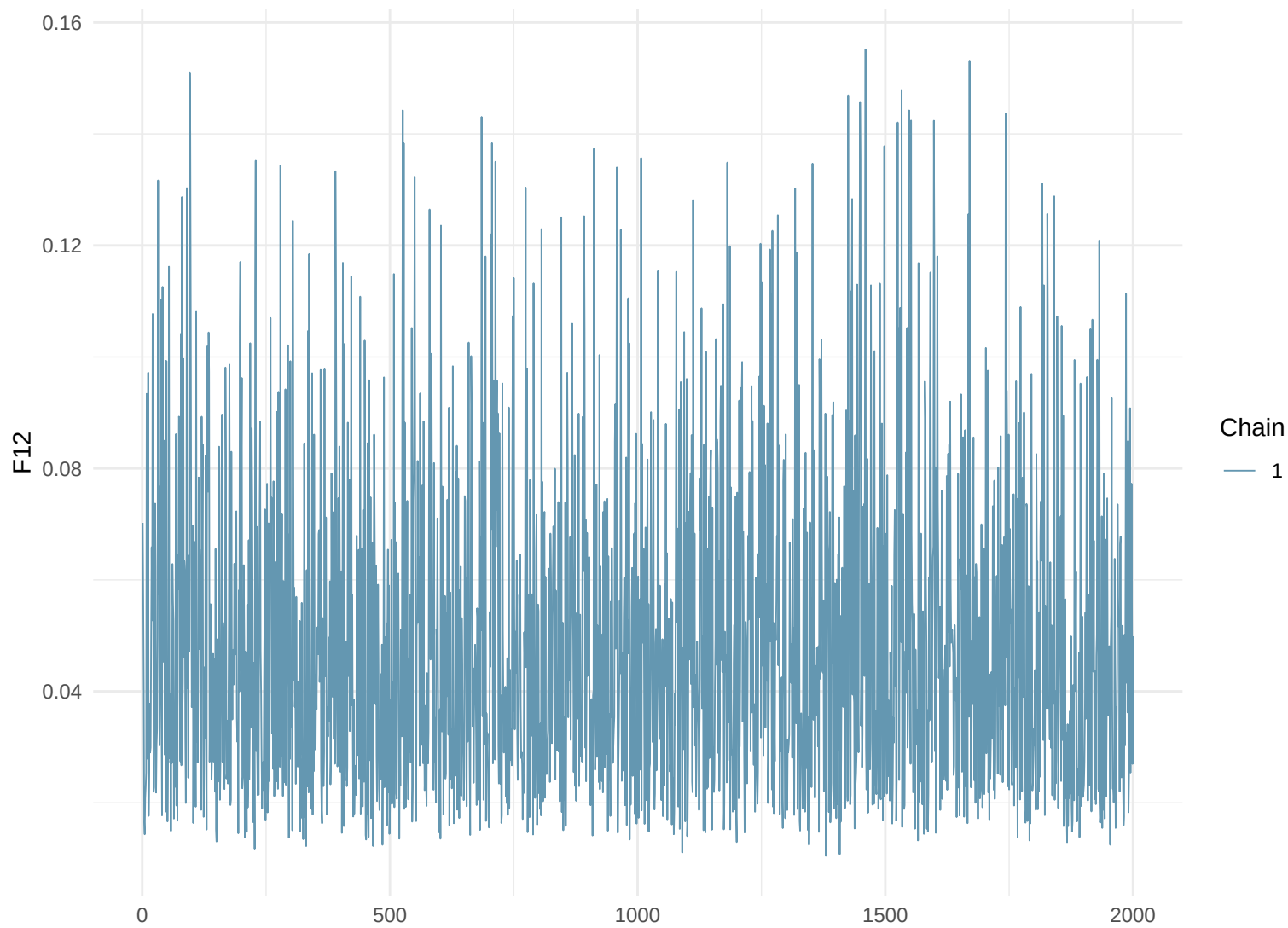
Trace Plot: F12
