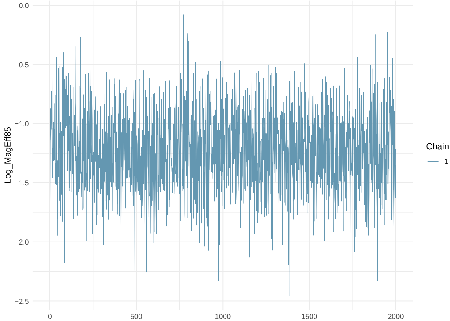
Trace Plot: Log_MagEff85
