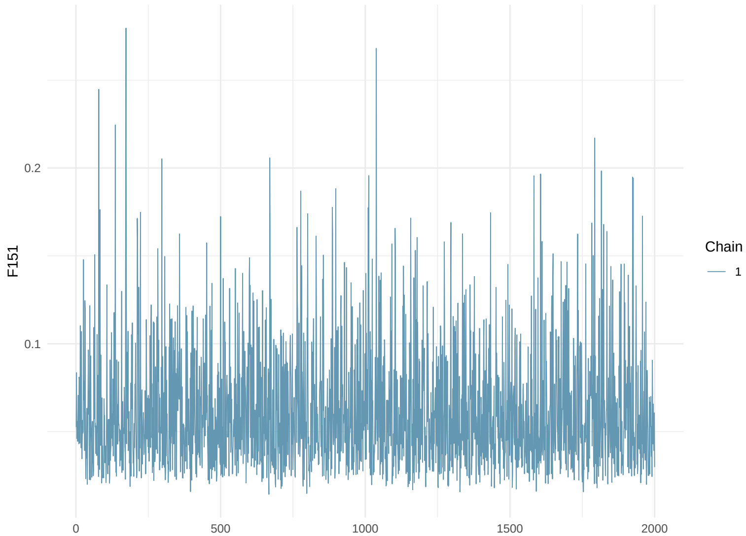
Trace Plot: F151
