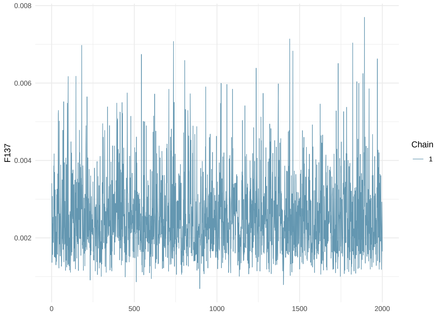
Trace Plot: F137
