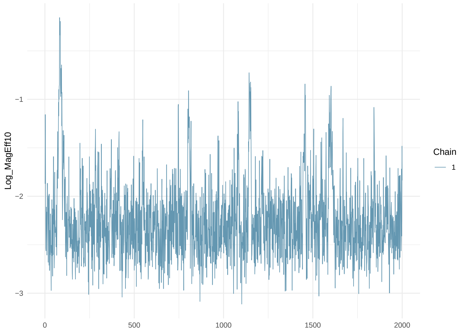
Trace Plot: Log_MagEff10
