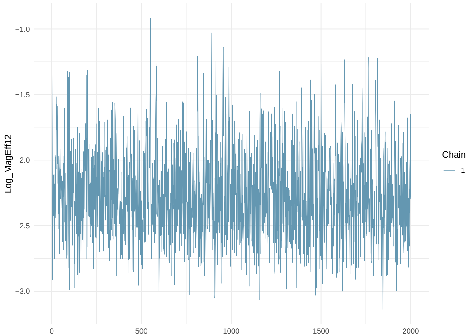
Trace Plot: Log_MagEff12
