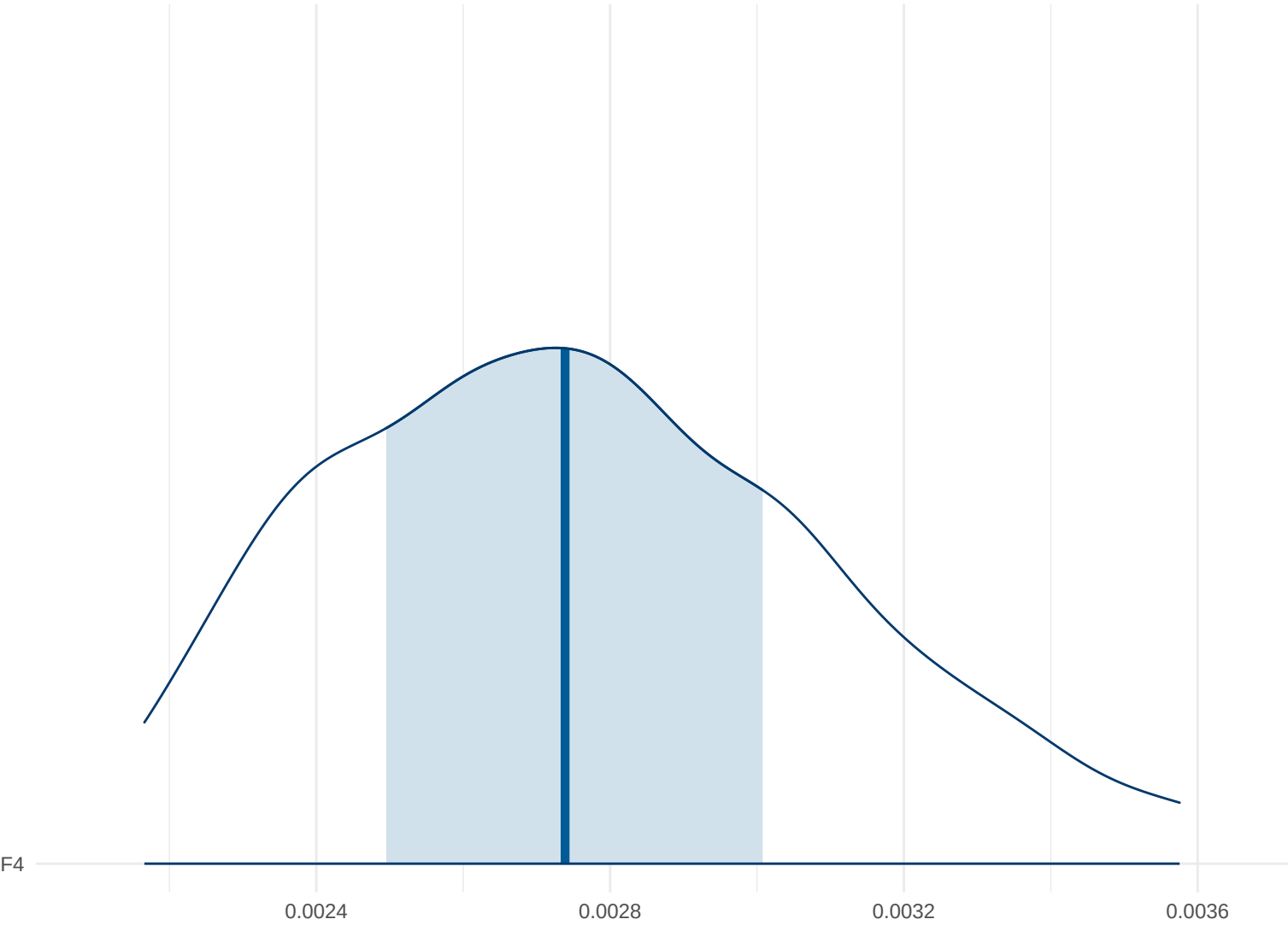
Posterior Density: F4
