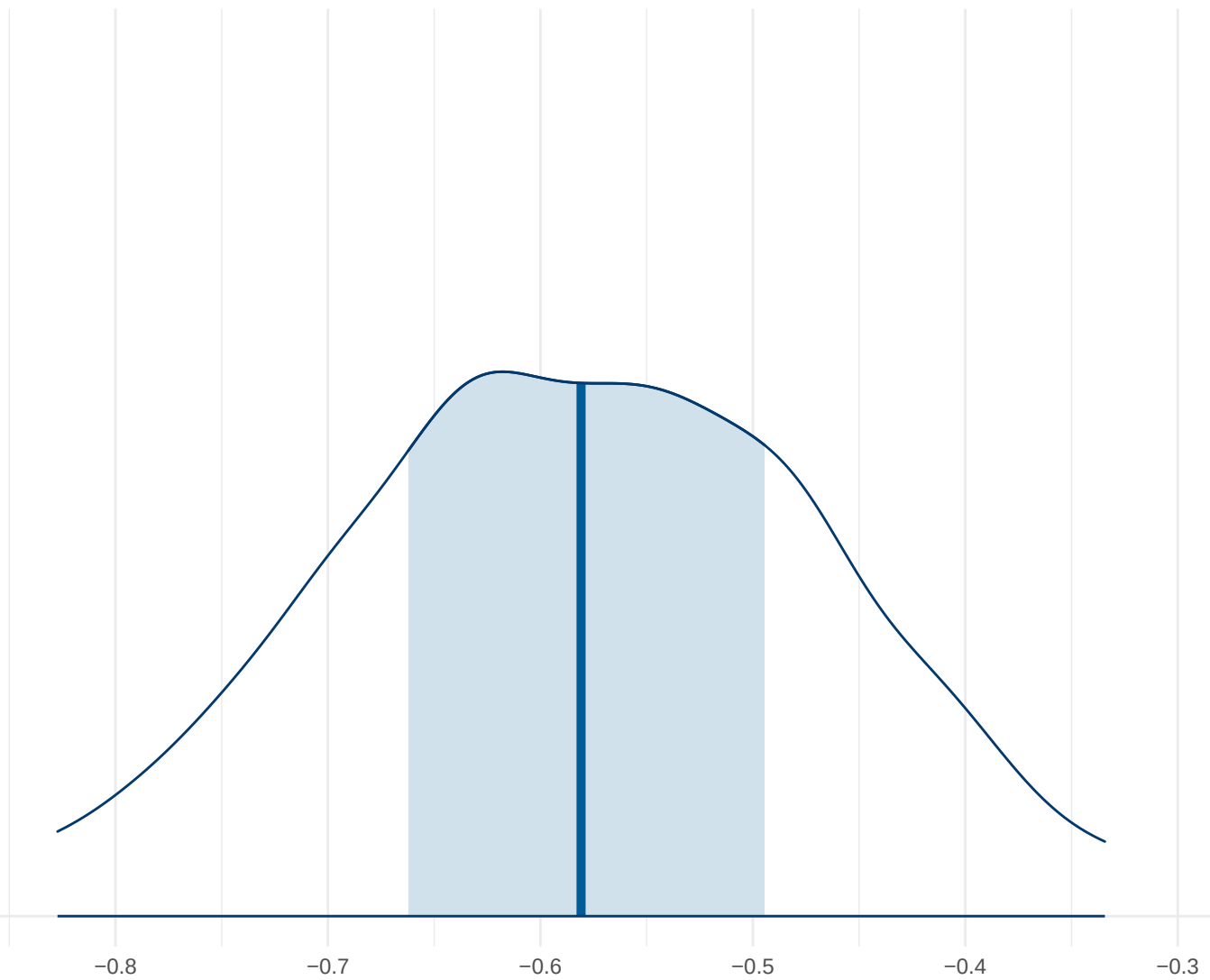
Posterior Density: Theta17
