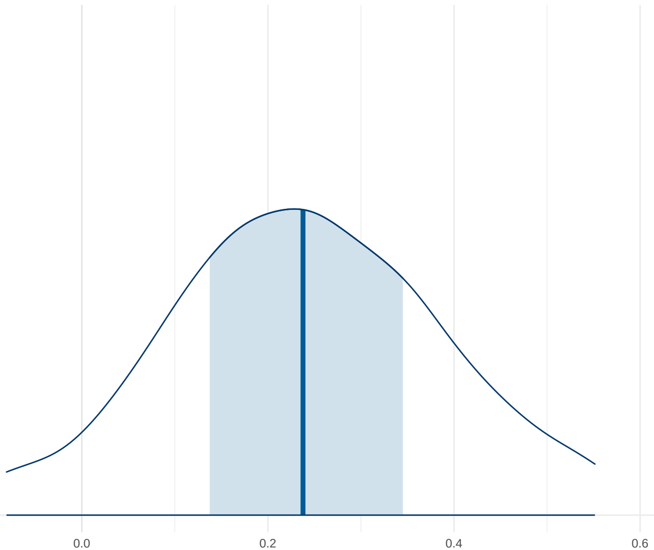
Posterior Density: Theta26
