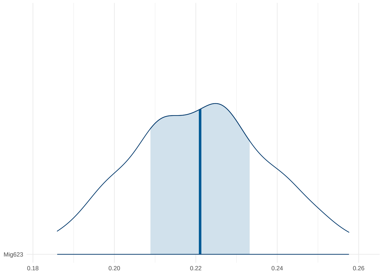
Posterior Density: Mig623
