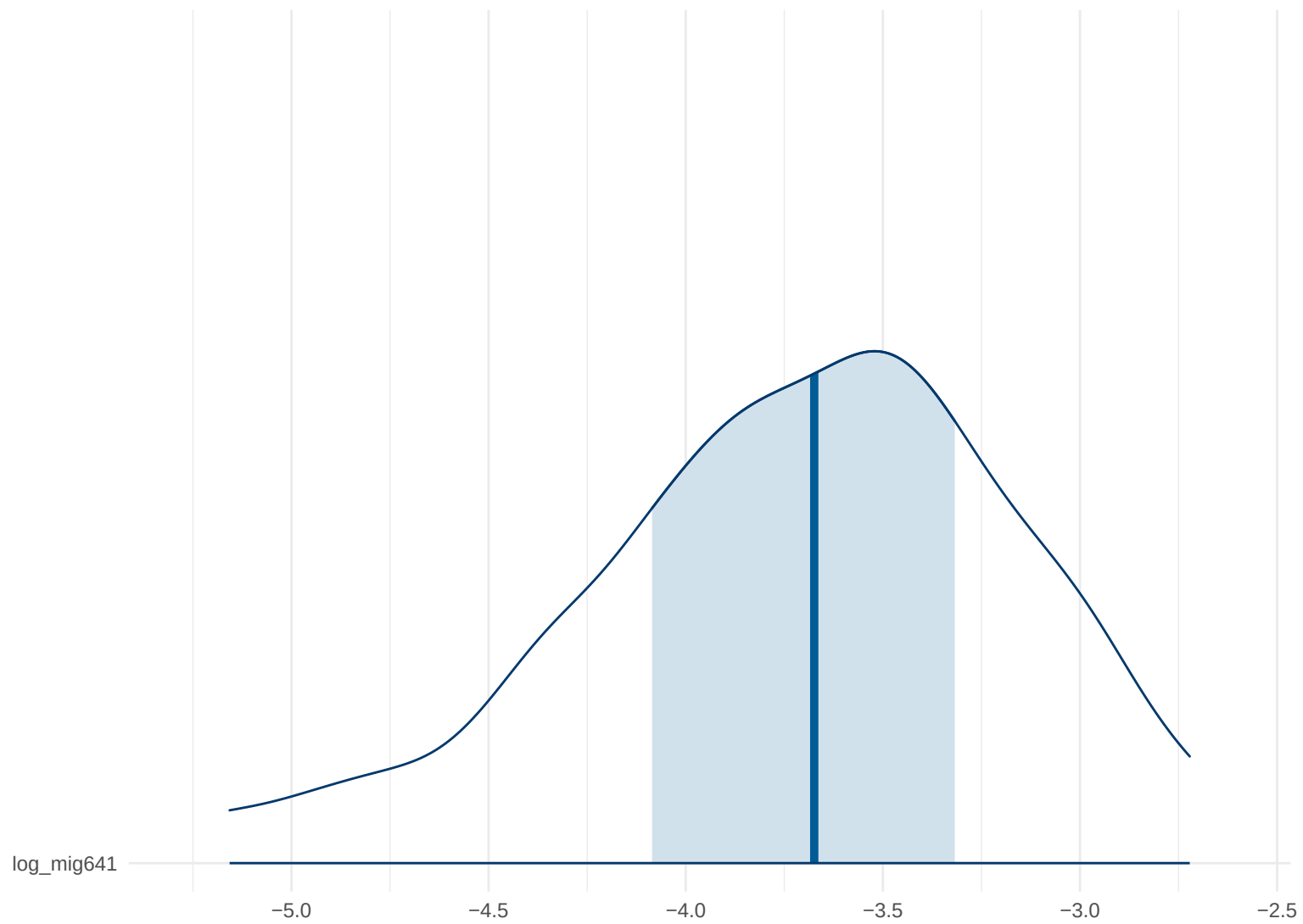
Posterior Density: log_mig641
