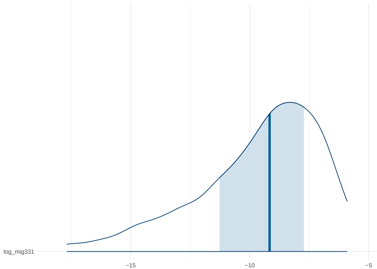
Posterior Density: log_mig331
