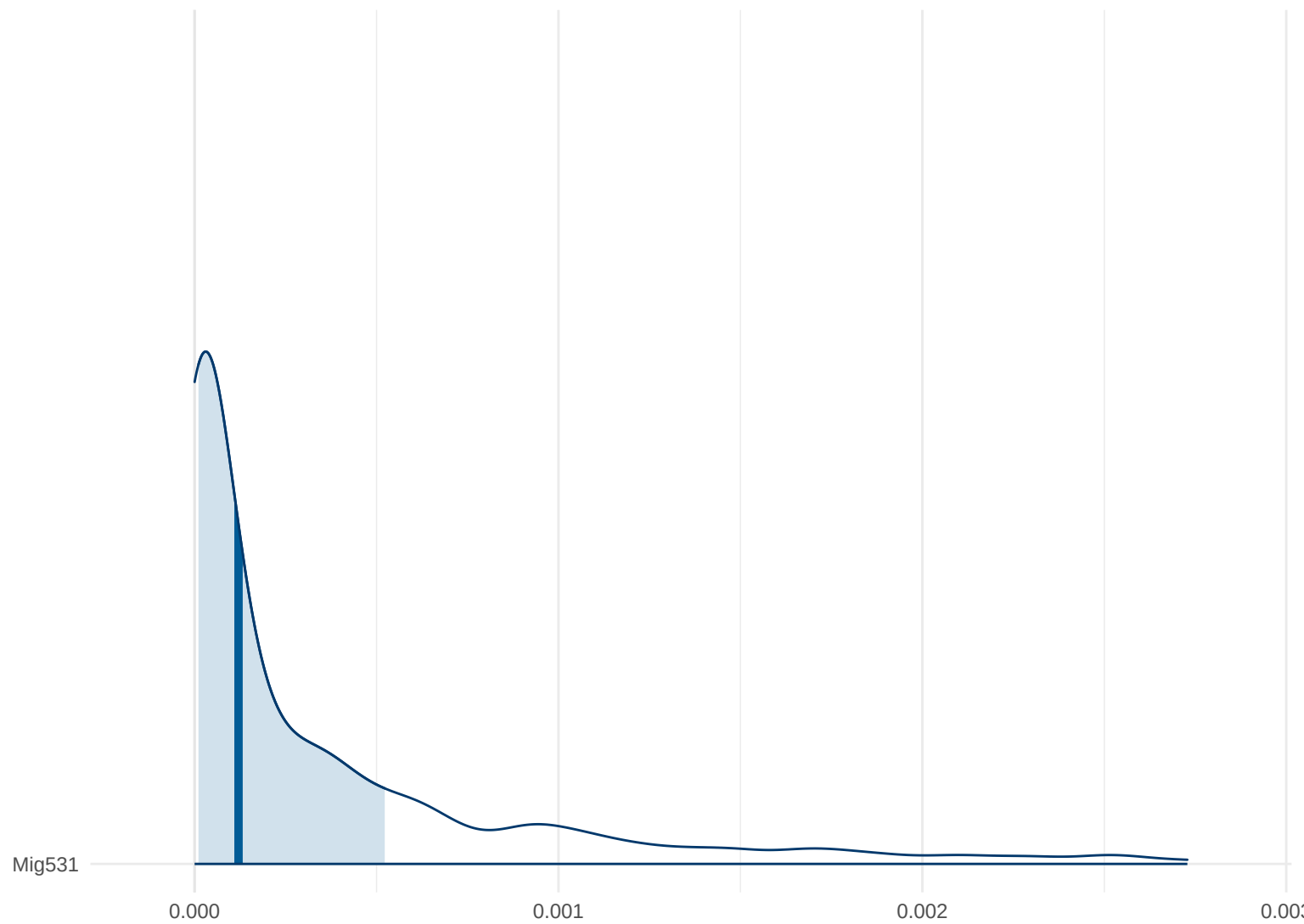
Posterior Density: Mig531
