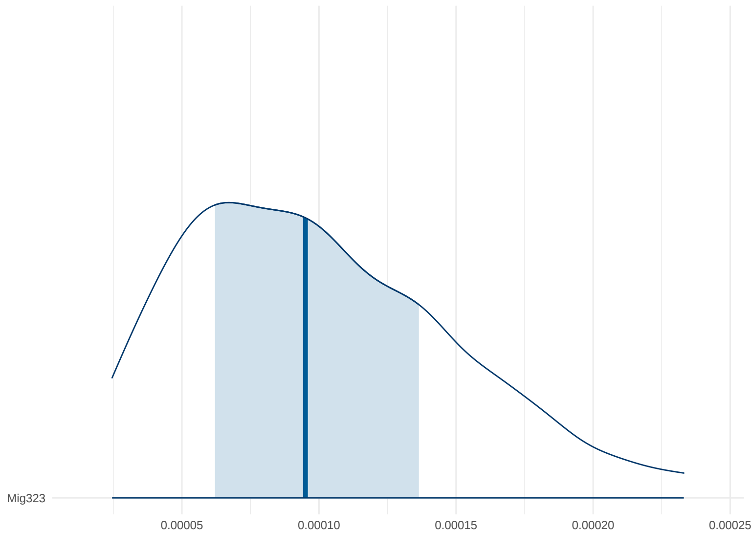
Posterior Density: Mig323
