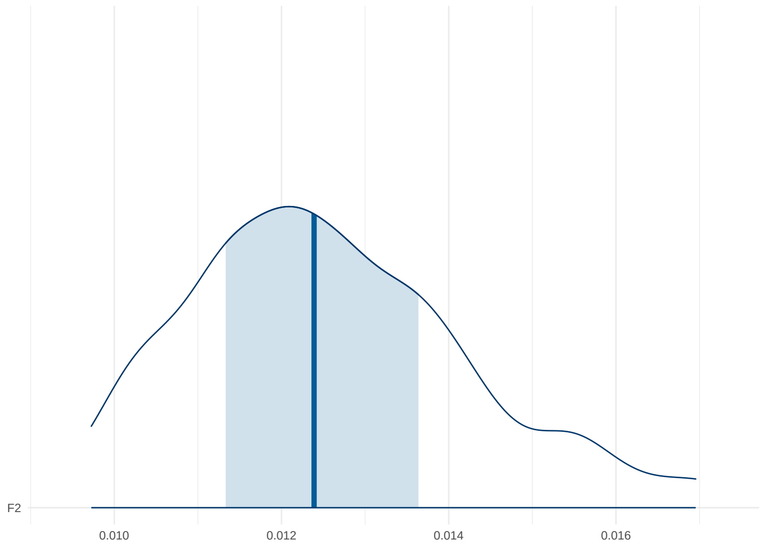
Posterior Density: F2
