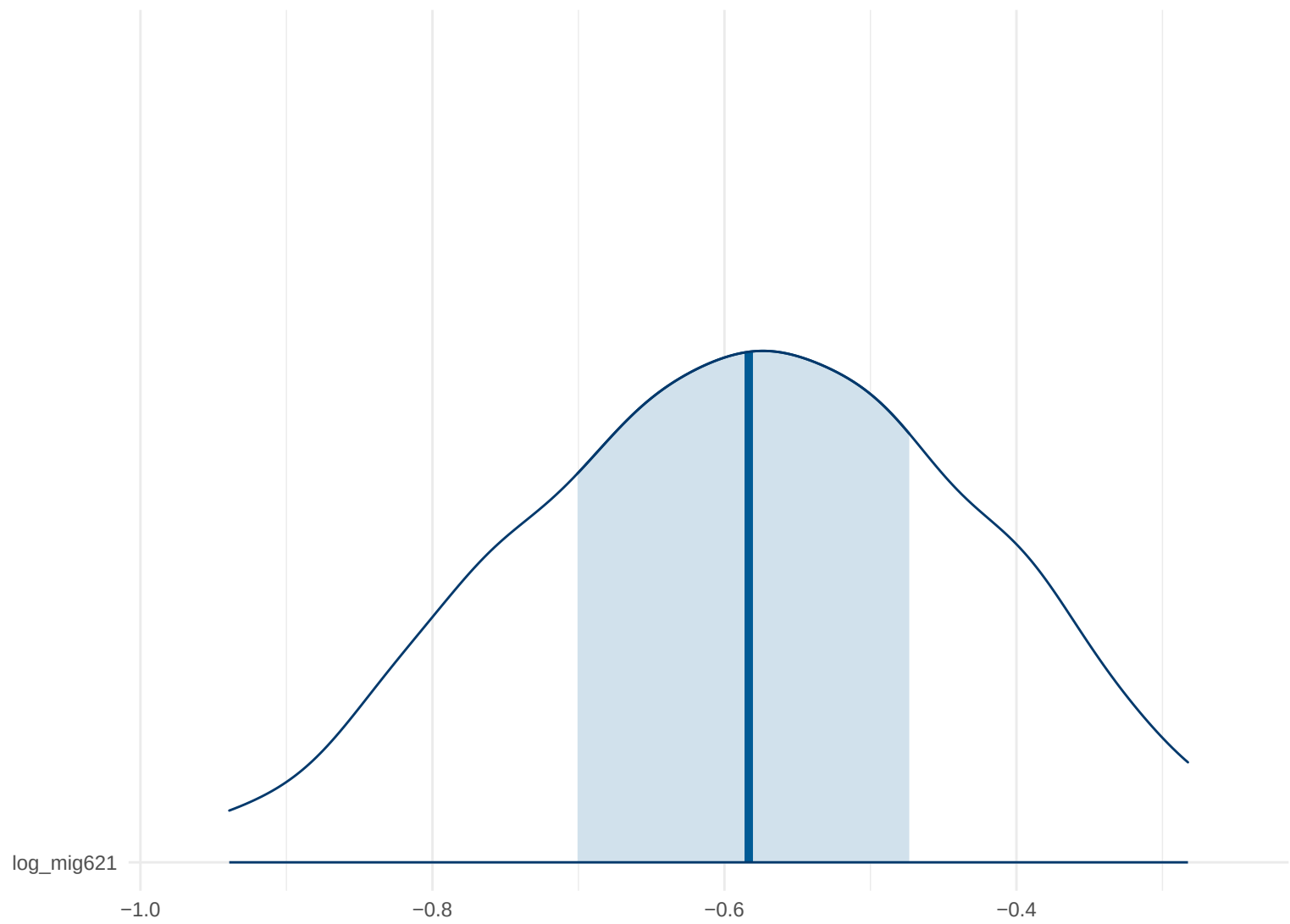
Posterior Density: log_mig621
