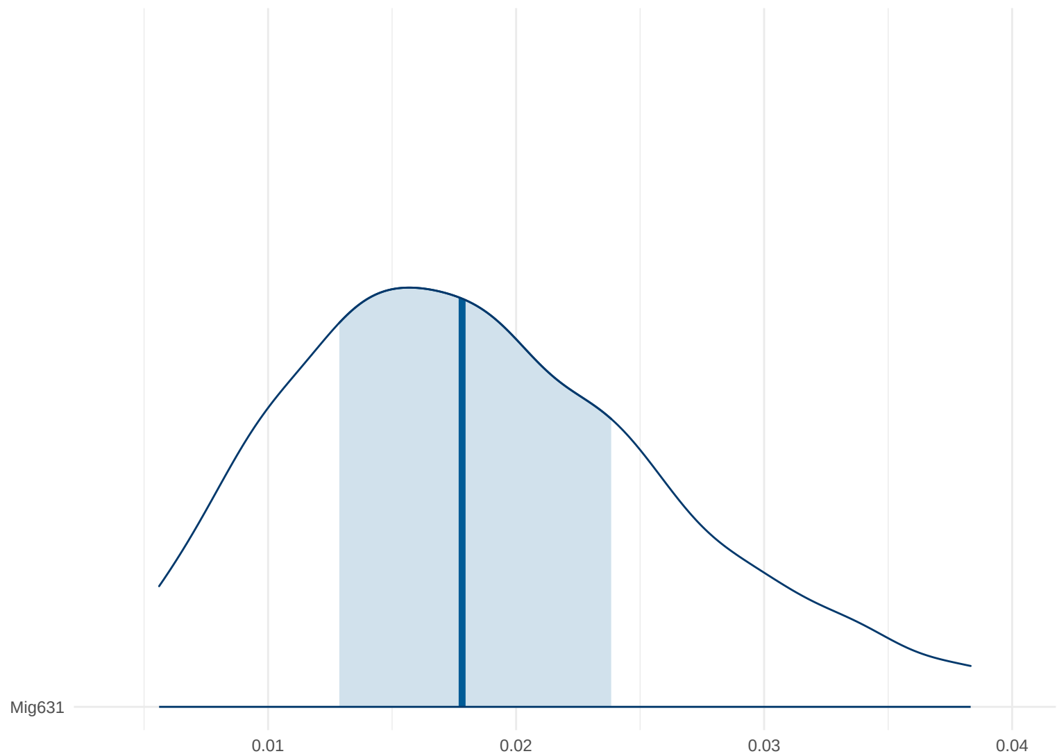
Posterior Density: Mig631
