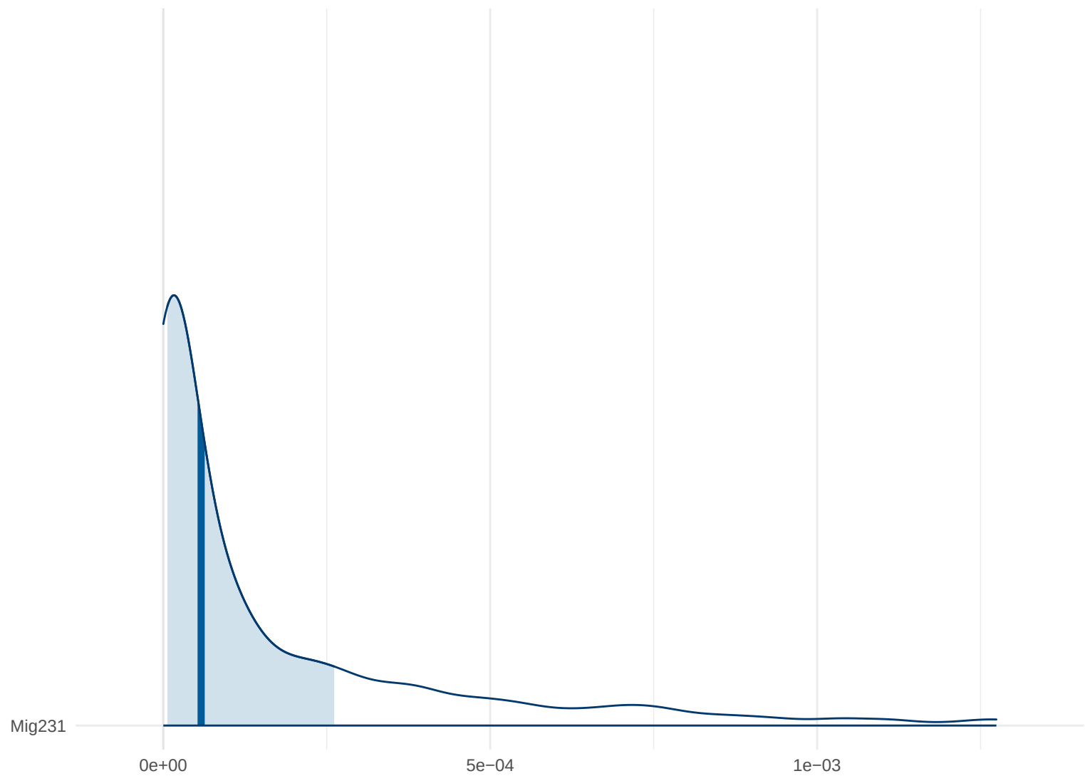
Posterior Density: Mig231
