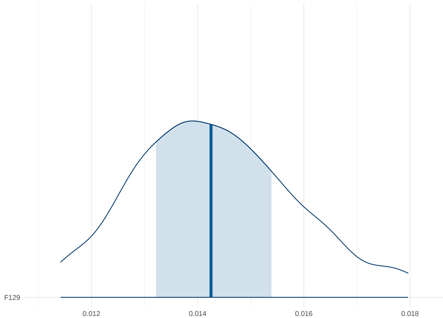
Posterior Density: F129
