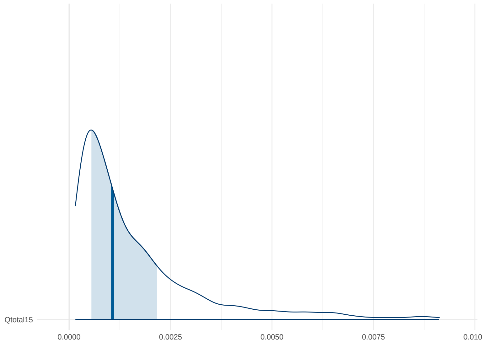
Posterior Density: Qtotal15
