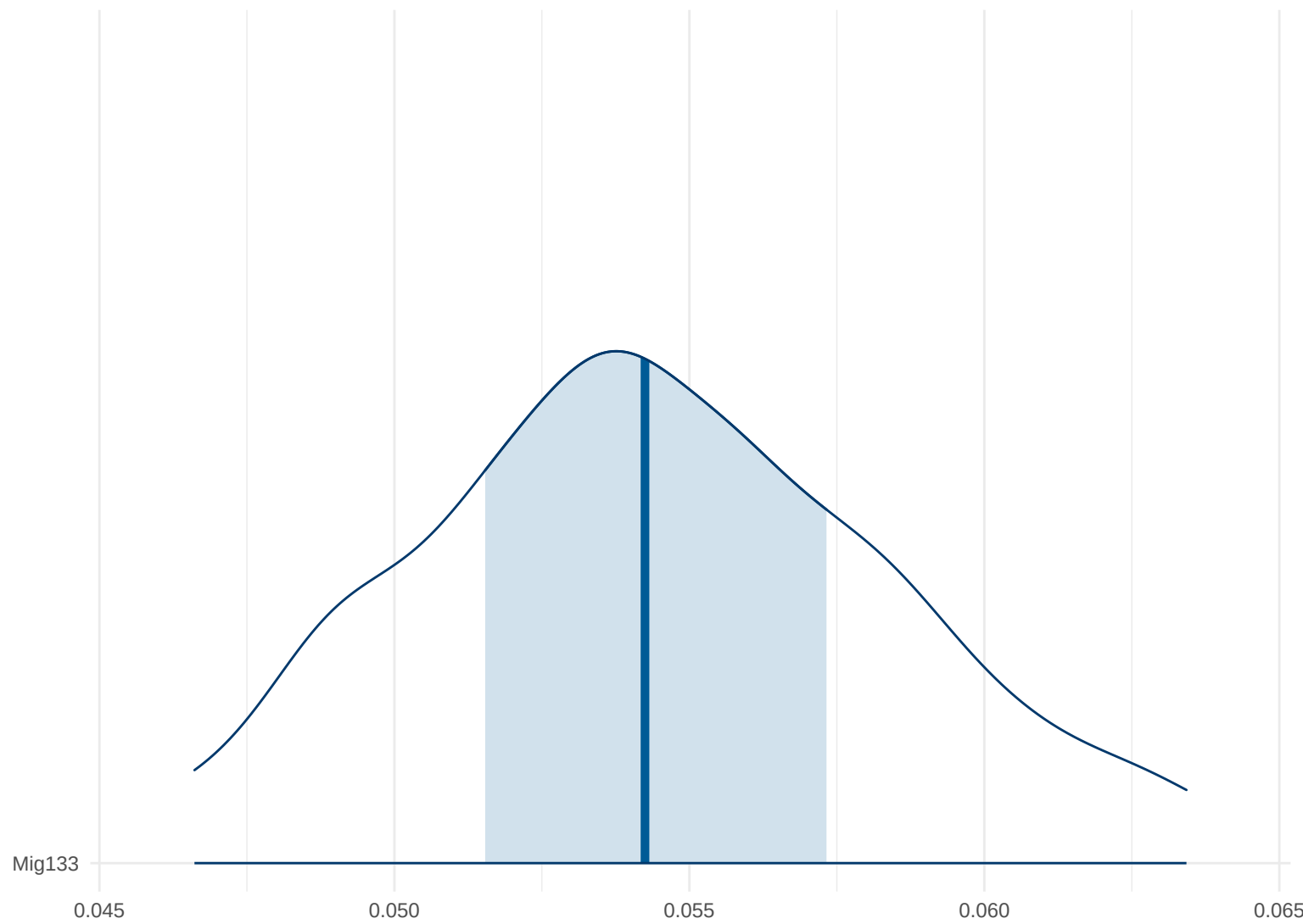
Posterior Density: Mig133
