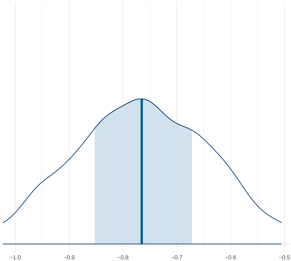
Posterior Density: Theta20
