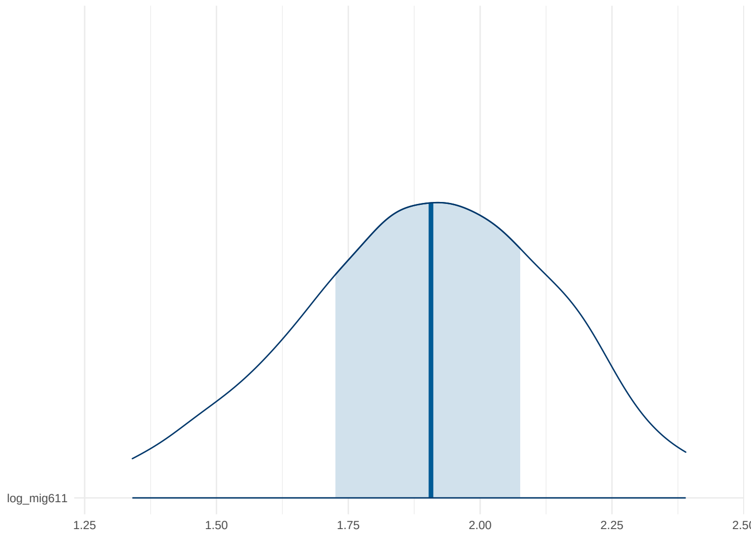
Posterior Density: log_mig611
