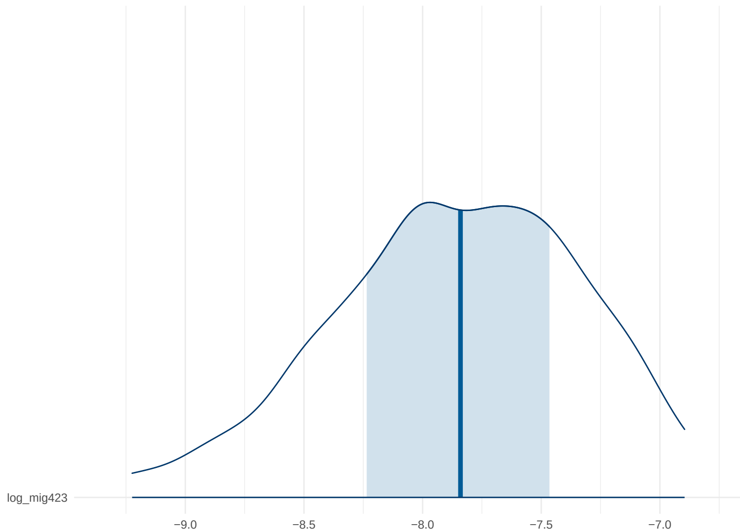
Posterior Density: log_mig423
