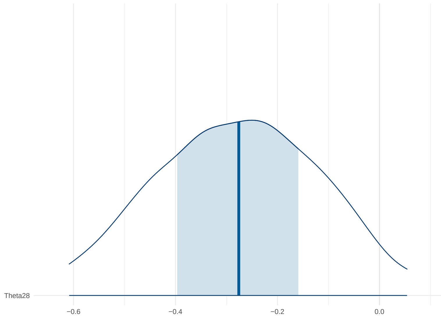
Posterior Density: Theta28
