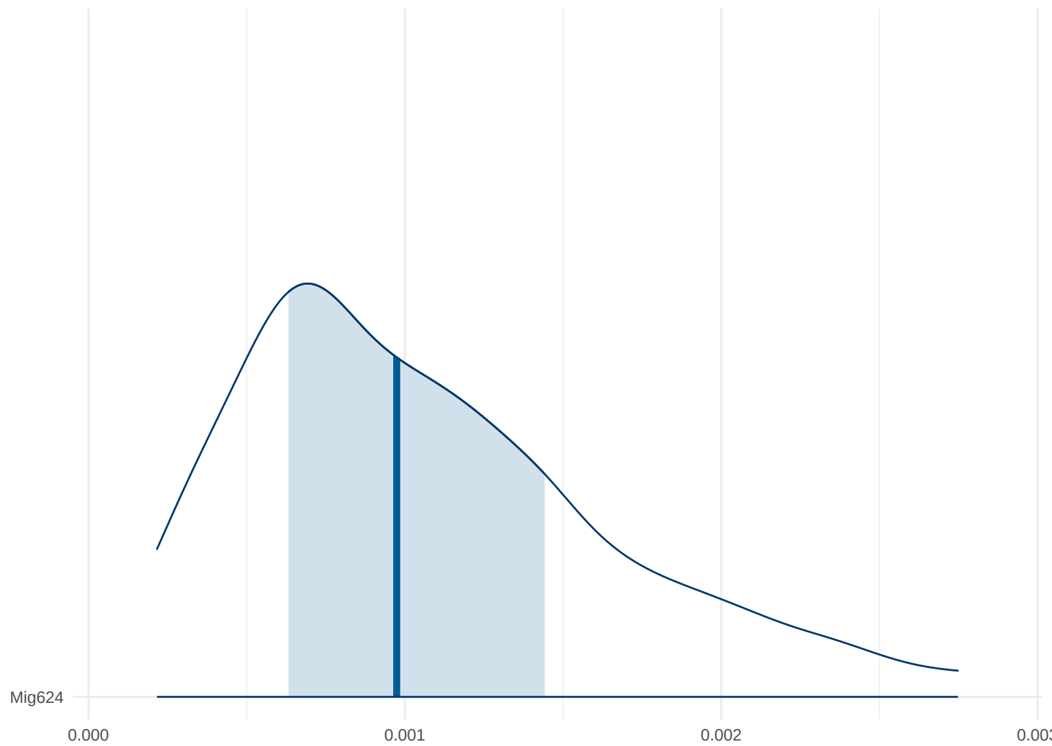
Posterior Density: Mig624
