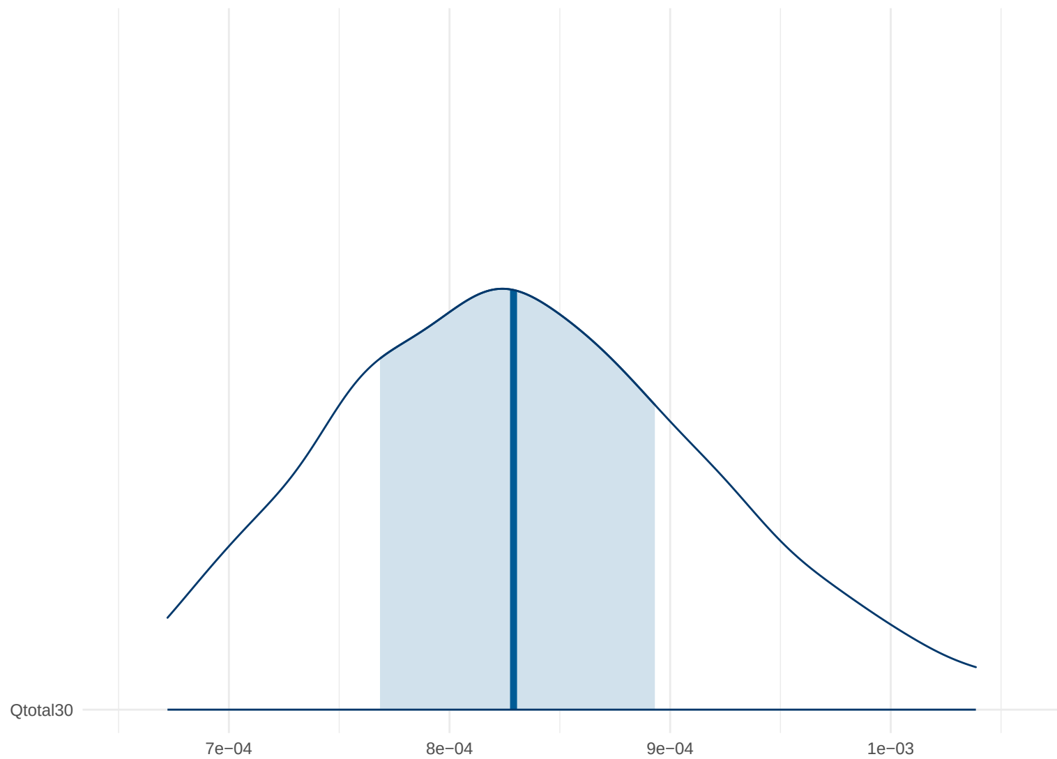
Posterior Density: Qtotal30
