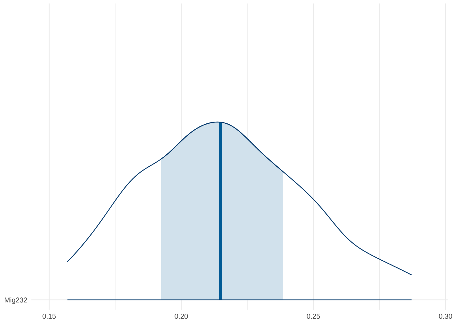
Posterior Density: Mig232
