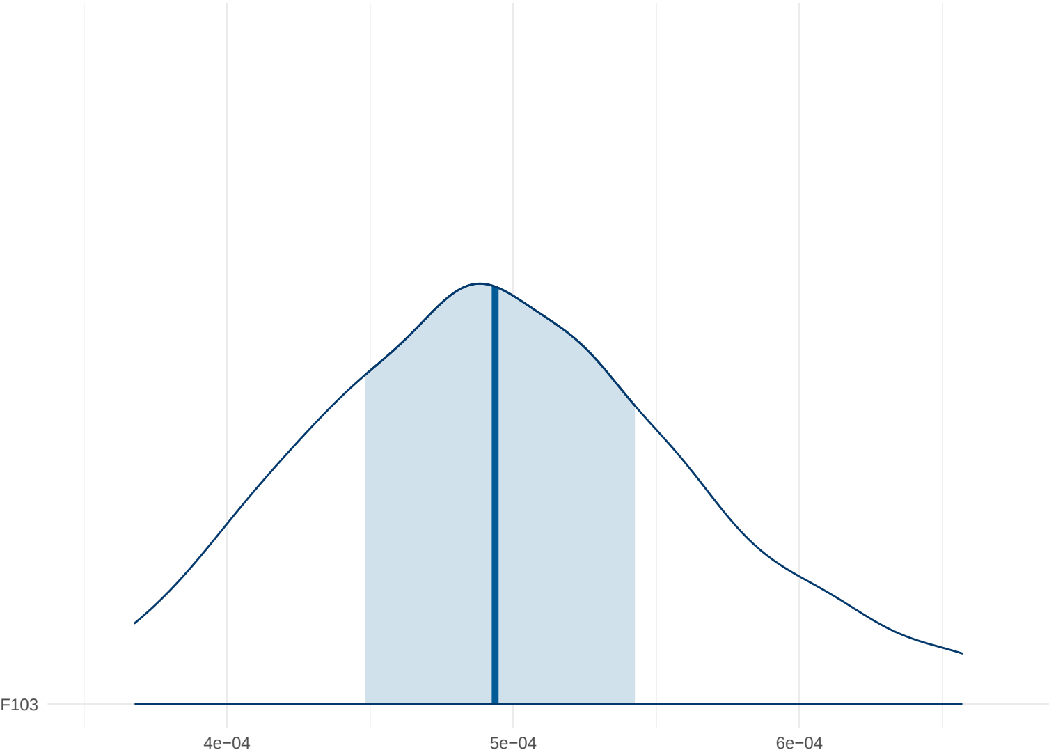
Posterior Density: F103
