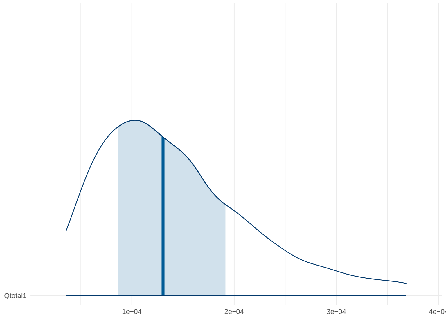
Posterior Density: Qtotal1
