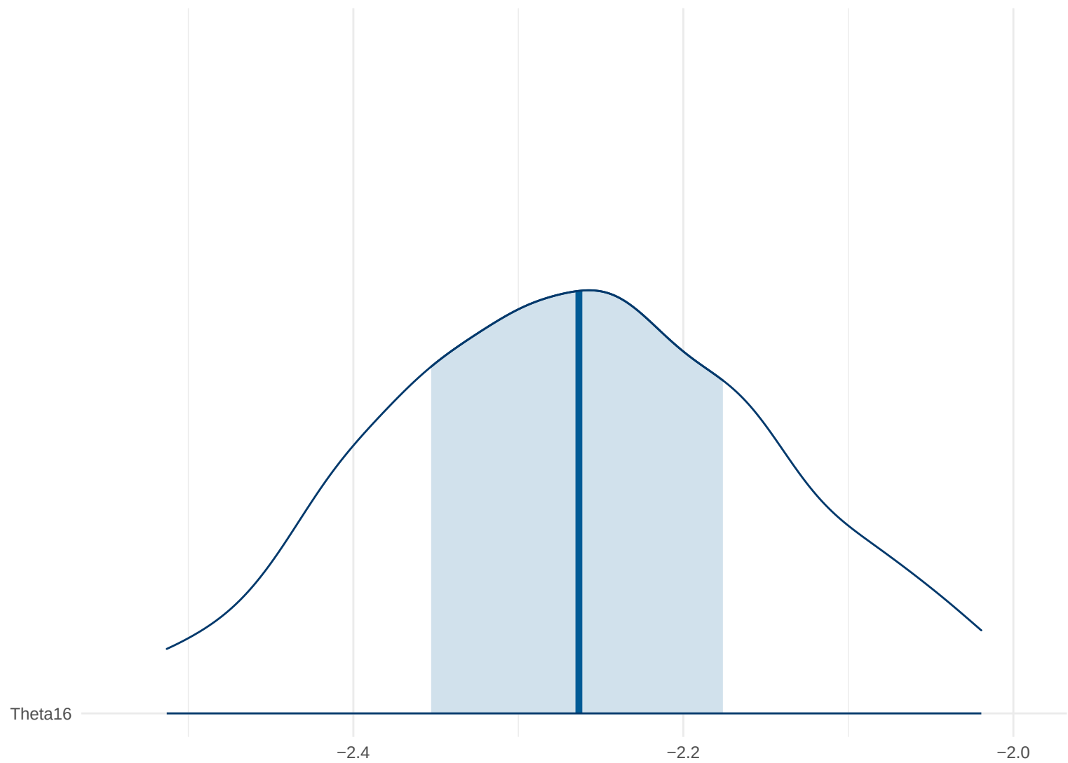
Posterior Density: Theta16
