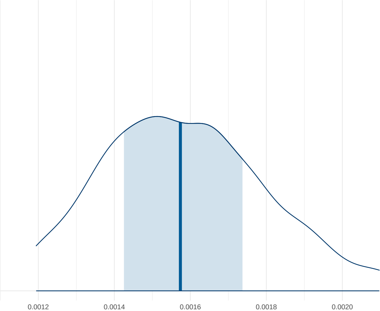
Posterior Density: F143
