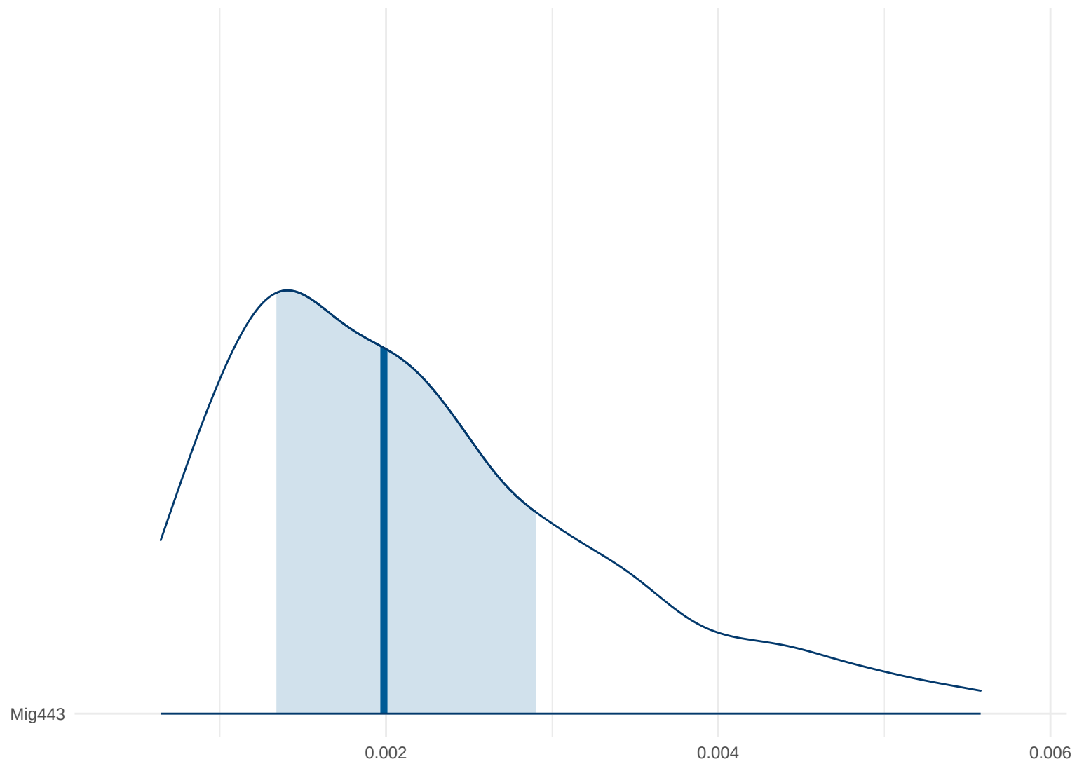
Posterior Density: Mig443
