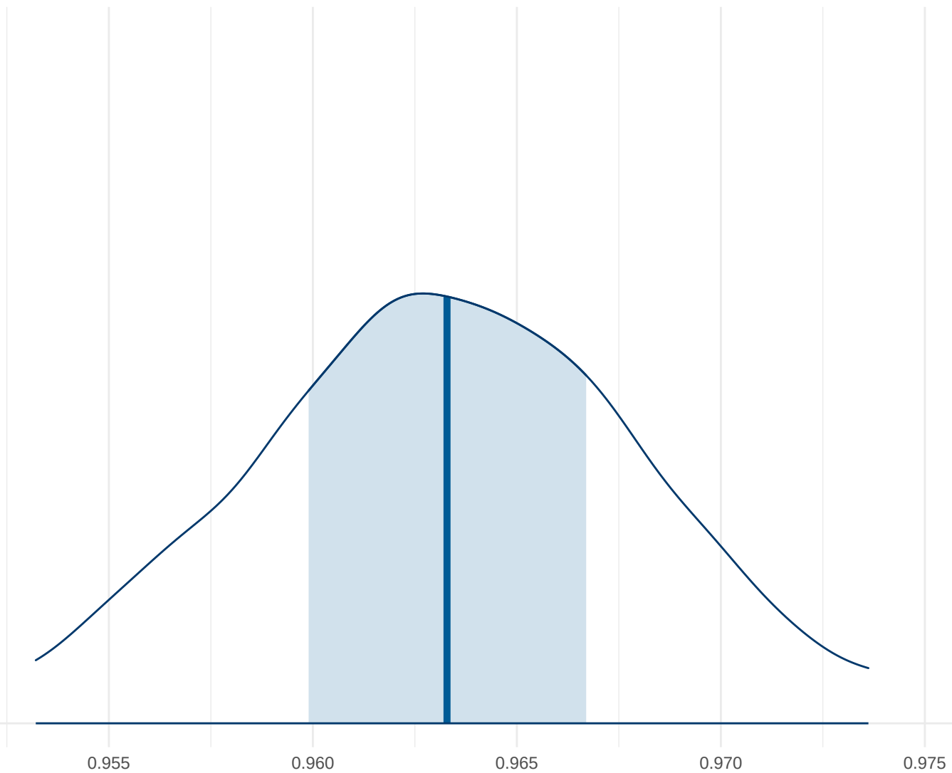
Posterior Density: Mig144
