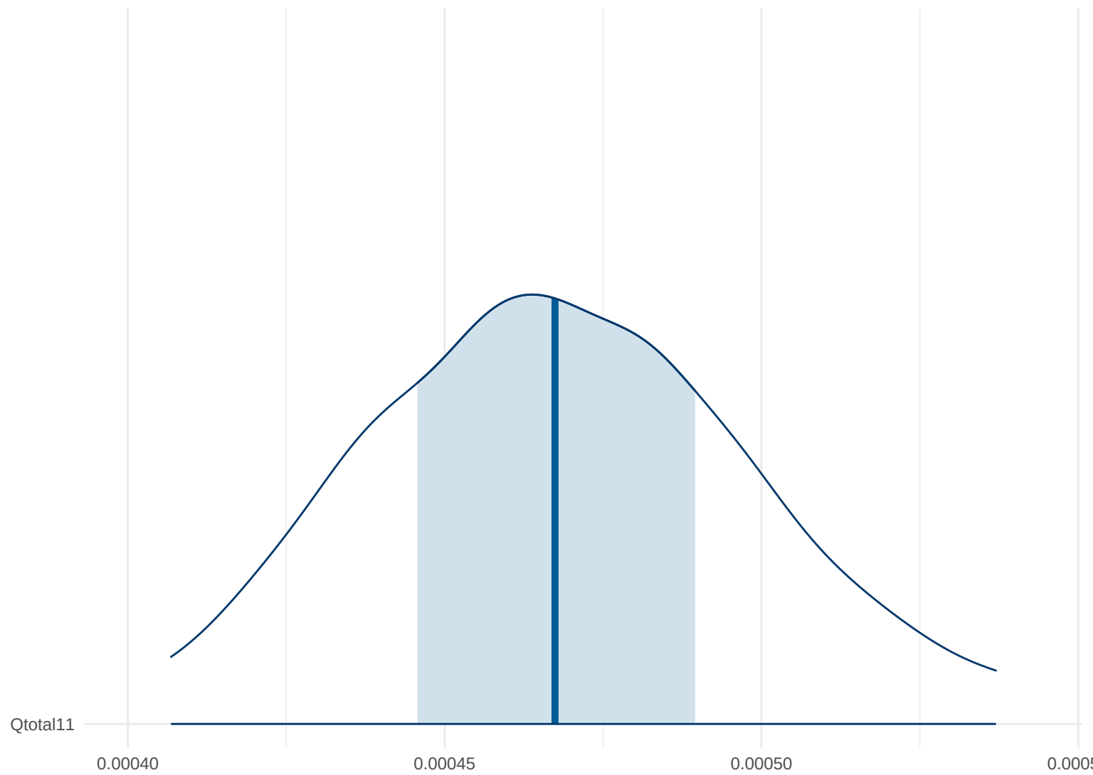
Posterior Density: Qtotal11
