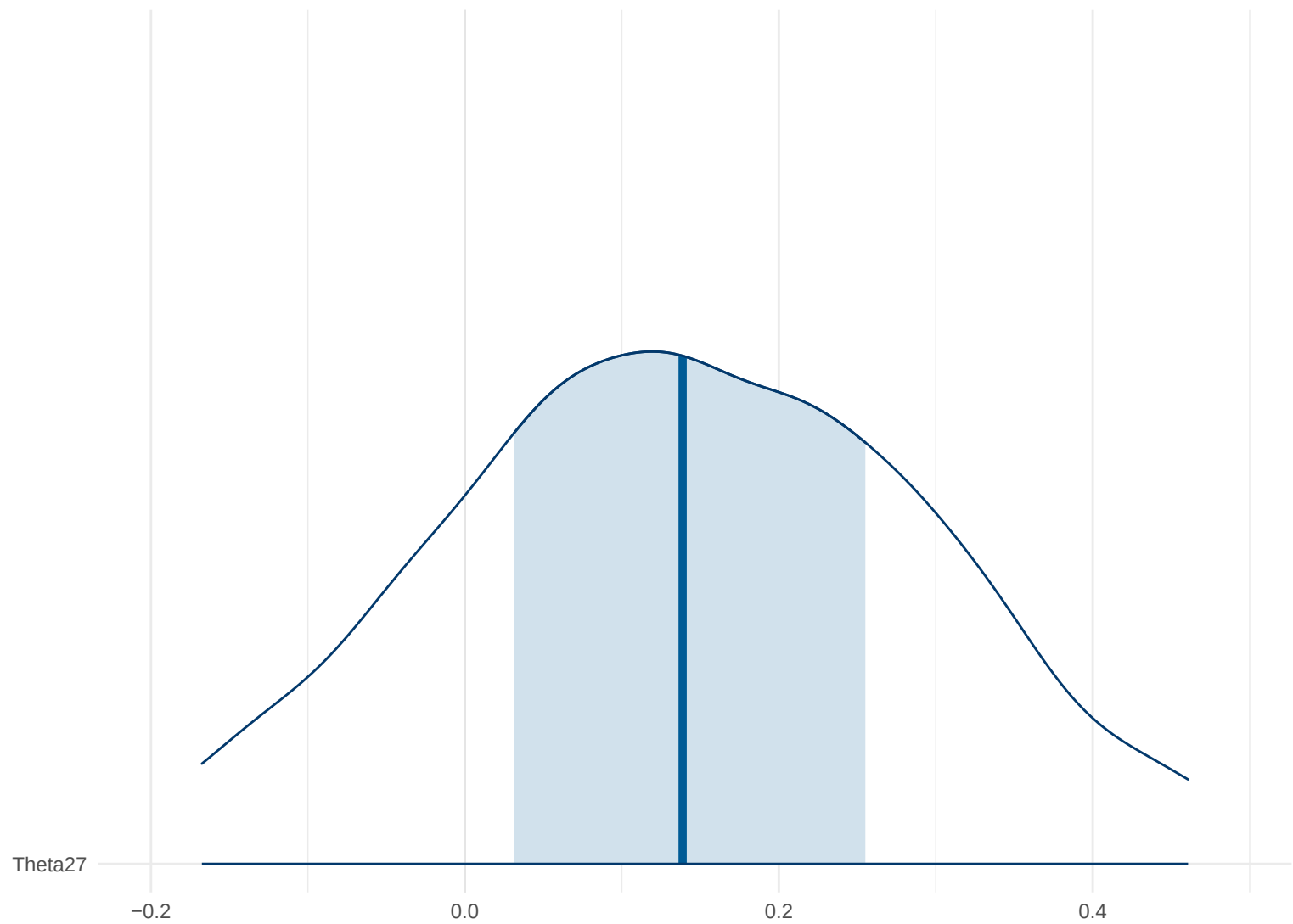
Posterior Density: Theta27
