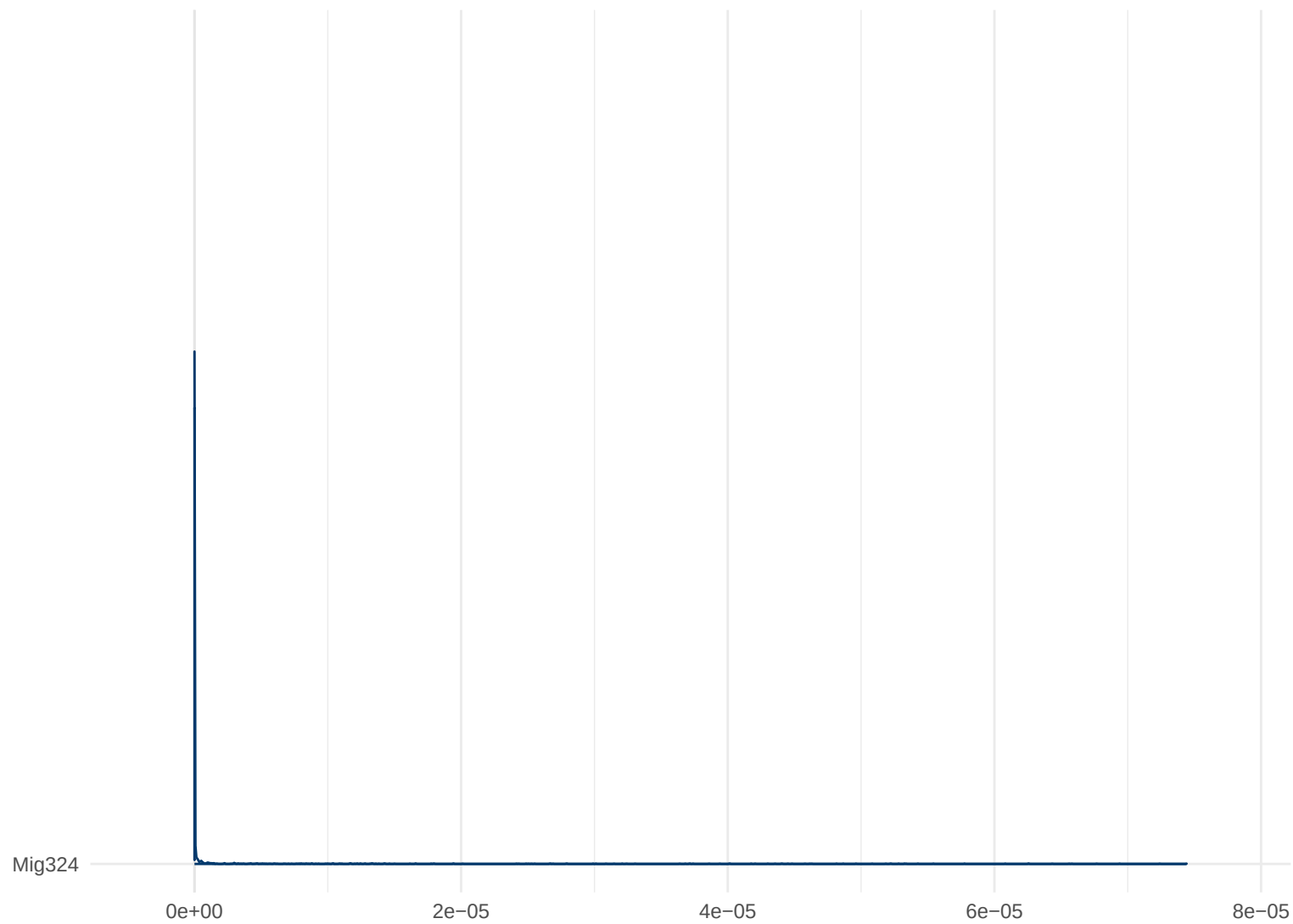
Posterior Density: Mig324
