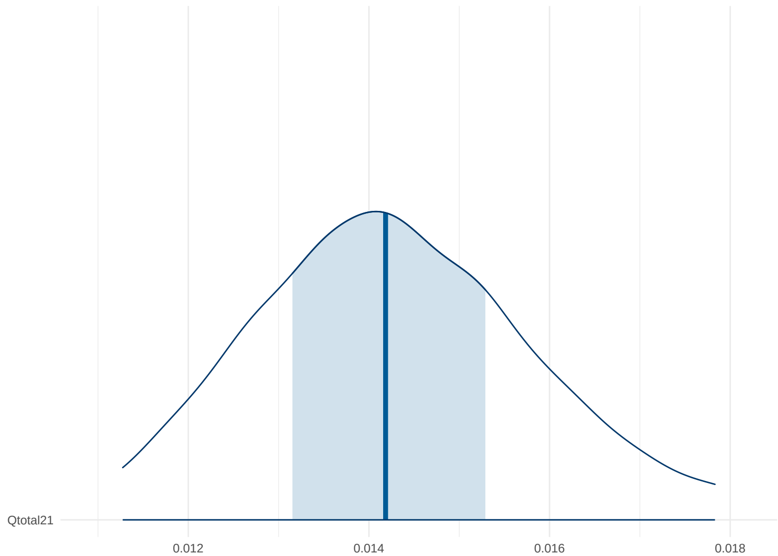
Posterior Density: Qtotal21
