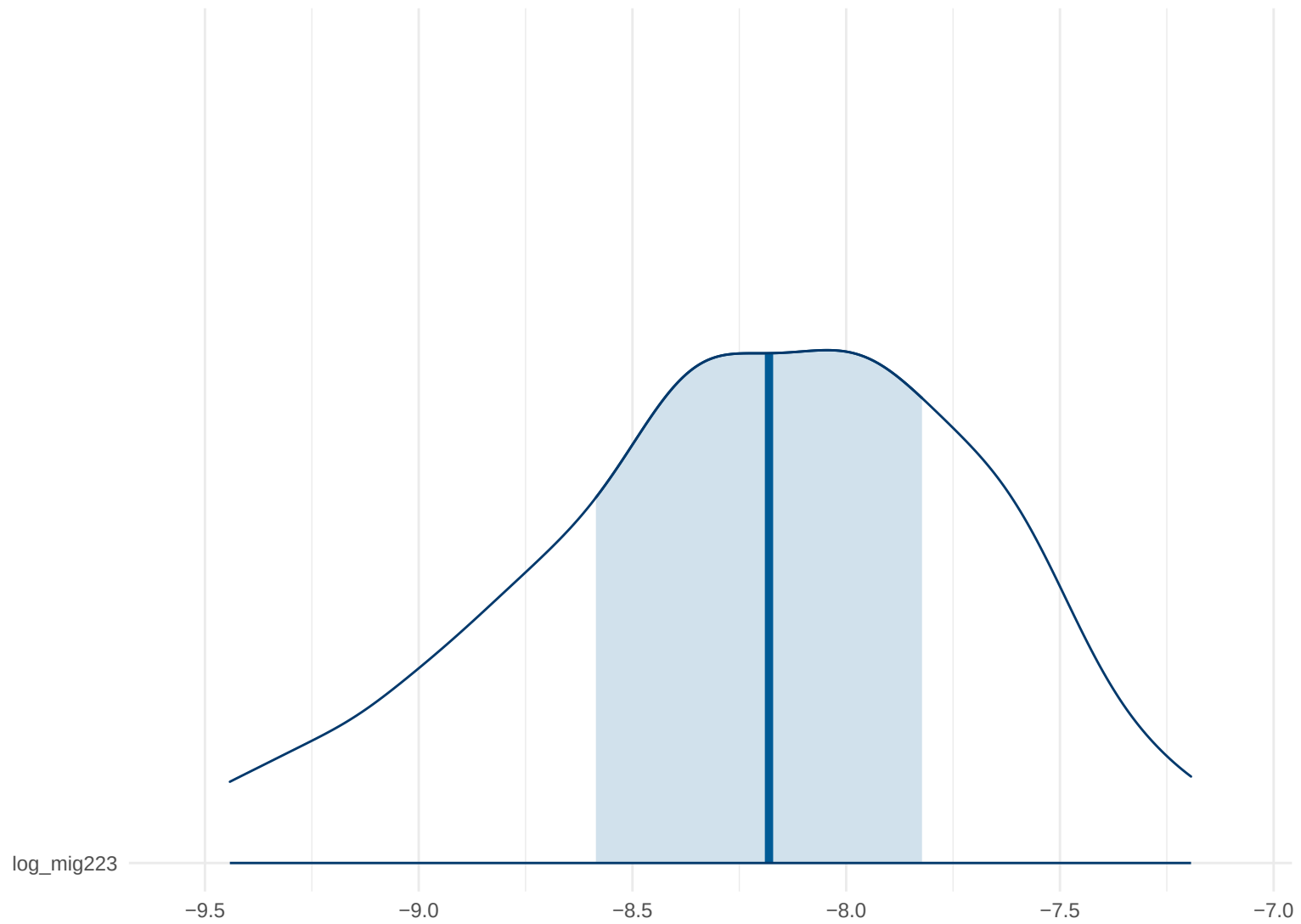
Posterior Density: log_mig223
