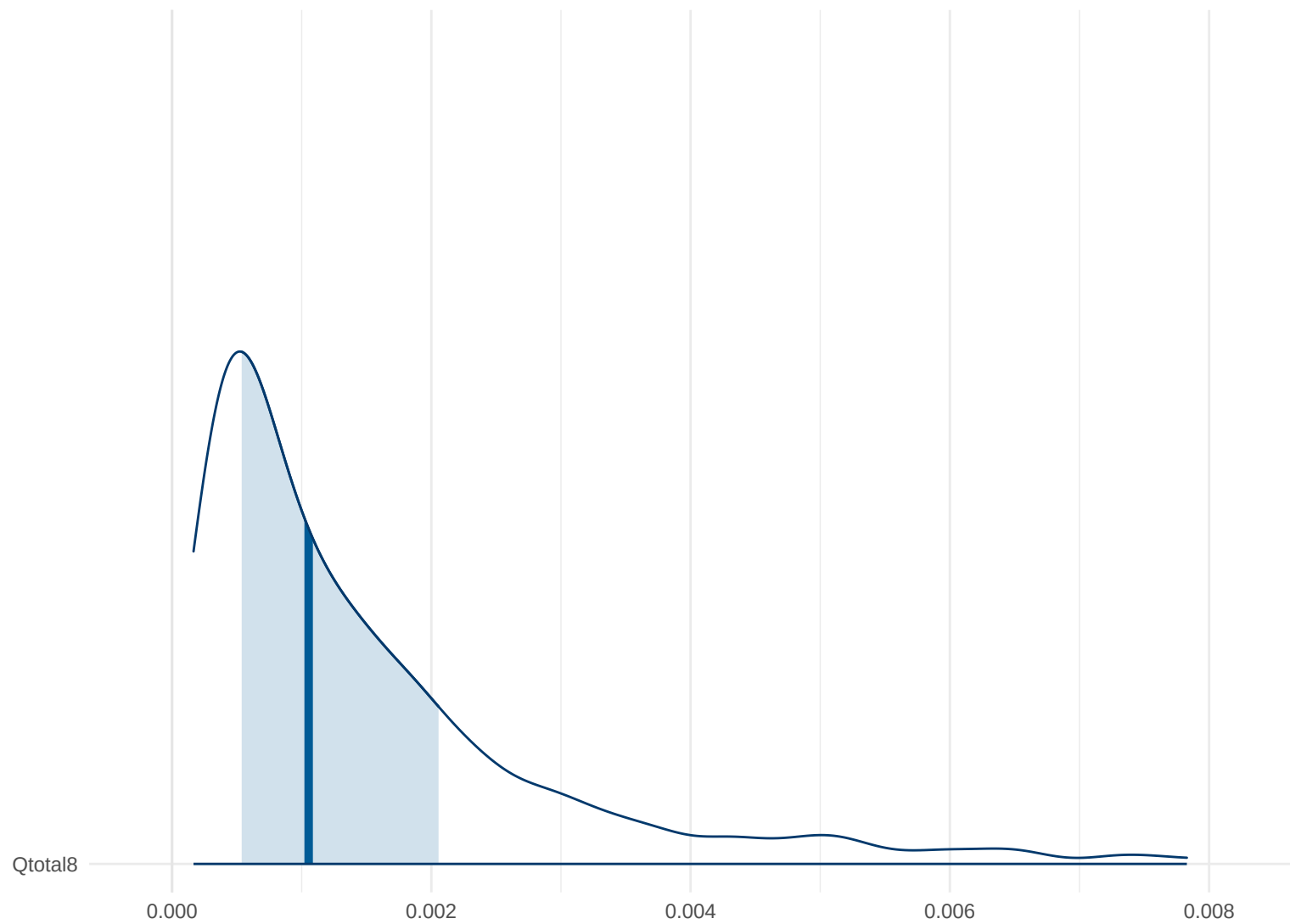
Posterior Density: Qtotal8
