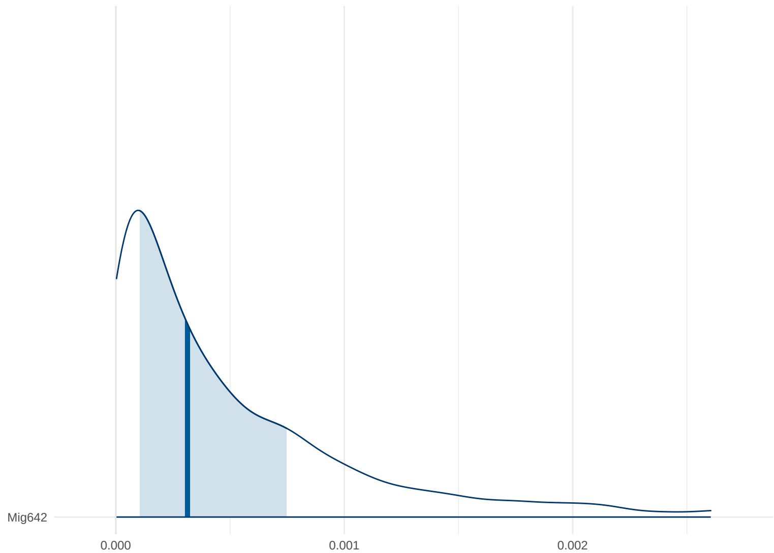
Posterior Density: Mig642
