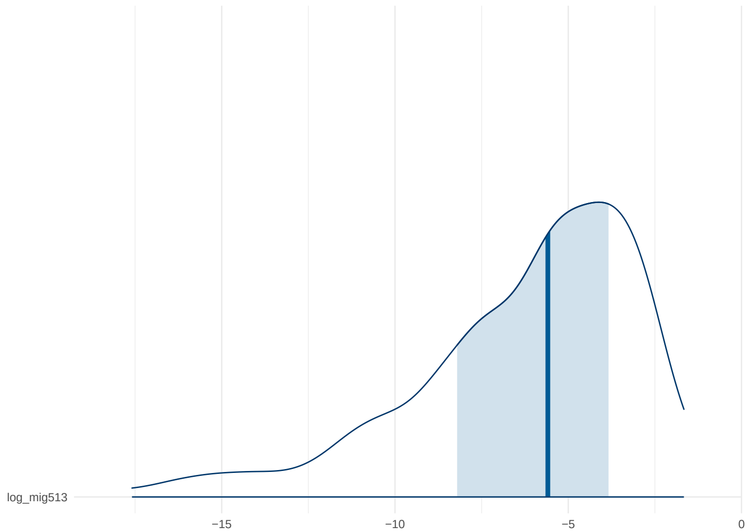
Posterior Density: log_mig513
