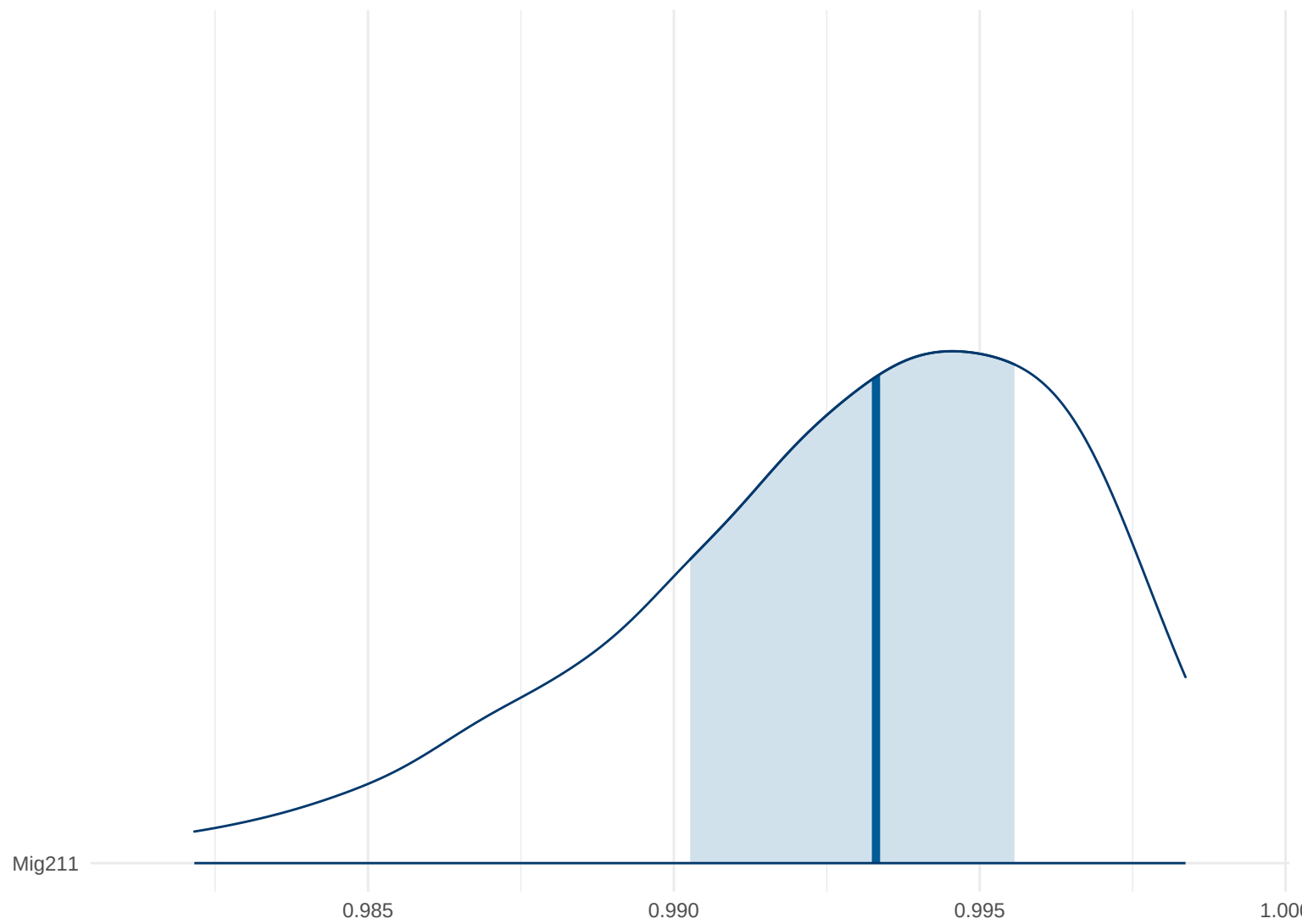
Posterior Density: Mig211
