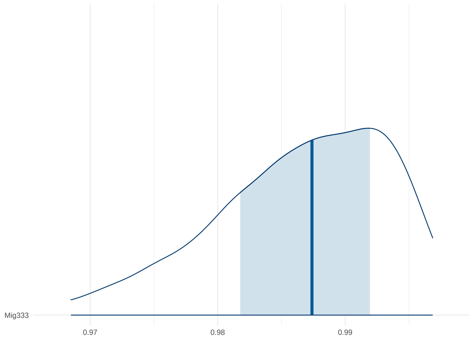
Posterior Density: Mig333
