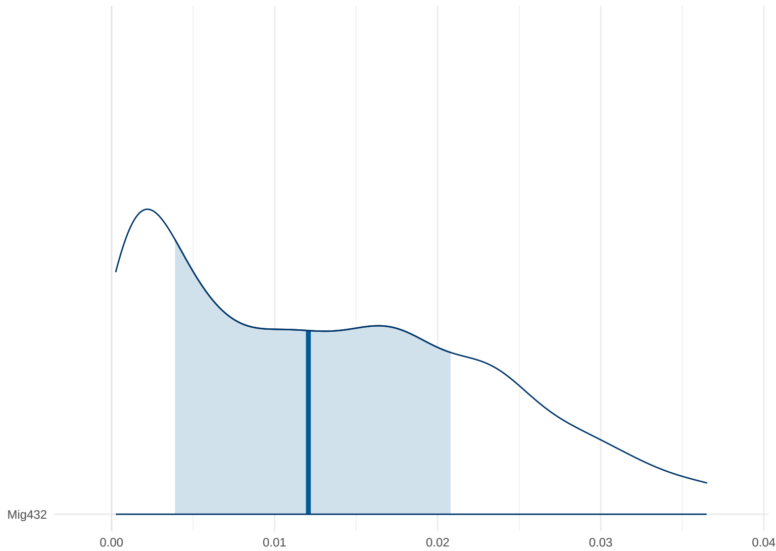
Posterior Density: Mig432
