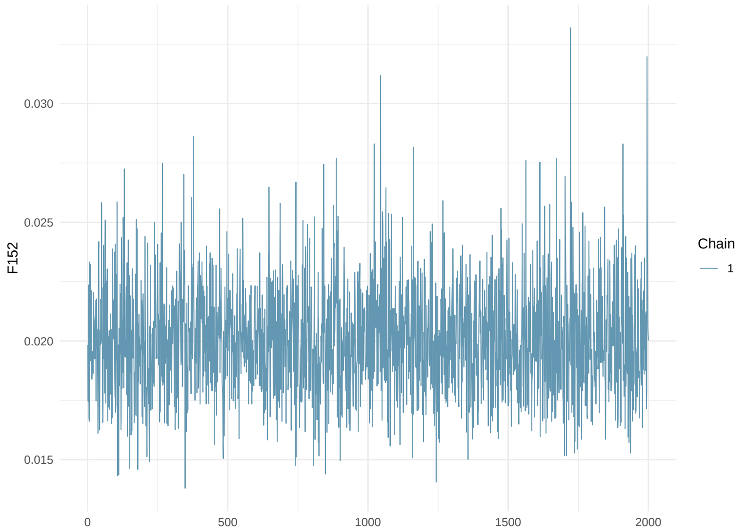
Trace Plot: F152
