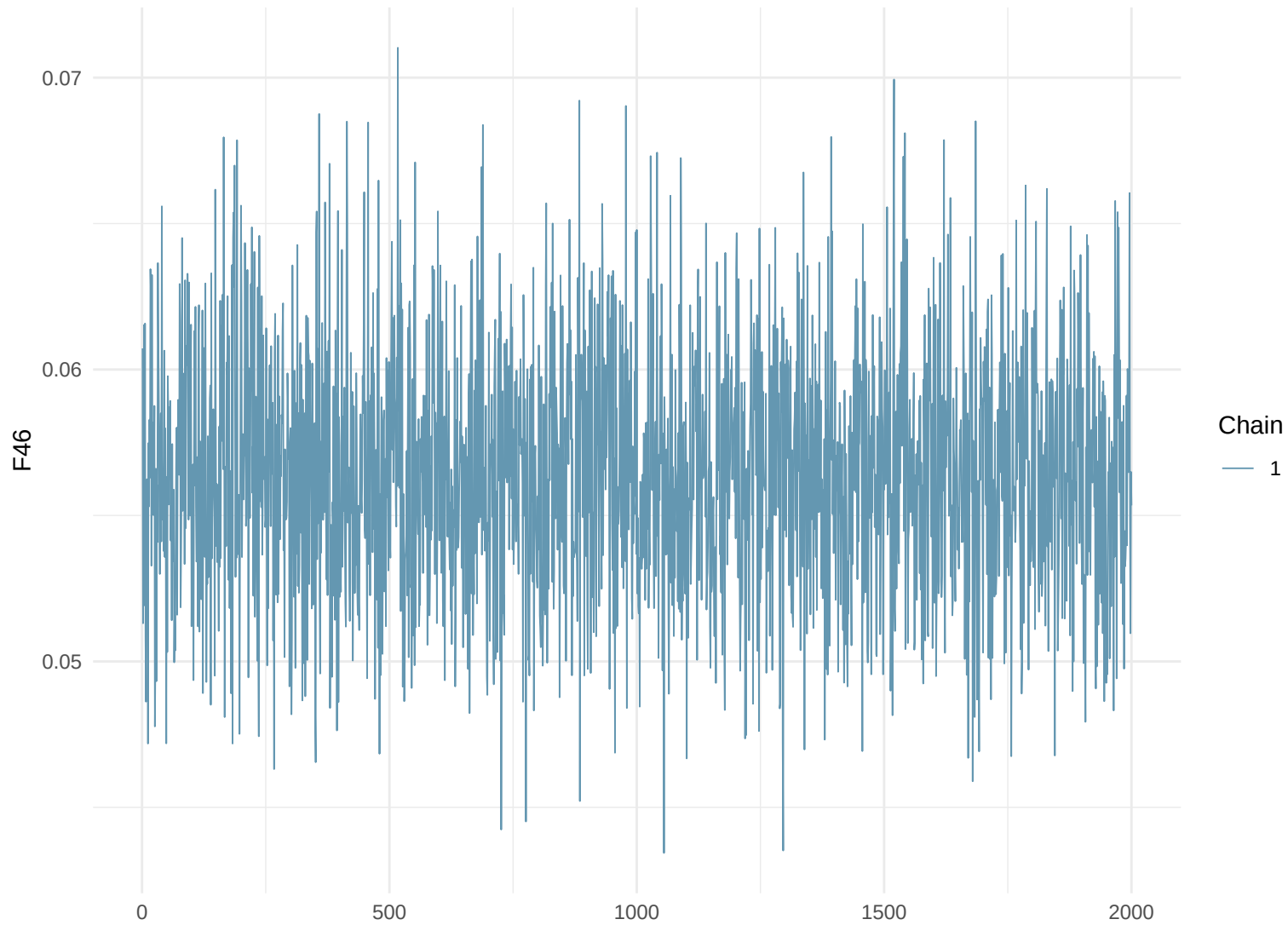
Trace Plot: F46
