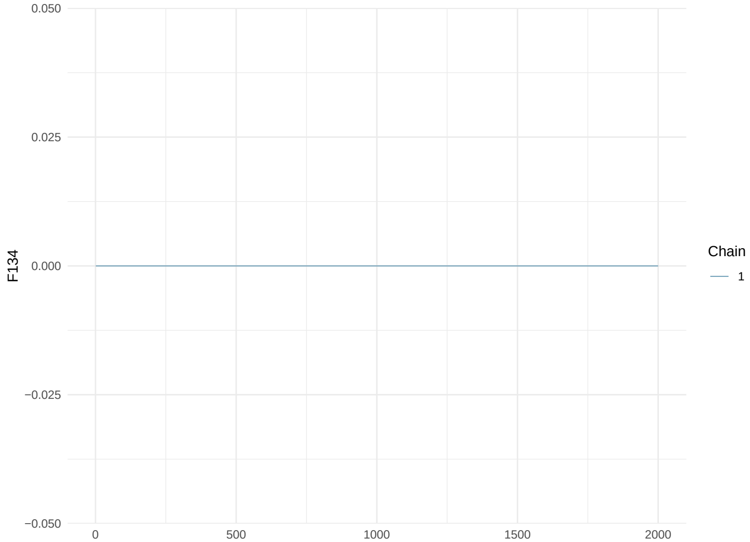
Trace Plot: F134
