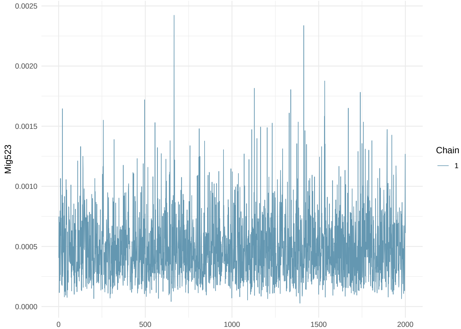
Trace Plot: Mig523
