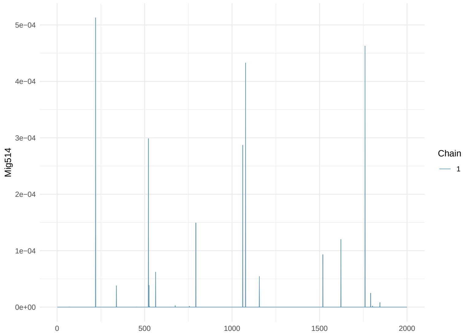
Trace Plot: Mig514
