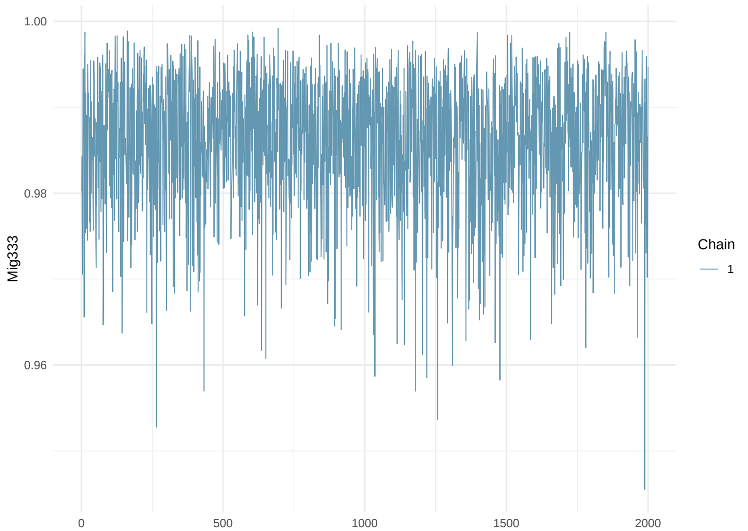
Trace Plot: Mig333
