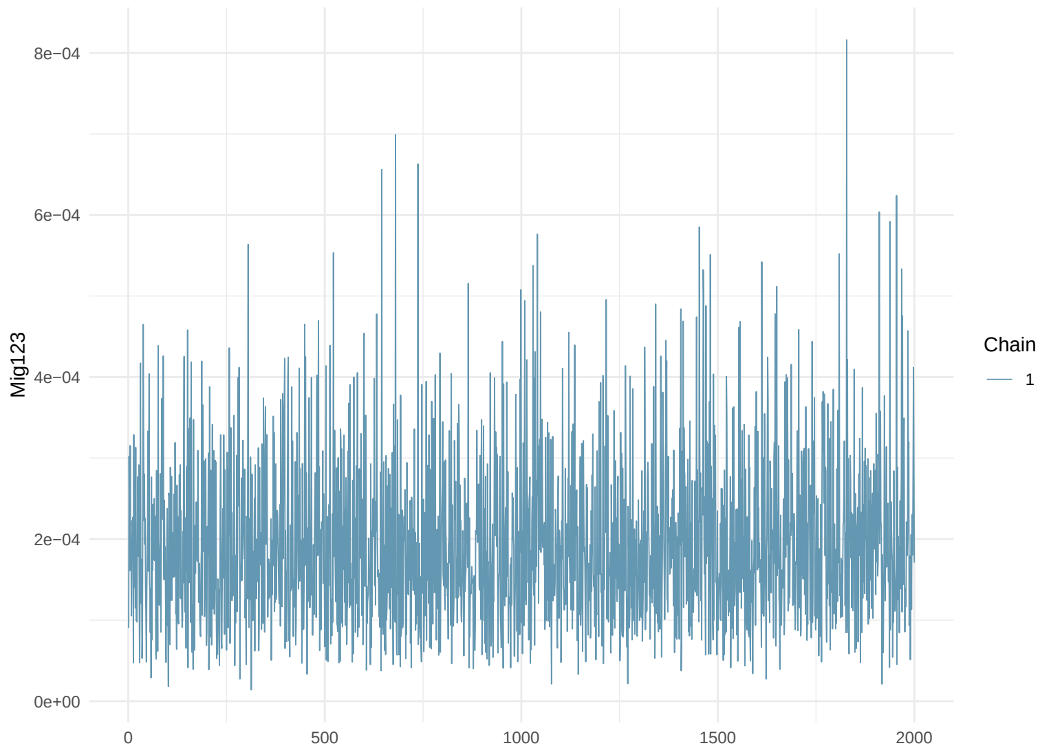
Trace Plot: Mig123
