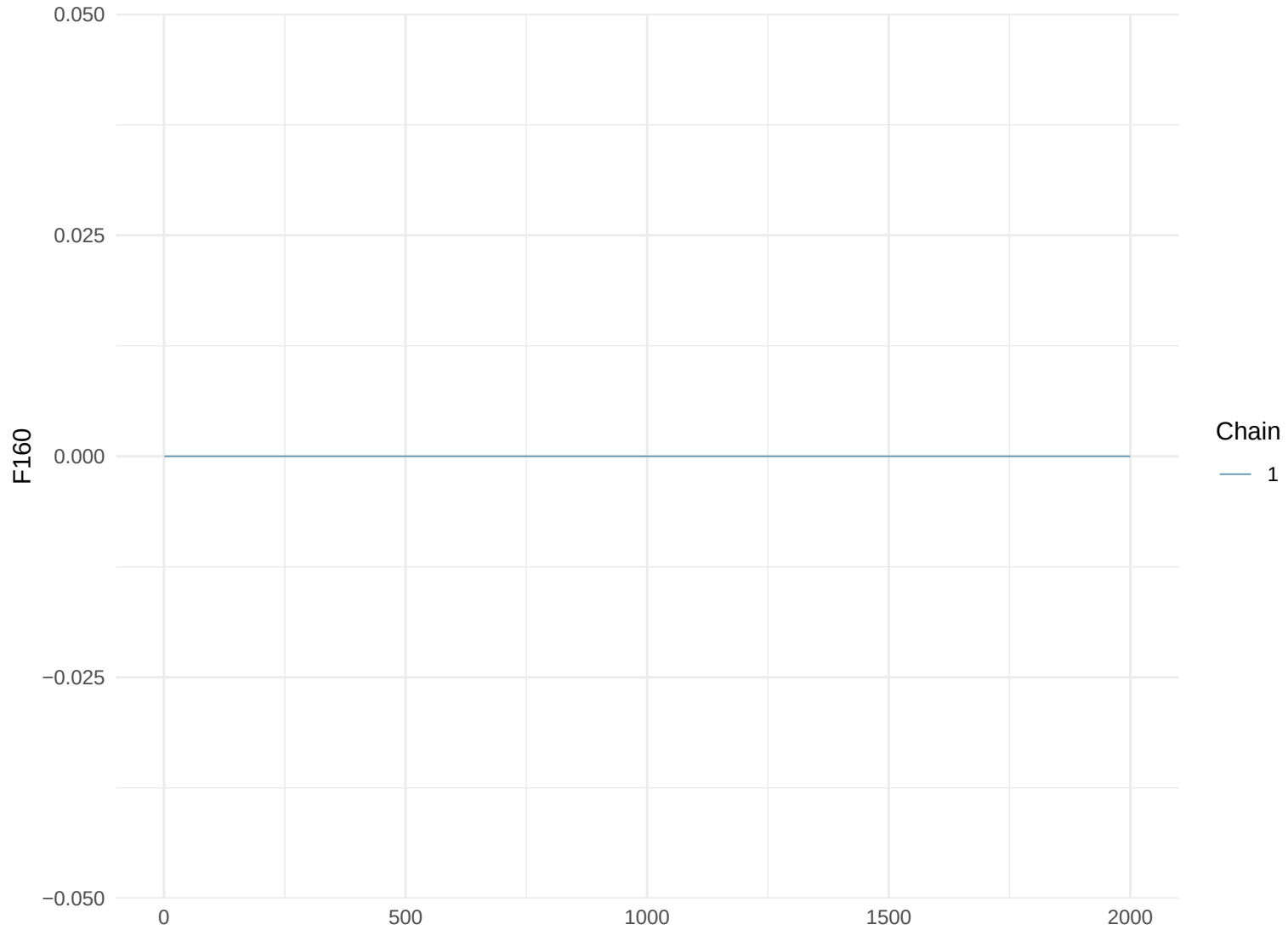
Trace Plot: F160
