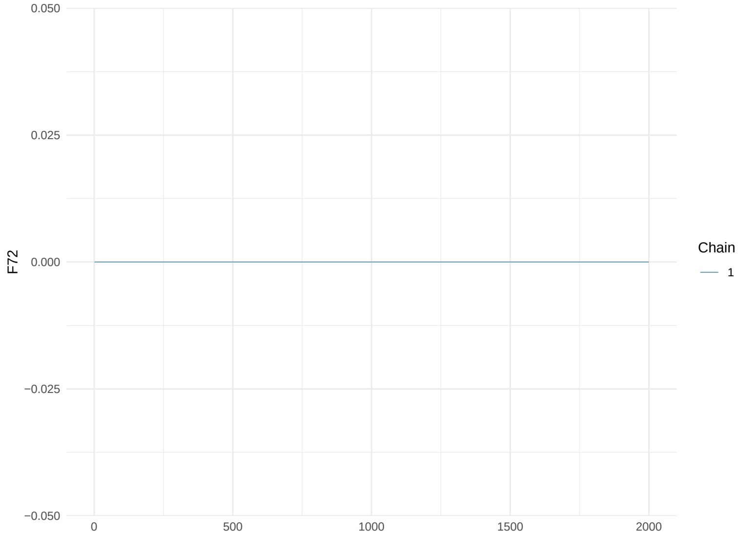
Trace Plot: F72
