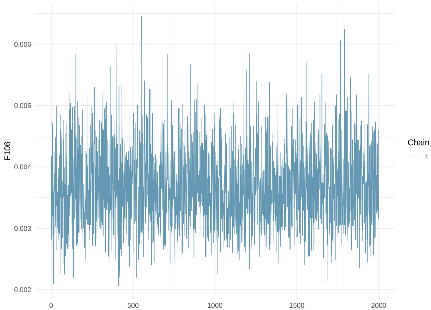
Trace Plot: F106
