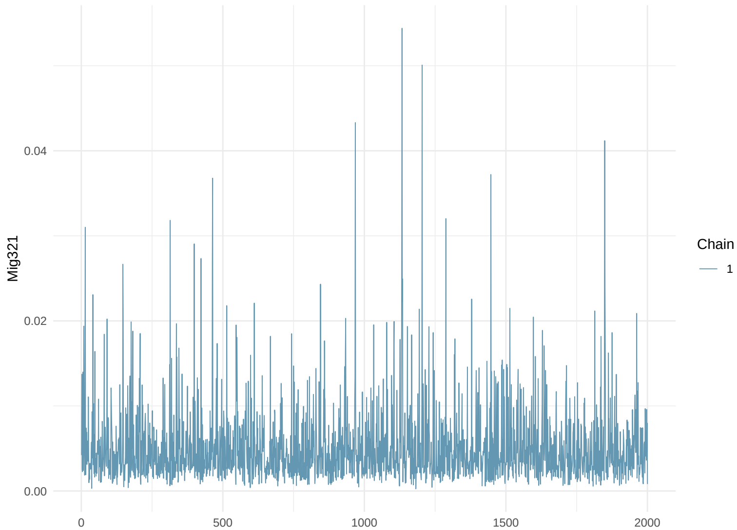
Trace Plot: Mig321
