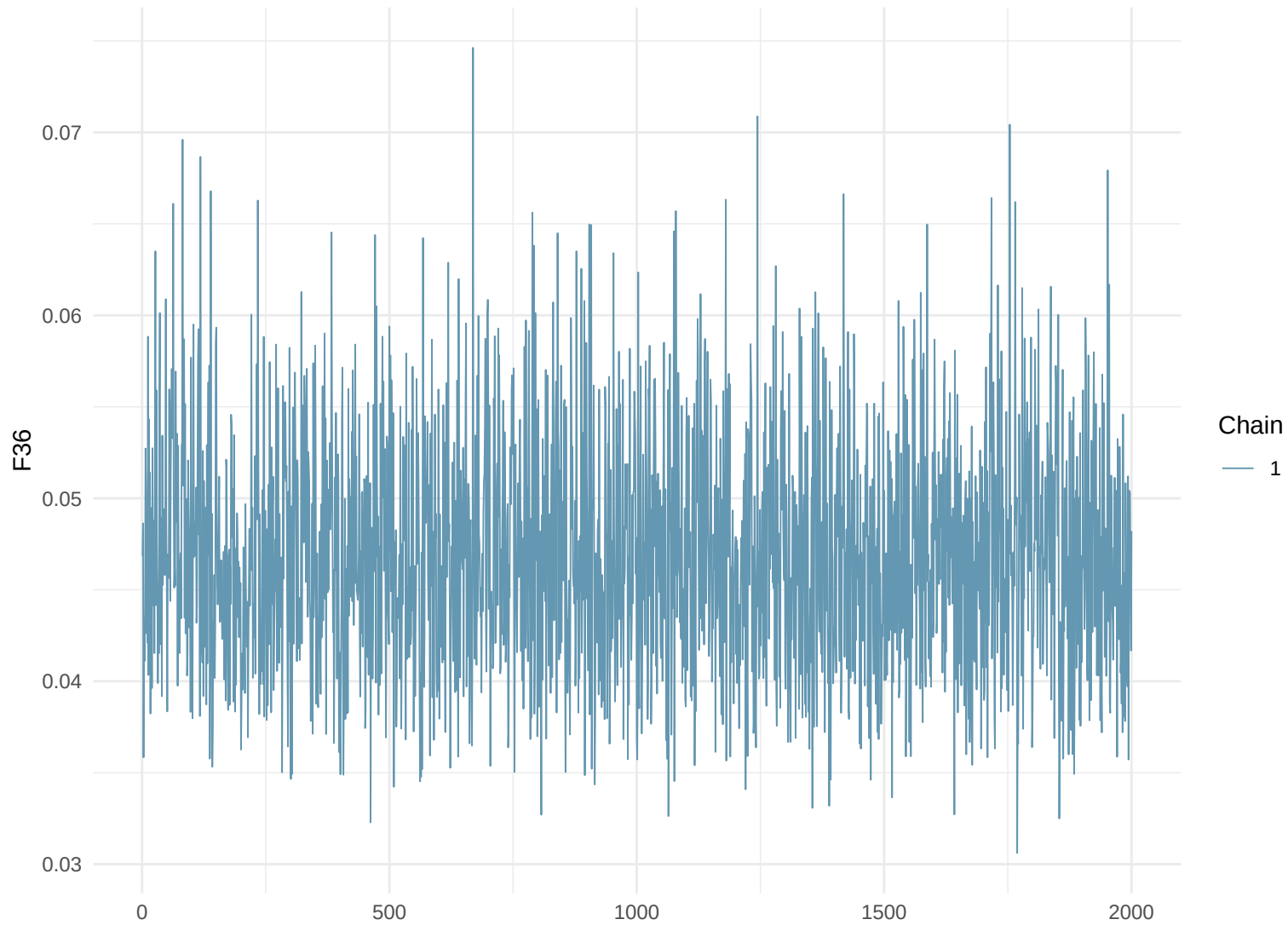
Trace Plot: F36
