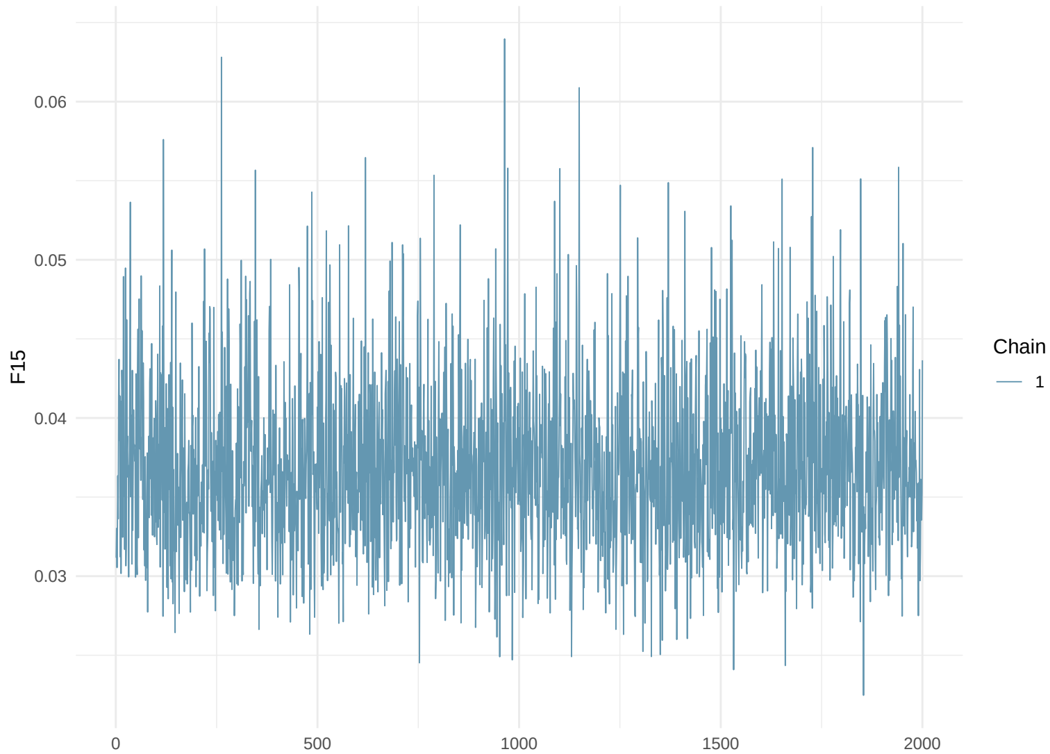
Trace Plot: F15
