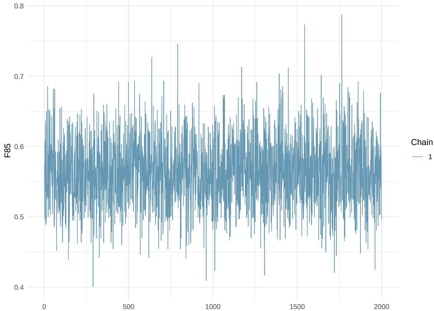
Trace Plot: F85
