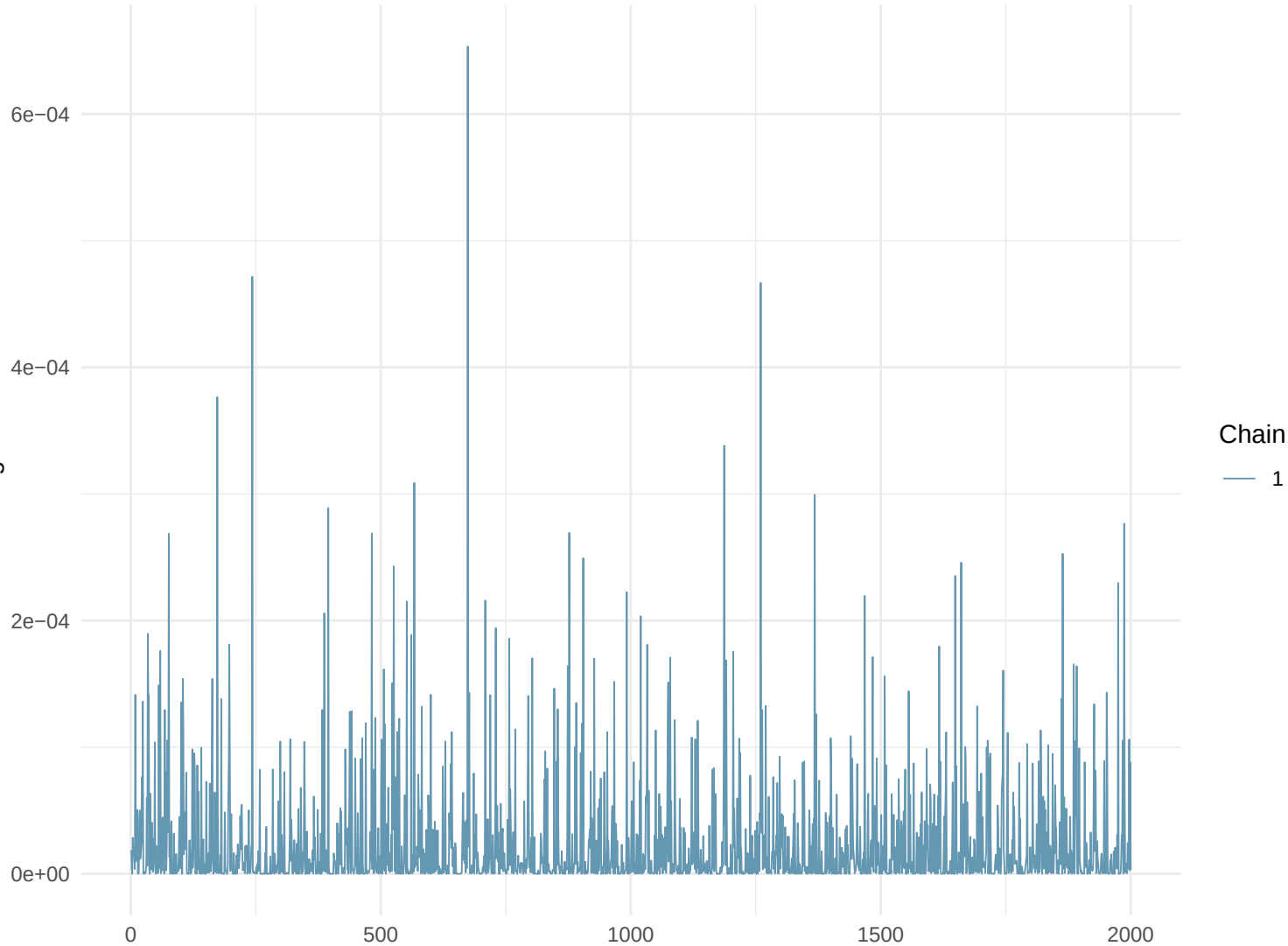
Trace Plot: Mig313
