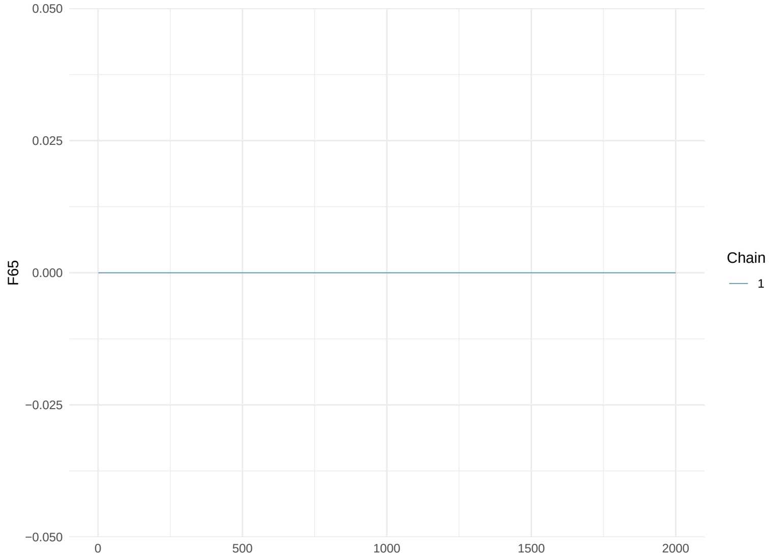
Trace Plot: F65
