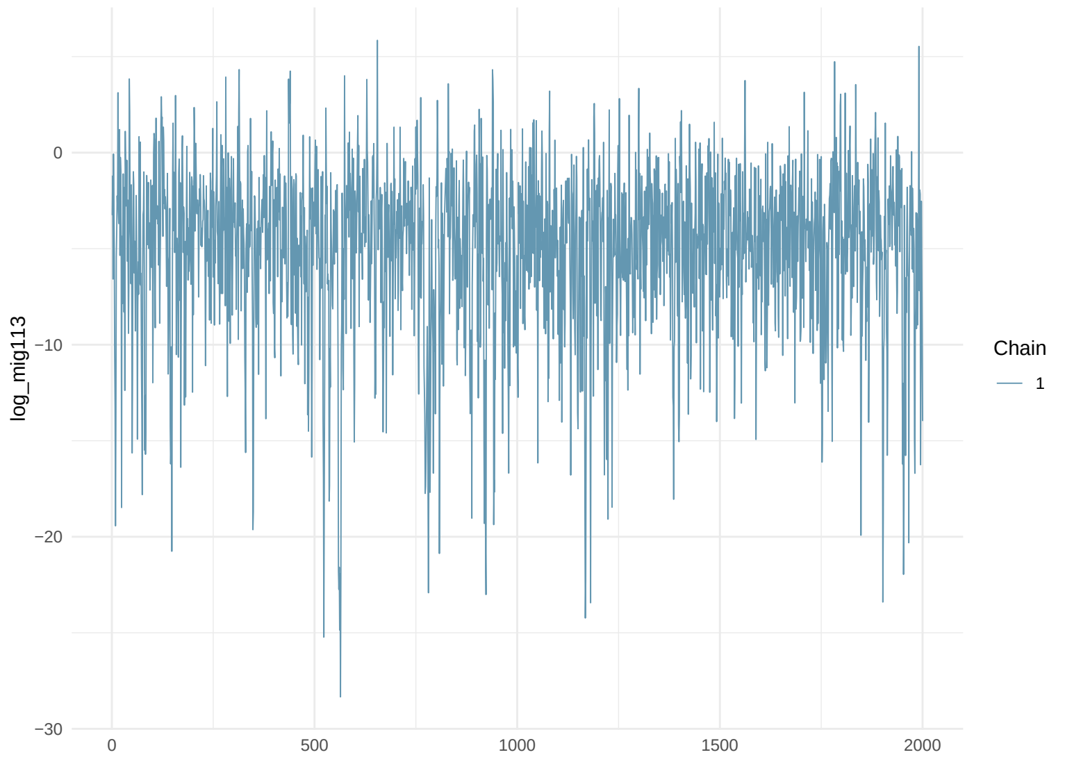
Trace Plot: log_mig113
