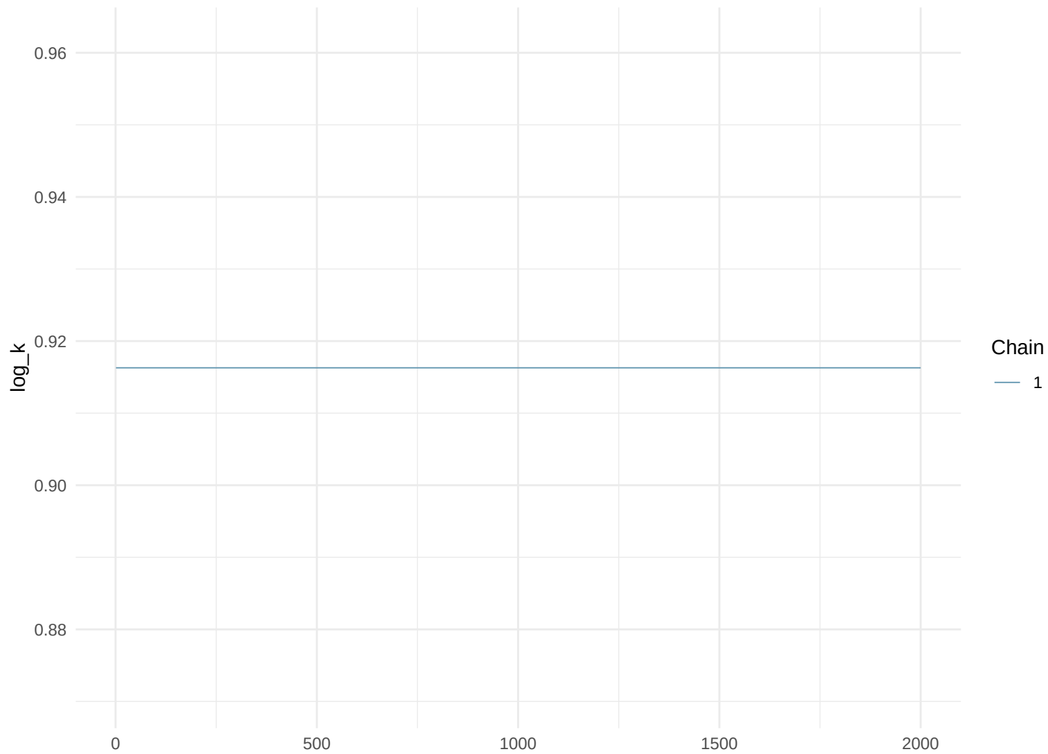
Trace Plot: log_k
