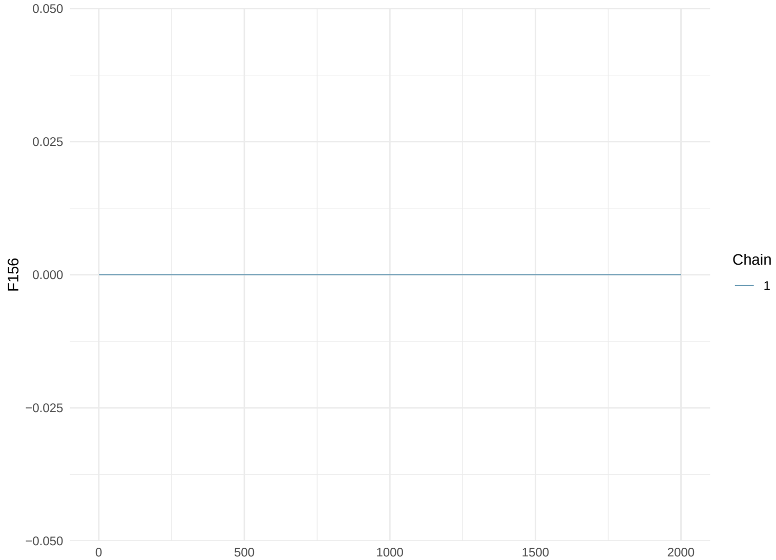
Trace Plot: F156
