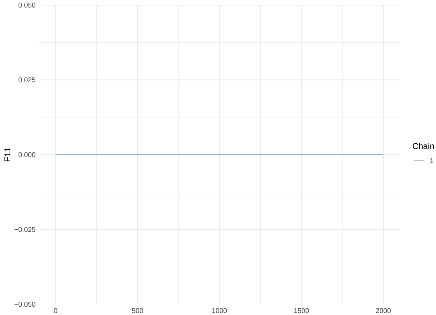
Trace Plot: F11
