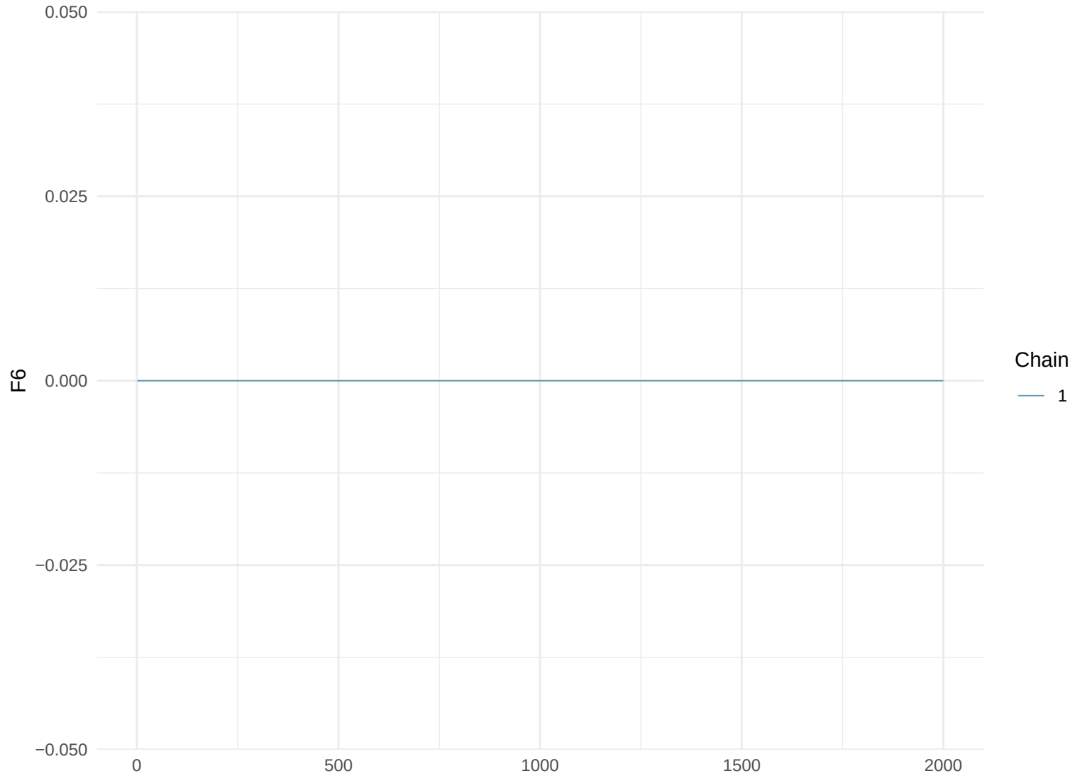
Trace Plot: F6
