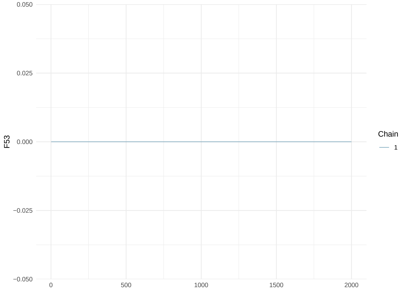
Trace Plot: F53
