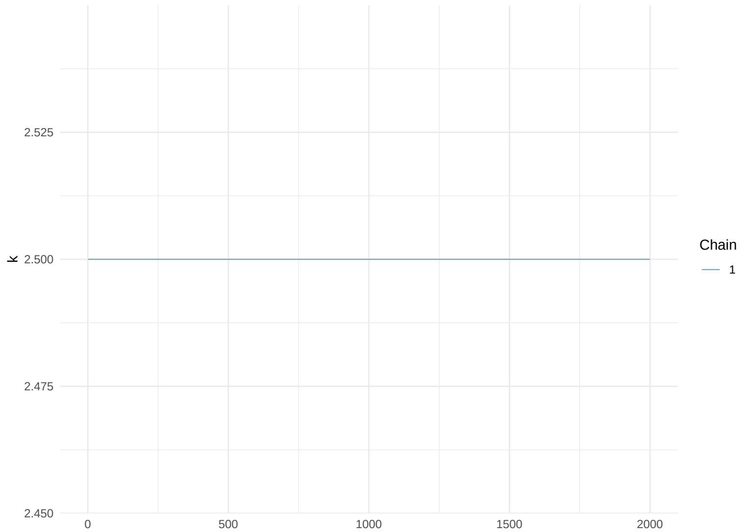
Trace Plot: k
