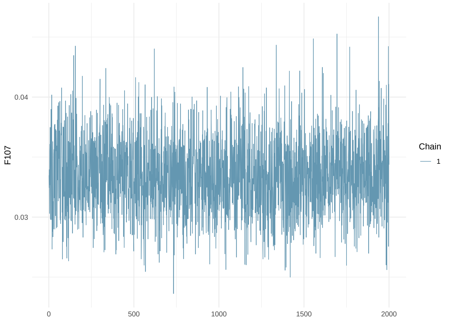
Trace Plot: F107
