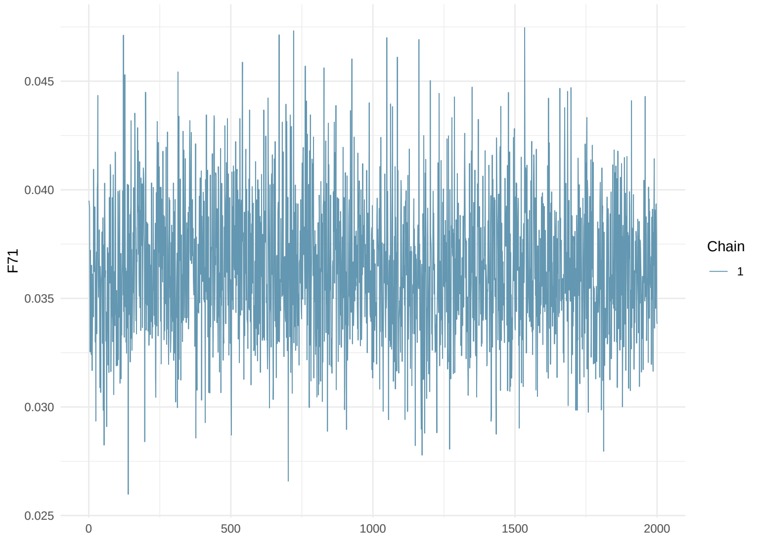
Trace Plot: F71
