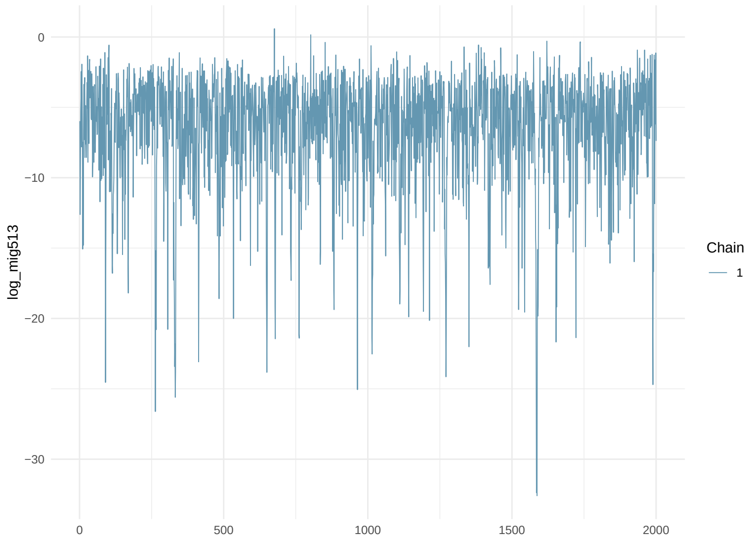
Trace Plot: log_mig513
