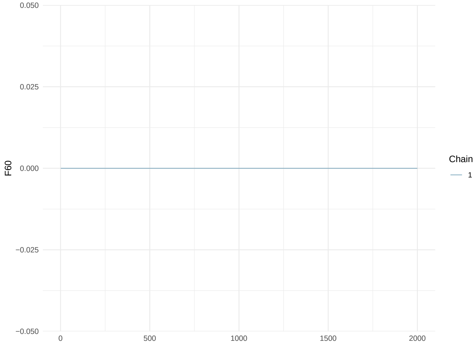
Trace Plot: F60
