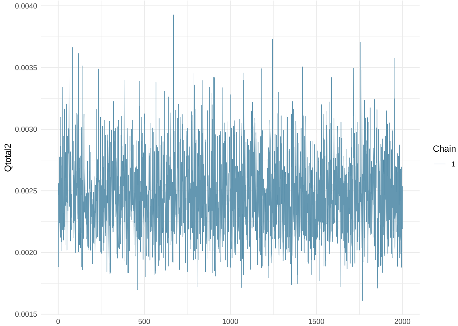
Trace Plot: Qtotal2
