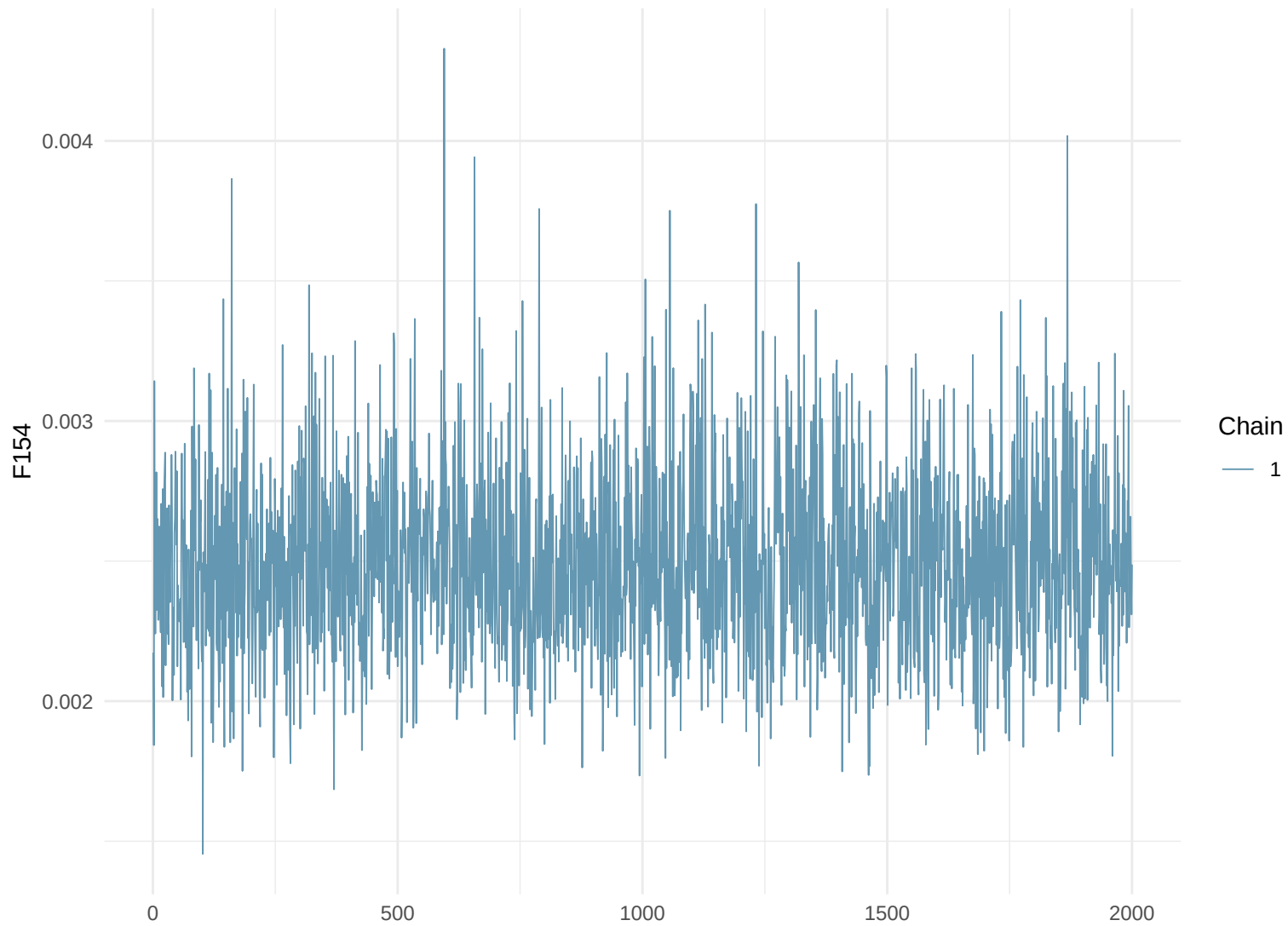
Trace Plot: F154
