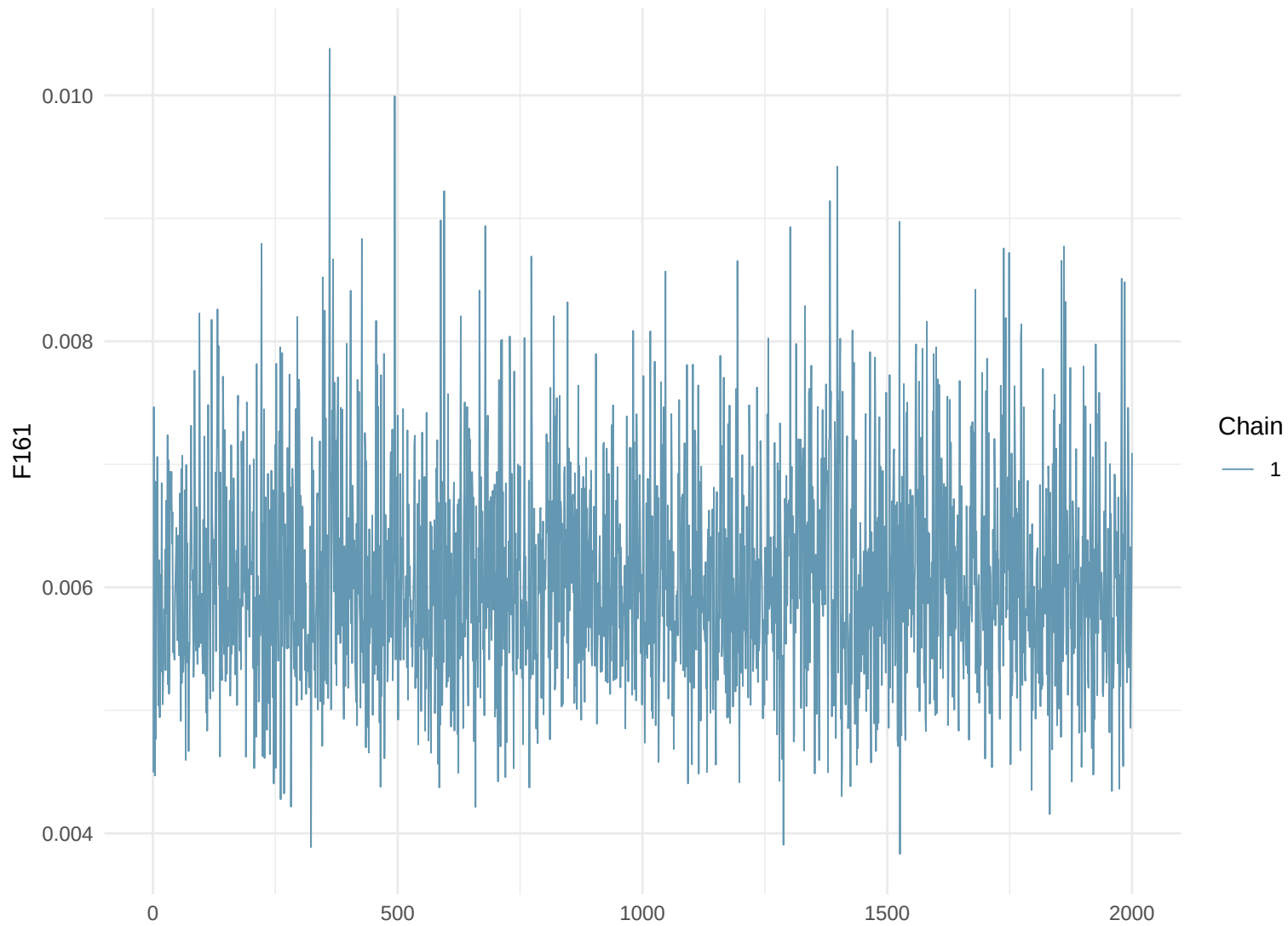
Trace Plot: F161
