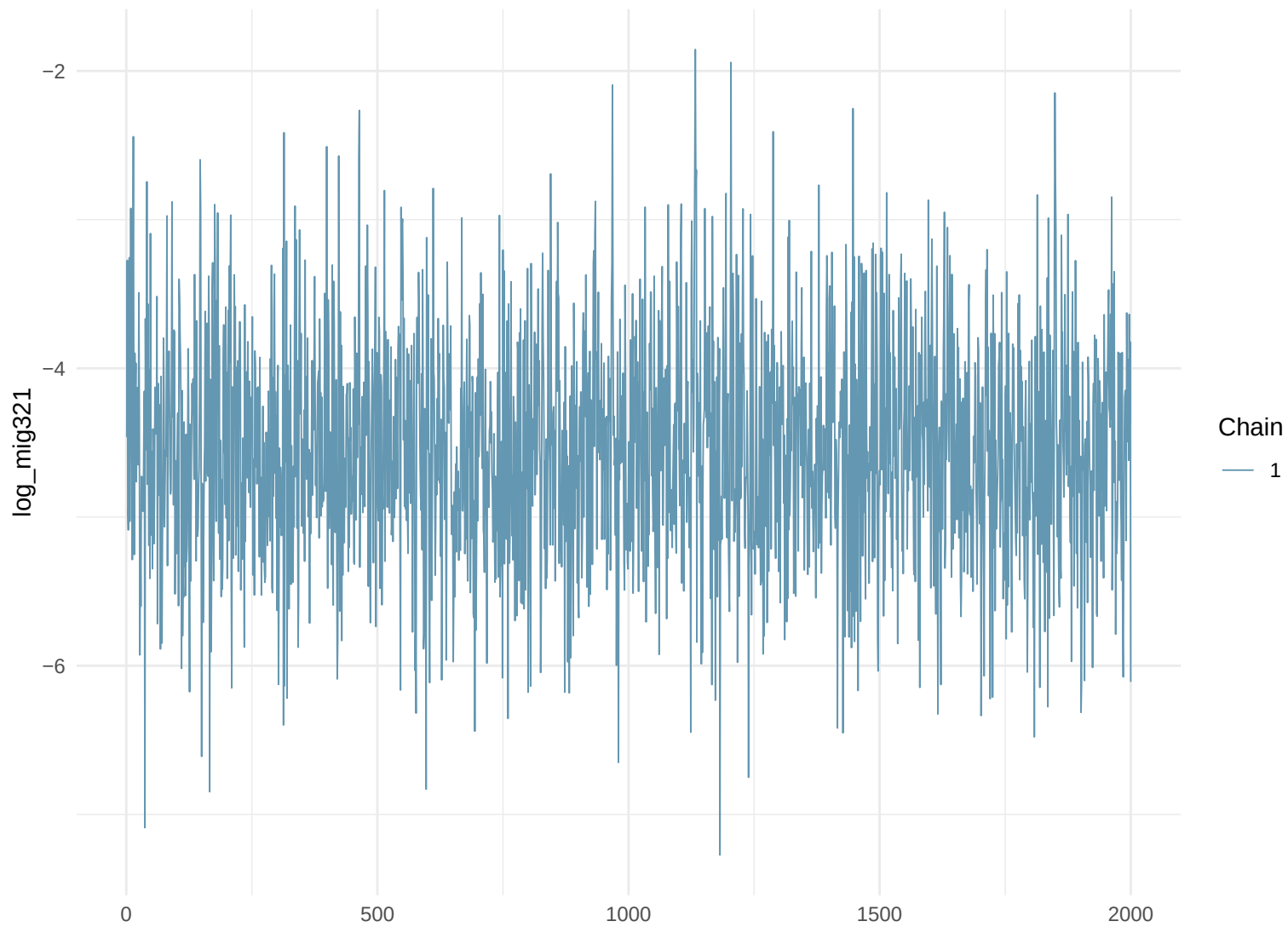
Trace Plot: log_mig321
