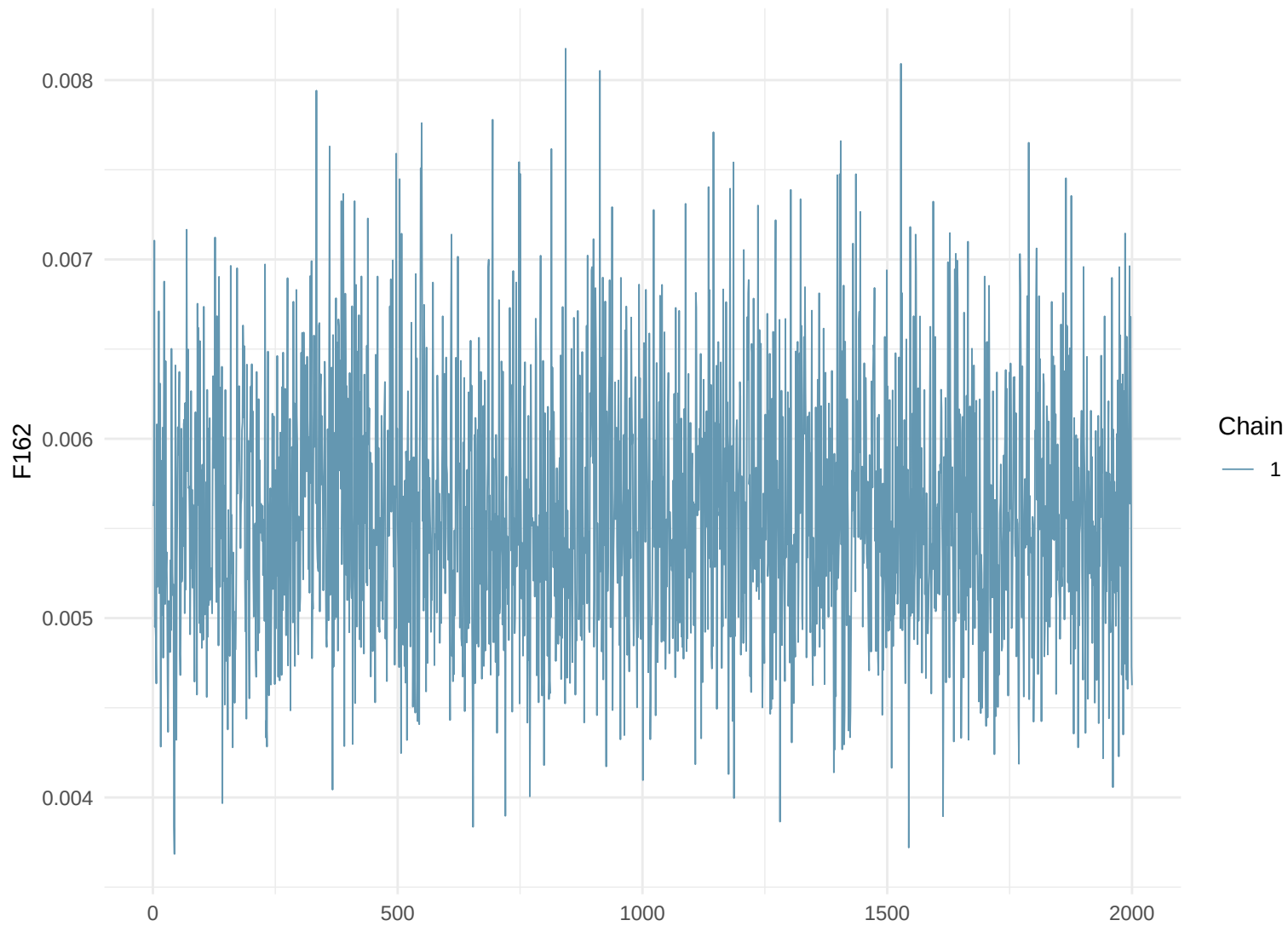
Trace Plot: F162
