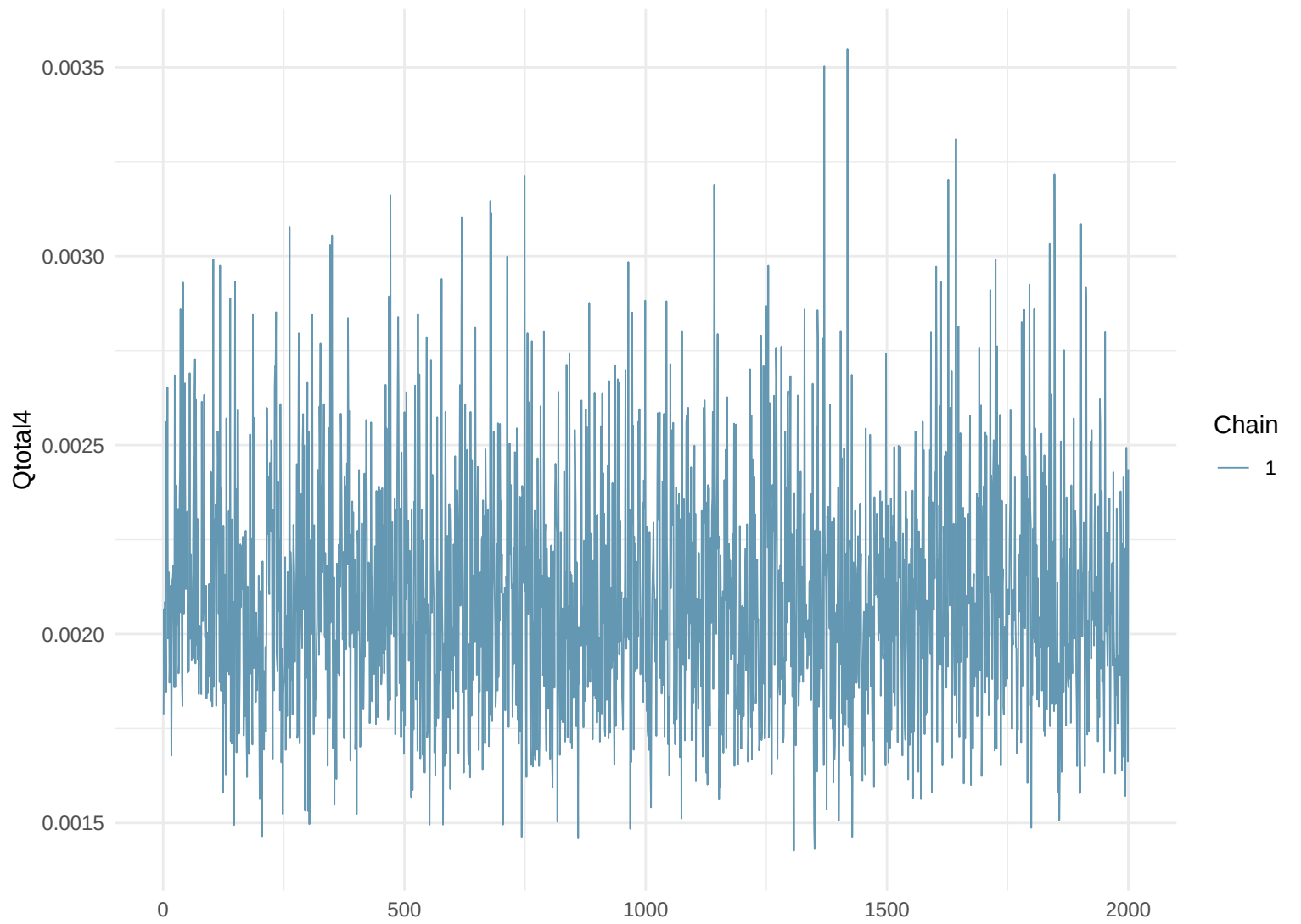
Trace Plot: Qtotal4
