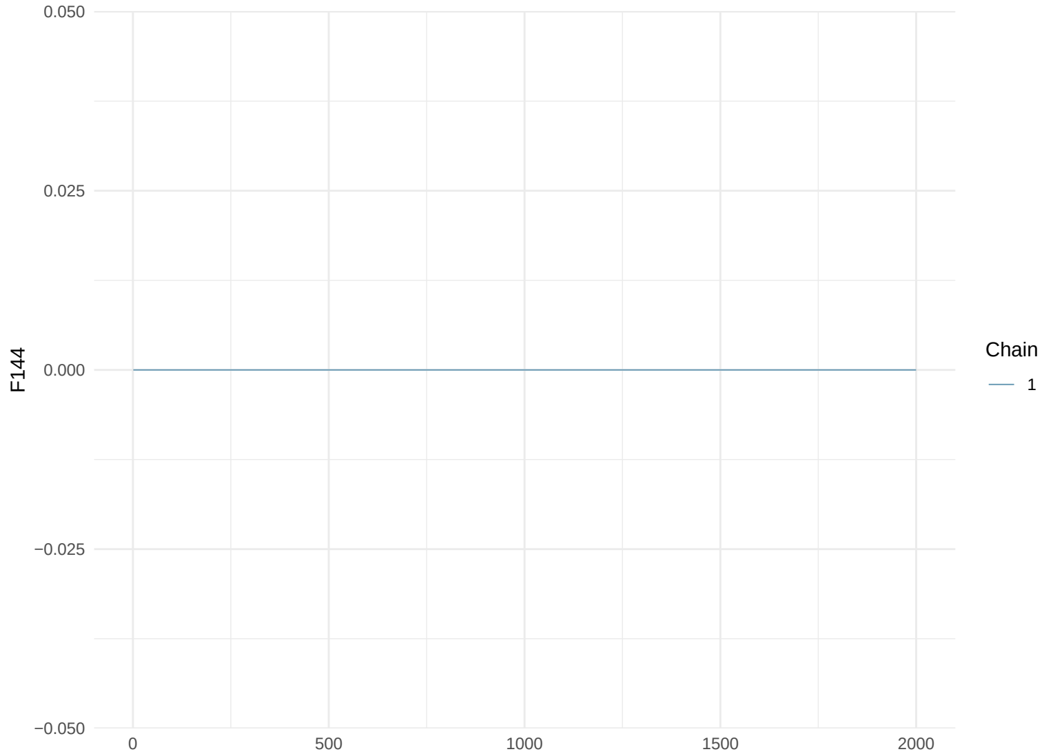
Trace Plot: F144
