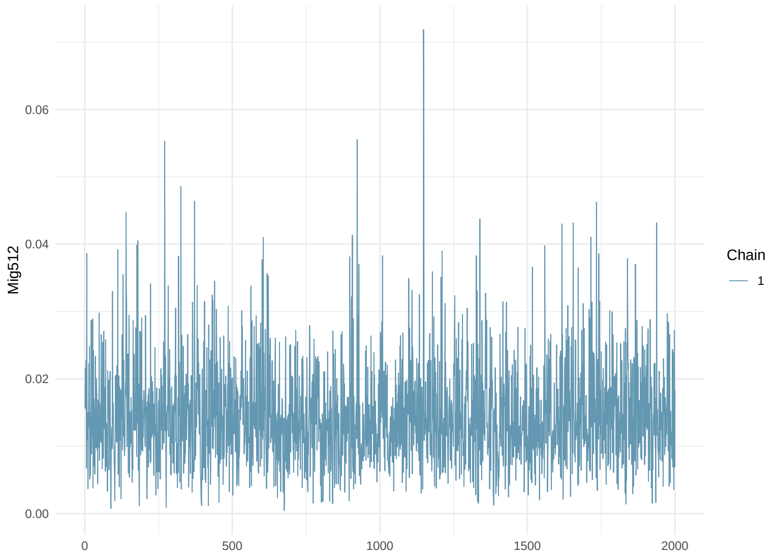
Trace Plot: Mig512
