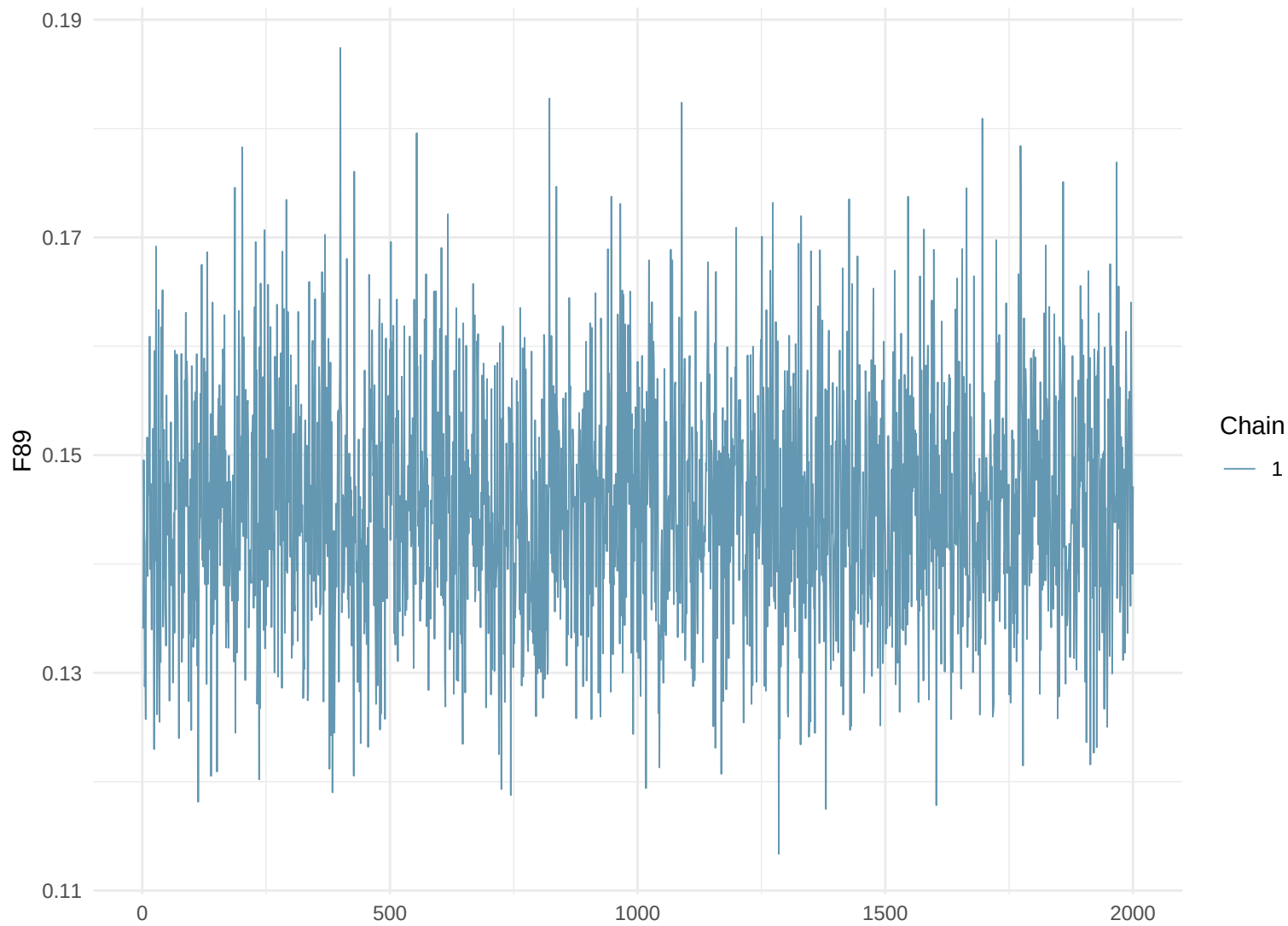
Trace Plot: F89
