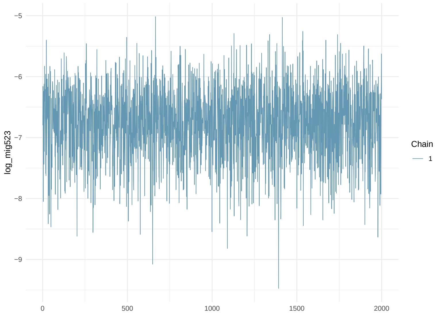
Trace Plot: log_mig523
