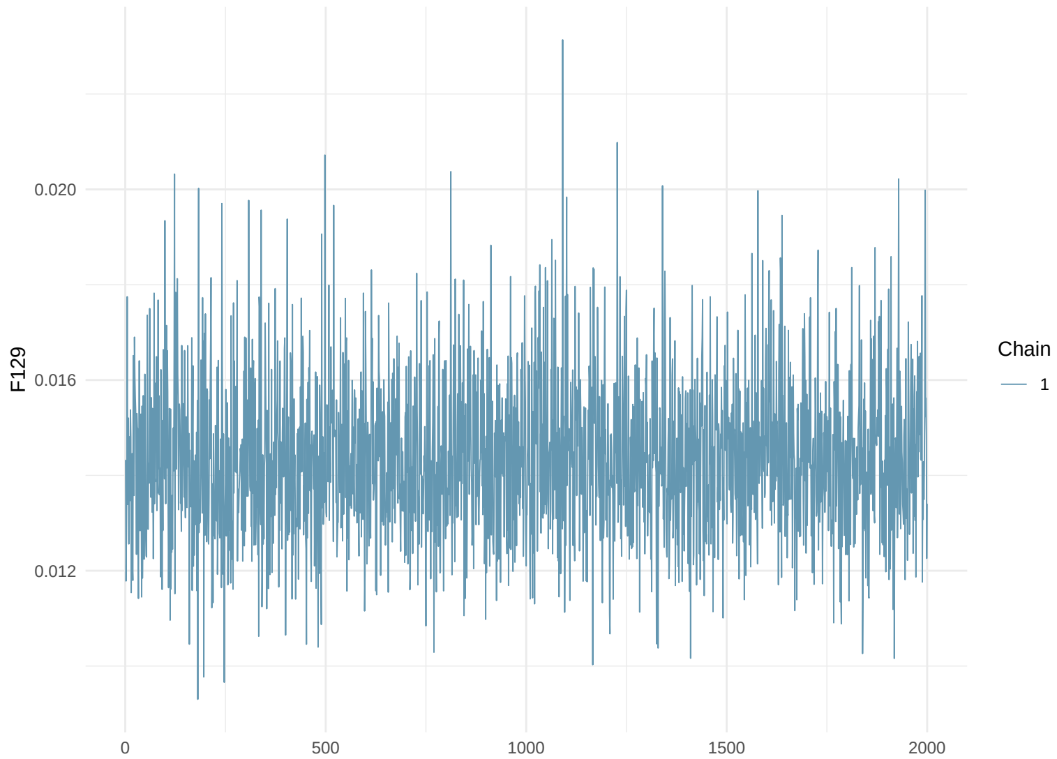
Trace Plot: F129
