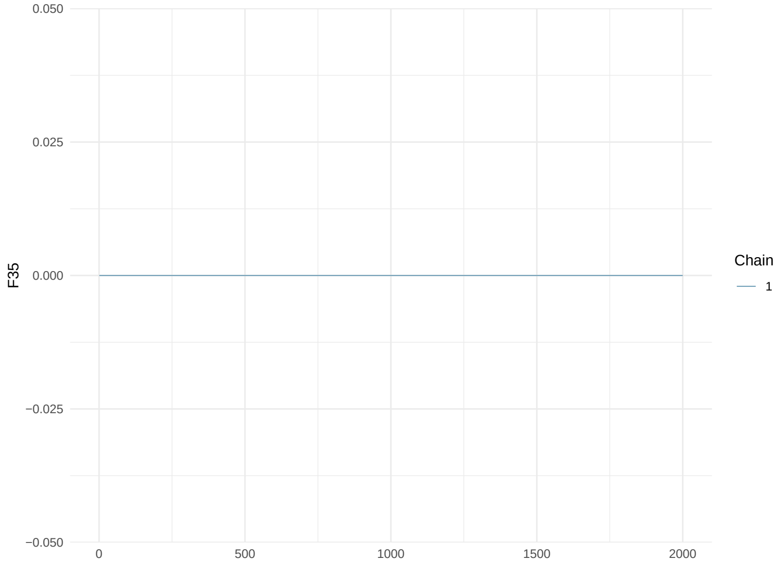
Trace Plot: F35
