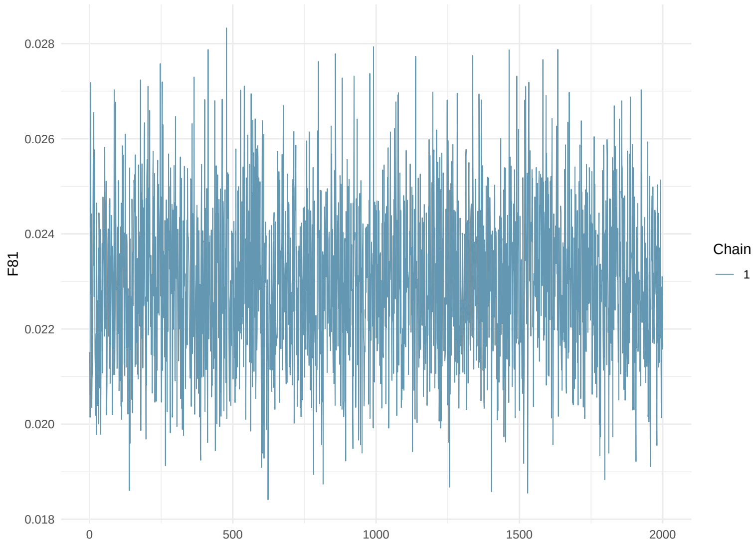
Trace Plot: F81
