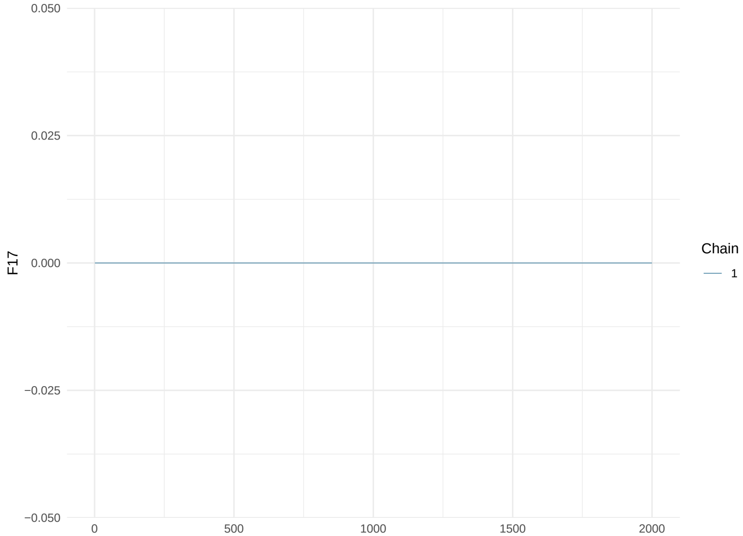
Trace Plot: F17
