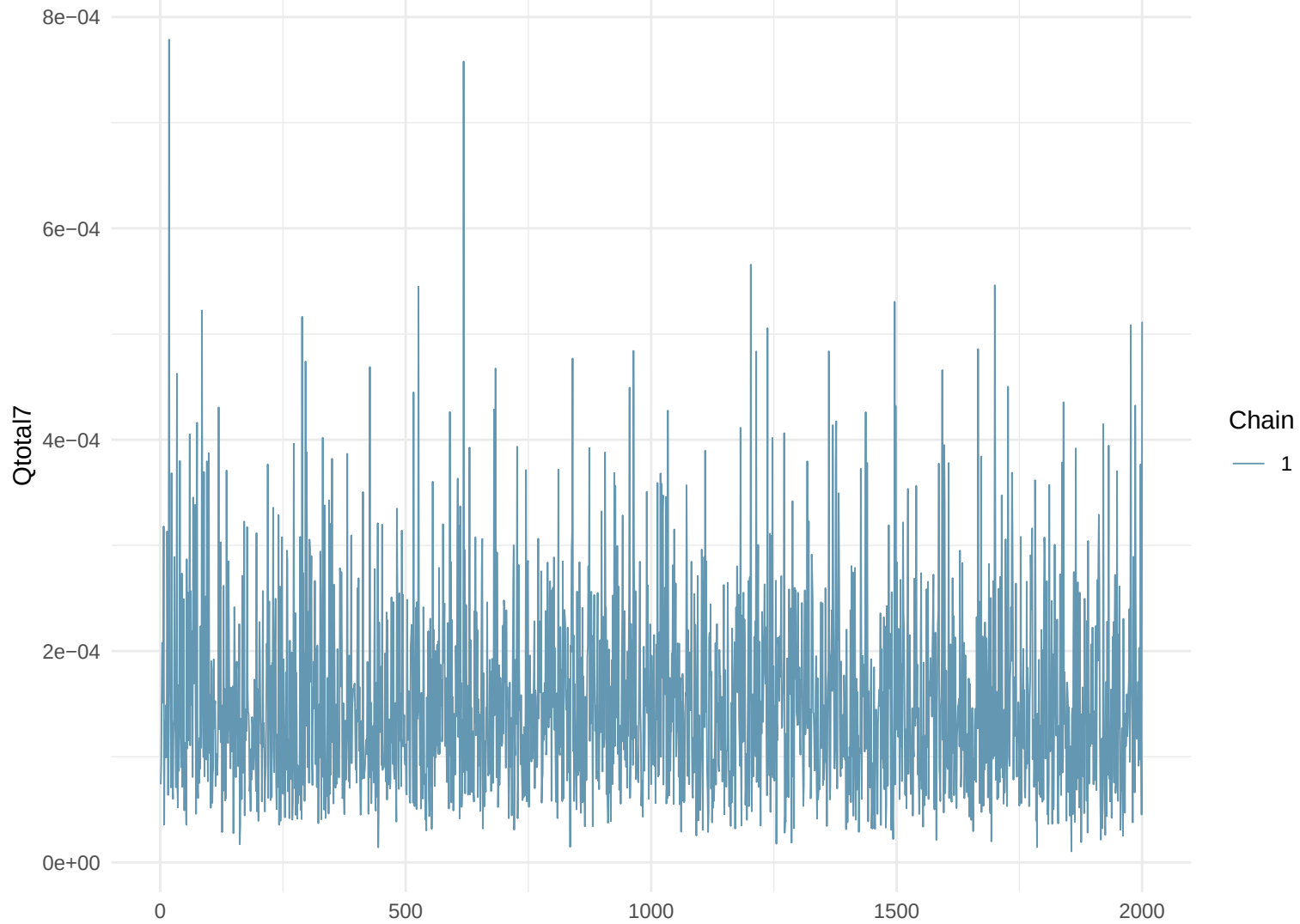
Trace Plot: Qtotal7
