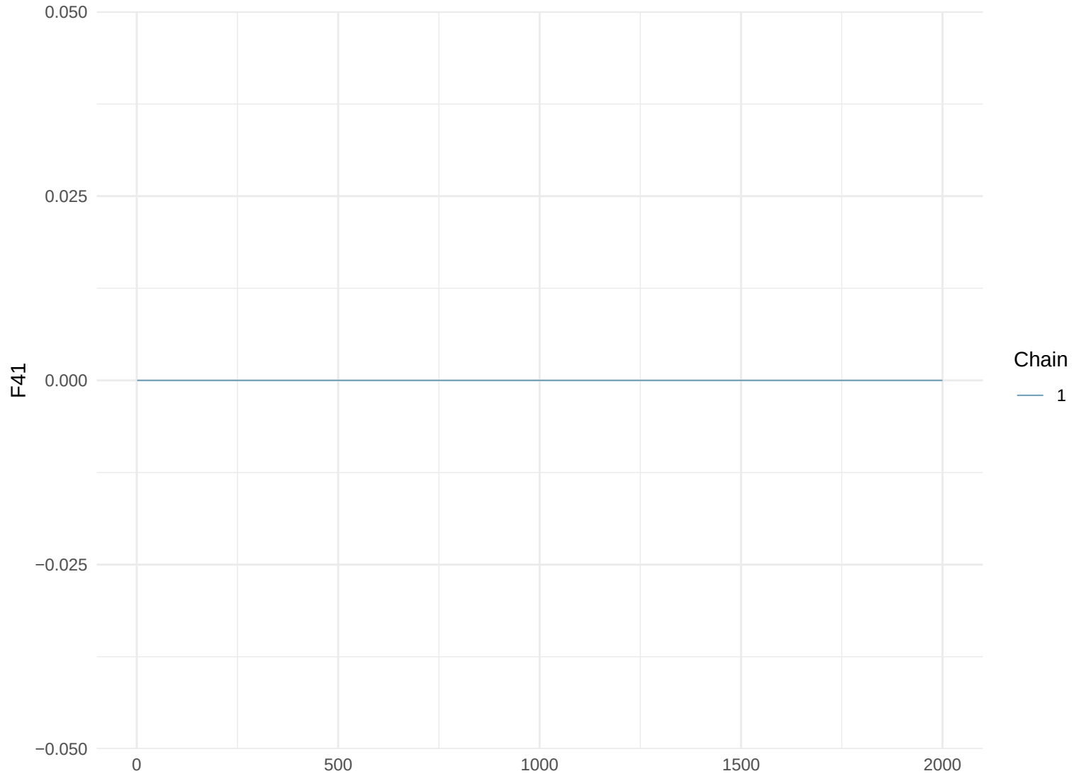
Trace Plot: F41
