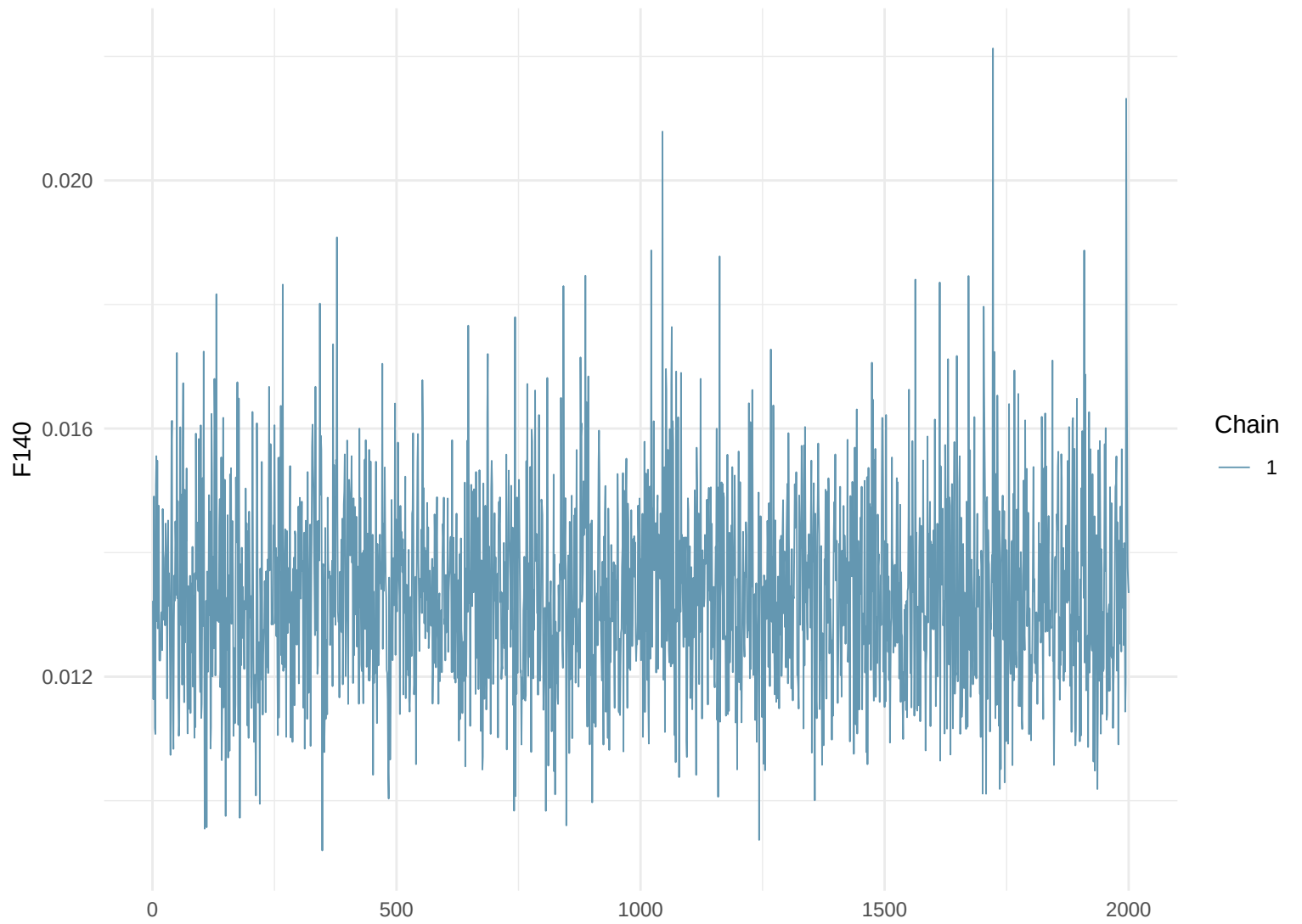
Trace Plot: F140
