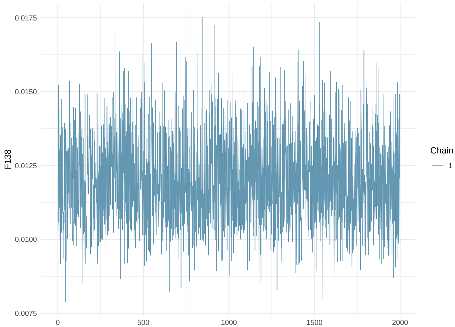
Trace Plot: F138
