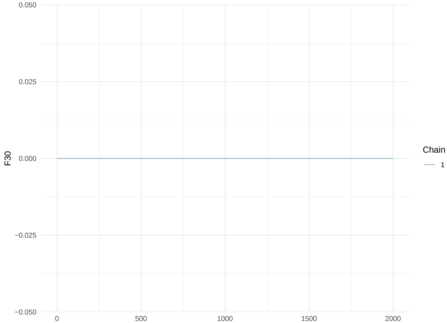
Trace Plot: F30
