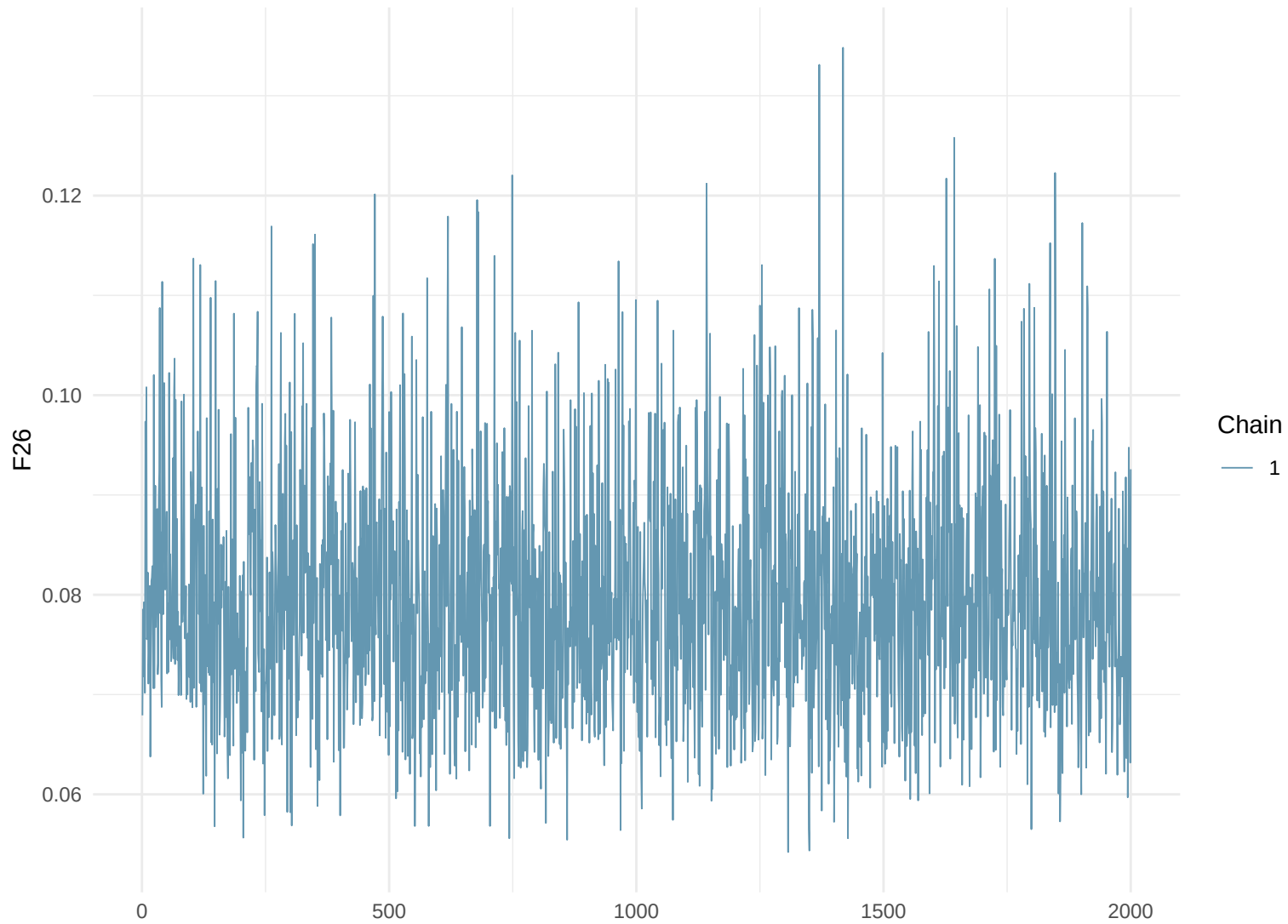
Trace Plot: F26
