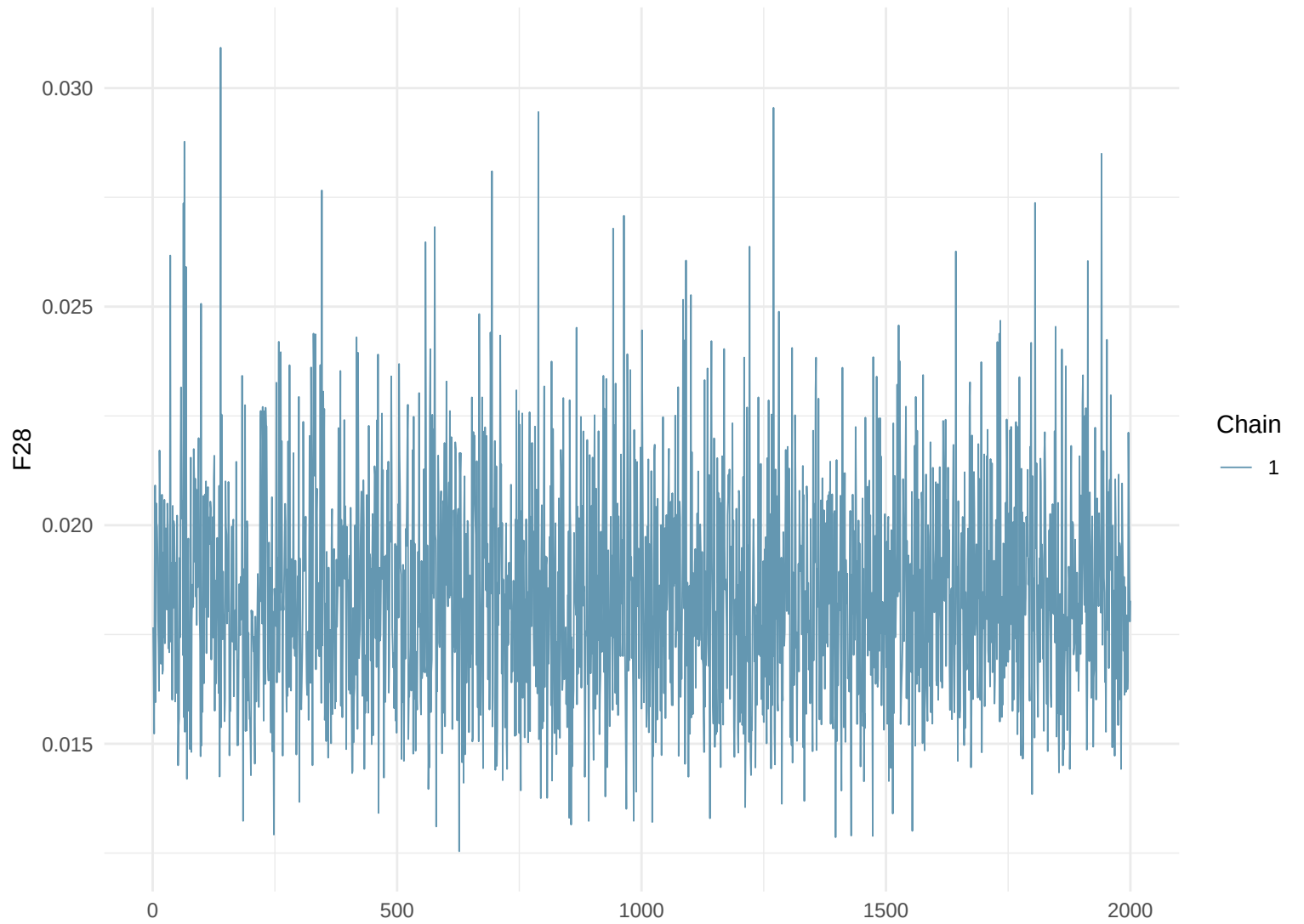
Trace Plot: F28
