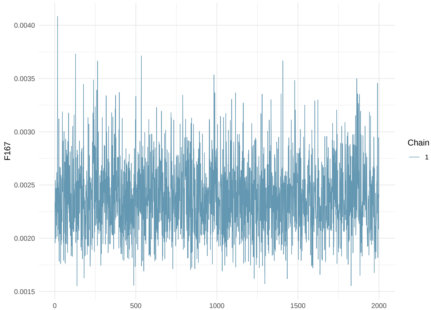
Trace Plot: F167
