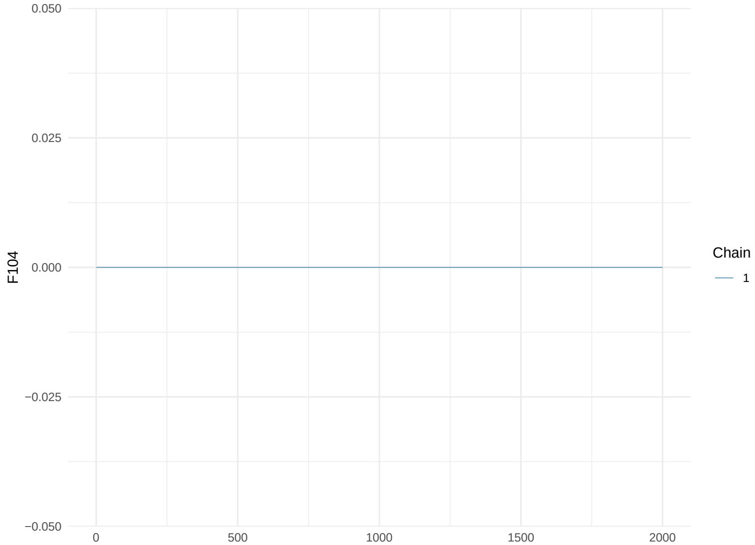
Trace Plot: F104
