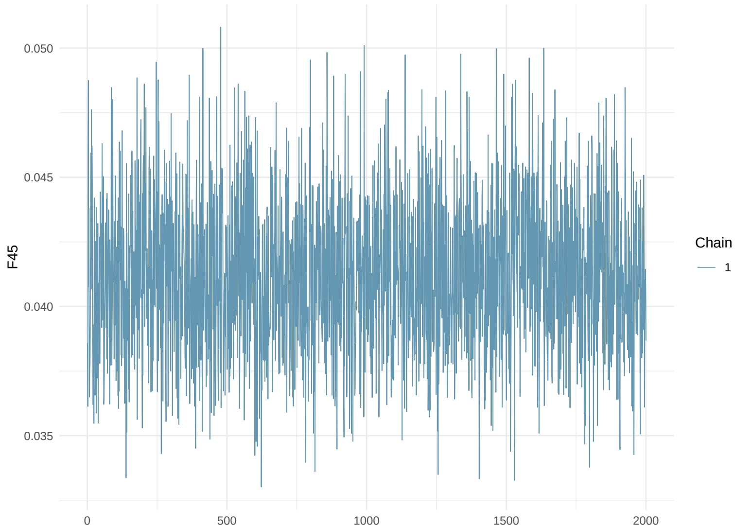
Trace Plot: F45
