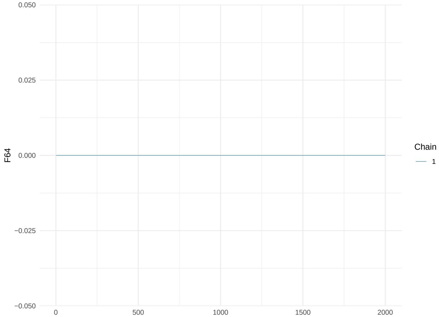
Trace Plot: F64
