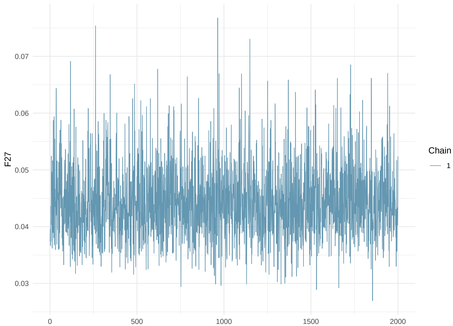
Trace Plot: F27
