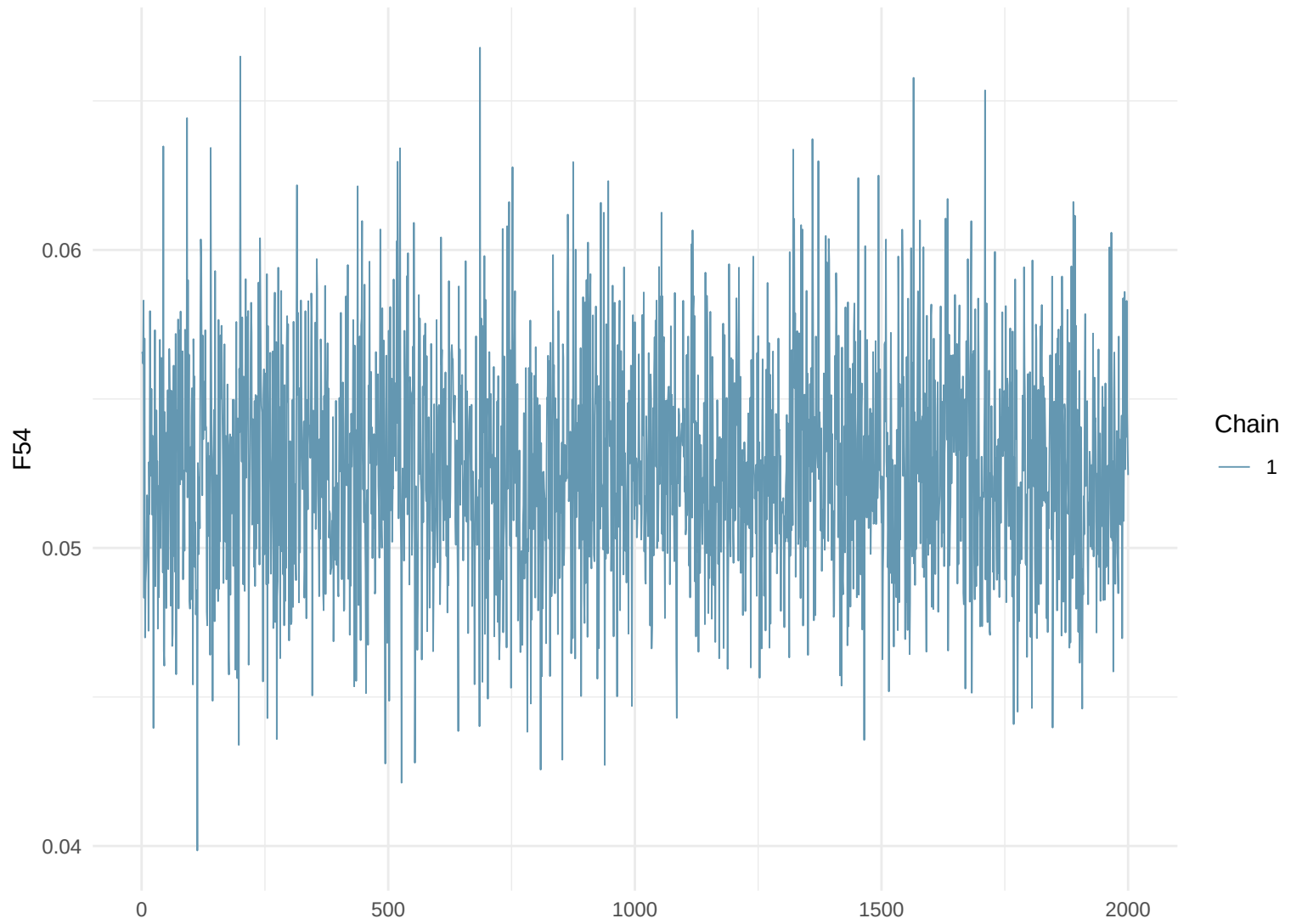
Trace Plot: F54
