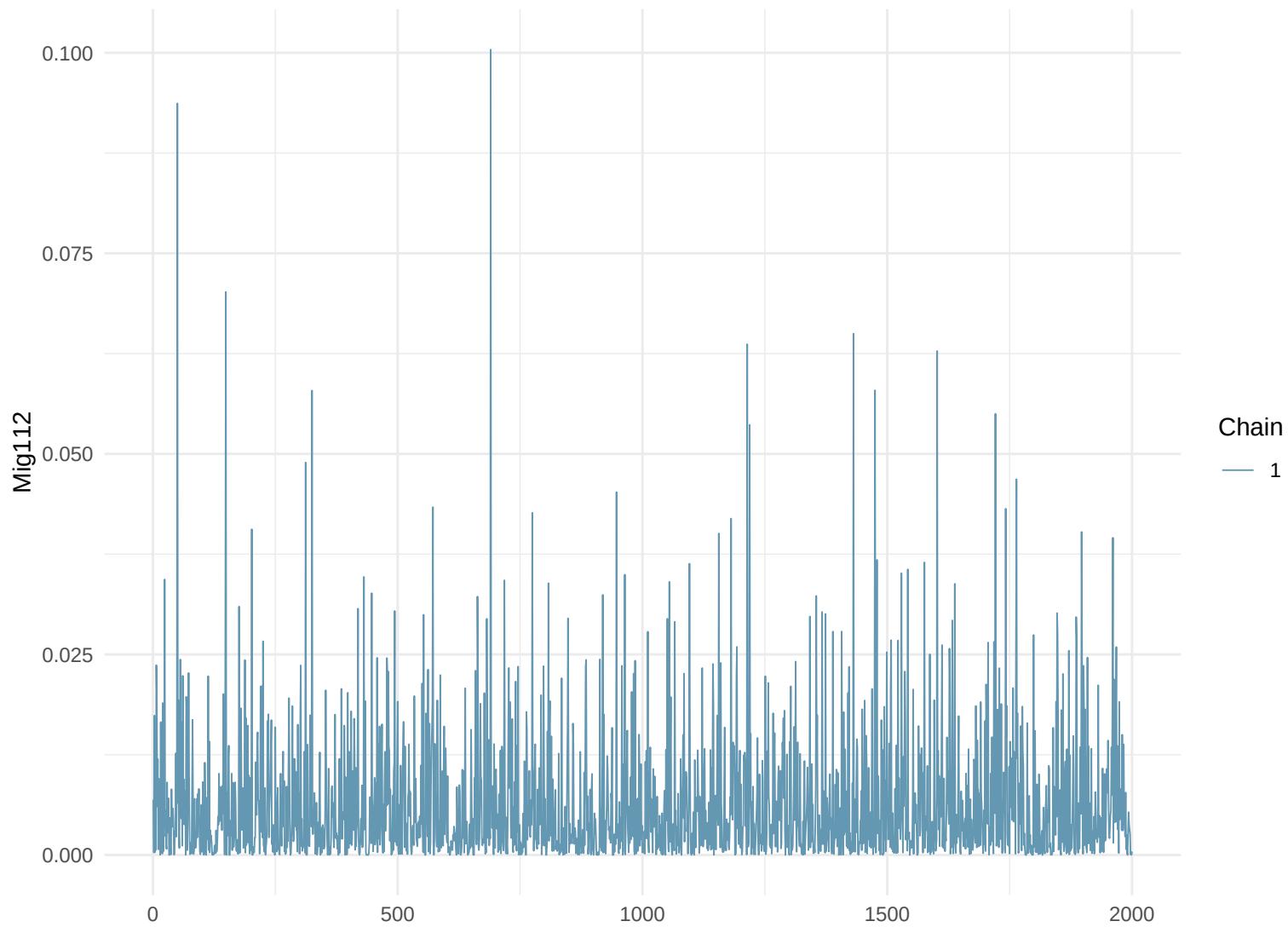
Trace Plot: Mig112
