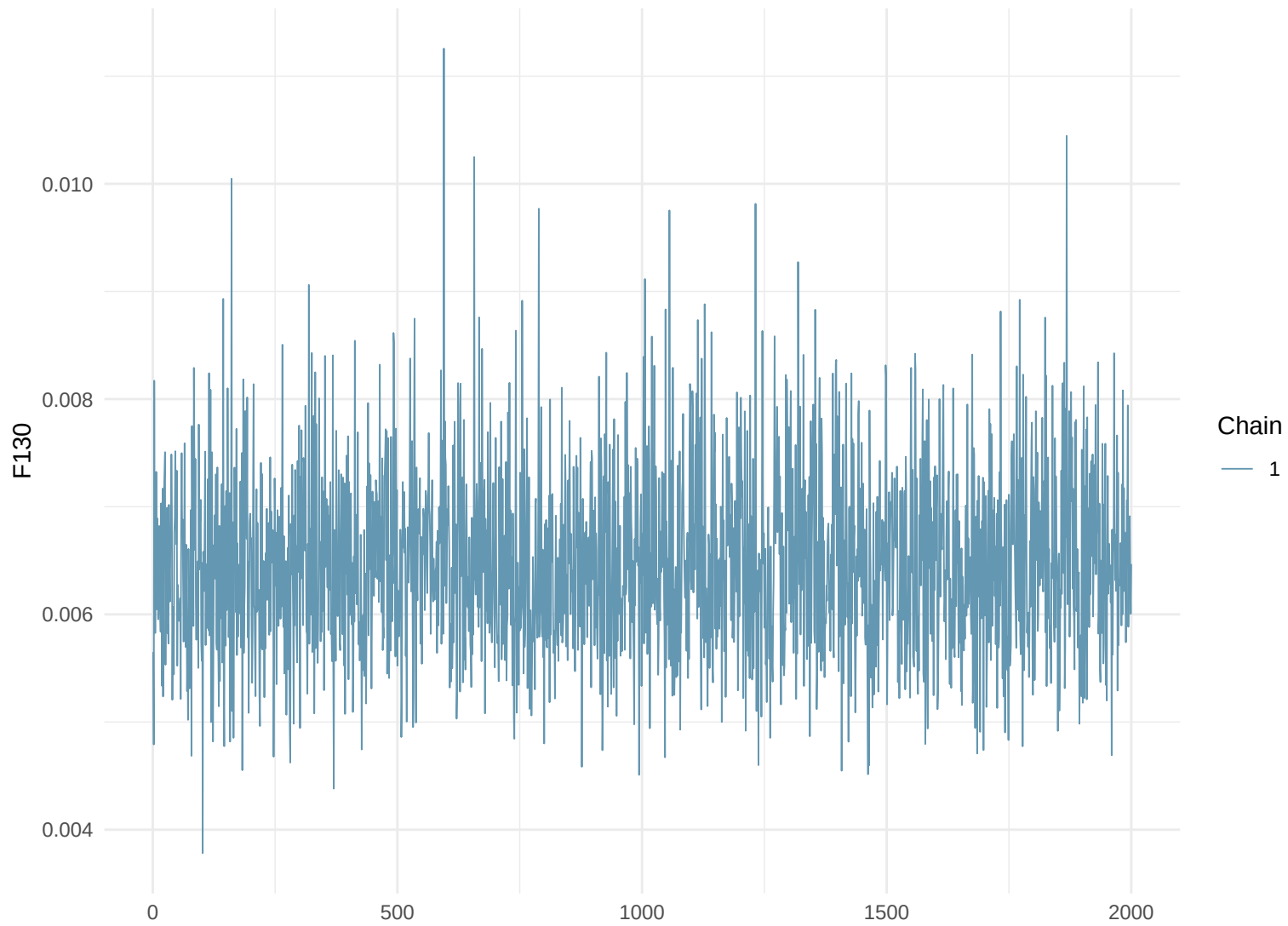
Trace Plot: F130
