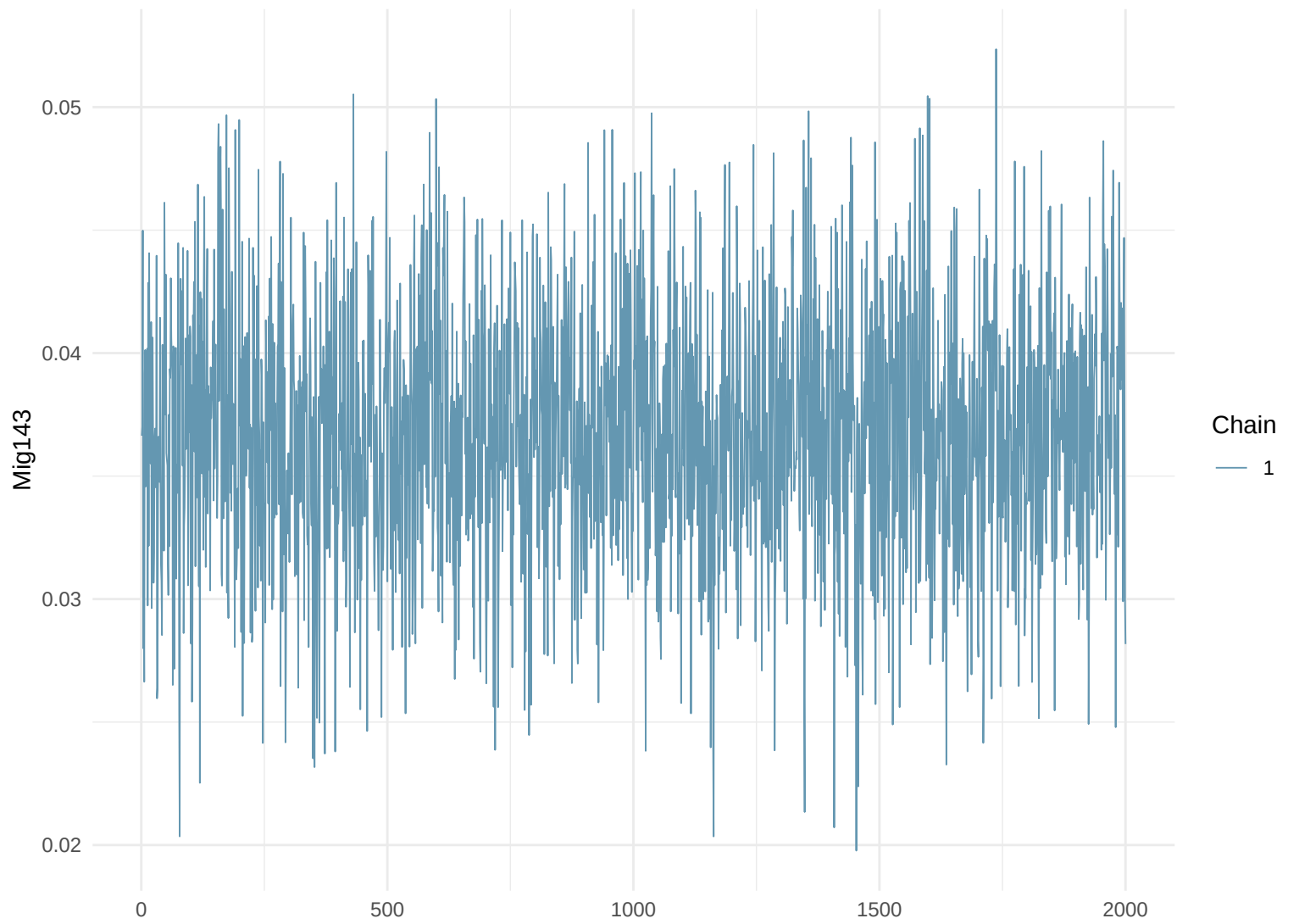
Trace Plot: Mig143
