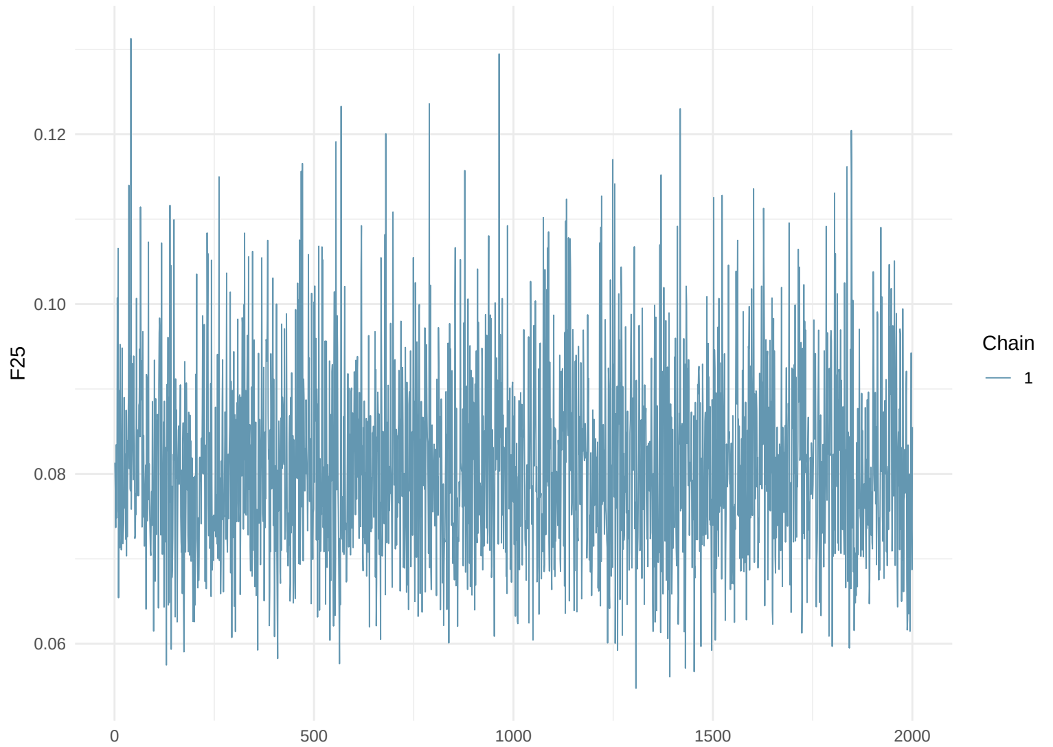
Trace Plot: F25
