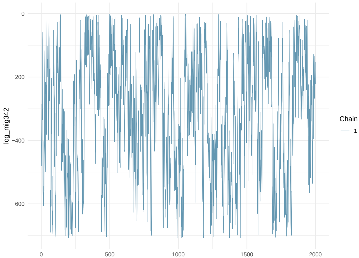
Trace Plot: log_mig342
