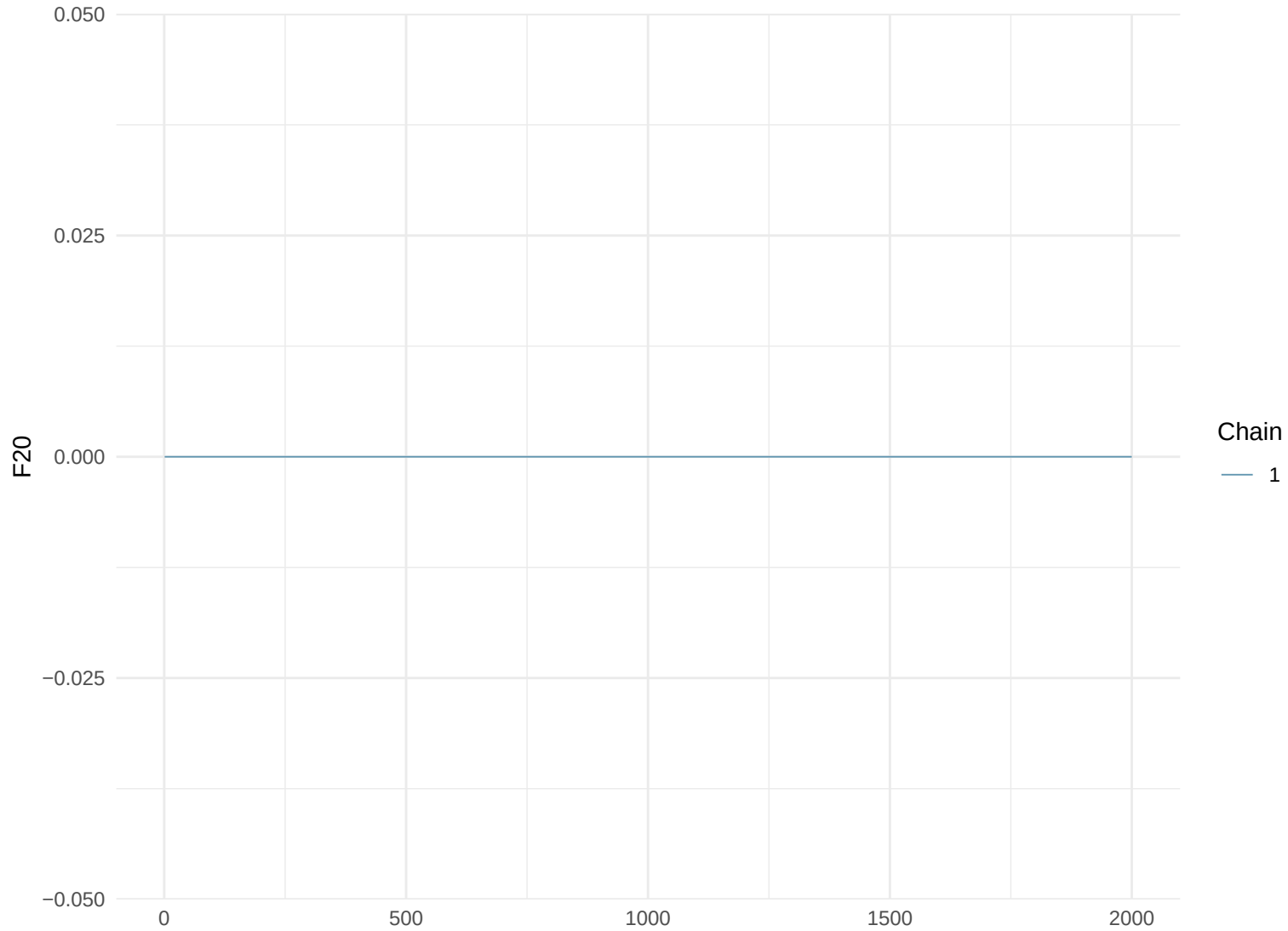
Trace Plot: F20
