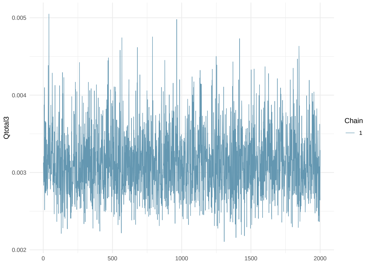
Trace Plot: Qtotal3
