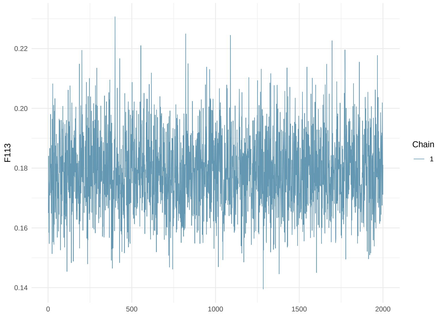
Trace Plot: F113
