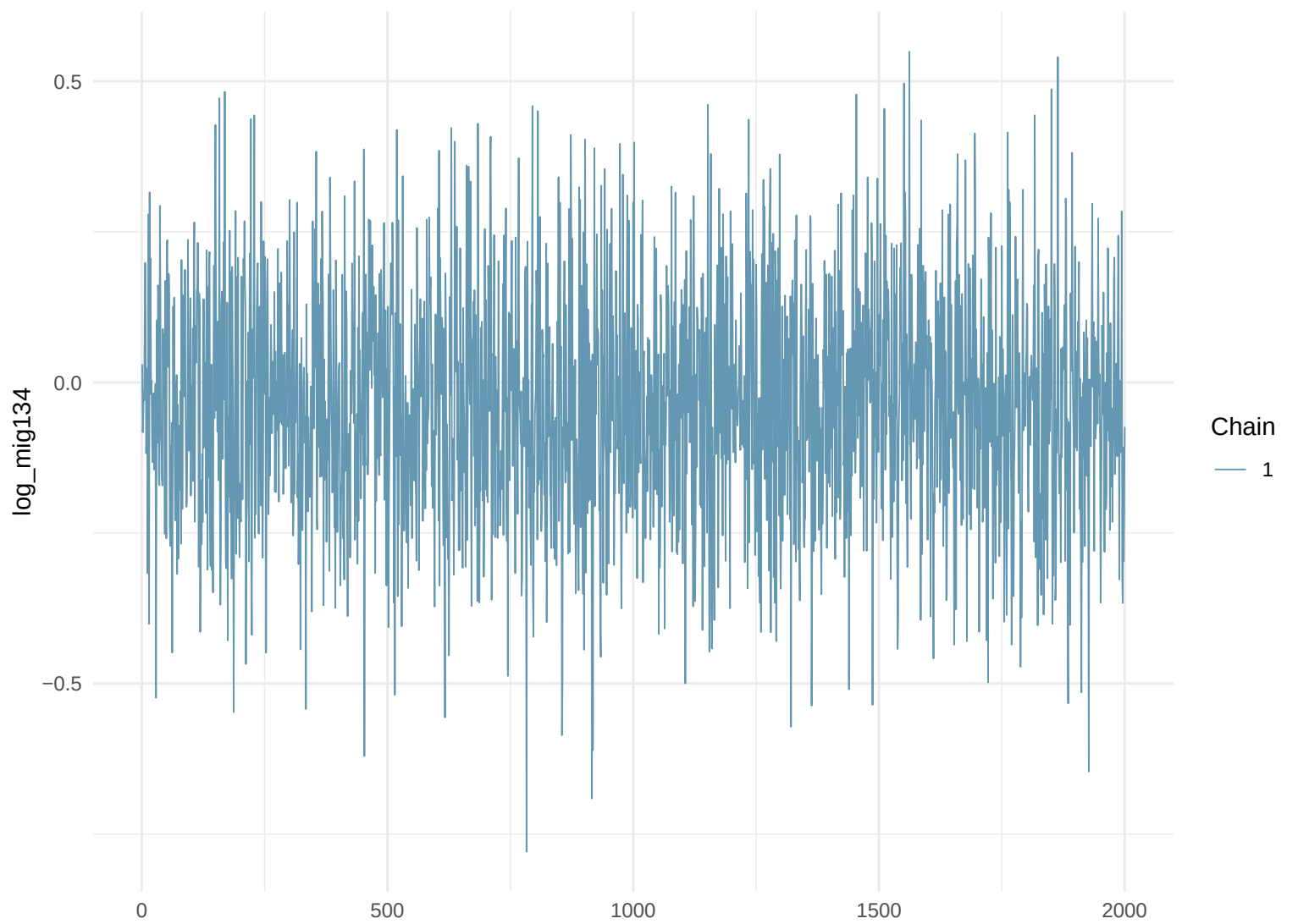
Trace Plot: log_mig134
