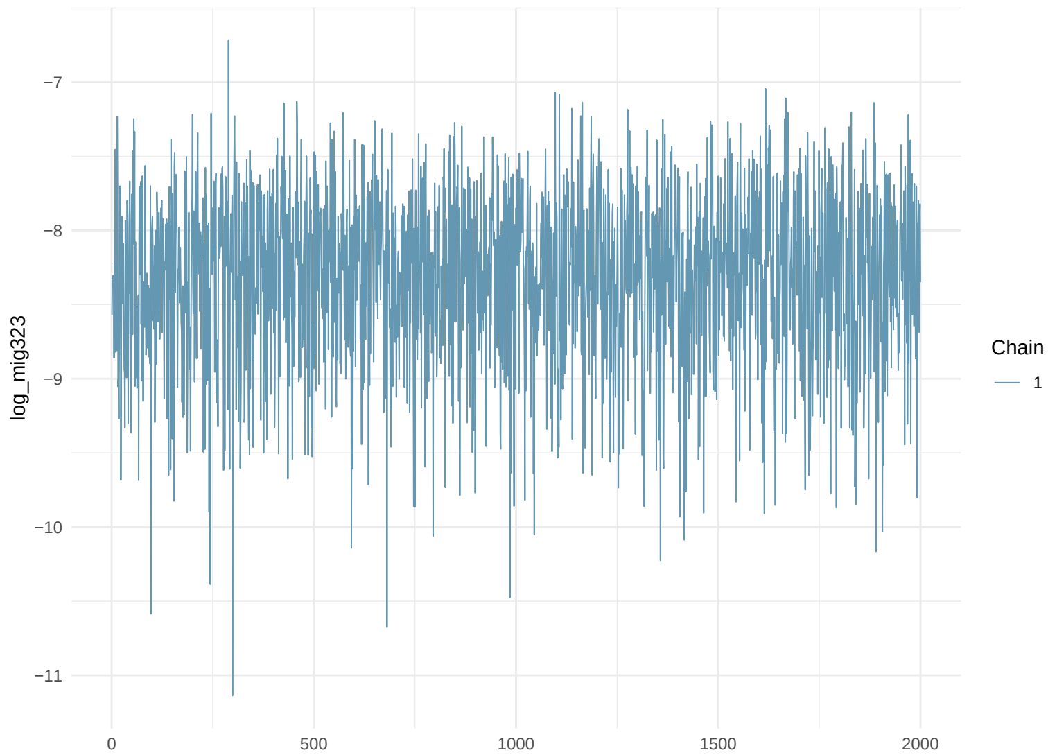
Trace Plot: log_mig323
