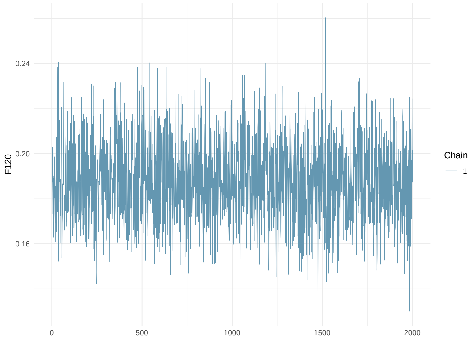
Trace Plot: F120
