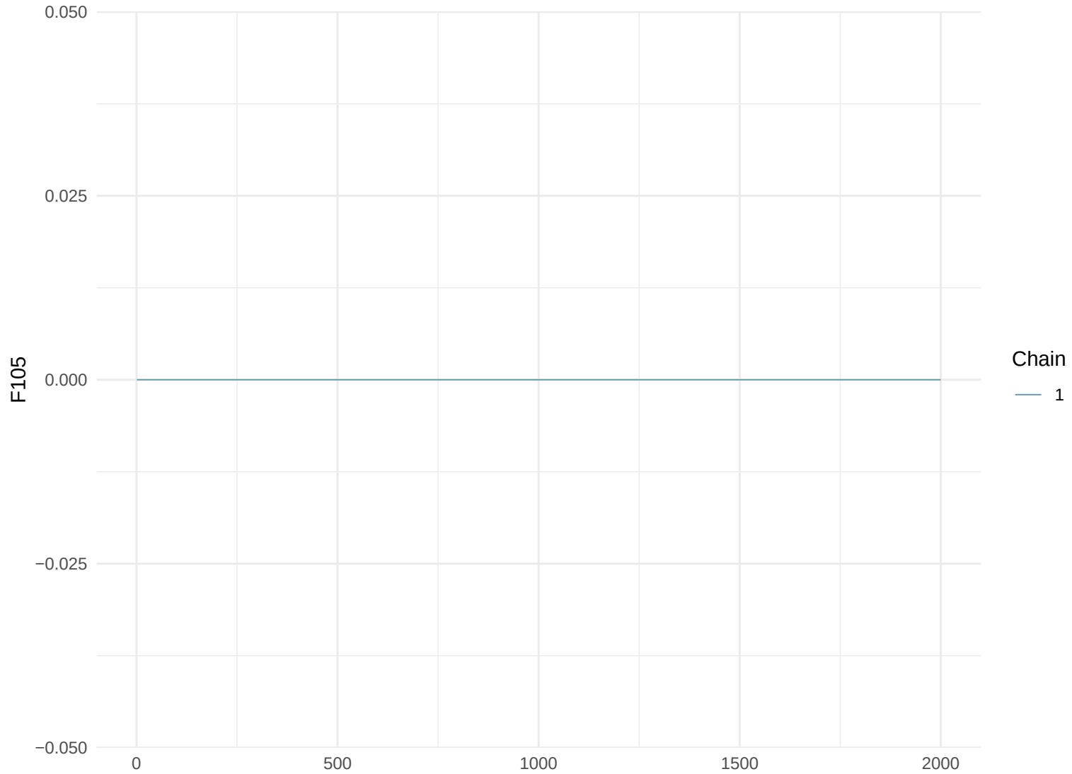
Trace Plot: F105
