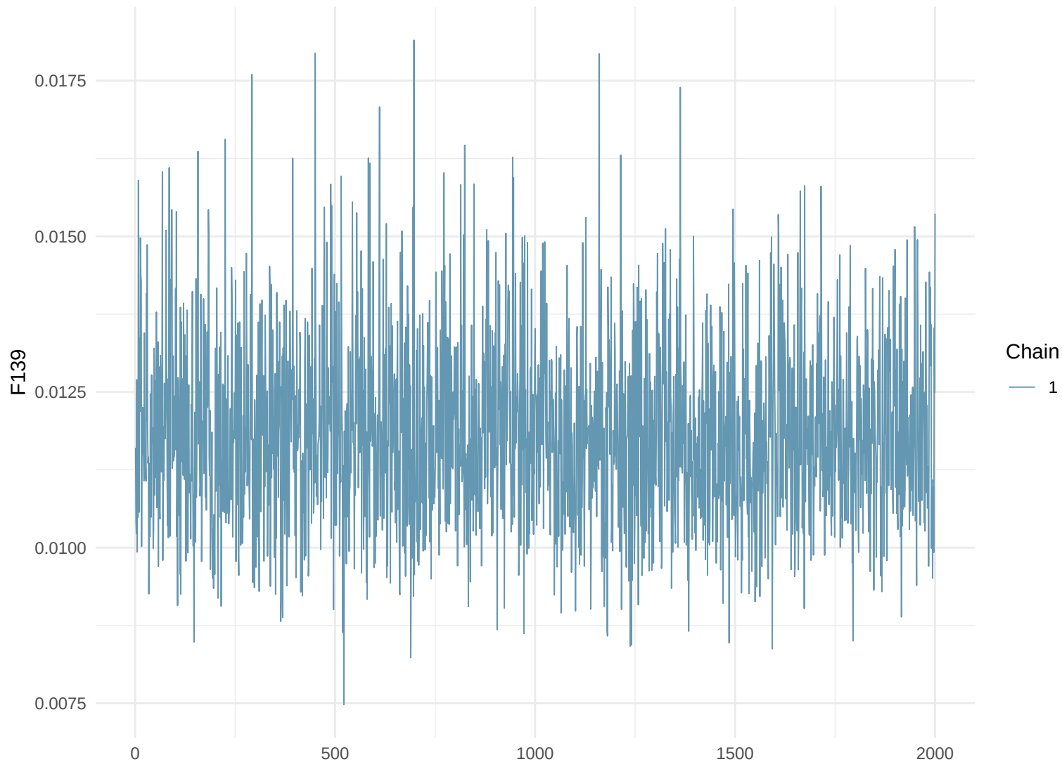
Trace Plot: F139
