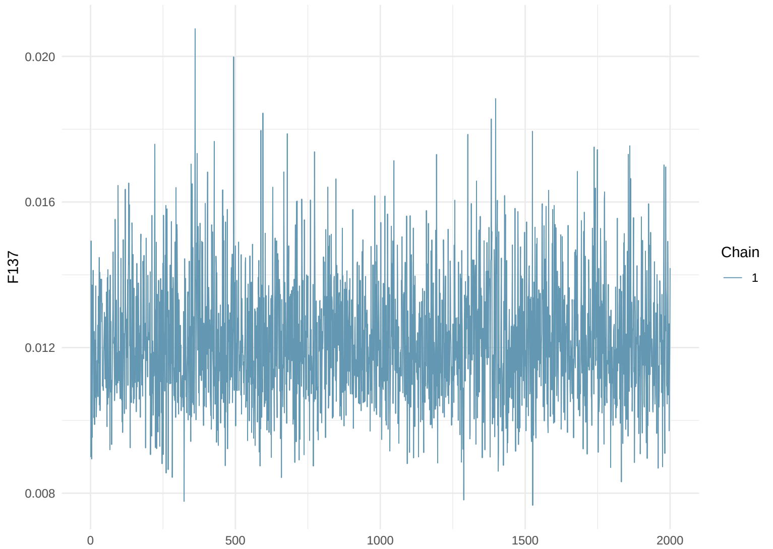
Trace Plot: F137
