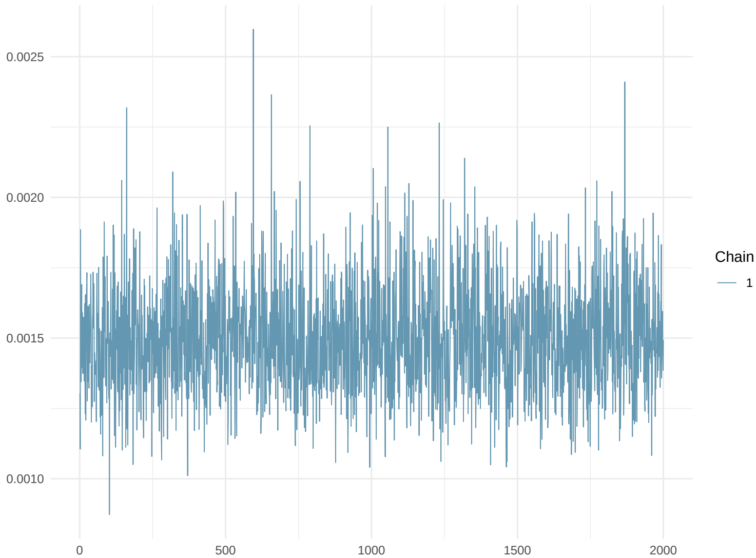
Trace Plot: F166
