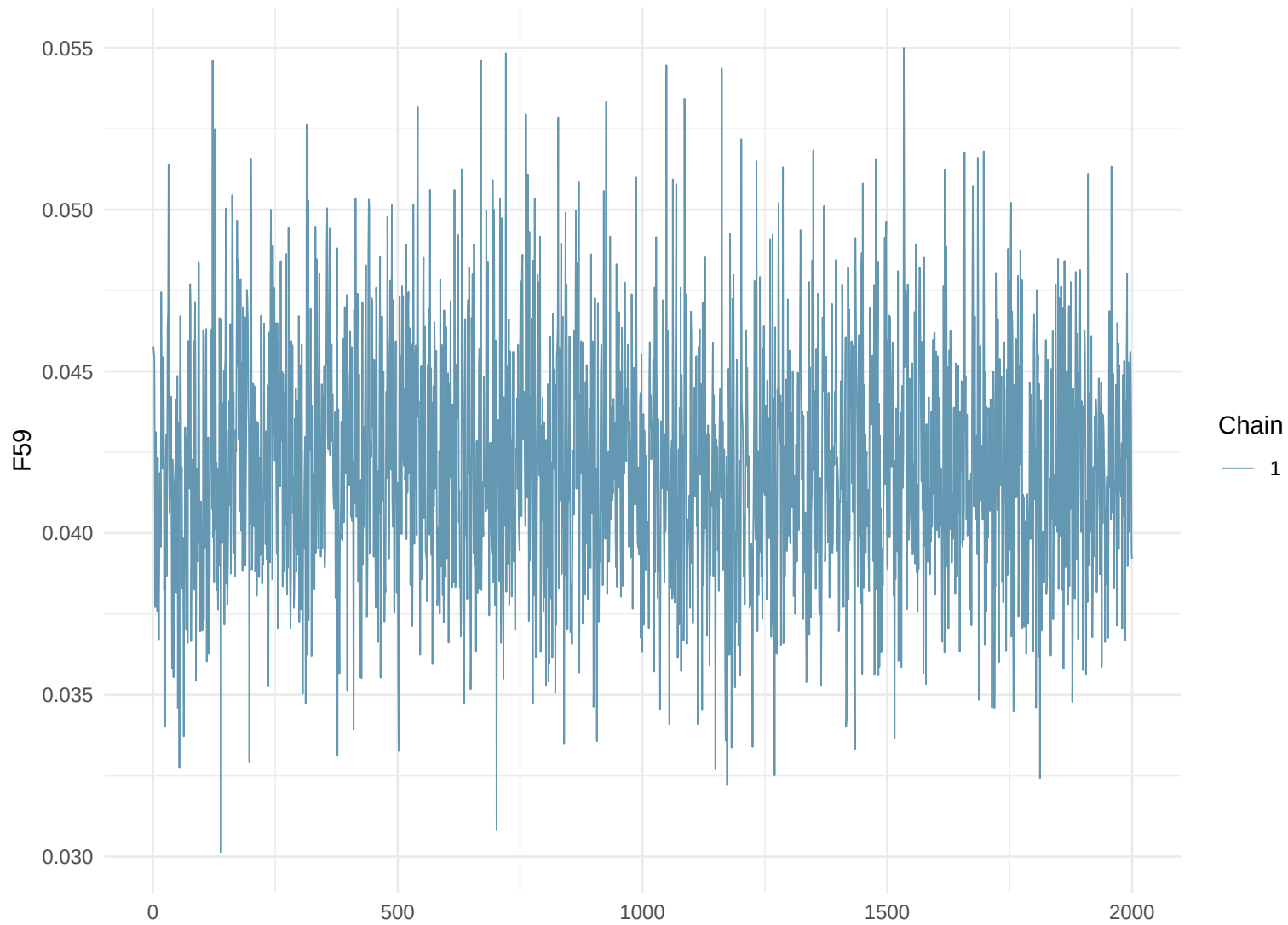
Trace Plot: F59
