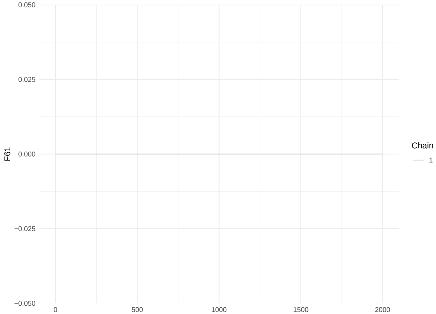
Trace Plot: F61
