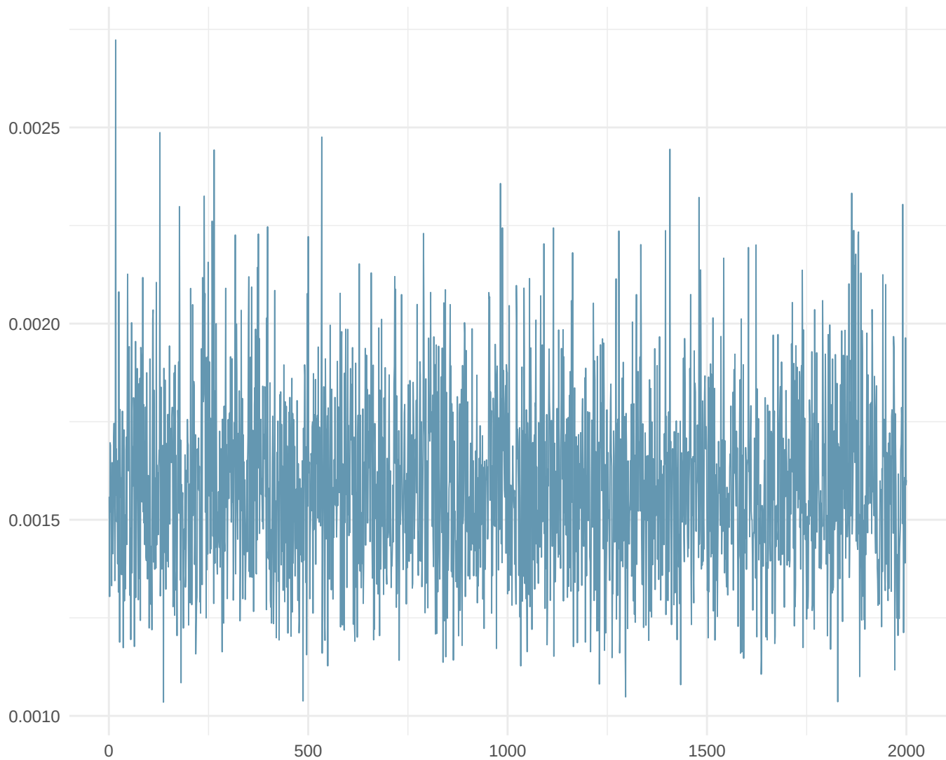
Trace Plot: F143
