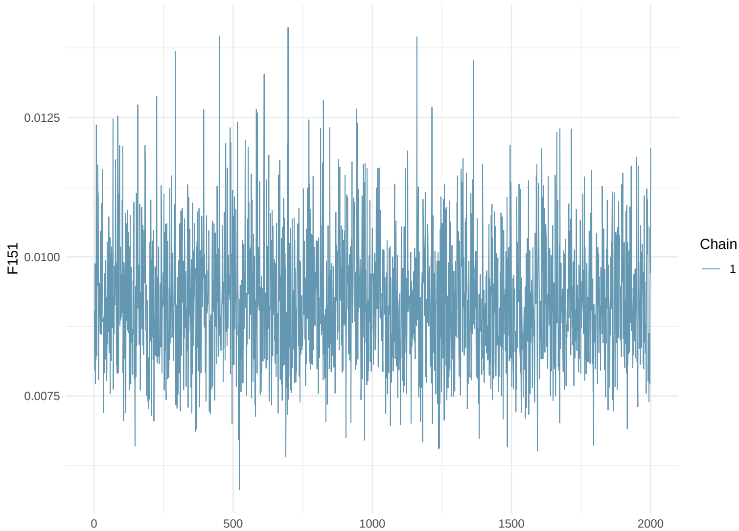
Trace Plot: F151
