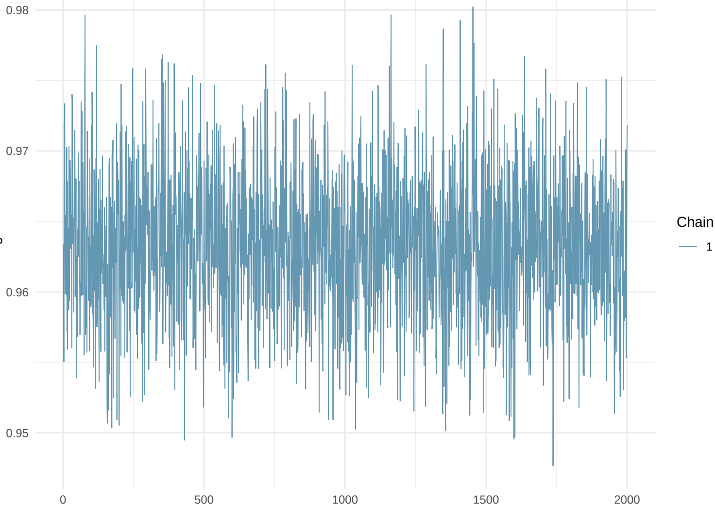
Trace Plot: Mig144
