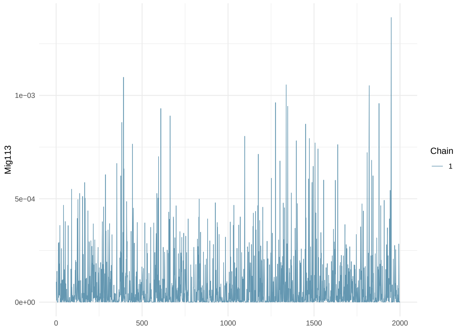
Trace Plot: Mig113
