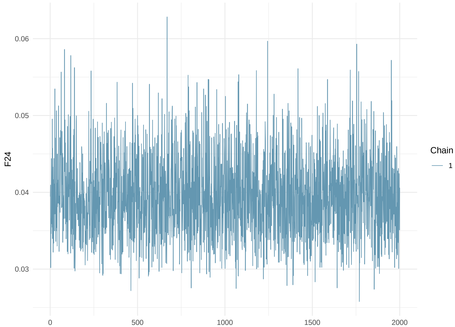
Trace Plot: F24
