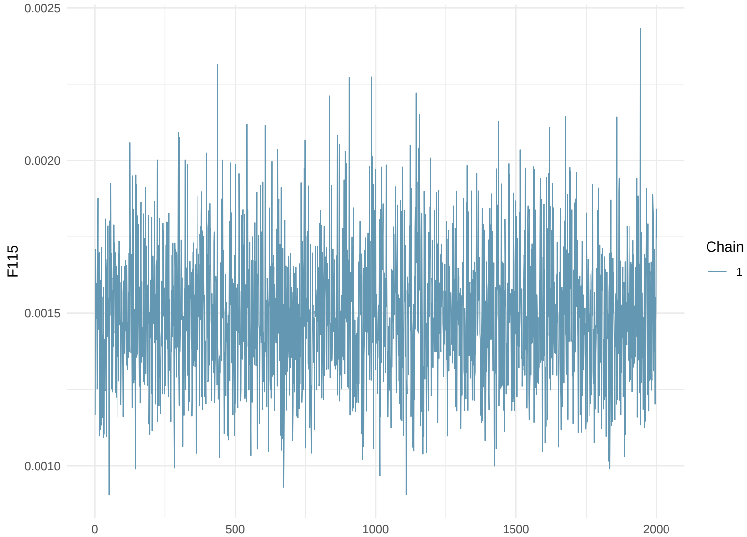
Trace Plot: F115
