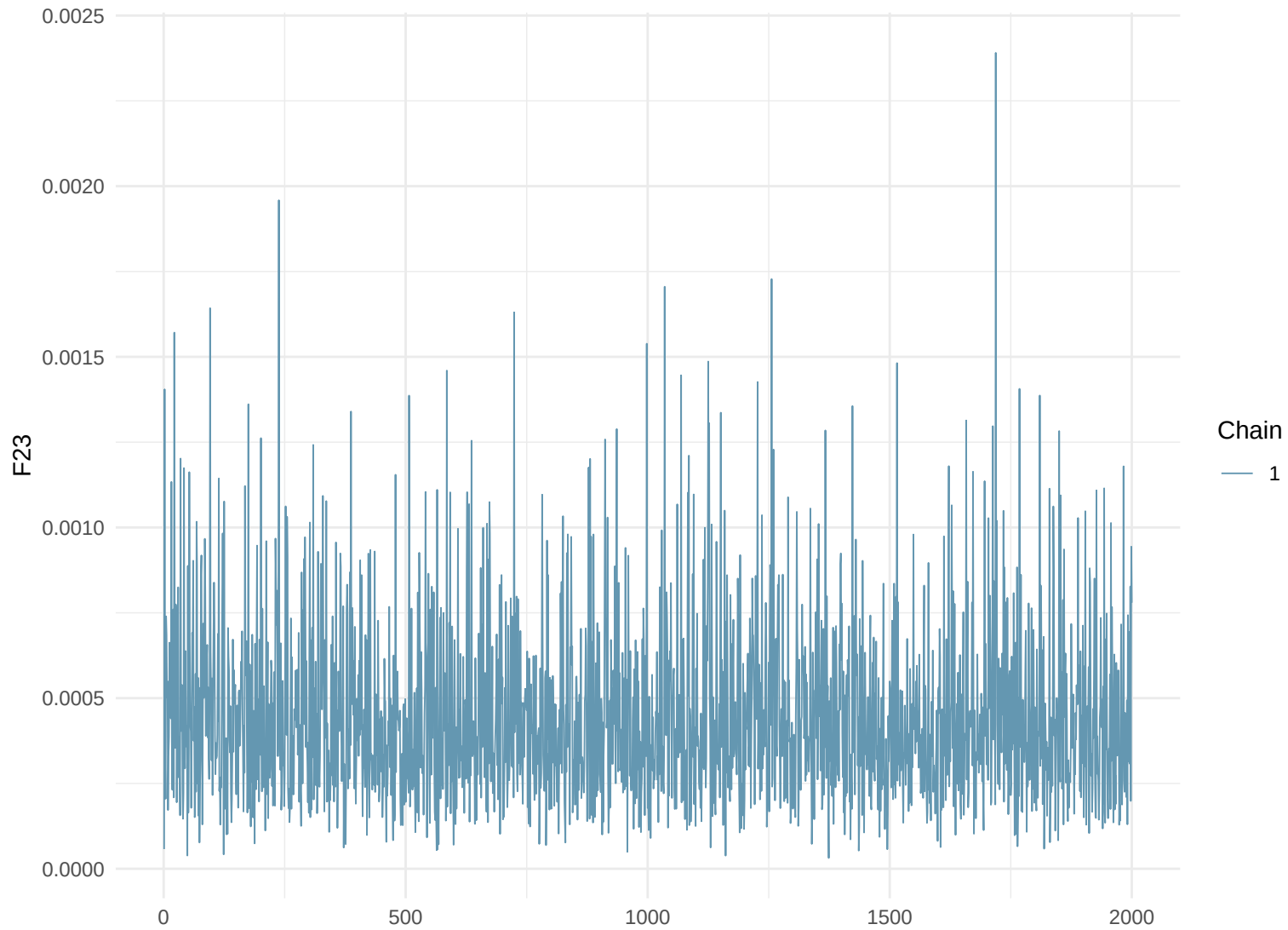
Trace Plot: F23
