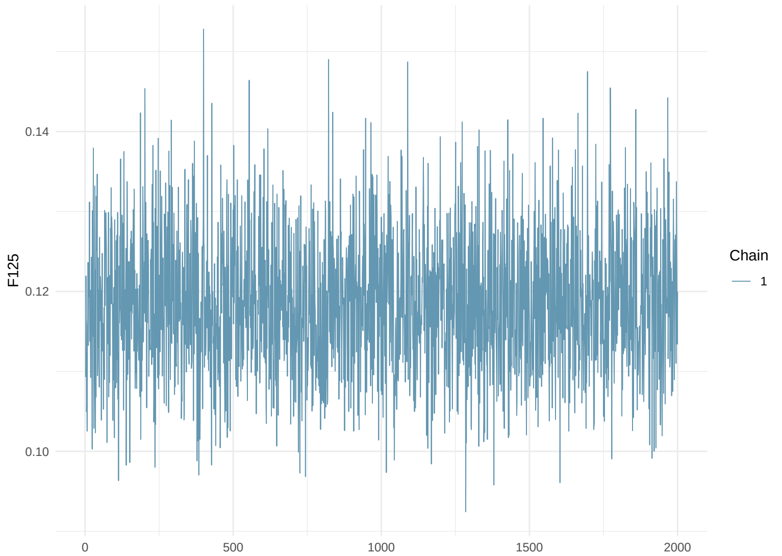
Trace Plot: F125
