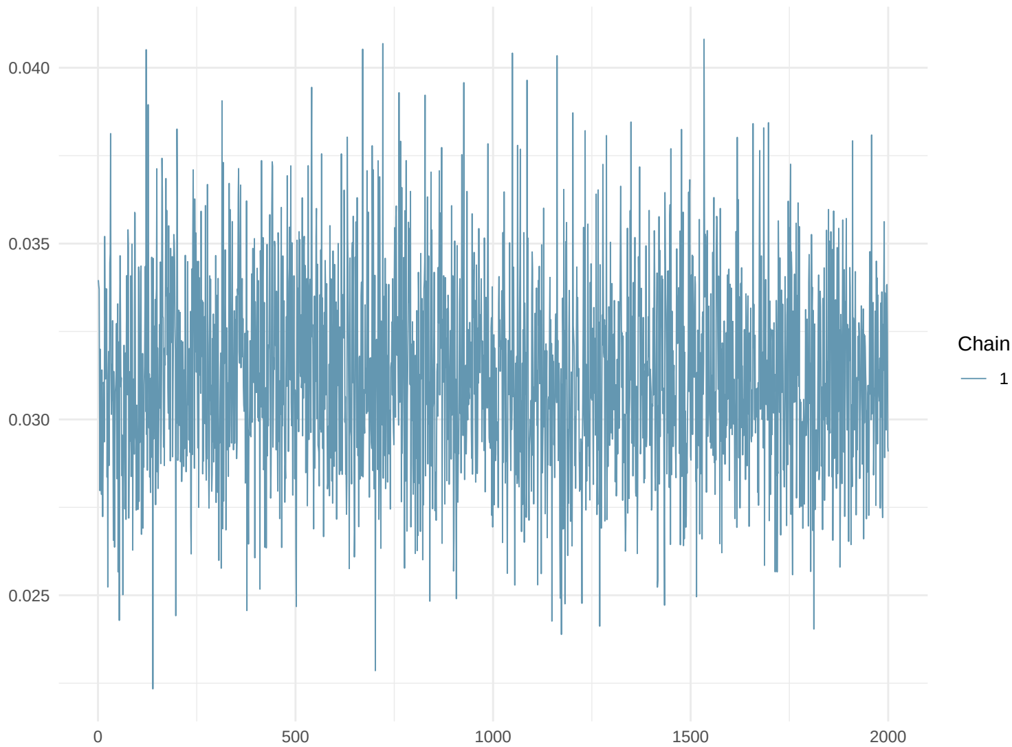
Trace Plot: F47
