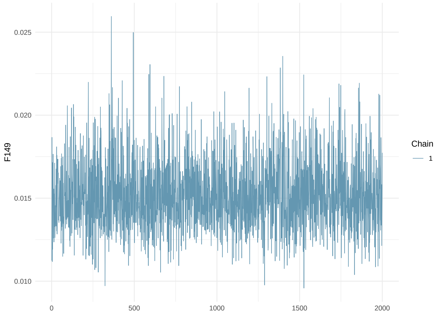
Trace Plot: F149
