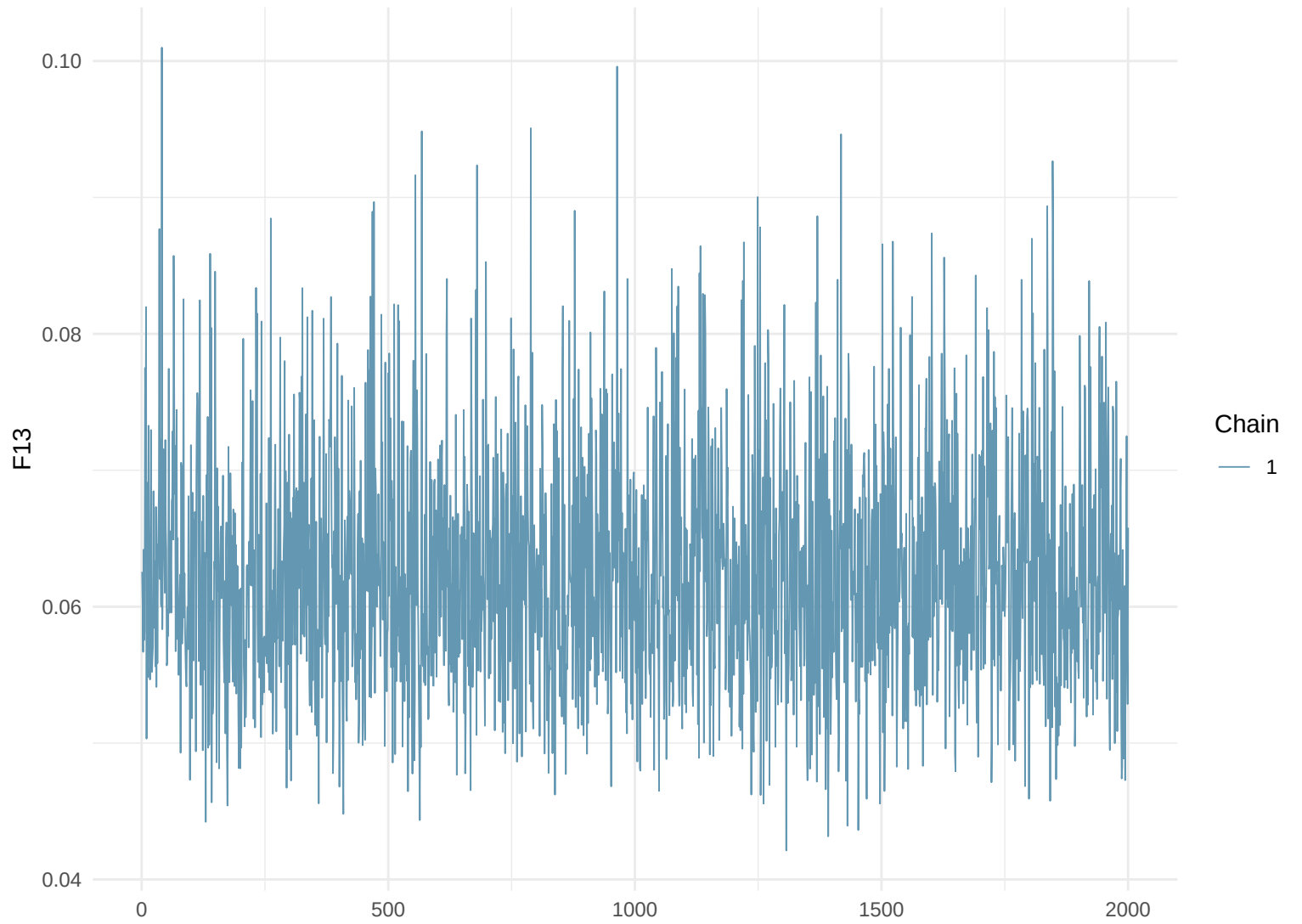
Trace Plot: F13
