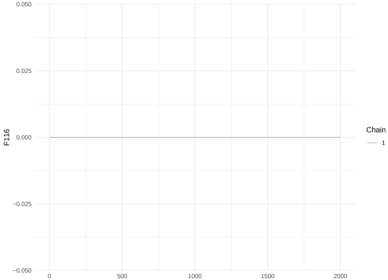
Trace Plot: F116
