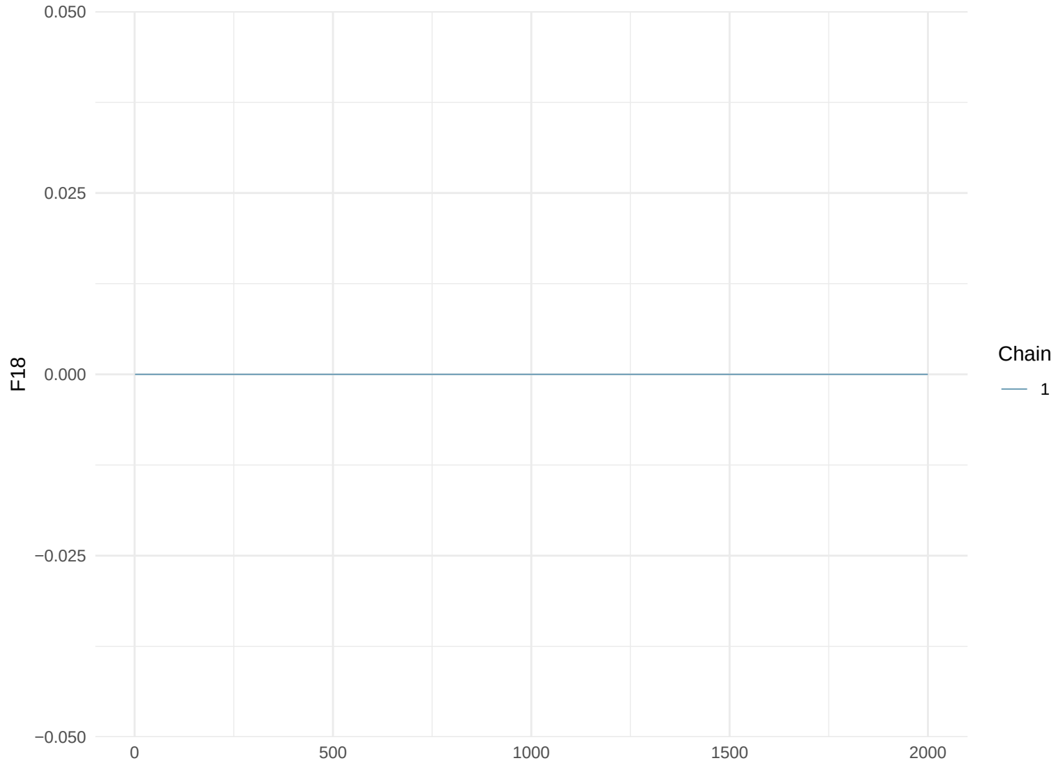
Trace Plot: F18
