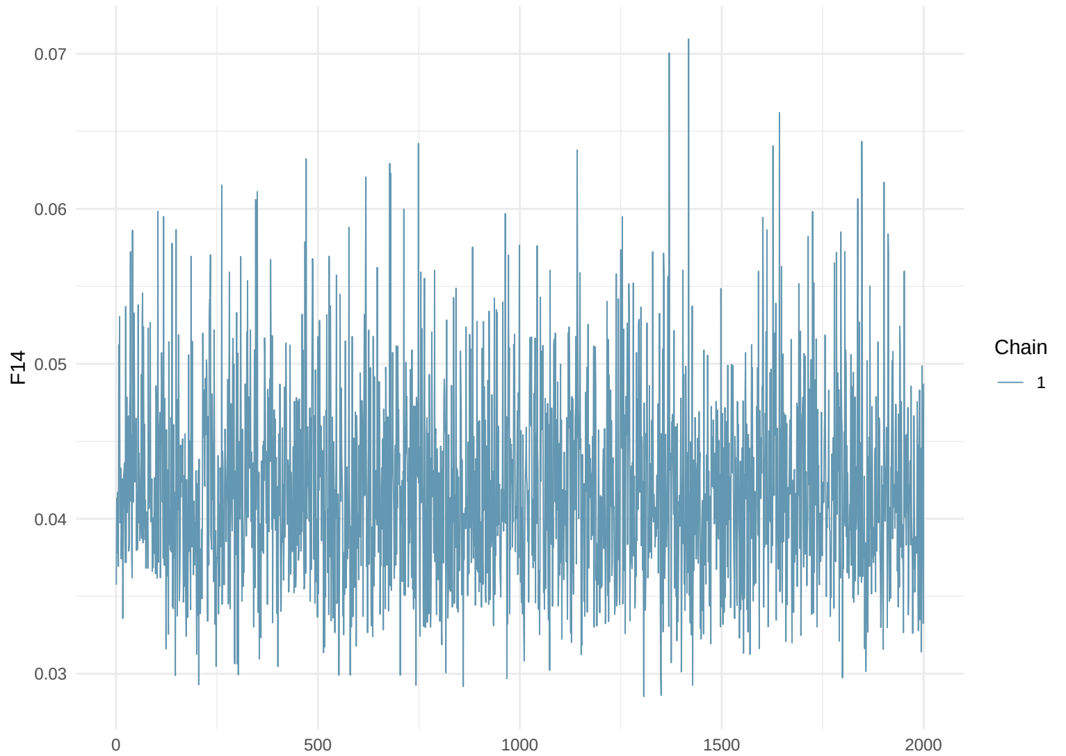
Trace Plot: F14
