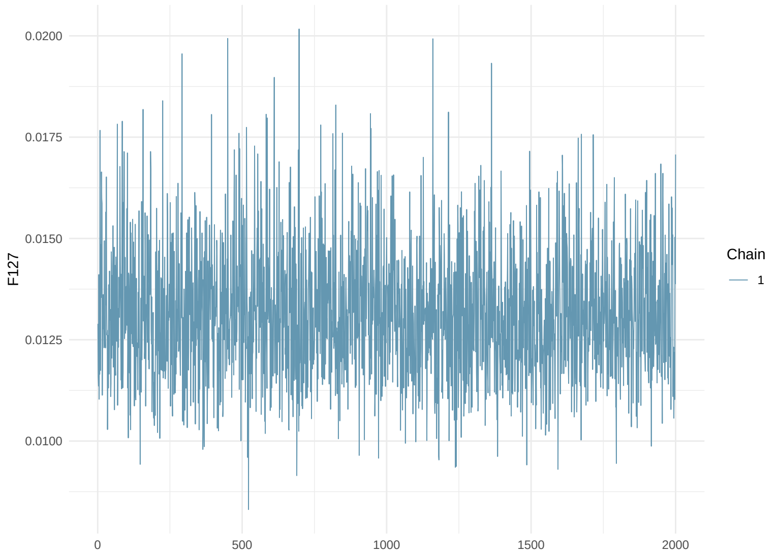
Trace Plot: F127
