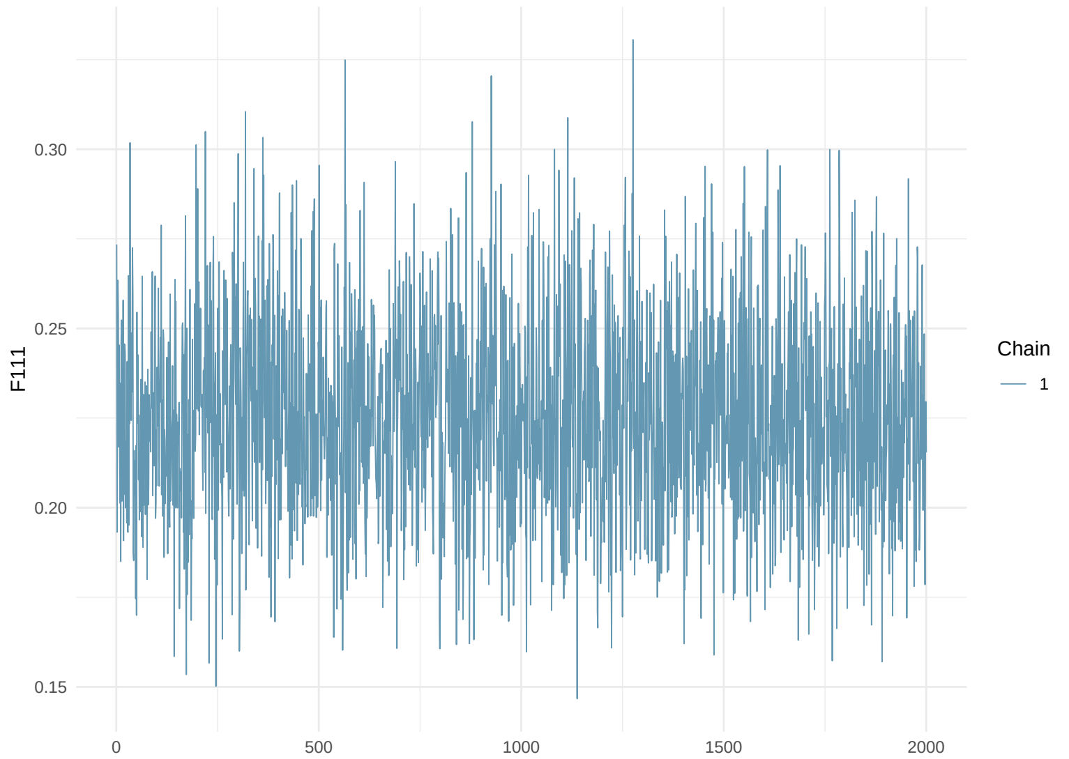
Trace Plot: F111
