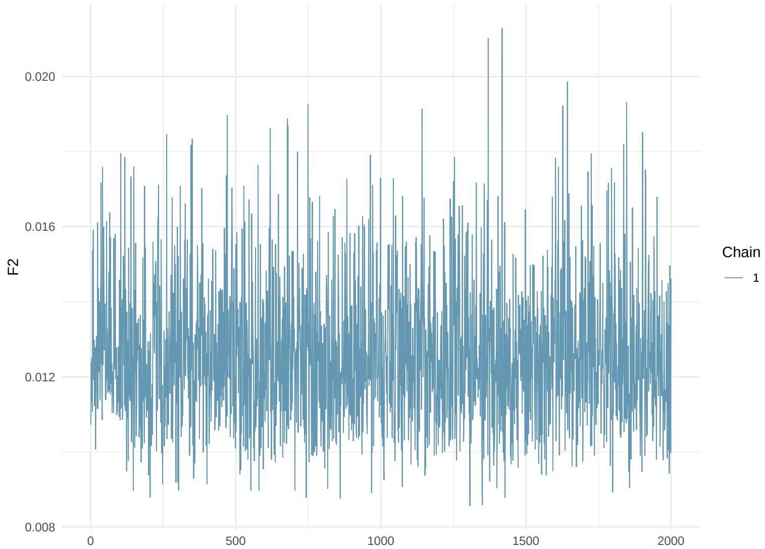
Trace Plot: F2
