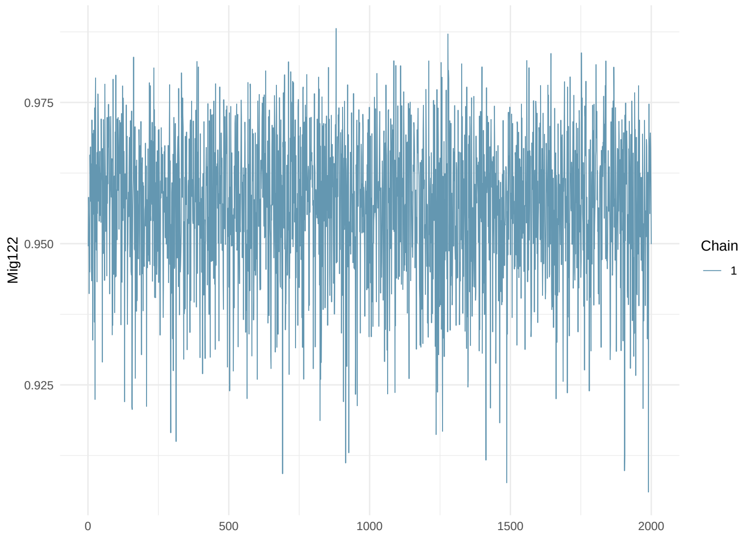
Trace Plot: Mig122
