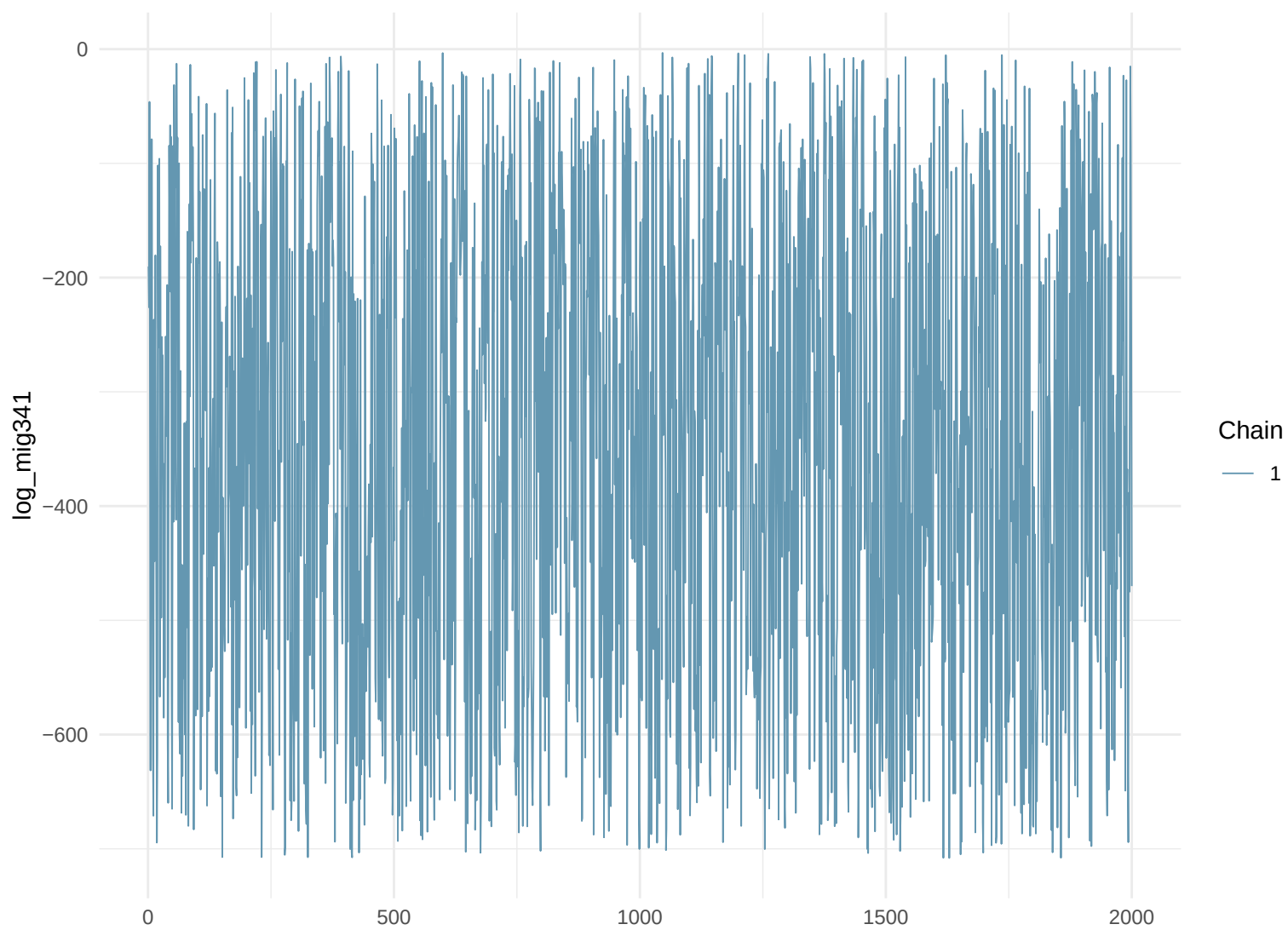
Trace Plot: log_mig341
