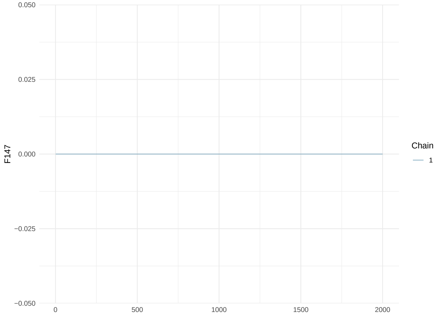
Trace Plot: F147
