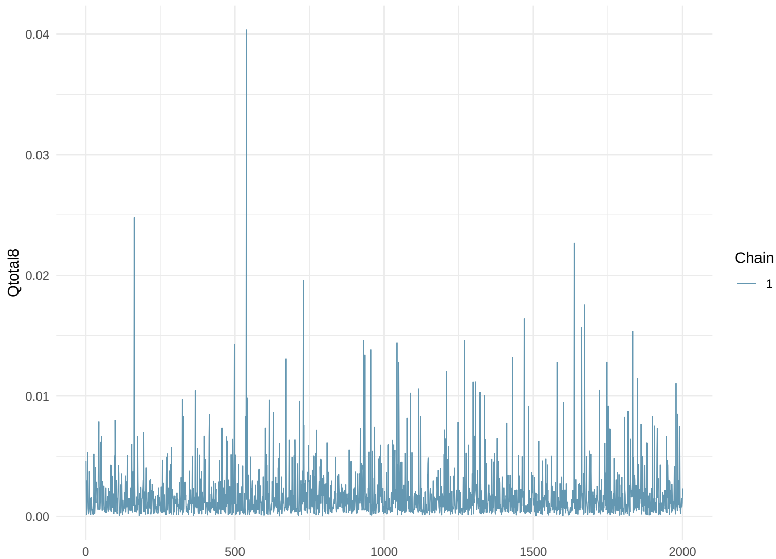
Trace Plot: Qtotal8
