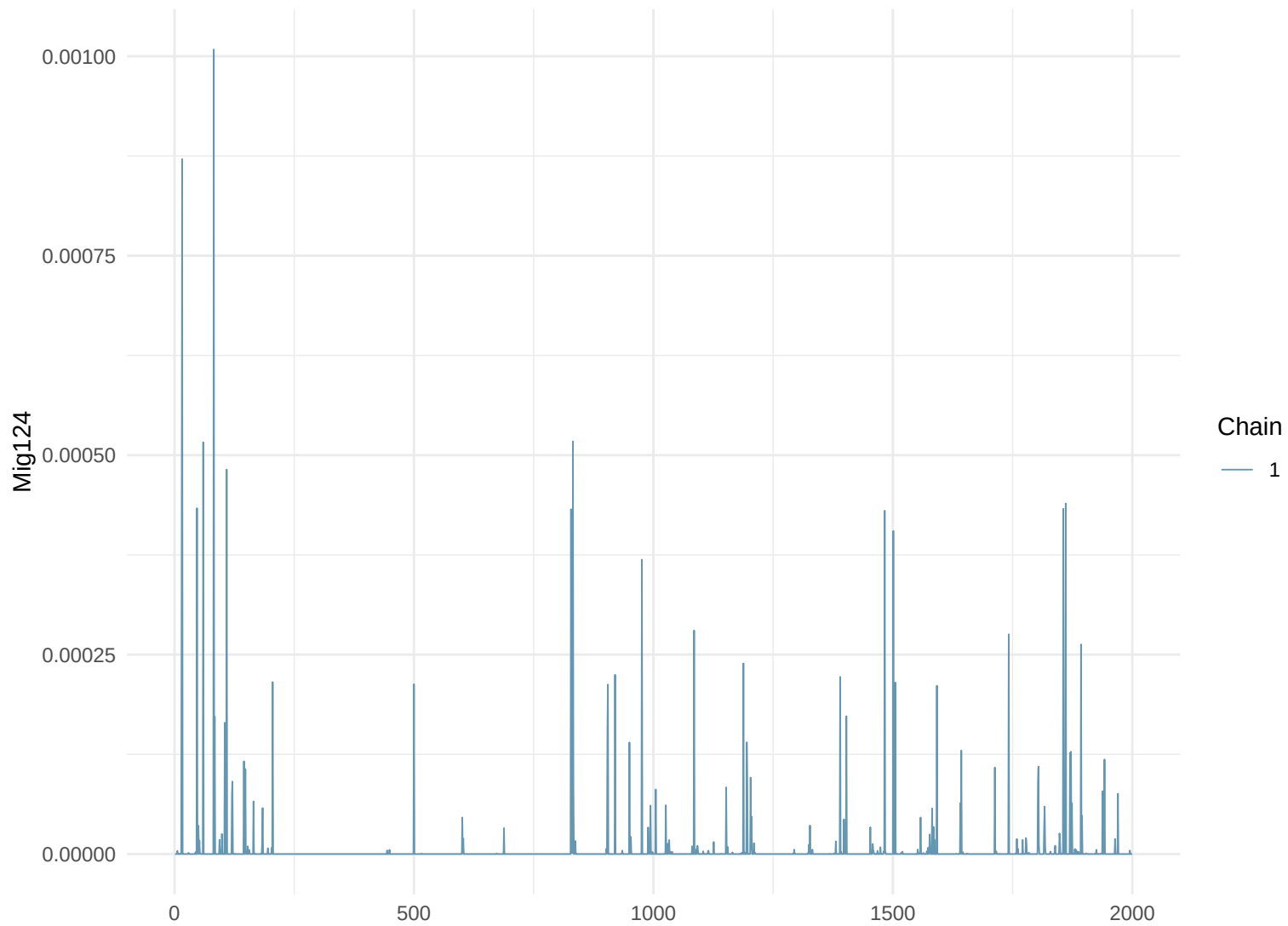
Trace Plot: Mig124
