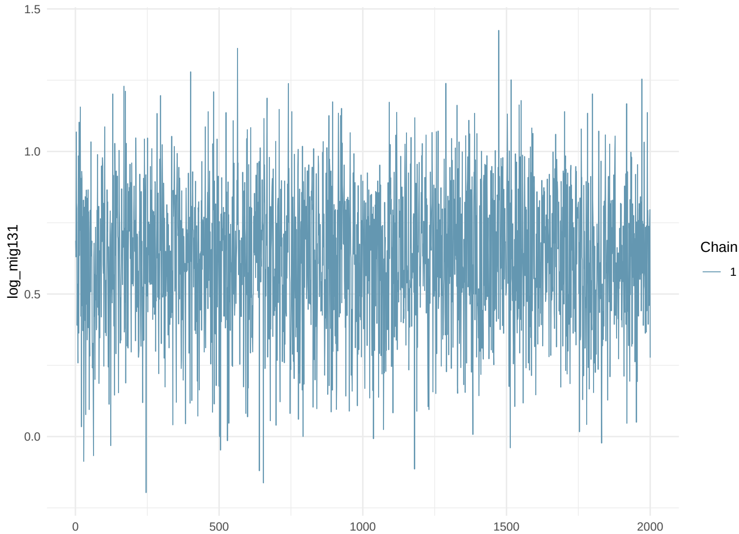
Trace Plot: log_mig131
