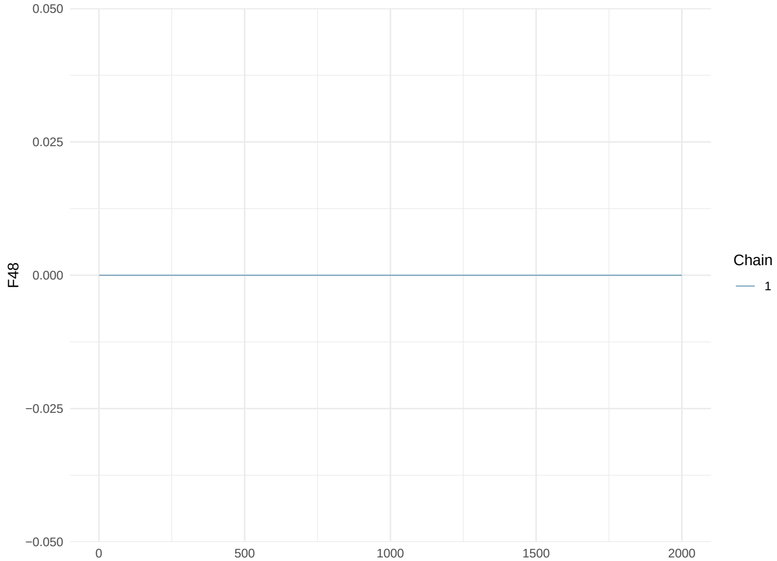
Trace Plot: F48
