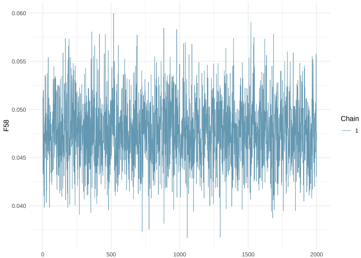
Trace Plot: F58
