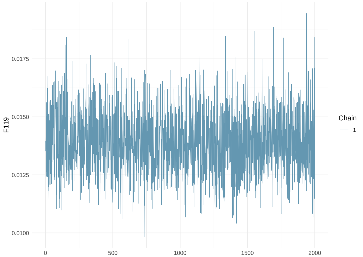
Trace Plot: F119
