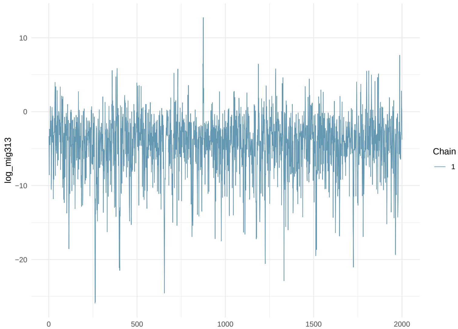
Trace Plot: log_mig313
