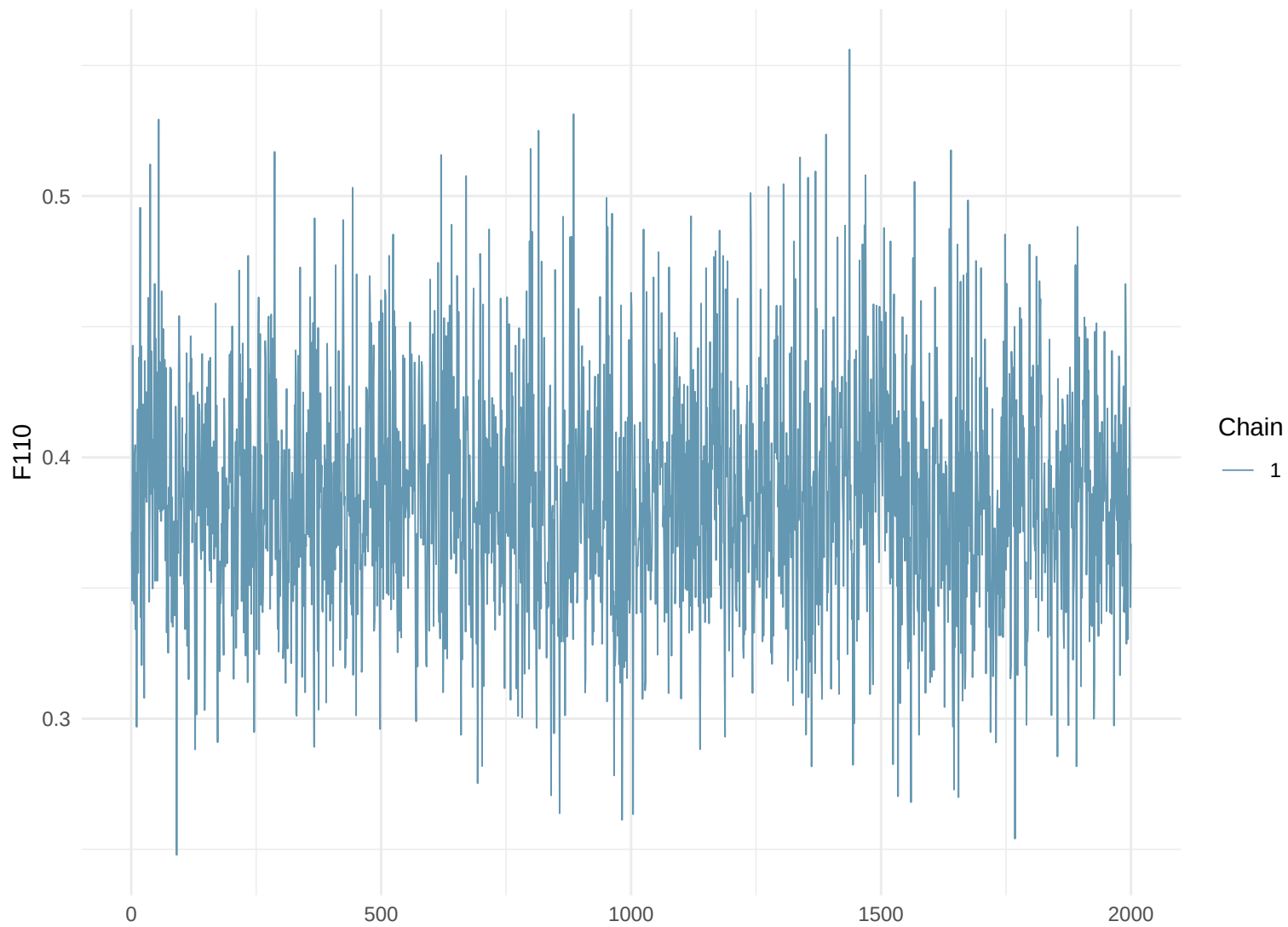
Trace Plot: F110
