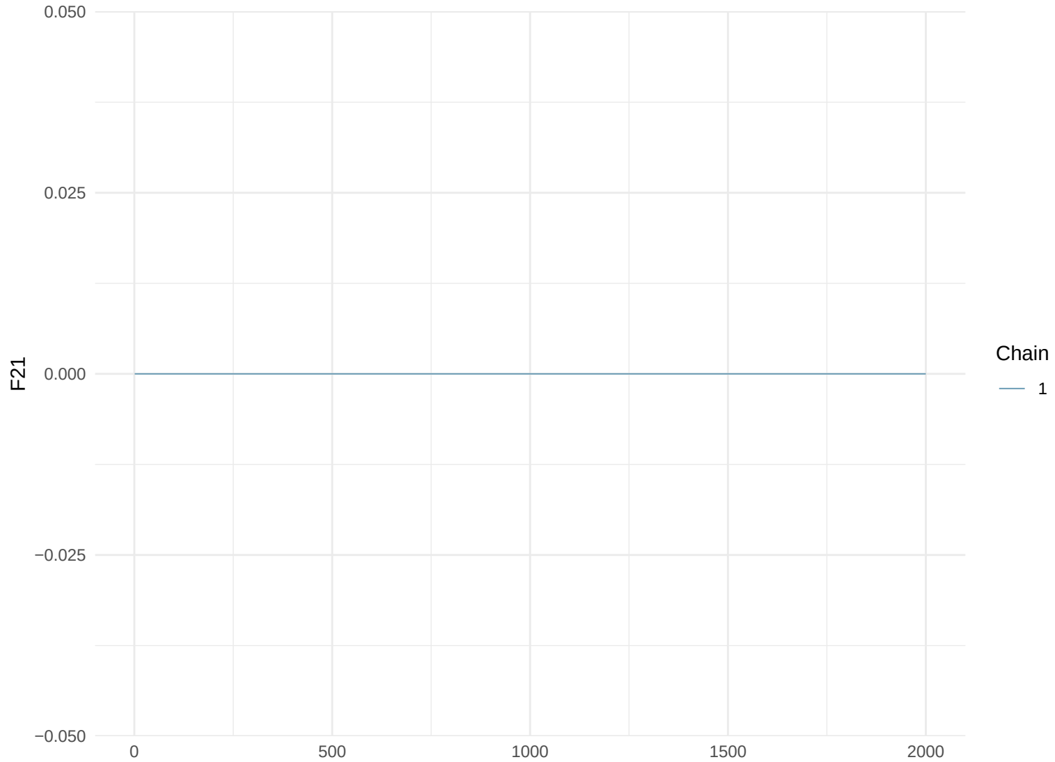
Trace Plot: F21
