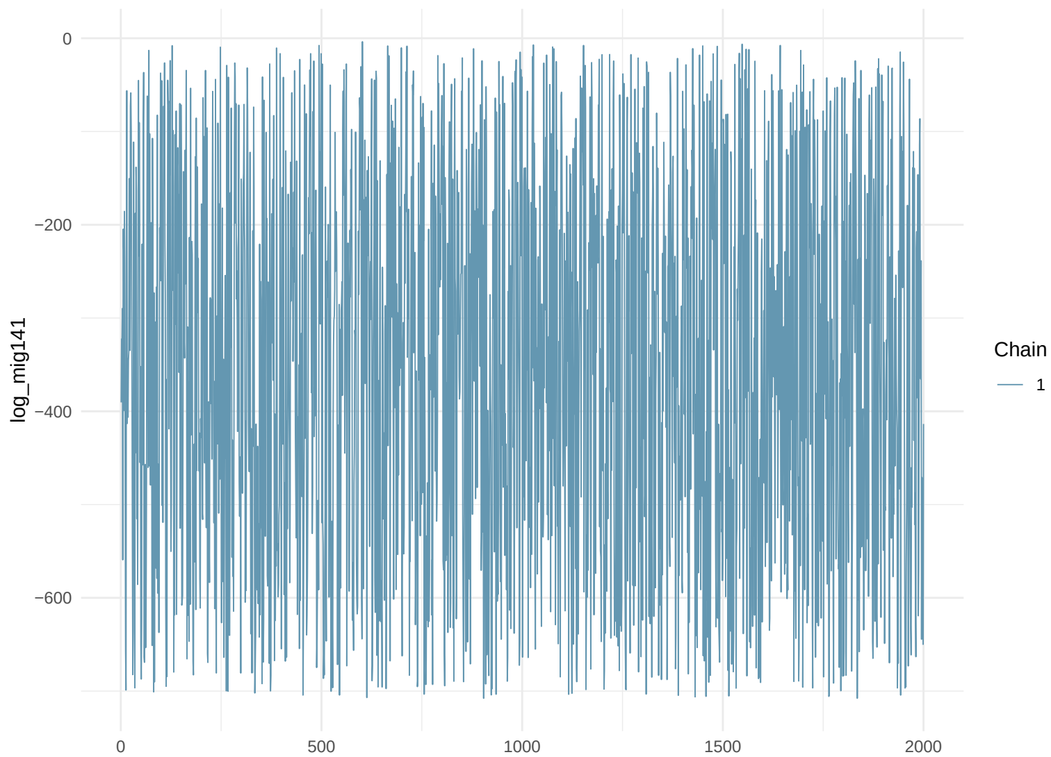
Trace Plot: log_mig141
