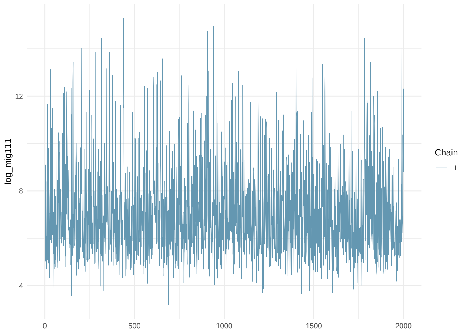
Trace Plot: log_mig111
