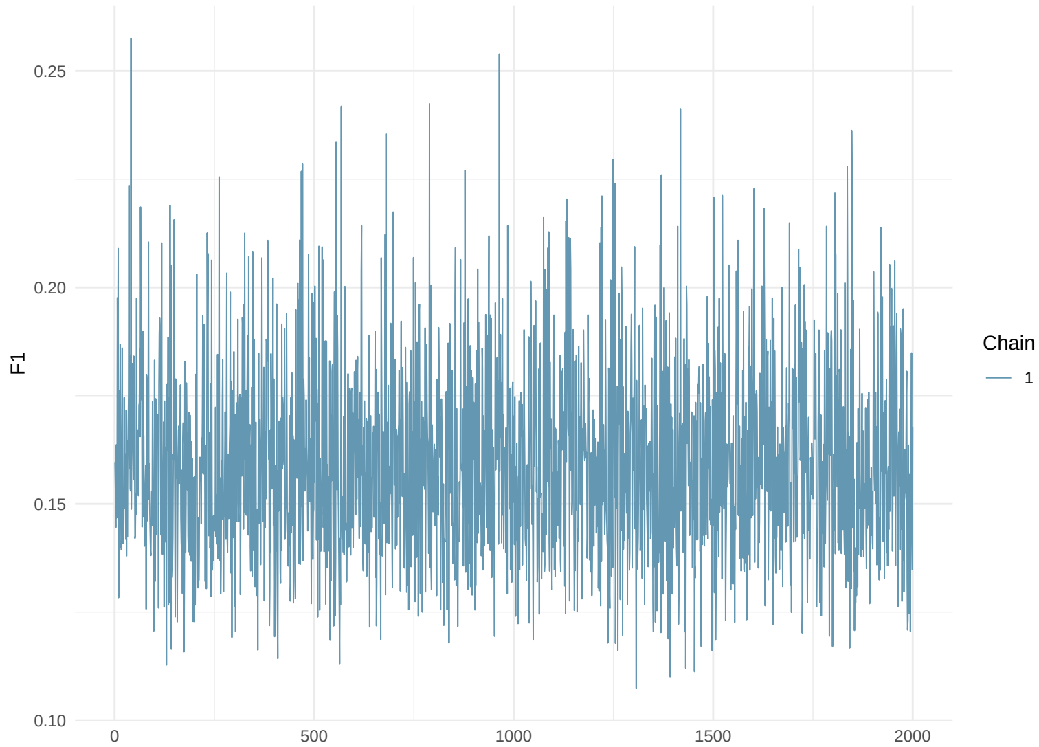
Trace Plot: F1
