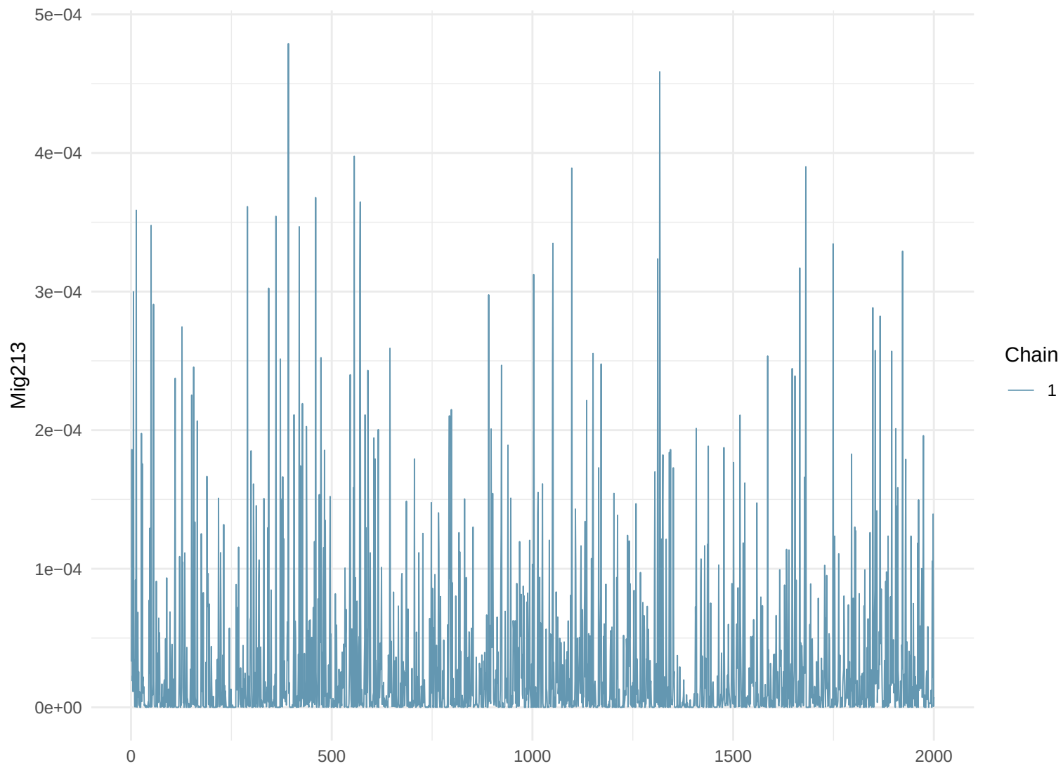
Trace Plot: Mig213
