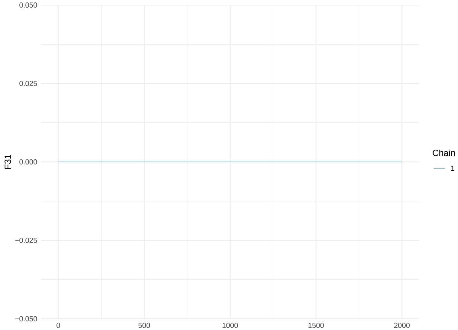
Trace Plot: F31
