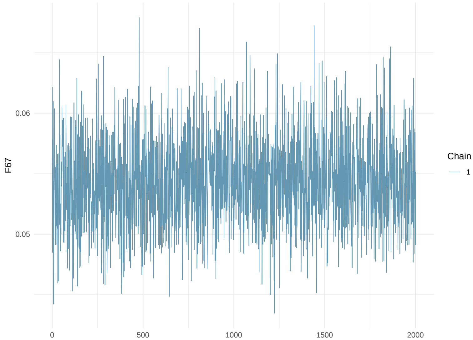
Trace Plot: F67
