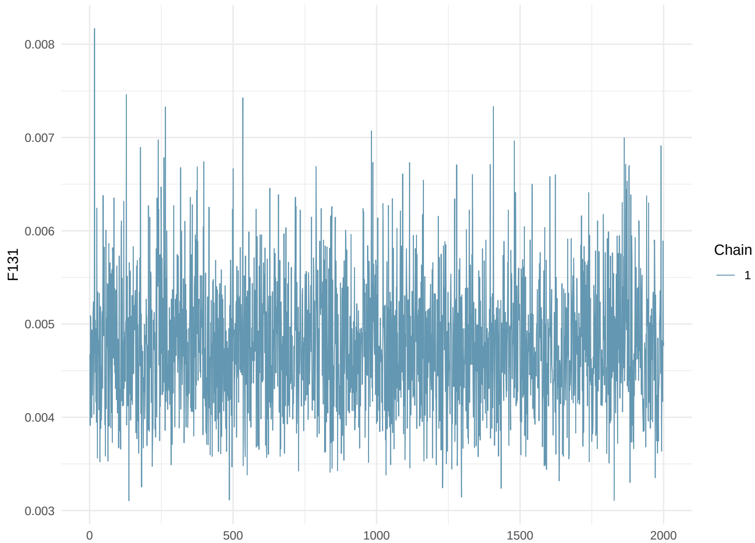
Trace Plot: F131
