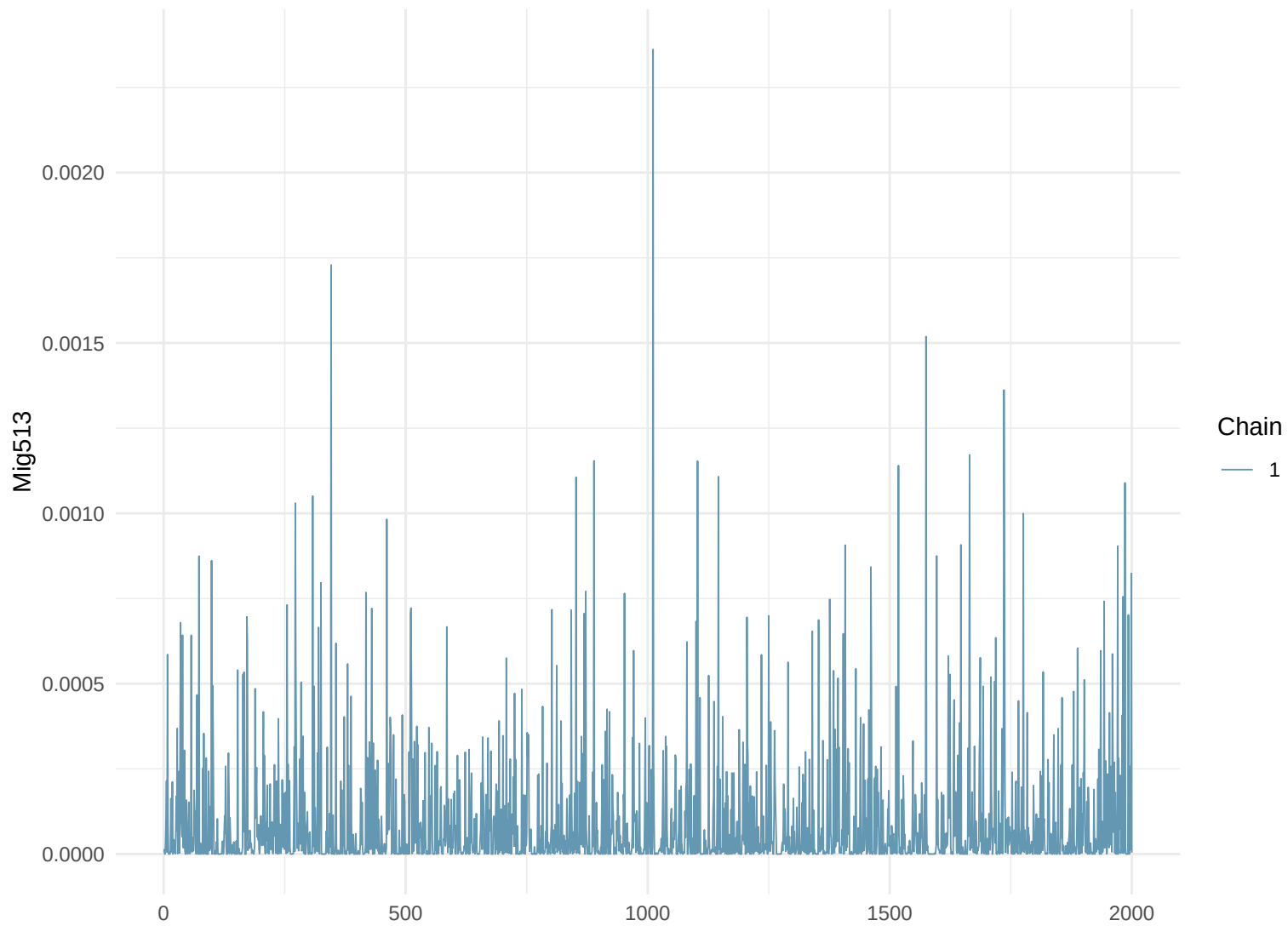
Trace Plot: Mig513
