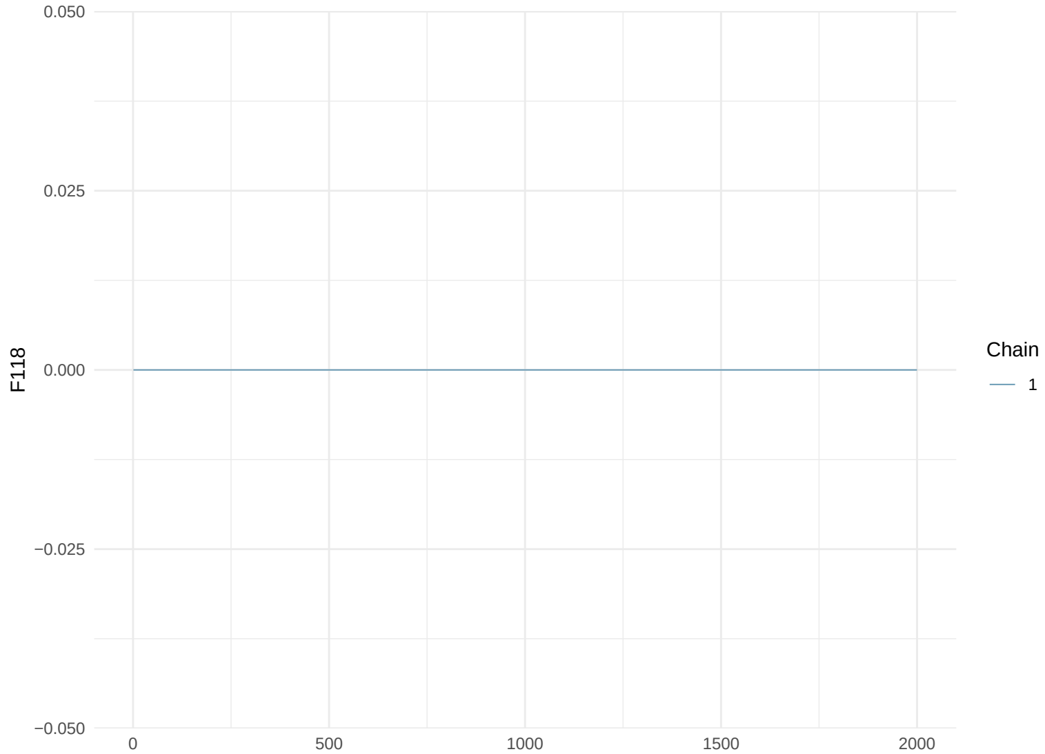
Trace Plot: F118
