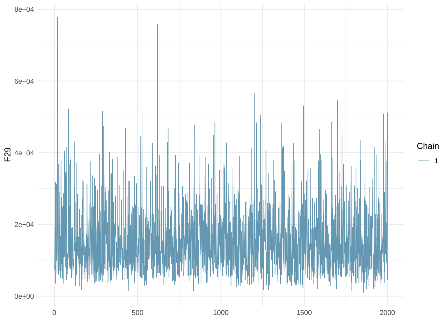
Trace Plot: F29
