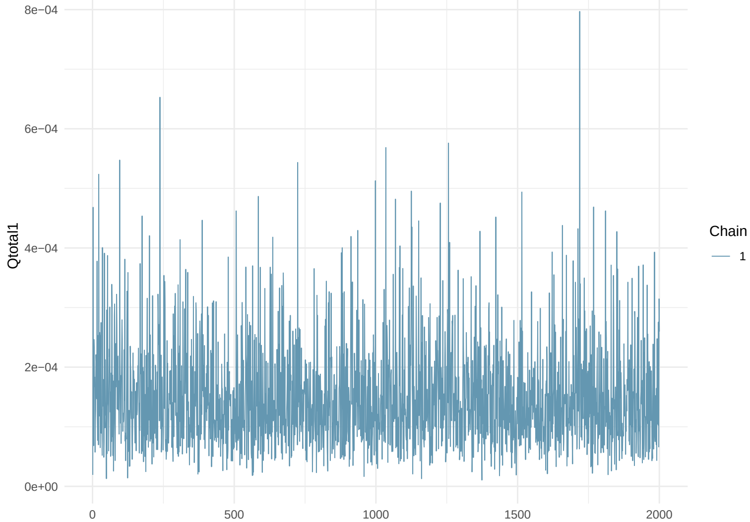
Trace Plot: Qtotal1
