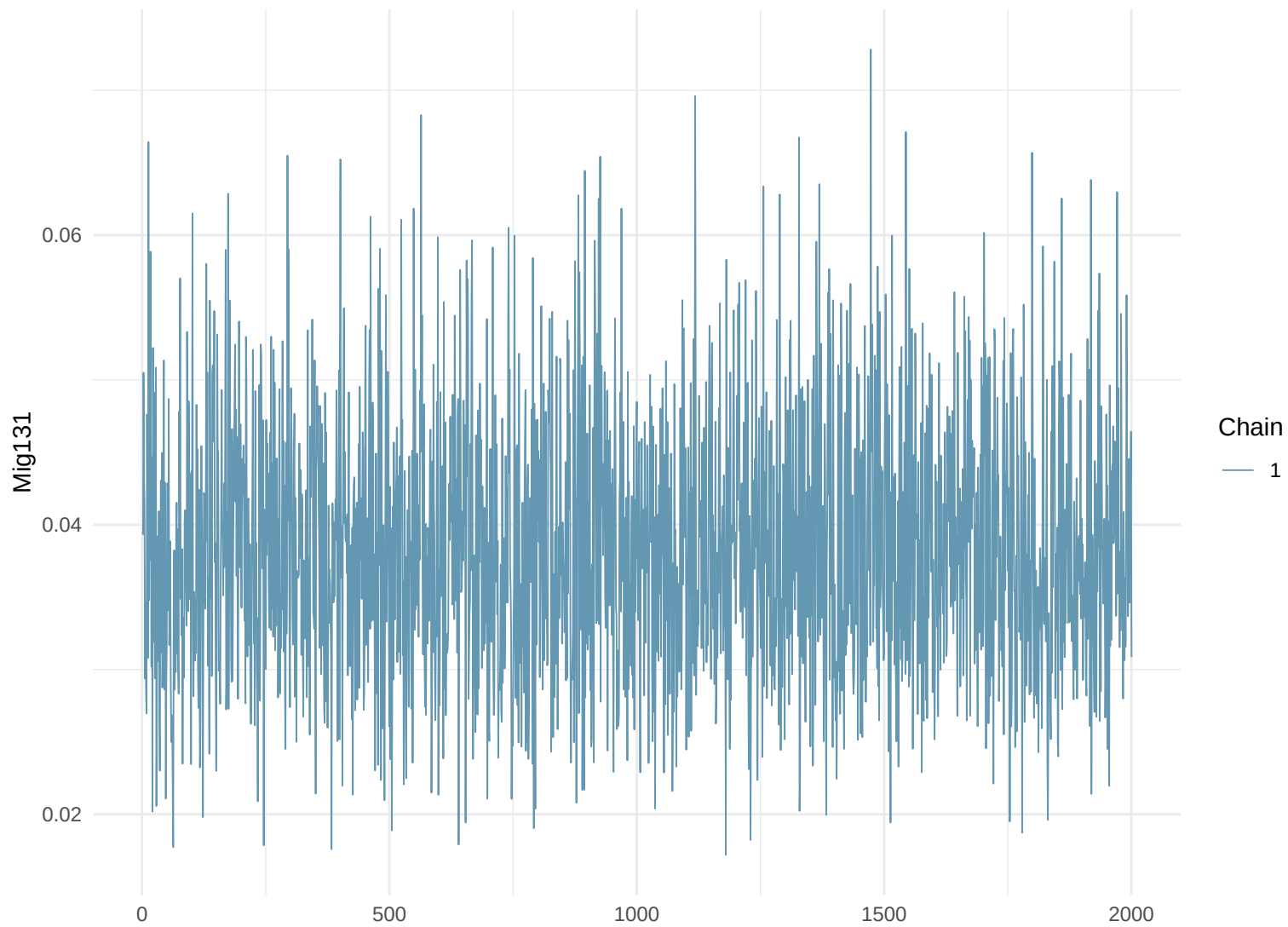
Trace Plot: Mig131
