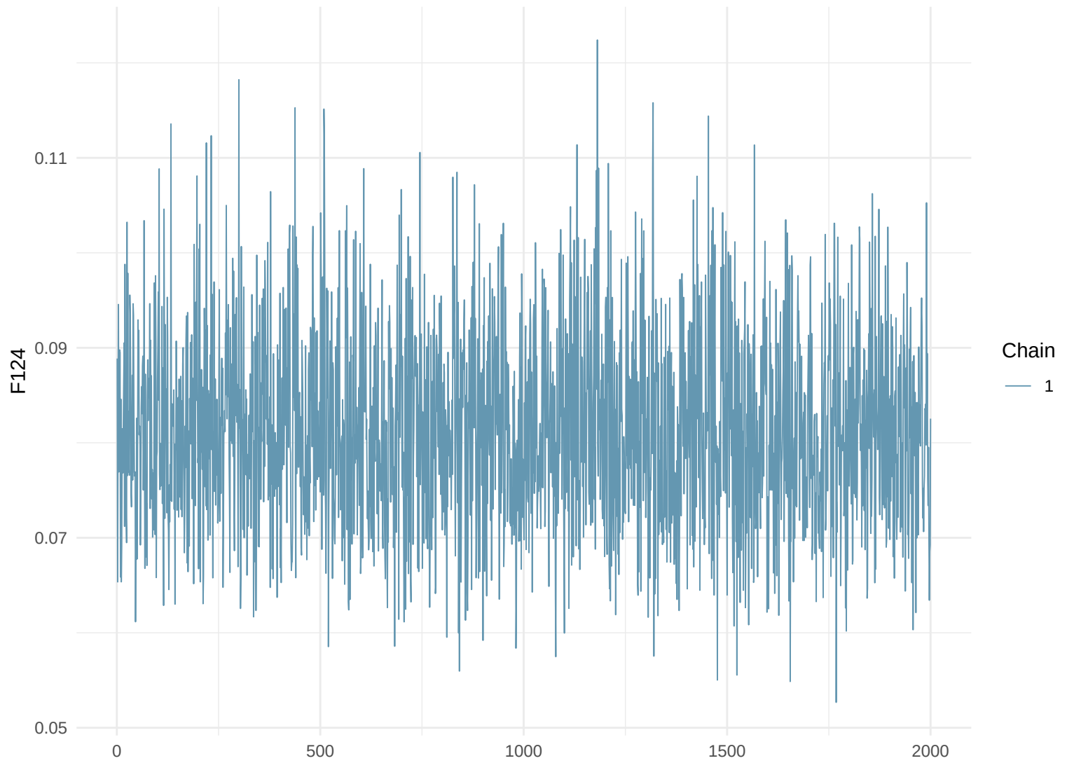
Trace Plot: F124
