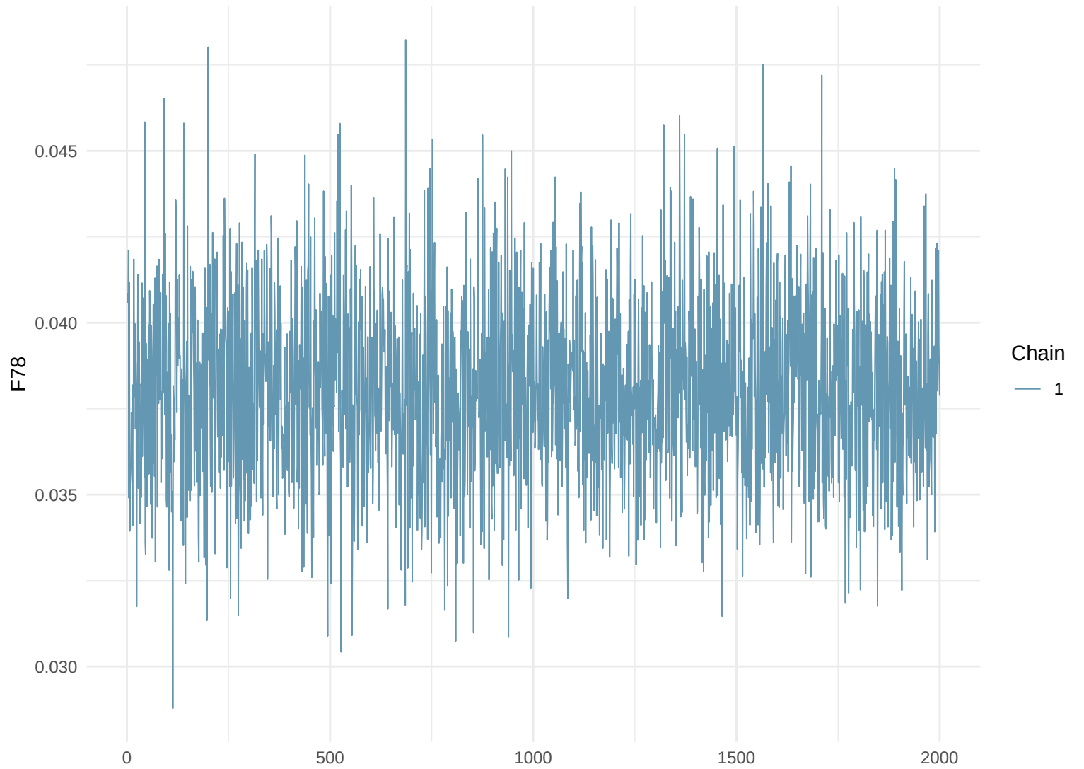
Trace Plot: F78
