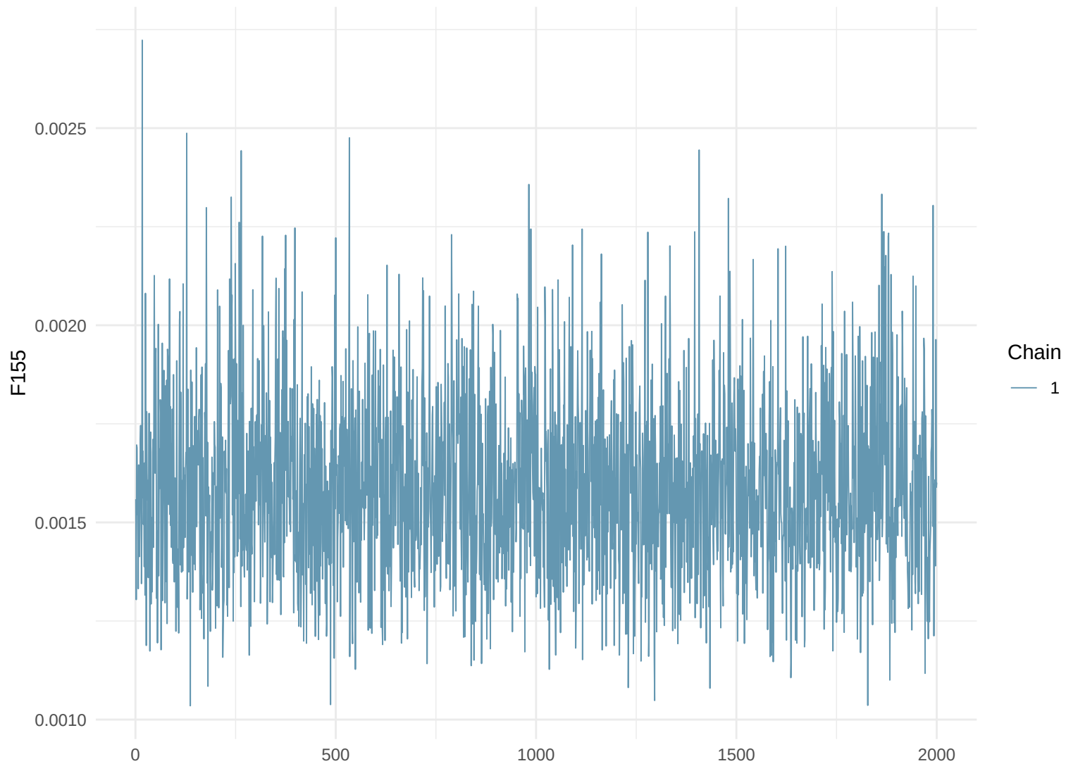
Trace Plot: F155
