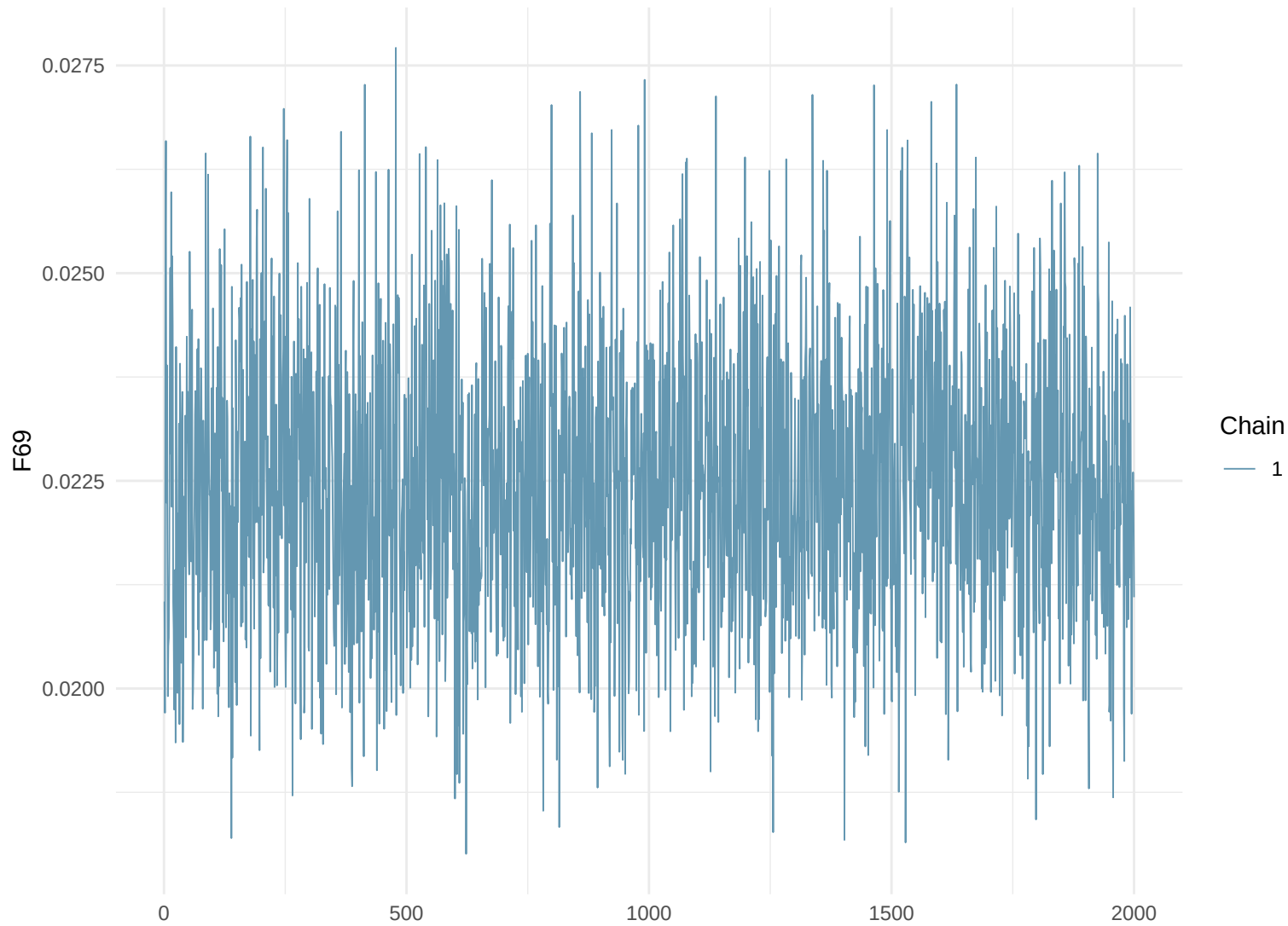
Trace Plot: F69
