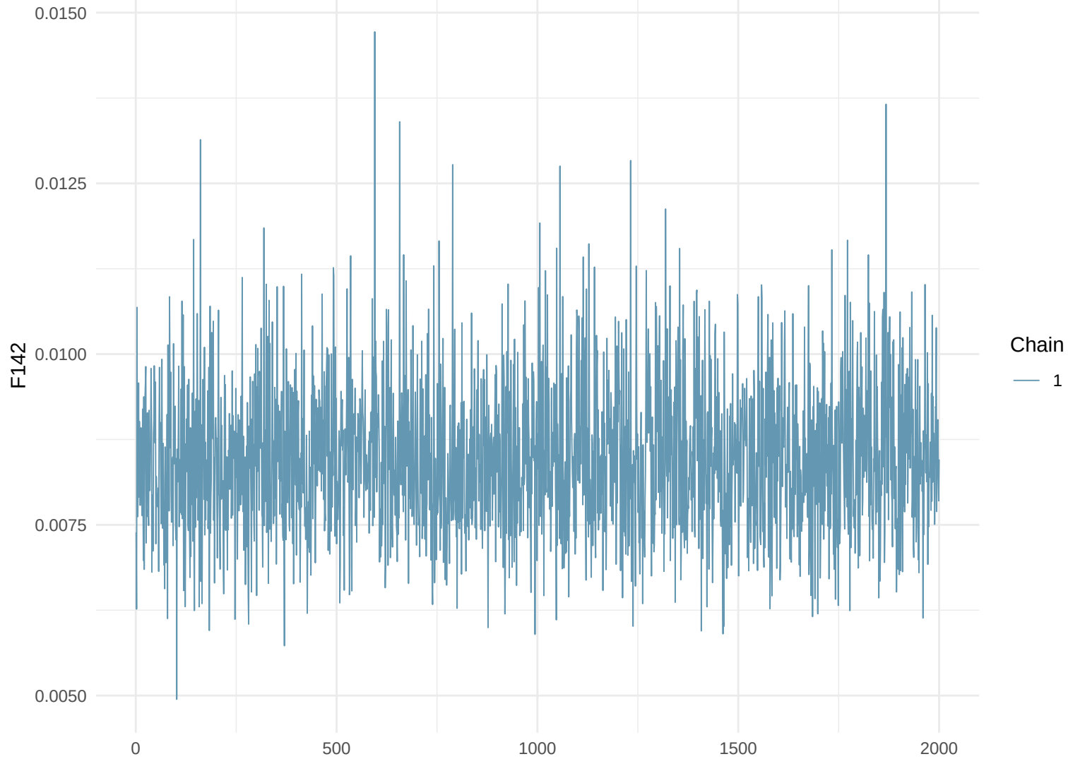
Trace Plot: F142
