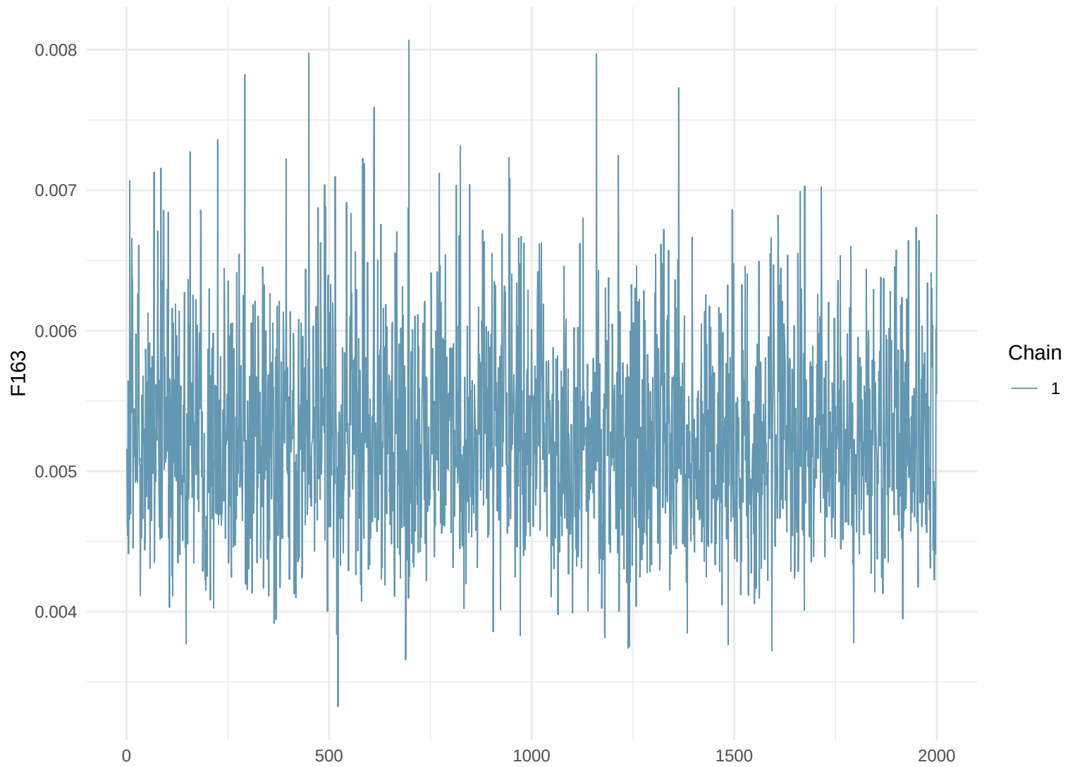
Trace Plot: F163
