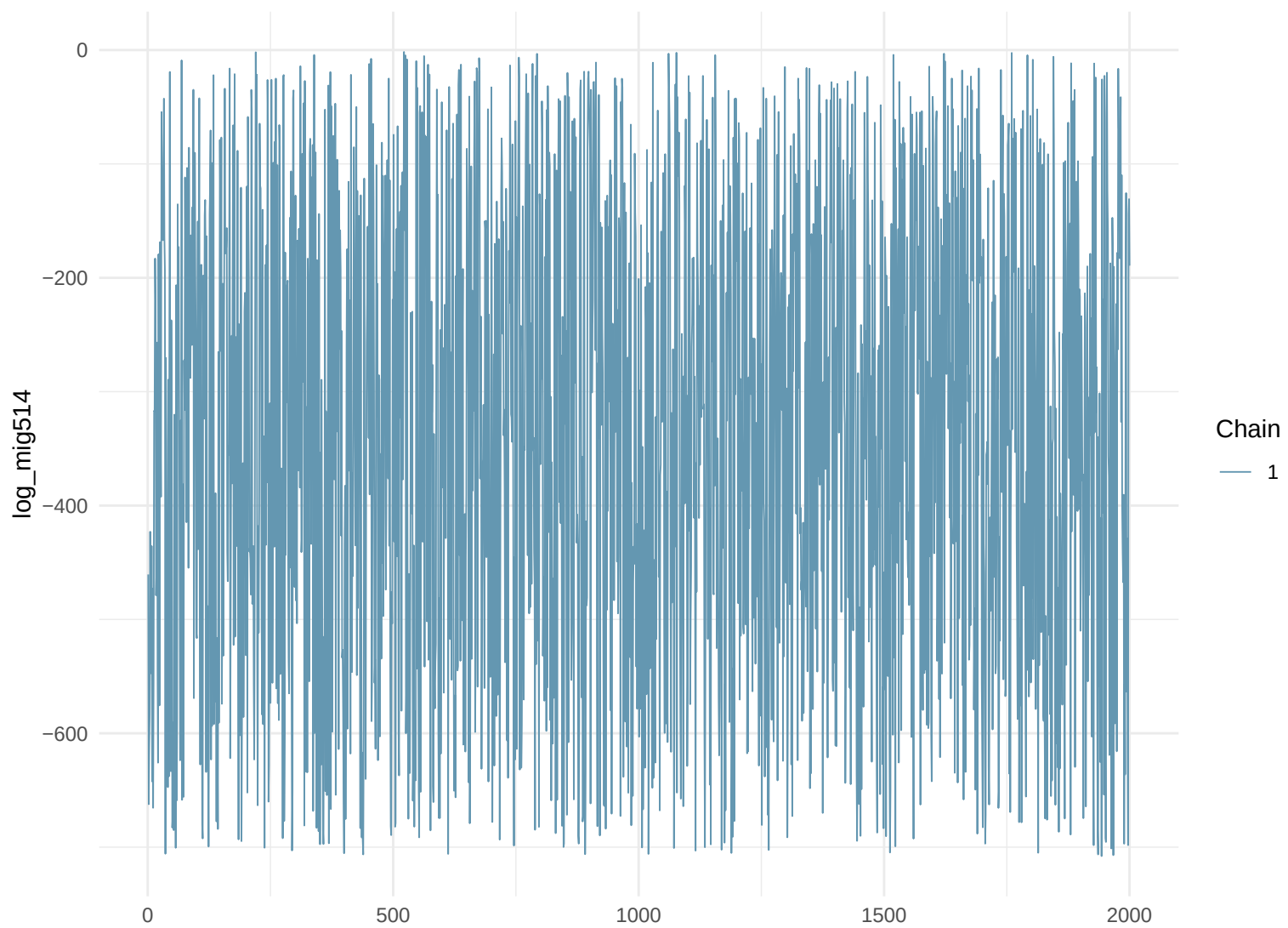
Trace Plot: log_mig514
