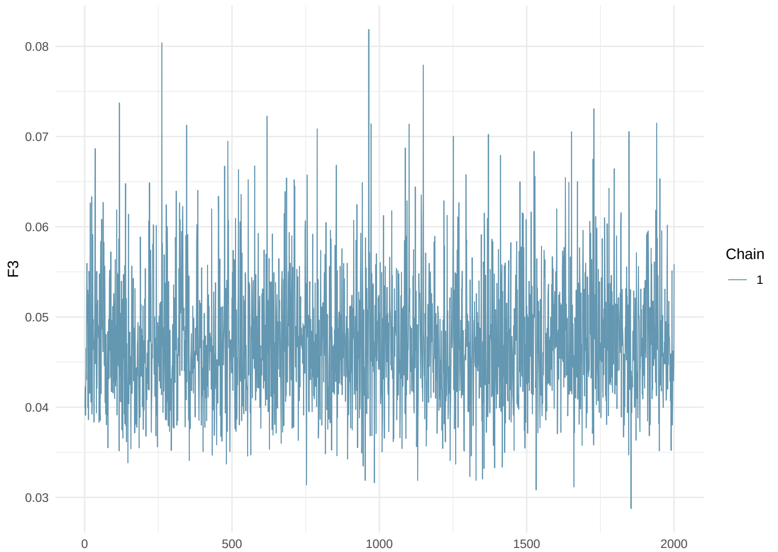
Trace Plot: F3
