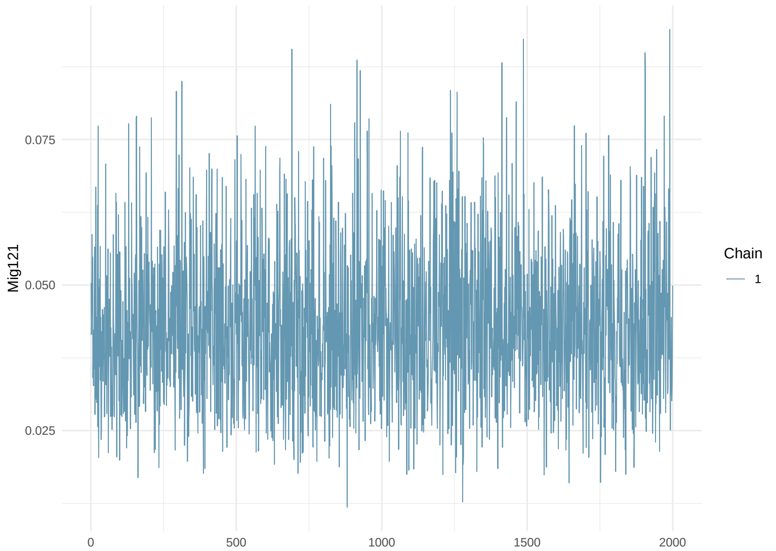
Trace Plot: Mig121
