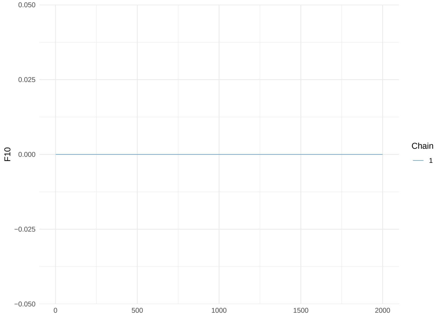
Trace Plot: F10
