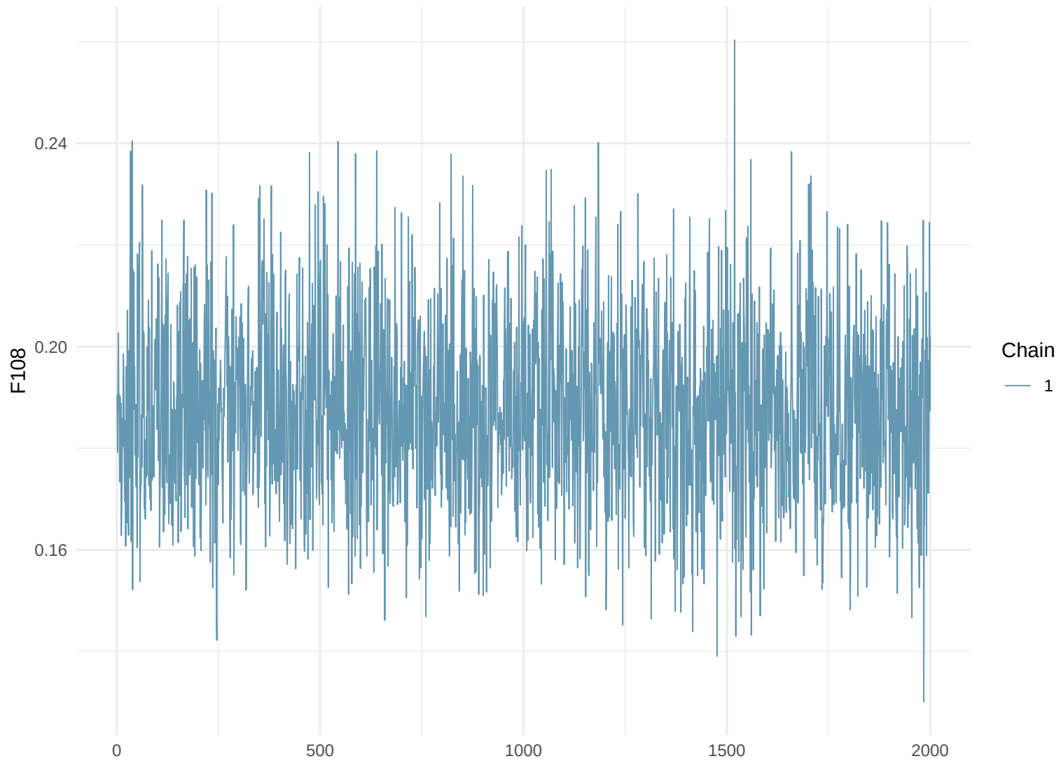
Trace Plot: F108
