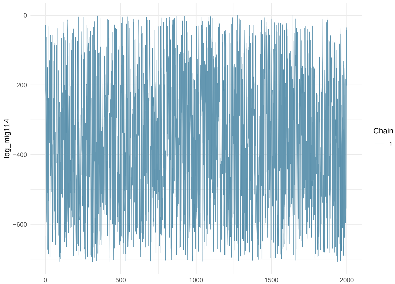
Trace Plot: log_mig114
