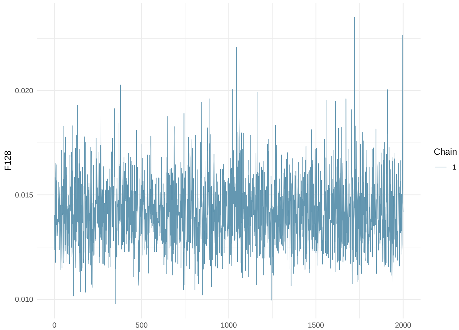
Trace Plot: F128
