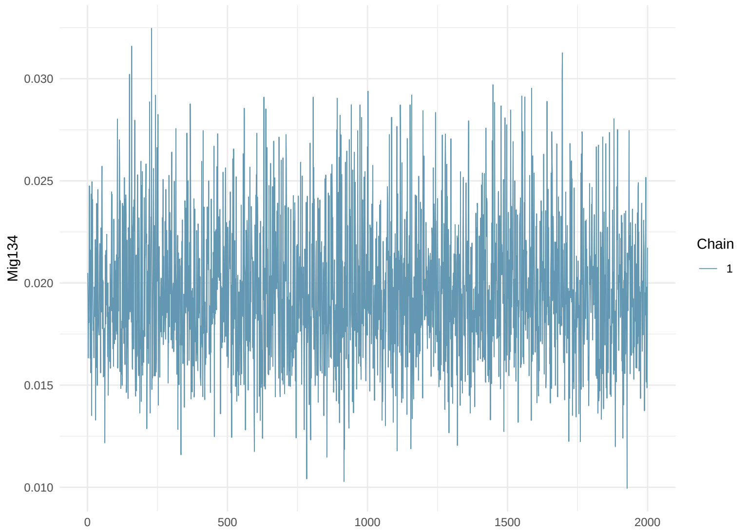
Trace Plot: Mig134
