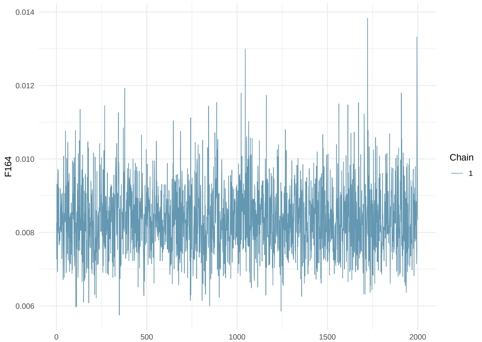
Trace Plot: F164
