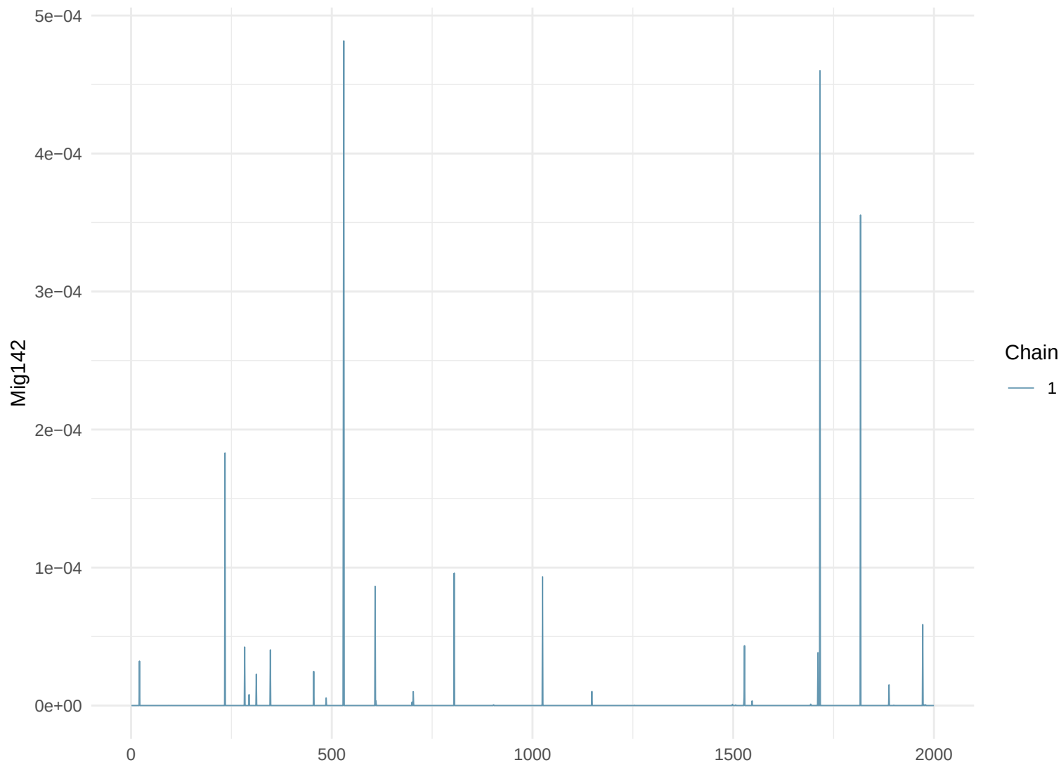
Trace Plot: Mig142
