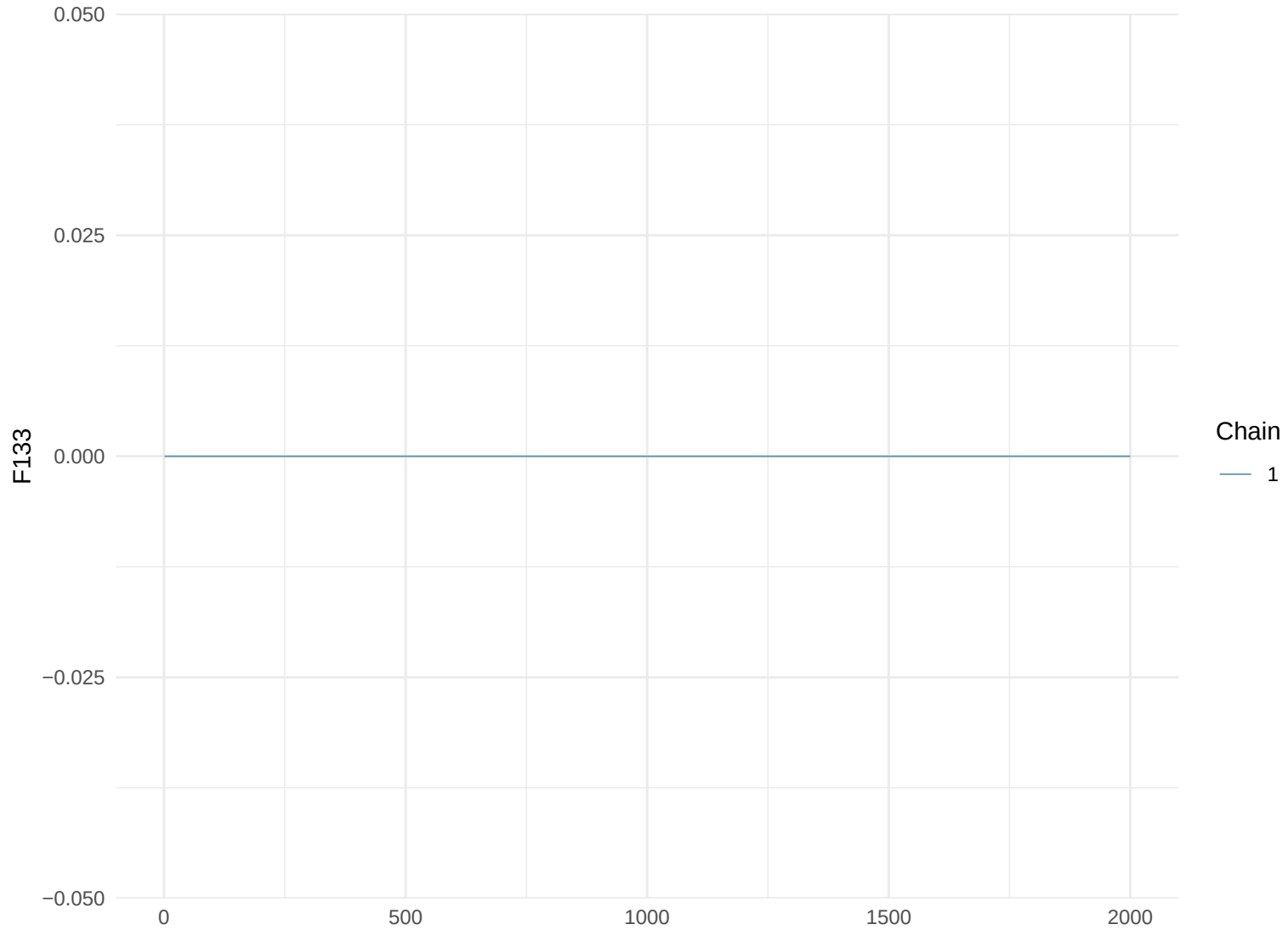
Trace Plot: F133
