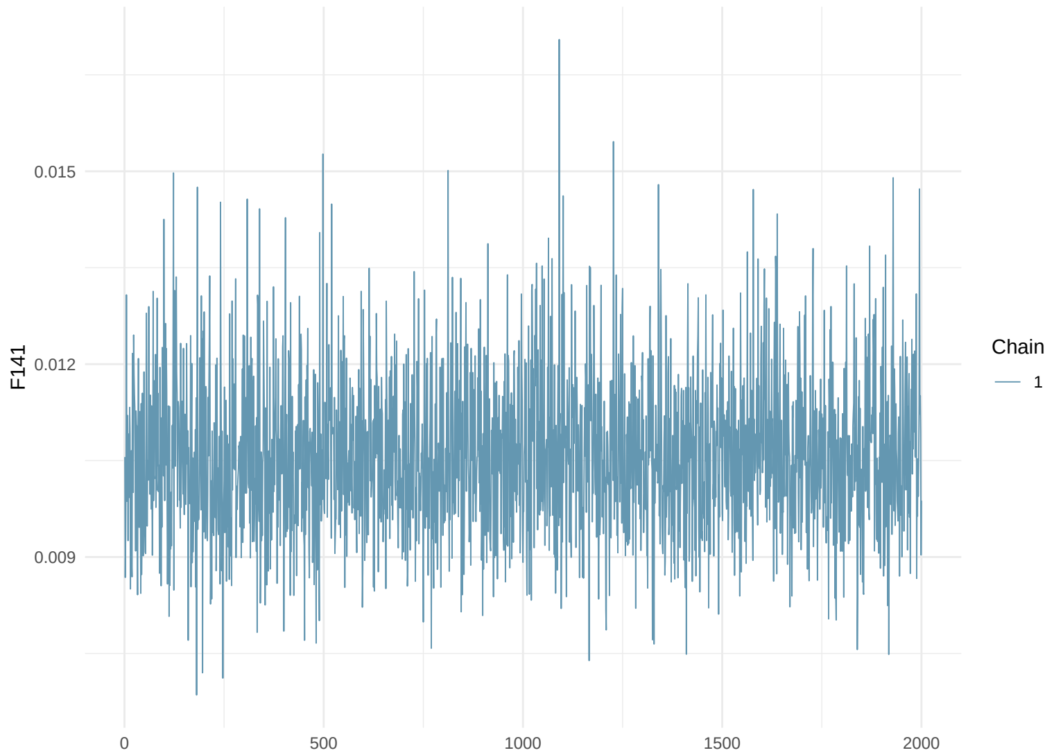
Trace Plot: F141
