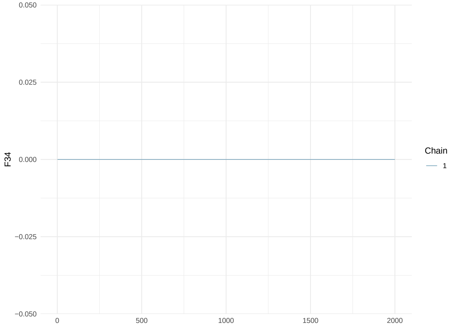
Trace Plot: F34
