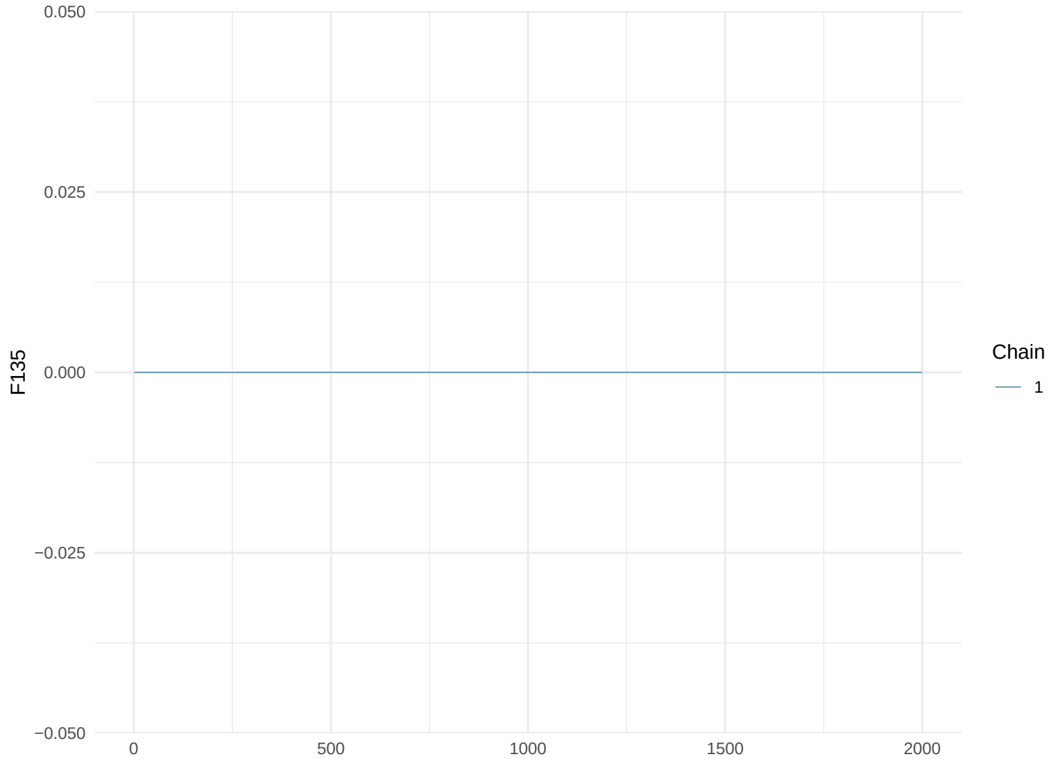
Trace Plot: F135
