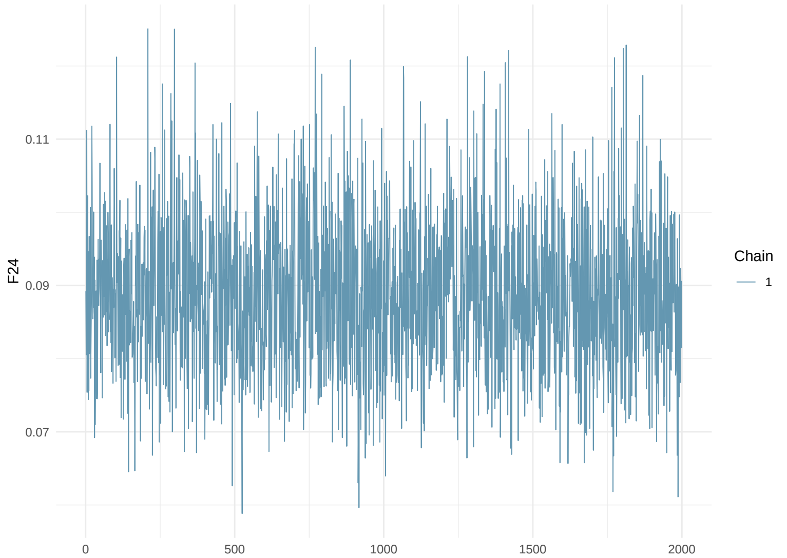
Trace Plot: F24
