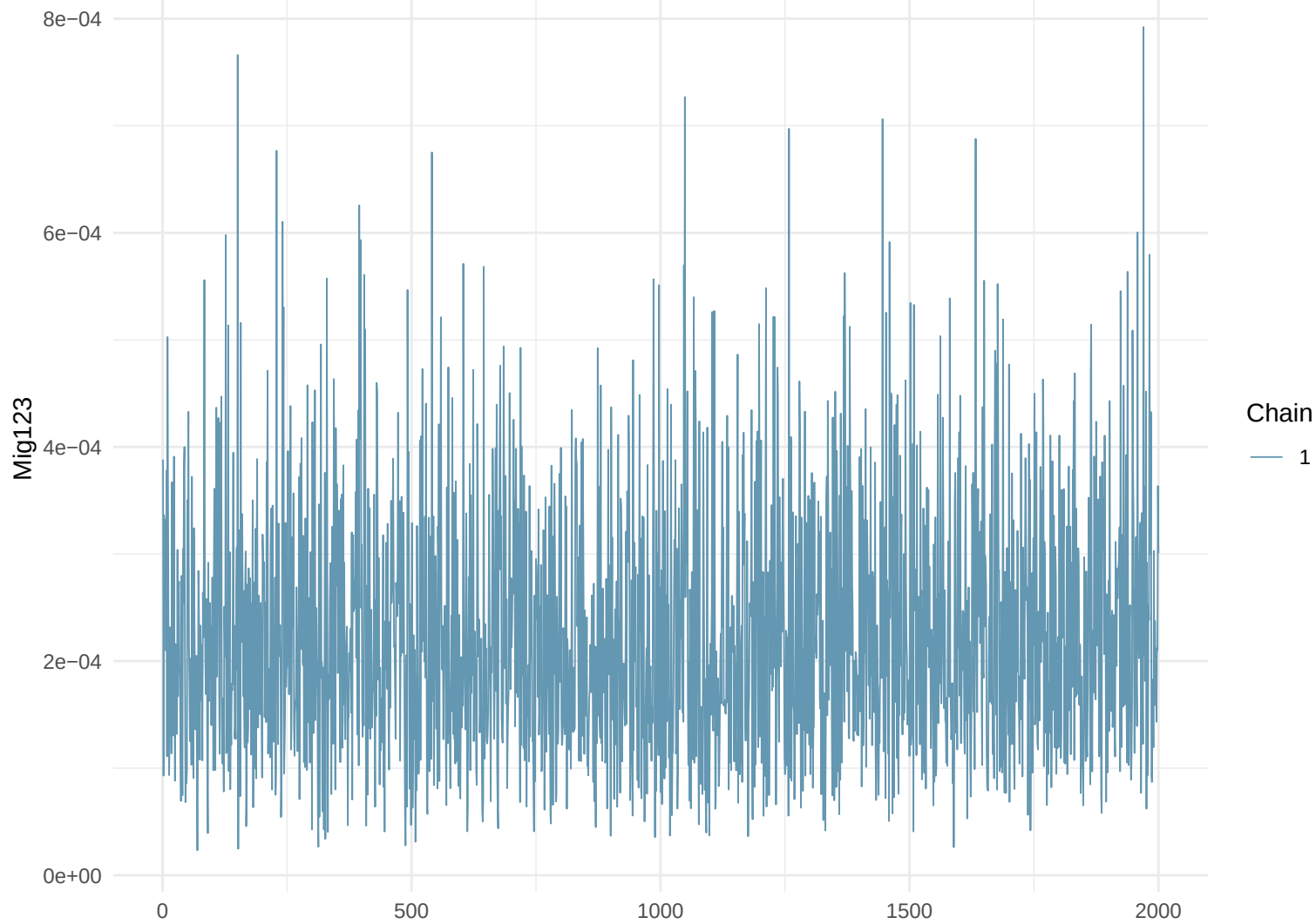
Trace Plot: Mig123
