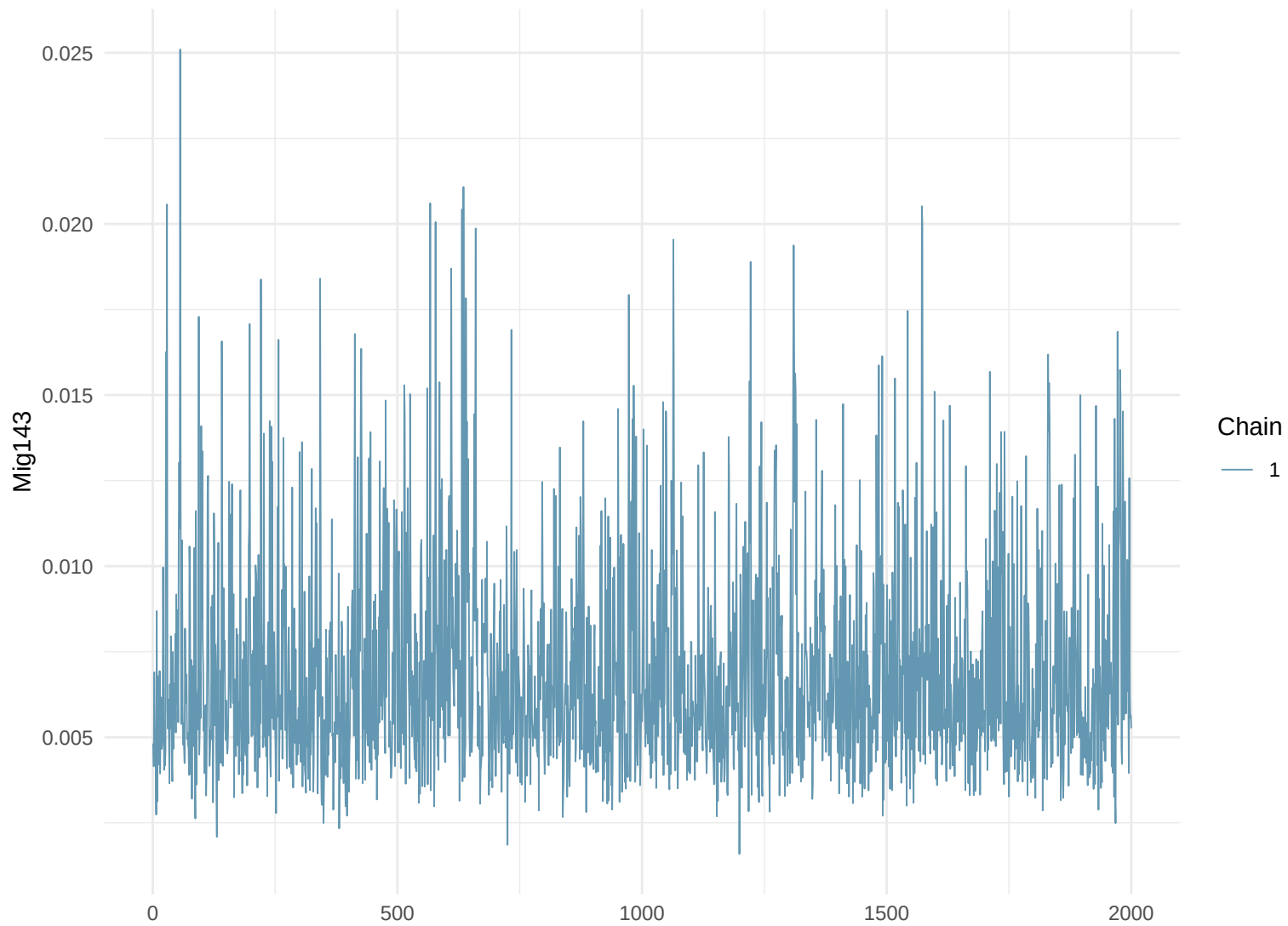
Trace Plot: Mig143
