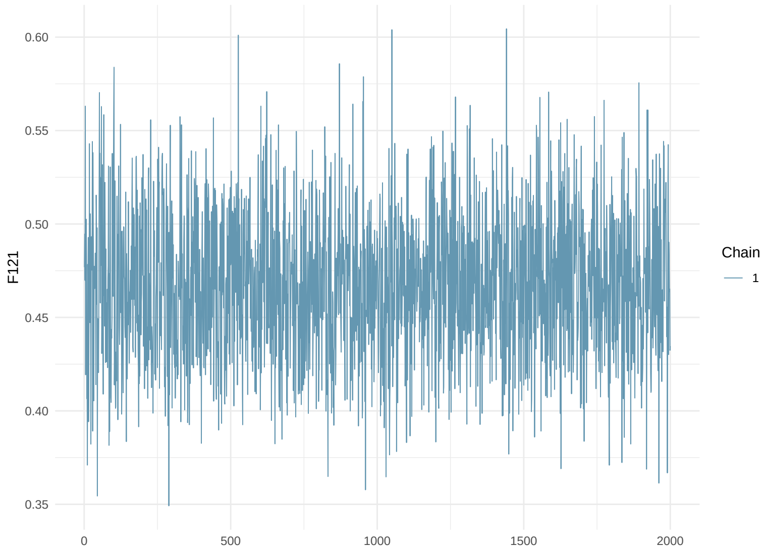
Trace Plot: F121
