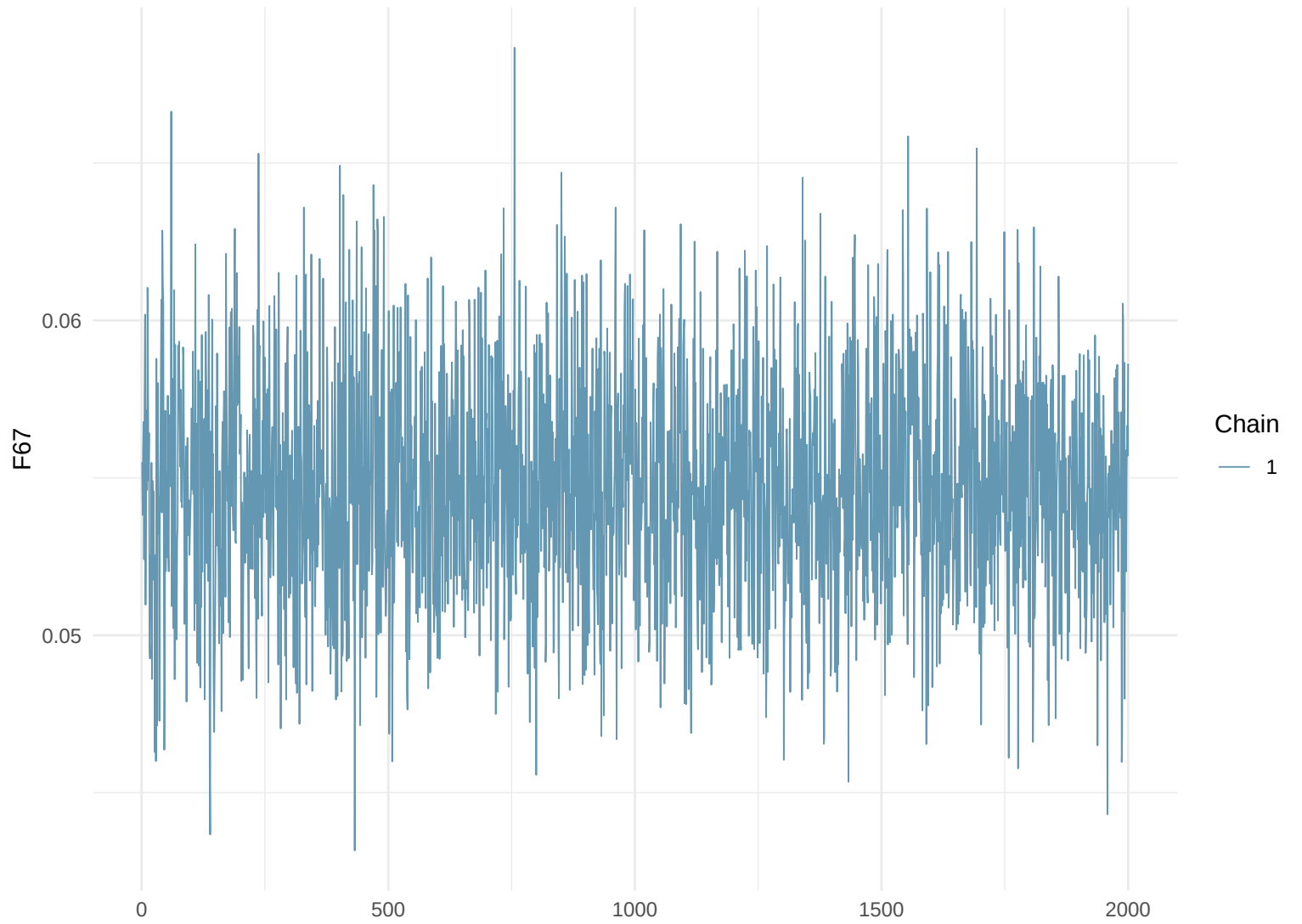
Trace Plot: F67
