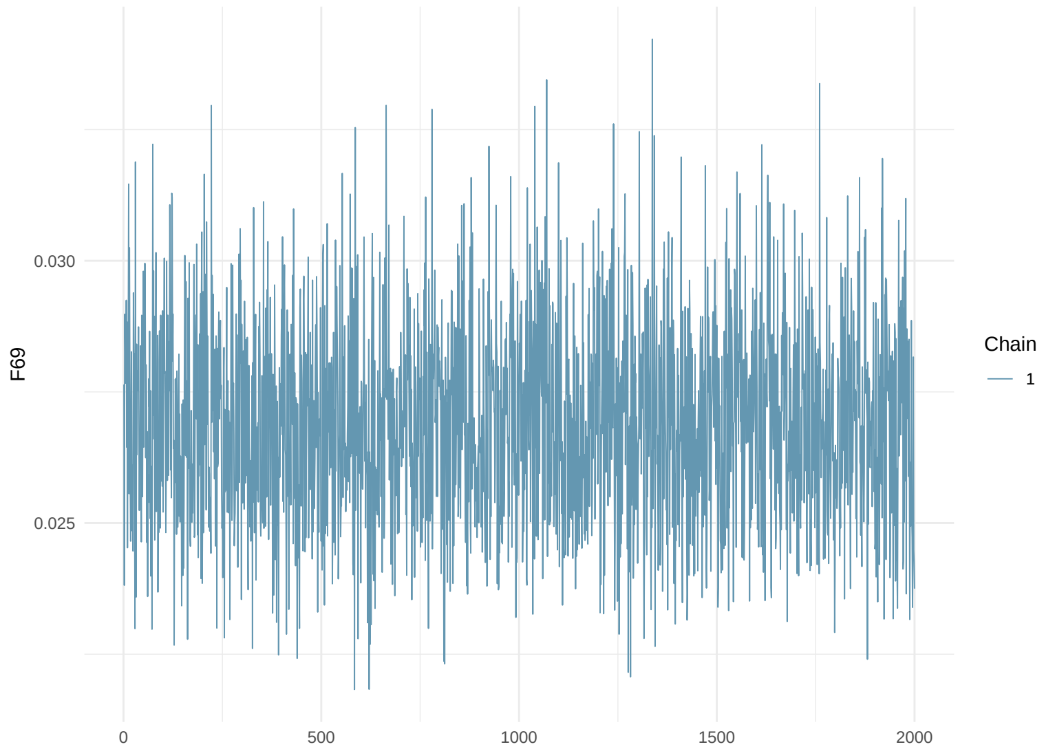
Trace Plot: F69
