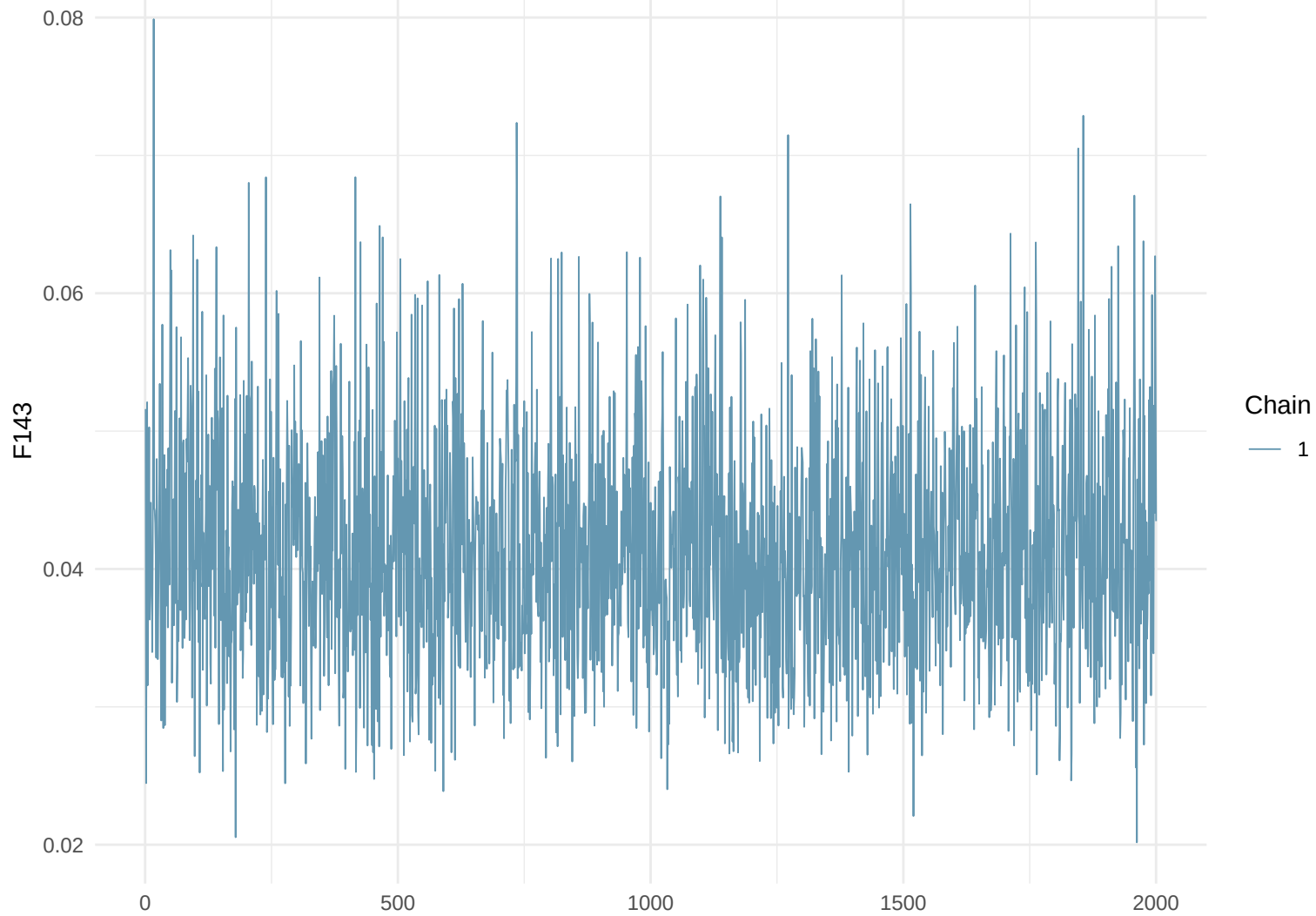
Trace Plot: F143
