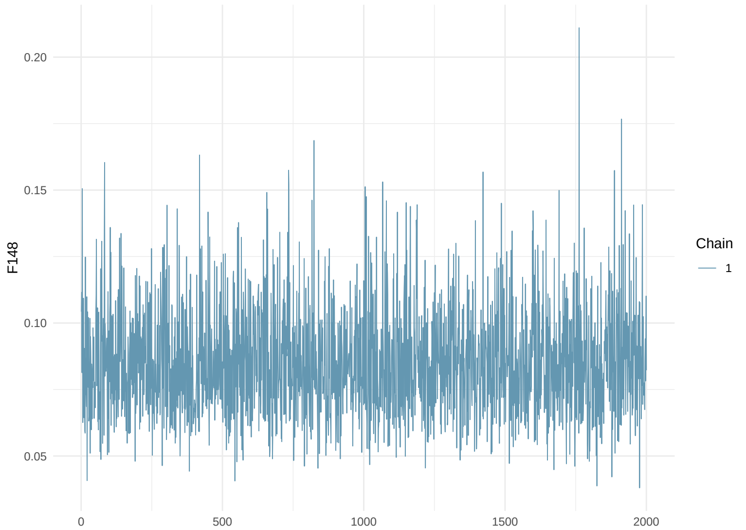
Trace Plot: F148
