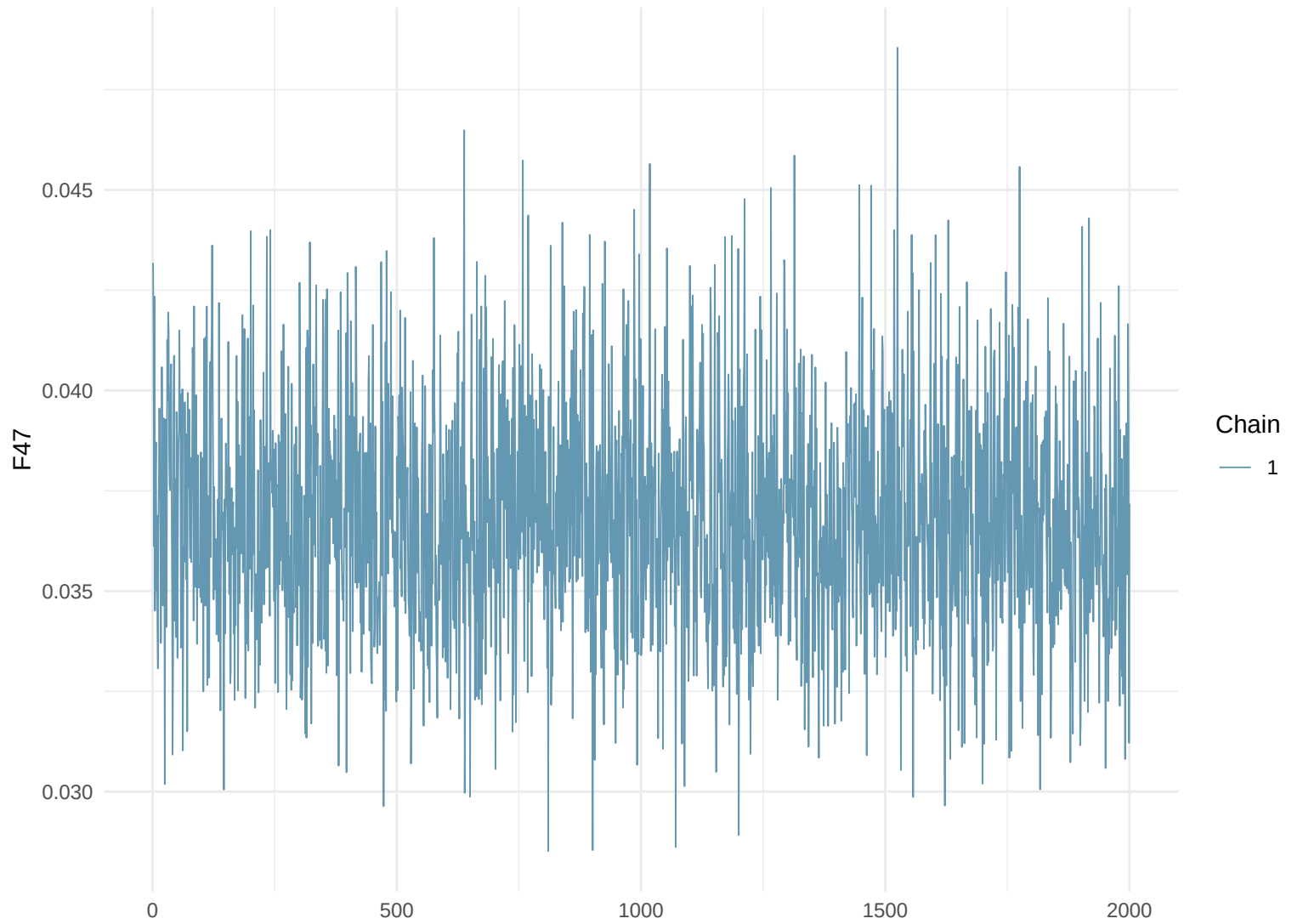
Trace Plot: F47
