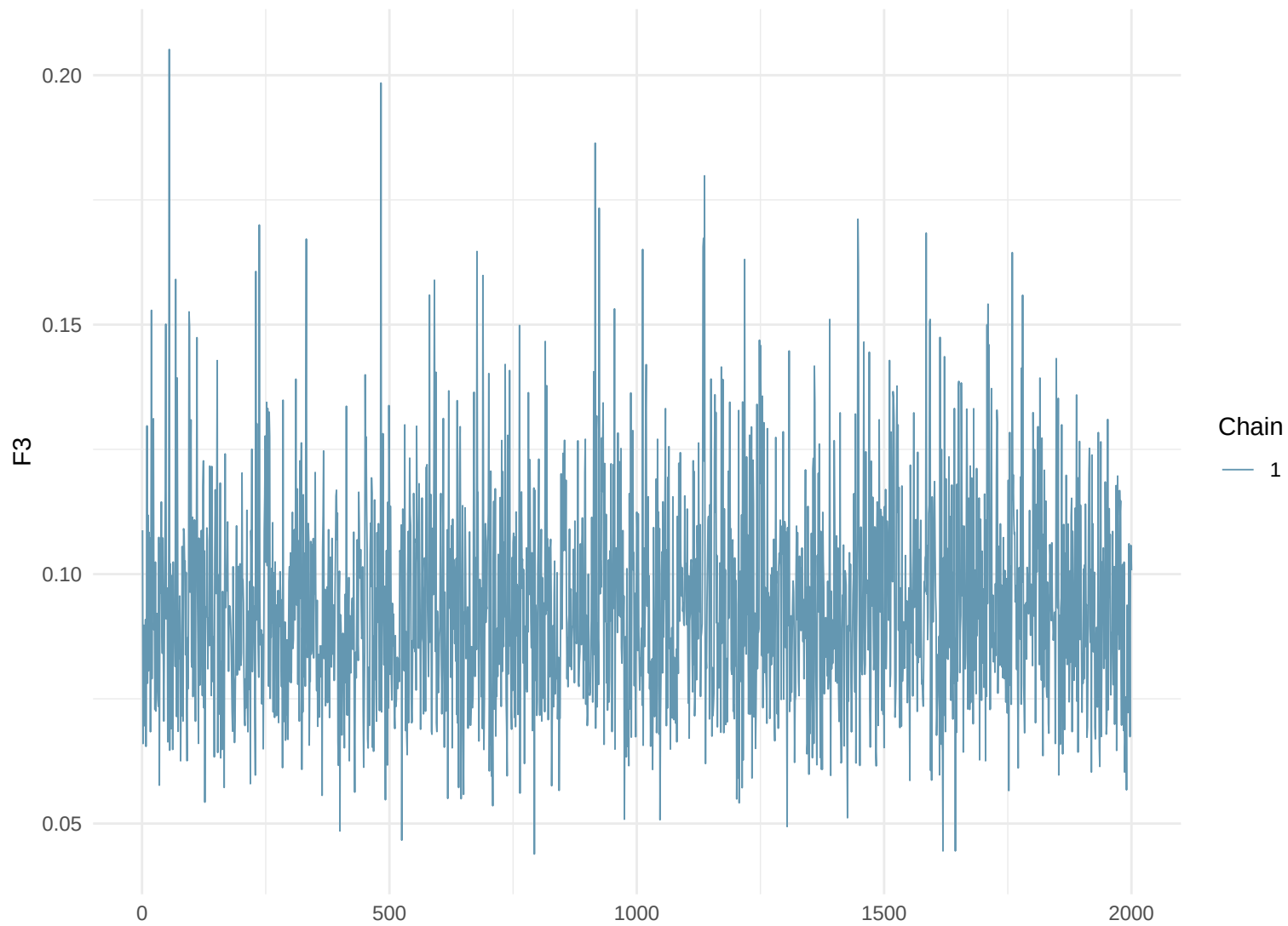
Trace Plot: F3
