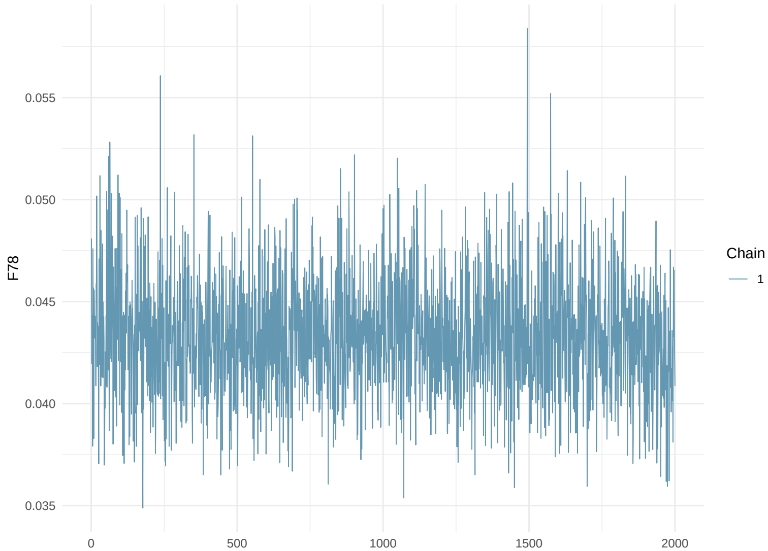
Trace Plot: F78
