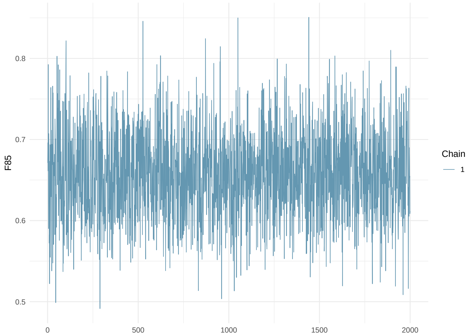
Trace Plot: F85
