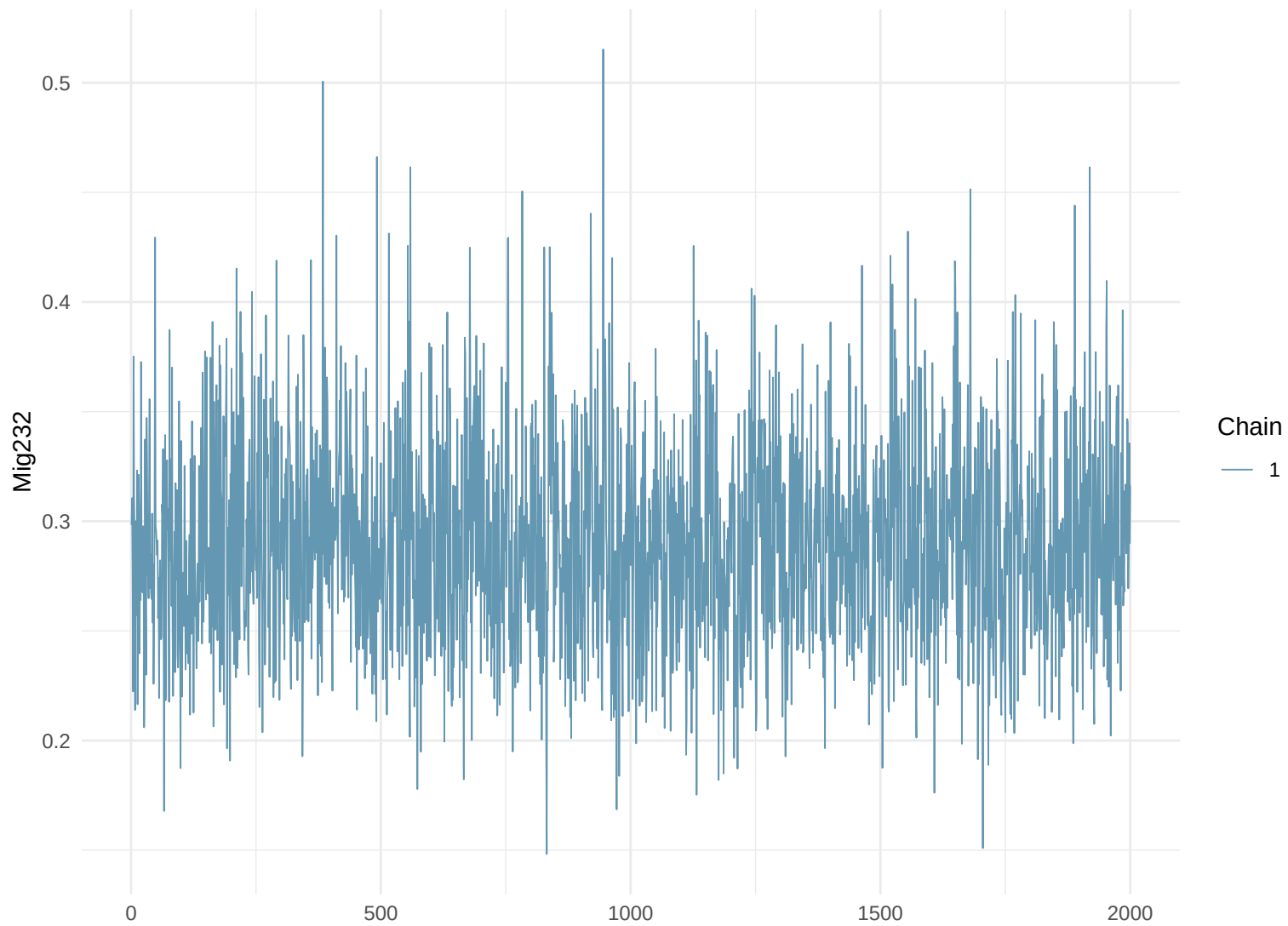
Trace Plot: Mig232
