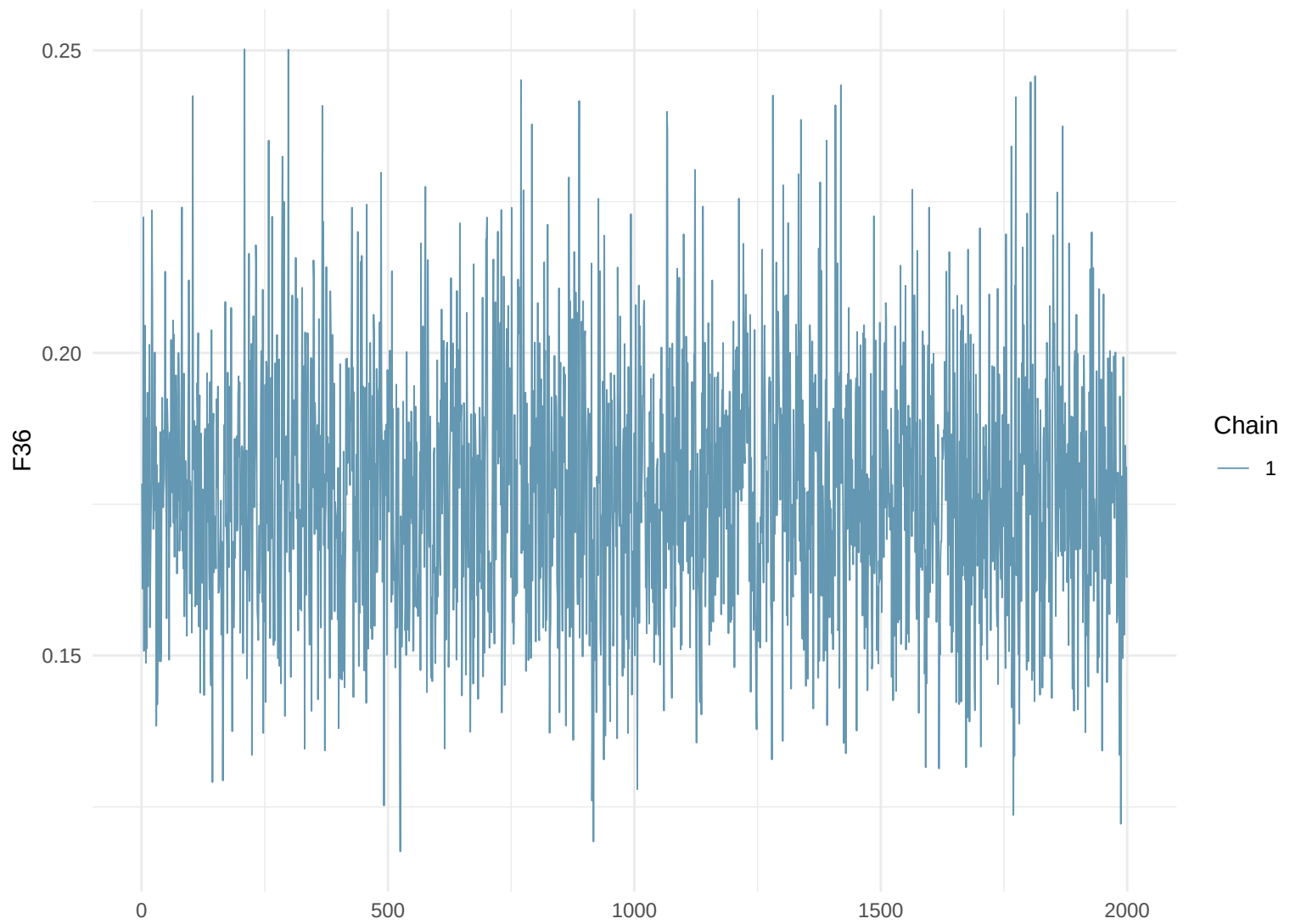
Trace Plot: F36
