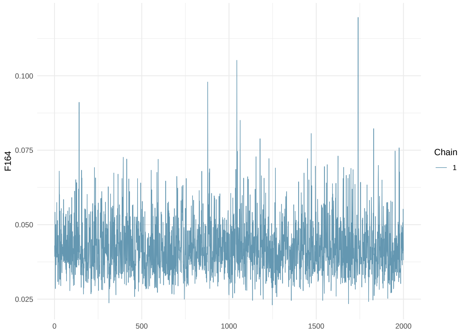
Trace Plot: F164
