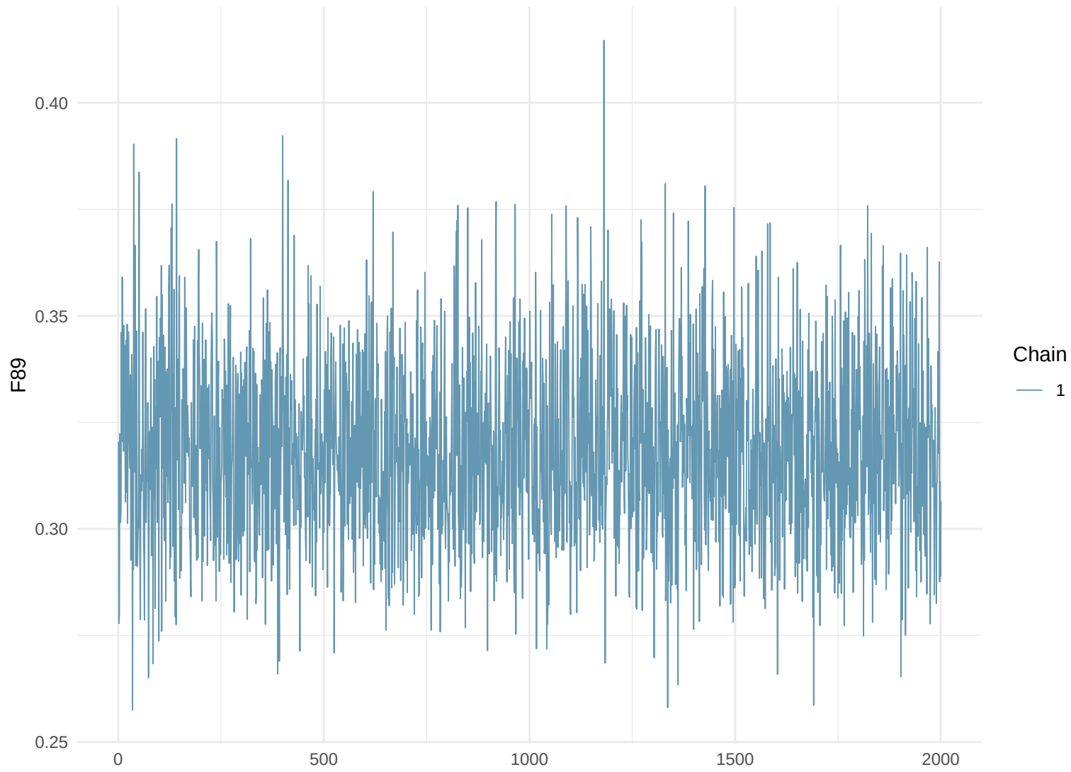
Trace Plot: F89
