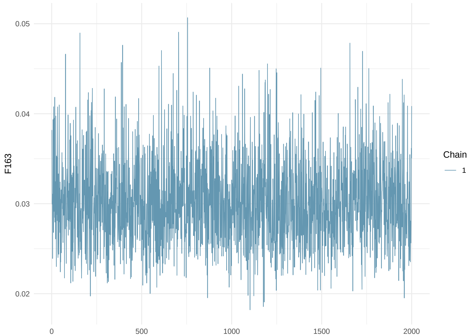
Trace Plot: F163
