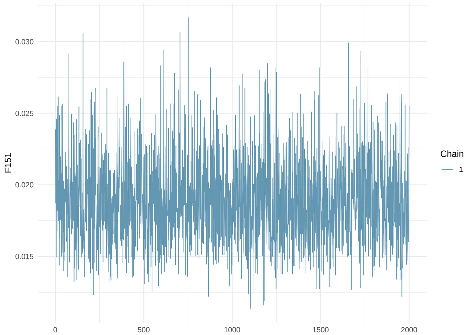
Trace Plot: F151
