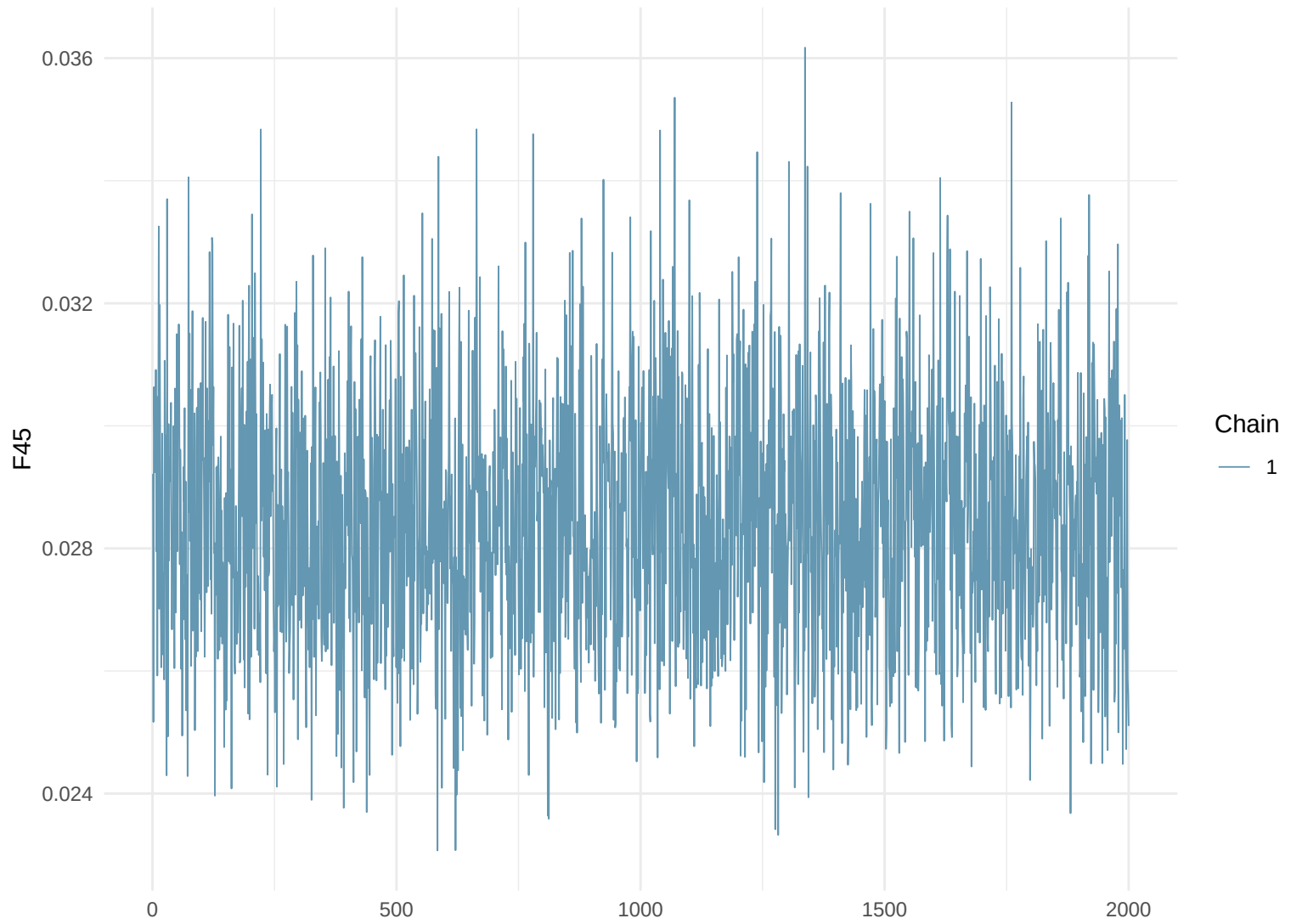
Trace Plot: F45
