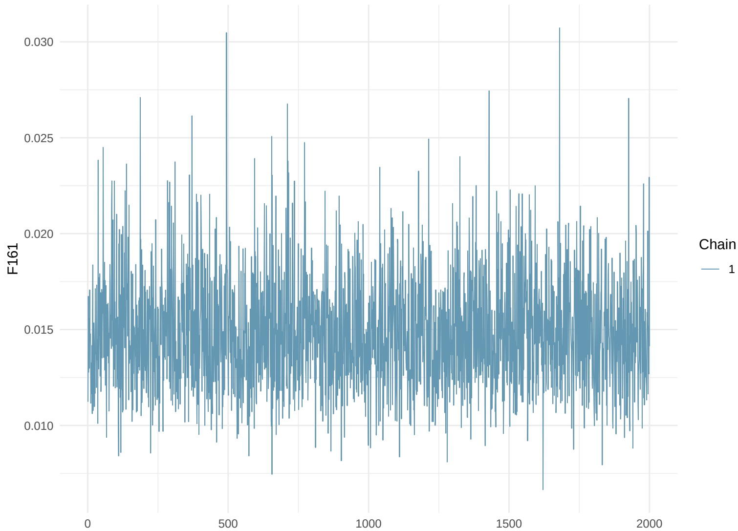
Trace Plot: F161
