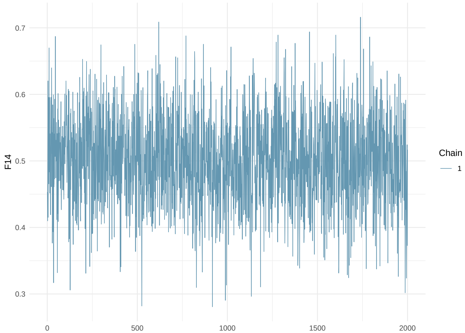
Trace Plot: F14
