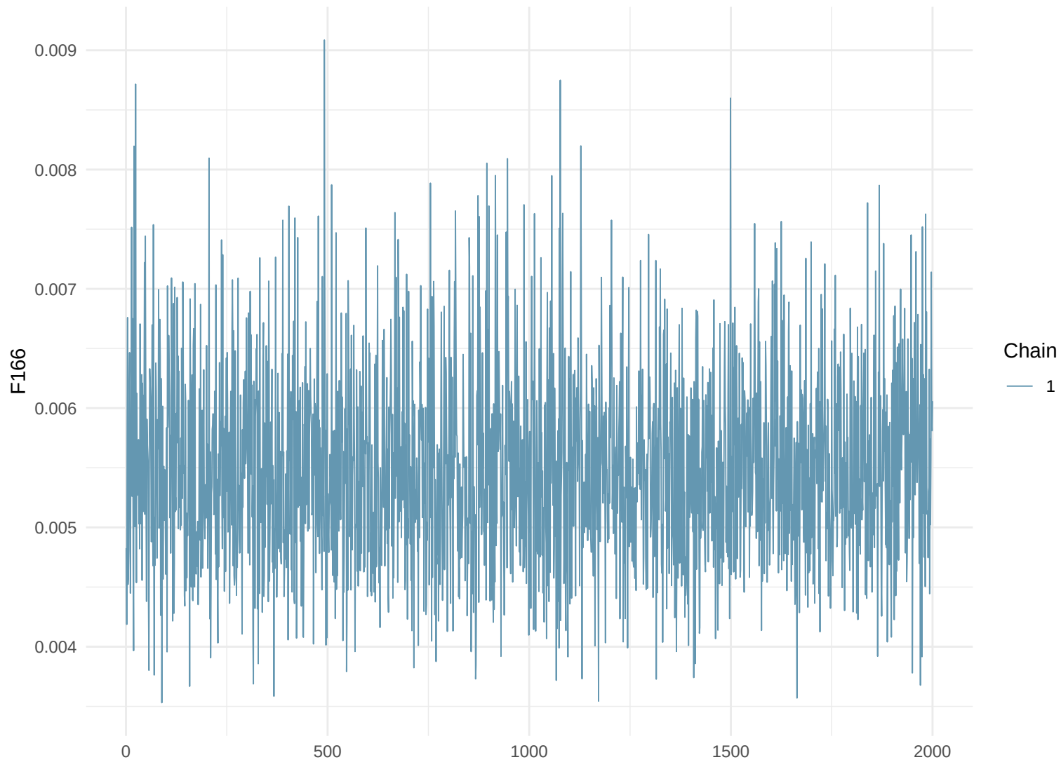
Trace Plot: F166
