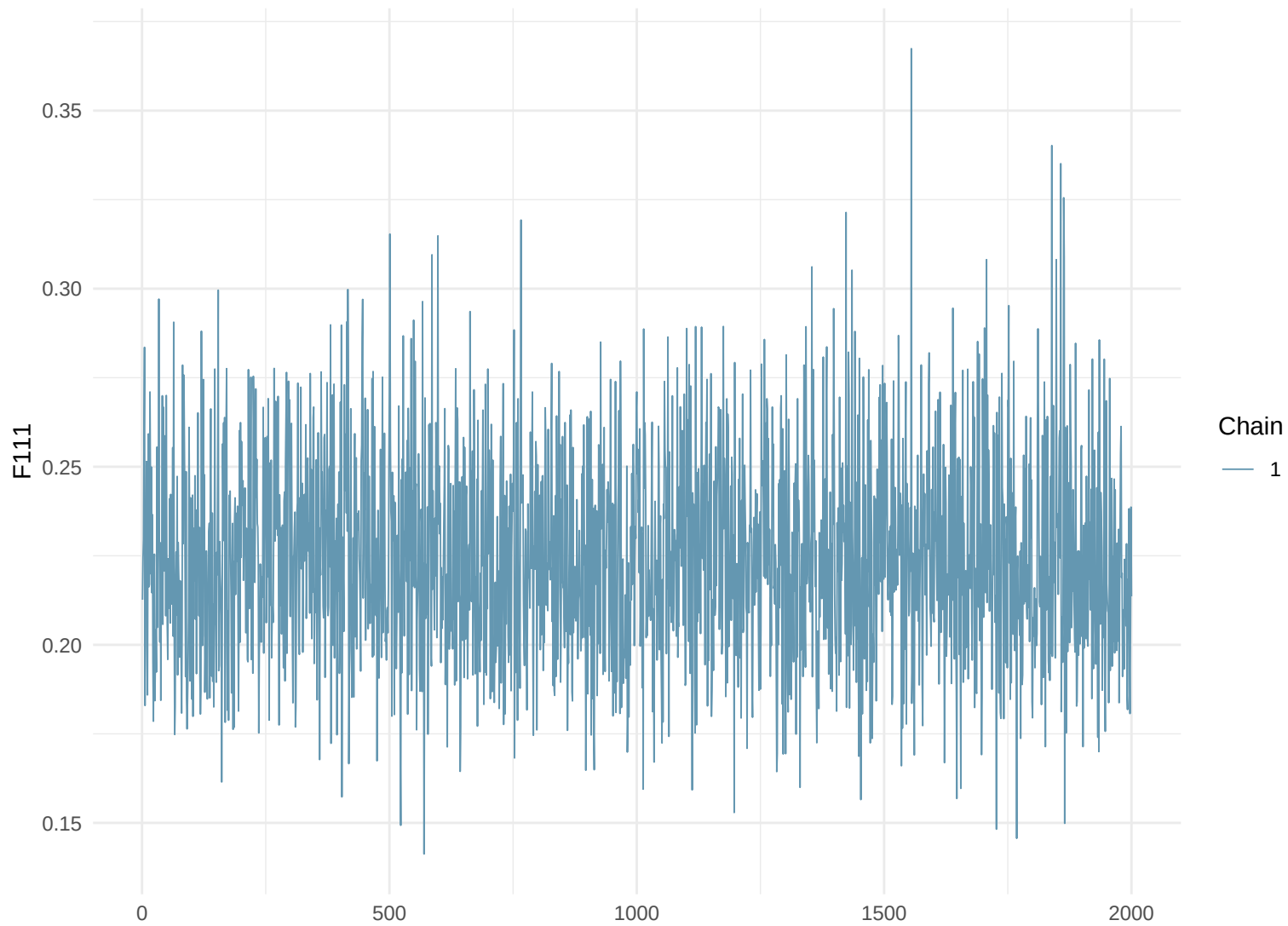
Trace Plot: F111
