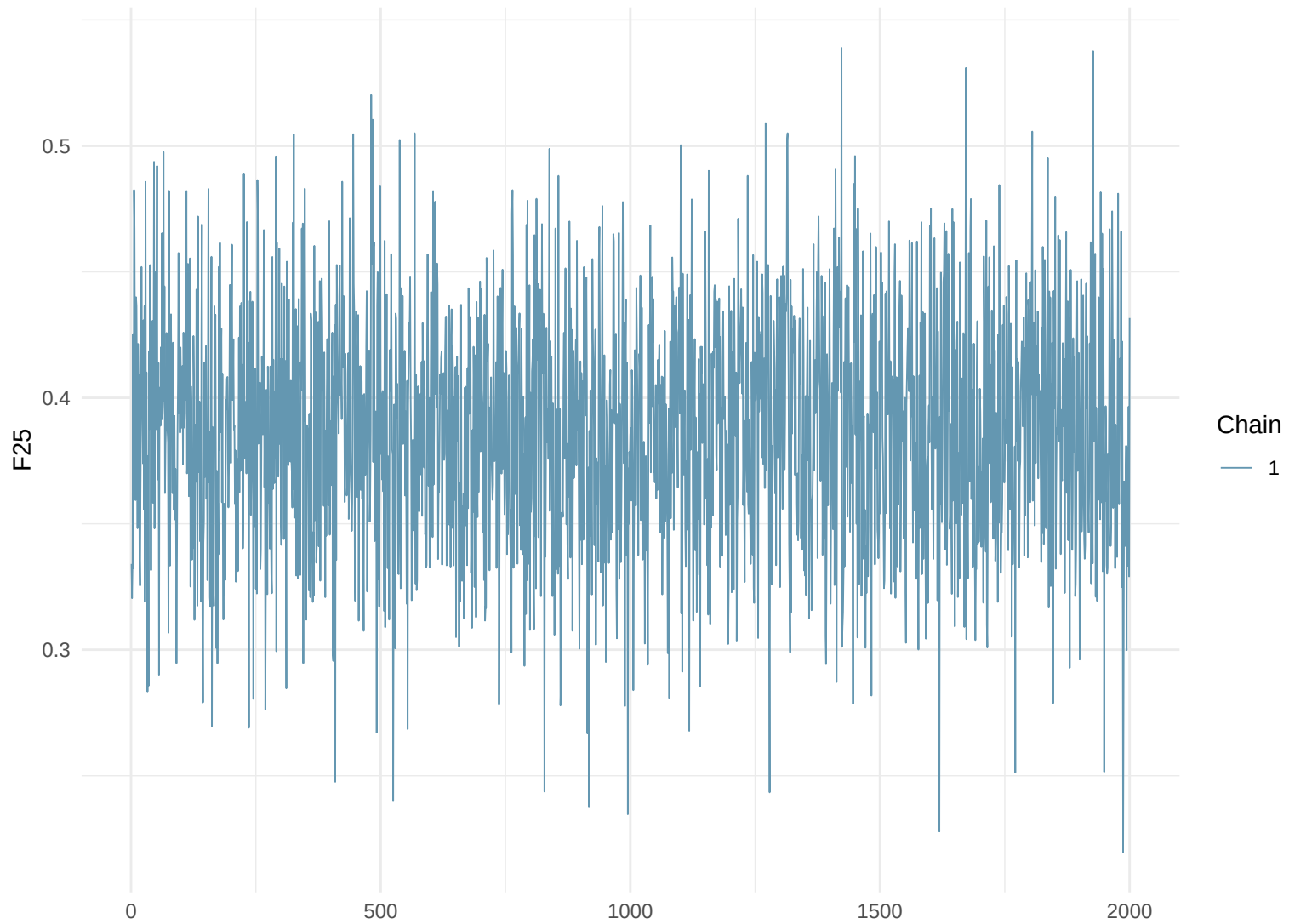
Trace Plot: F25
