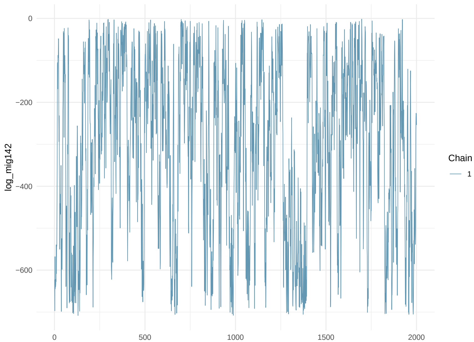
Trace Plot: log_mig142
