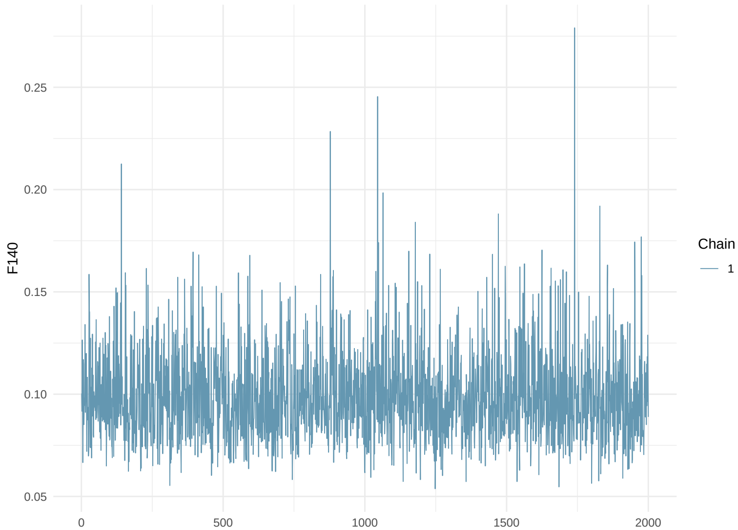
Trace Plot: F140
