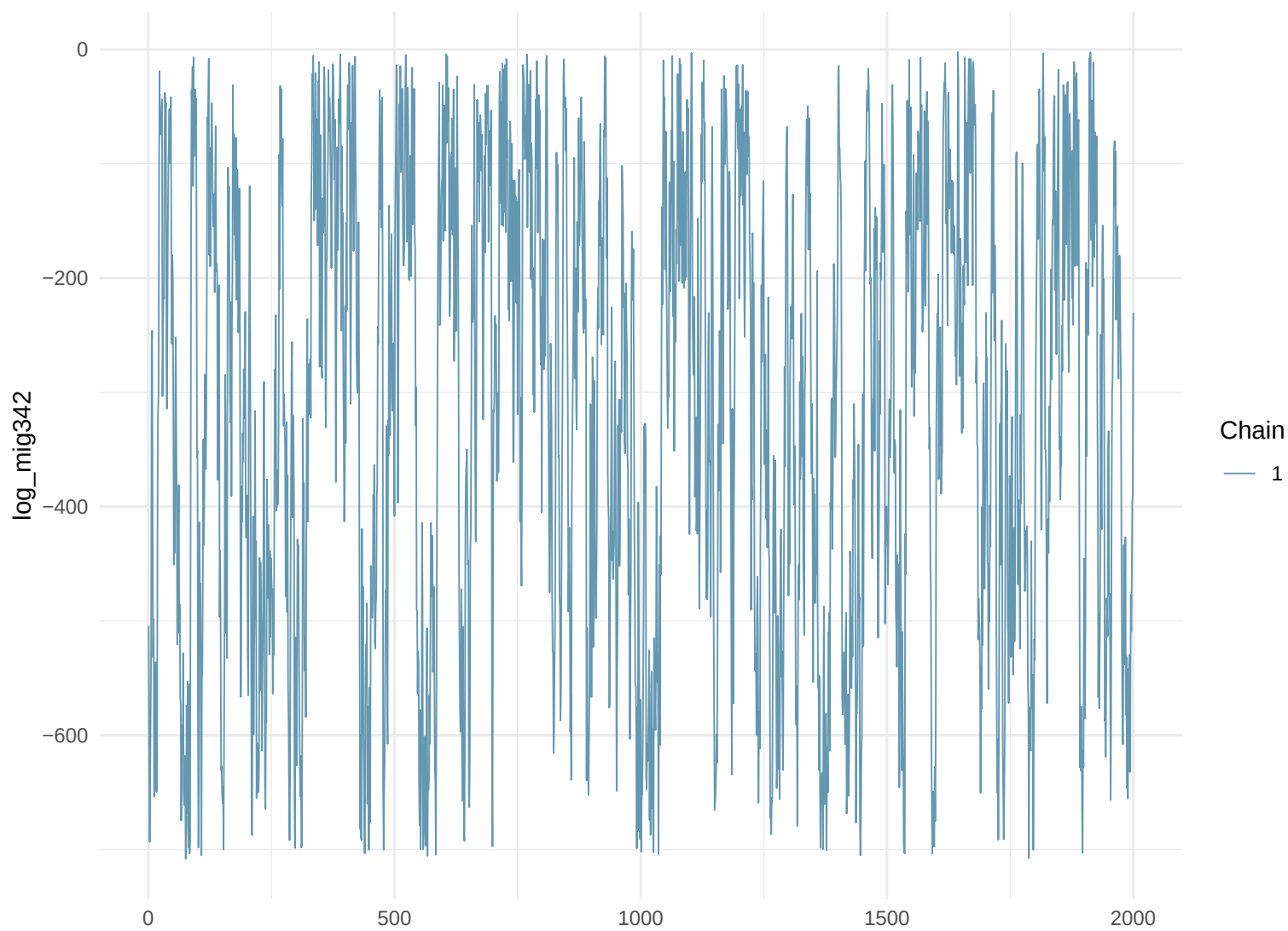
Trace Plot: log_mig342
