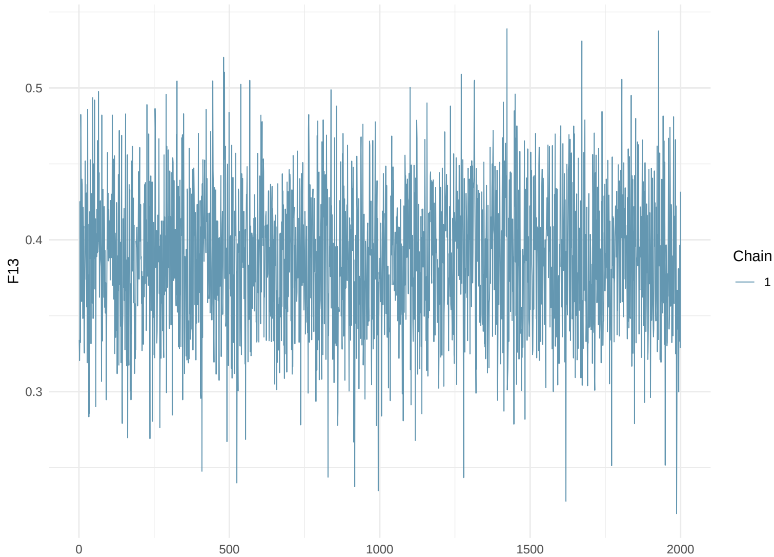
Trace Plot: F13
