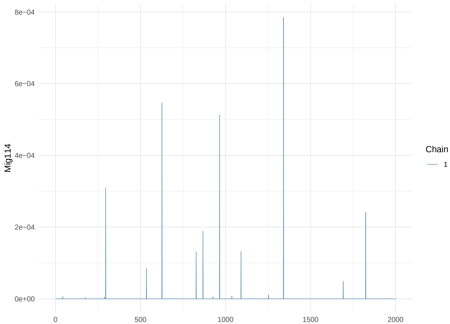
Trace Plot: Mig114
