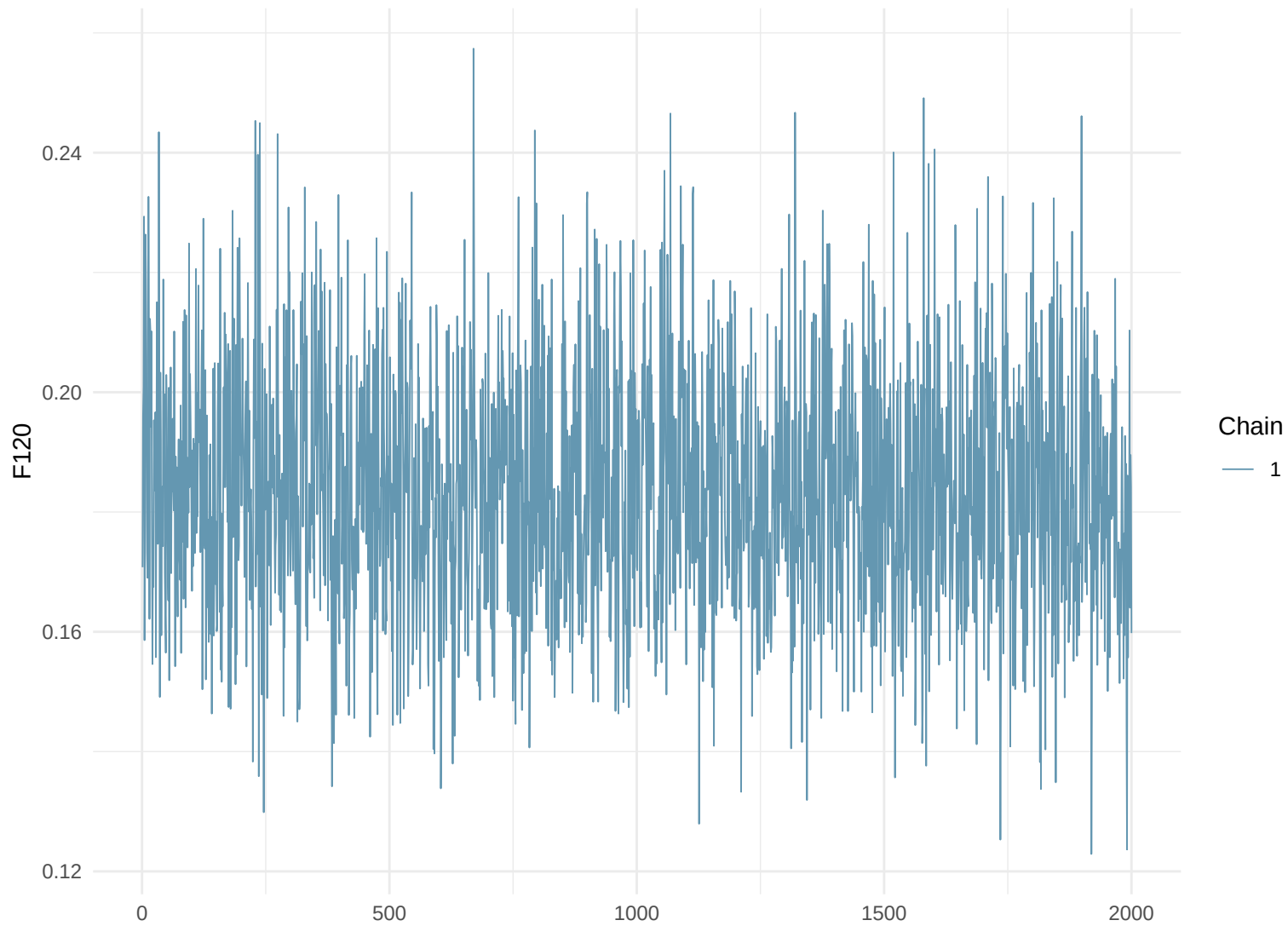
Trace Plot: F120
