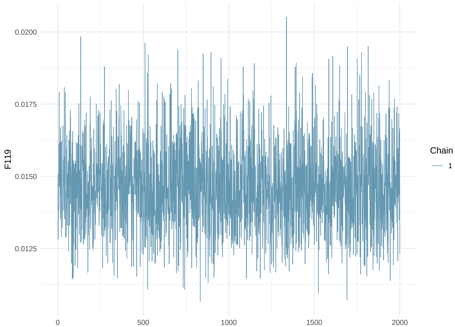
Trace Plot: F119
