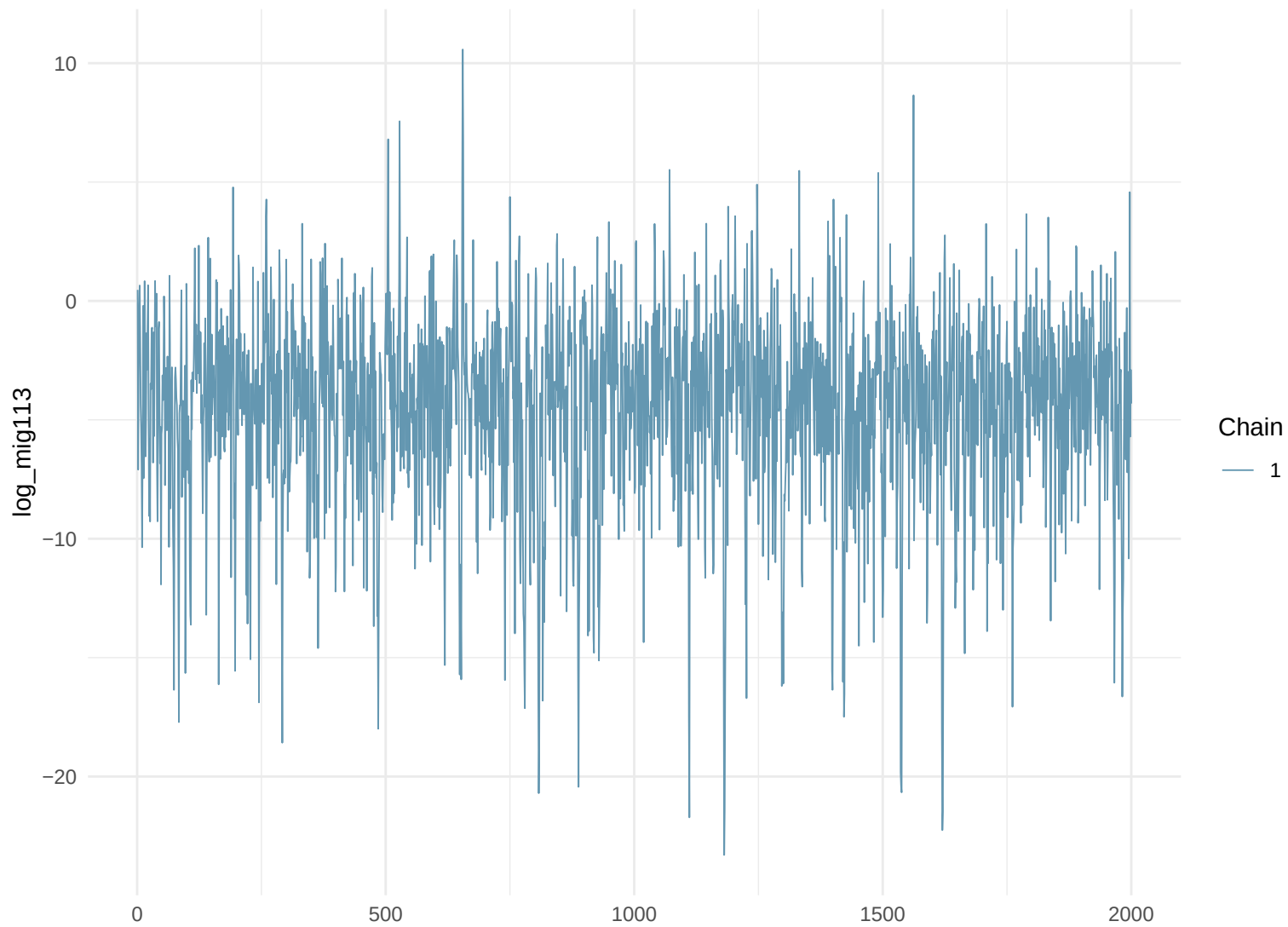
Trace Plot: log_mig113
