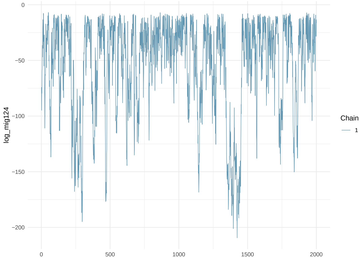
Trace Plot: log_mig124
