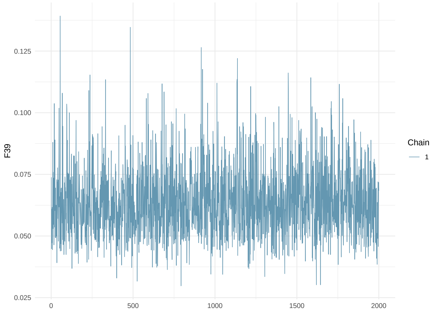
Trace Plot: F39
