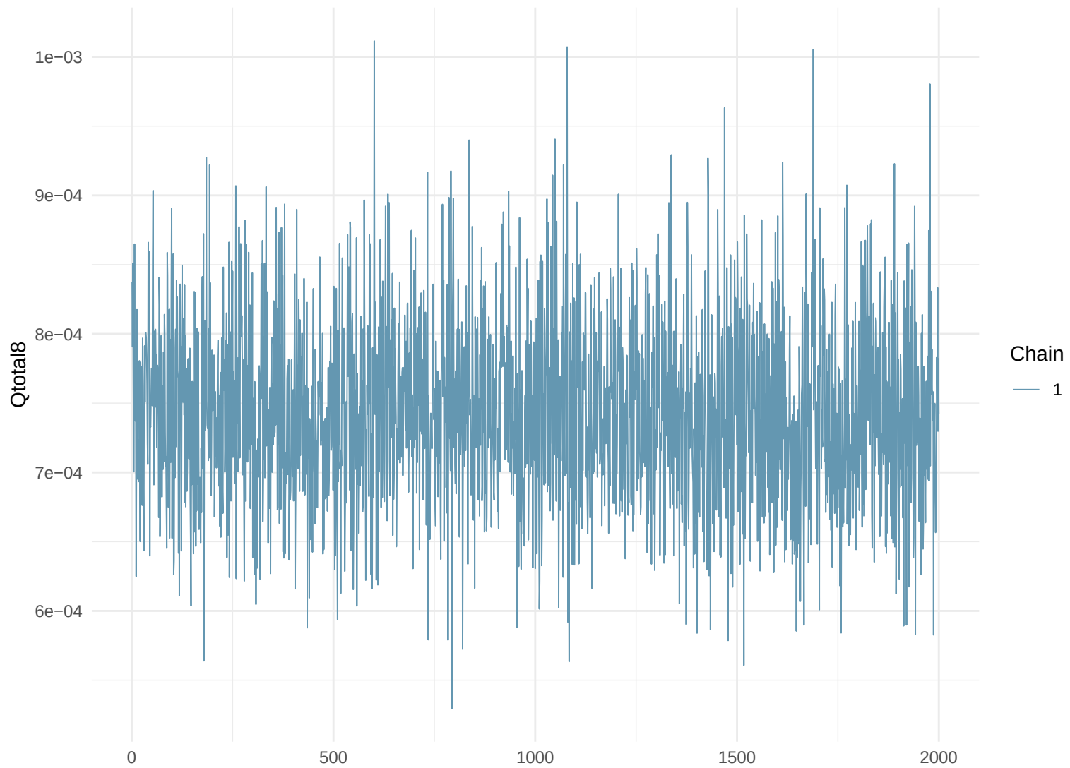
Trace Plot: Qtotal8
