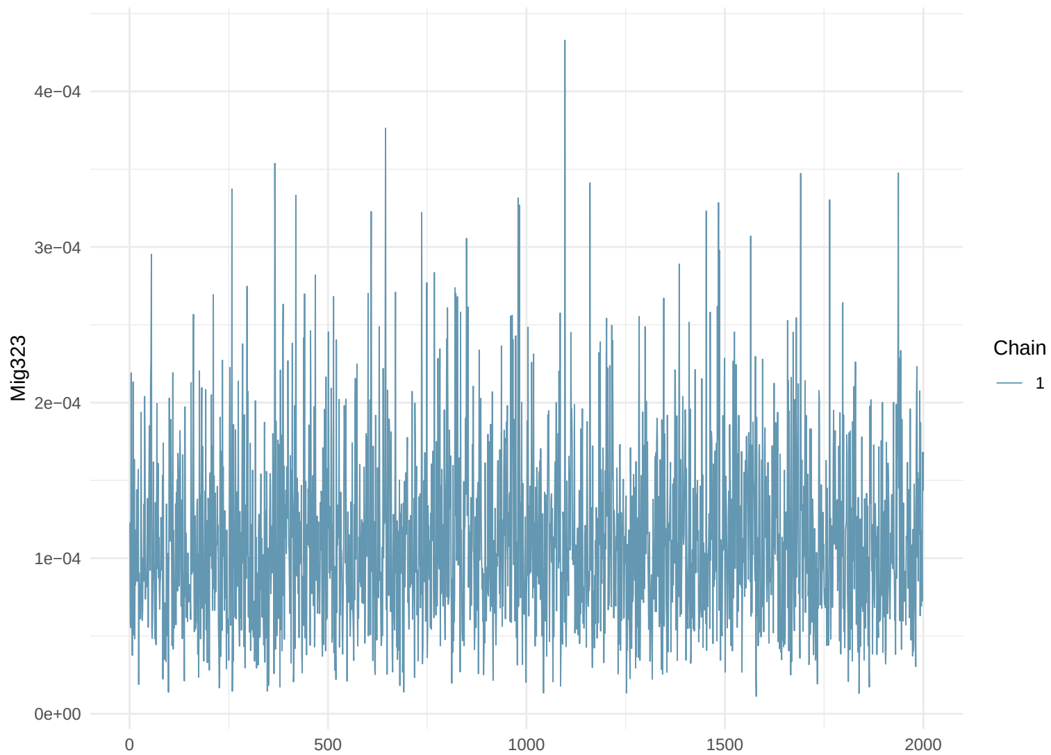
Trace Plot: Mig323
