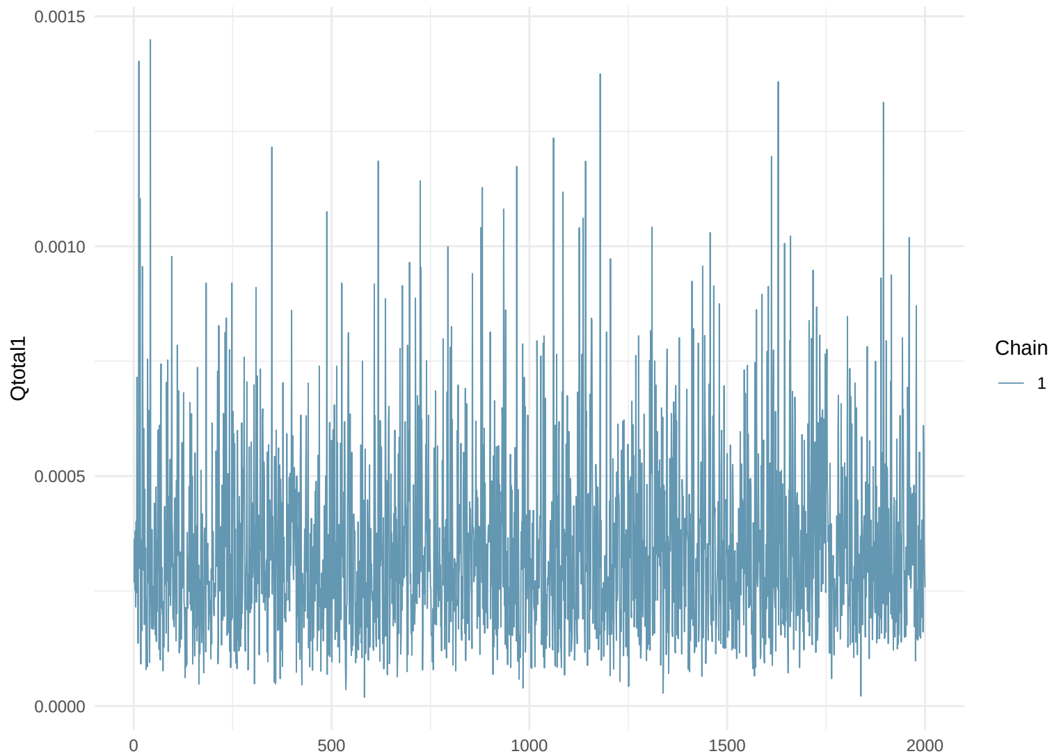
Trace Plot: Qtotal1
