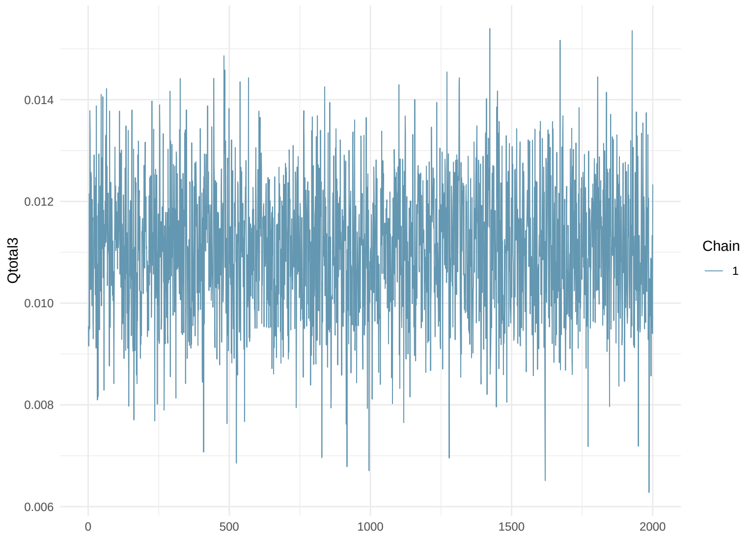
Trace Plot: Qtotal3
