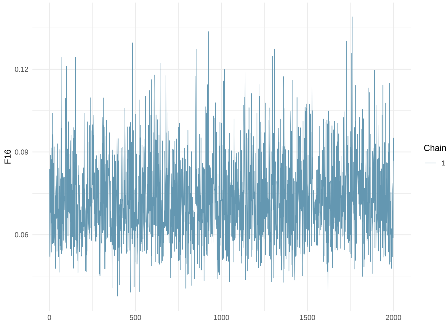
Trace Plot: F16
