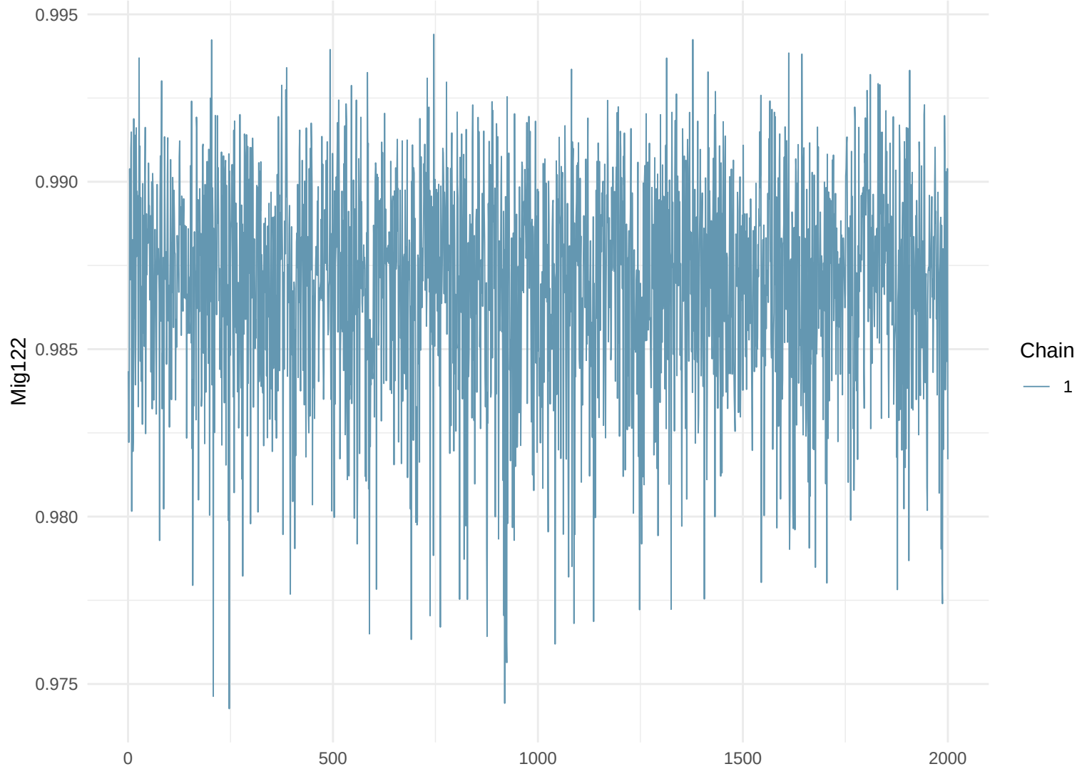
Trace Plot: Mig122
