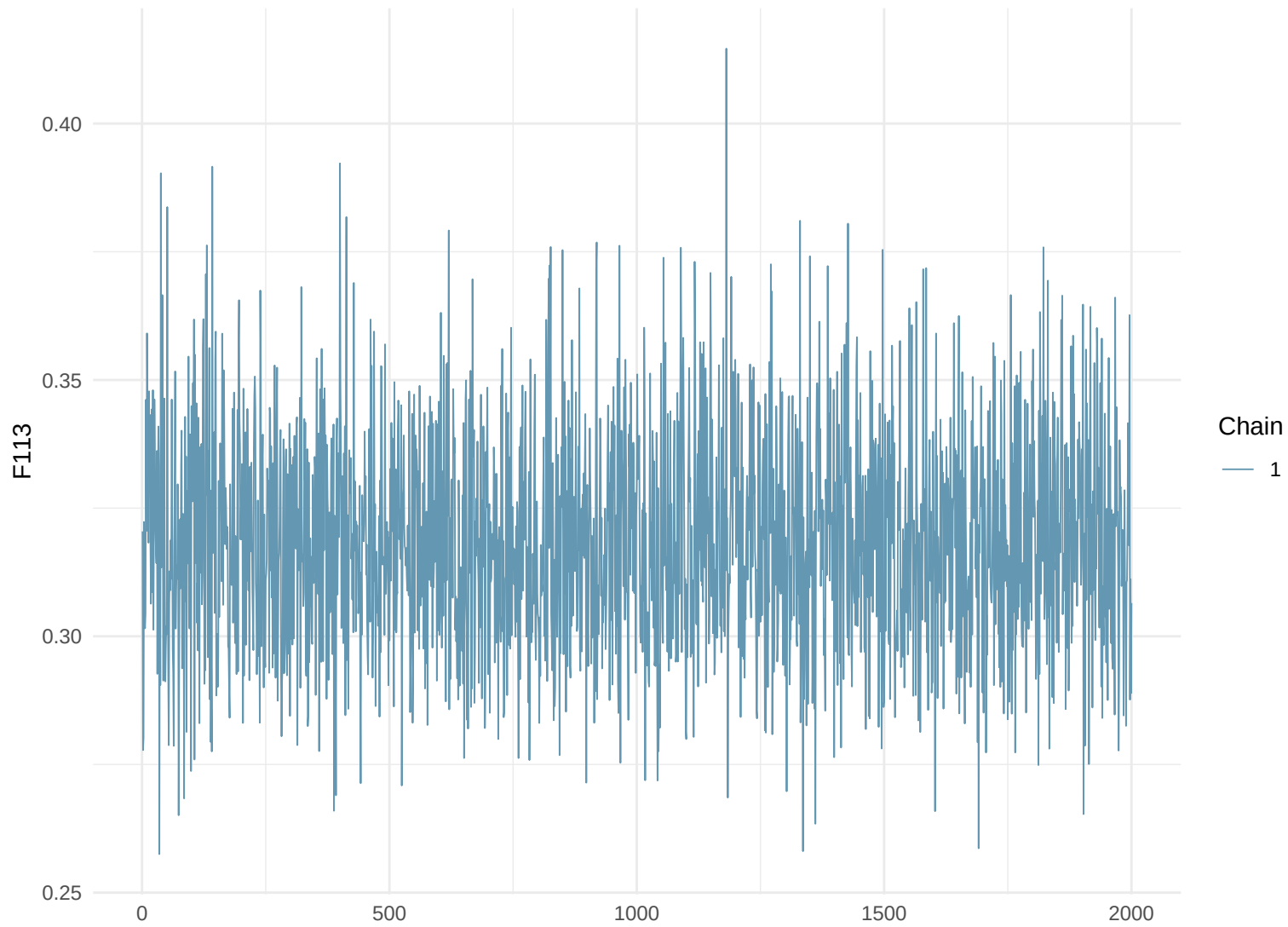
Trace Plot: F113
