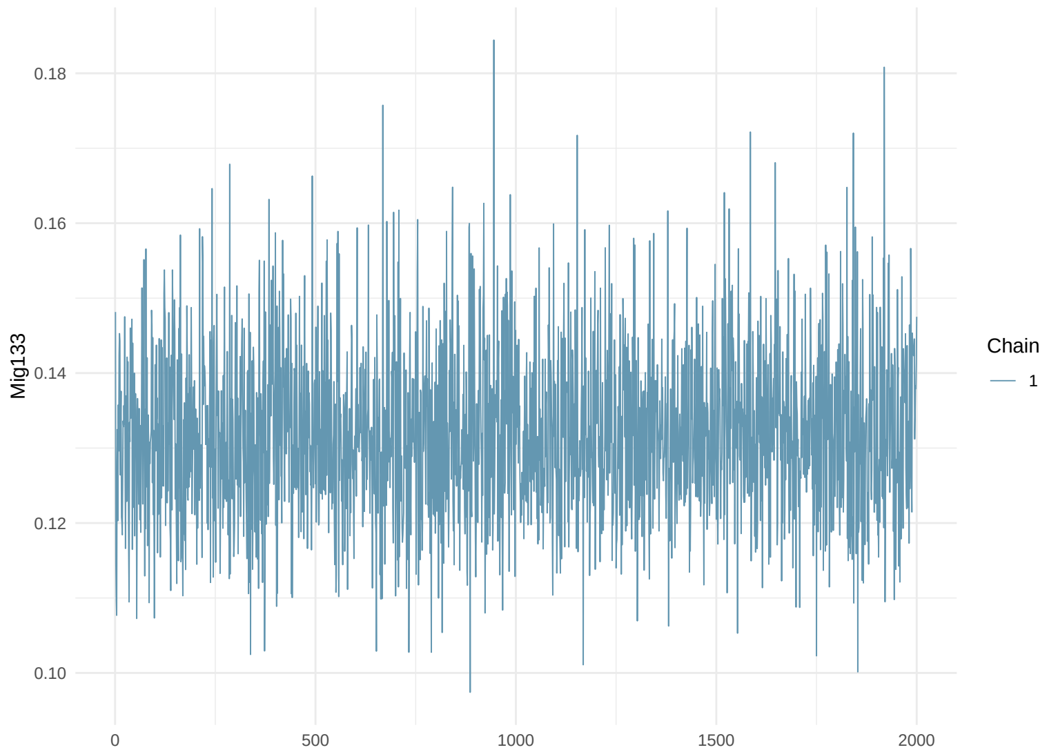
Trace Plot: Mig133
