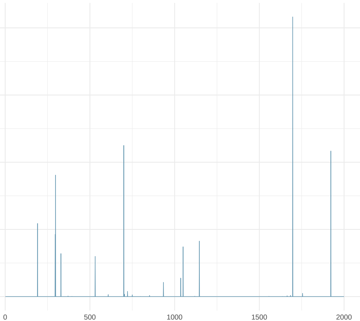
Trace Plot: Mig142
