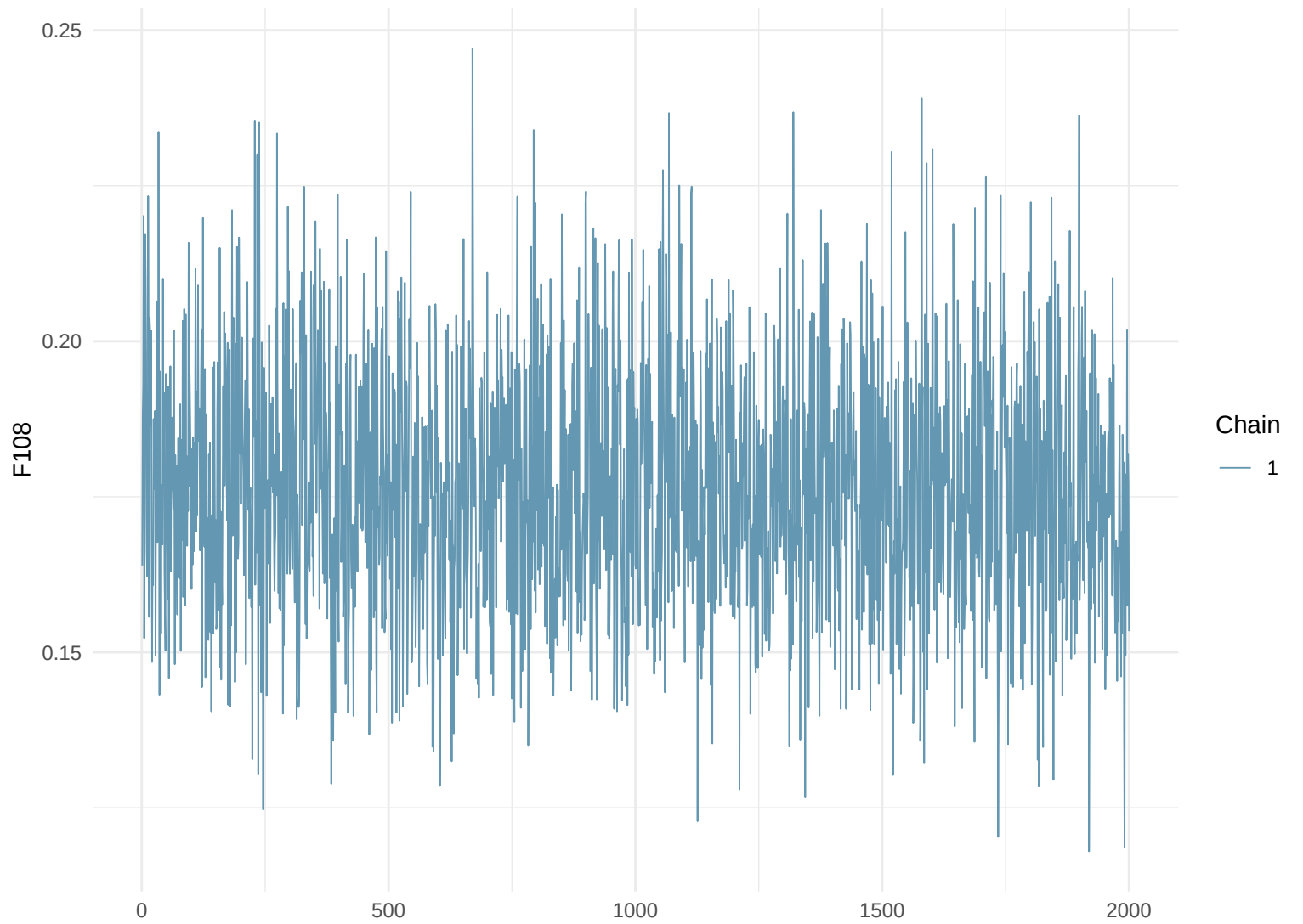
Trace Plot: F108
