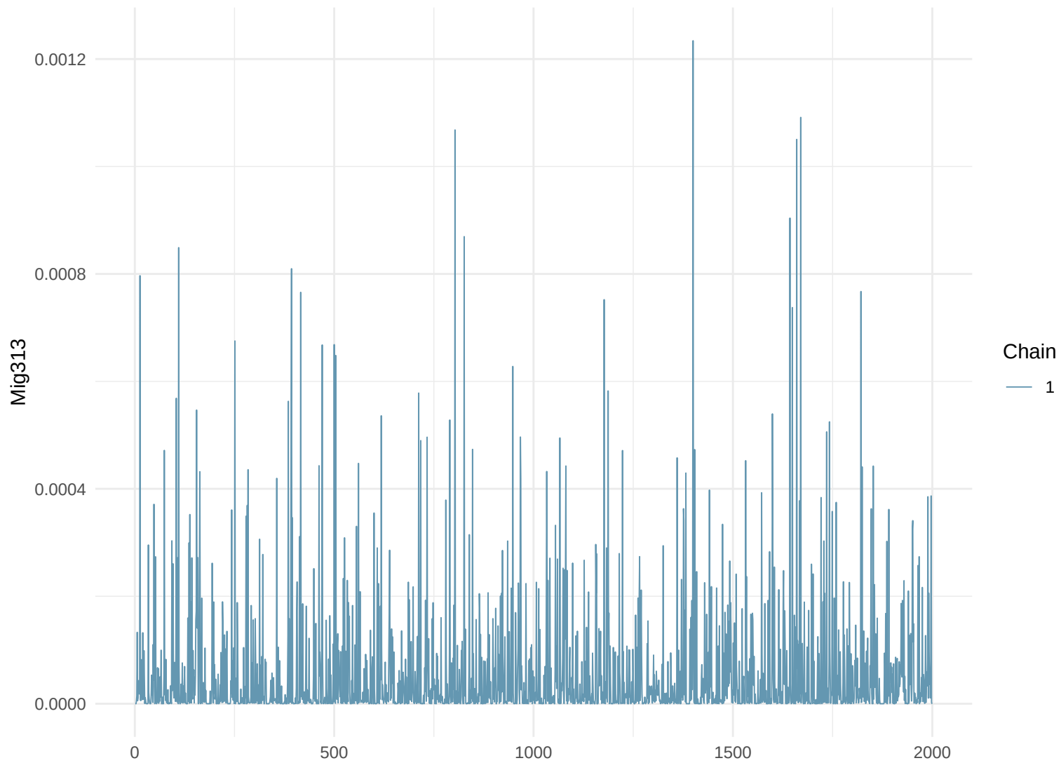
Trace Plot: Mig313
