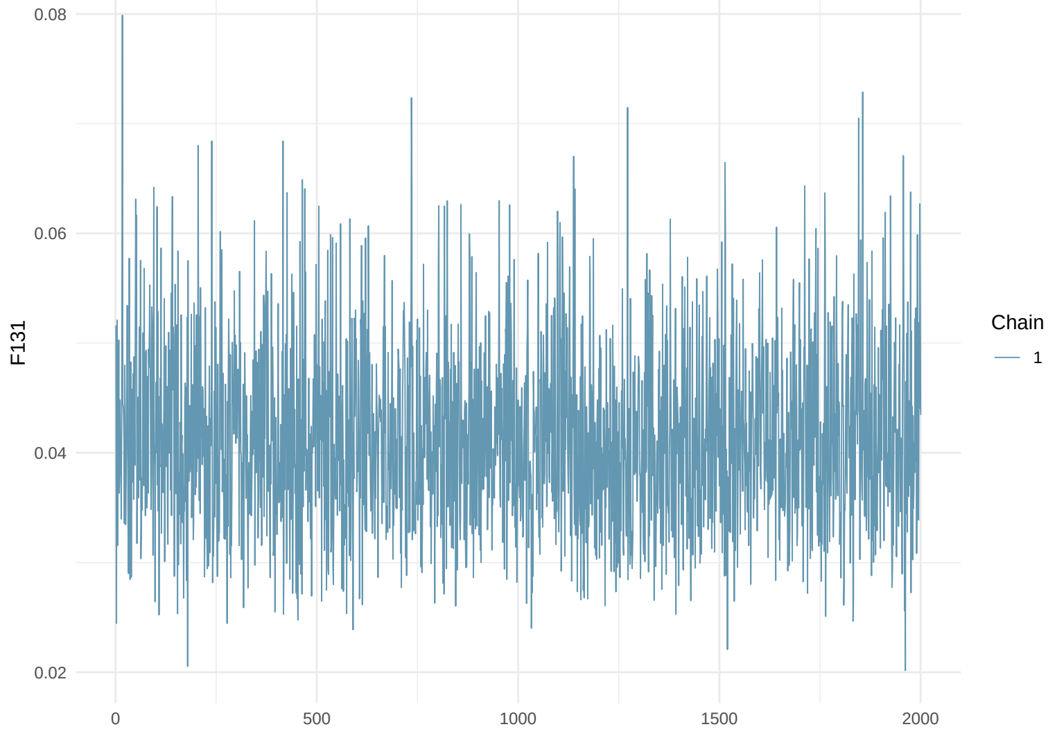
Trace Plot: F131
