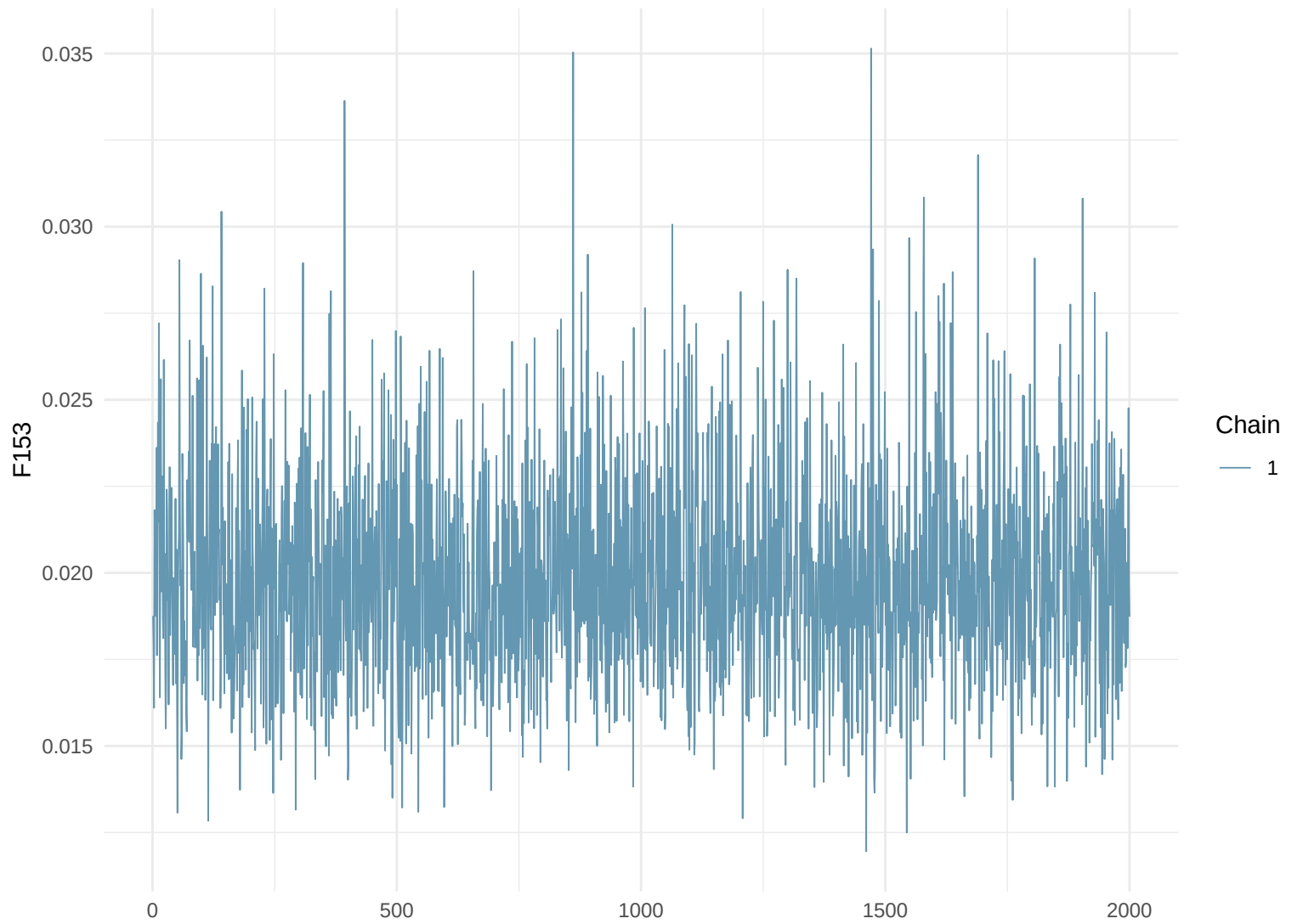
Trace Plot: F153
