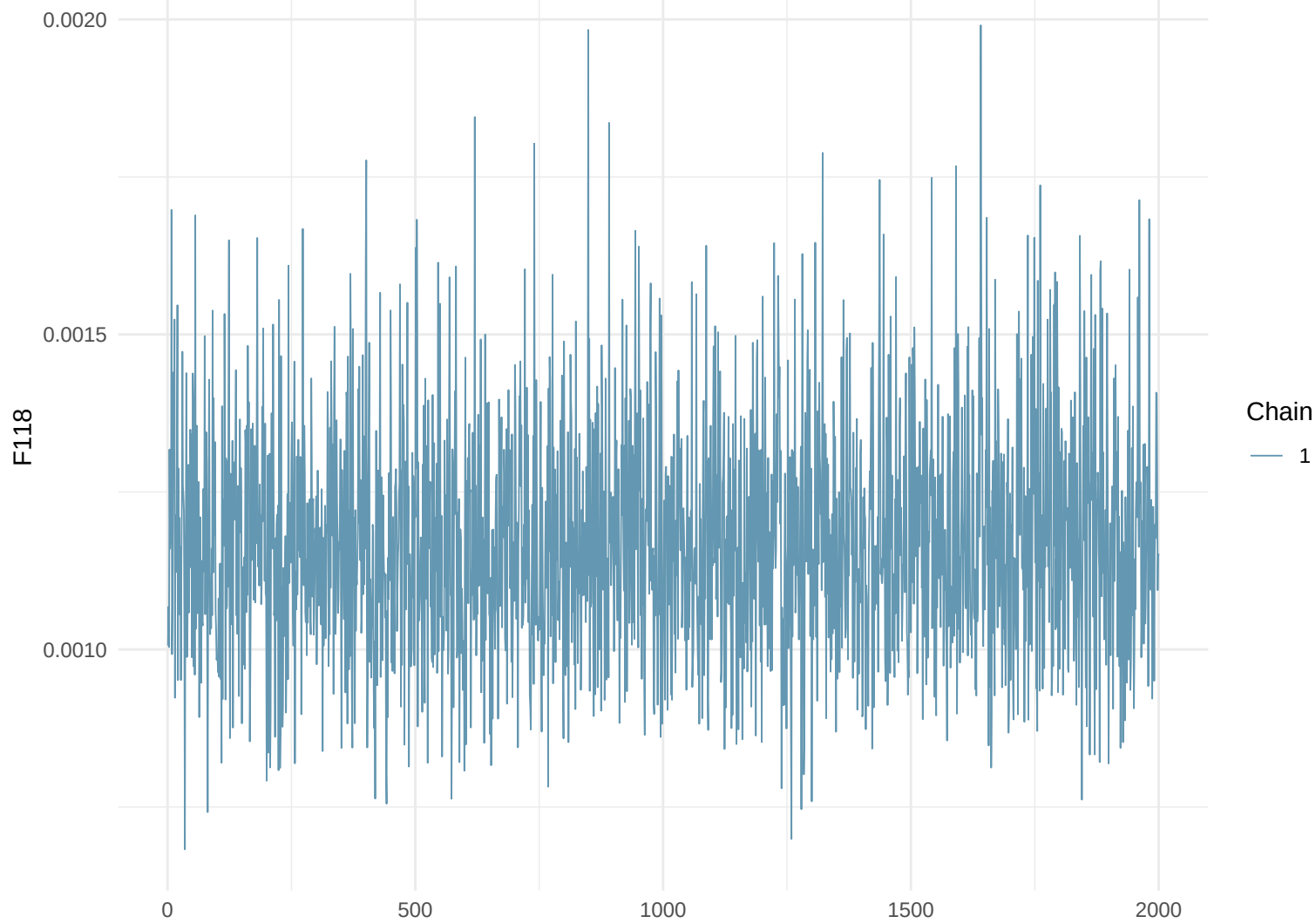
Trace Plot: F118
