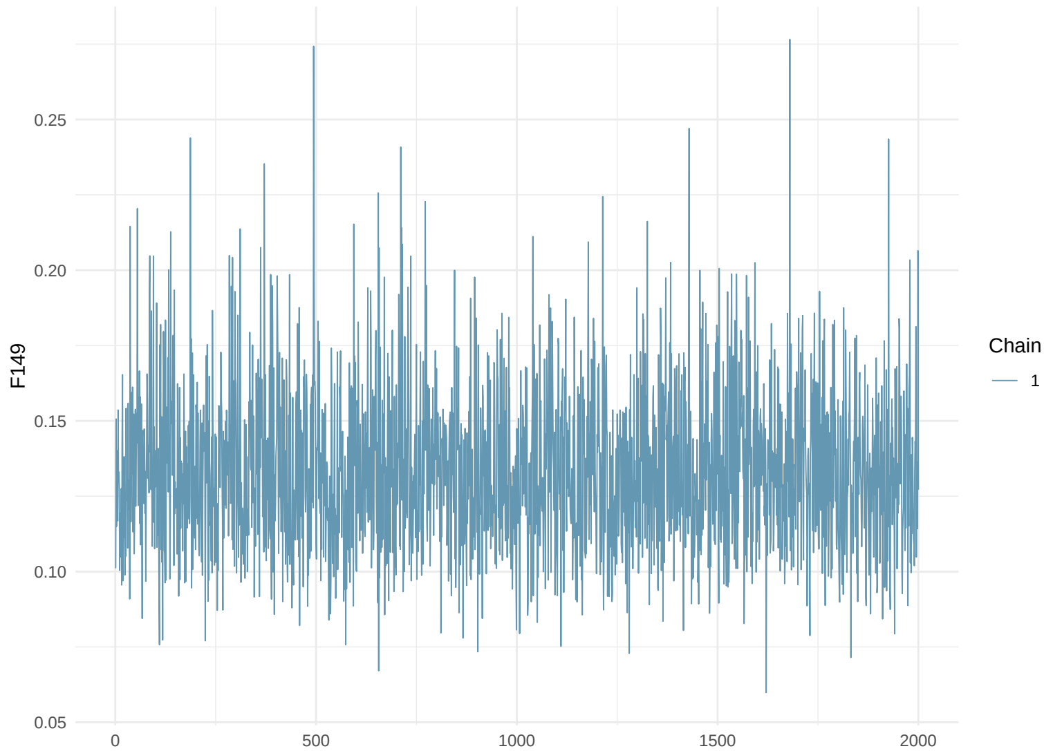
Trace Plot: F149
