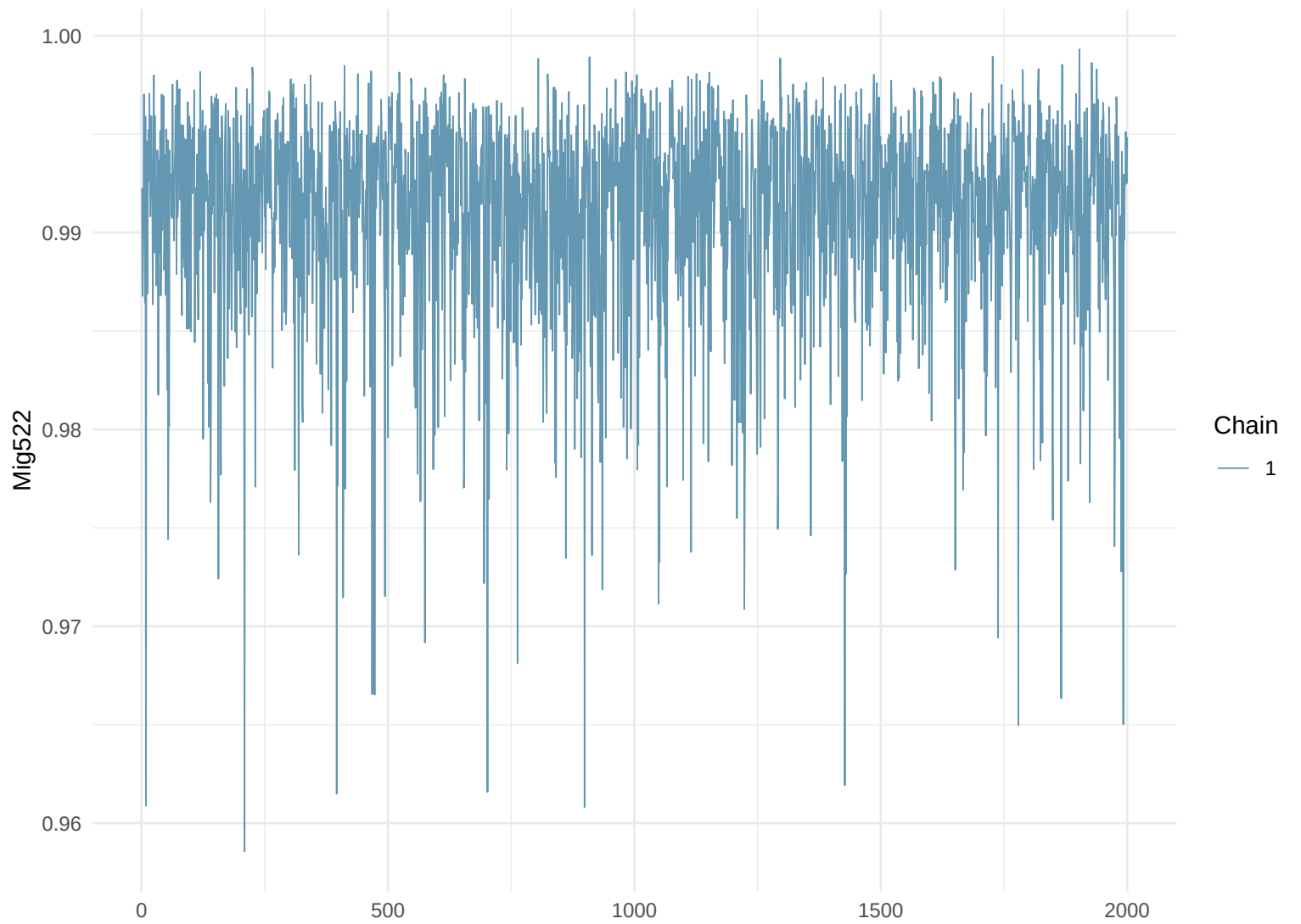
Trace Plot: Mig522
