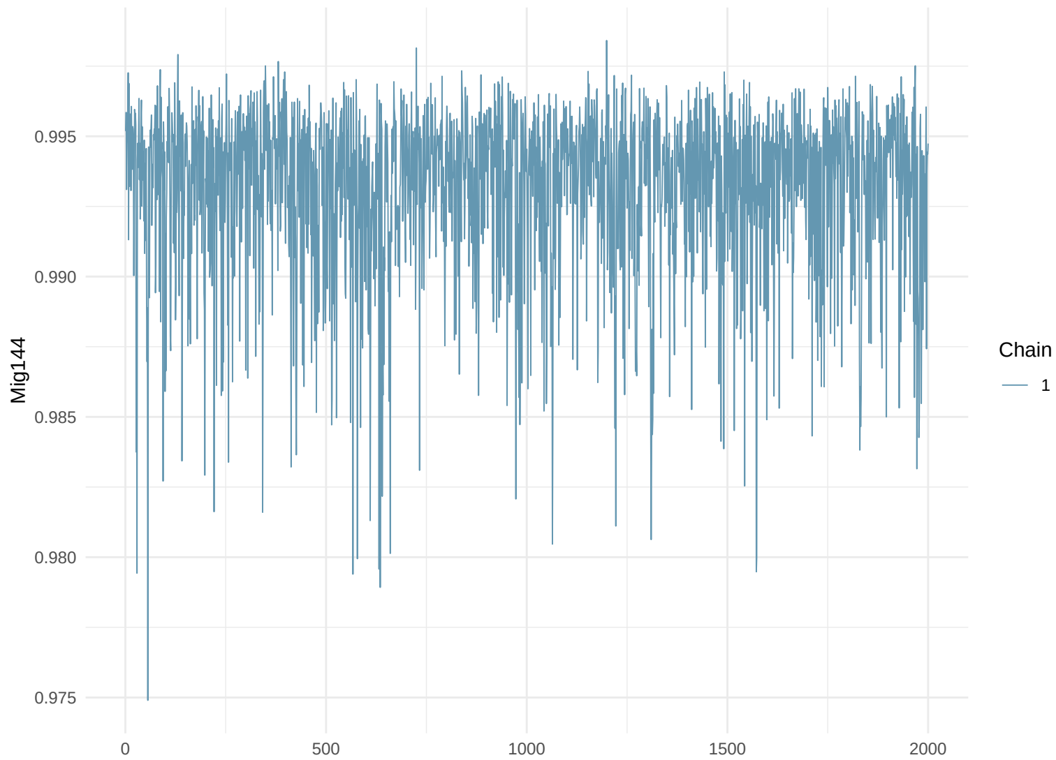
Trace Plot: Mig144
