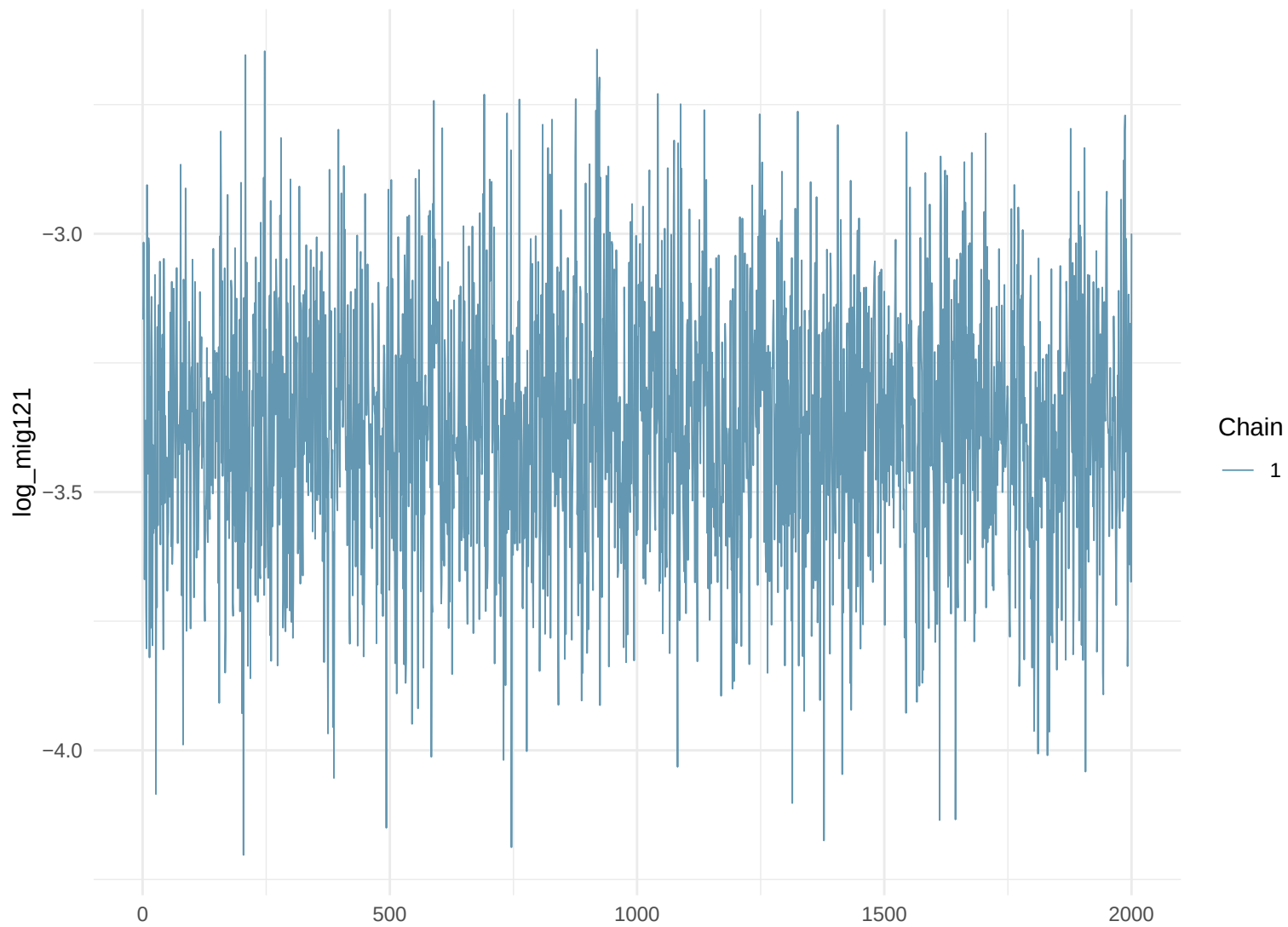
Trace Plot: log_mig121
