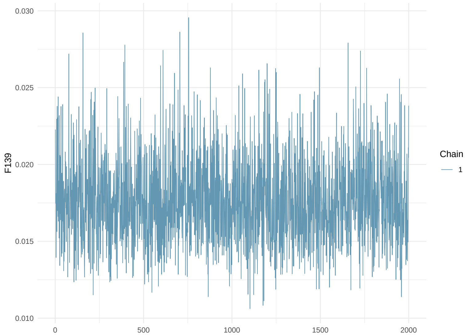
Trace Plot: F139
