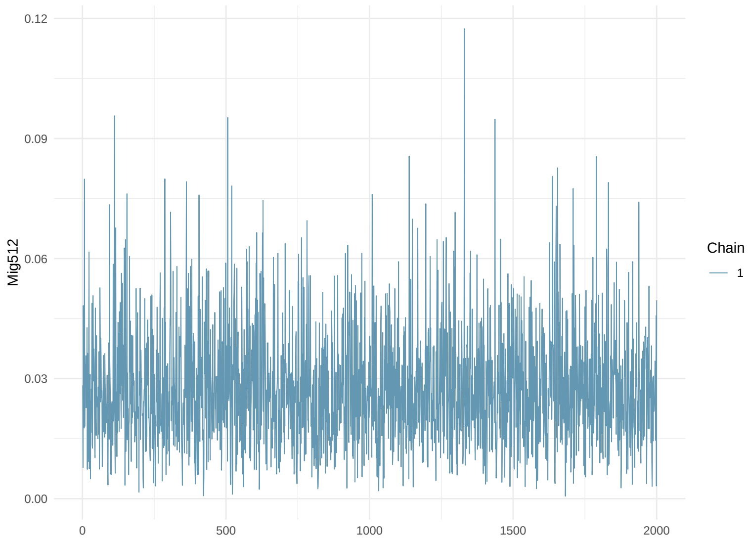
Trace Plot: Mig512
