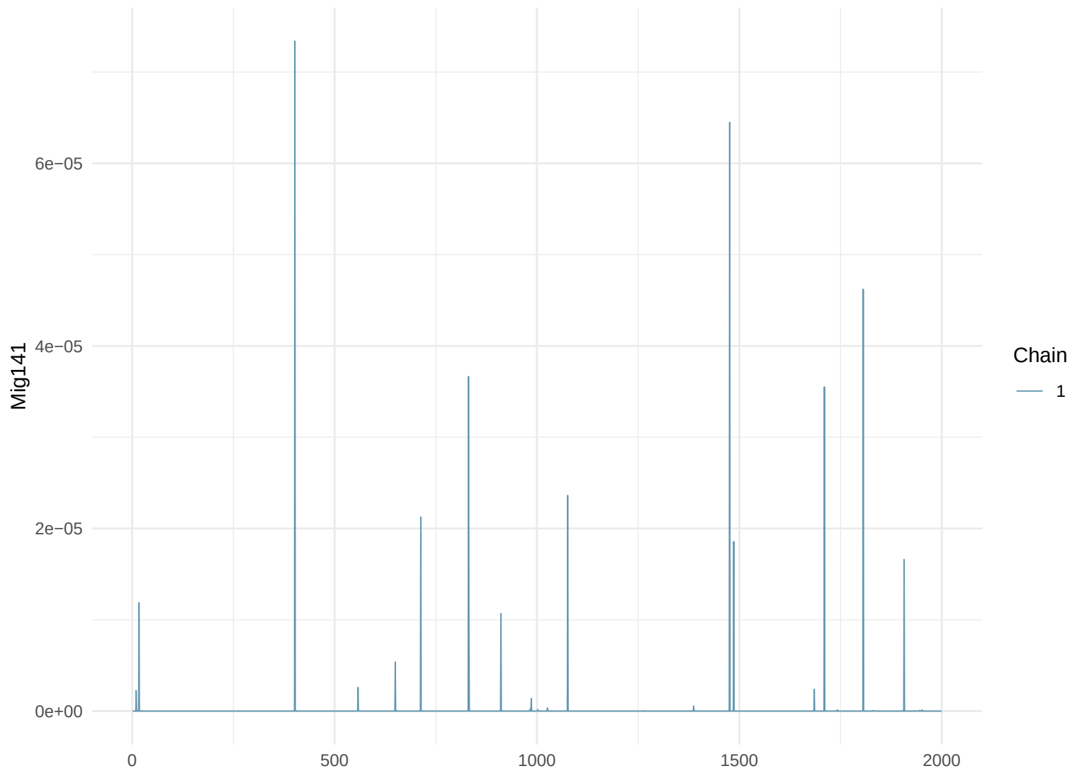
Trace Plot: Mig141
