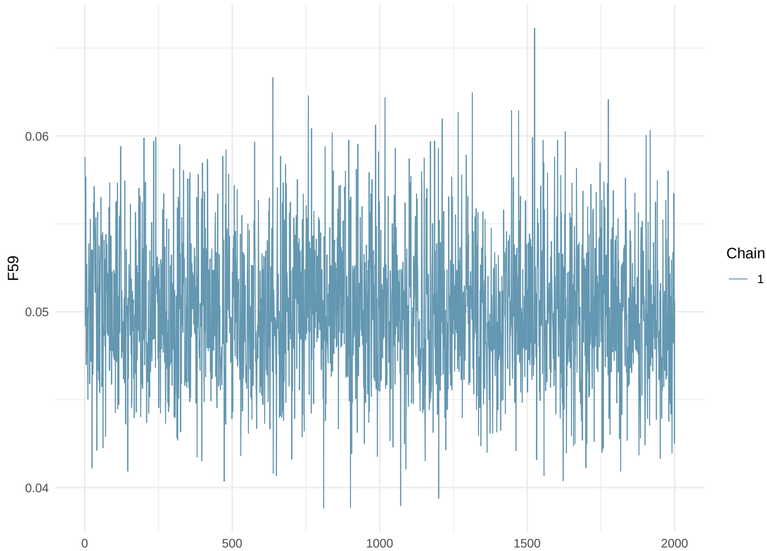
Trace Plot: F59
