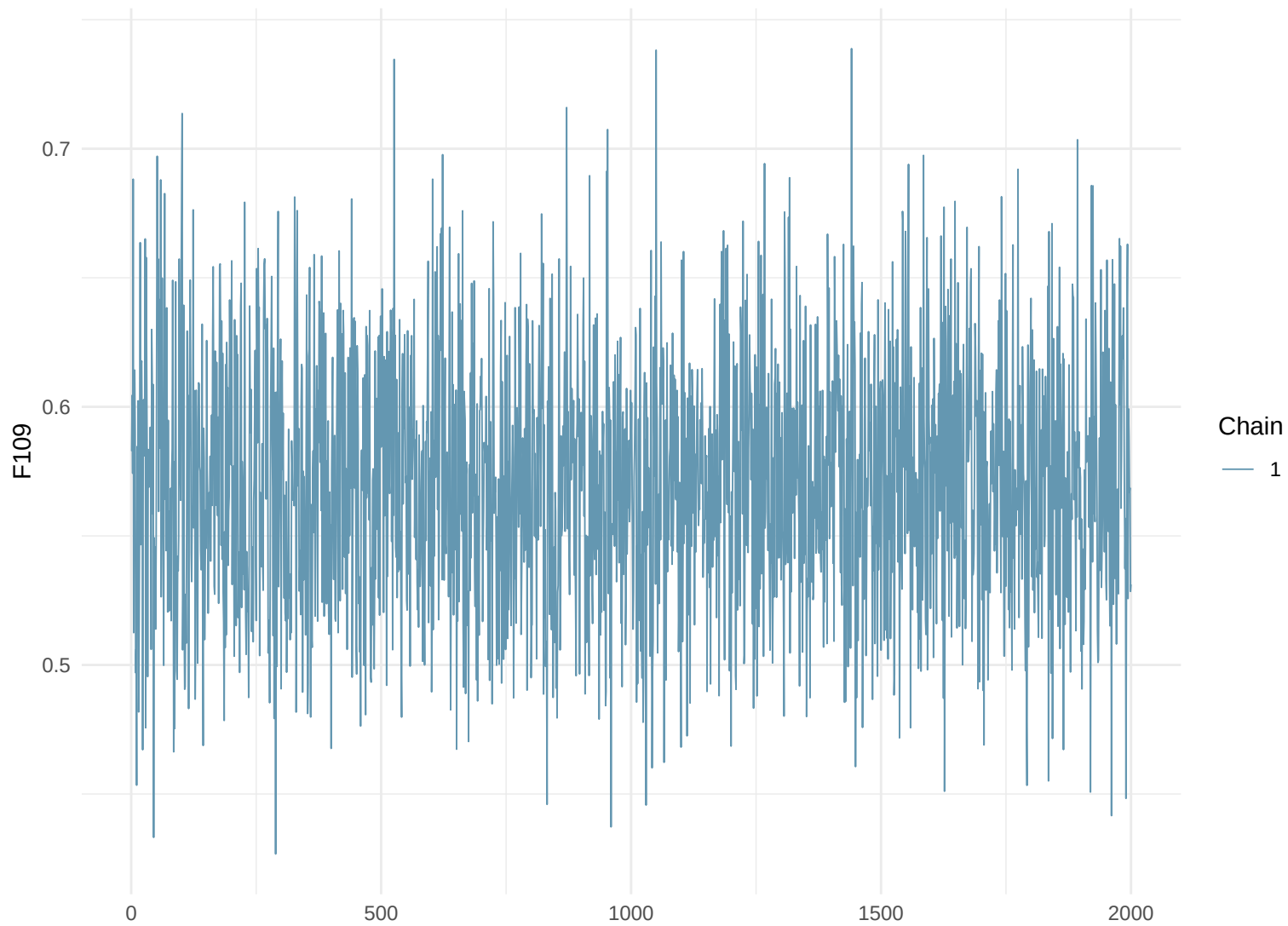
Trace Plot: F109
