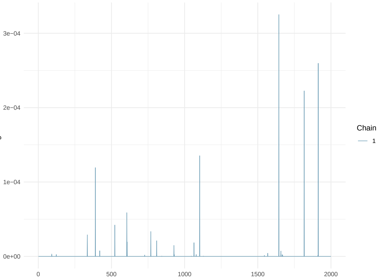
Trace Plot: Mig342
