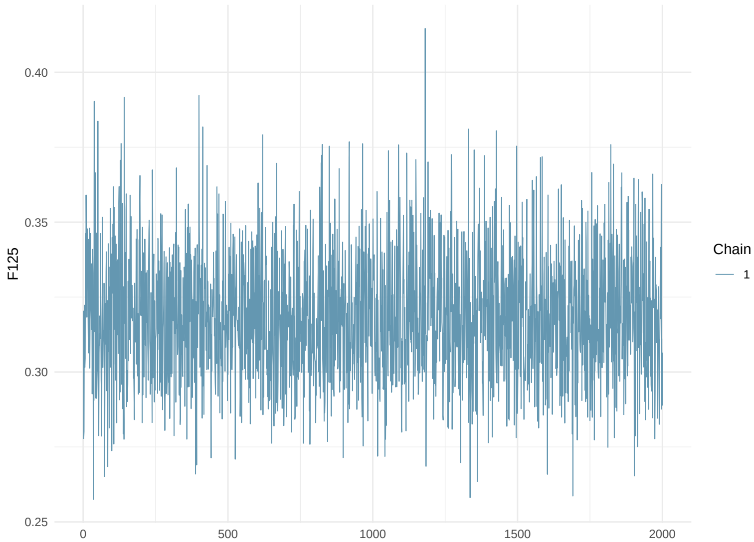
Trace Plot: F125
