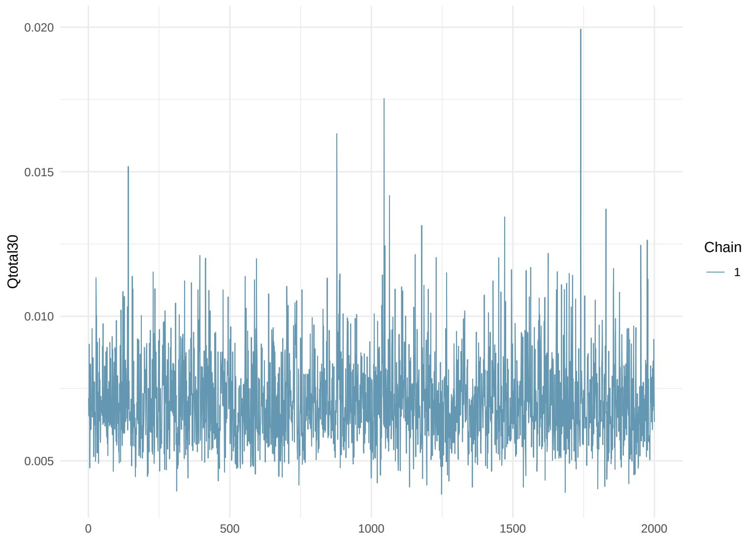
Trace Plot: Qtotal30
