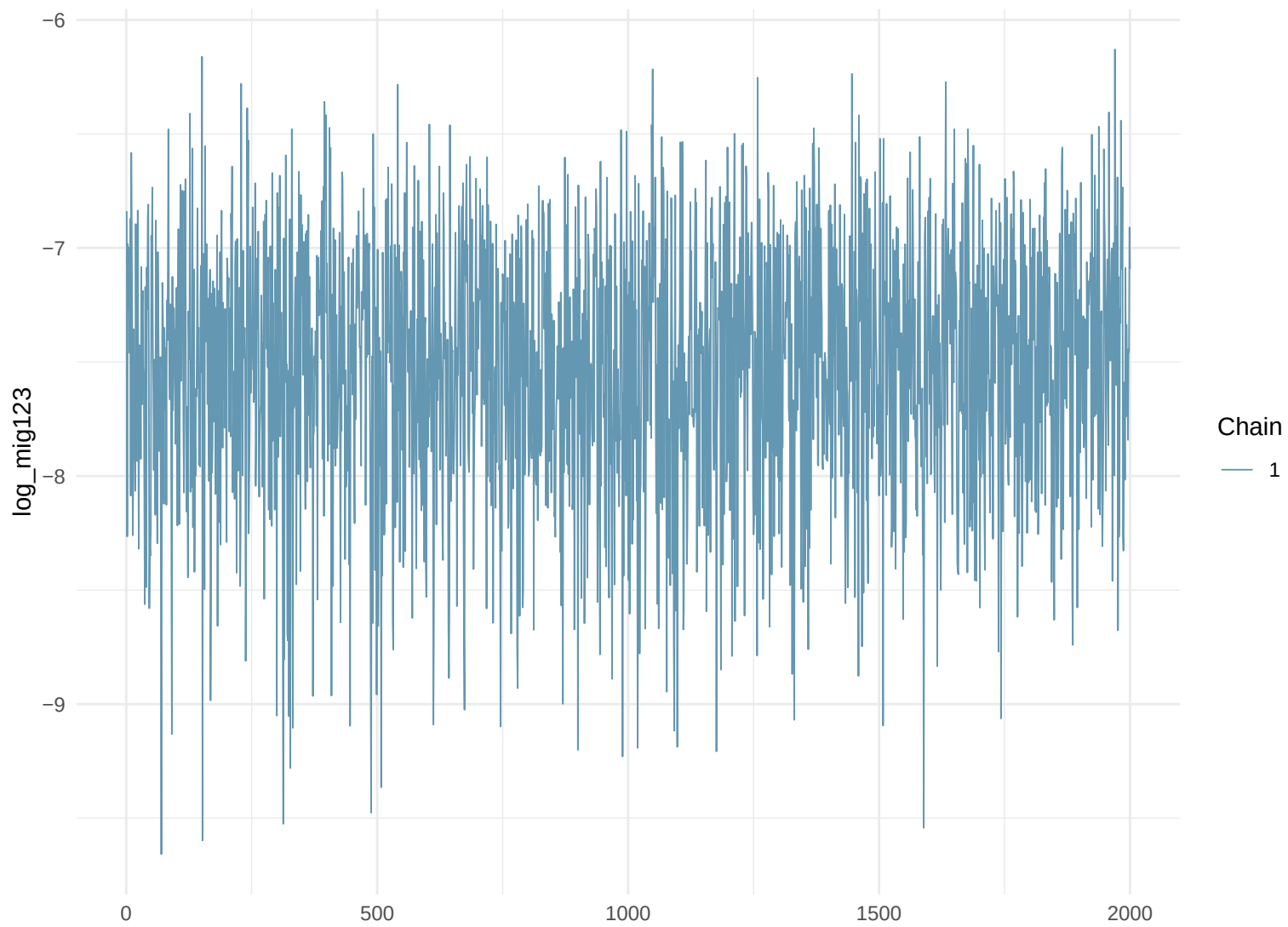
Trace Plot: log_mig123
