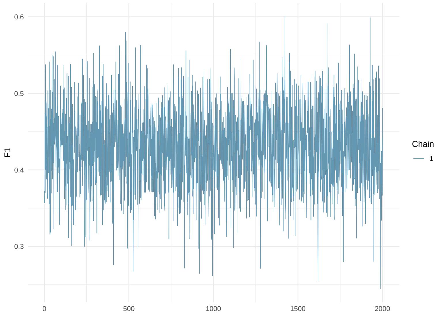
Trace Plot: F1
