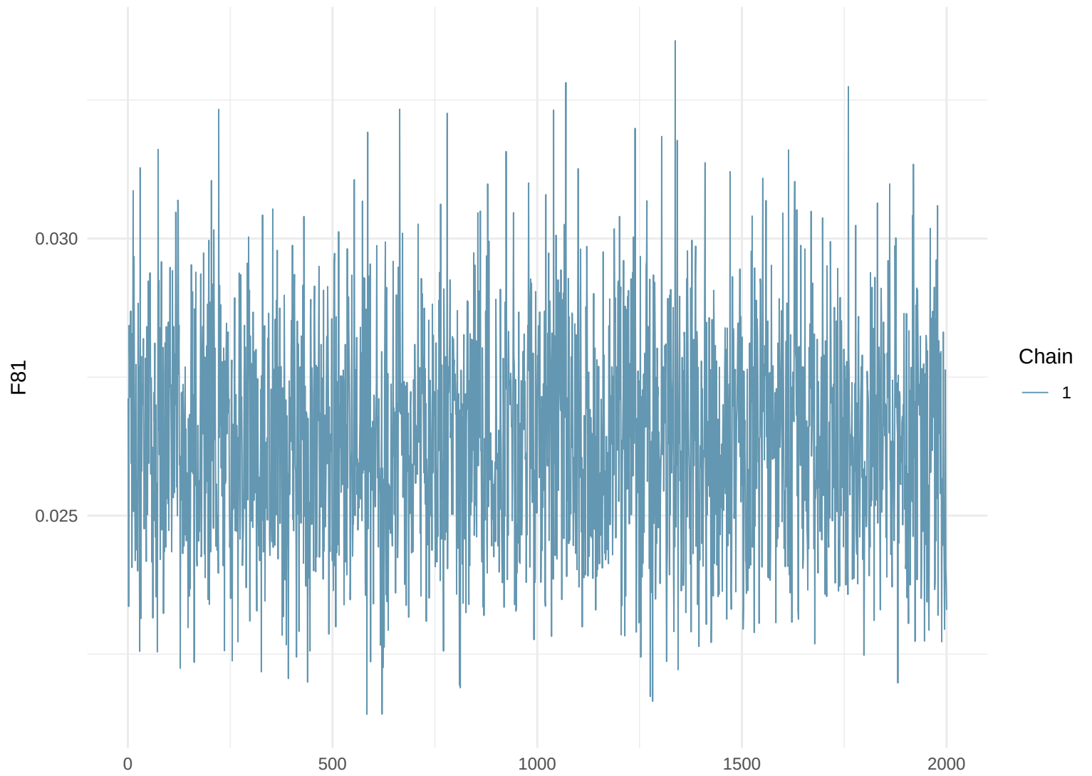
Trace Plot: F81
