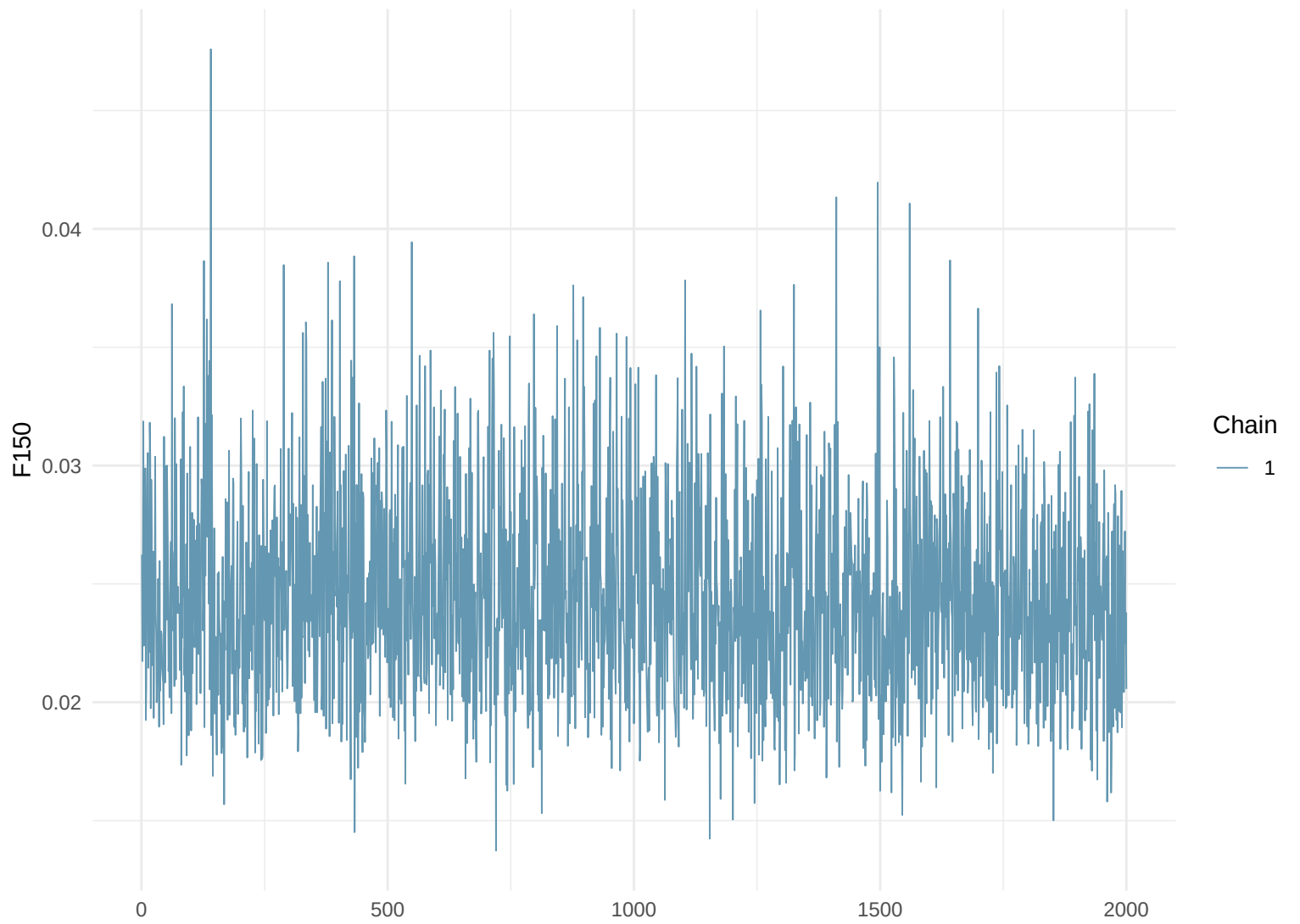
Trace Plot: F150
