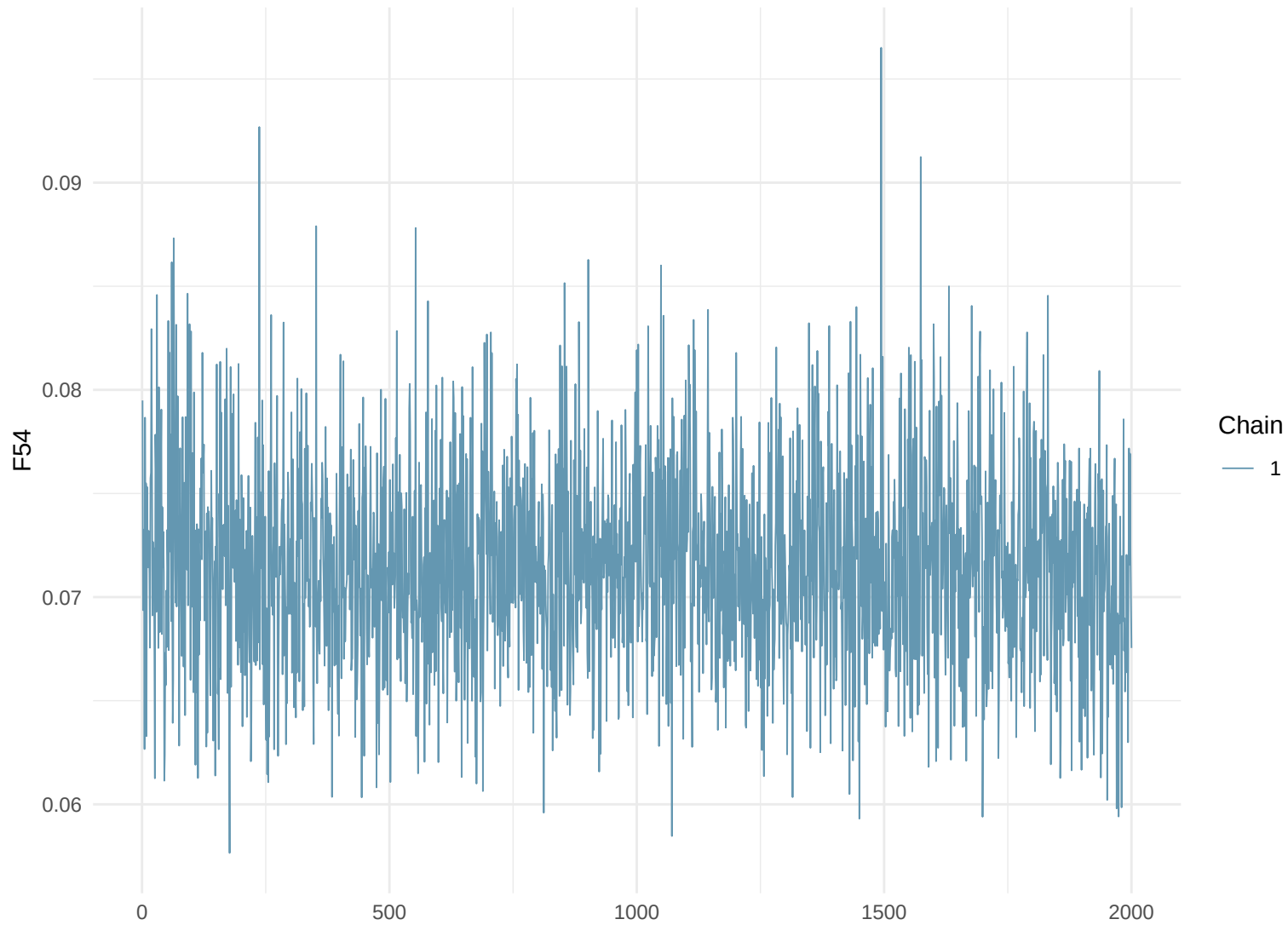
Trace Plot: F54
