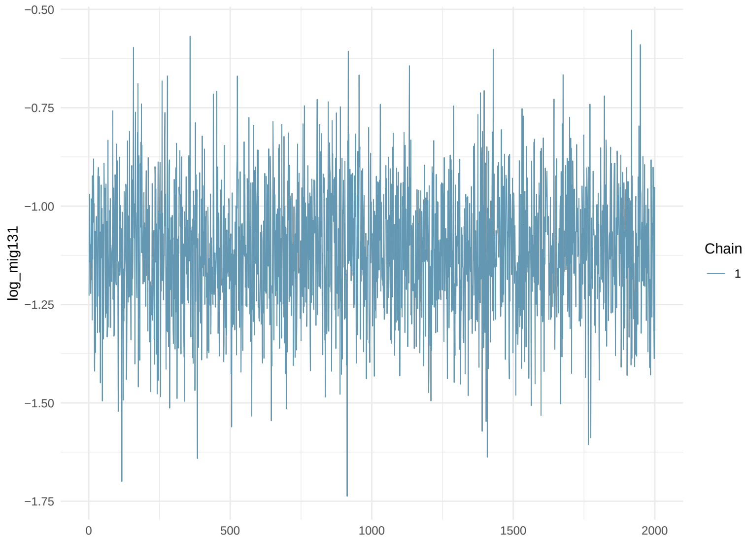
Trace Plot: log_mig131
