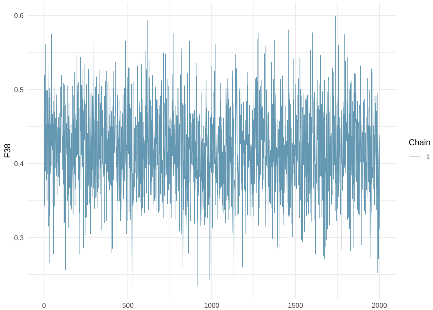
Trace Plot: F38
