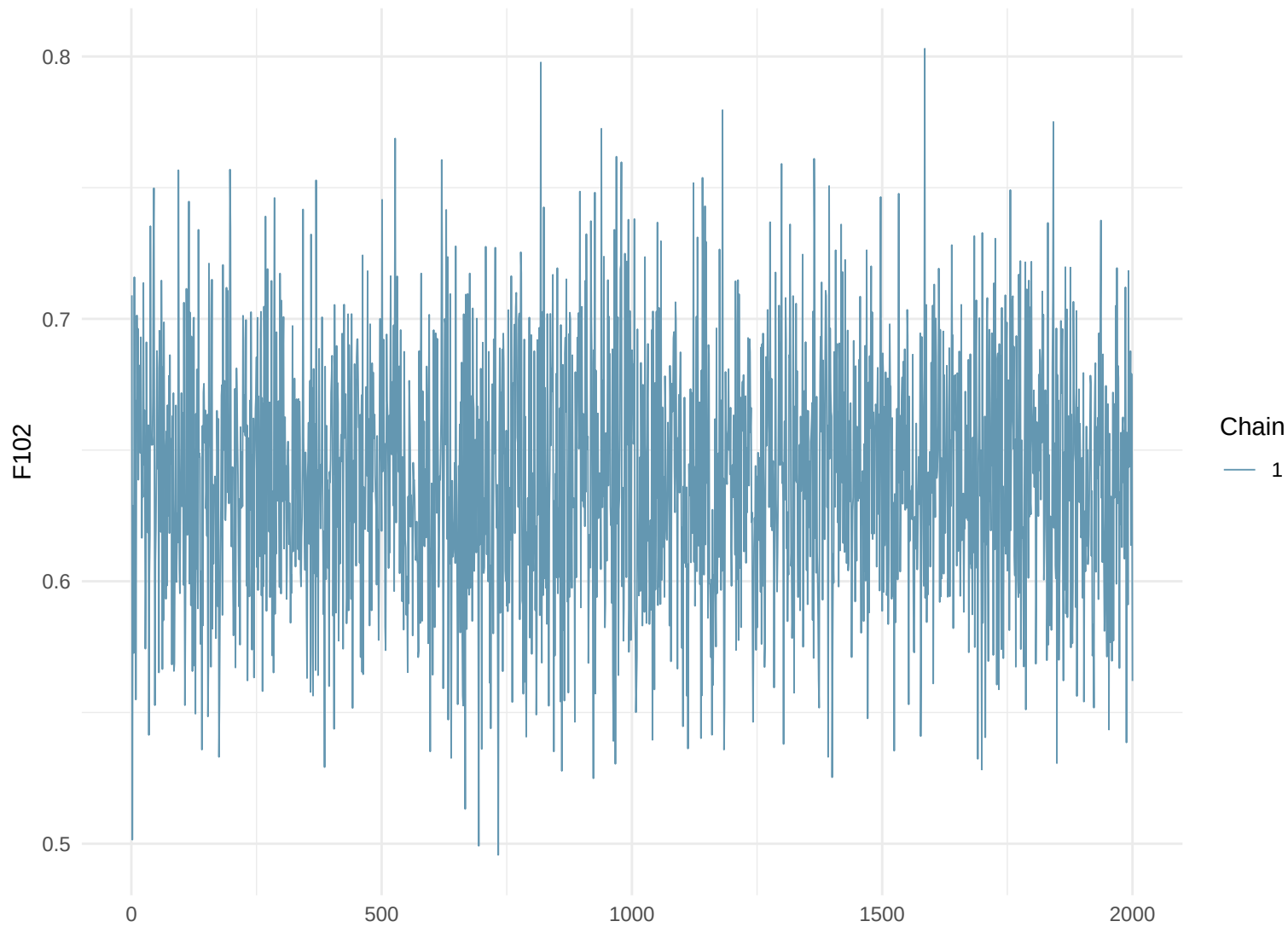
Trace Plot: F102
