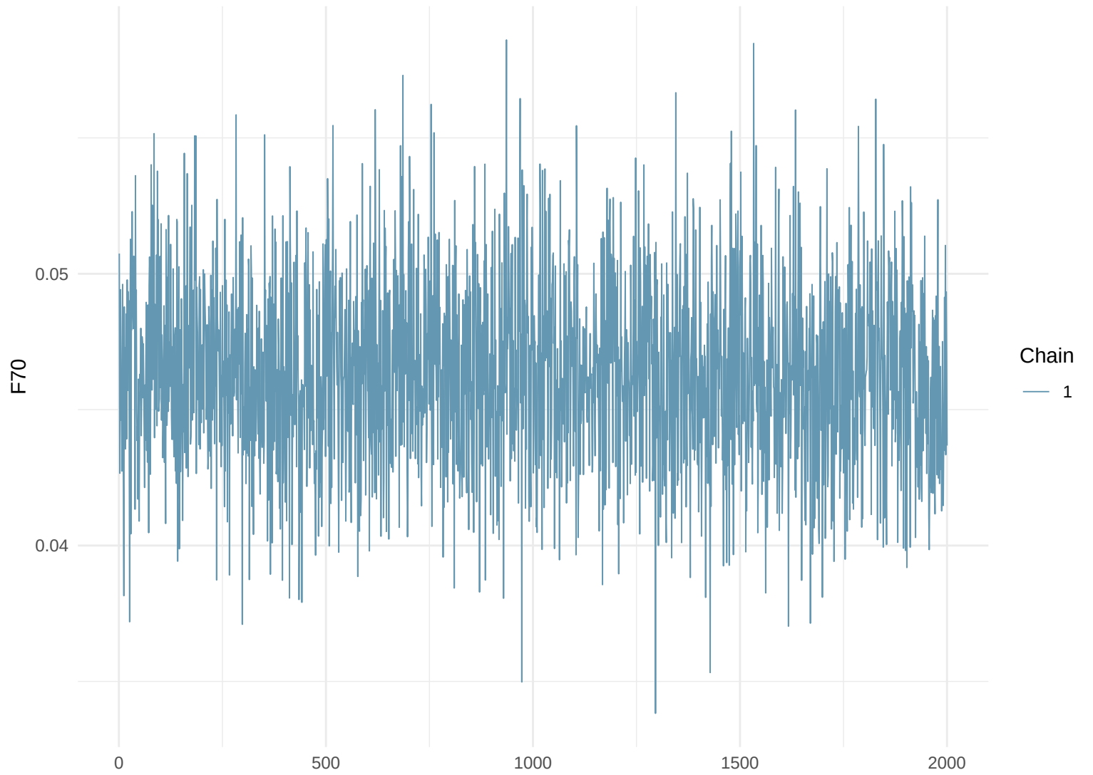
Trace Plot: F70
