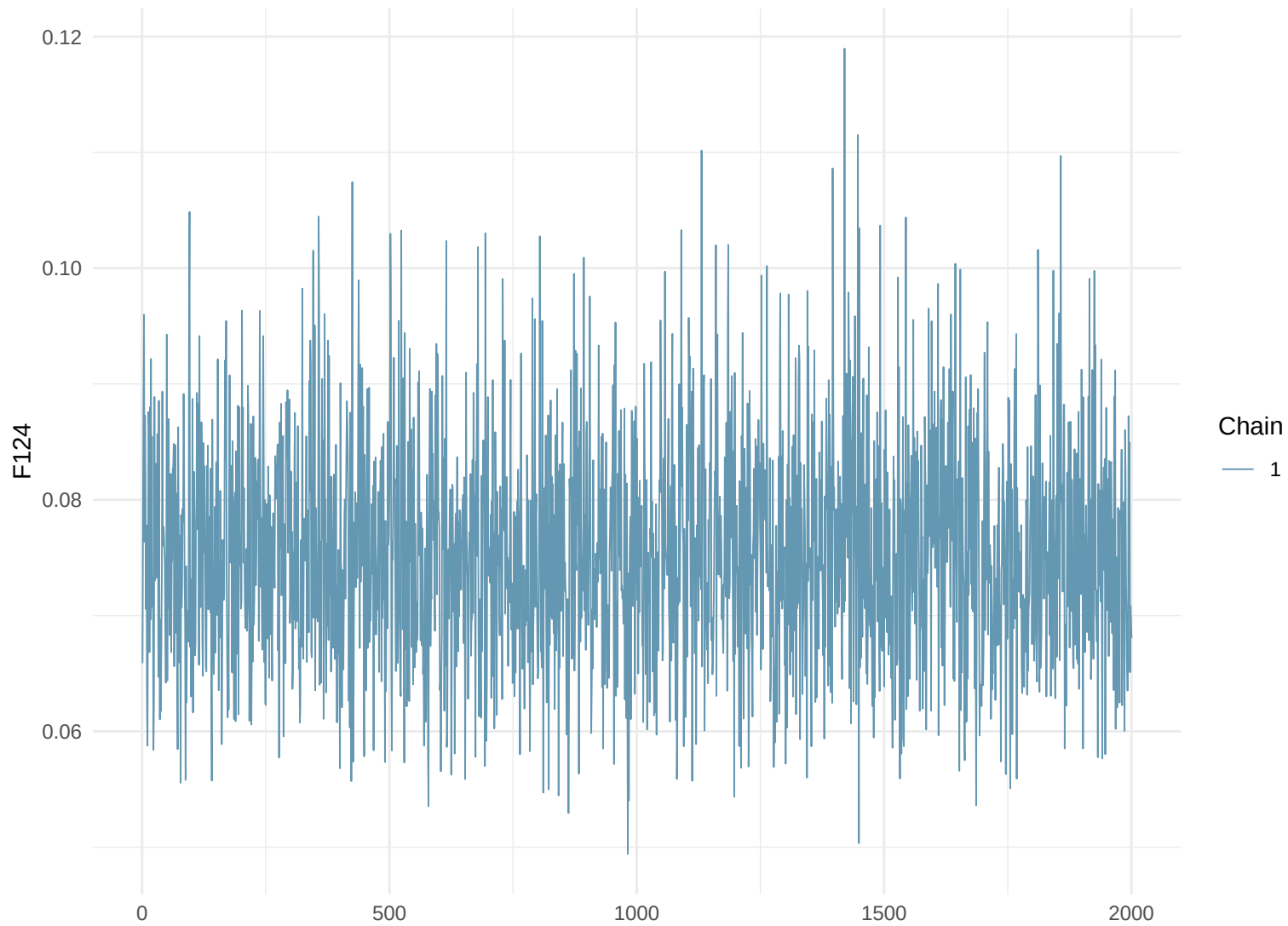
Trace Plot: F124
