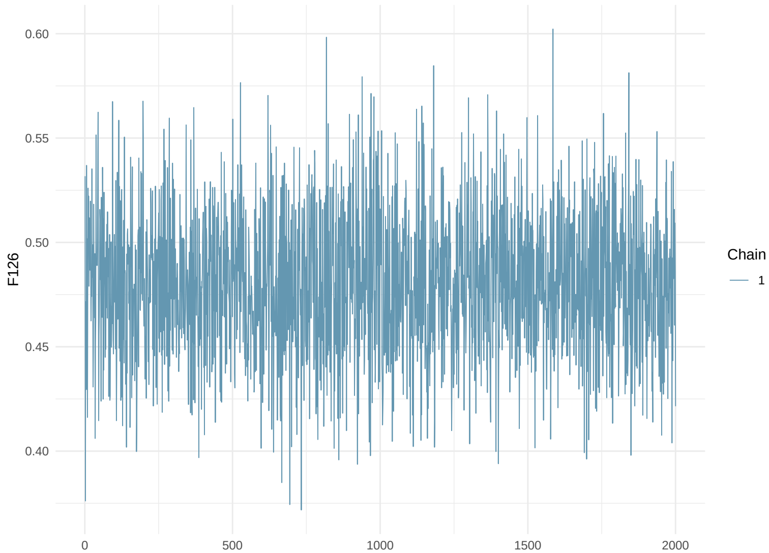
Trace Plot: F126
