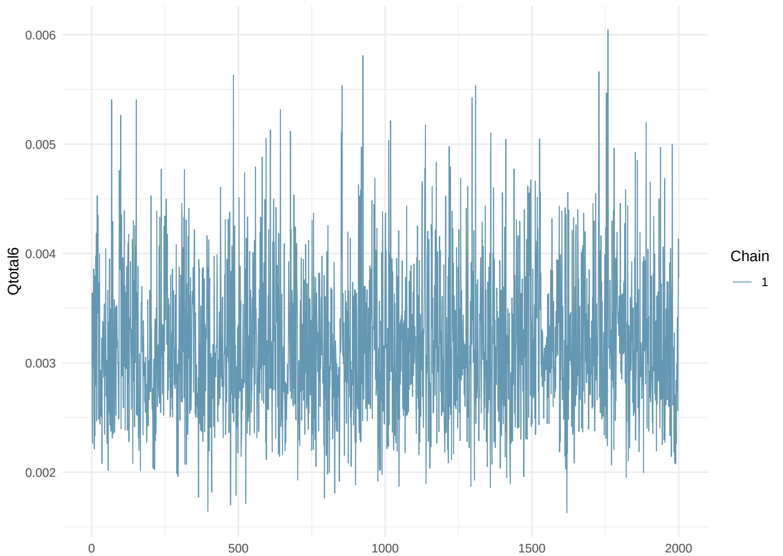
Trace Plot: Qtotal6
