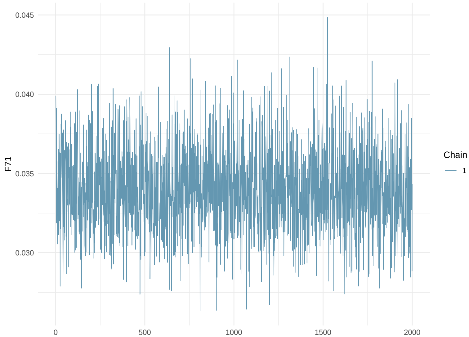
Trace Plot: F71
