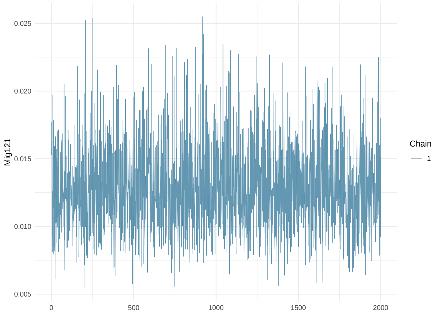
Trace Plot: Mig121
