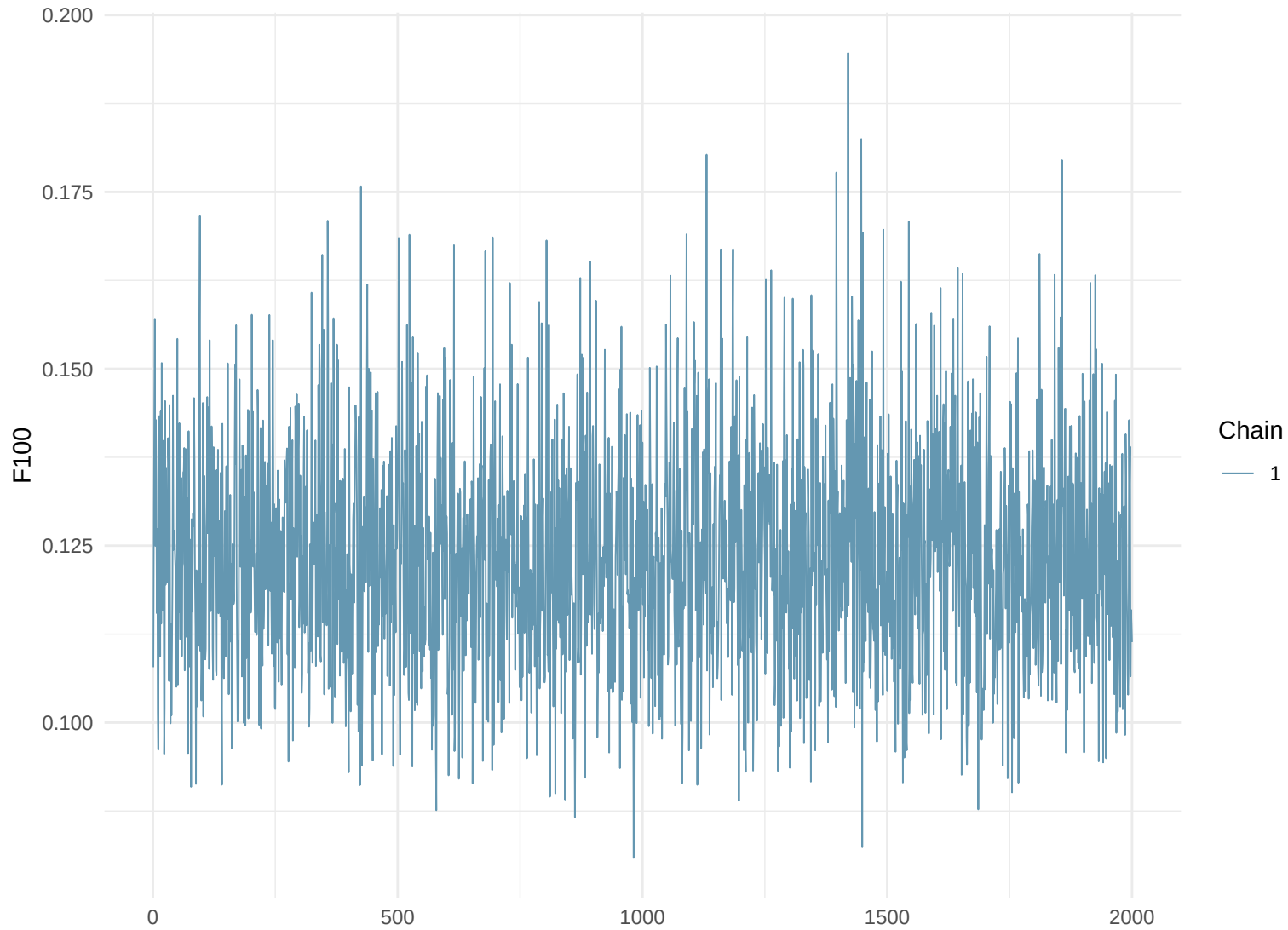
Trace Plot: F100
