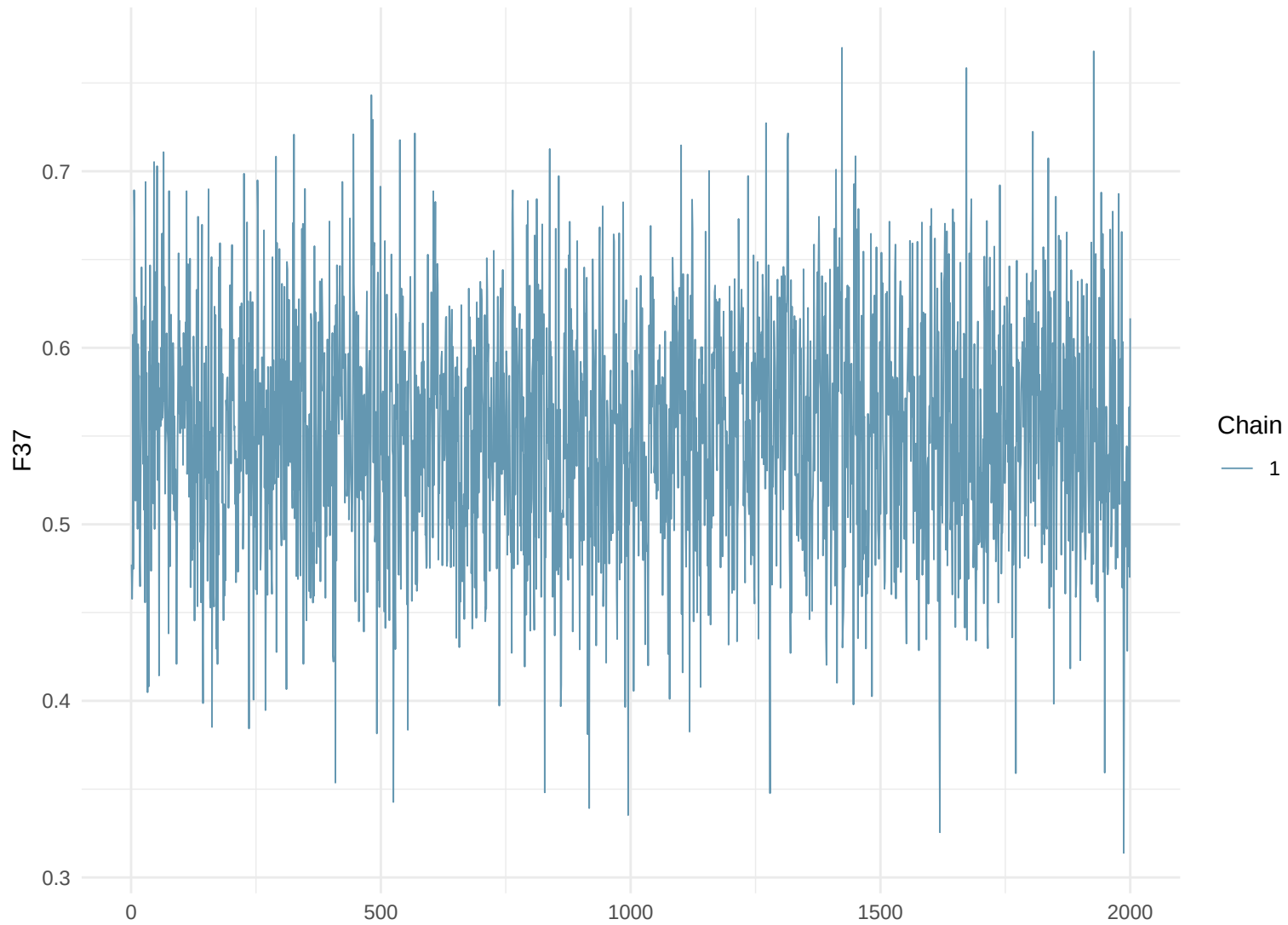
Trace Plot: F37
