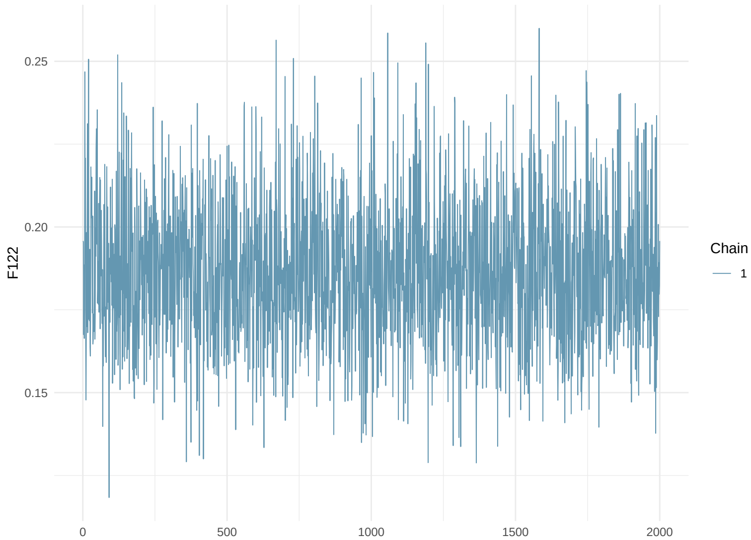
Trace Plot: F122
