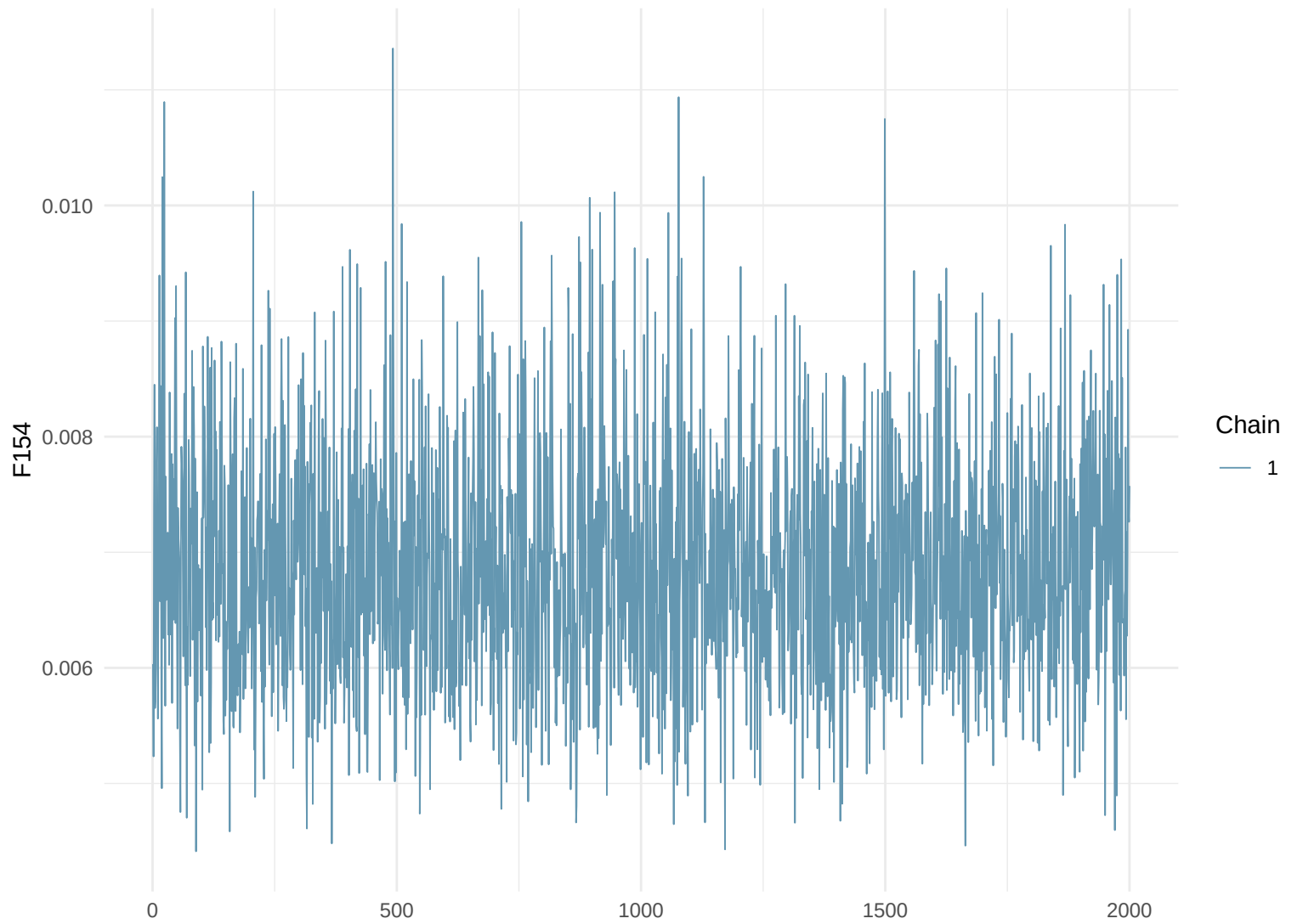
Trace Plot: F154
