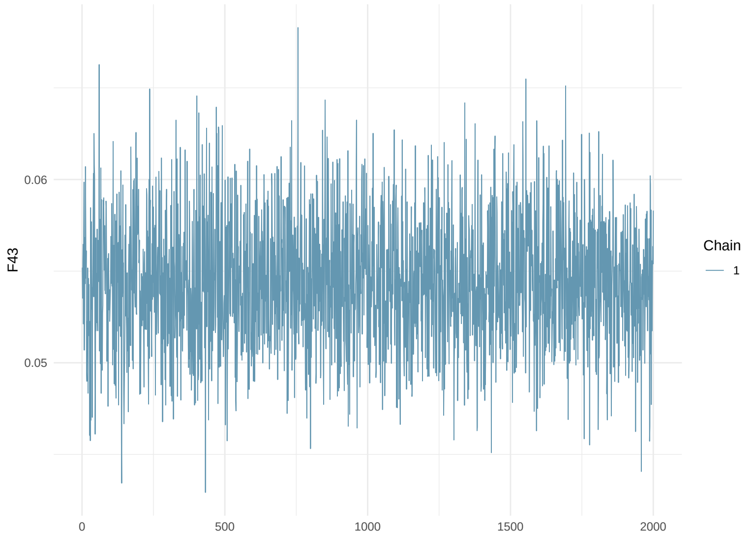
Trace Plot: F43
