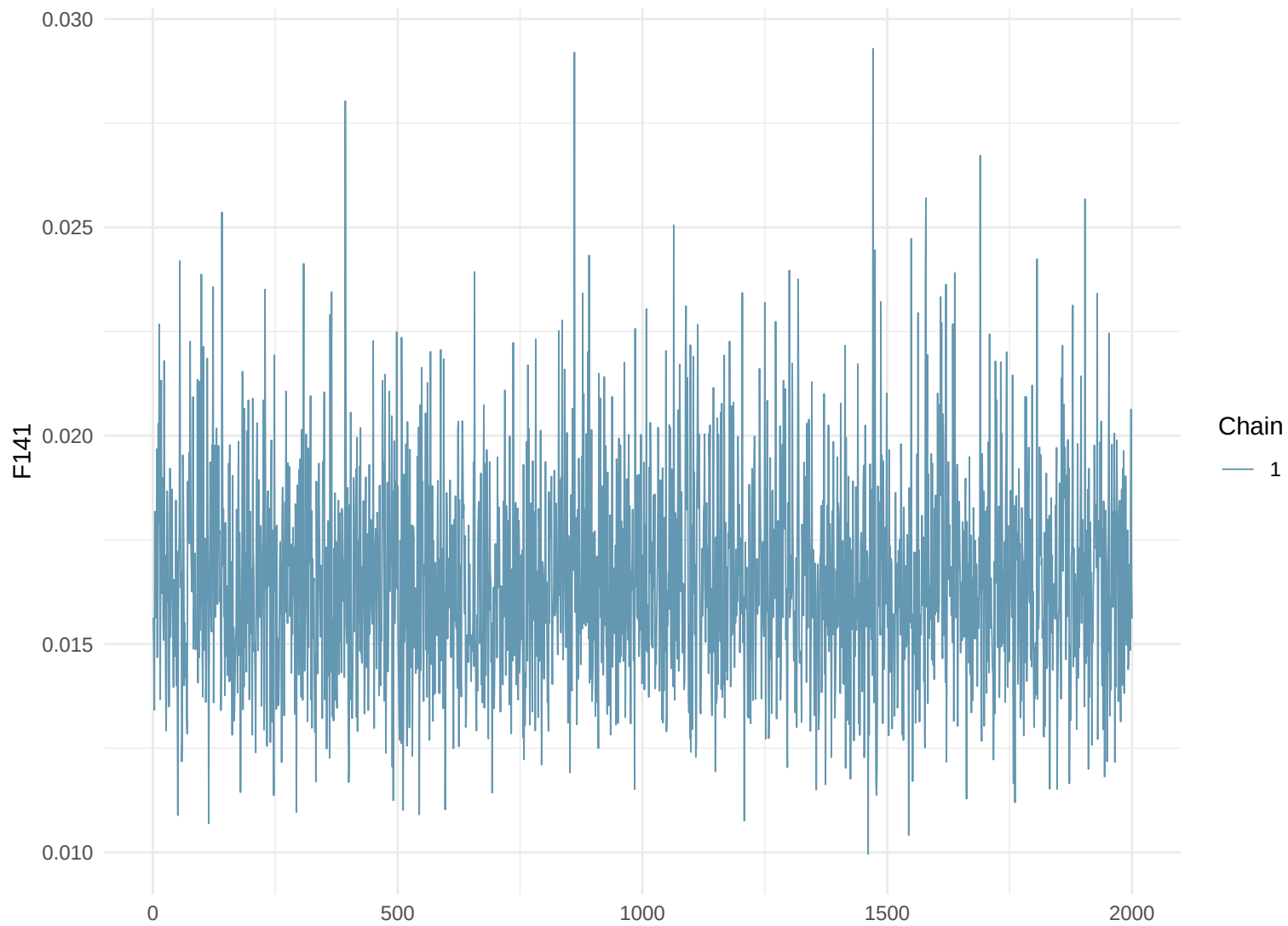
Trace Plot: F141
