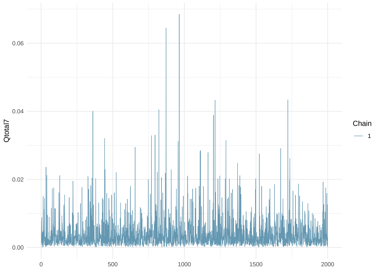
Trace Plot: Qtotal7
