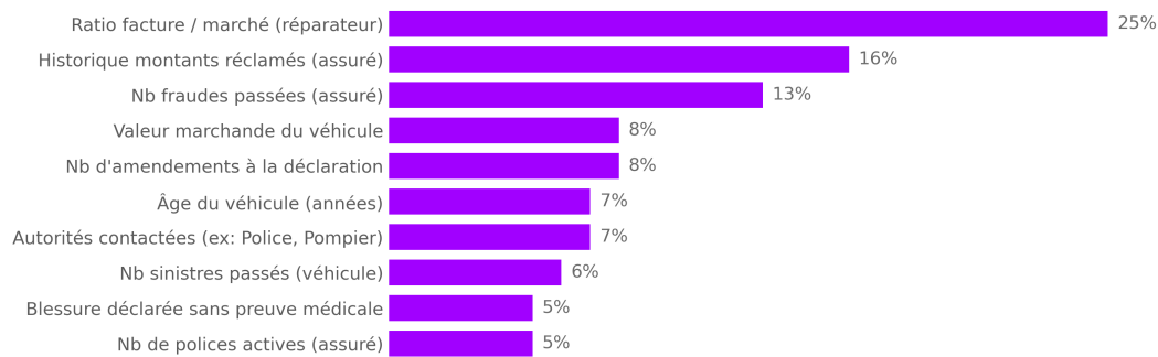
FIGURE 5.22 – Hiérarchie de l'importance globale des variables dans le modèle « Gradient Boosting »
