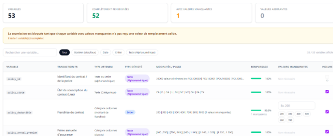
FIGURE 4.7 – Sortie de l'outil « Analyse de la qualité des données de la base » avec une valeur manquante
