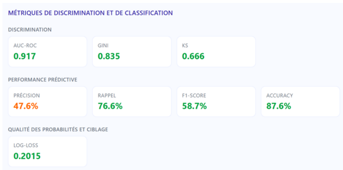
FIGURE 5.9 – Synthèse des métriques de performance et de stabilité du modèle de scoring en points
