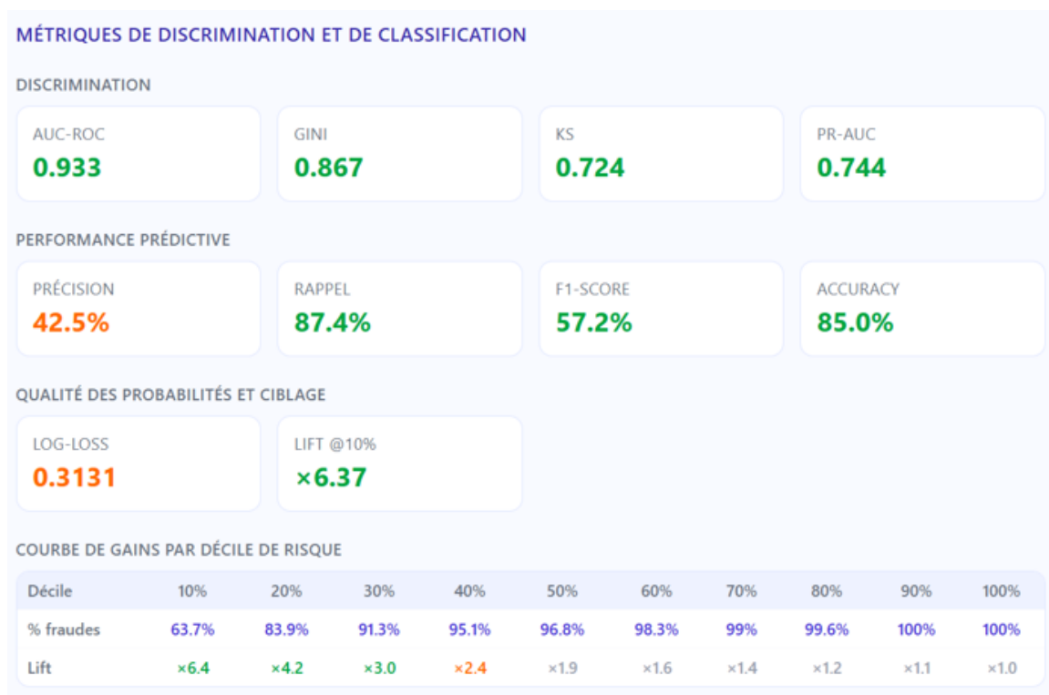
FIGURE 5.27 – Synthèse des métriques de discrimination et classification du modèle Gradient Boosting au seuil 45 %
