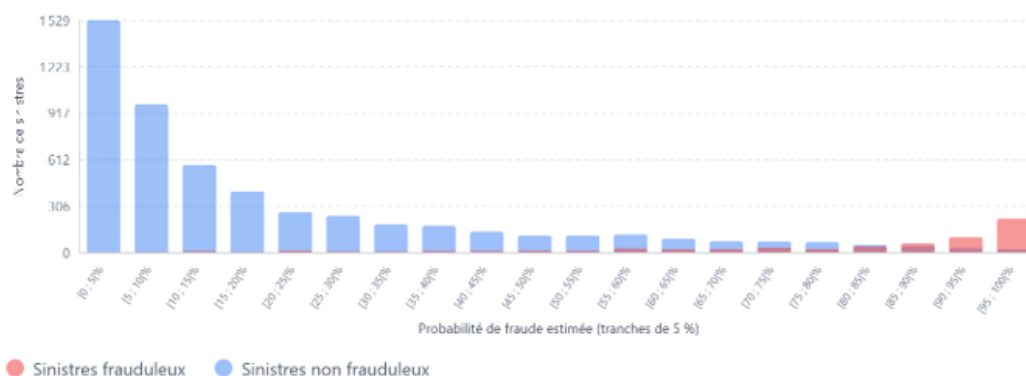
FIGURE 5.22 – Distribution des scores par classe (fraudeur/non fraudeur)
