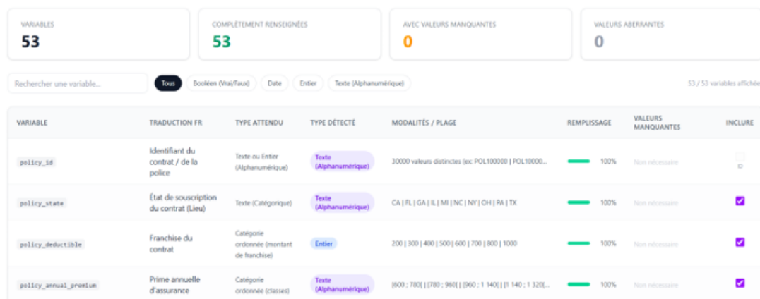
FIGURE 4.8 – Sortie de l'outil « Analyse de la qualité des données de la base » sans valeur manquante
