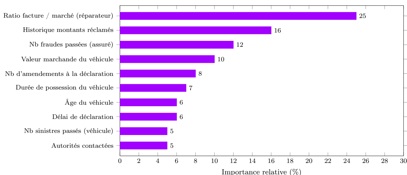
FIGURE 1 – Importance relative des variables dans le modèle retenu (Gradient Boosting)
