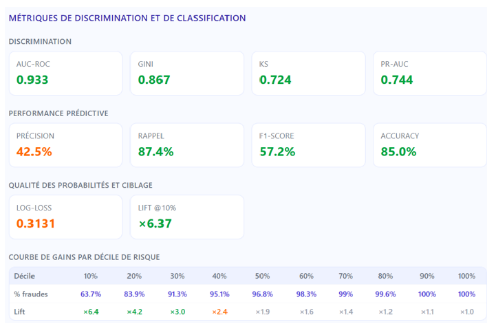
FIGURE 5.27 – Synthèse des métriques de performance et de stabilité du modèle Gradient Boosting au seuil 45 %
