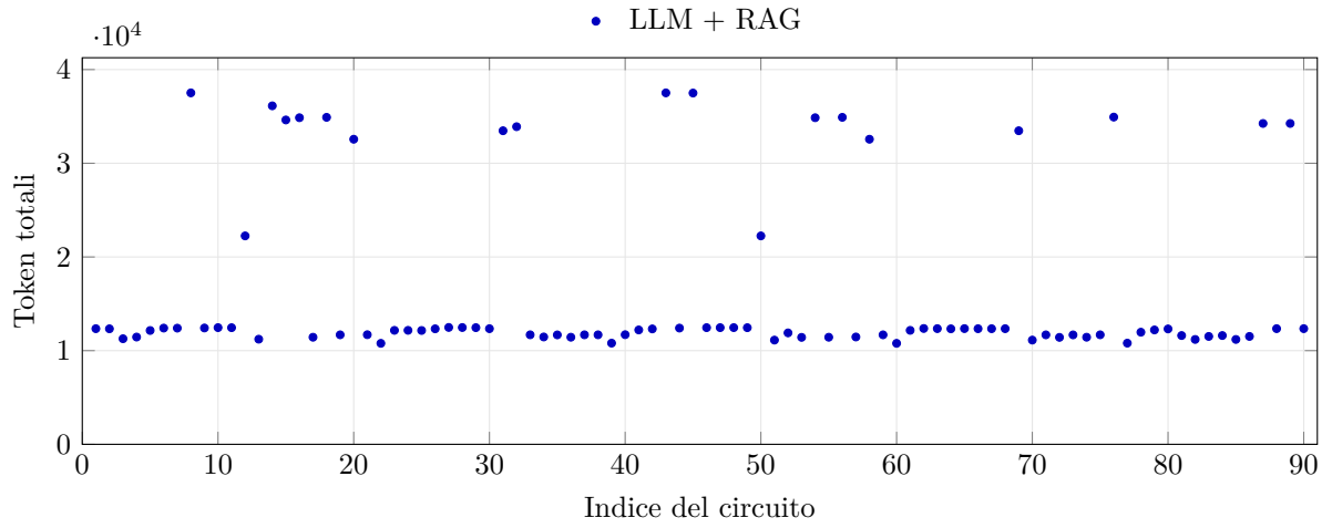
Figura 5: Token di ingresso e uscita cumulativi di tutte le chiamate dell'episodio. Con più episodi si usa la media per circuito.
