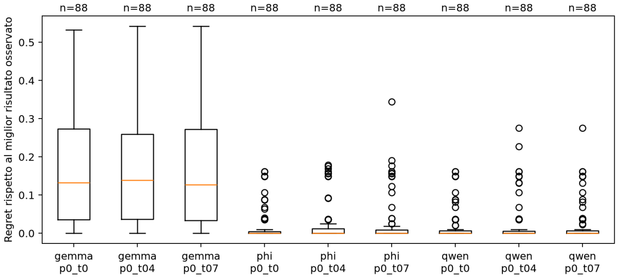
Figura 1: Regret osservato. Ogni punto statistico rappresenta un circuito; n indica i circuiti valutabili.
