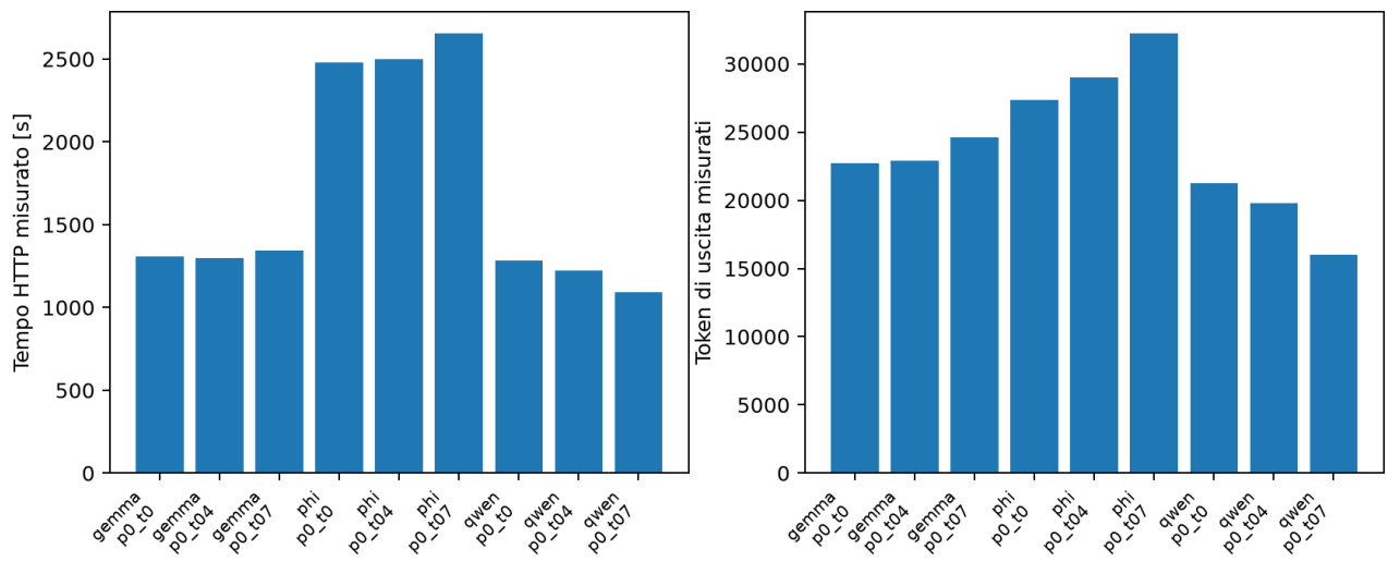
Figura 4: Totali solo quando tutte le chiamate sono misurabili. I valori mancanti non diventano zero; attese e caricamenti sono nei registri del supervisore.
