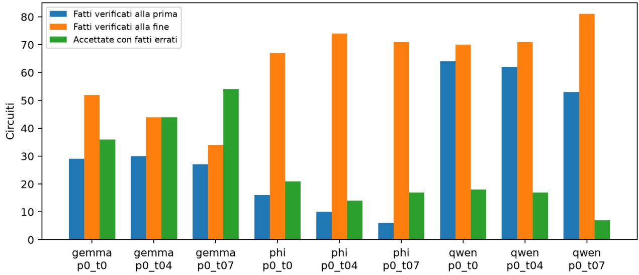
Figura 2: Esiti dei controlli sui fatti. La motivazione libera non viene validata semanticamente.
