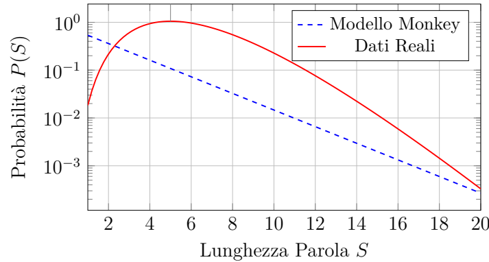
Figura 5.1: Confronto tra la previsione teorica e la distribuzione reale della lunghezza delle parole.
