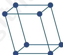
Monoclino Semplice (P)
