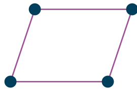
Monoclino (Obliquo)
