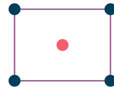
Ortorombico centrato
