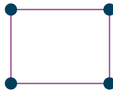
Ortorombico (Rettangolare)
