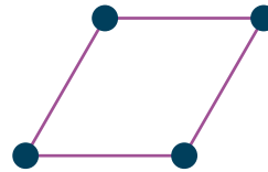
Esagonale (120°)
