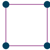
Tetragonale (Quadrato)
