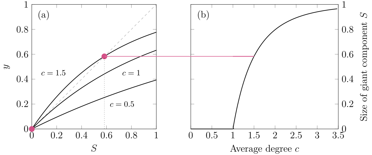
Figura 8.1: Soluzione dell'equazione della Componente Gigante nei grafi casuali. (a) Soluzione grafica dell'equazione di autoconsistenza S = 1 - e^{-cS} . Le curve mostrano il comportamento per diversi valori del grado medio c = \langle k \rangle . L'intersezione con la bisettrice y = S fornisce le soluzioni. Oltre alla soluzione banale S = 0 , una soluzione non banale S > 0 emerge quando c > 1 . (b) Dimensione della componente gigante S in funzione del grado medio c . La transizione di fase avviene a c = 1 ; per c \leq 1 , non esiste una componente gigante ( S = 0 ), mentre per c > 1 , una frazione finita dei nodi appartiene alla GC.
