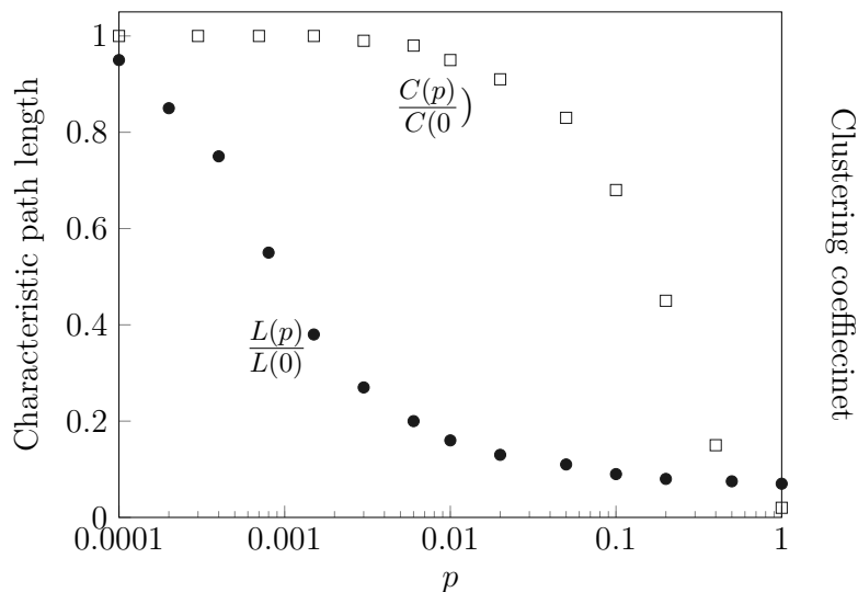
Figura 8.2: Il grafico mostra la lunghezza del cammino caratteristica normalizzata L(p)/L(0) e il coefficiente di clustering normalizzato C(p)/C(0) in funzione della probabilità di ri-cablaggio p . Si nota un ampio intervallo di p dove la rete mantiene un alto clustering (tipico dei reticoli regolari) ma acquisisce una bassa lunghezza di cammino (tipica dei grafi casuali).
