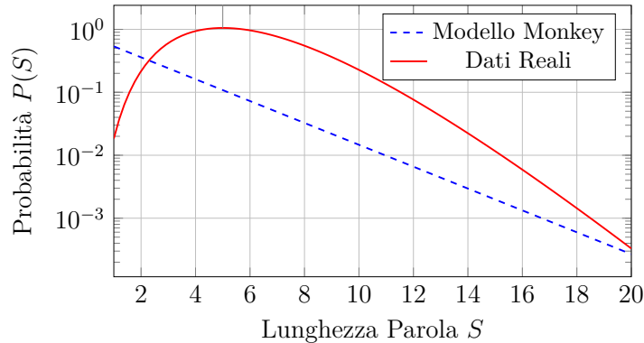
Figura 4.1: Confronto tra la previsione teorica e la distribuzione reale della lunghezza delle parole.
