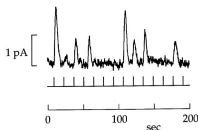
Figura 10.5: Picchi multipli in corrispondenza dell'assorbimento dei fotoni.
