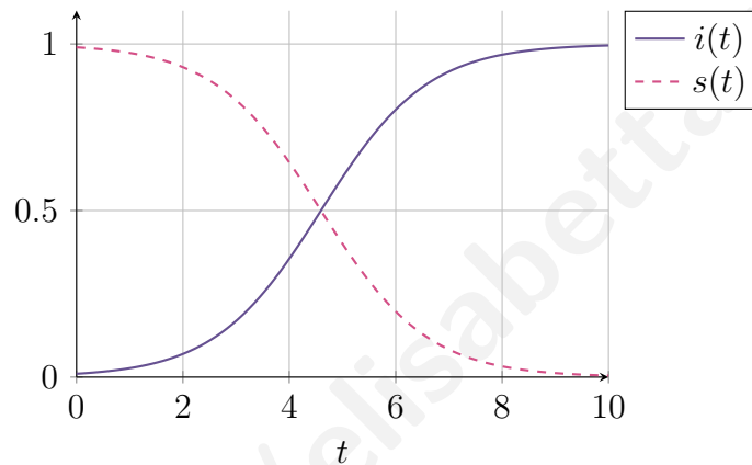
Figura 10.2: Andamento complementare di suscettibili s(t) e infetti i(t) nel modello SI.
