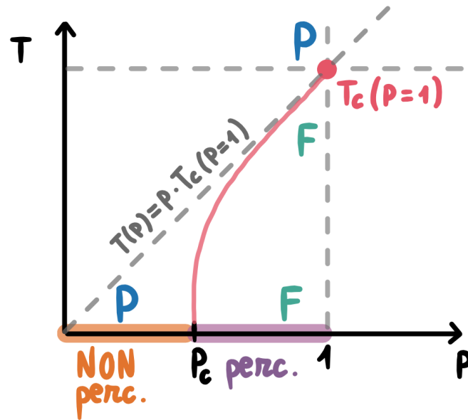
Figura 8.1: Diagramma di fase nel piano (p, T) per il modello di Ising diluito. La linea rossa è la temperatura critica T_c(p) che separa la fase P da quella F. La linea tratteggiata è la temperatura critica del modello omogeneizzato T_c^{homo}(p) , che funge da limite superiore (bound) per la temperatura critica reale.
