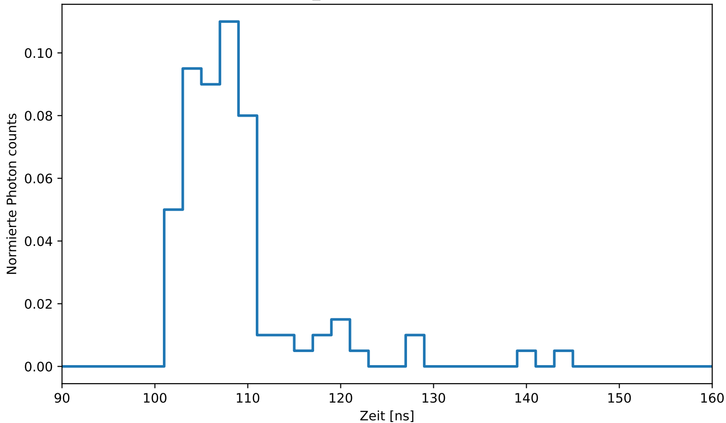
Eismodell spice_3.2.1 (1 Layer) mit theia (update)
