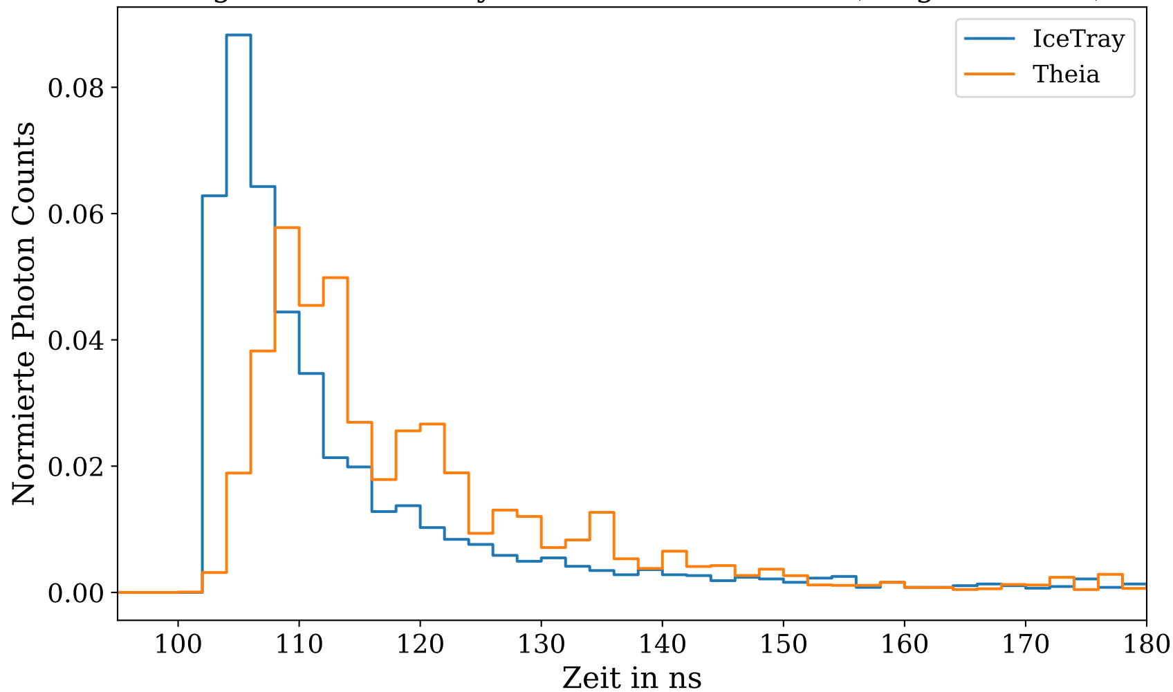
Vergleich von IceTray und Theia Simulation (Bingröße: 2 ns)
