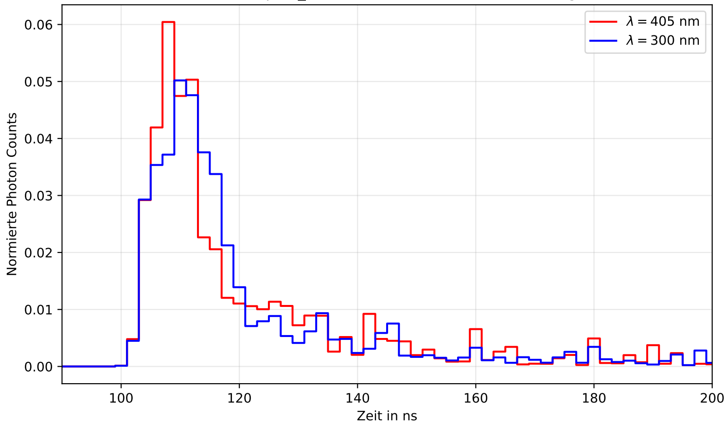
Eismodell spice_3.2.1 mit theia für zwei Wellenlängen
