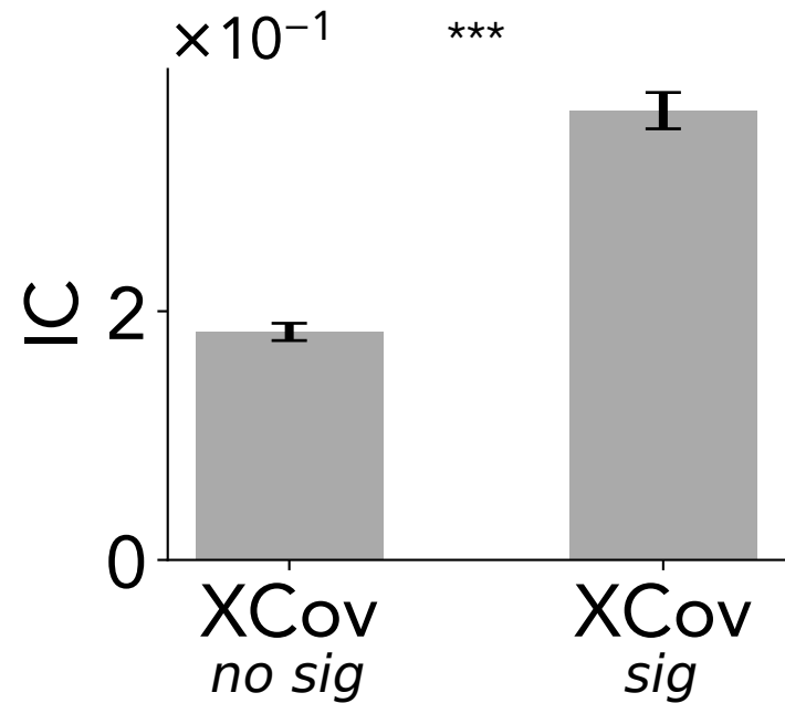
stim. chan. 594
