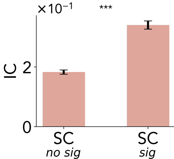
stim. chan. 594
