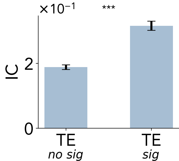
stim. chan. 594
