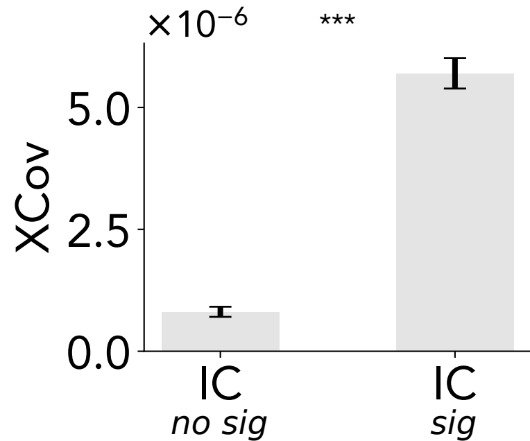
stim. chan. 594
