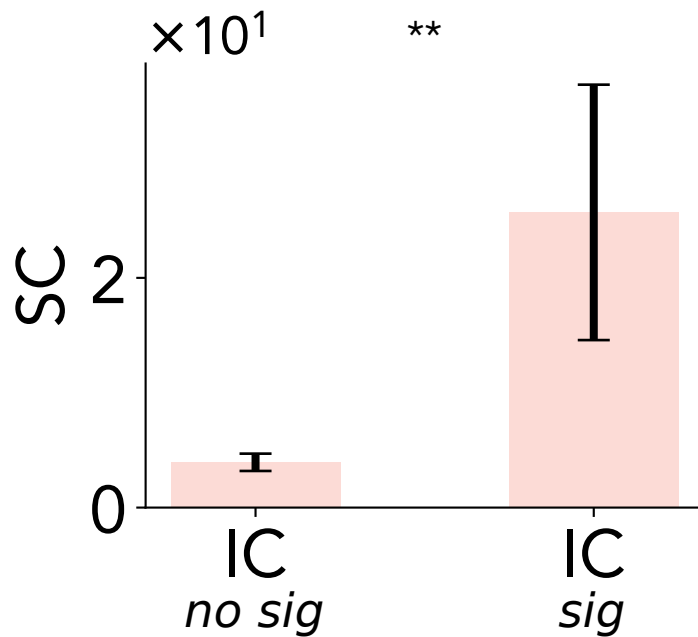
stim. chan. 813
