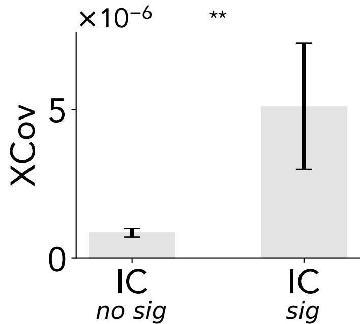
stim. chan. 813
