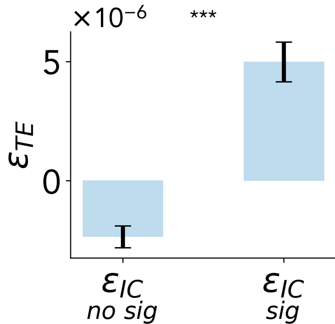
stim. chan. 142
