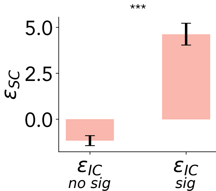
stim. chan. 142
