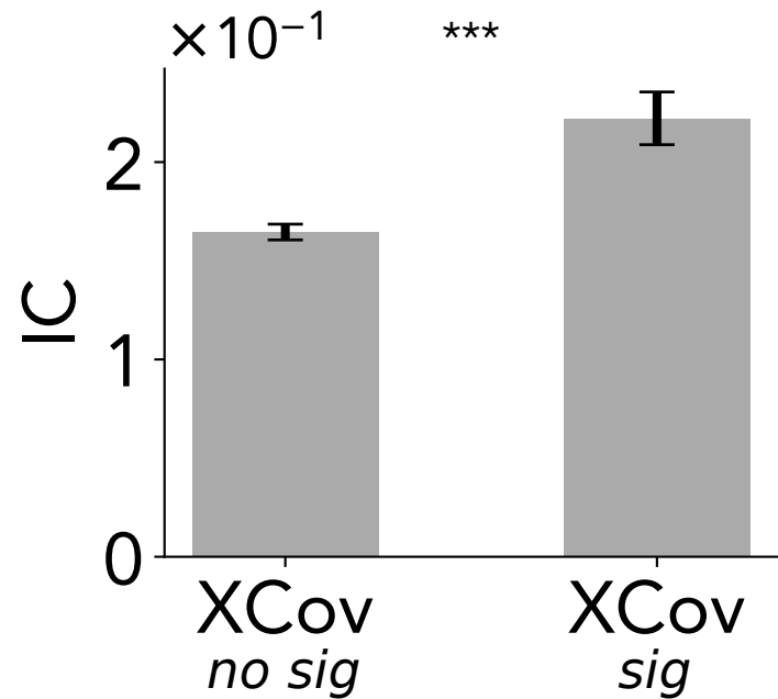
stim. chan. 627
