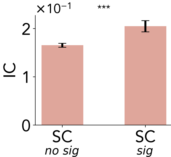
stim. chan. 627
