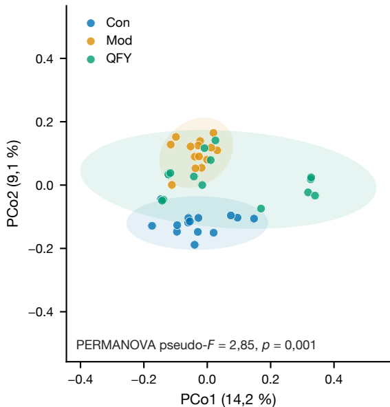
UniFrac no ponderada
