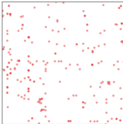
\beta_0
