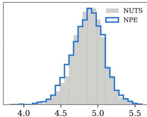
\beta_0
